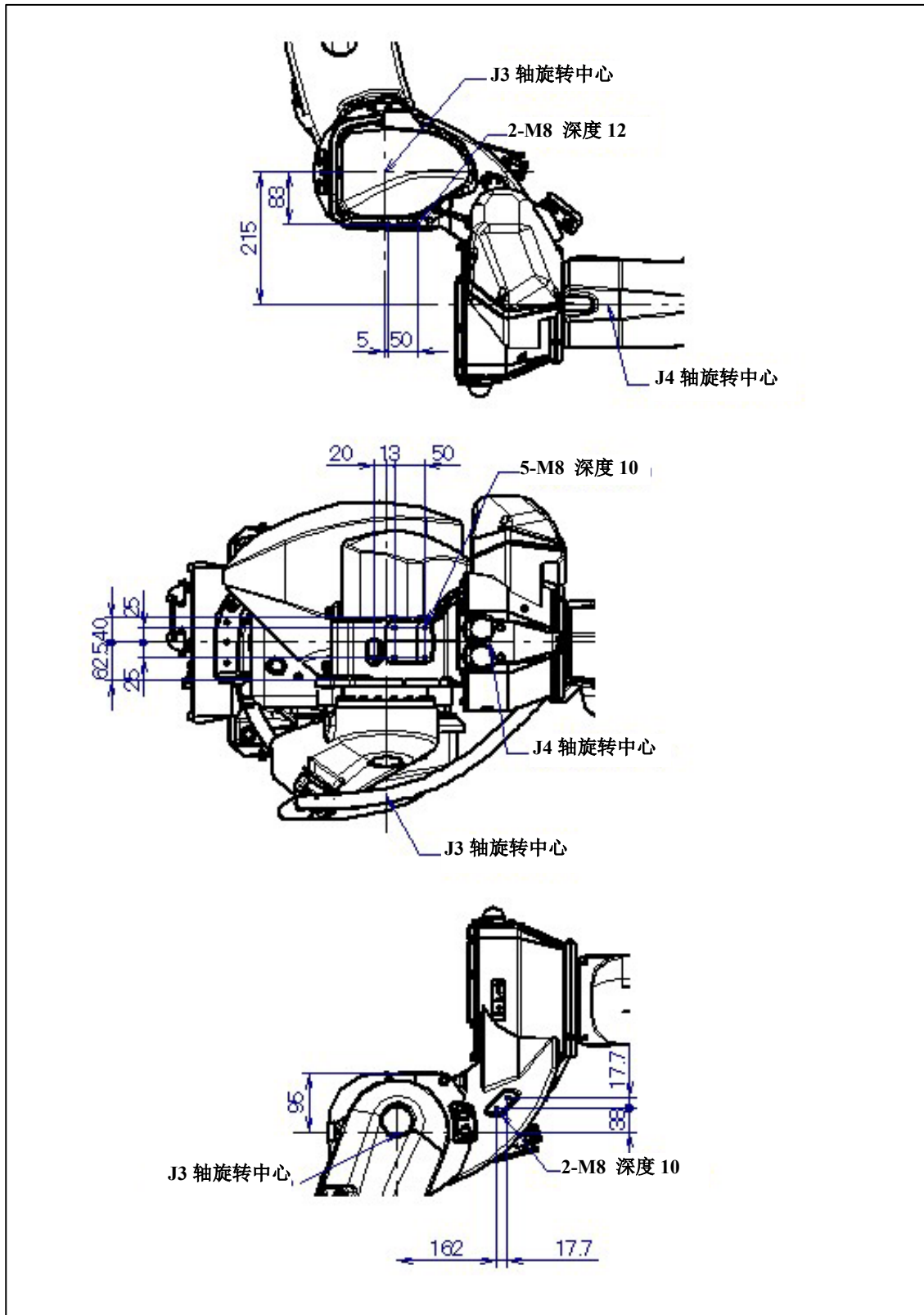
图 4.2 (b) 设备安装面尺寸 (1/2) (A+B+C 部)
