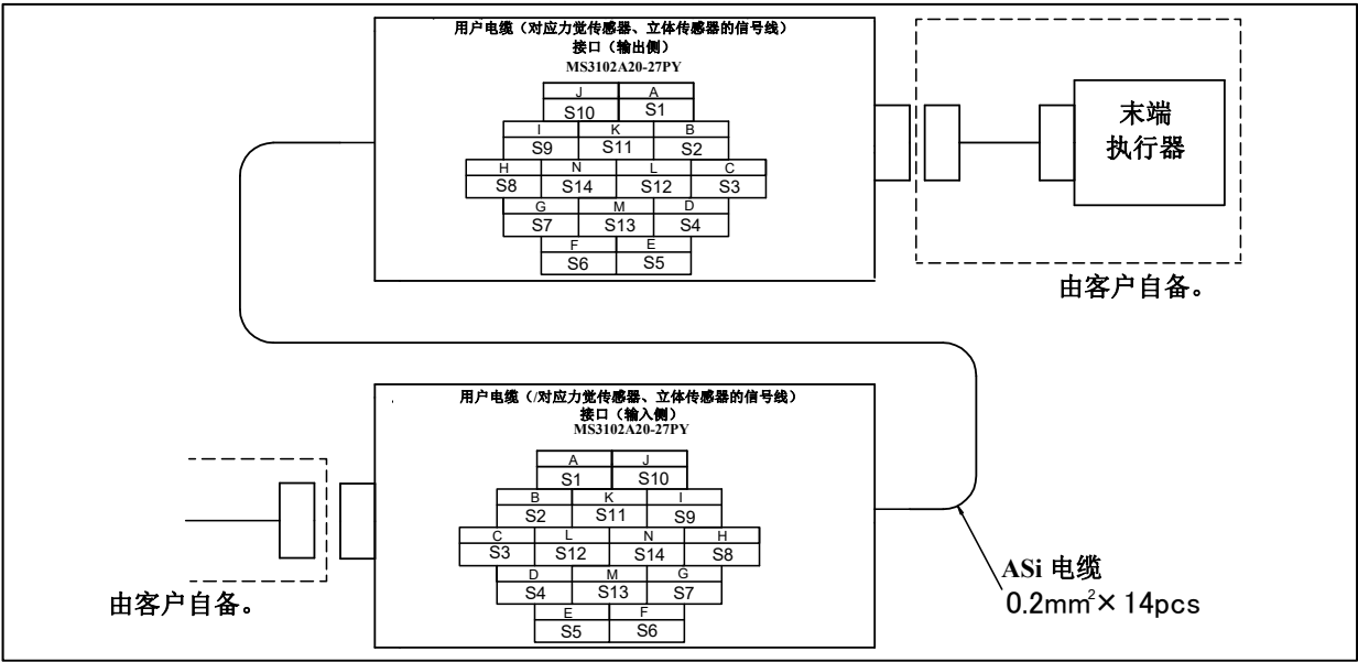
图 5.3 (e) 用户电缆（对应力觉传感器、立体传感器的信号线）(ASi)接口的插针排列（可选项）
