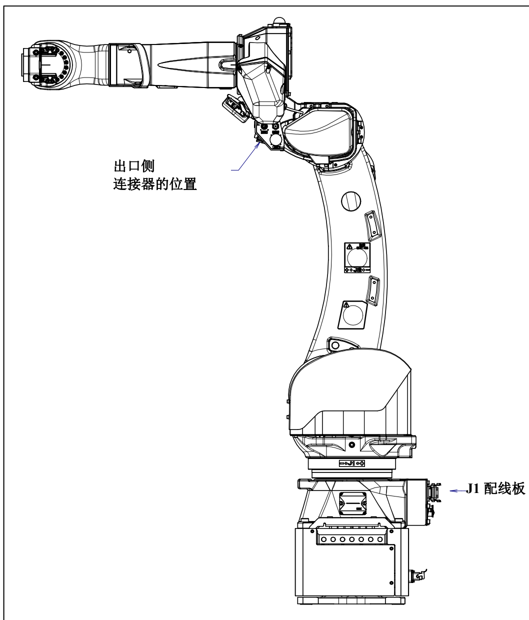
图 5.3 (a) 可选项项电缆用接口的位置（可选项项）
