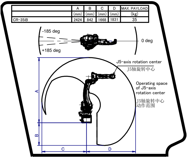
图 5.11 (f) 动作范围、可搬运重量标签
