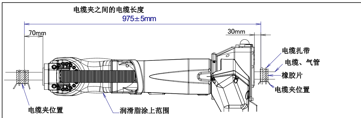
图 10.1 (a) 电缆夹之间的距离
