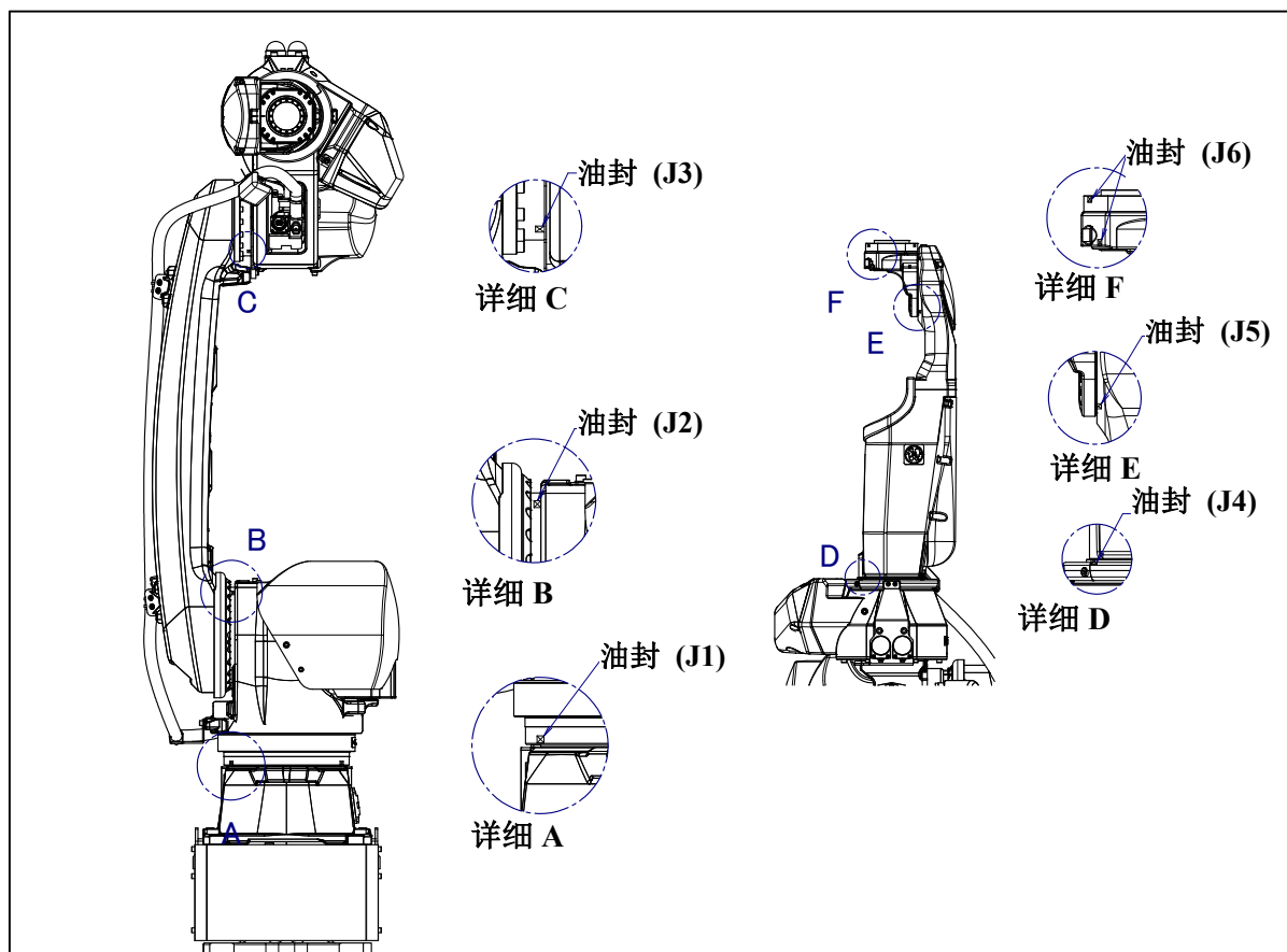
图 7.2.1 (a) 渗油的检查部位
