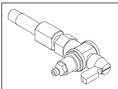
图 7.3.2.4 (c) 油注入口带有阀门 (A05B-1224-K006)
