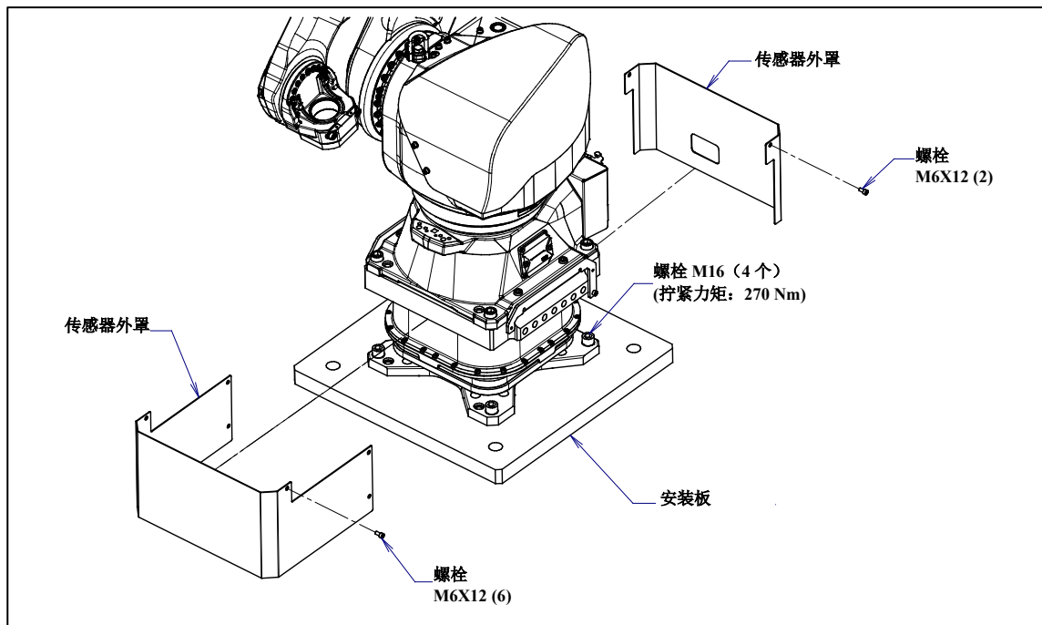
图 1.2.1 (d) 机器人的安装
