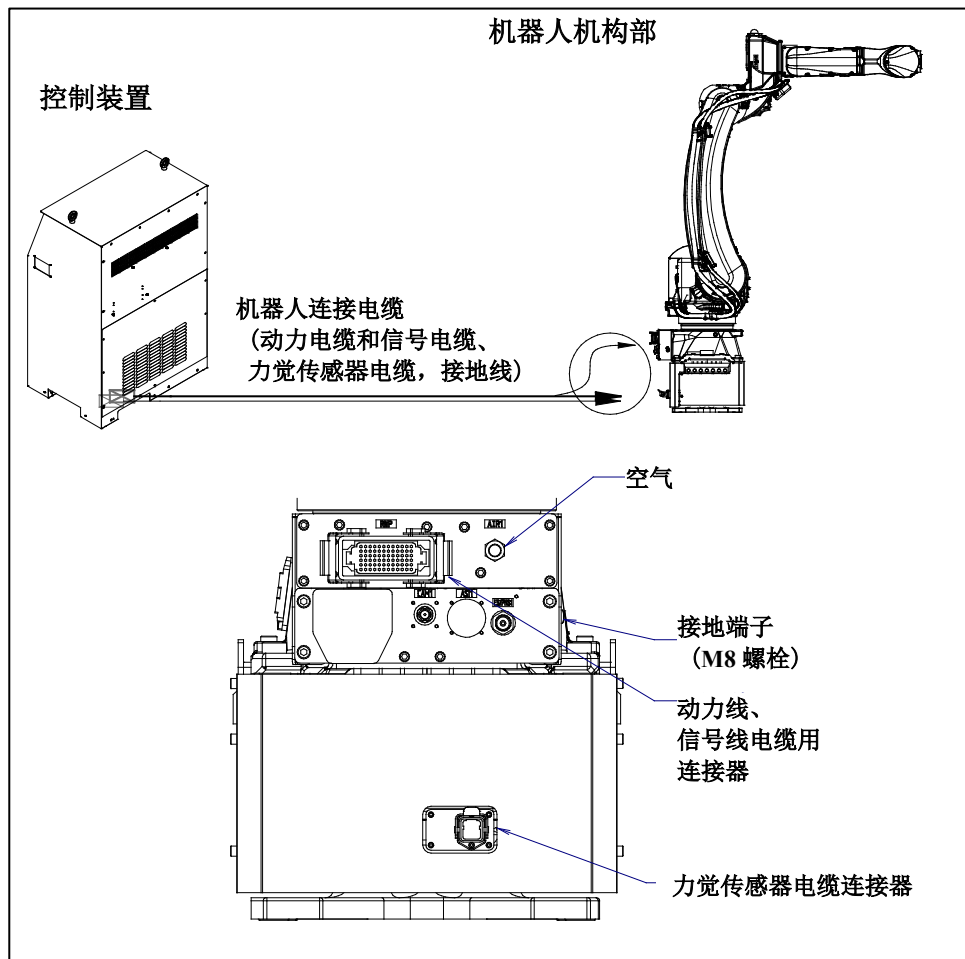
图 2 (a) 电缆连接图
