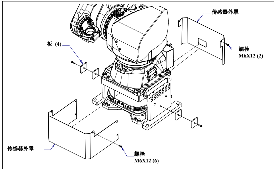
图 1.2.1 (a) 板和传感器外罩的取下
