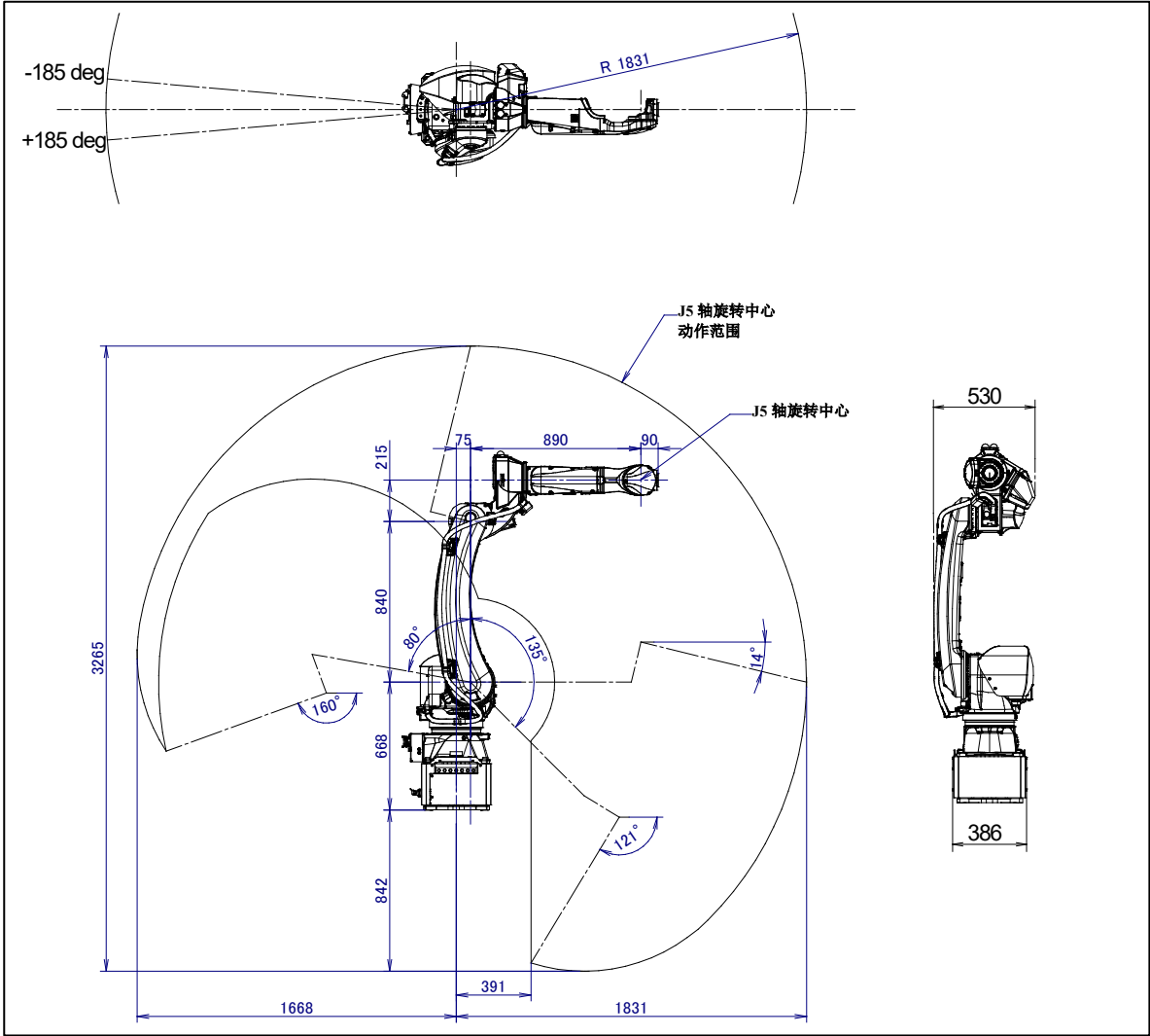
图 3.2 (a) 动作范围图
