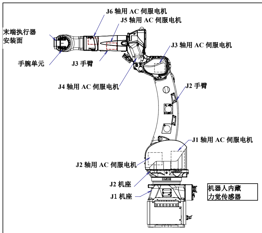
图 3.1 (a) 机构部的构成
