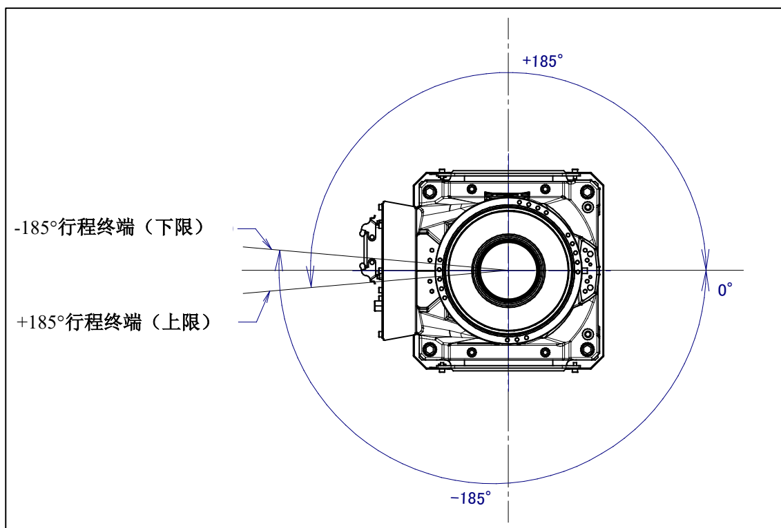
图 3.3 (a) J1 轴可动范围
