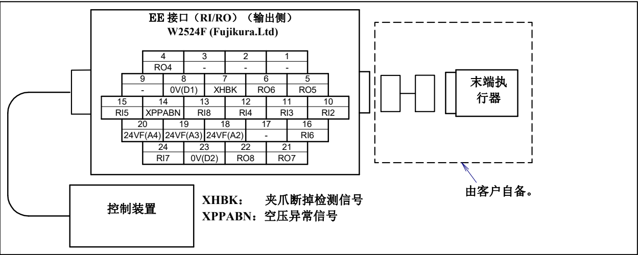
图 5.3 (d) EE 接口(RI/RO)的插针排列 RI 7 点 RO 5 点（可选项项）
