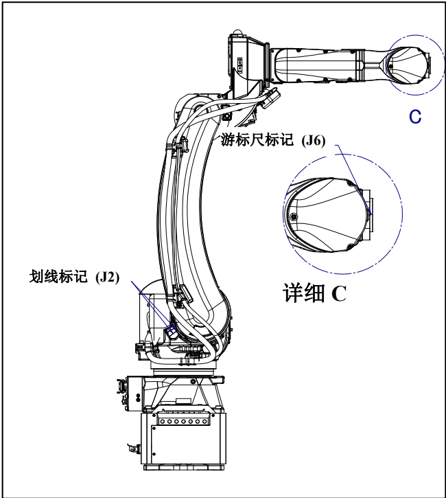
图 8.3 (b) 各轴的对合标记位置
