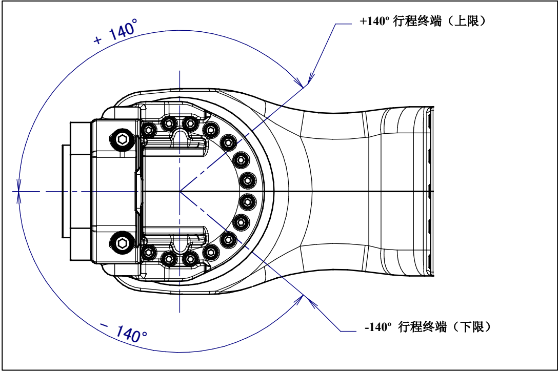
图 3.3 (e) J5 轴可动范围
