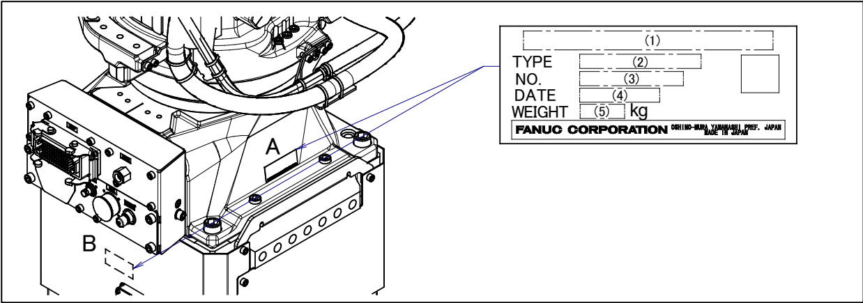
机构部规格编号标贴位置
