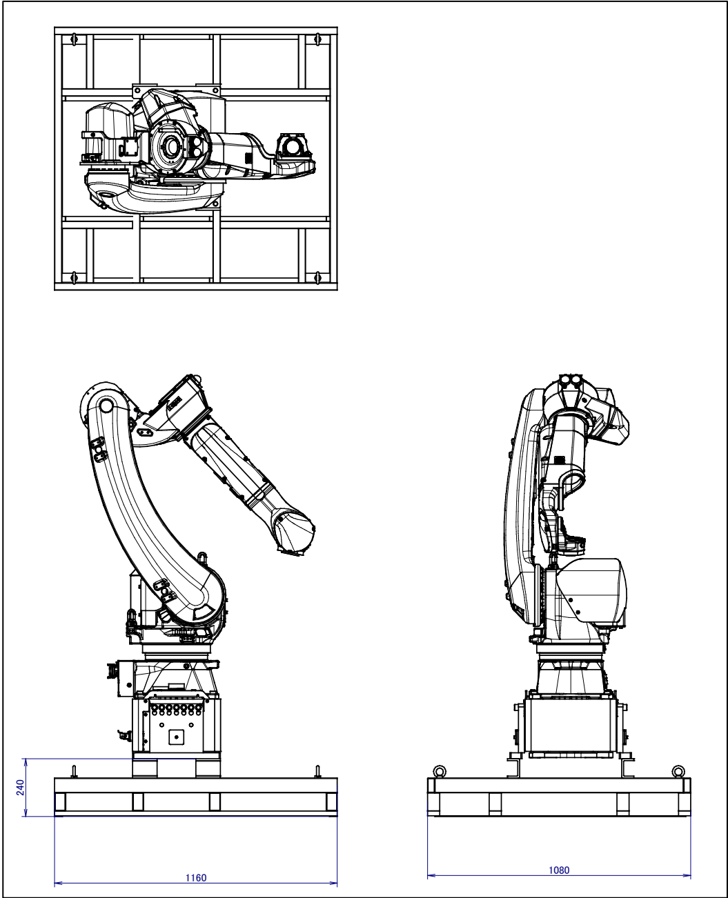
图 1.1 (f) 托盘尺寸
