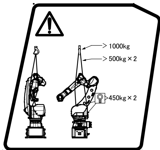
图 5.11 (b) 搬运标签 1
