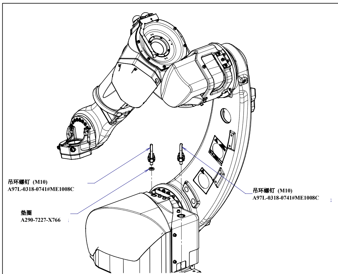
图 1.1 (b) 搬运构件的安装
