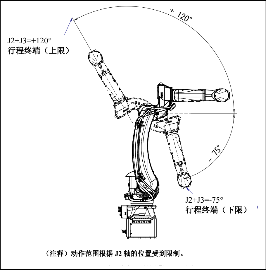
图 3.3 (c) J3 轴可动范围
