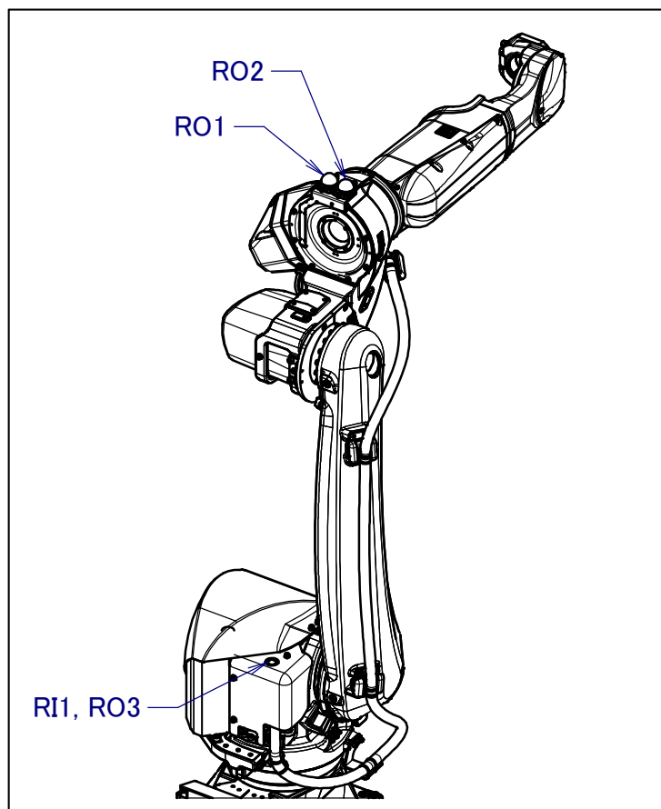
图 3.6 (d) 机器人手臂上的 LED 和按钮
