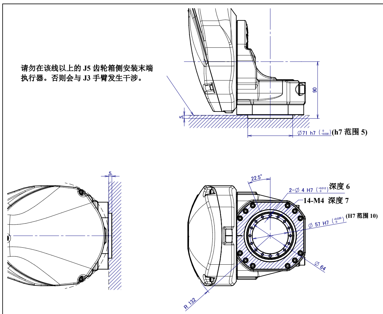
图 4.1 (a) 末端执行器安装面
