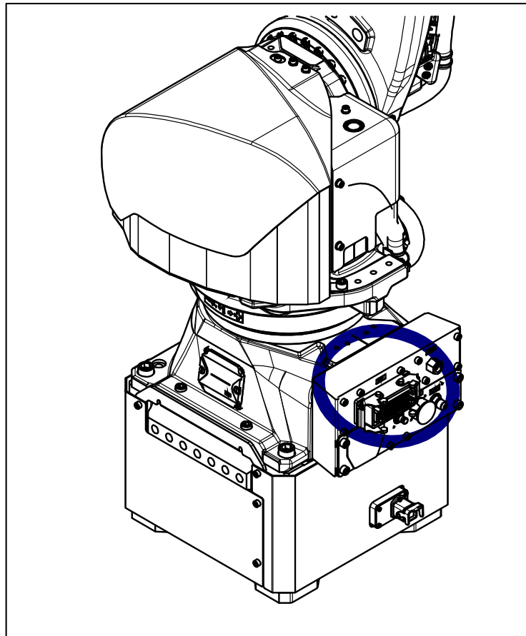
图 7.2.3 (b) 连接器的检修部位
