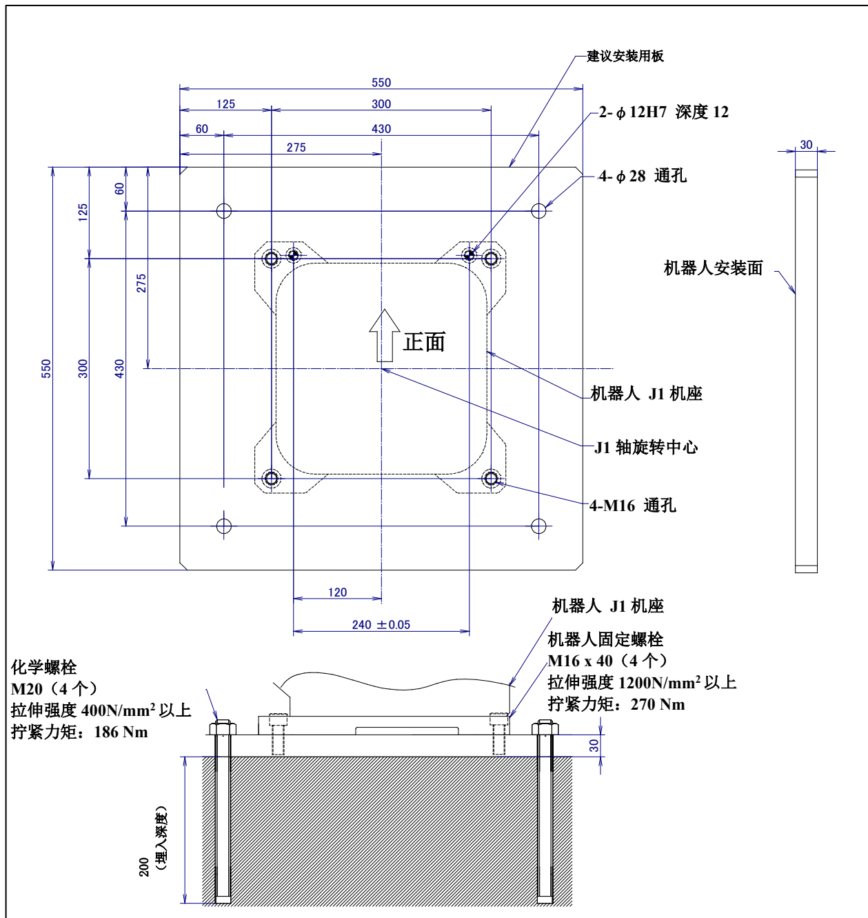
图 1.2.1 (e) 机器人安装具体例
