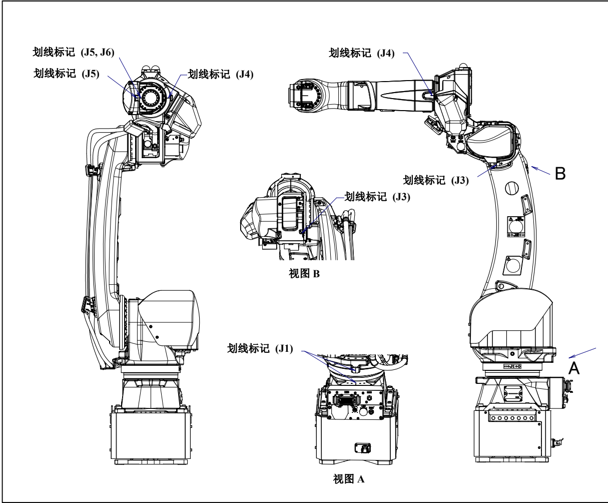
图 8.3 (a) 各轴的对合标记位置
