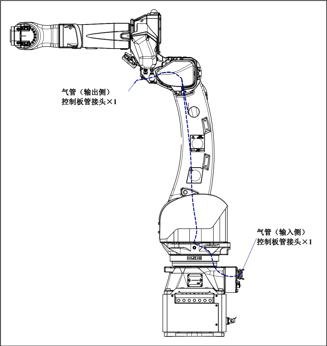
图 5.1 (a) 气压供应口（可选项）
