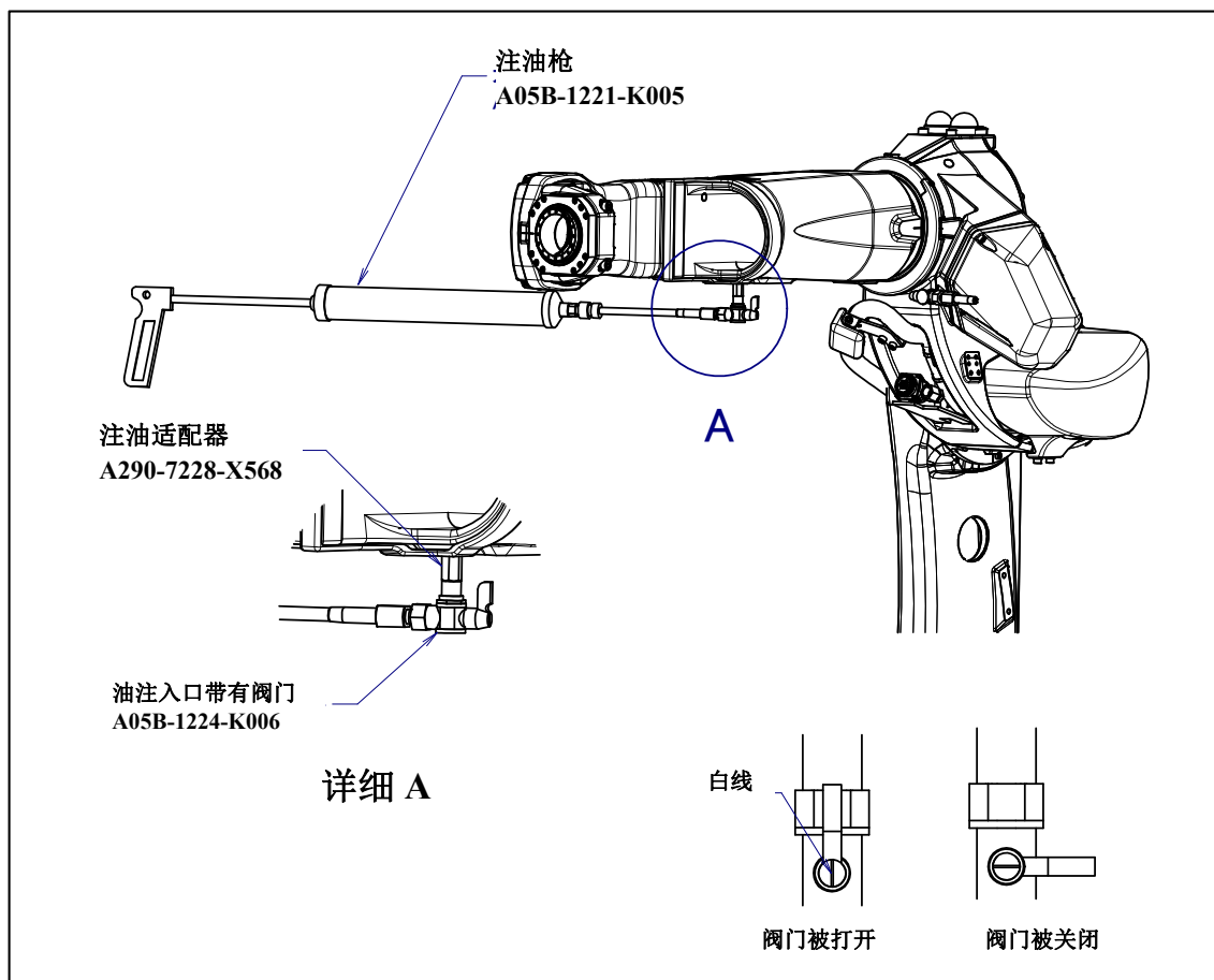
图 7.3.2.44 (b) 用注油枪供油
