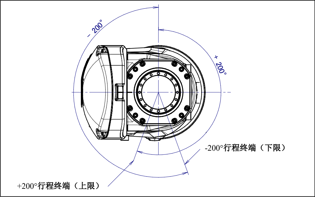
图 3.3 (d) J4 轴可动范围
