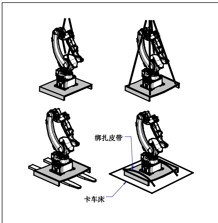
图 1.1 (e) 错误的机器人的发货形态
