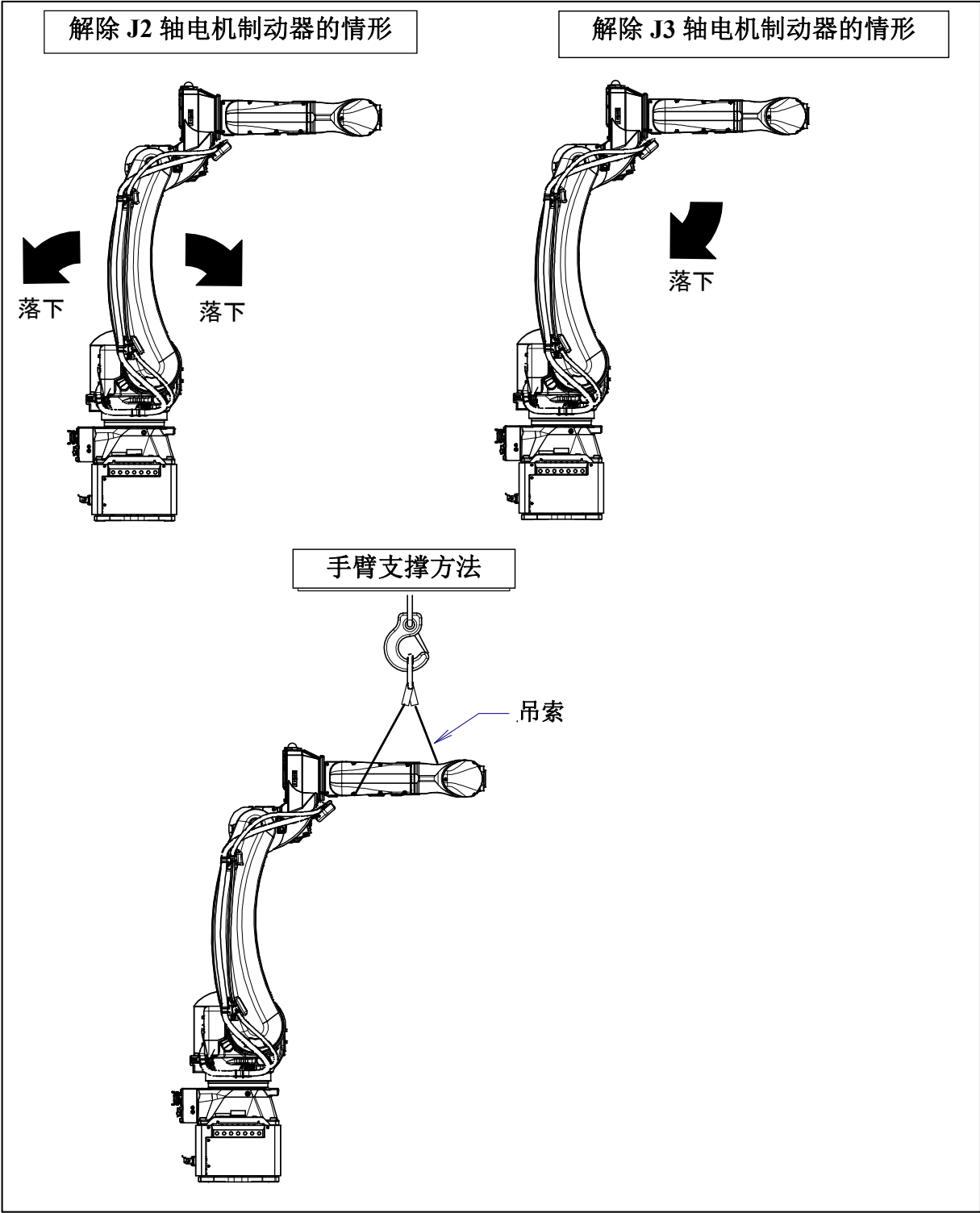
图 5.10 (a) 解除 J2、J3 轴的电机制动器造成的手臂动作和事先采取的措施例
