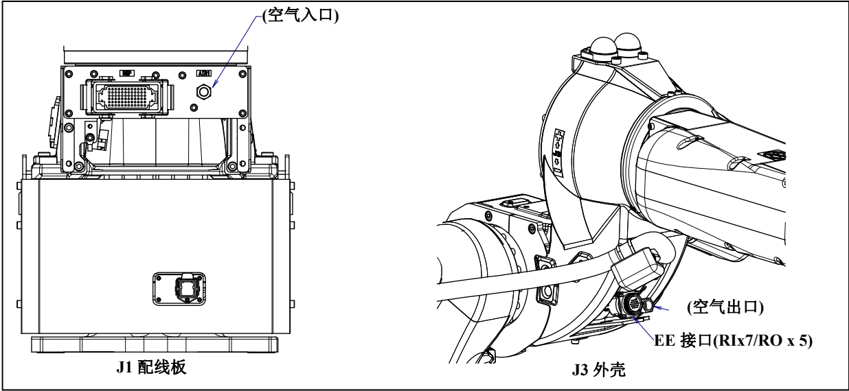
图 5.3 (b) 可选项项电缆用接口（指定 A05B-1228-H621#12 时）
