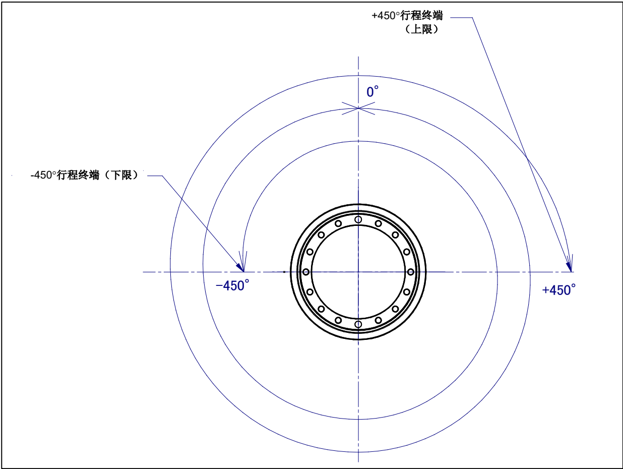
图 3.3 (f) J6 轴可动范围
