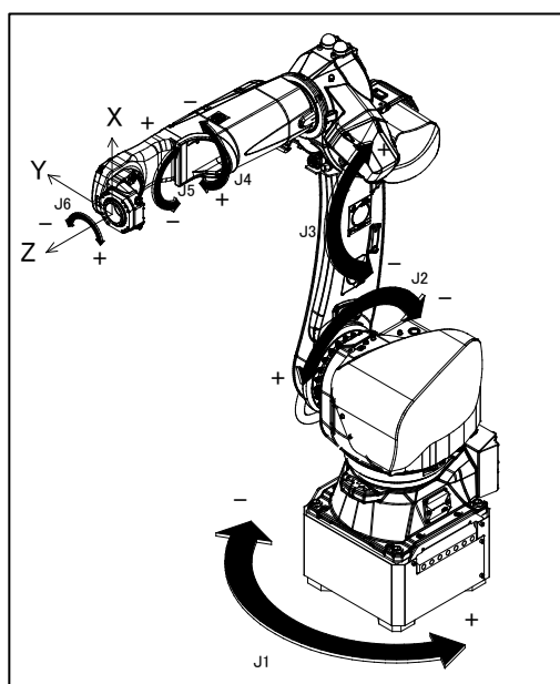
图 3.1 (b) 各轴坐标和机械接口坐标
