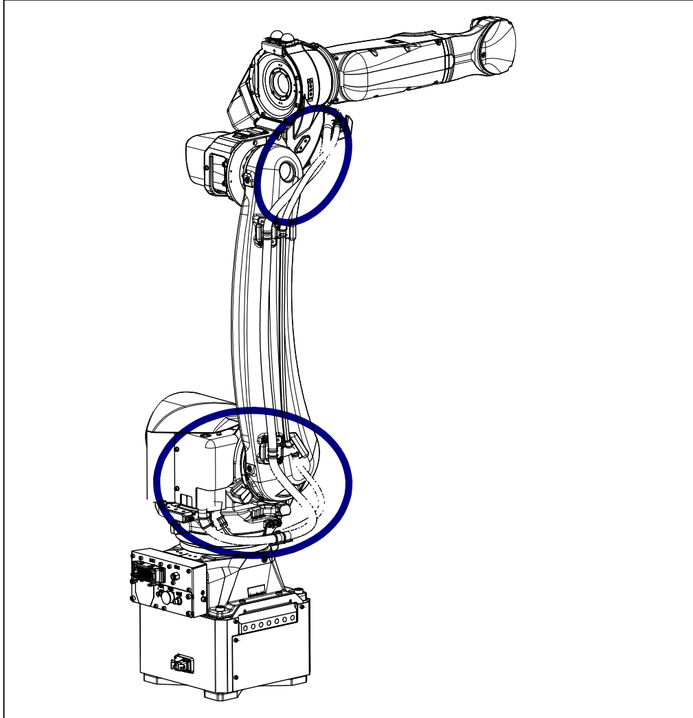
图 7.2.3 (a) 机构部内电缆的检修部位
