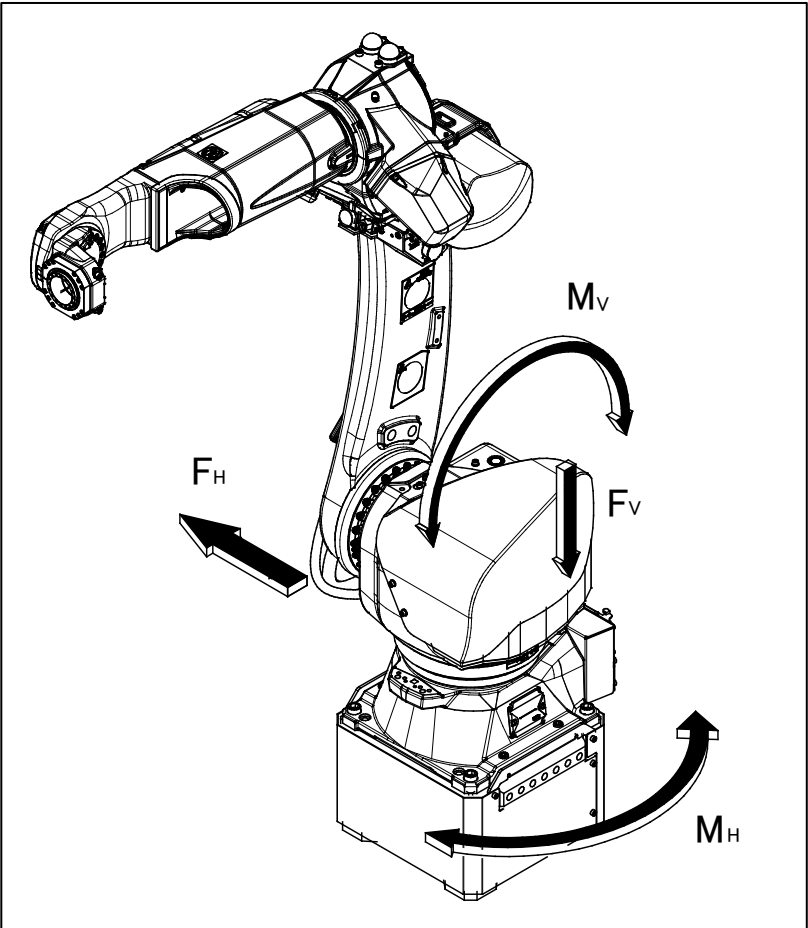
图 1.2.1 (g) 作用于机器人机座的力和力矩
