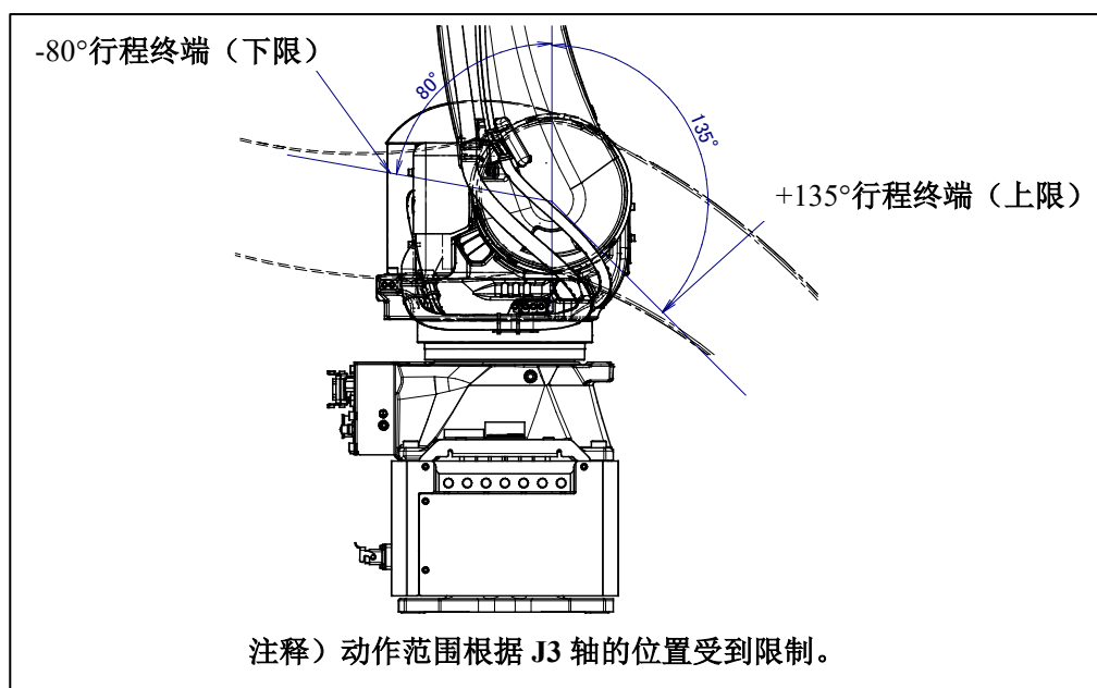
图 3.3 (b) J2 轴可动范围
