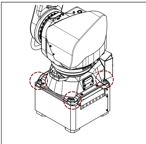
图 7.1.2 (a)检查部位
