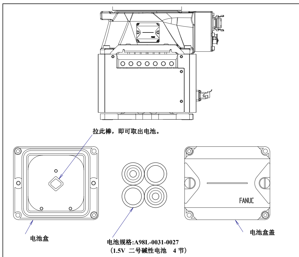
图 7.3.1 (a) 电池的更换
