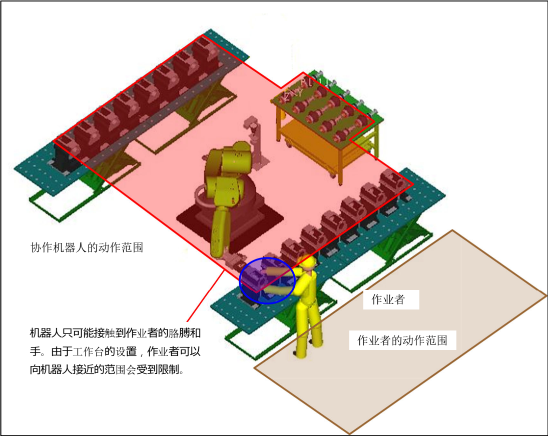
图 3.6 (b) 系统的例
