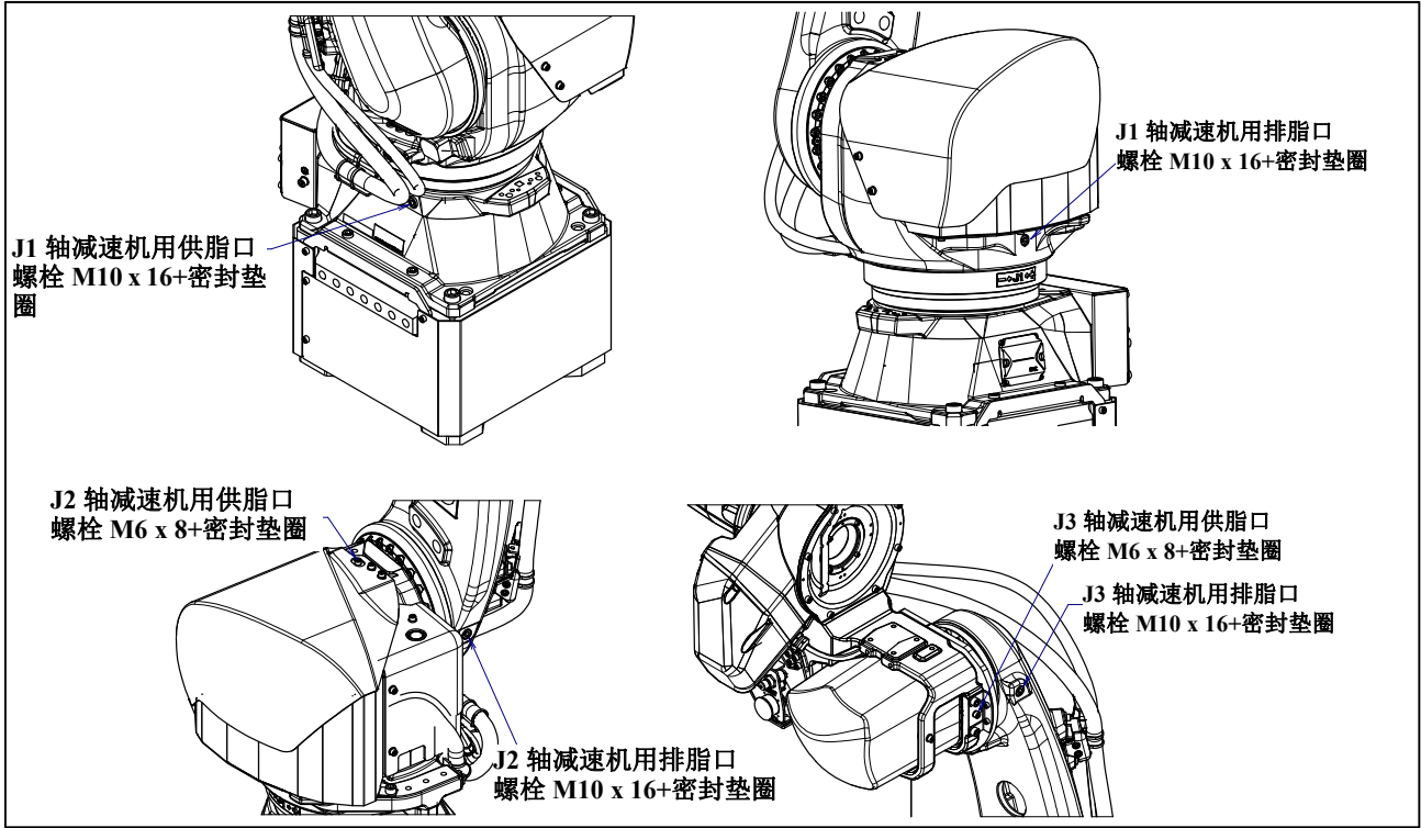
图 7.3.2.1 (a) J1,J2, J3 轴的供脂部位
