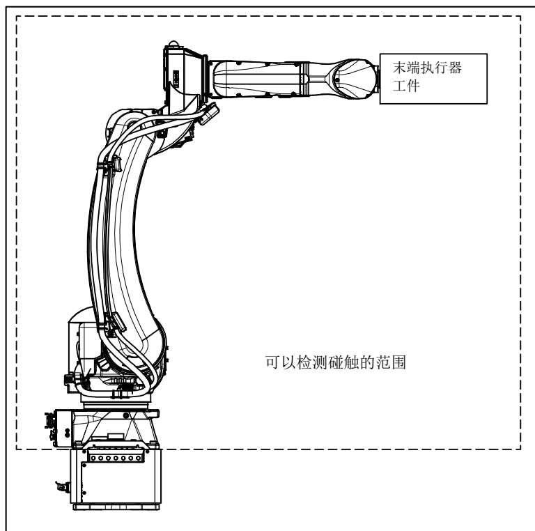
图 3.6 (a) 碰触停止的部分
