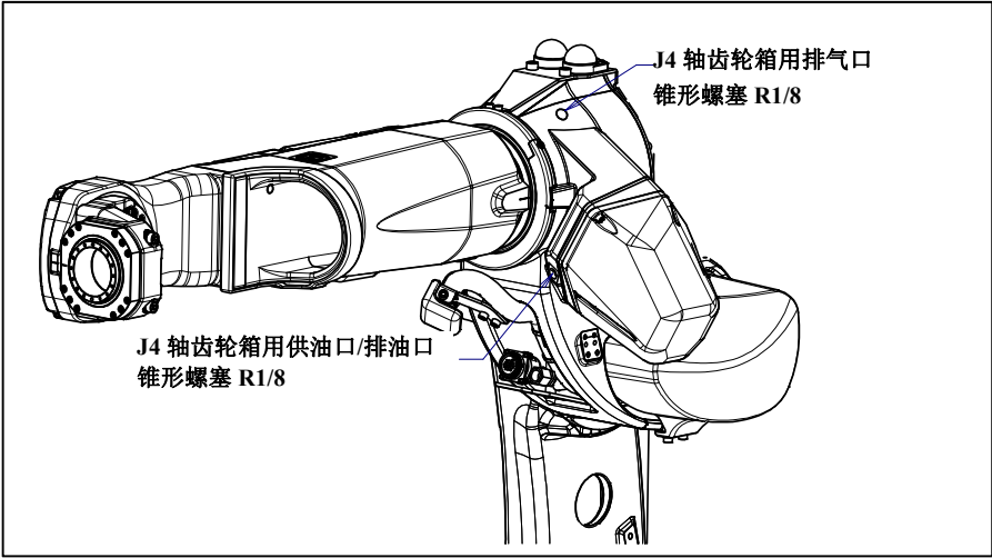
图 7.3.2.3 (a) J4 轴齿轮箱的供脂部位
