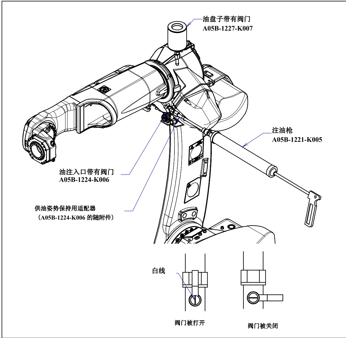
图 7.3.2.5 (b) 用注油枪供油 (J4 轴齿轮箱的供油)
