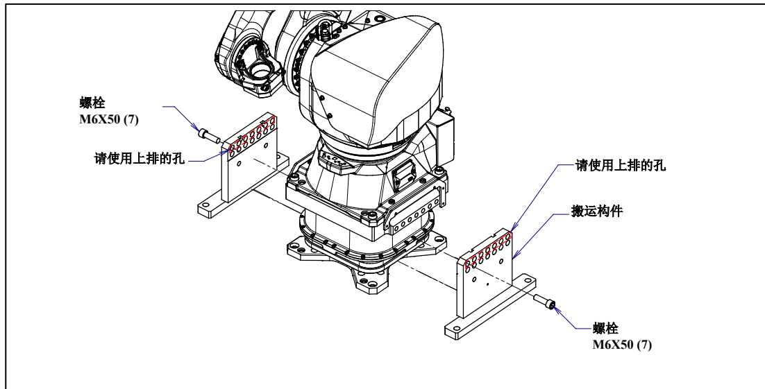
图 1.2.1 (c) 搬运构件的取下
