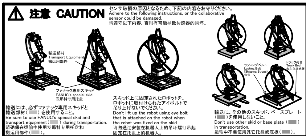
图 5.11 (d) 搬运标签 3
