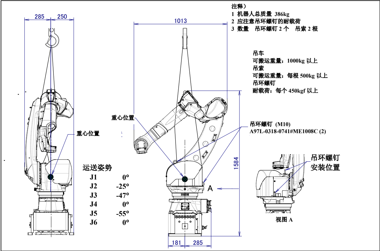
图 1.1 (c) 用吊车搬运
