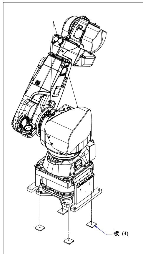
图 1.2.1 (b) 板的插入
