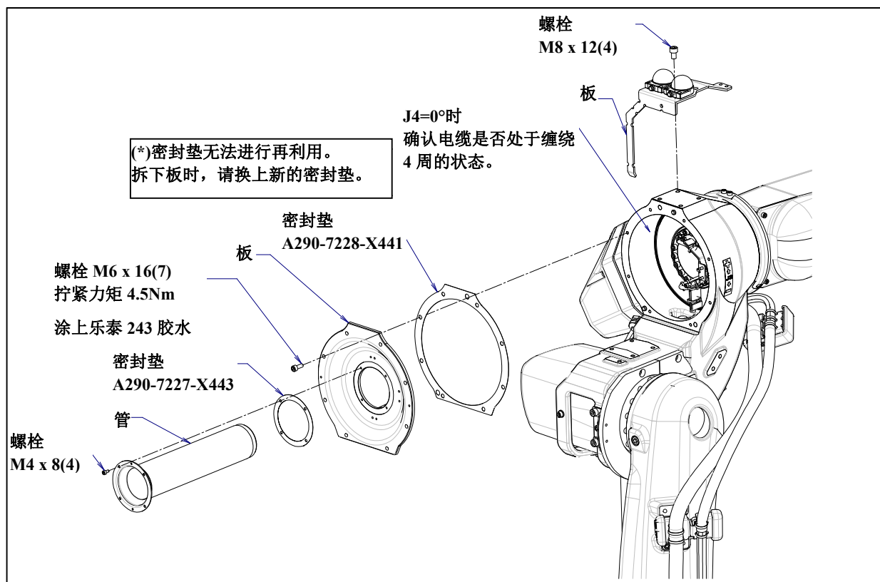
图 8.1 (b) 确认电缆的状态 (J4 轴)
