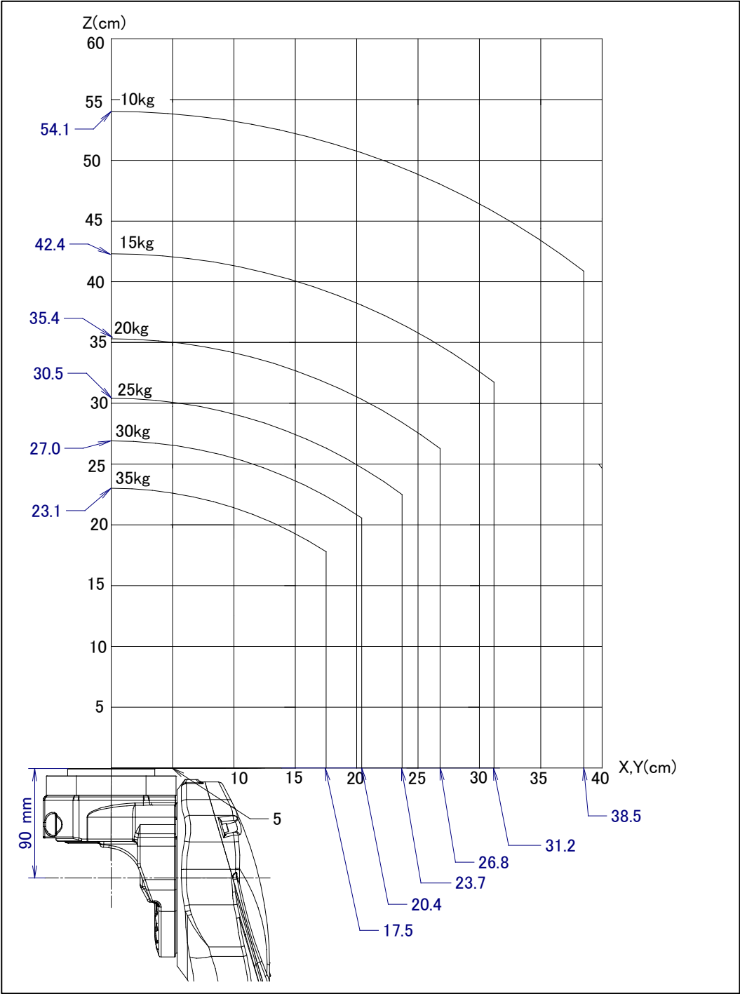
图 3.4 (a) 手腕部允许负载线图
