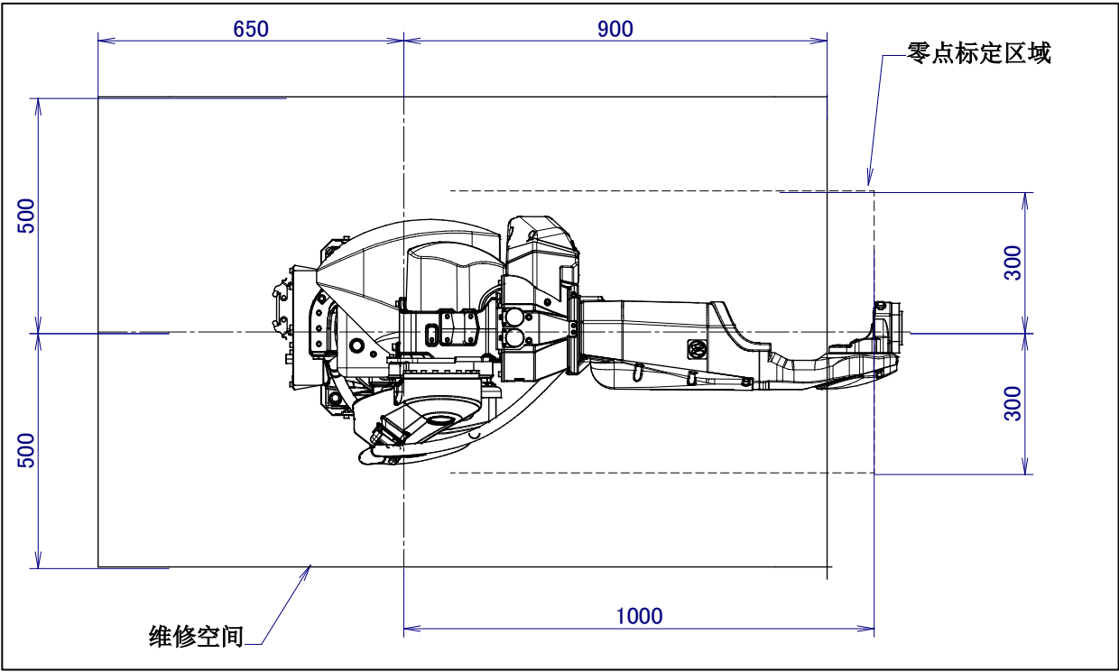
图 1.3 (a) 维修空间的布局图
