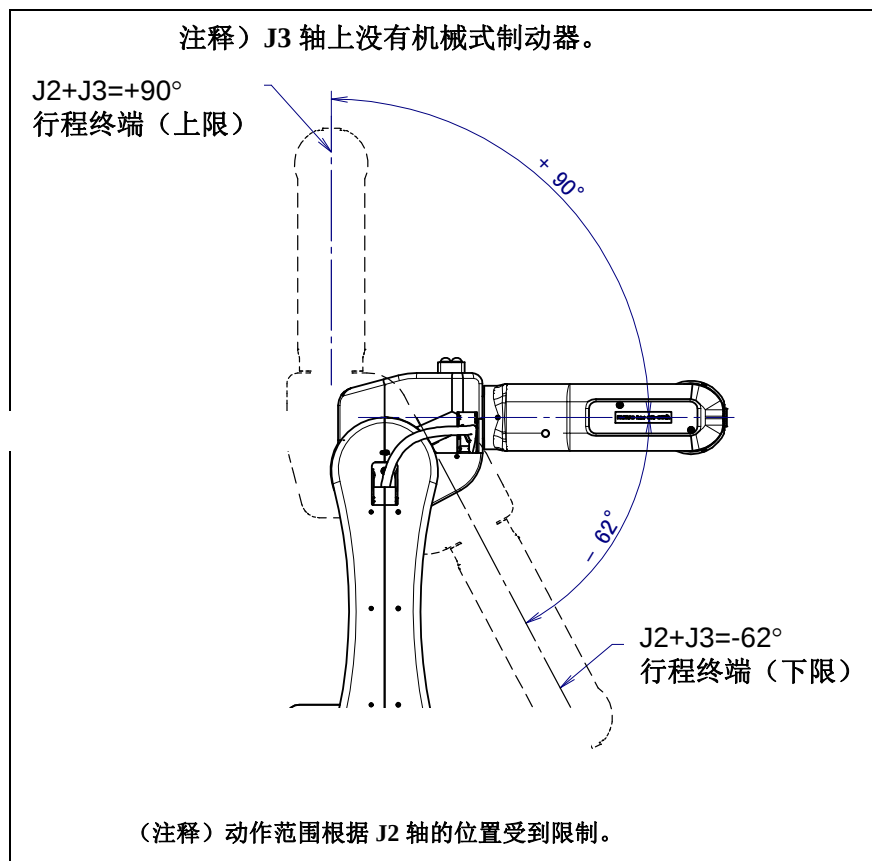
图 3.3 (e) J3 轴可动范围
