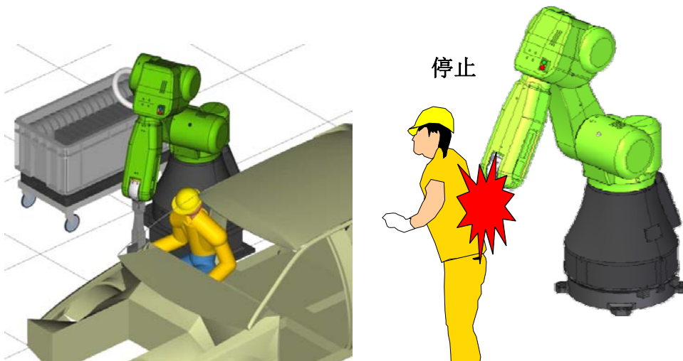
系统例子：向人提供部件
