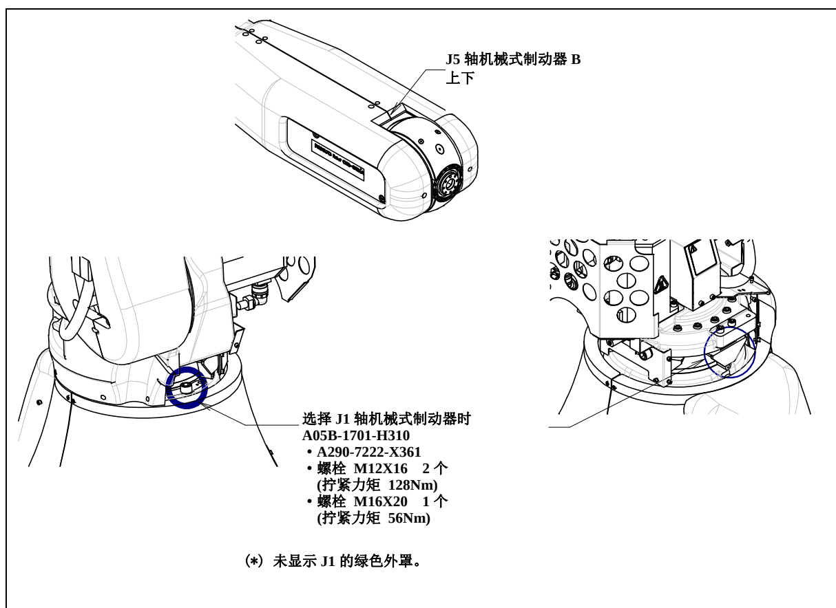
图 3.3 (a) 机械式制动器的位置
