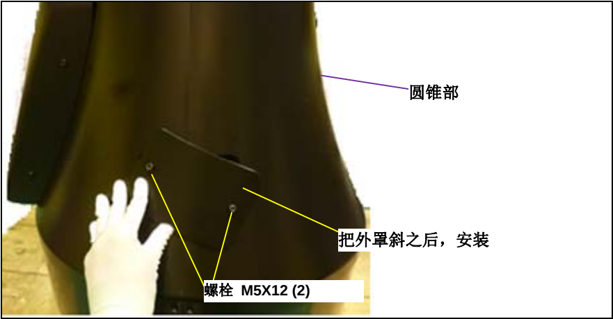
图 1.2 (g) 外罩安装方法
