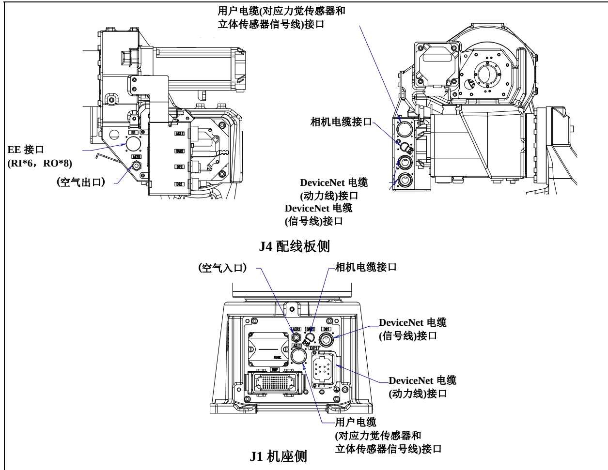
图 5.3 (e) 可选项项电缆用接口(指定 A05B-1701-H202 时)
