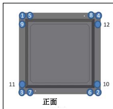
图 1.2 (e) 机器人固定螺栓的拧紧顺序
