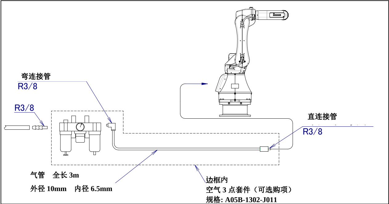
图 5.2 (a) 空气配管（可选项项）
