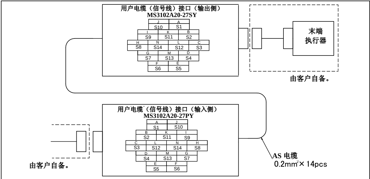
图 5.3 (g) 用户电缆(信号线)(AS)接口的插针排列(可选项)
