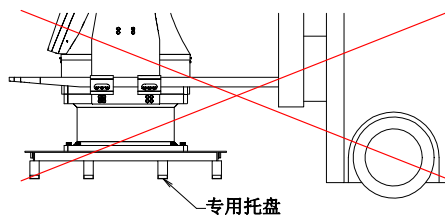
图 1.1 (c) 用叉车起重机搬运
