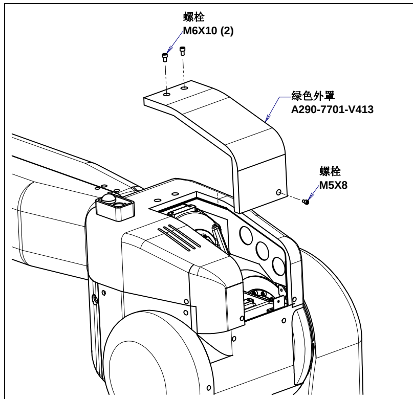
图 5.3 (d) J3 外罩的拆除 (2/2)
