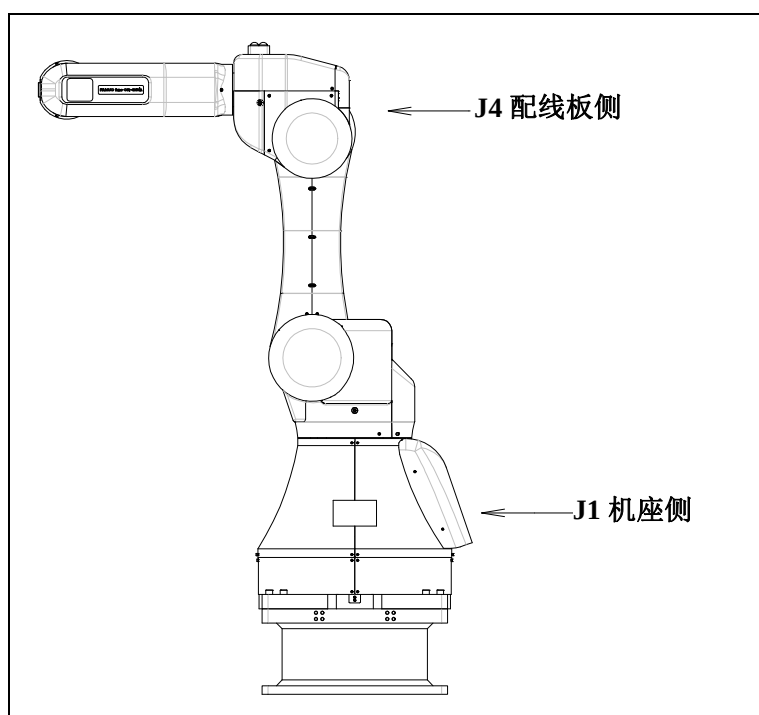
图 5.3 (a) 可选项项电缆用接口的位置(可选项项)
