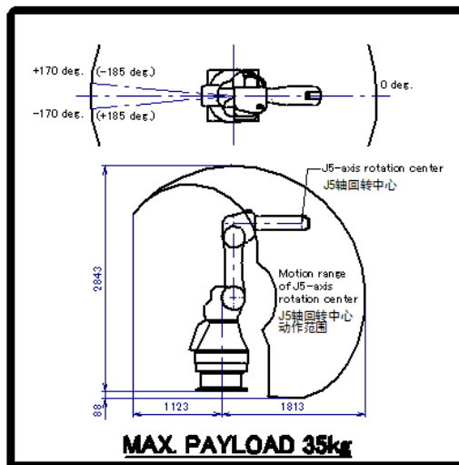
图 5.11 (g) 动作范围、可搬运重量标签
