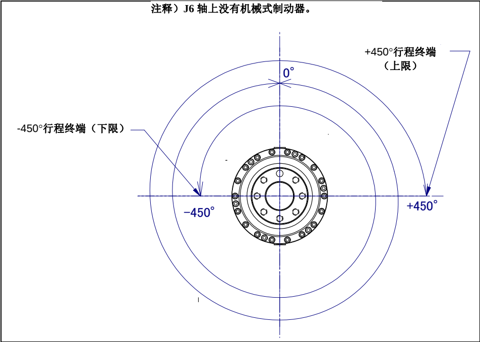
图 3.3 (h) J6 轴可动范围
