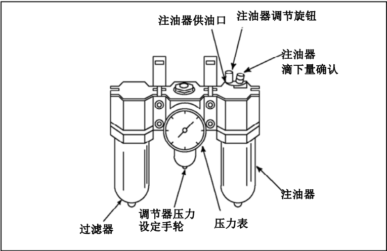
图 7.2.2 (a) 空气 3 点套件(选项)
