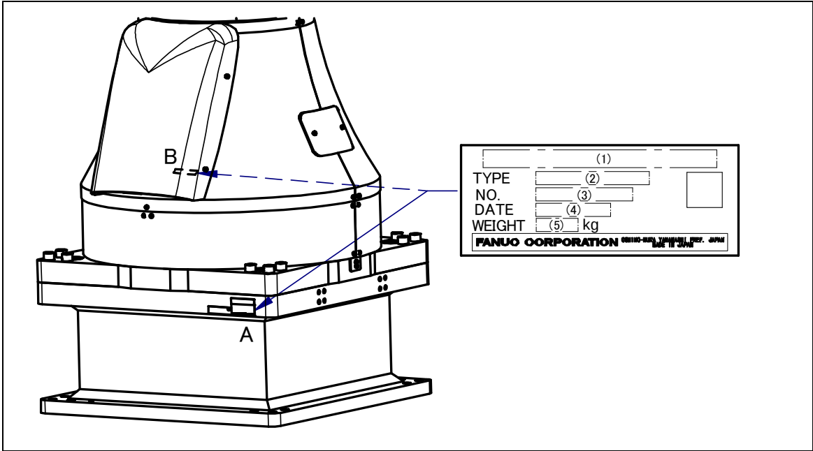
机构部规格编号标贴位置
