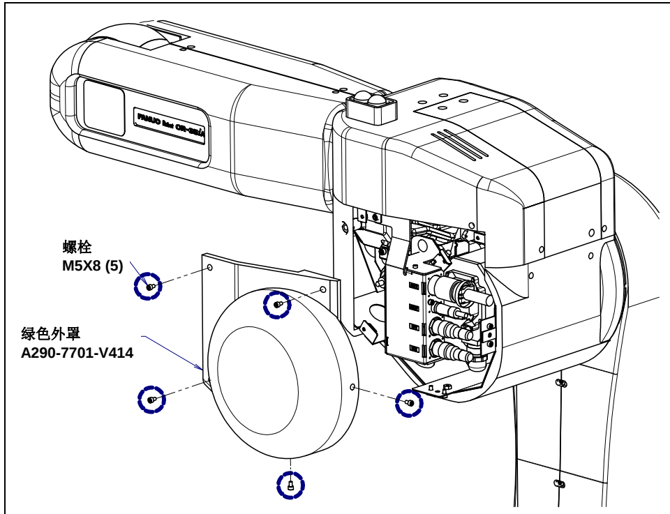
图 5.3 (c) J3 外罩的拆除 (1/2)
