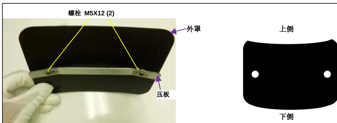
图 1.2 (f) 外罩
