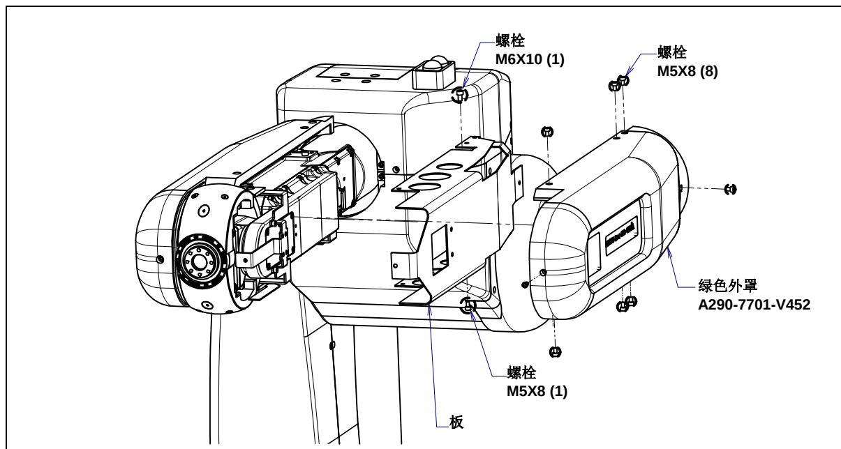
图 4.2 (d) 外罩的拆除
