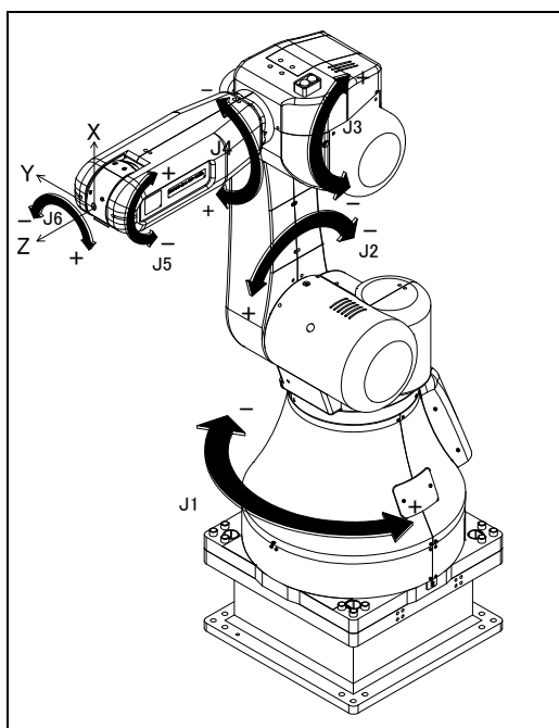
图 3.1 (b) 各轴坐标和机械接口坐标
