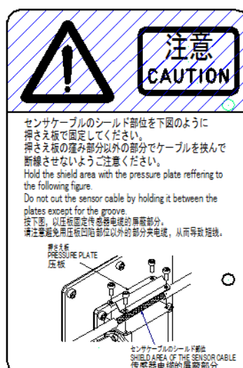
图 5.11 (f) 连接注意标签
