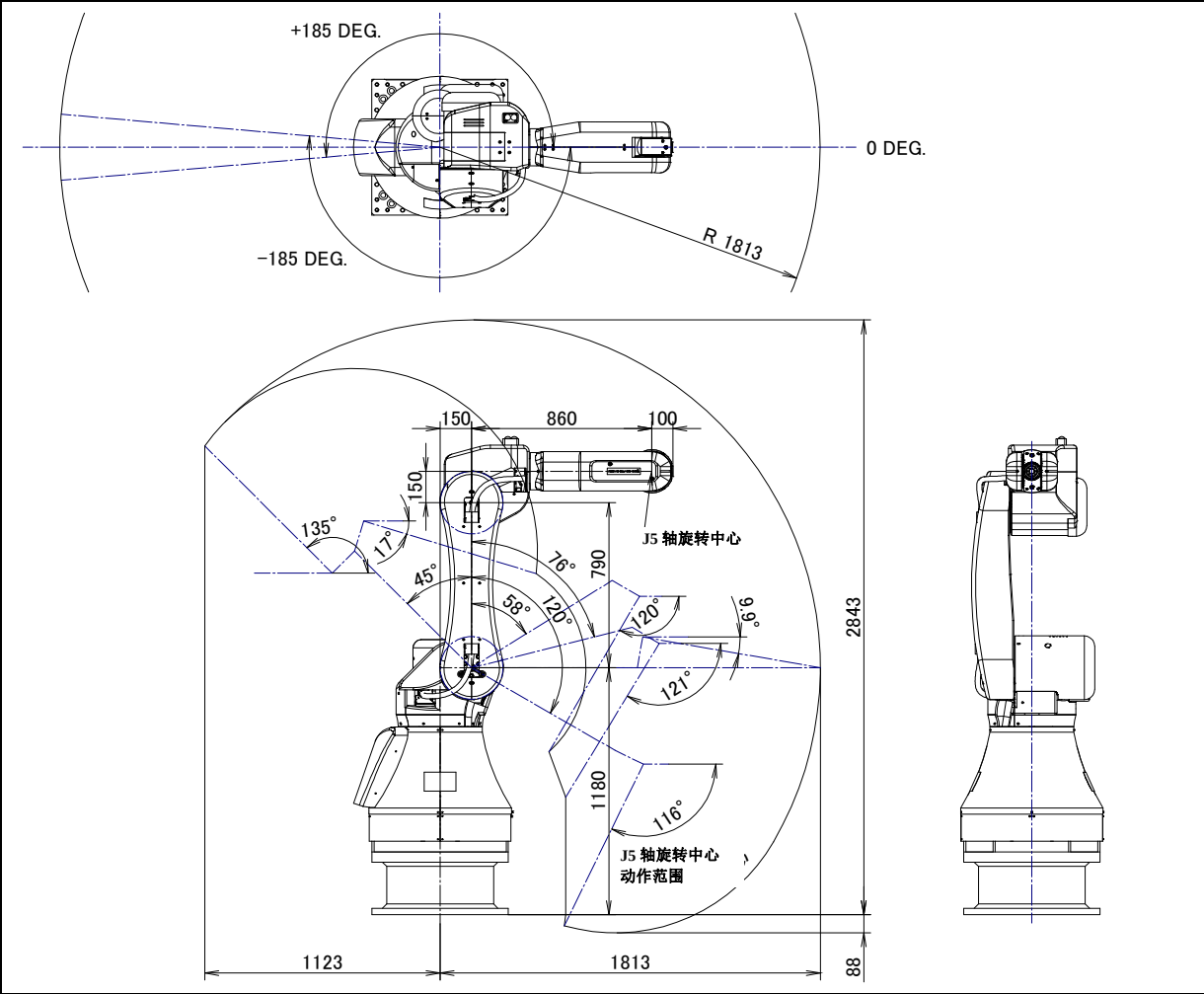
图 3.2 动作范围图
