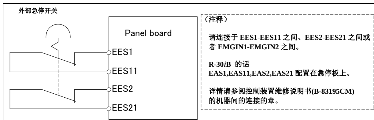
图 2.4.4 外部急停按钮的连接图
