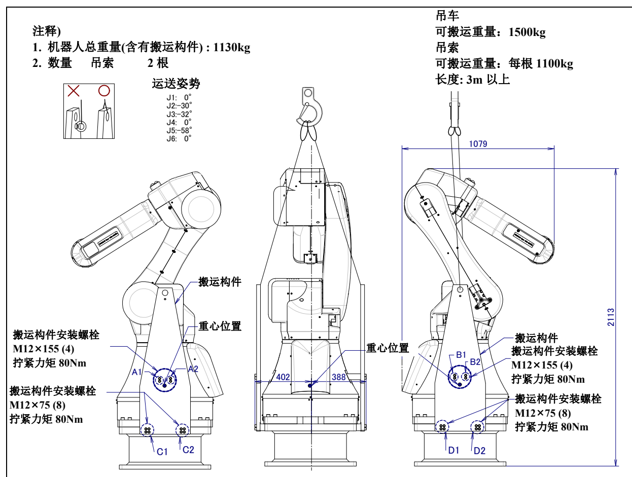
图 1.1 (b) 用吊车搬运
