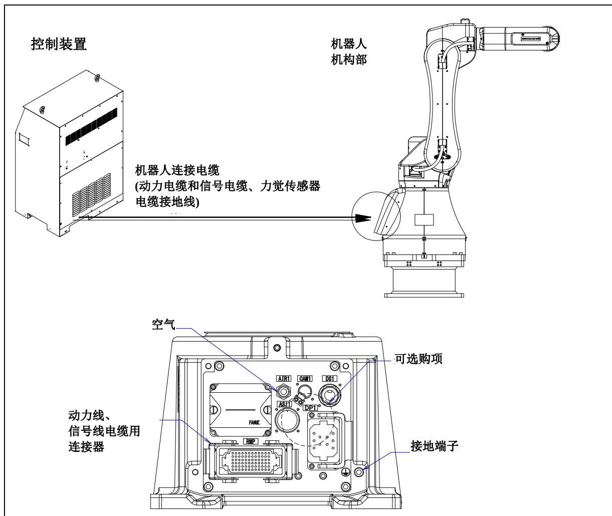
图 2.1 (d) 电缆连接图 (4/4)
