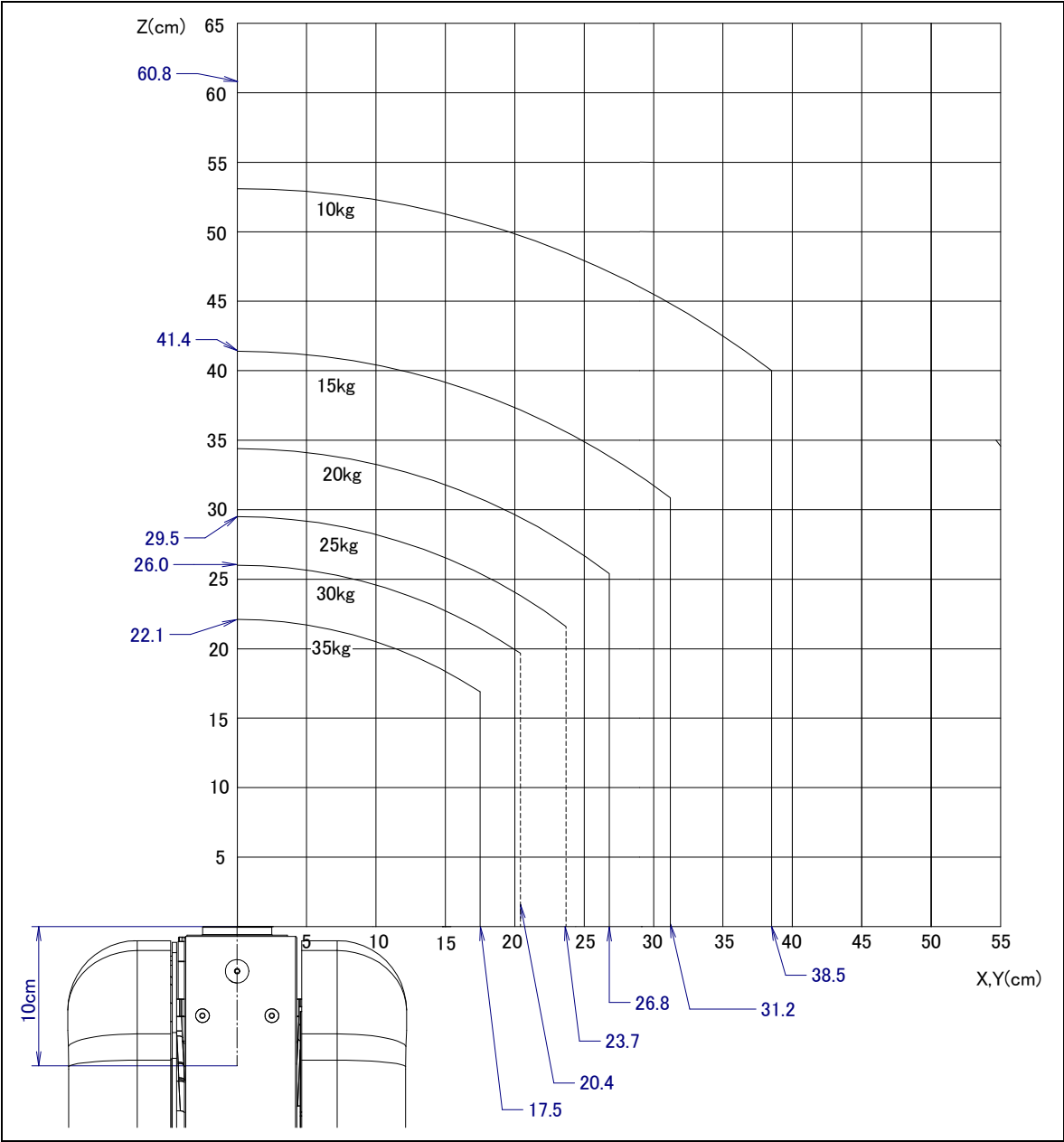
图 3.4 手腕部允许负载线图
