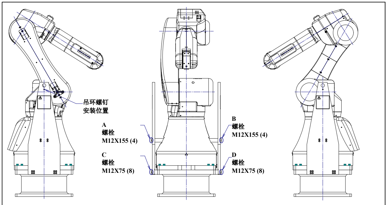
图 1.2 (c) 搬运构件的拆除
