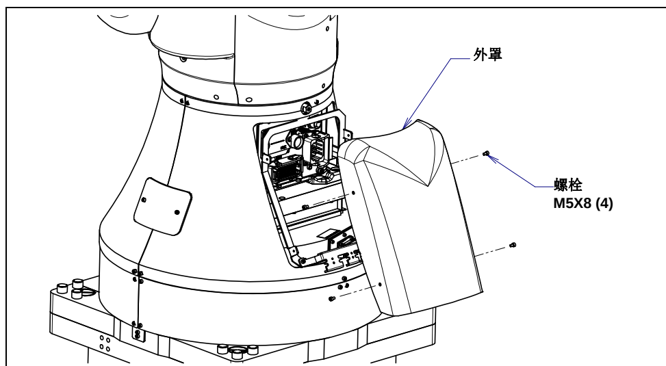
图 5.3 (b) J1 外罩的拆除
