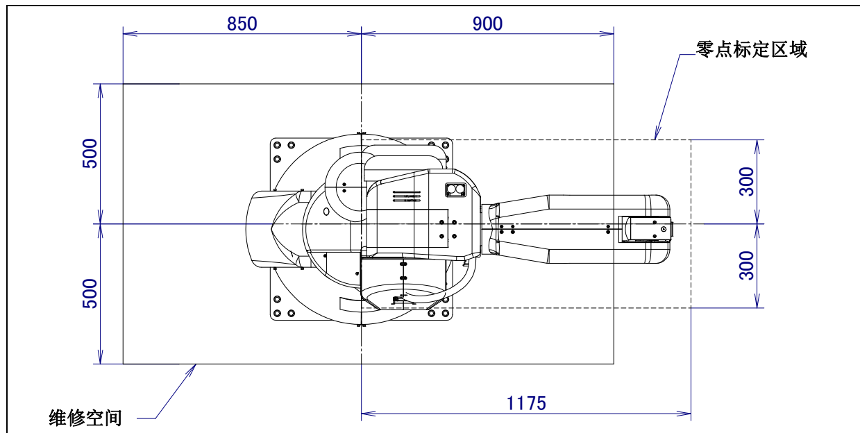
图 1.3 (a) 维修空间的布局图
