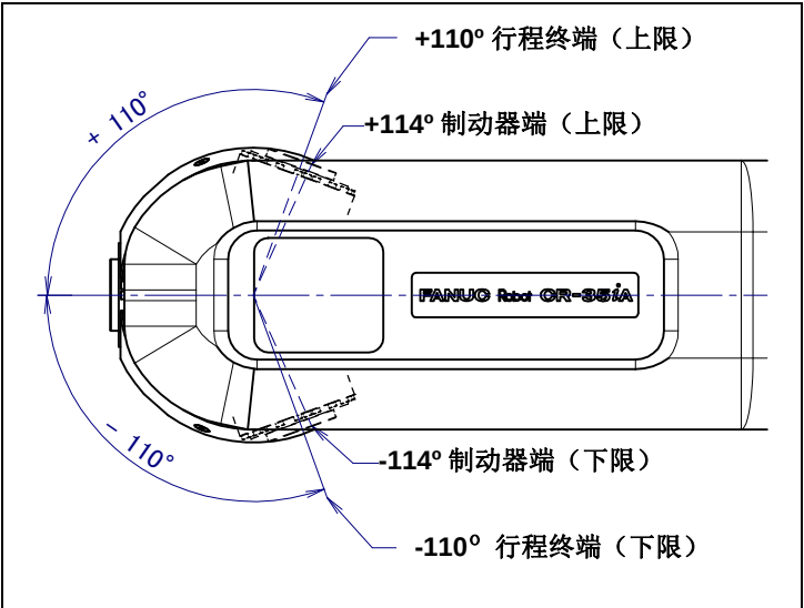
图 3.3 (g) J5 轴可动范围
