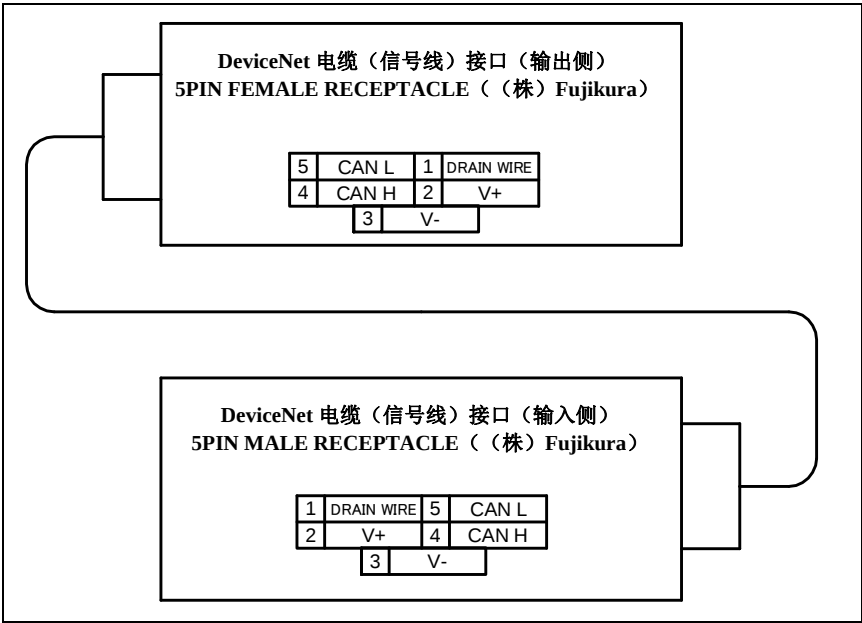
图 5.3 (h) DeviceNet 电缆（信号线）(DS) 接口的插销排列（可选项）
