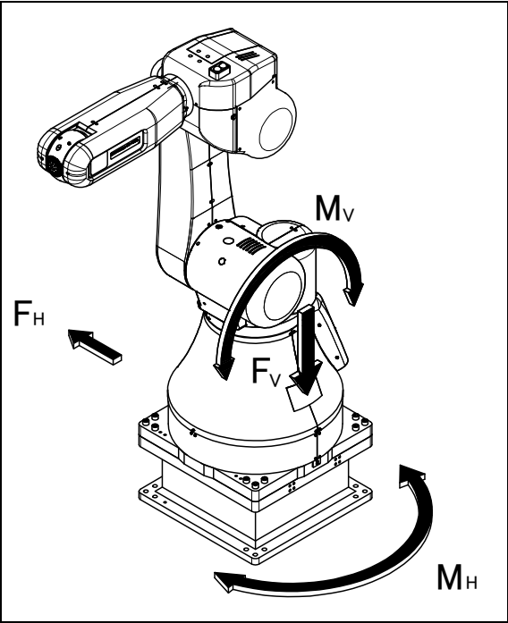
图 1.2 (j) 作用于机器人机座的力和力矩
