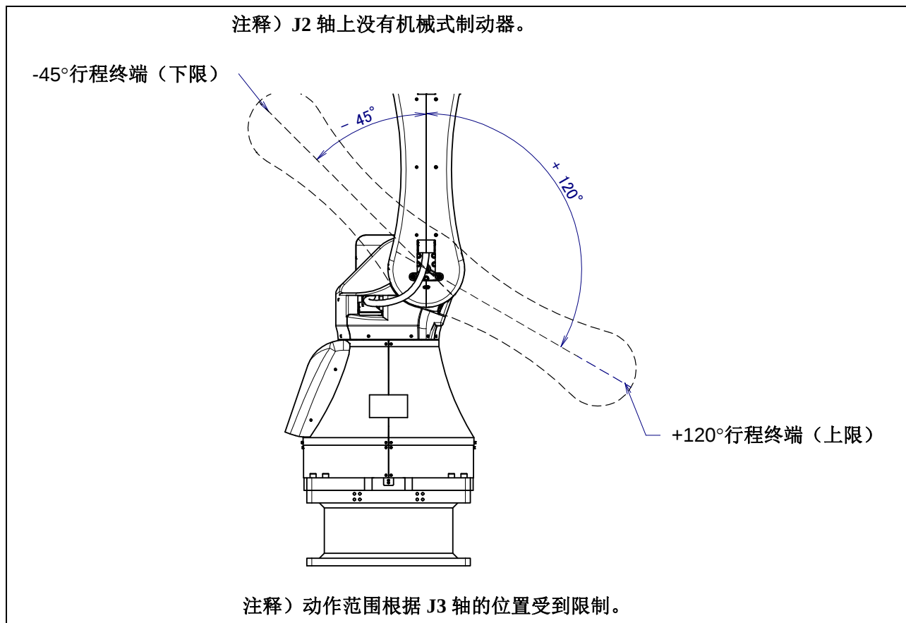
图 3.3 (d) J2 轴可动范围
