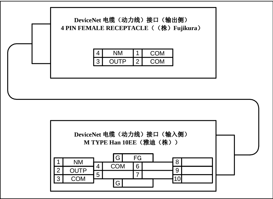
图 5.3 (i) DeviceNet 电缆（动力线）(DP)接口的插销排列（可选项项）
