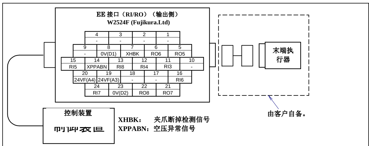
图 5.3 (f) EE 接口(RI/RO)的插针排列 RI*6 点 RO*4 点(可选项项)
