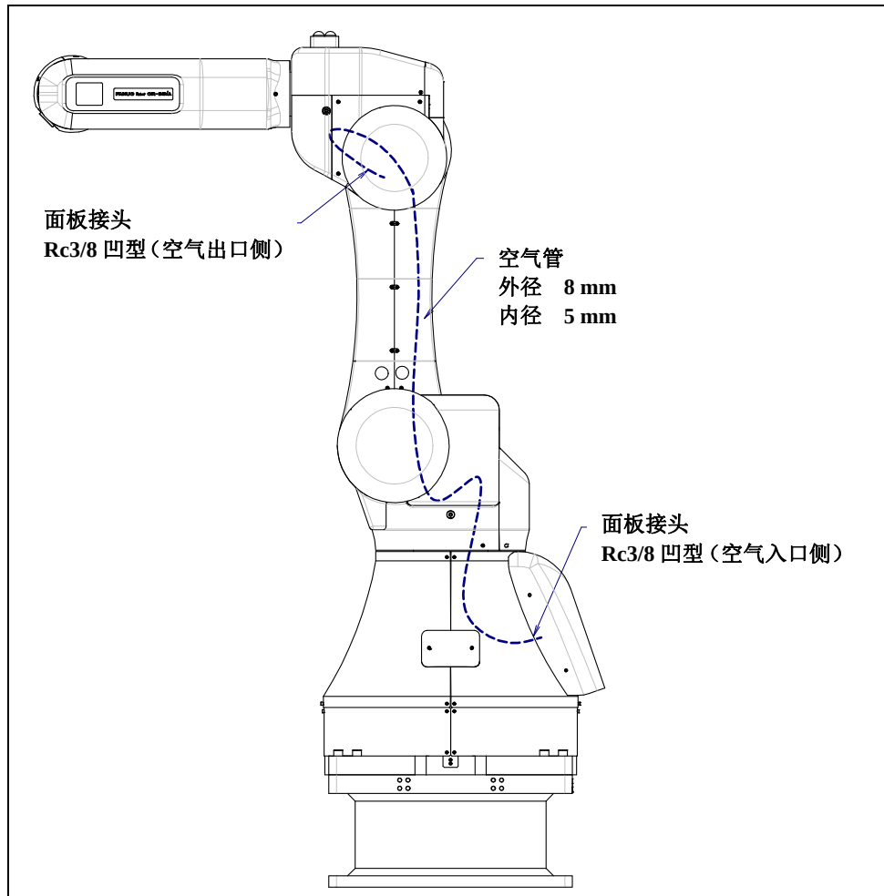
图 5.1 (a) 气压供应口（可选项）
