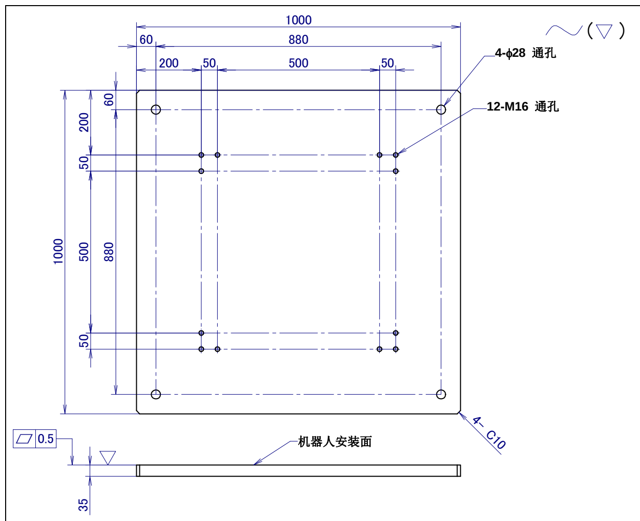
图 1.2 (b) 建议安装用板
