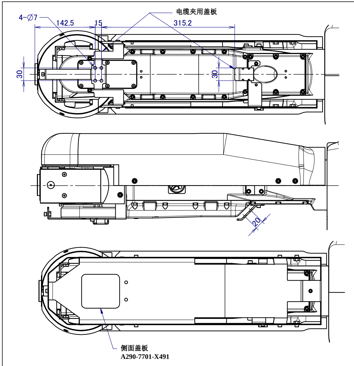
图 4.2 (c) 设备安装面尺寸 (电缆夹用)
