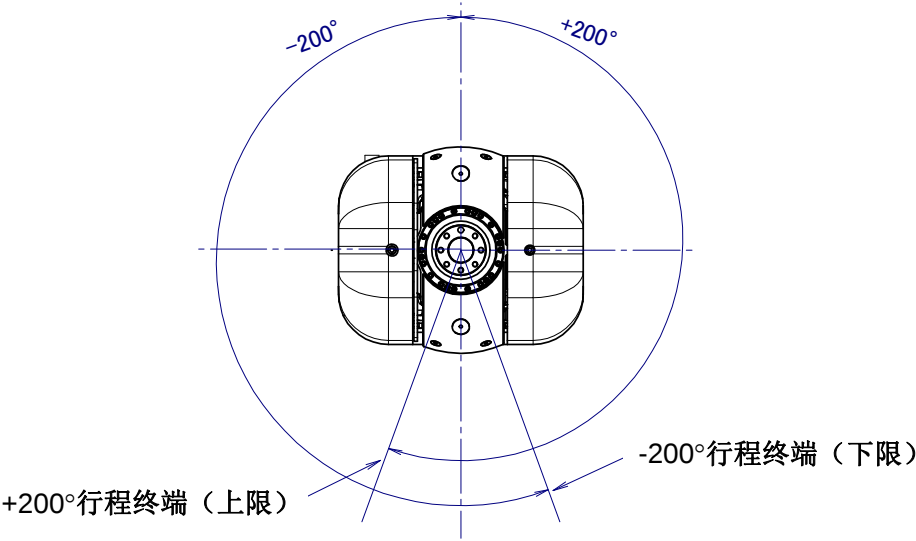
图 3.3 (f) J4 轴可动范围
