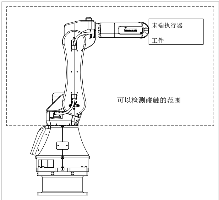
图 3.6 (a) 碰触停止的部分
