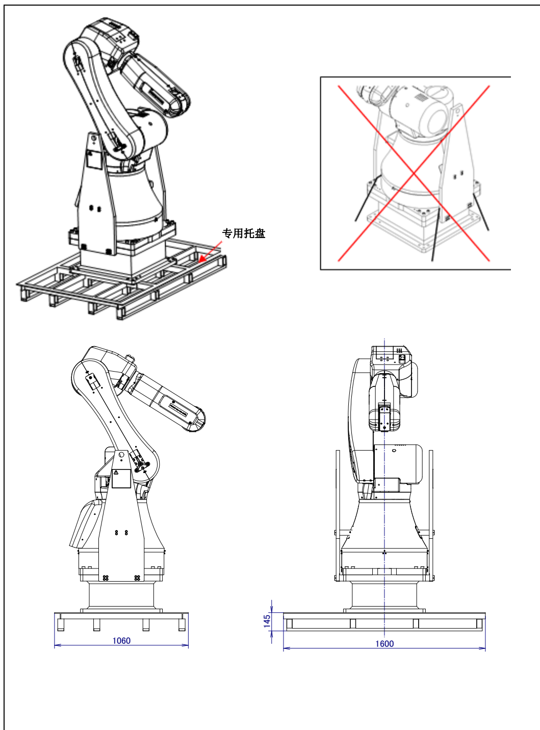
图 1.1 (d) 机器人的发货形态
