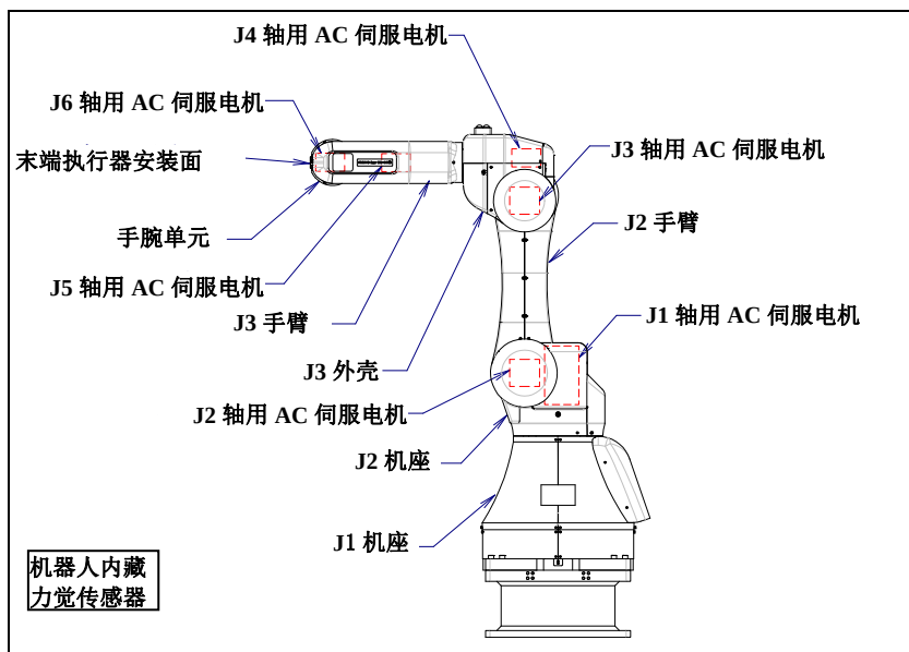
图 3.1 (a) 机构部的构成
