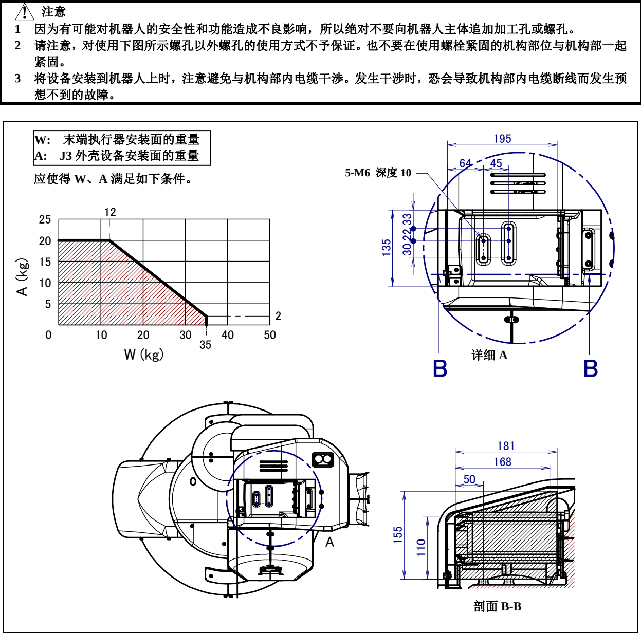
图 4.2 (a) 备安装面尺寸及负载的限制
