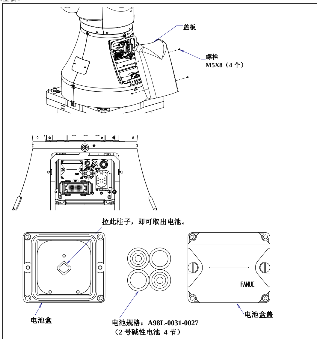
图 7.3.1 (a) 电池的更换
