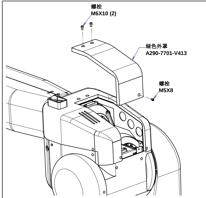
图 4.2 (b) 外罩的拆除
