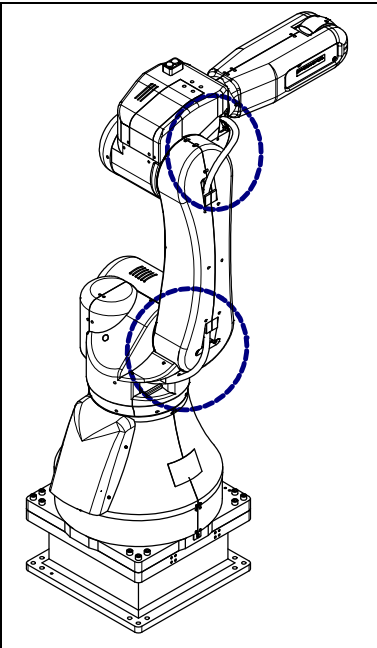
图 7.2.3 (a) 机构部内电缆的检修部位
