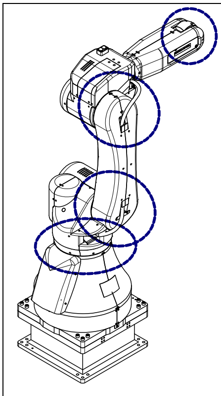
图 7.2.1 (a) 渗油的检查部位
