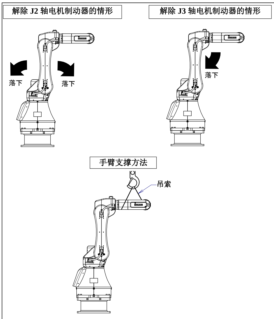
图 5.10 (a) 解除 J2、J3 轴的电机制动器造成的手臂动作和事先采取的措施例
