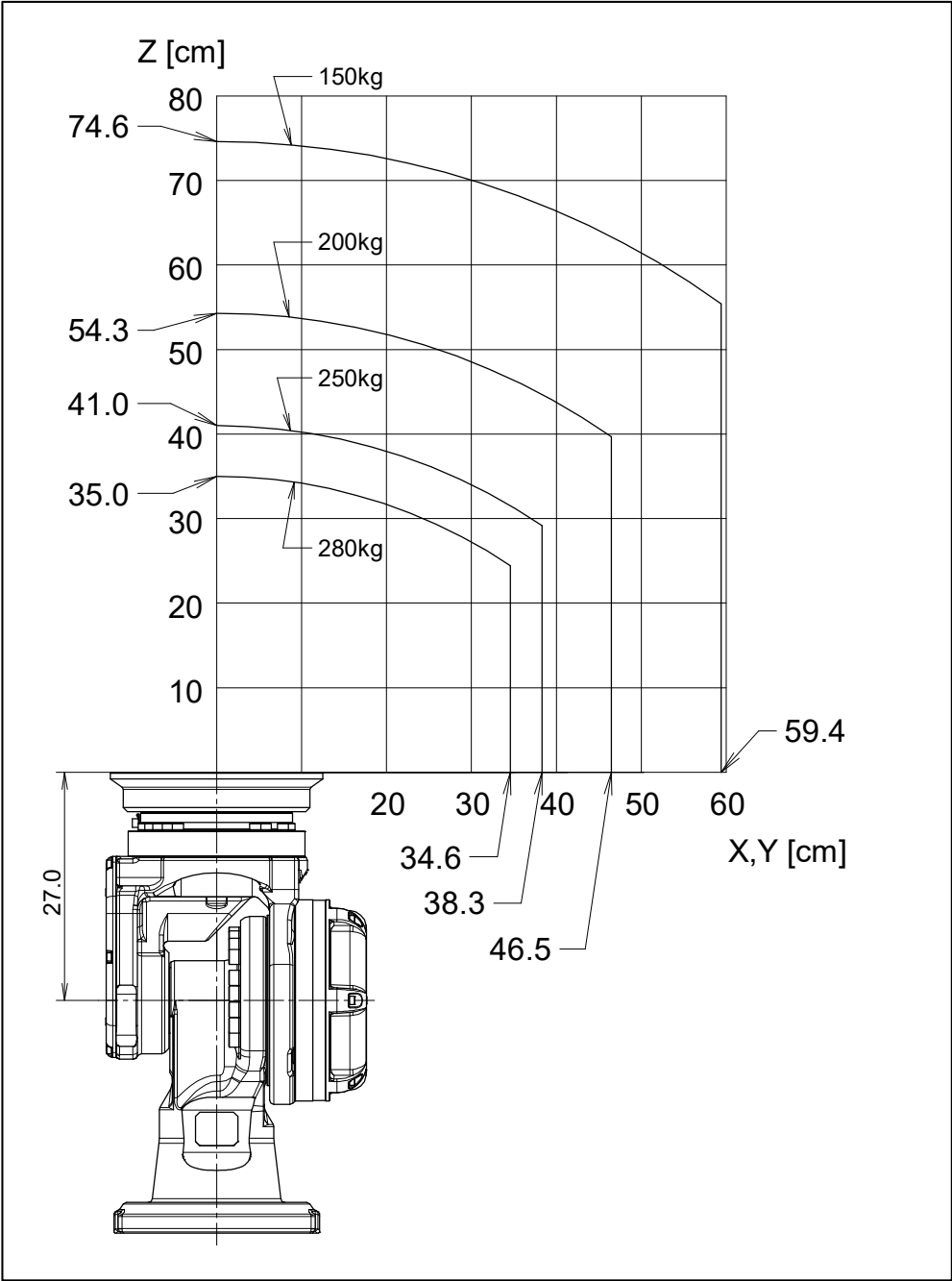
图 3.4 (d) 手腕部允许负载线图 (绝缘 ISO 法兰盘) (M-900iB/280L)
