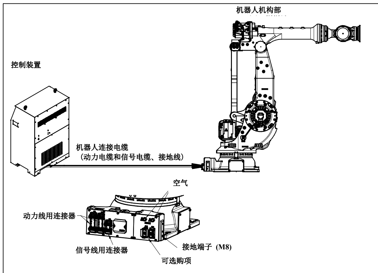
图 2 (a) 电缆连接图
