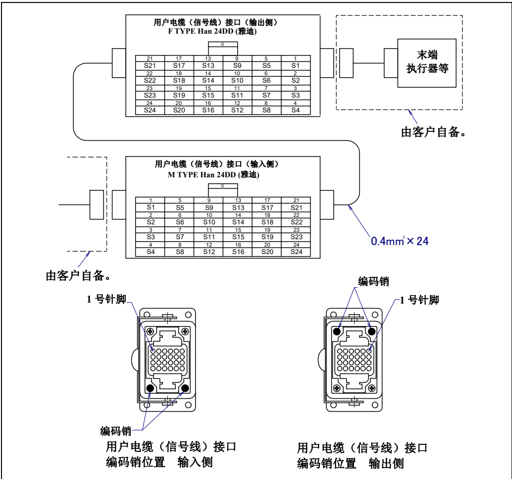
图 5.3 (g) 用户电缆（信号线）(AS) 接口的插针排列和编码销的配置位置（可选项项）
