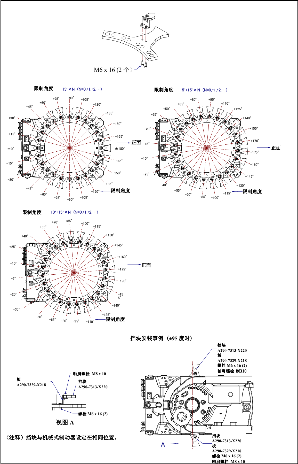
图 6.3 (a) J1 轴的挡块位置和动作范围 (可选项)
