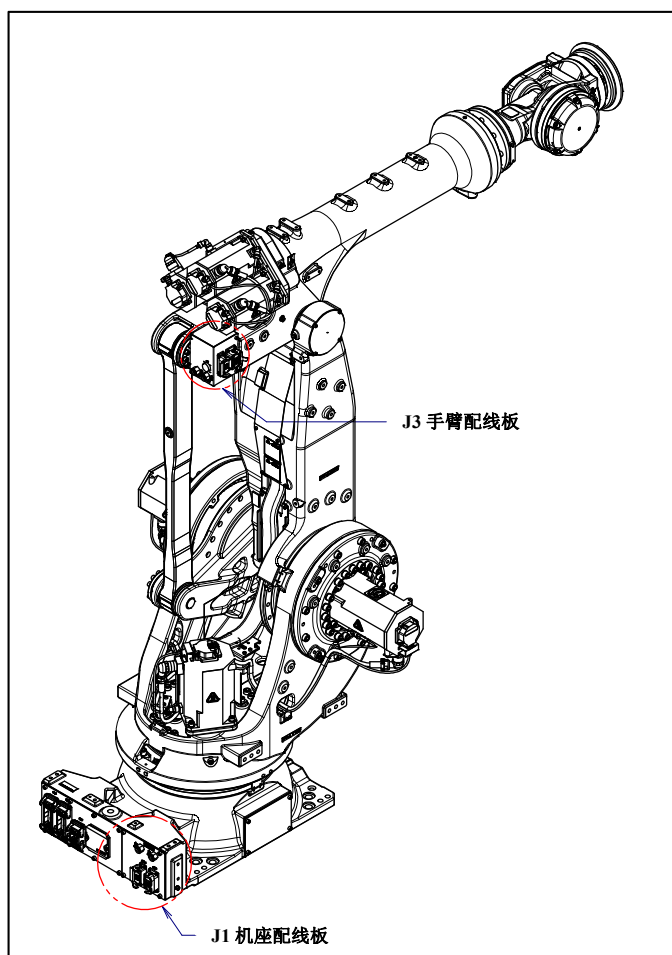
图 5.3 (a) 可选项项电缆用接口的位置（可选项项）
