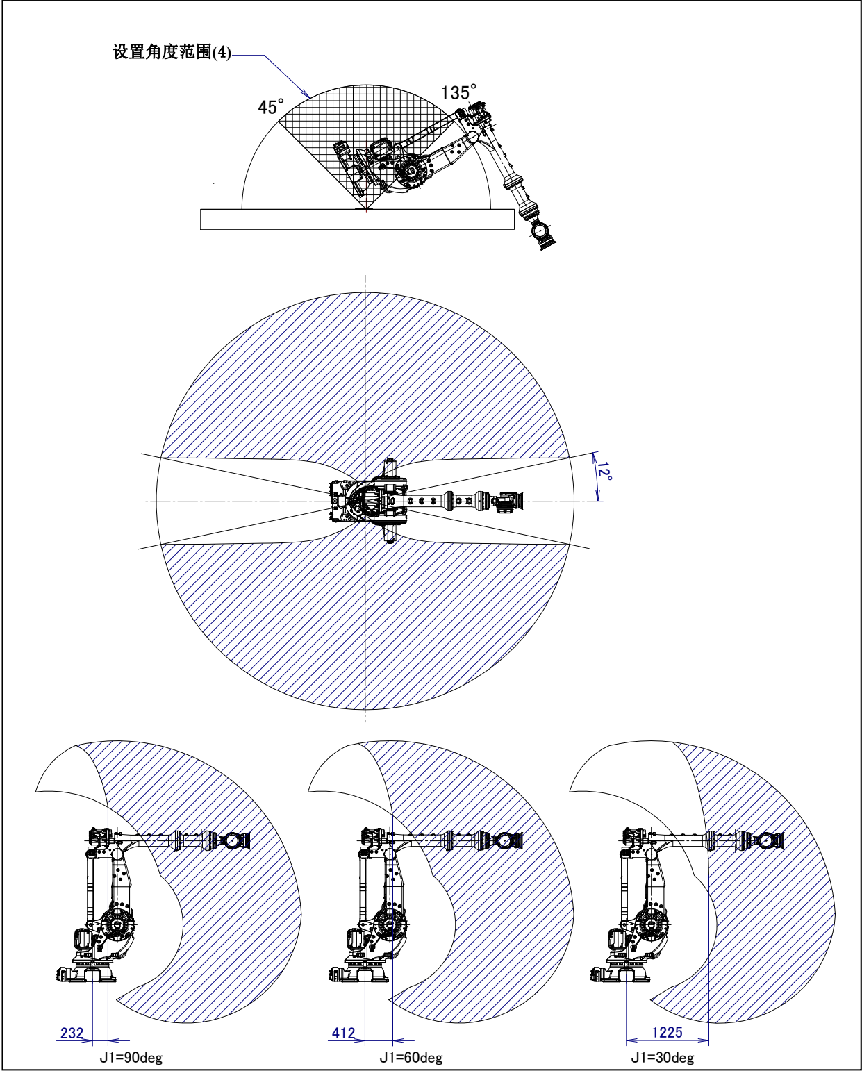
图 3.6 (h) 机器人设置角度范围(4)的动作范围 (45°< \phi <135°) (M-900iB/280L)
