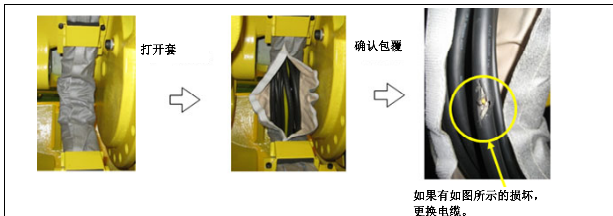
图 7.2.3 (c) 电缆的确认方法
