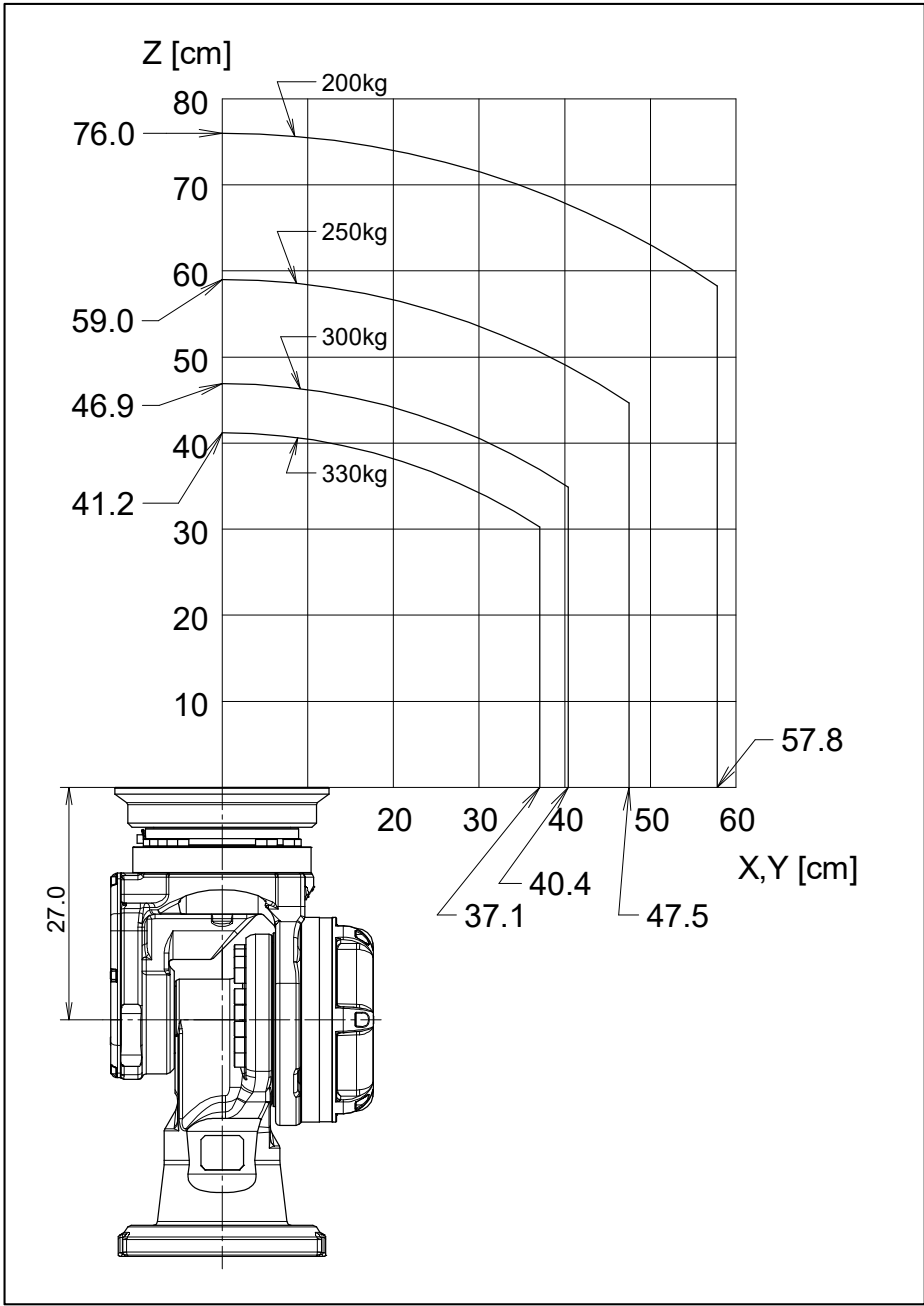
图 3.4 (h) 手腕部允许负载线图（绝缘 ISO 法兰盘） (M-900iB/330L)
