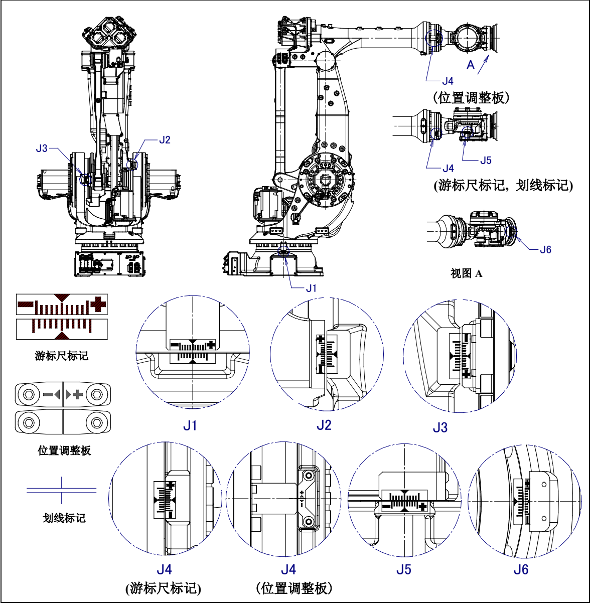
图 8.3 (a) 各轴的对合标记位置
