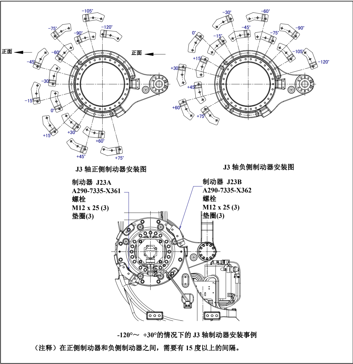
图 6.2.1 (e) J3 轴机械式可变制动器的安装
