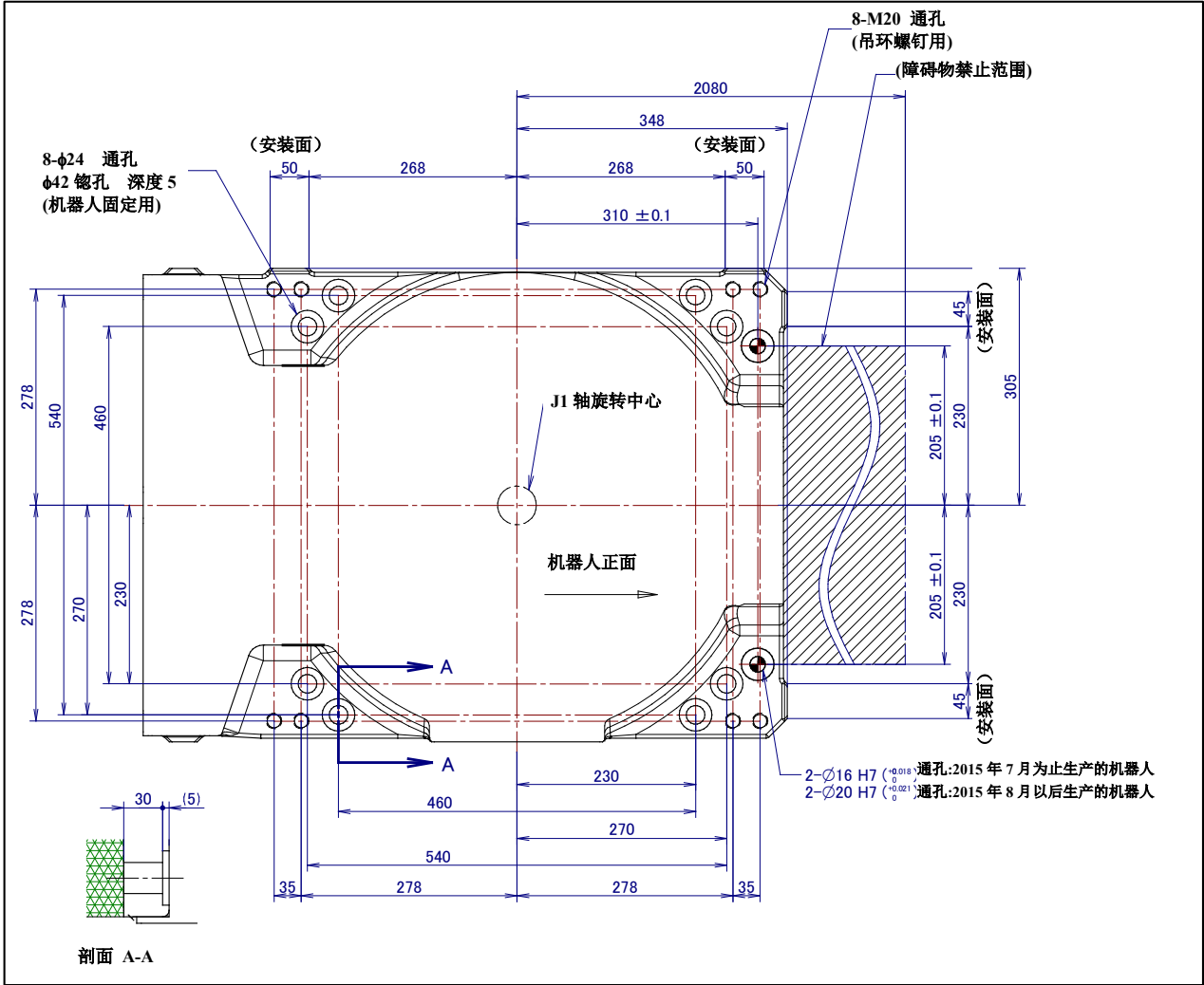
图 1.2 (a) 机器人机座尺寸
