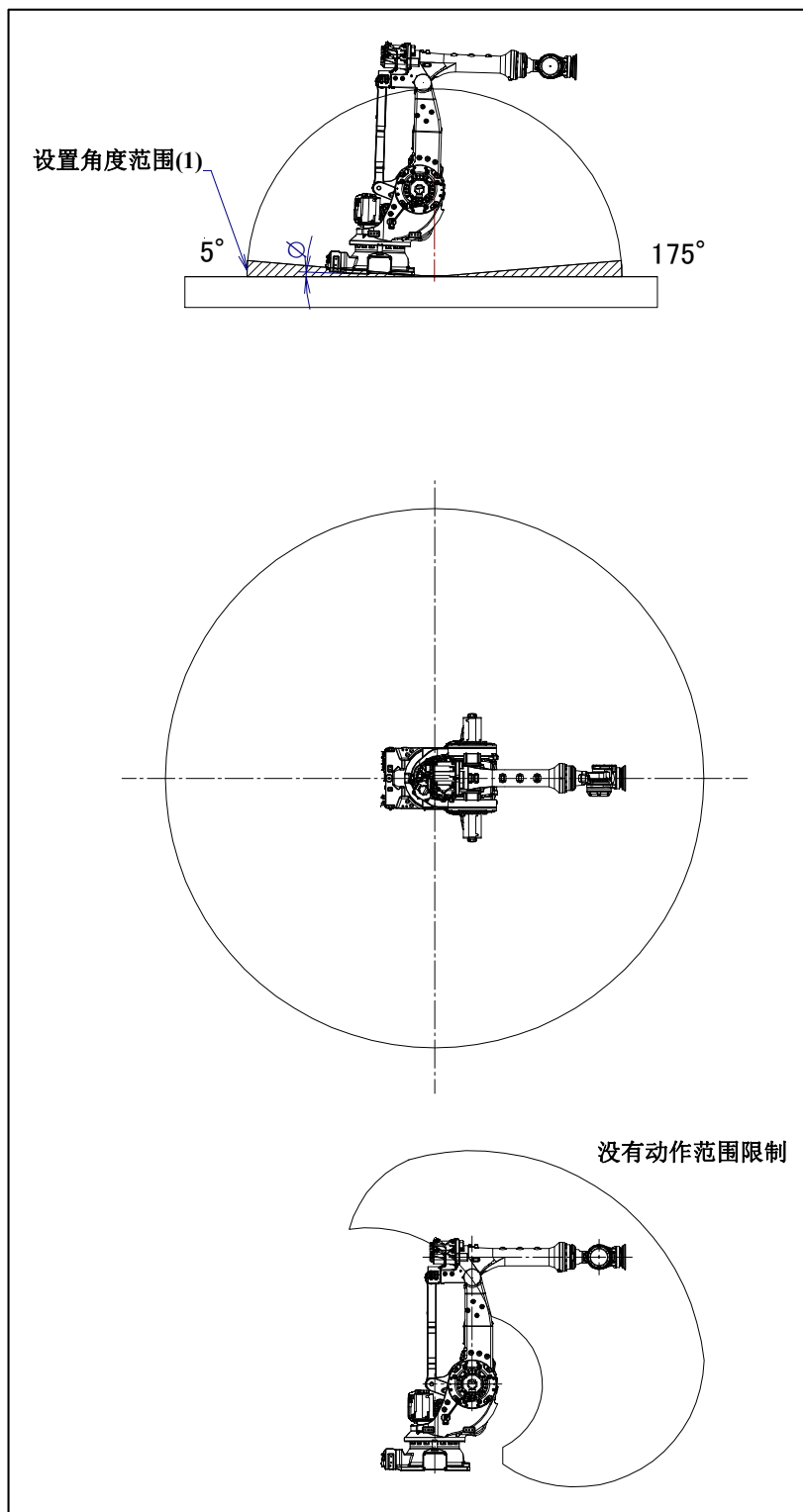
图 3.6 (a) 机器人设置角度范围(1)的动作范围 (0^\circ \leq \phi \leq 5^\circ, 175^\circ \leq \phi \leq 180^\circ) (M-900iB/360)
