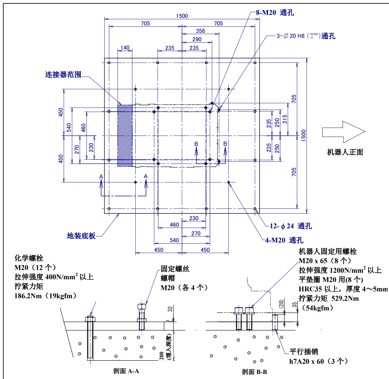
图 1.2.1 (b) 具体安装例 II
