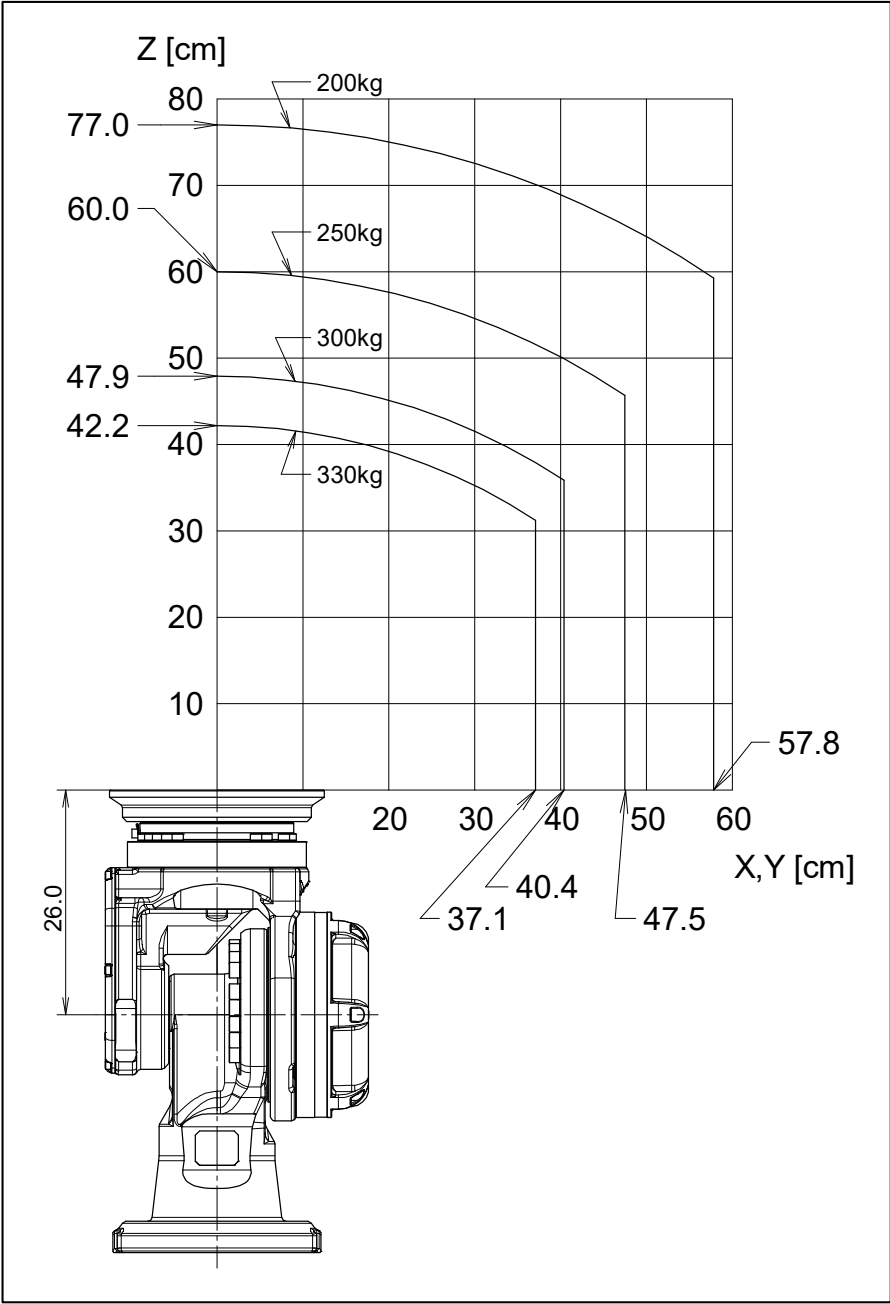
图 3.4 (g) 手腕部允许负载线图 (ISO 法兰盘) (M-900iB/330L)
