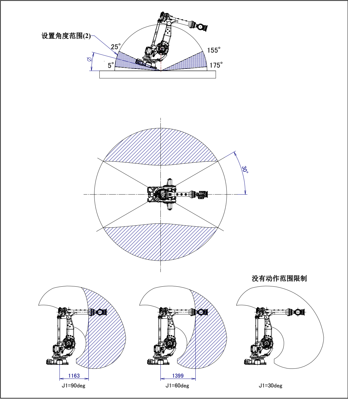
图 3.6 (b) 机器人设置角度范围(2)的动作范围 ( 5^\circ < \phi \leq 25^\circ , 155^\circ \leq \phi < 175^\circ ) (M-900iB/360)
