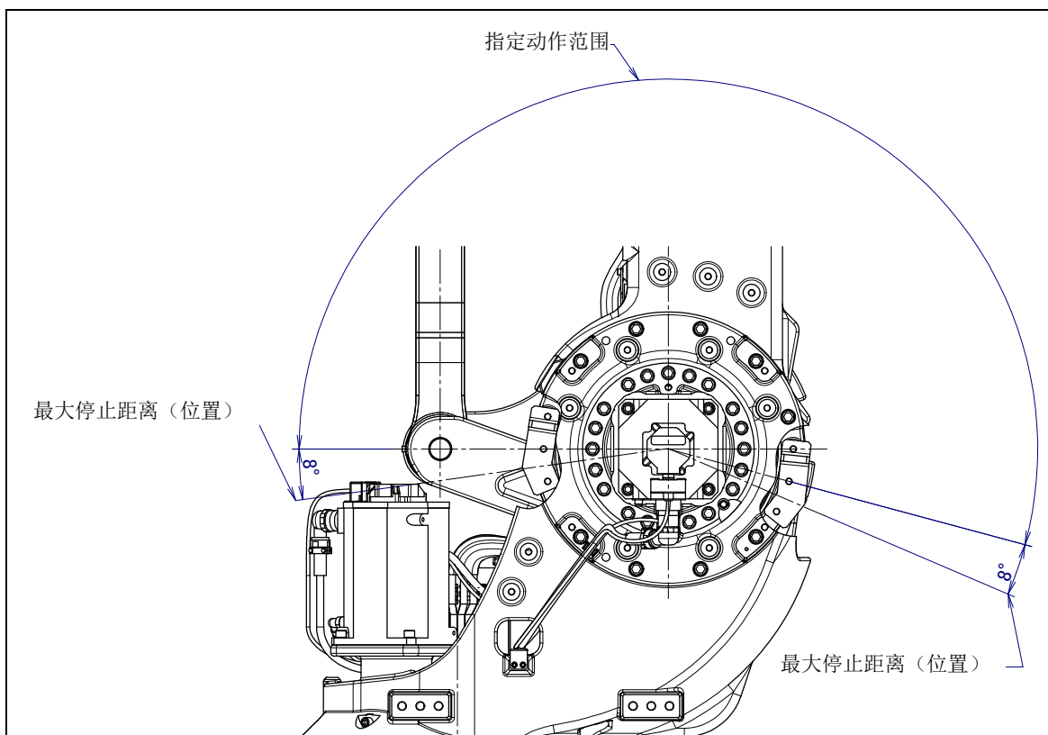
图 6.2.3 (b) J2 轴机械式可变制动器的最大停止距离 (位置)
