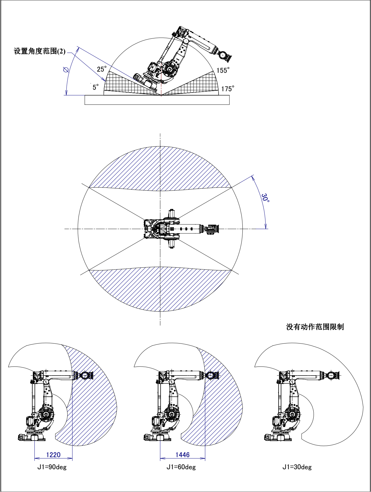
图 3.6 (j) 机器人设置角度范围(2)的动作范围 ( 5^\circ < \phi \leq 25^\circ , 155^\circ \leq \phi < 175^\circ ) (M-900iB/280)
