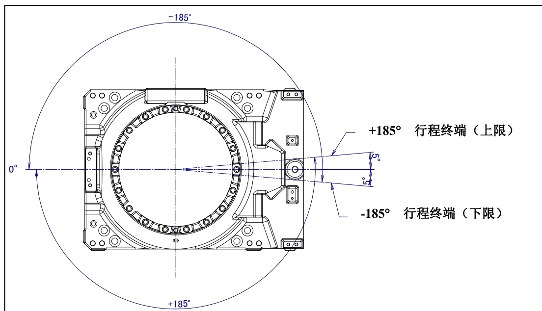
图 3.3 (b) J1 轴可动范围（不指定机械式制动器时）
