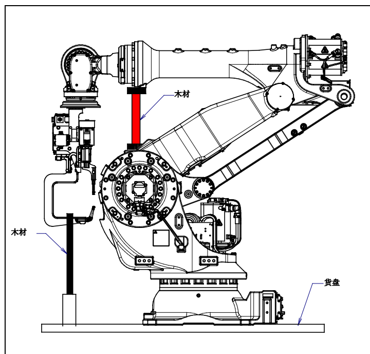
图 1.1.1 (a) 安装着末端执行器时搬运时的固定例
