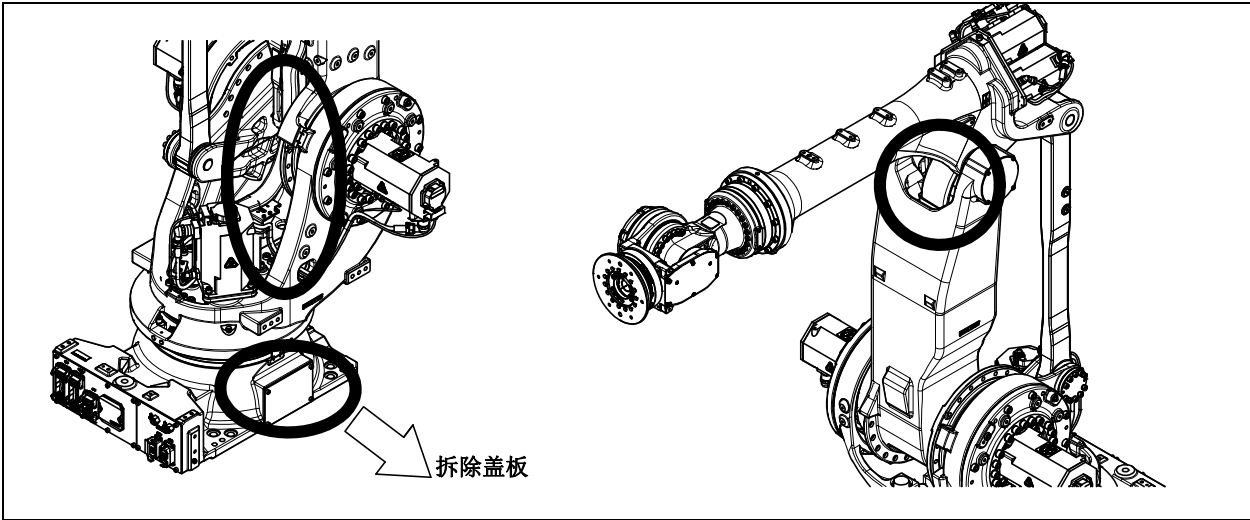
图 7.2.3 (a) 机构部内电缆的确认部位
