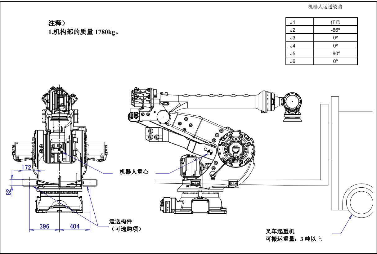
图 1.1 (i) 采用叉车起重机搬运(M-900iB/330L)
