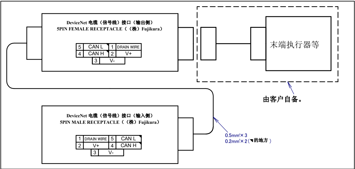
图 5.3 (j) DeviceNet 电缆（信号线）(DS)接口的插针排列（可选项）
