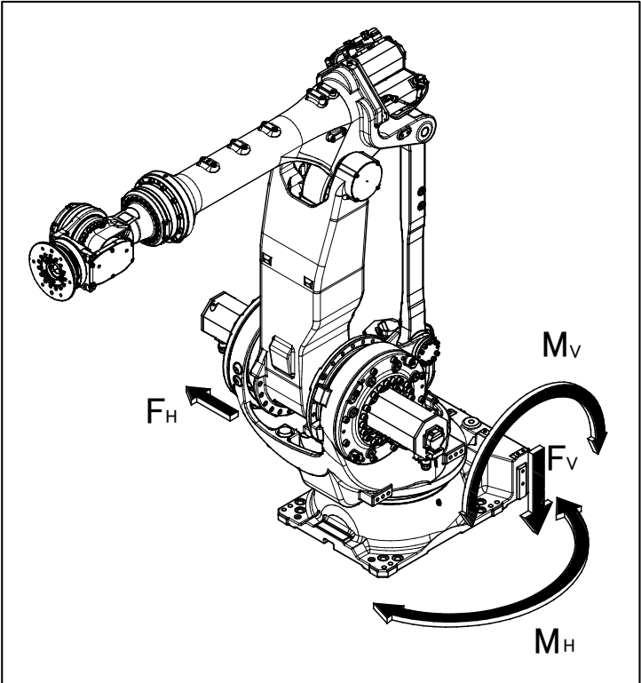
图 1.2.1 (d) 断电停止时作用的力以及力矩
