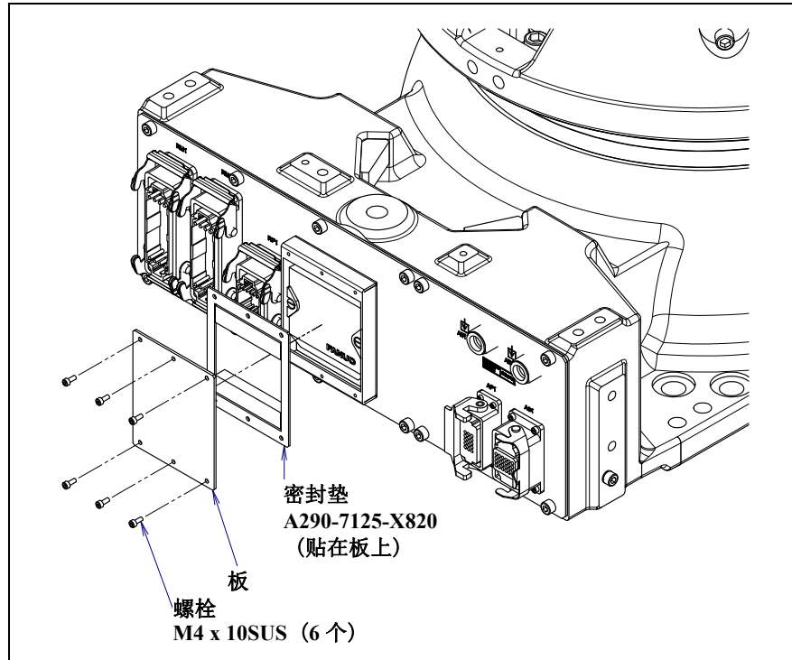
图 7.3.1 (b) 电池盖板的拆除 (指定防尘防液强化可选项时)
