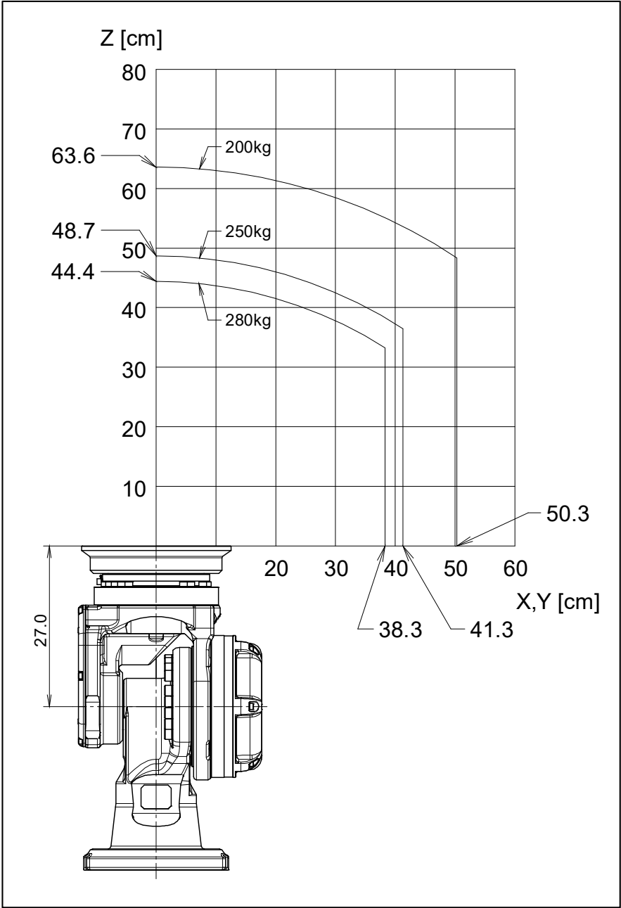
图 3.4 (f) 手腕部允许负载线图（绝缘 ISO 法兰盘） (M-900iB/280)
