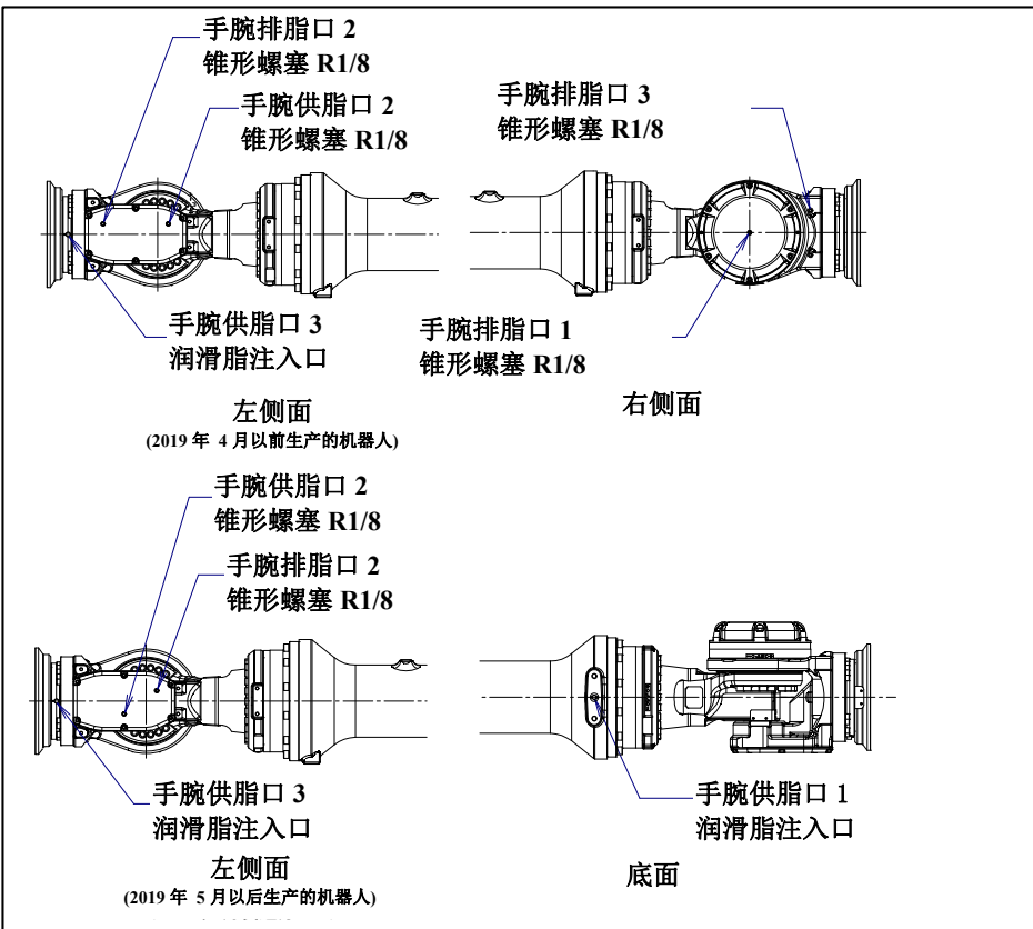
图 7.3.3 (b) 手腕的润滑脂的更换
