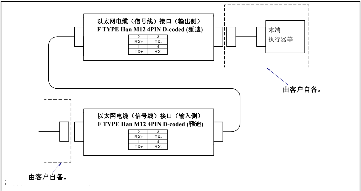
图 5.3 (n) 以太网电缆（信号线）(ES)接口的插针排列（可选项项）
