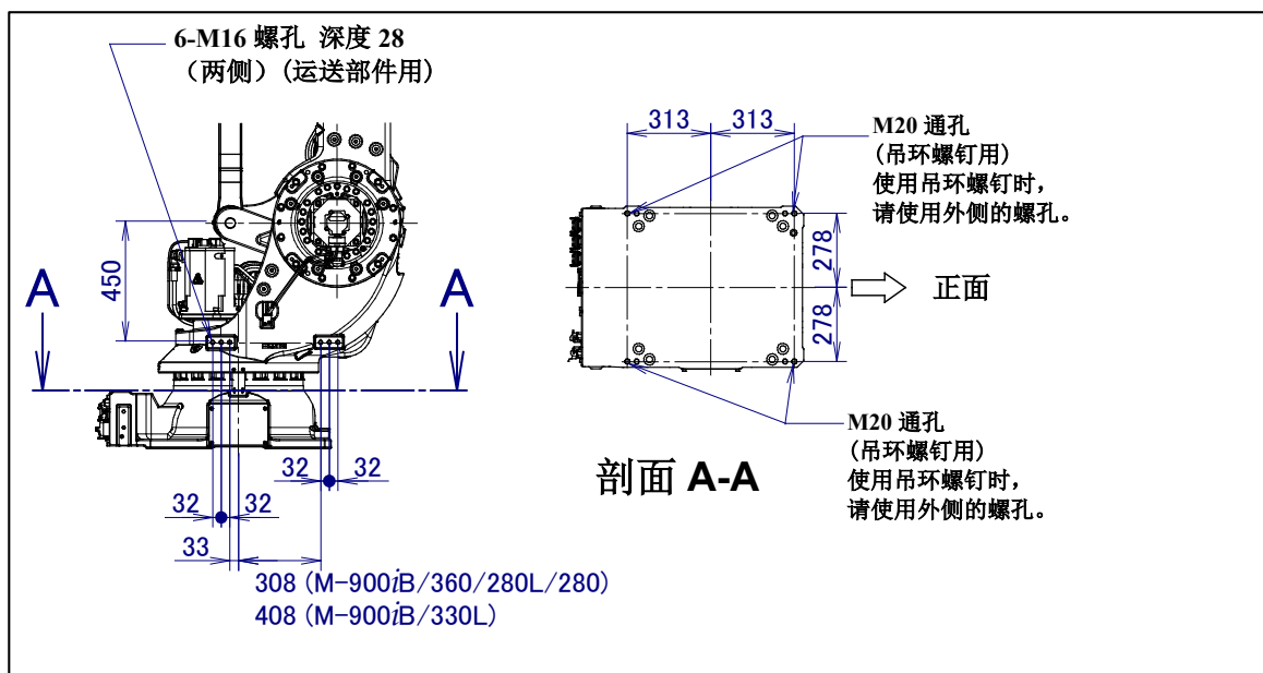
图 1.1 (a) 吊环螺钉、搬运构件安装位置
