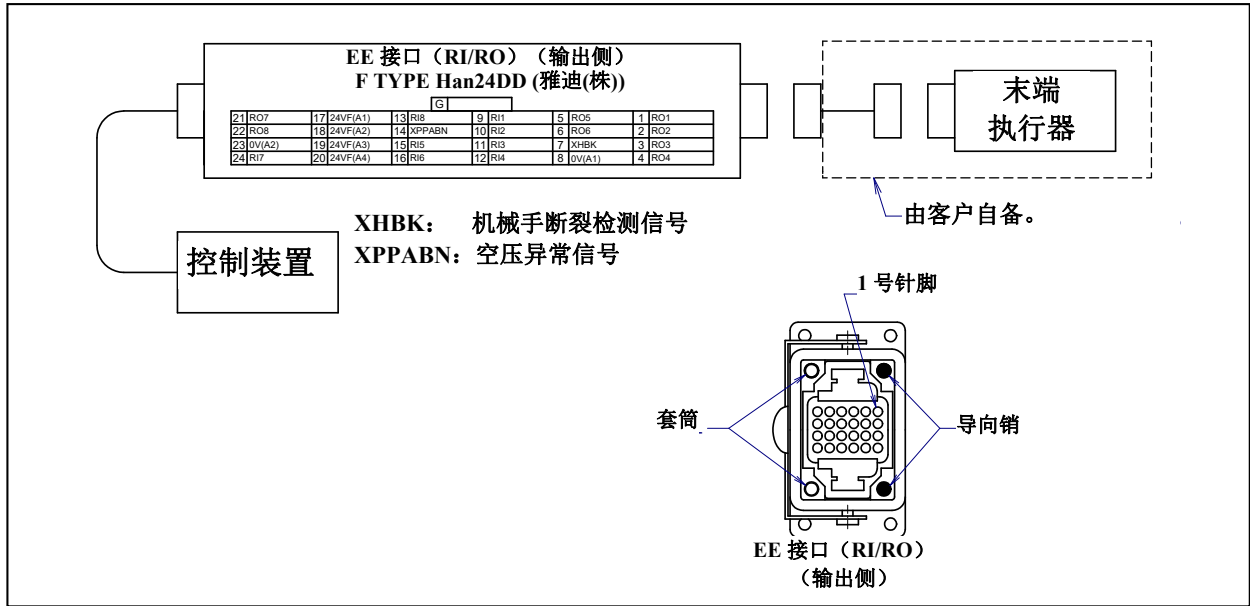
图 5.3 (p) EE 接口(RI/RO)的插针排列 (可选项)
