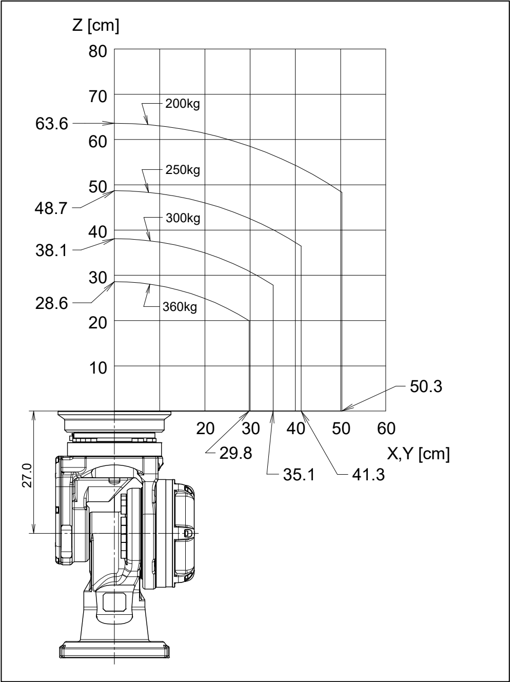
图 3.4 (b) 手腕部允许负载线图（绝缘 ISO 法兰盘） (M-900iB/360)
