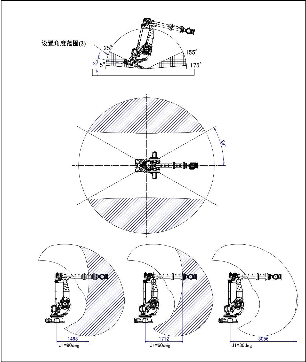
图 3.6 (f) 机器人设置角度范围(2)的动作范围 ( 5^\circ < \phi \leq 25^\circ , 155^\circ \leq \phi < 175^\circ ) (M-900iB/280L)
