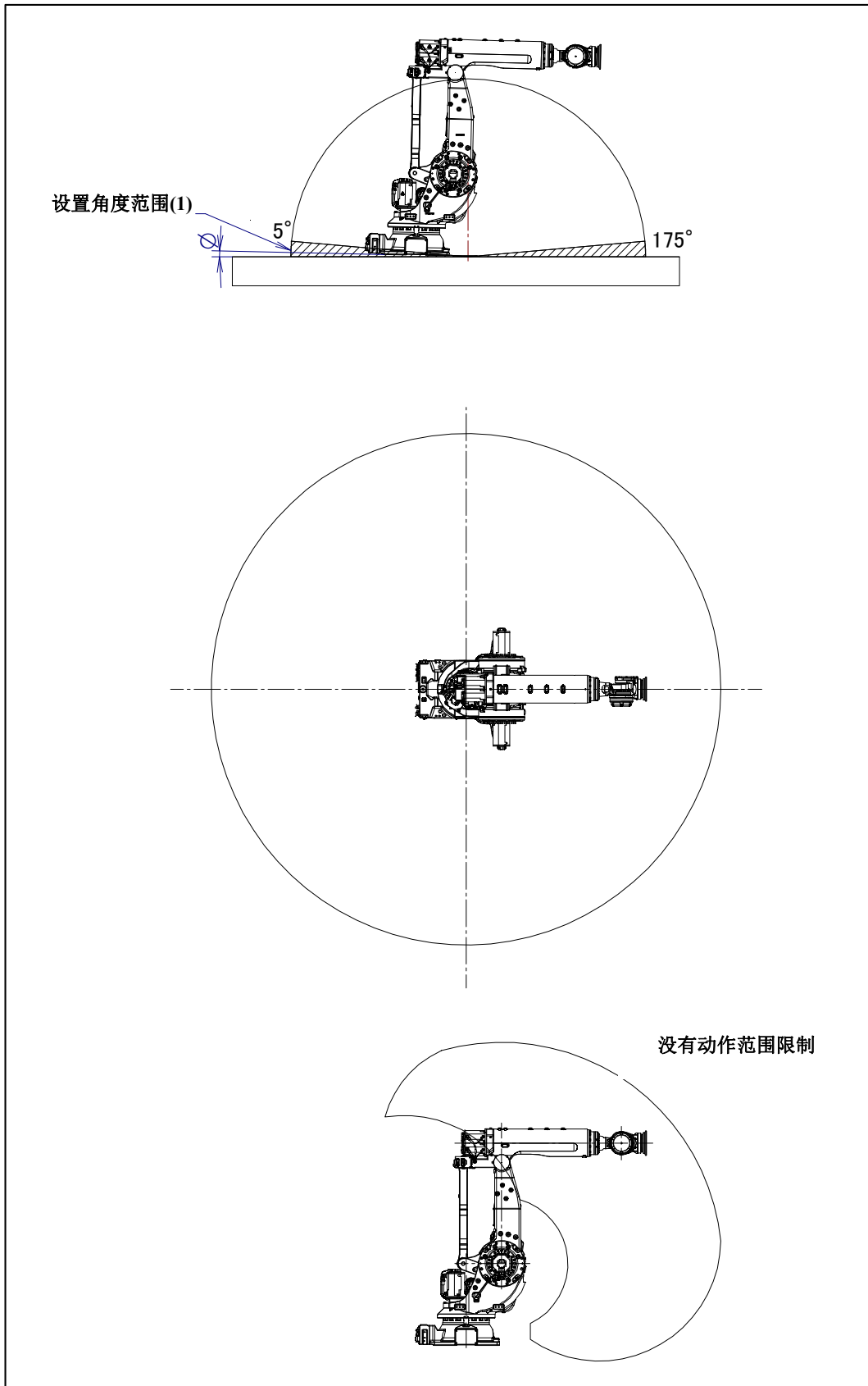
图 3.6 (i) 机器人设置角度范围(1)的动作范围 (0^\circ \leq \phi \leq 5^\circ, 175^\circ \leq \phi \leq 180^\circ) (M-900iB/280)
