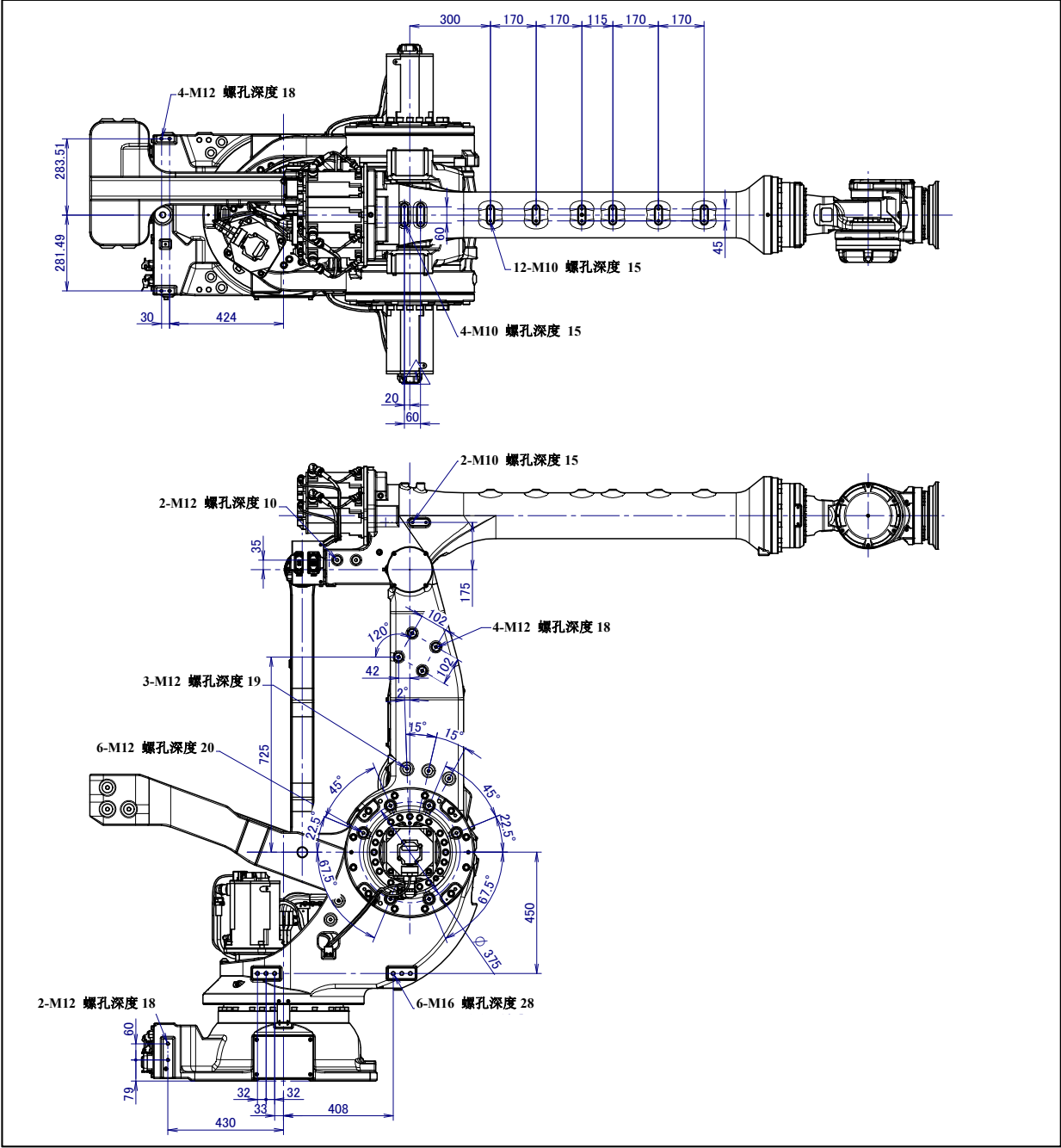
图 4.2 (g) 设备安装面尺寸 (M-900iB/330L (1/2))
