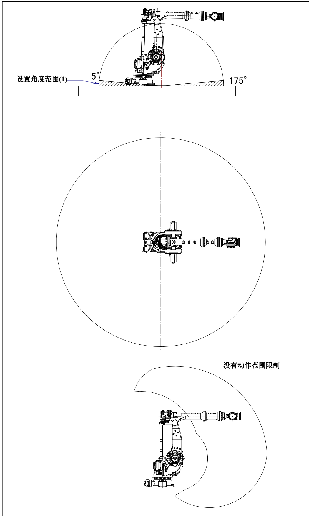
图 3.6 (e) 机器人设置角度范围(1)的动作范围 ( 0^{\circ} \leq \phi \leq 5^{\circ} , 175^{\circ} \leq \phi \leq 180^{\circ} ) (M-900iB/280L)
