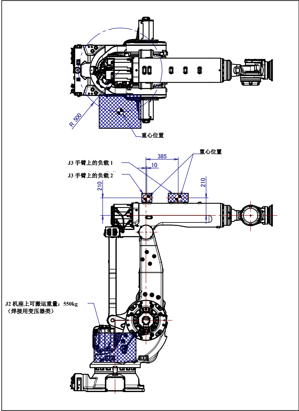
图 3.5 (b) J2 机座/J3 手臂上的负载条件 (M-900iB/280)
