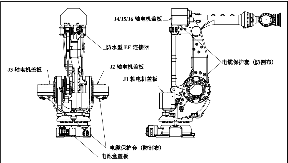
图 10.2 (a) 防尘防液强化组件的构成
