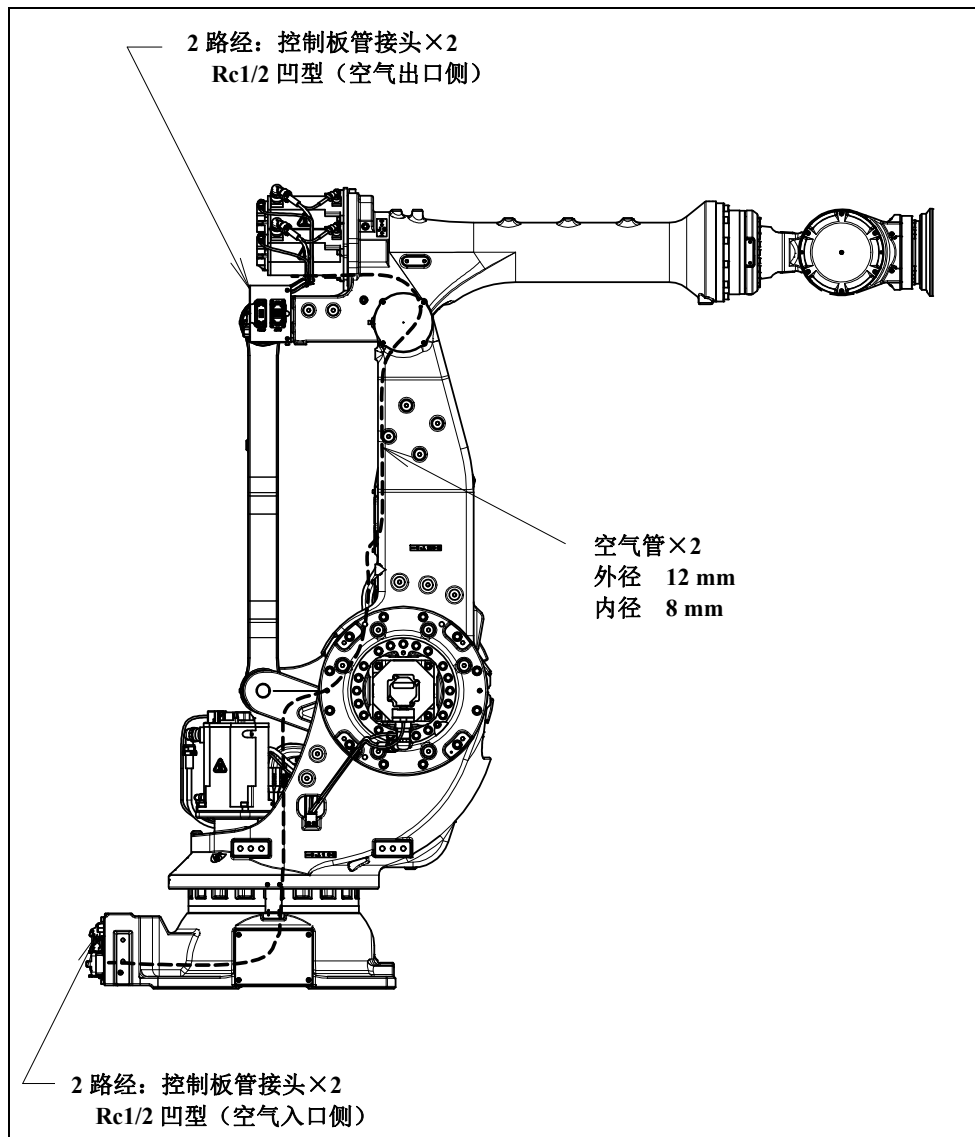
图 5.1 (a) 气压供应口（可选项）
