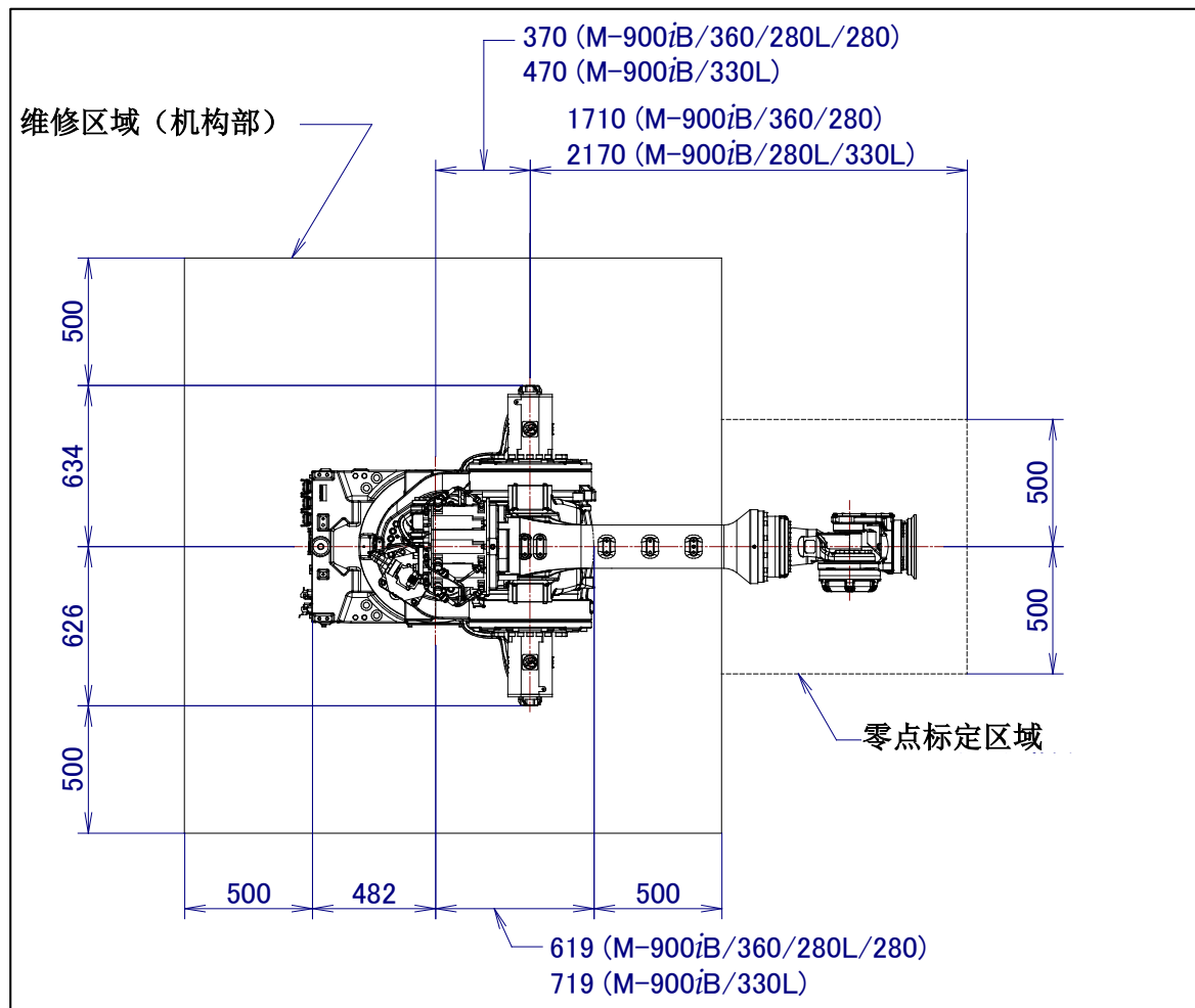
图 1.3 (a) 维修空间的布局图
