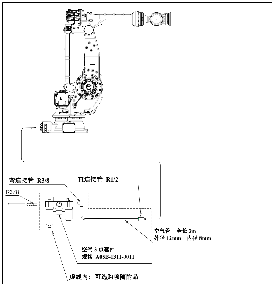
图 5.2 (a) 空气配管（可选项项）
