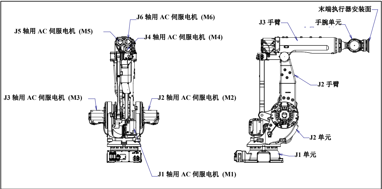
图 3.1 (b) 机构部的构成 (M-900iB/280)
