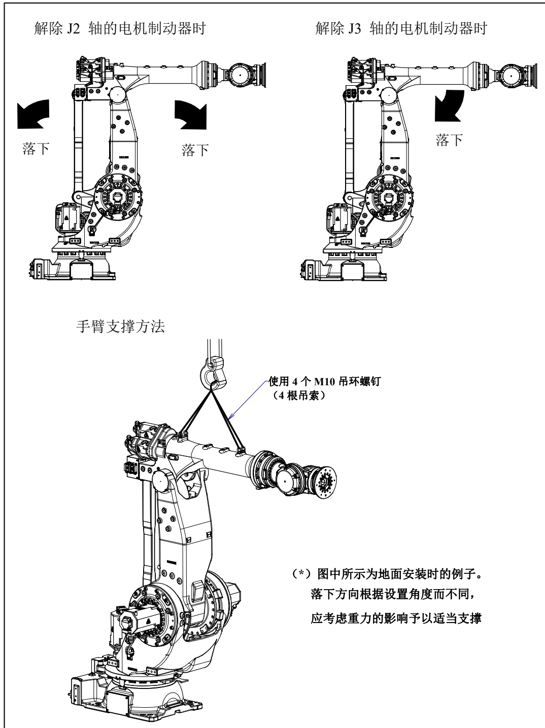
图 3 (a) 解除 J2/J3 轴的电机制动器造成的手臂动作和事先采取的措施例
