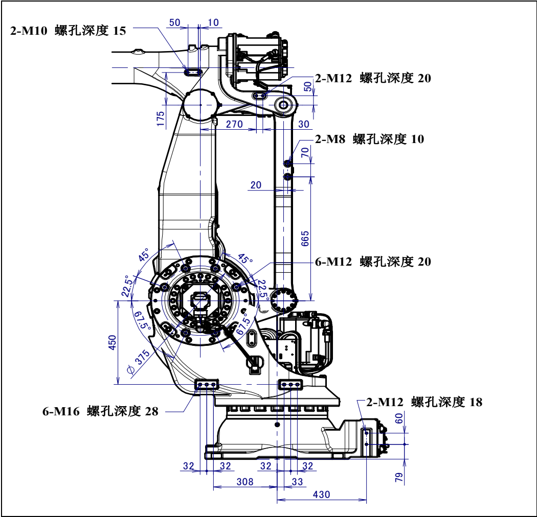
图 4.2 (d) 设备安装面尺寸 (M-900iB/280L (2/2))
