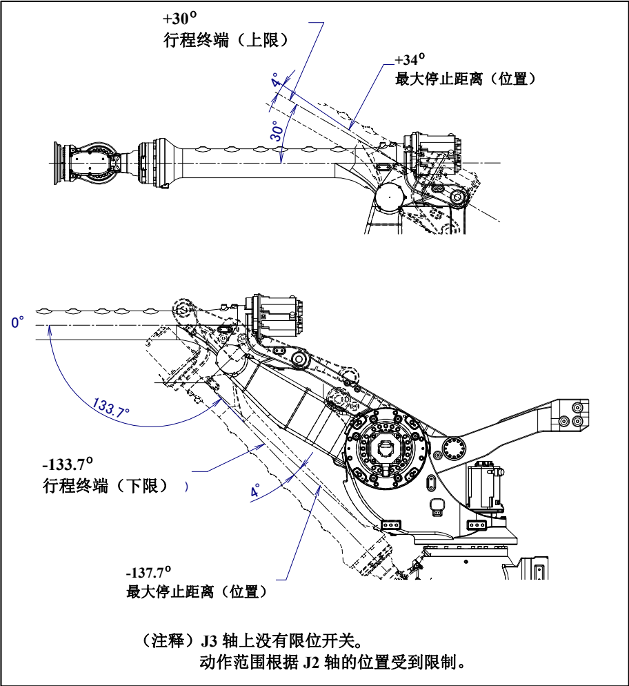
图 3.3 (f) J3 轴可动范围(M-900iB/330L)
