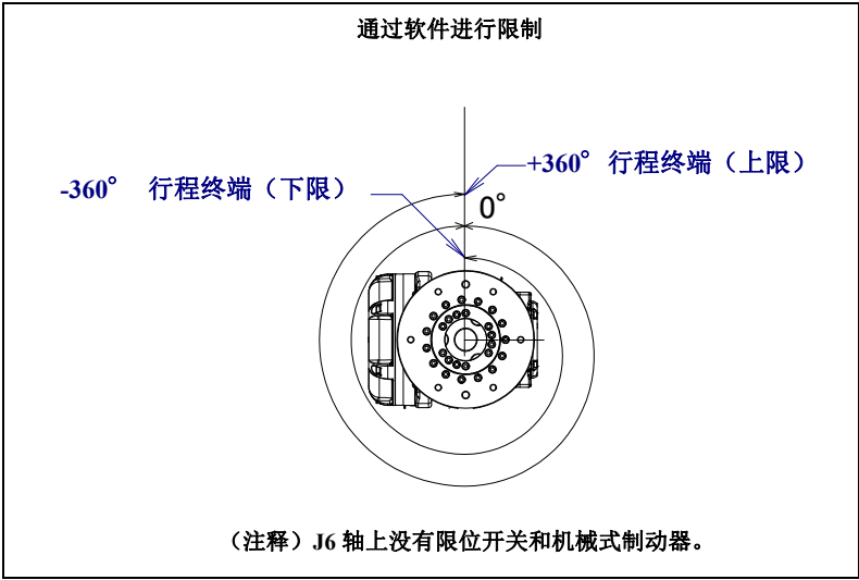
图 3.3 (i) J6 轴可动范围
