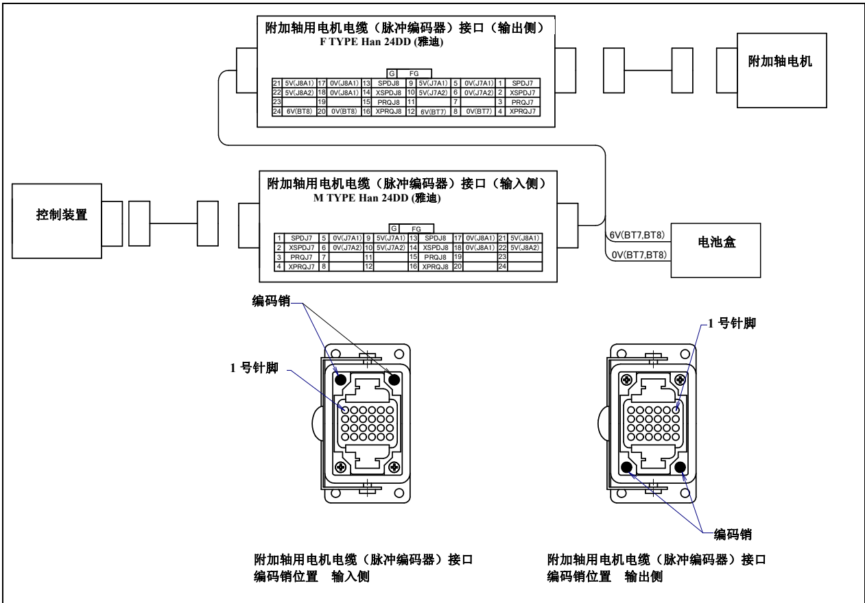
图 5.3 (I) 附加轴用电机电缆（脉冲编码器线）(ARP)接口的插针排列和编码销配置位置（可选项项）
