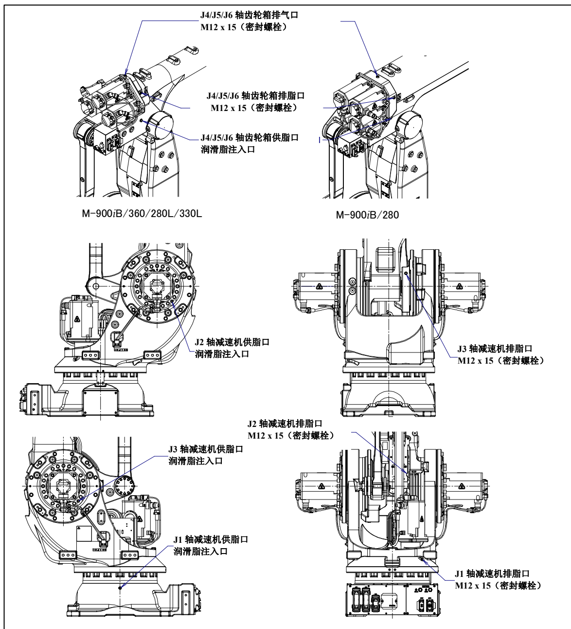
图 7.3.3 (a) J1, J2, J3 轴减速机和 J4/J5/J6 轴齿轮箱的润滑脂的更换
