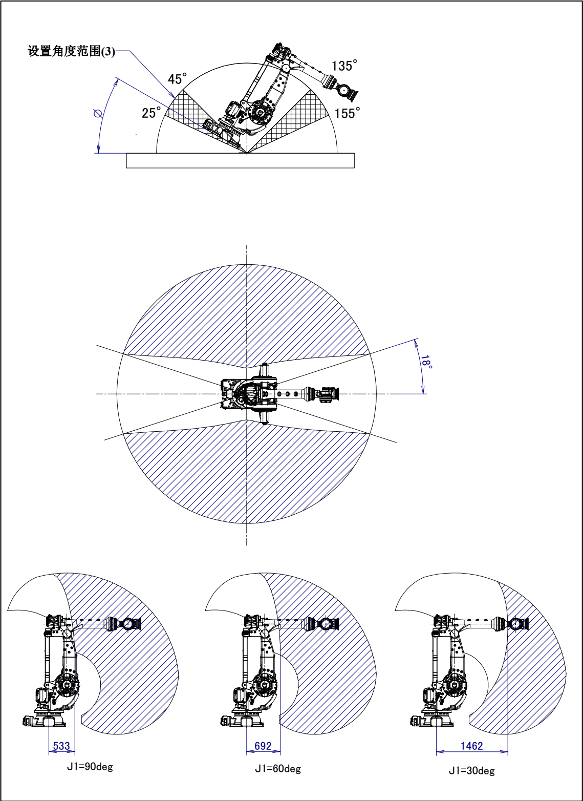
图 3.6 (c) 机器人设置角度范围(3)的动作范围 ( 25^{\circ} < \phi \leq 45^{\circ} , 135^{\circ} \leq \phi < 155^{\circ} ) (M-900iB/360)
