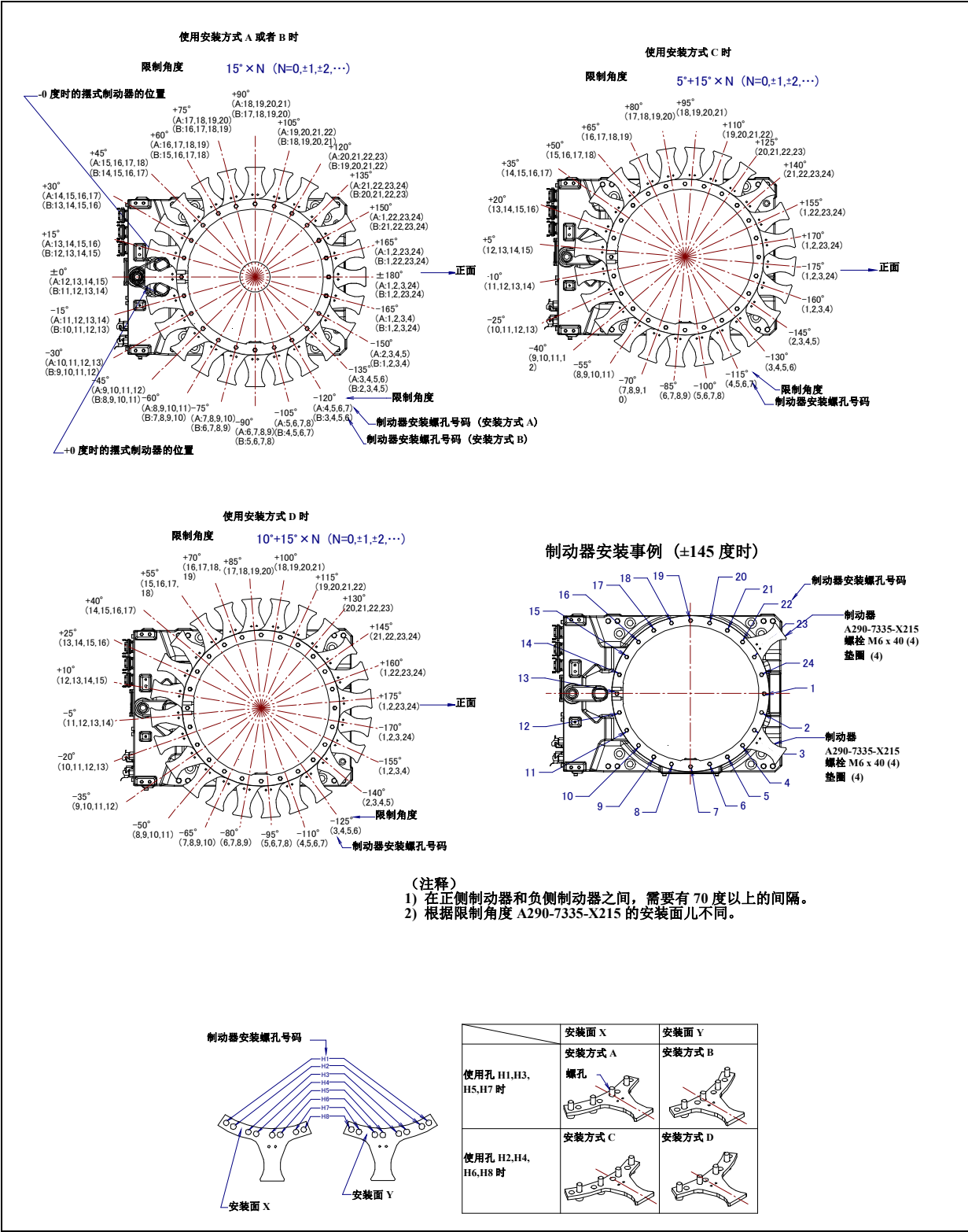
图 6.2.1 (b) J1 轴机械式可变制动器的安装
