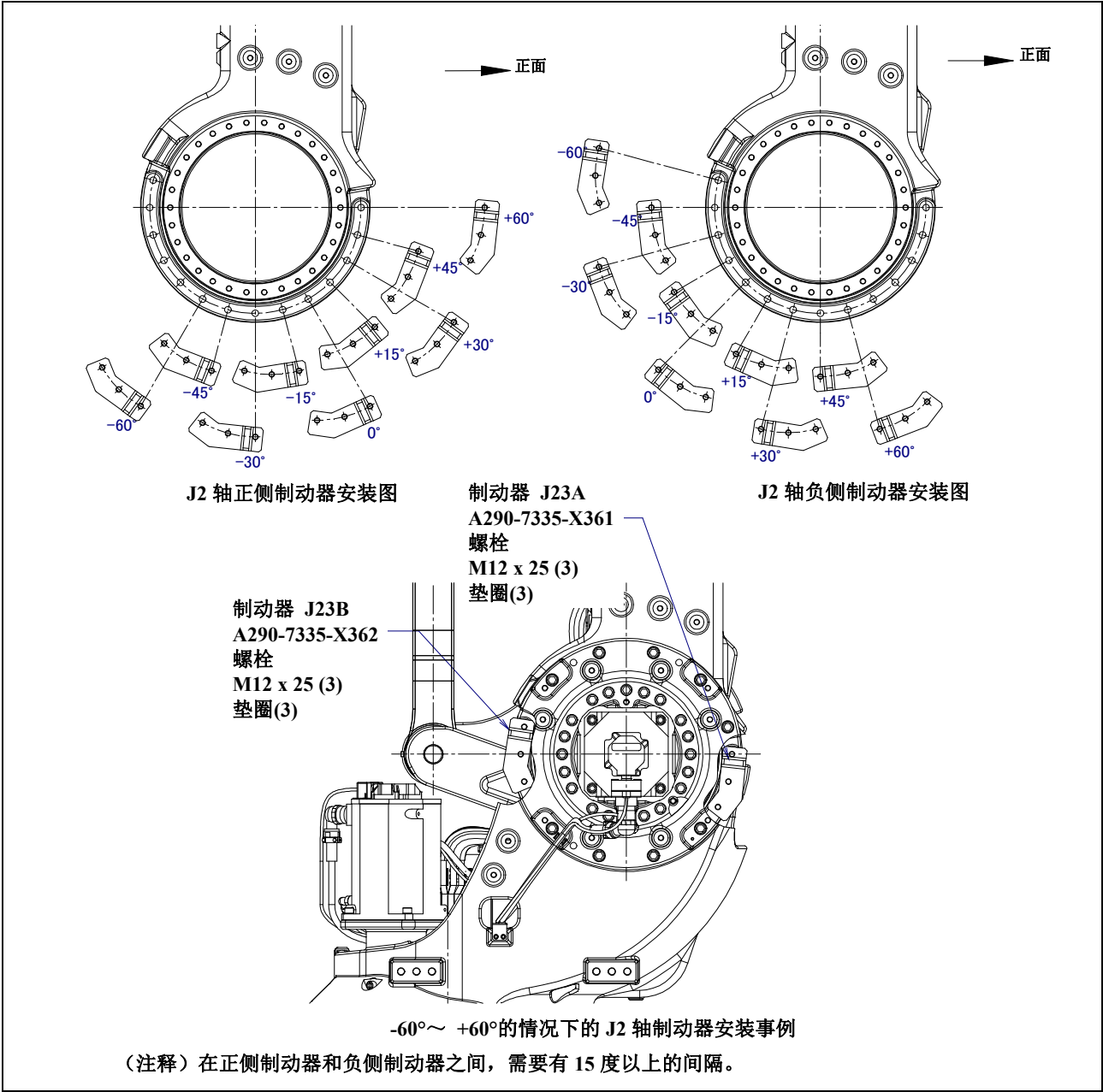
图 6.2.1 (d) J2 轴机械式可变制动器的安装
