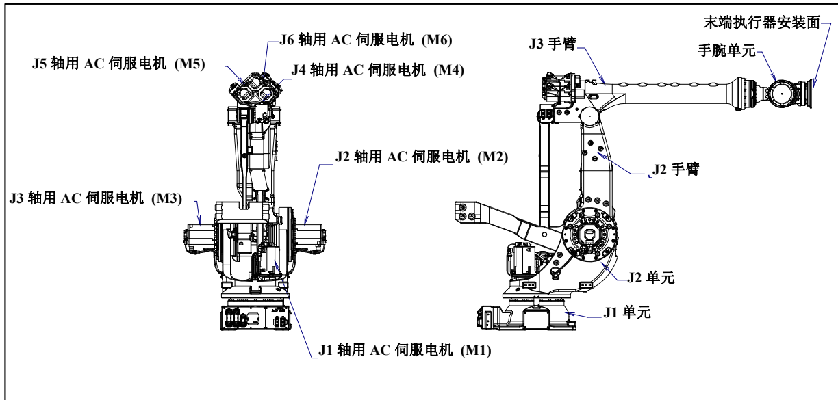
图 3.1 (c) 机构部的构成 (M-900iB/330L)
