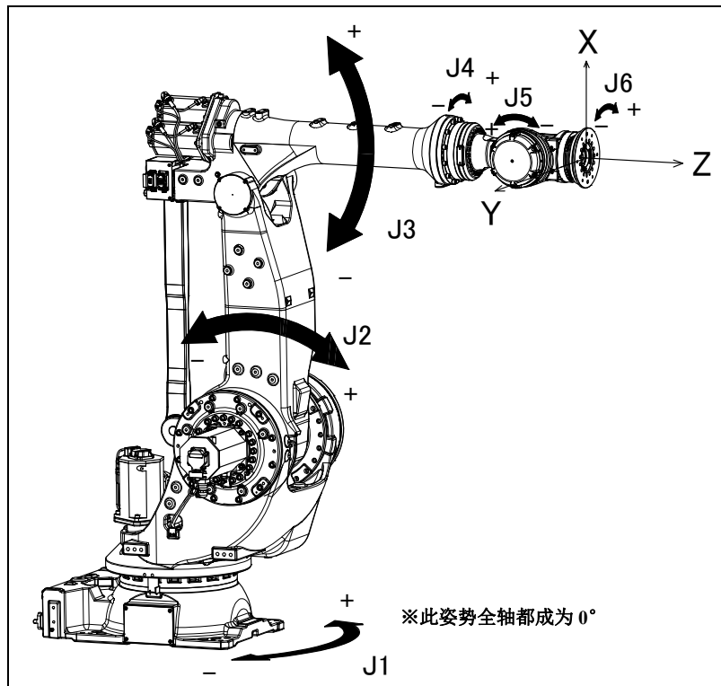
图 3.1 (d) 各轴坐标和机械接口坐标
