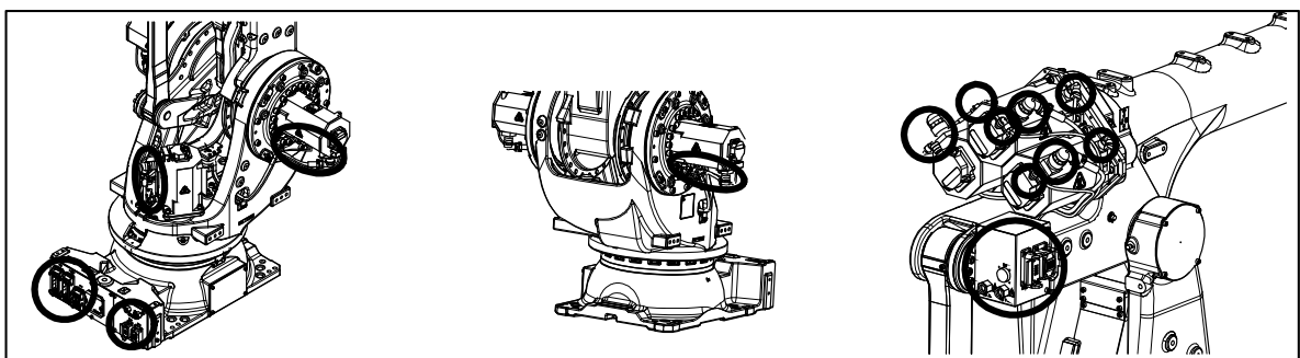
图 7.2.3 (d) 连接器的检修部位
