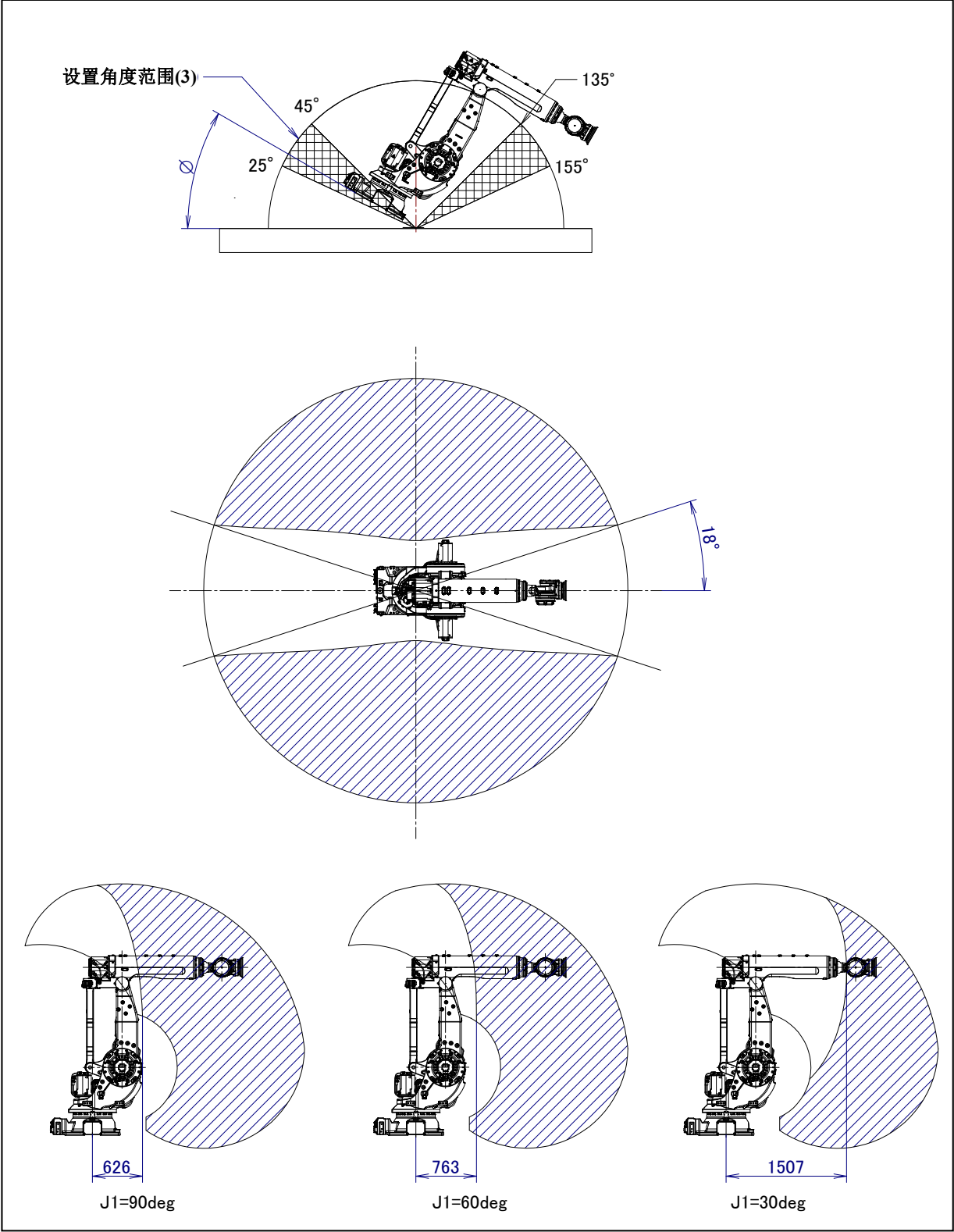
图 3.6 (k) 机器人设置角度范围(3)的动作范围 ( 25^\circ < \phi \leq 45^\circ, 135^\circ \leq \phi < 155^\circ ) (M-900iB/280)
