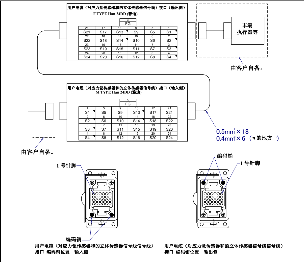
图 5.3 (h) 用户电缆（对应应力觉传感器和的立体传感器信号线）(ASi) 接口的插针排列和编码销的配置位置（可选项项）
