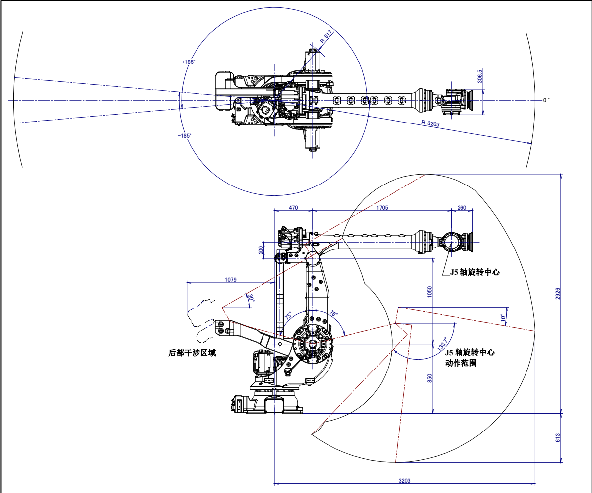
图 3.2 (d) 动作范围图 (M-900iB/330L)
