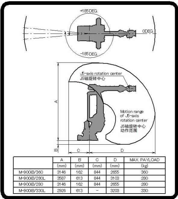
图 4 (e) 动作范围、可搬运重量标签
