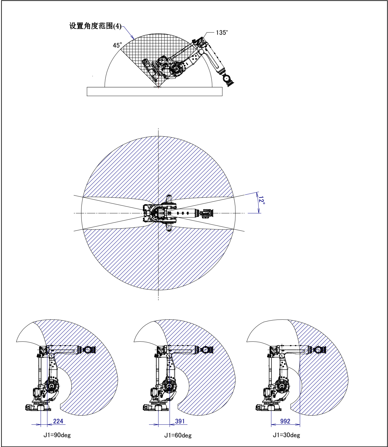
图 3.6 (I) 机器人设置角度范围(4)的动作范围 ( 45^{\circ} < \phi < 135^{\circ} ) (M-900iB/280)
