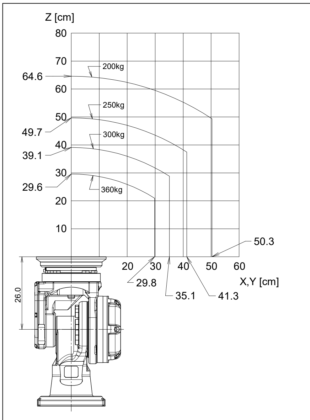
图 3.4 (a) 手腕部允许负载线图 (ISO 法兰盘) (M-900iB/360)
