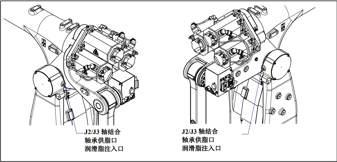
图 7.3.2 (a) J2/J3 轴结合轴承供脂部位
