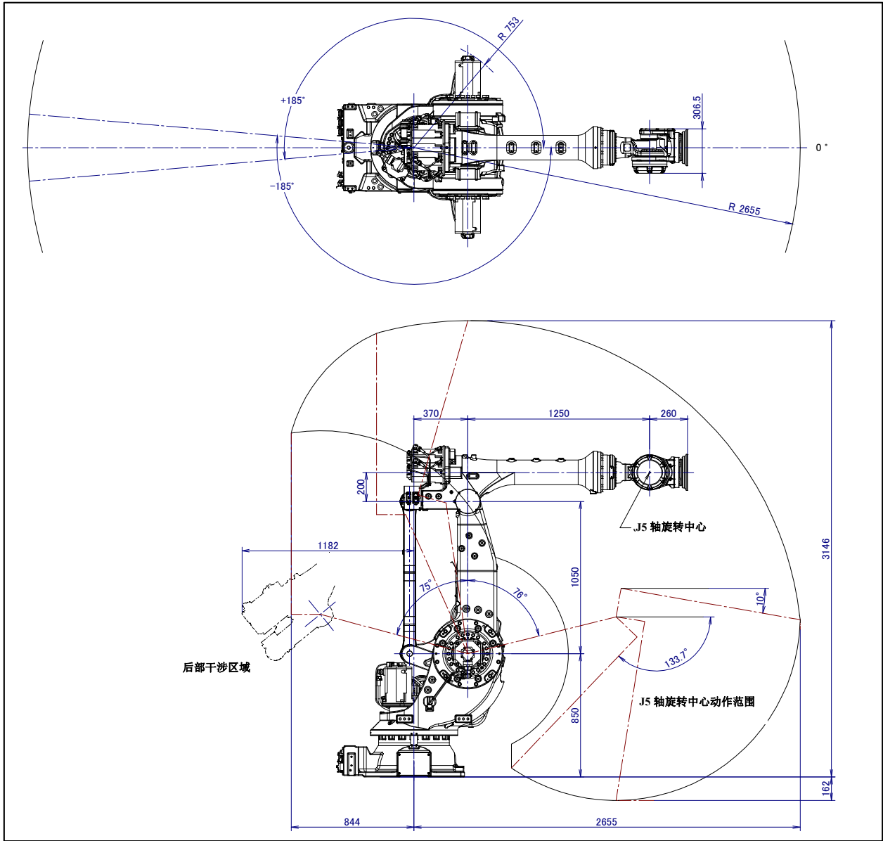
图 3.2 (a) 动作范围图 (M-900iB/360)
