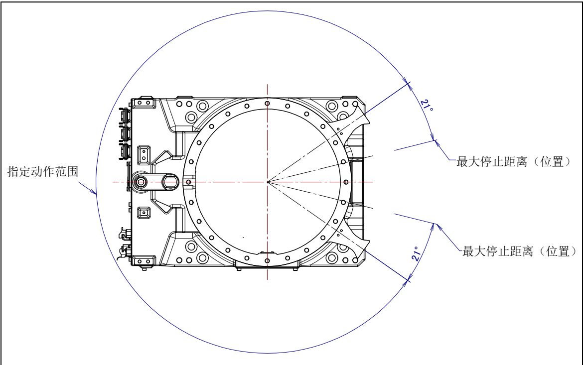
图 6.2.3 (a) J1 轴机械式可变制动器的最大停止距离（位置）
