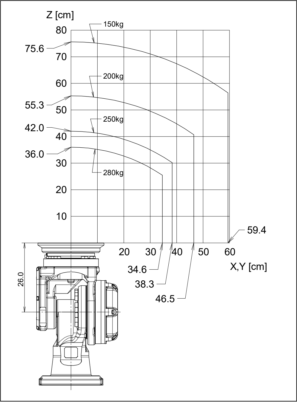
图 3.4 (c) 手腕部允许负载线图 (ISO 法兰盘) (M-900iB/280L)
