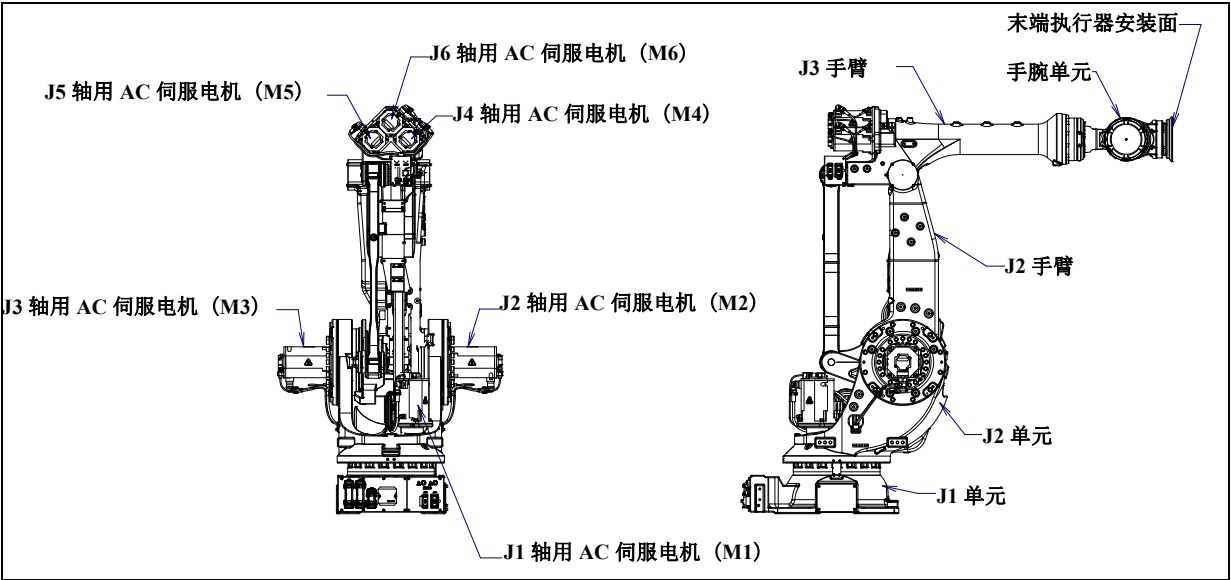
图 3.1 (a) 机构部的构成 (M-900iB/360/280L)
