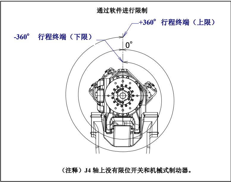
图 3.3 (g) J4 轴可动范围
