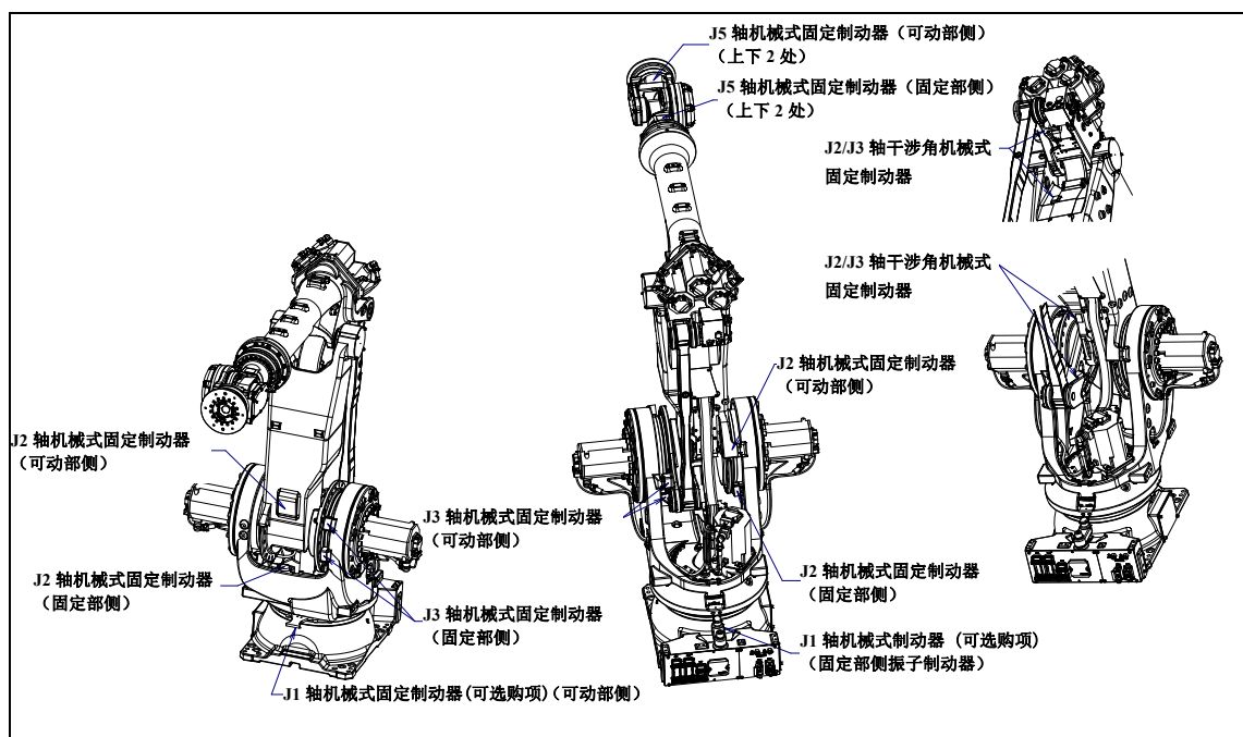
图 3.3 (a) 机械式制动器的位置
