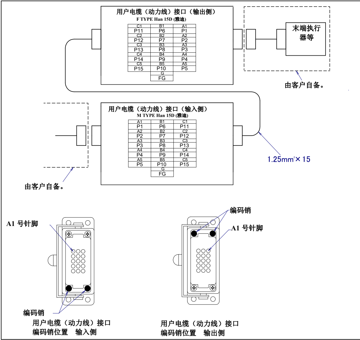
图 5.3 (i) 用户电缆（动力线）(AP)接口的插针排列和编码销配置位置（可选项项）
