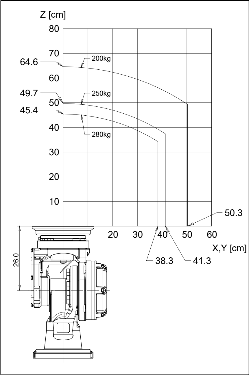
图 3.4 (e) 手腕部允许负载线图 (ISO 法兰盘) (M-900iB/280)
