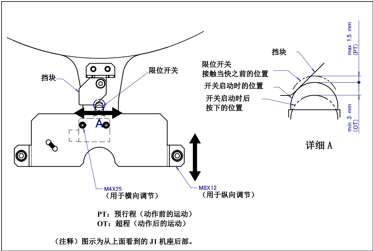
图 6.4 (a) J1 轴限位开关的调节（可选项项）
