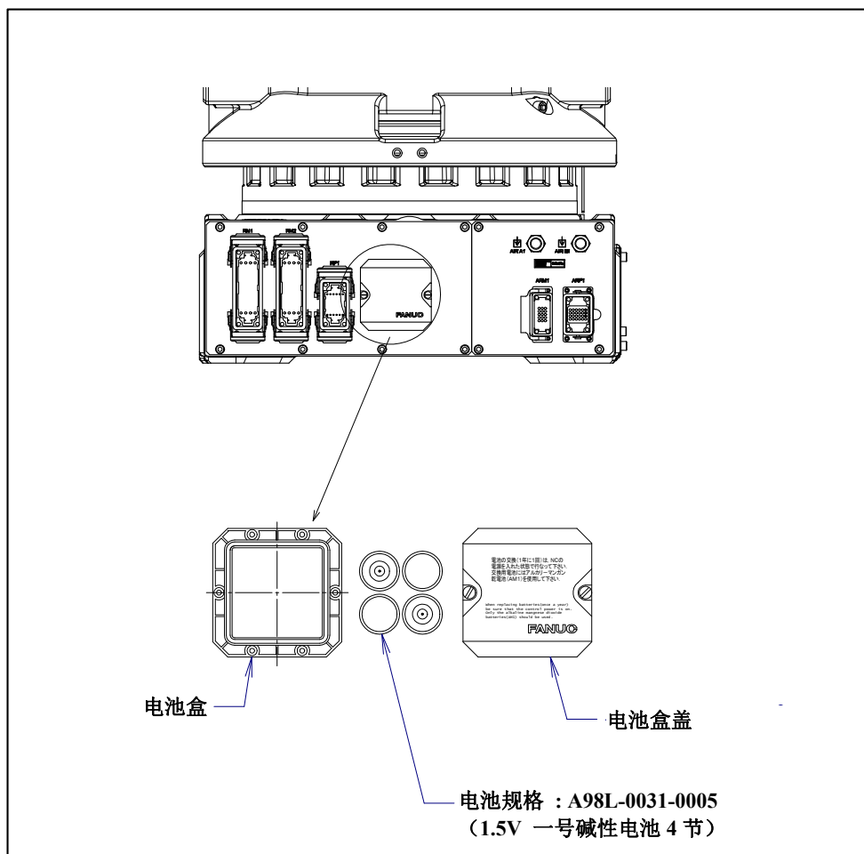
图 7.3.1 (a) 电池的更换
