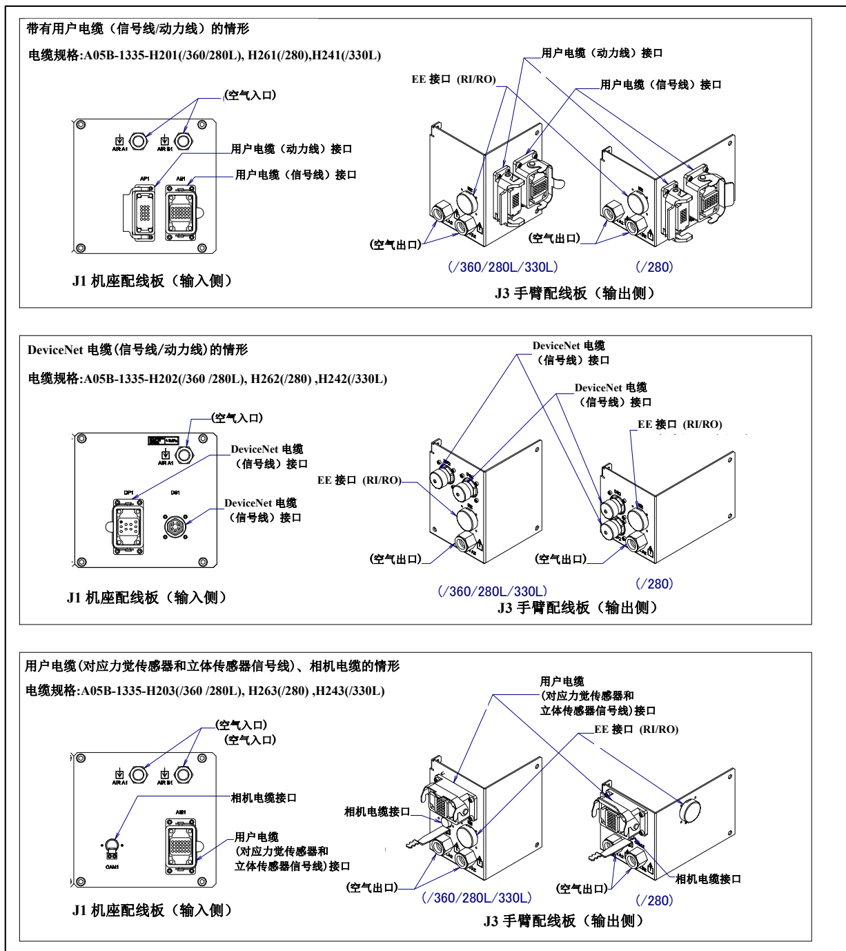
图 5.3 (b) 可选项电缆用接口 (1/2)
