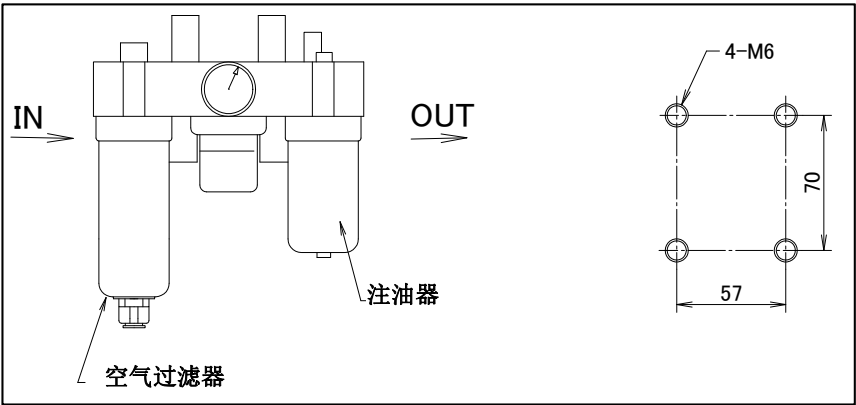
图 5.2 (b) 空气 3 点套件（可选购项）
