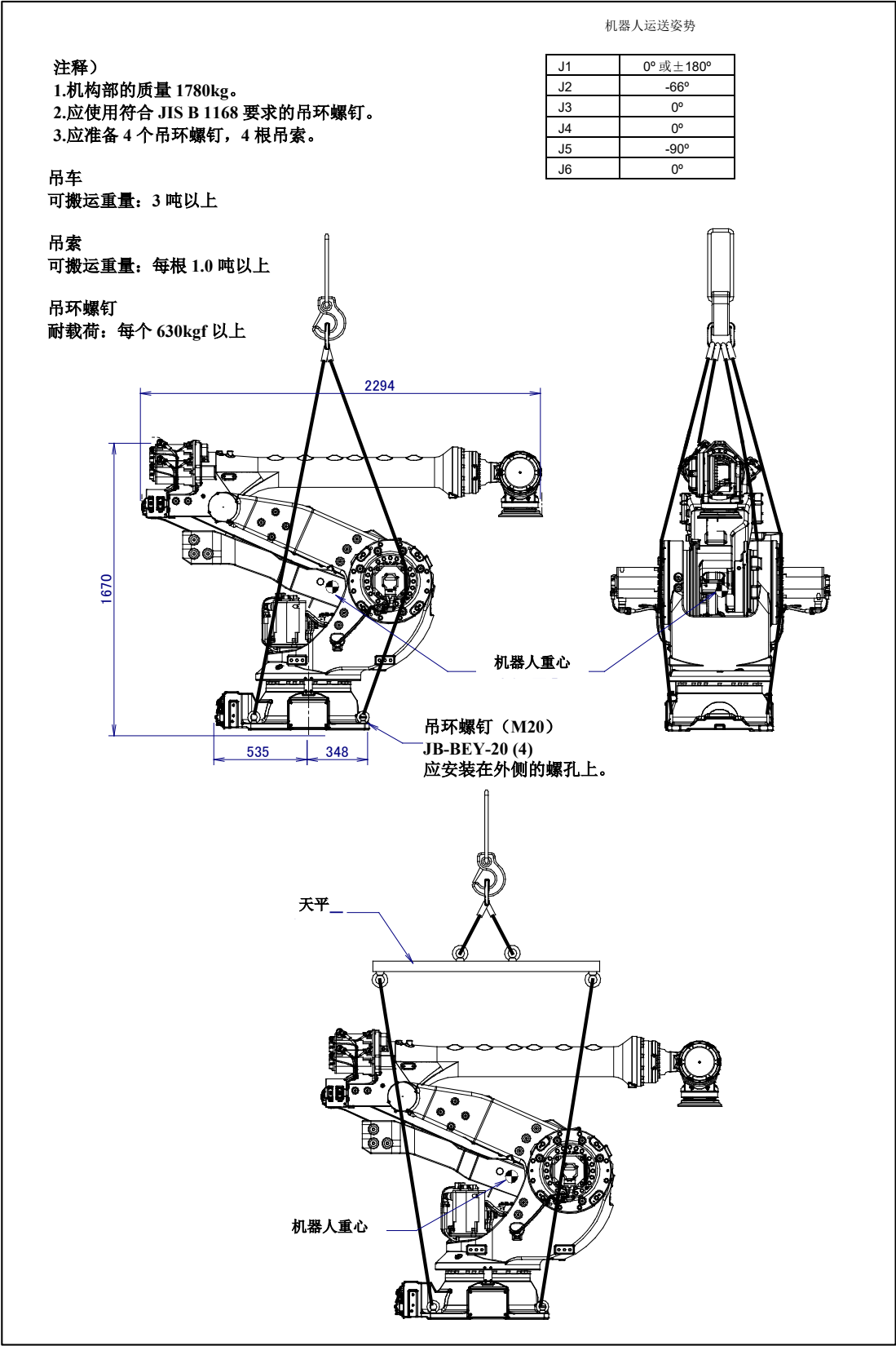
图 1.1 (e) 采用吊车搬运(M-900iB/330L)
