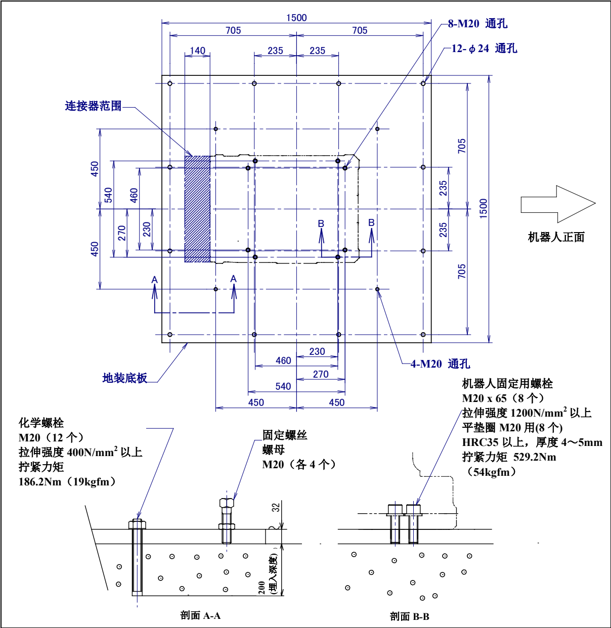
图 1.2.1 (c) 具体安装例Ⅲ
