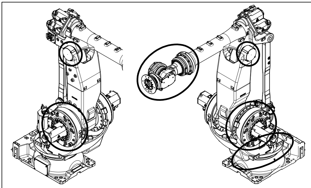
图 7.2.1 (a) 渗油的检查部位
