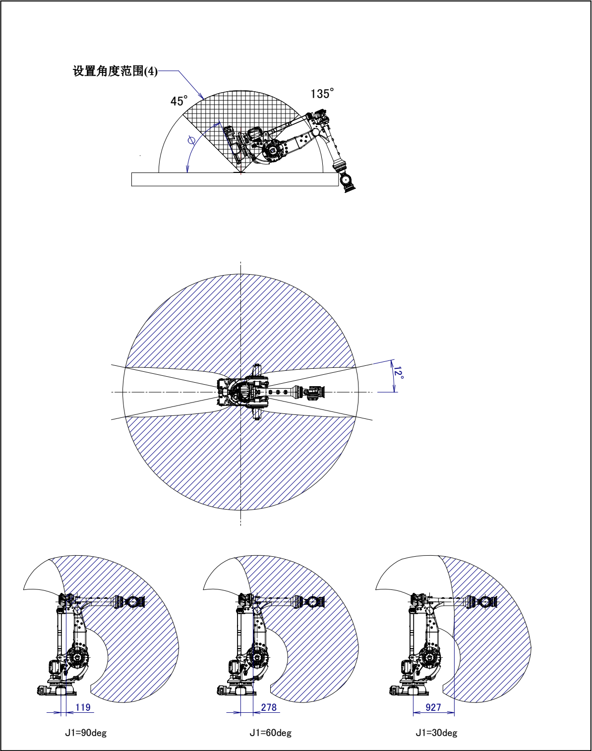
图 3.6 (d) 机器人设置角度范围(4)的动作范围 ( 45^\circ < \phi < 135^\circ ) (M-900iB/360)
