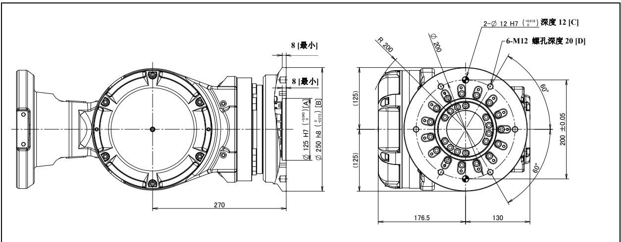
图 4.1 (b) 绝缘 ISO 法兰盘
