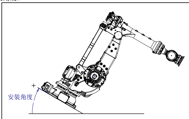
图 1.2.2 (a) 机器人的安装角度
