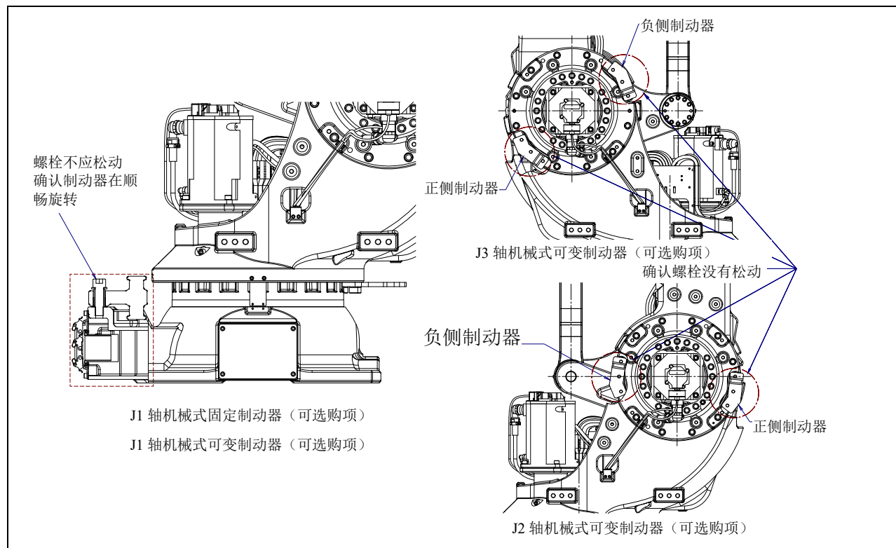
图 7.2.4 (a) 机械式固定制动器、机械式可变制动器的检修
