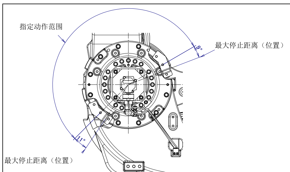
图 6.2.3 (c) J3 轴机械式可变制动器的最大停止距离 (位置)
