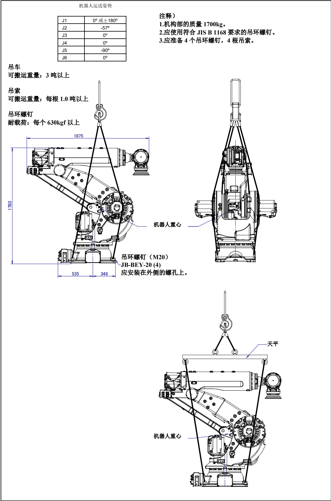
图 1.1 (d) 采用吊车搬运(M-900iB/280)
