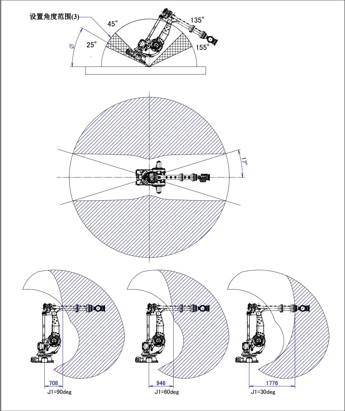
图 3.6 (g) 机器人设置角度范围(3)的动作范围 ( 25^\circ < \phi \leq 45^\circ , 135^\circ \leq \phi < 155^\circ ) (M-900iB/280L)
