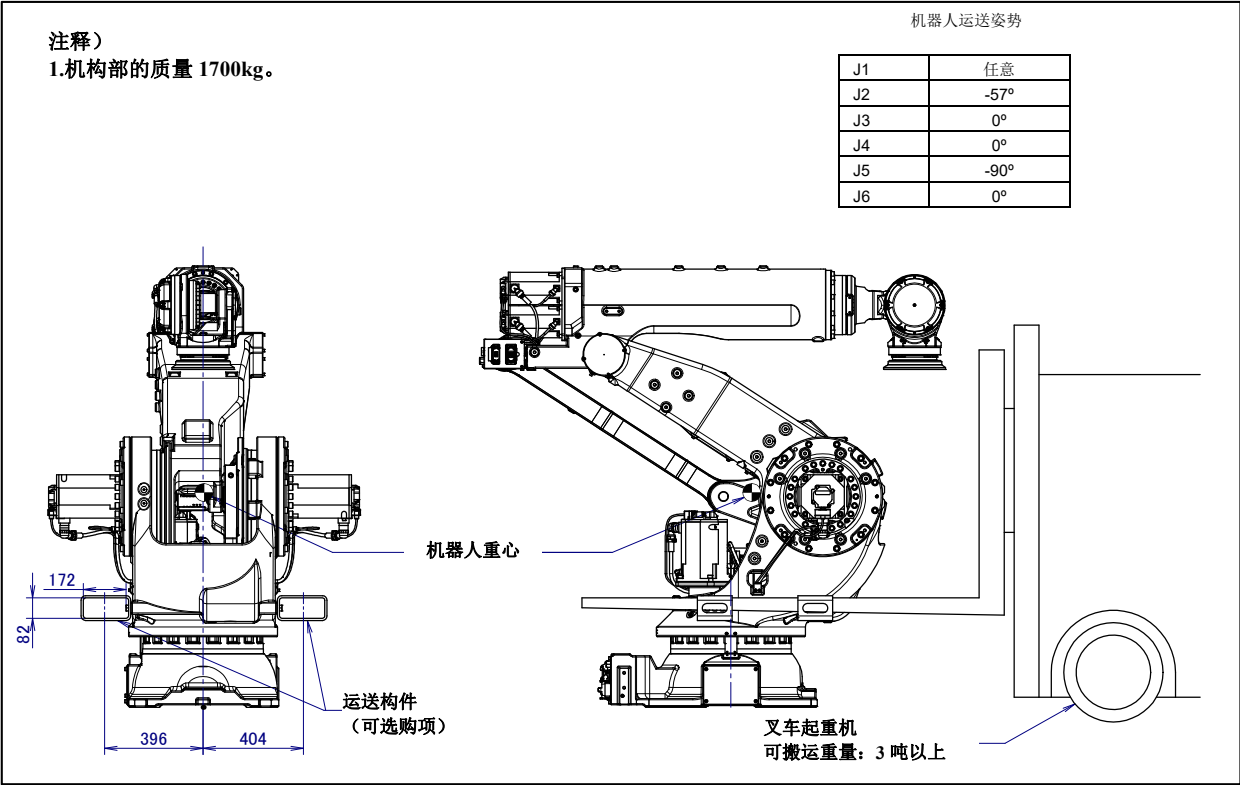
图 1.1 (h) 采用叉车起重机搬运(M-900iB/280)
