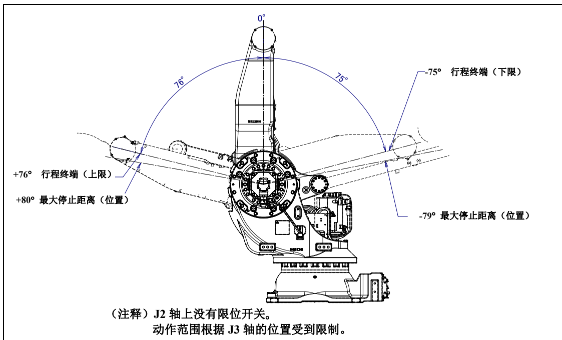
图 3.3 (d) J2 轴可动范围
