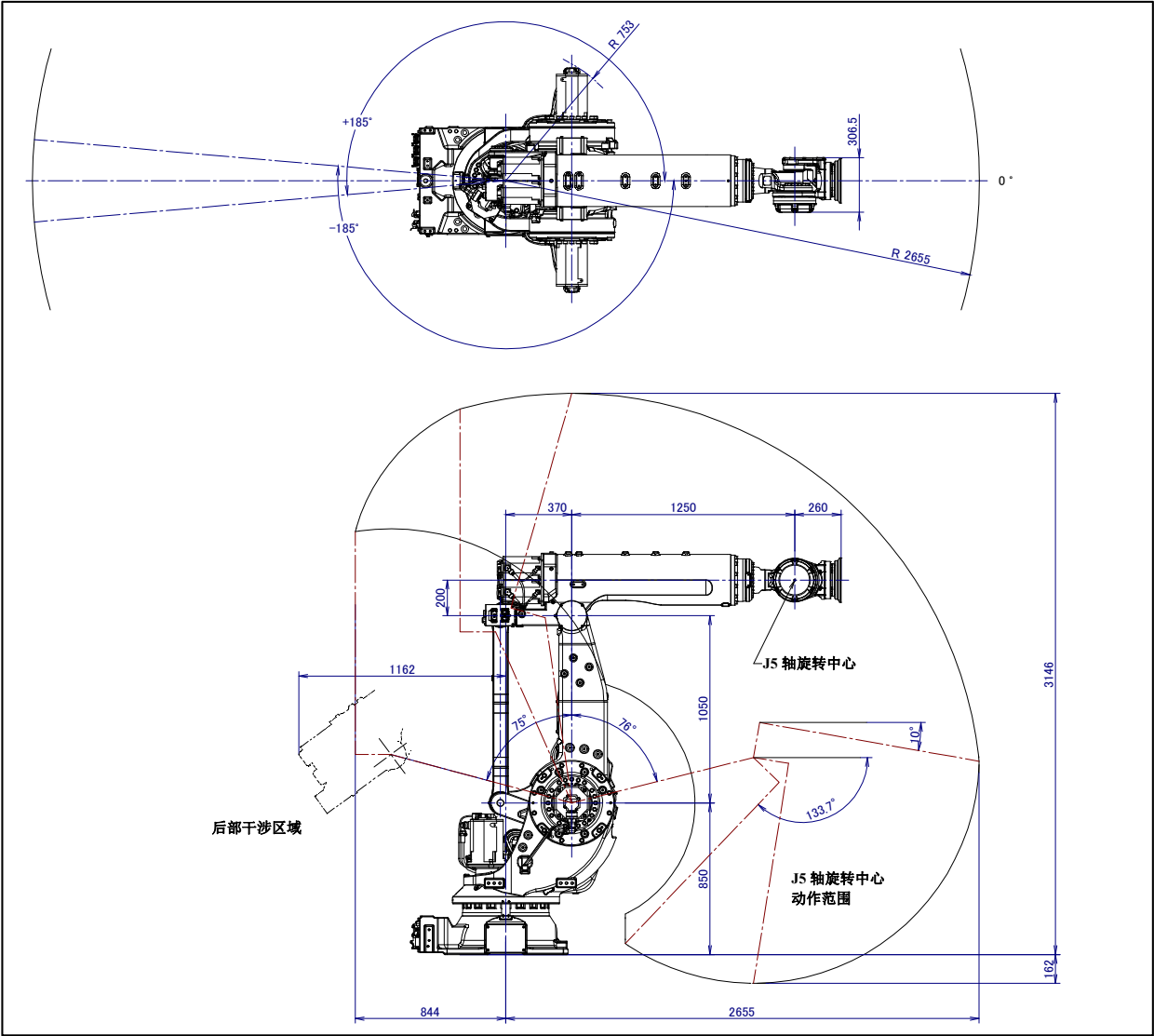
图 3.2 (c) 动作范围图 (M-900iB/280)
