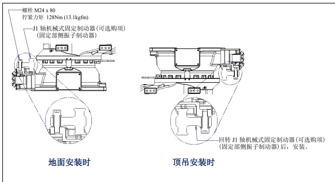
图 1.2.3 (a) J1 轴机械式固定制动器(可选项) (固定部侧振子制动器)
