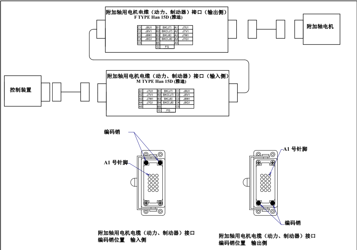
图 5.3 (m) 附加轴用电机电缆（动力线和制动器线）(ARM) 接口的插针排列和编码销配置位置（可选项项）
