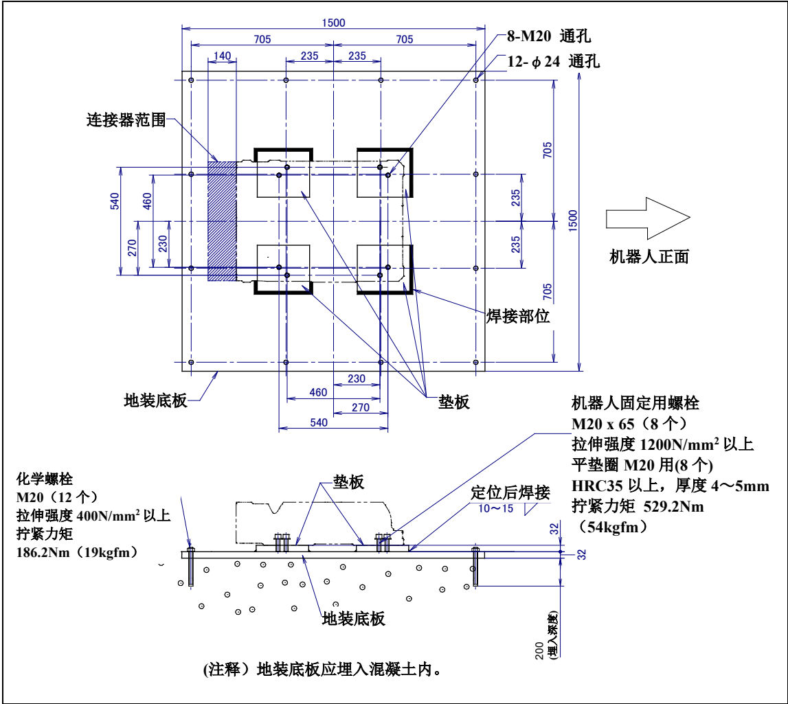
图 1.2.1 (a) 具体安装例 I
