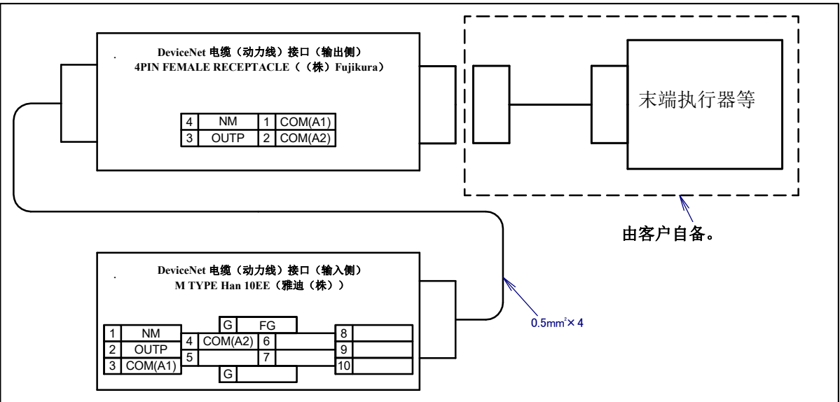
图 5.3 (k) DeviceNet 电缆（动力线）(DP)接口的插针排列（可选项）
