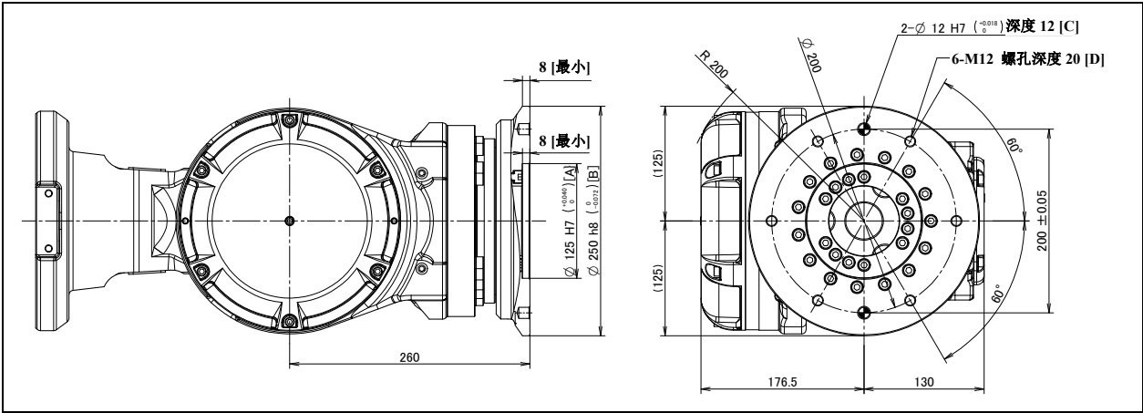
图 4.1 (a) ISO 法兰盘
