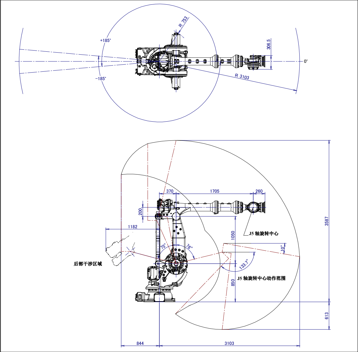
图 3.2 (b) 动作范围图 (M-900iB/280L)
