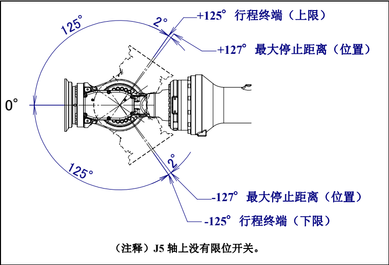
图 3.3 (h) J5 轴可动范围
