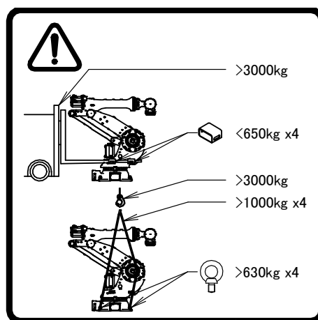
图 4 (d) 搬运标签
