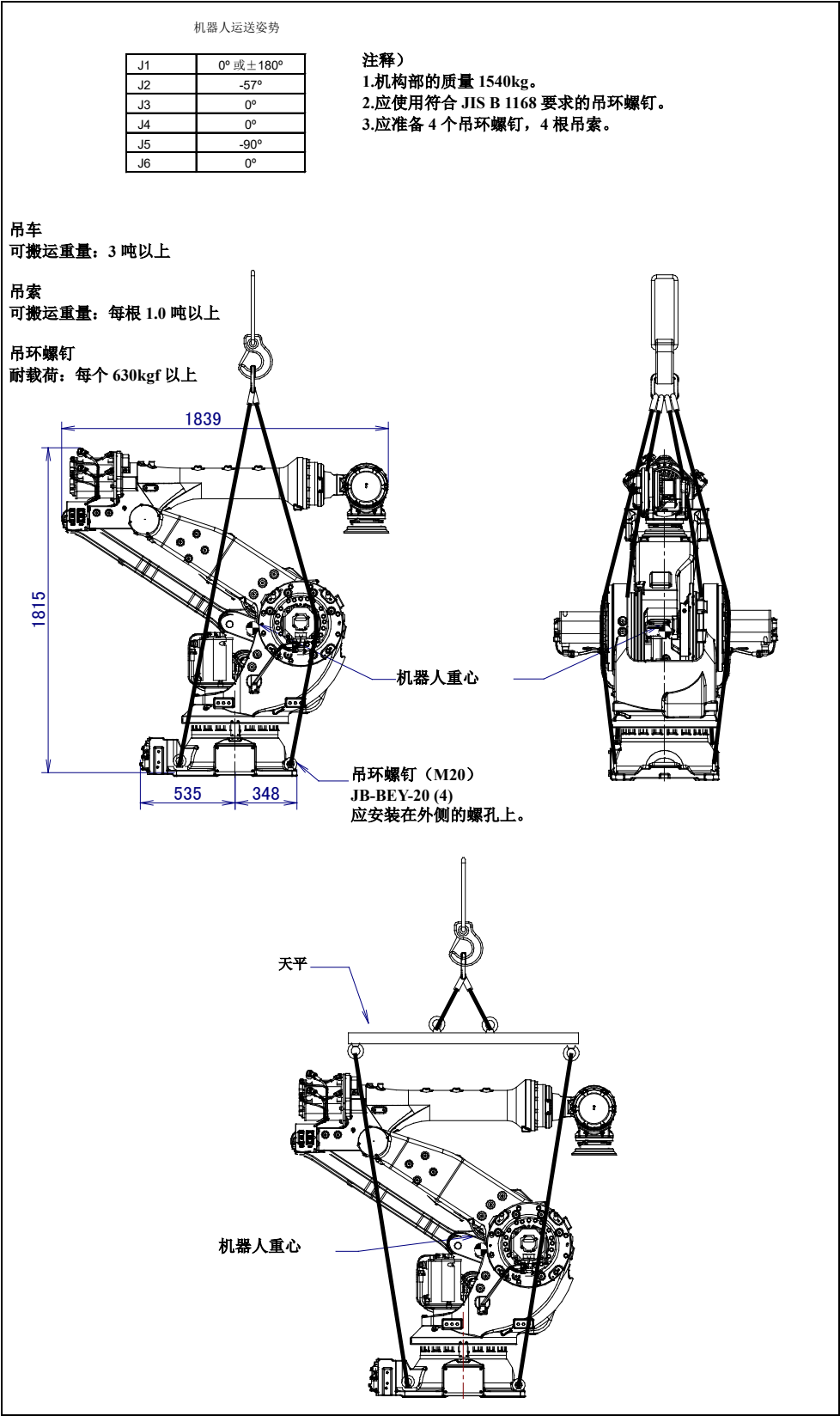
图 1.1 (b) 采用吊车搬运 (M-900iB/360)
