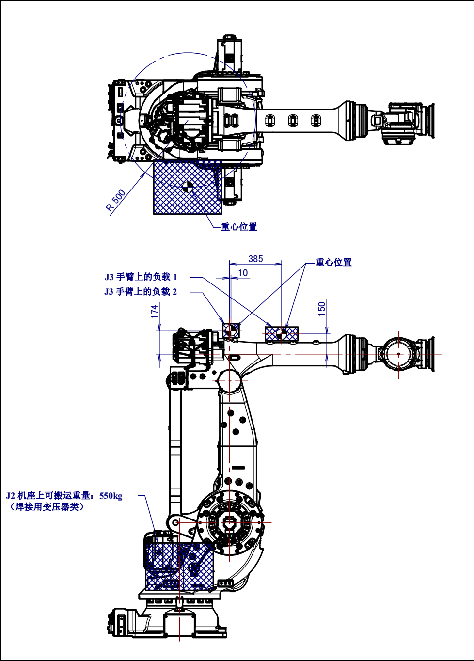
图 3.5 (a) J2 机座/J3 手臂上的负载条件 (M-900iB/360/280L/330L)
