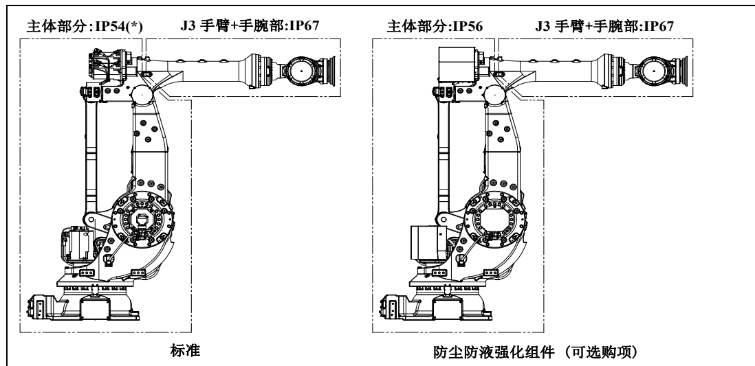
图 3.1 (e) M-900iB 的防尘防液性能
