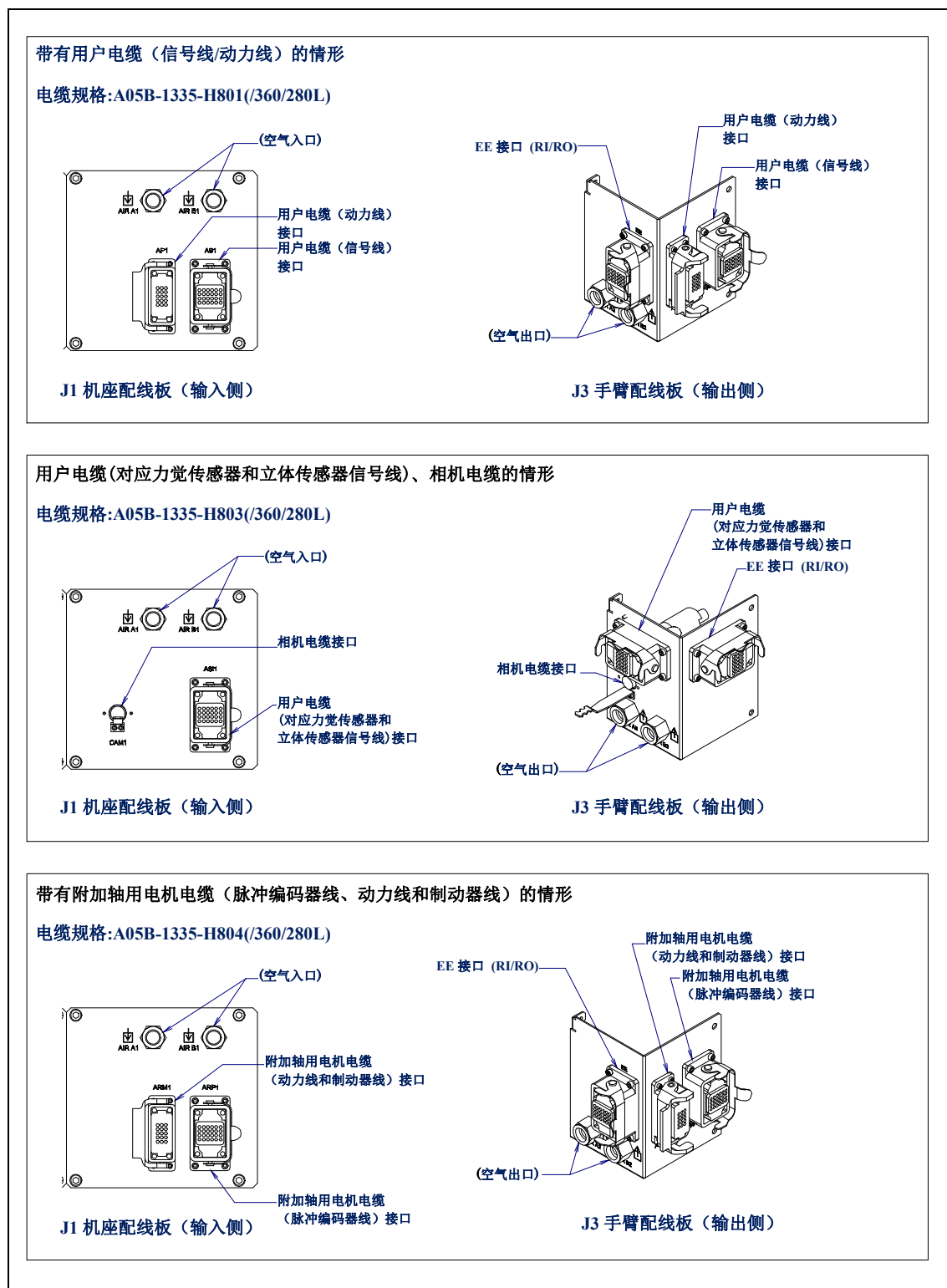
图 5.3 (d) 可选项电缆用接口 （选择防尘防液强化组件时）
