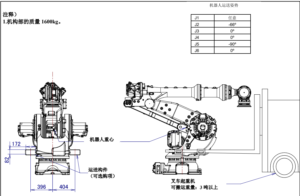
图 1.1 (g) 采用叉车起重机搬运(M-900iB/280L)
