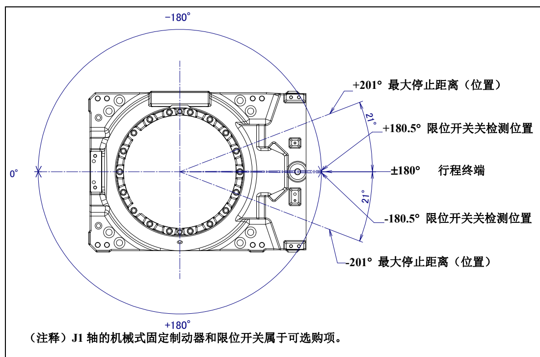
图 3.3 (c) J1 轴可动范围（指定机械式制动器时）
