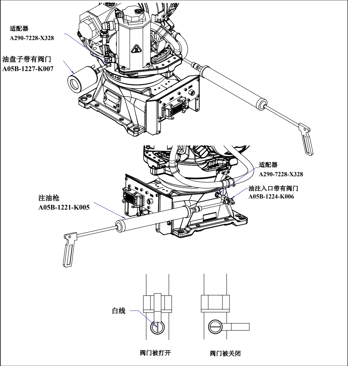
图 7.3.2.3 (b) 用注油枪供油（J1 轴减速机的供油）（地面安装的例）
