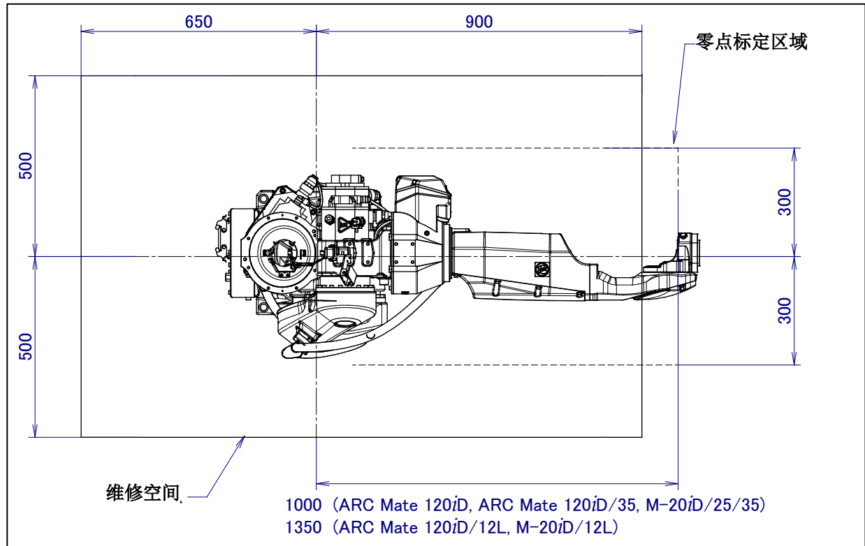
图 1.3 (a) 维修空间的布局图
