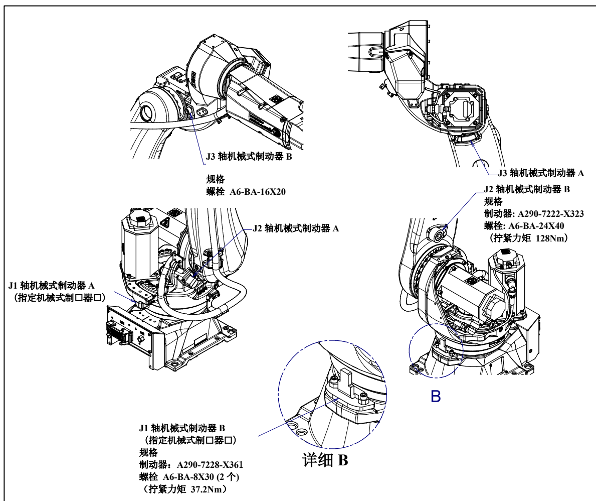
图 7.2.4 (a) 机械式固定制动器、机械式可变制动器的检修
