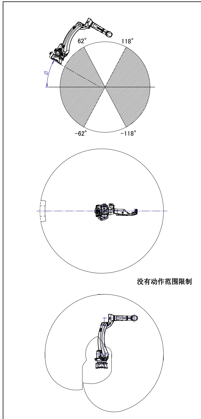
图 3.6 (b) 设置范围 (1) 动作范围图(ARC Mate 120iD, M-20iD/25) (-180^\circ \leq \phi \leq 118^\circ, -62^\circ \leq \phi \leq 62^\circ, 118^\circ \leq \phi \leq 180^\circ)
