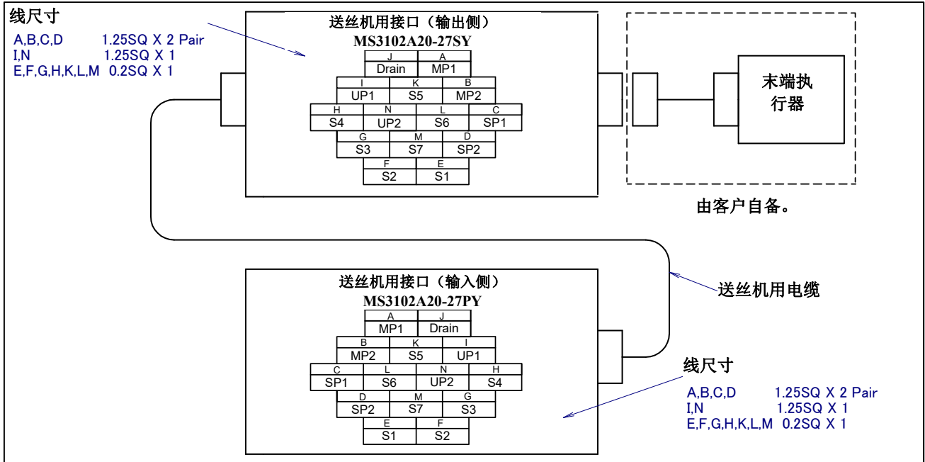
图 5.3 (j) 林肯电气送丝机用接口的插脚排列 (可选项) (指定 A05B-1228-H205#25L, H205#HLL 时)
