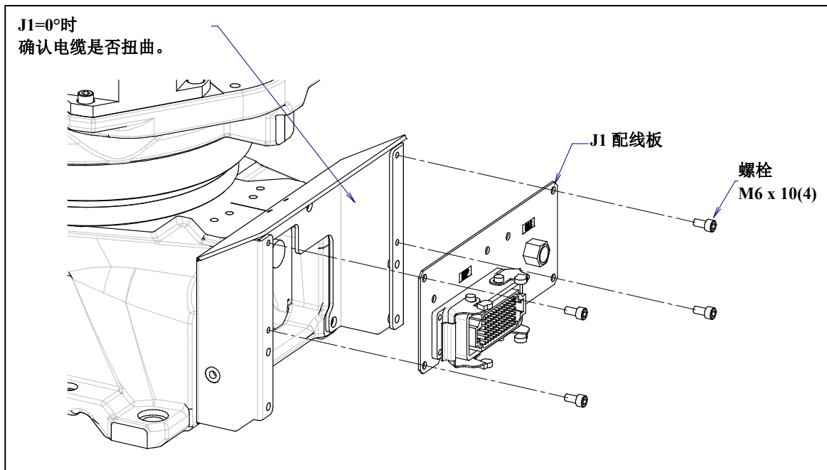
图 8.1 (a) 确认电缆的状态 (J1 轴)
