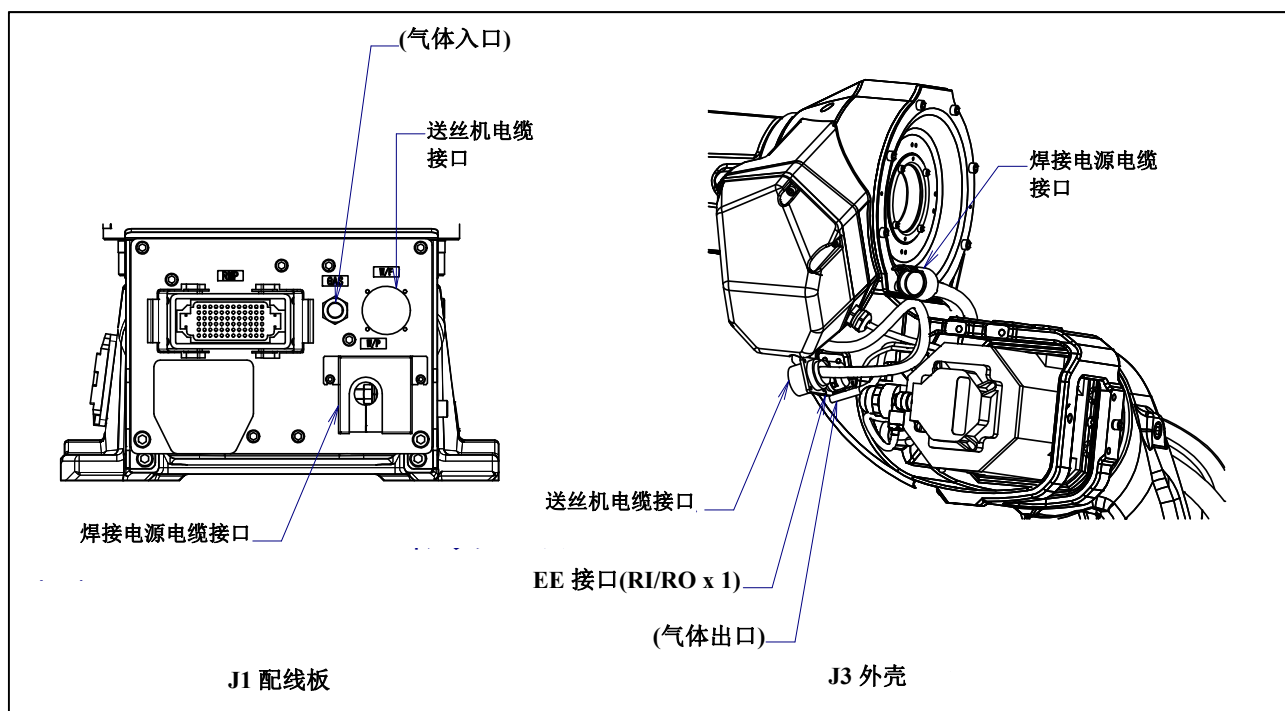
图 5.3 (c) 可选项电缆用接口 (指定 A05B-1228-H205#□□时)
