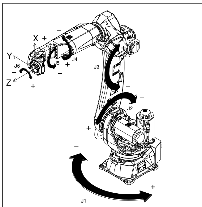
图 3.1 (b) 各轴坐标和机械接口坐标
