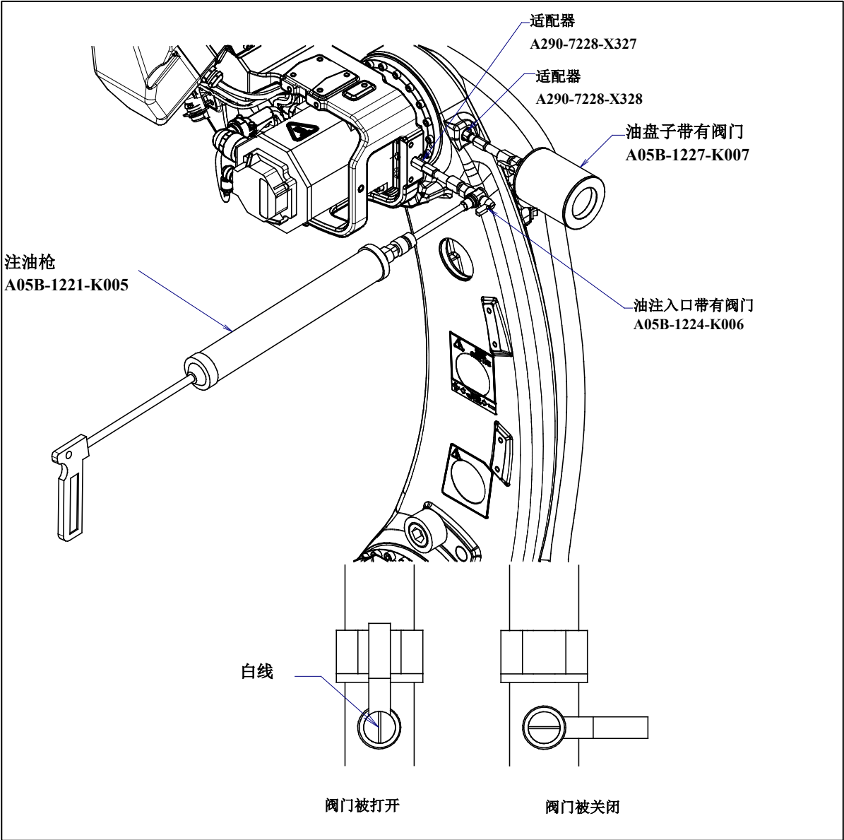
图 7.3.2.3 (d) 用注油枪供油（J3 轴减速机的供油）（地面安装的例）
