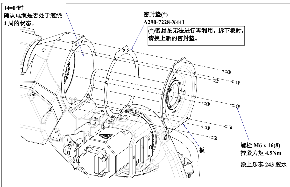
图 8.1 (b) 确认电缆的状态 (J4 轴)
