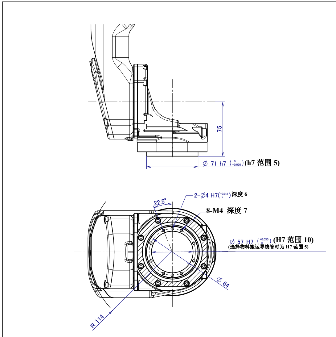
图 4.1 (c) 末端执行器安装面(ARC Mate 120iD/12L, M-20iD/12L)
