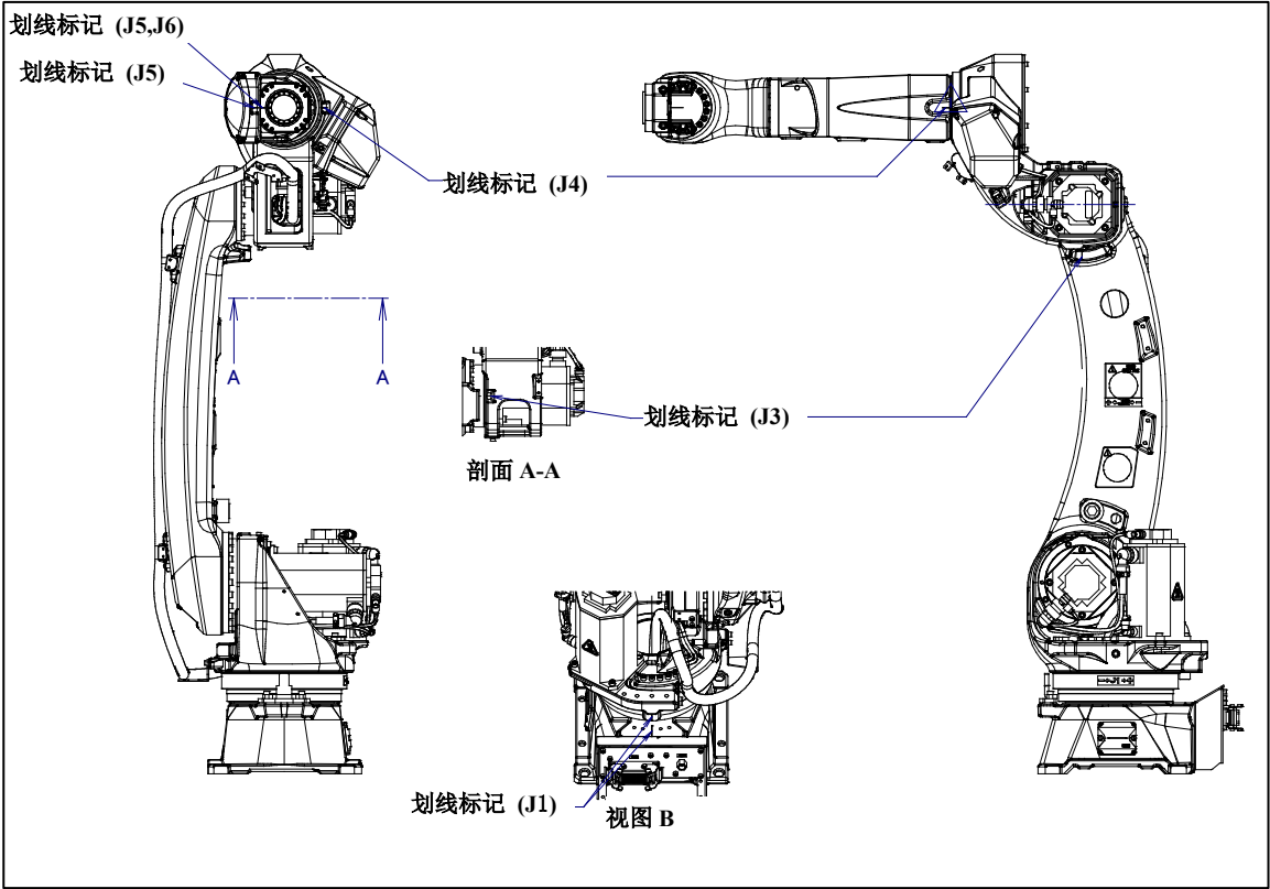
图 8.3 (a) 各轴的对合标记位置
