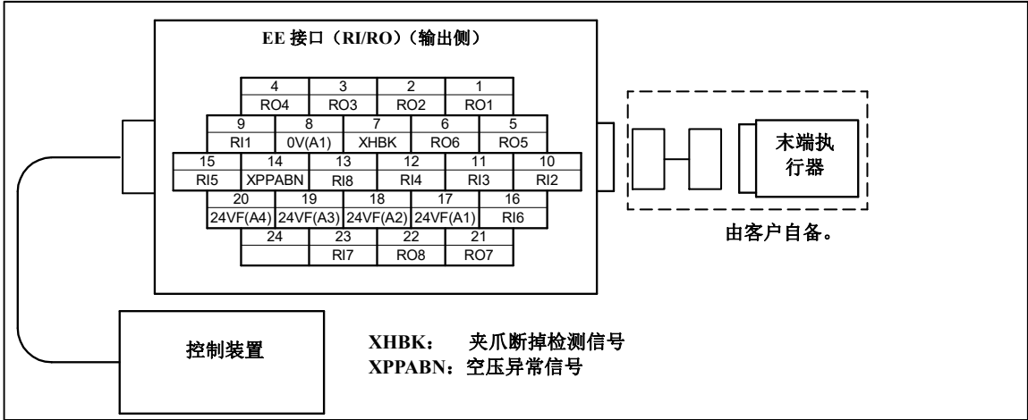
图 5.3 (i) EE 接口(RI/RO)的插脚排列 RI/RO 各 8 点 (可选项) (指定 A05B-1228- H223#□□, H224#□□时)
