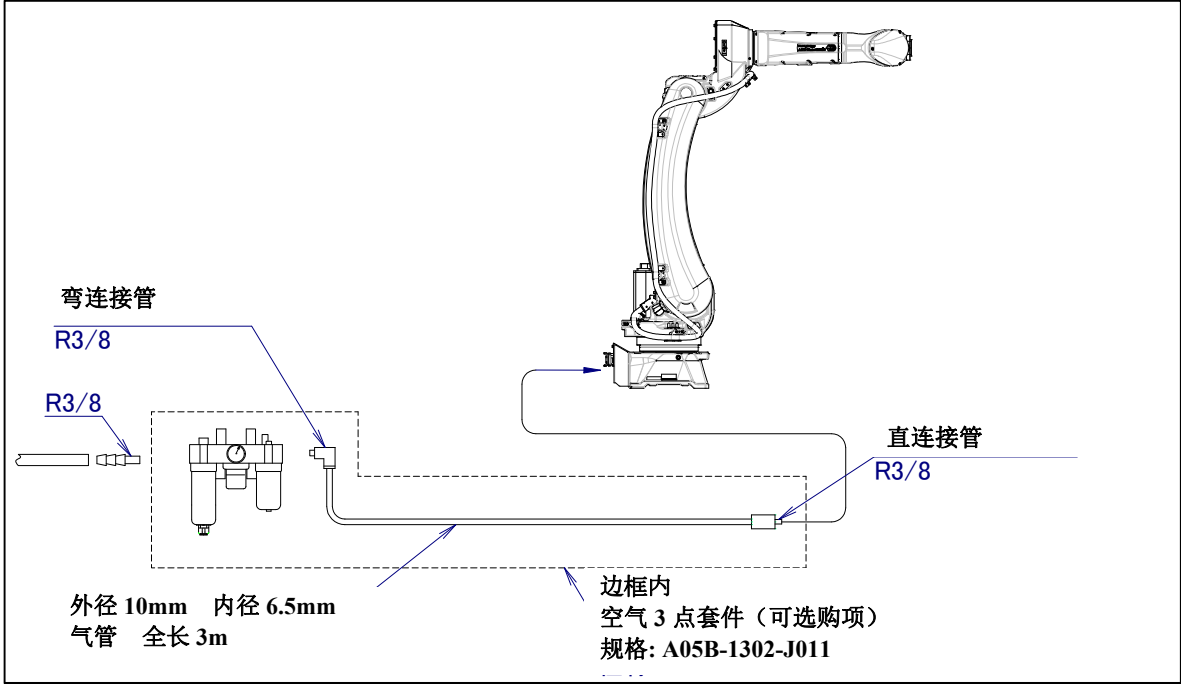
图 5.2 (a) 空气配管（可选项）
