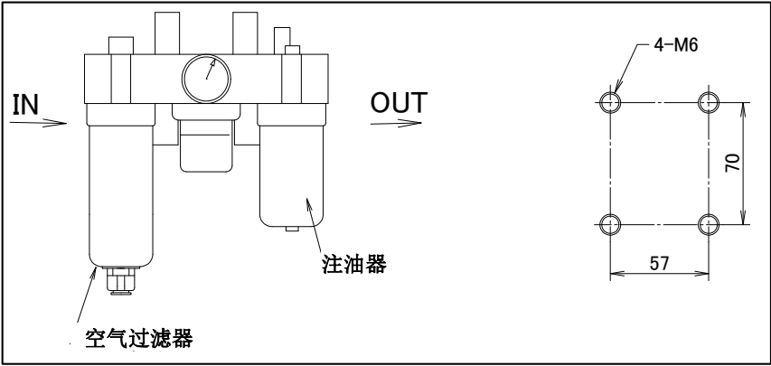
图 5.2 (b) 空气 3 点套件（可选项）
