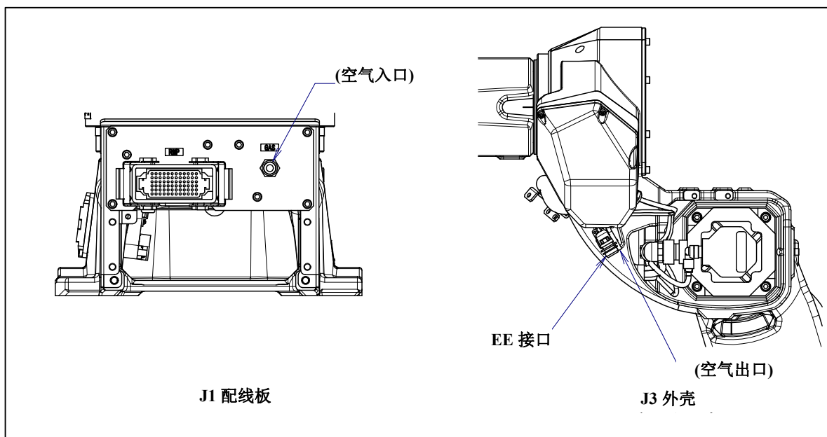
图 5.3 (b) 可选项电缆用接口 (指定 A05B-1228-H201#25, H221#25 时)
