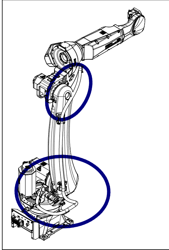
图 7.2.3 (a) 机构部内电缆的检修部位
