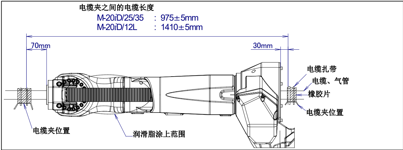
图 10.1 (a) 电缆夹之间的距离
