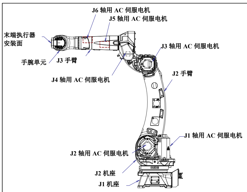
图 3.1 (a) 机构部的构成
