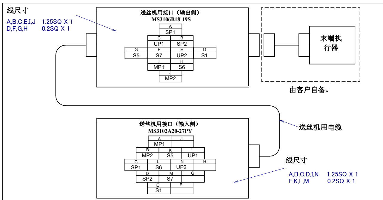
图 5.3 (l) FANUC 丝机(W/F)用接口的插针排列 (可选项) (A05B-1228- H205#25H, H205#HLH 指定時)
