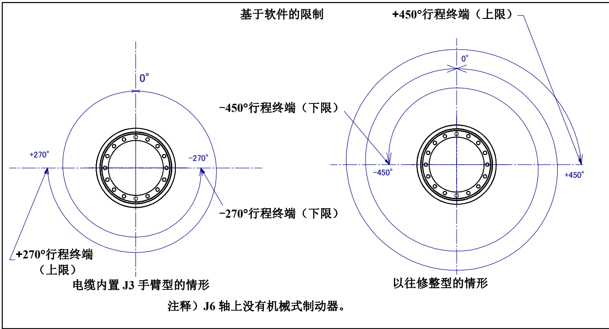
图 3.3 (i) J6 轴可动范围
