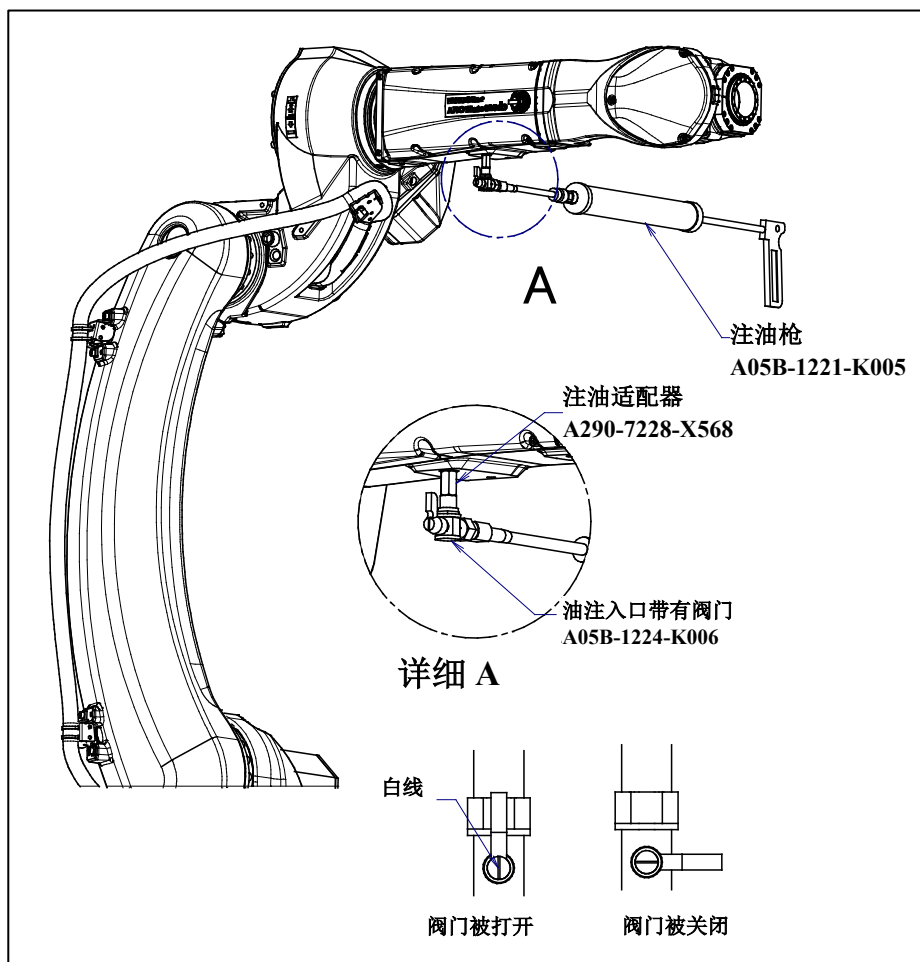
图 7.3.2.6 (b) 用注油枪供油
