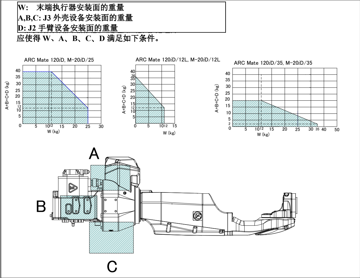
图 4.2 (a) 负载条件
