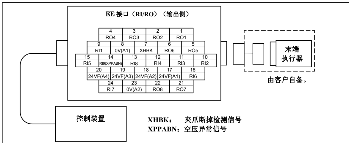
图 5.3 (h) EE 接口(RI/RO)的插针排列 RI/RO 各 8 点 (可选项) (指定 A05B-1228- H221#□□, H222#□□时)
