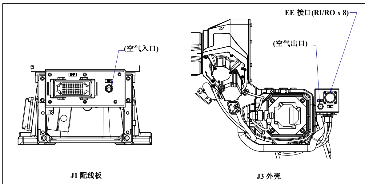
图 5.3 (e) 可选项电缆用接口 (指定 A05B-1228-H223#□□时)
