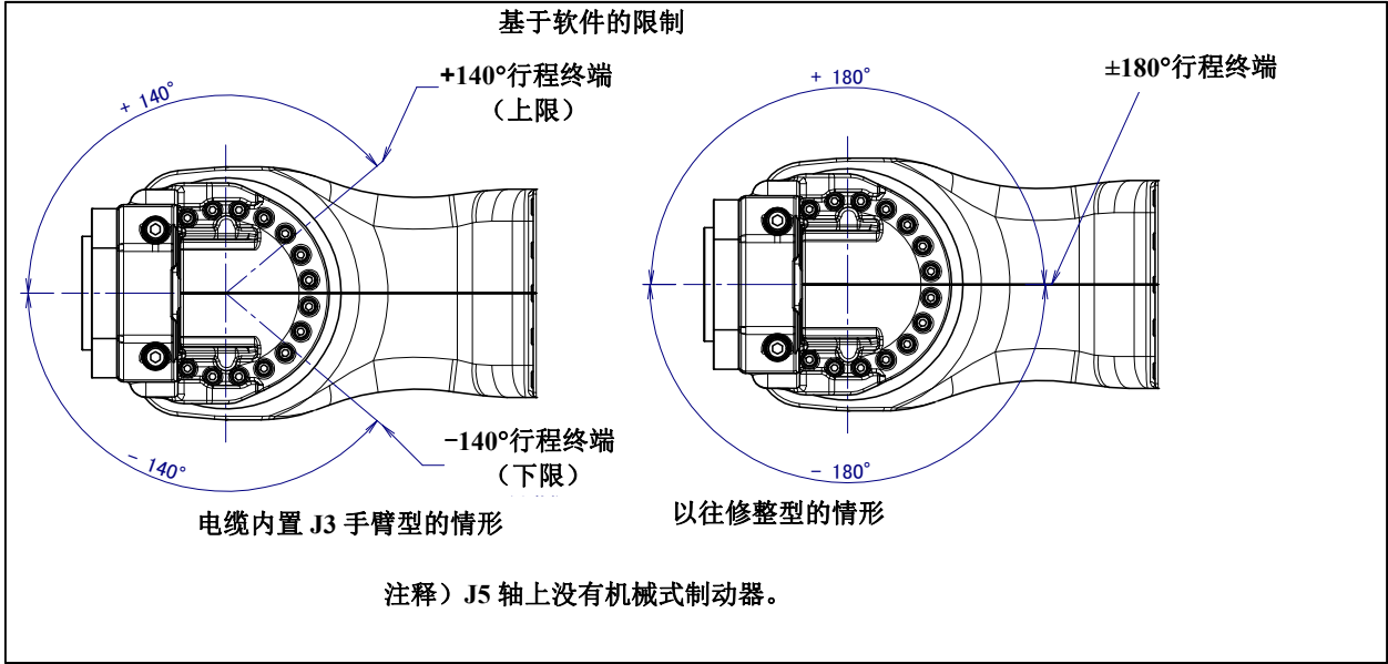
图 3.3 (h) J5 轴可动范围
