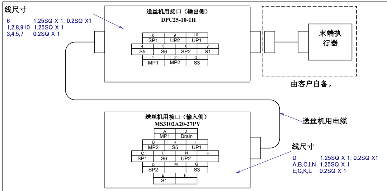
图 5.3 (k) DAIHEN 送丝机(W/F)用接口的插针排列 (可选项) (A05B-1228- H205#25D, H205#HLD 指定時)
