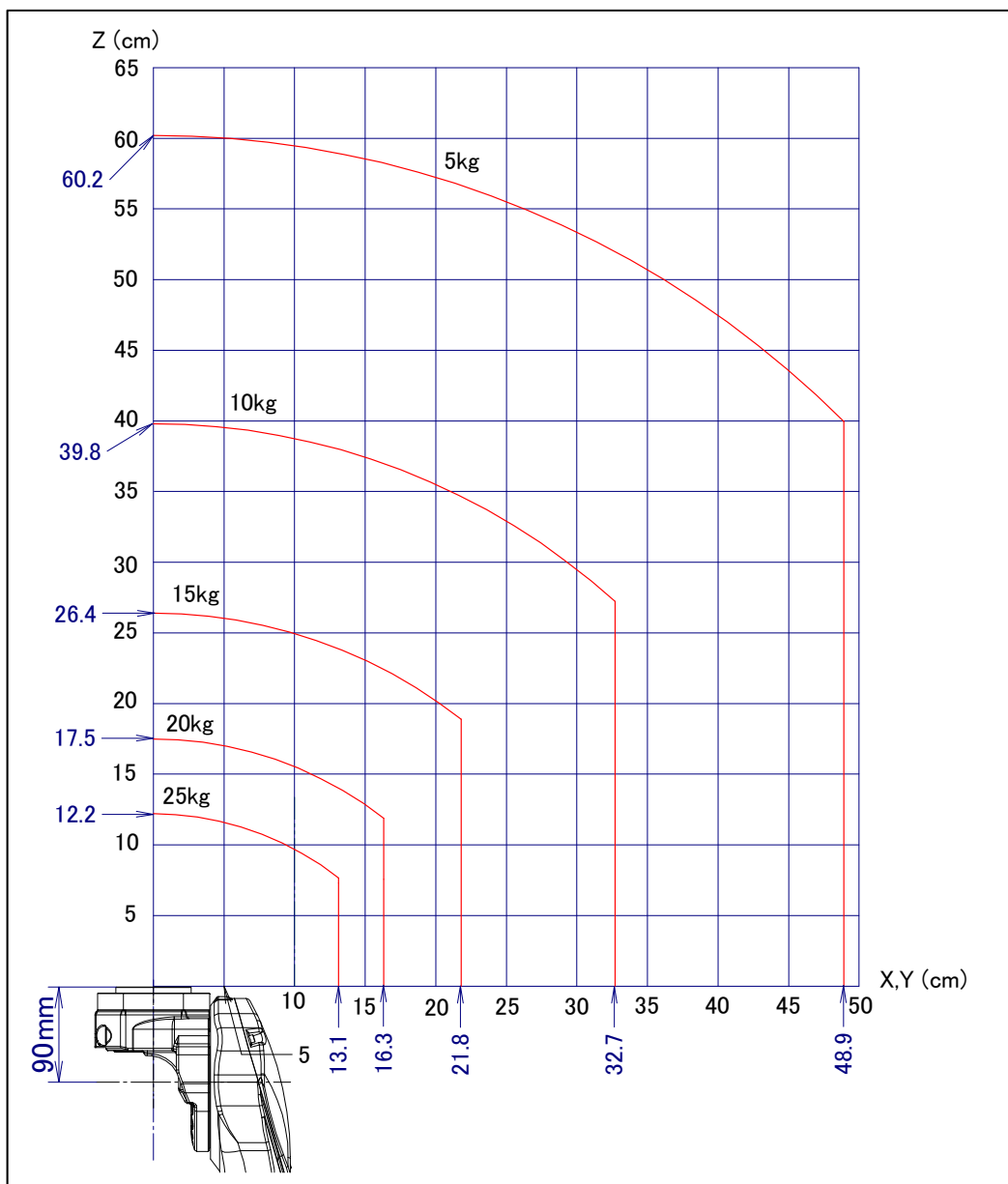
图 3.5 (a) 手腕部允许负载线图 (ARC Mate 120iD, M-20iD/25)
