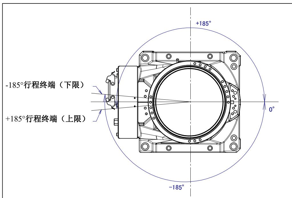
图 3.3 (c) J1 轴可动范围（未选择机械式制动器时）
