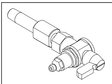
图 7.3.2.7 (c) 油注入口带有阀门 (A05B-1224-K006)
