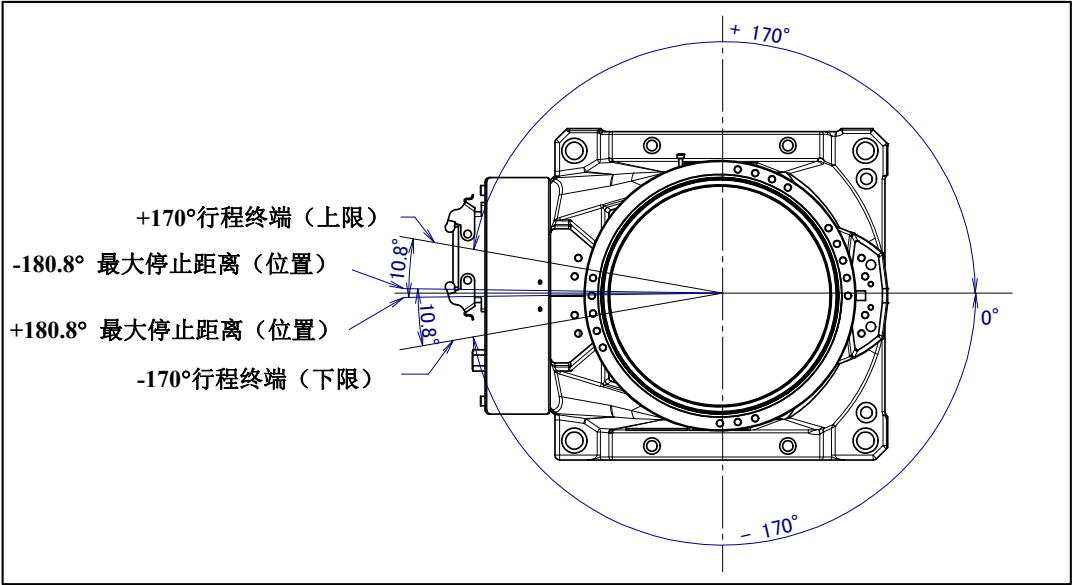
图 3.3 (d) J1 轴可动范围 (选择机械式制动器时)
