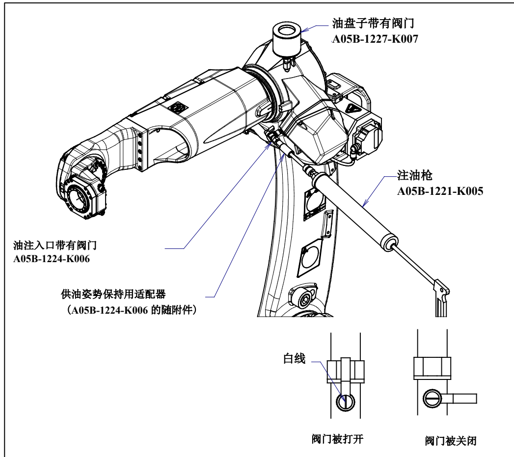
图 7.3.2.5 (b) 用注油枪供油 (J4 轴齿轮箱的供油)
