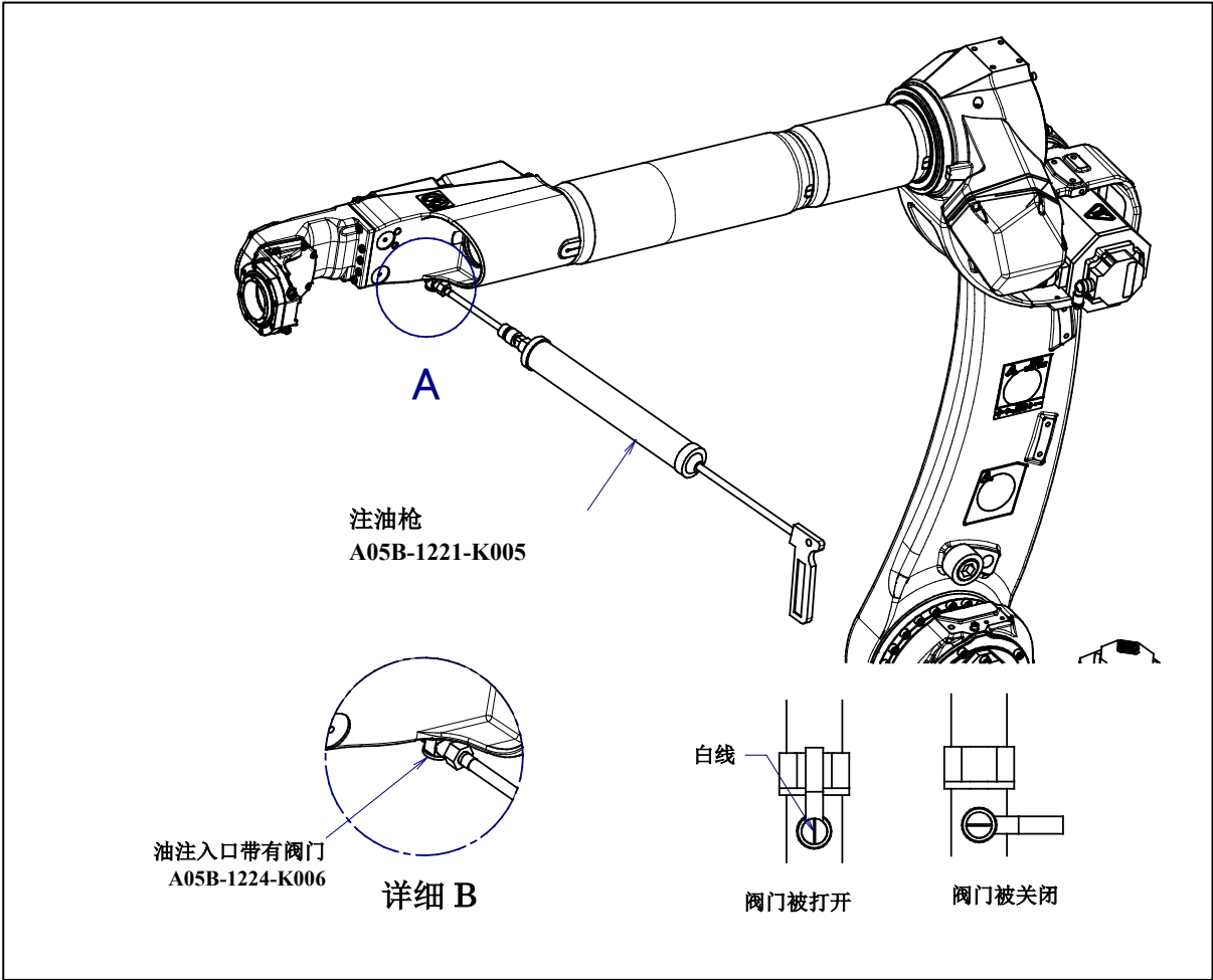
图 7.3.2.7 (b) 用注油枪供油
