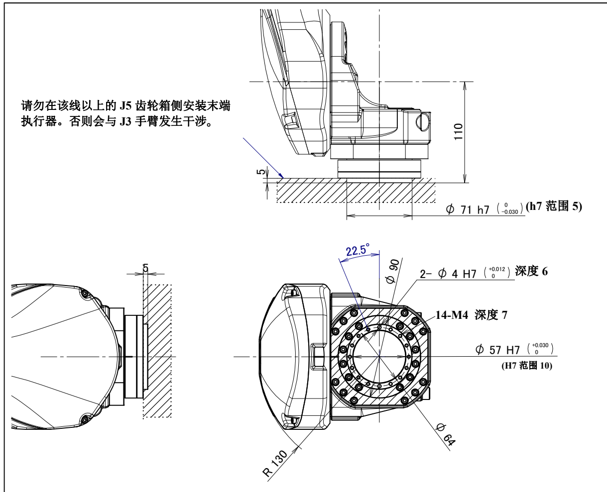
图 4.1 (b) 末端执行器安装面(M-20iD/25 食品润滑油规格)
