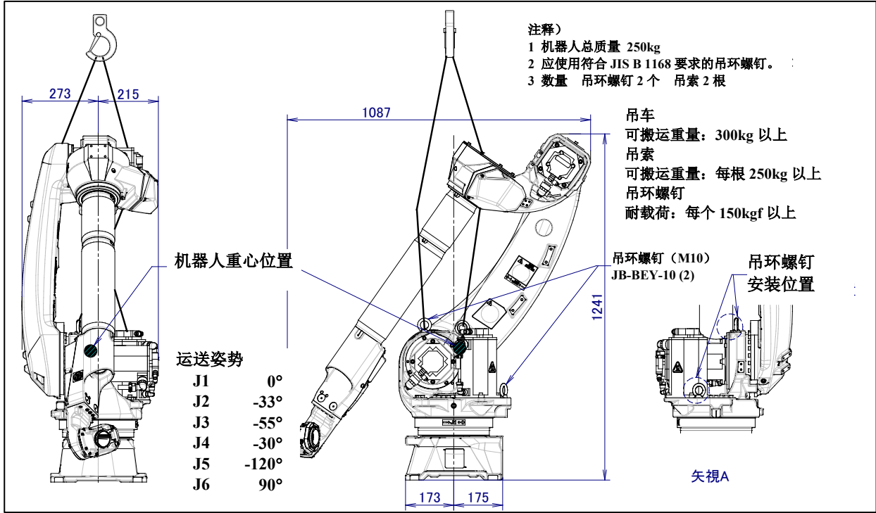
□ 1.1 (b) 用吊口搬运 (ARC Mate 120iD/12L, M-20iD/12L)
