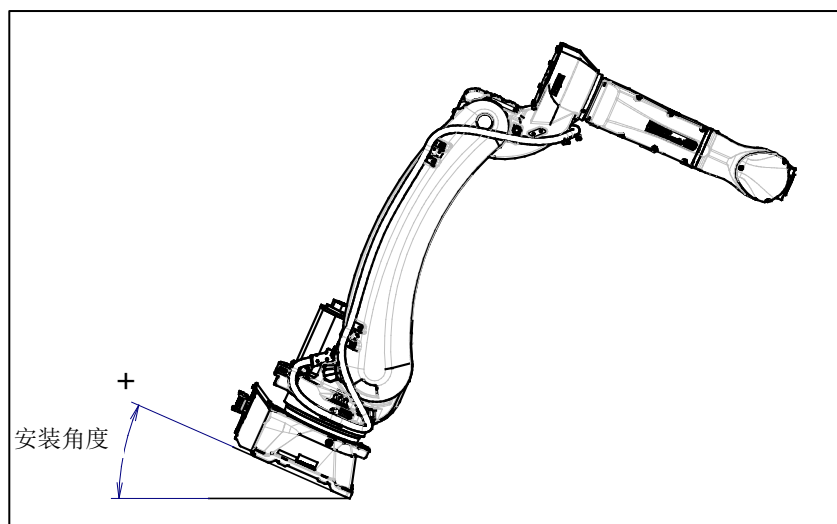
图 1.2.2 (a) 机器人的安装角度
