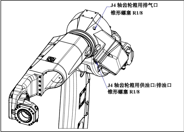
图 7.3.2.5 (a) J4 轴齿轮箱的供脂部位
