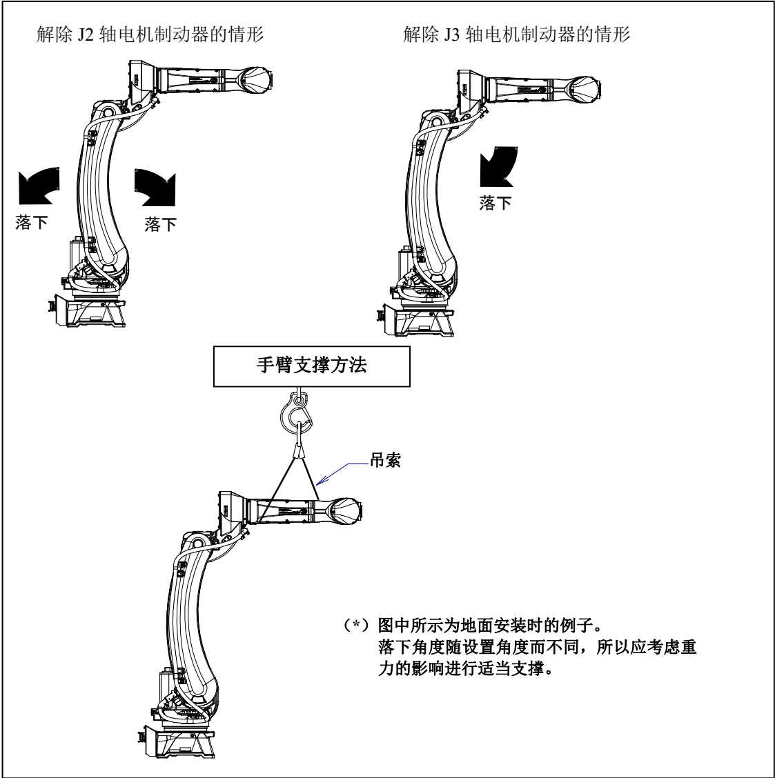
图 3 (a) 解除 J2/J3 轴的电机制动器造成的手臂动作和事先采取的措施例
