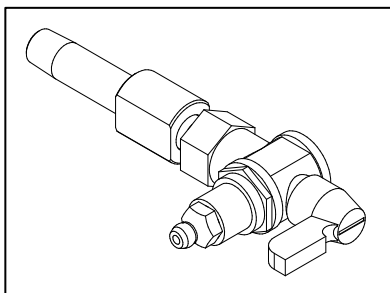
图 7.3.2.6 (c) 油注入口带有阀门 (A05B-1224-K006)
