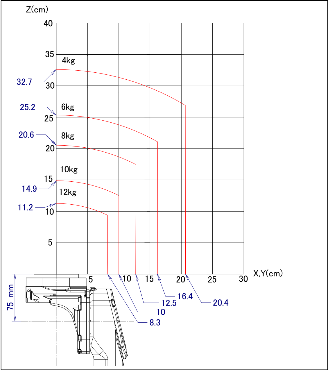
图 3.5 (c) 手腕部允许负载线图 (ARC Mate 120iD/12L, M-20iD/12L)
