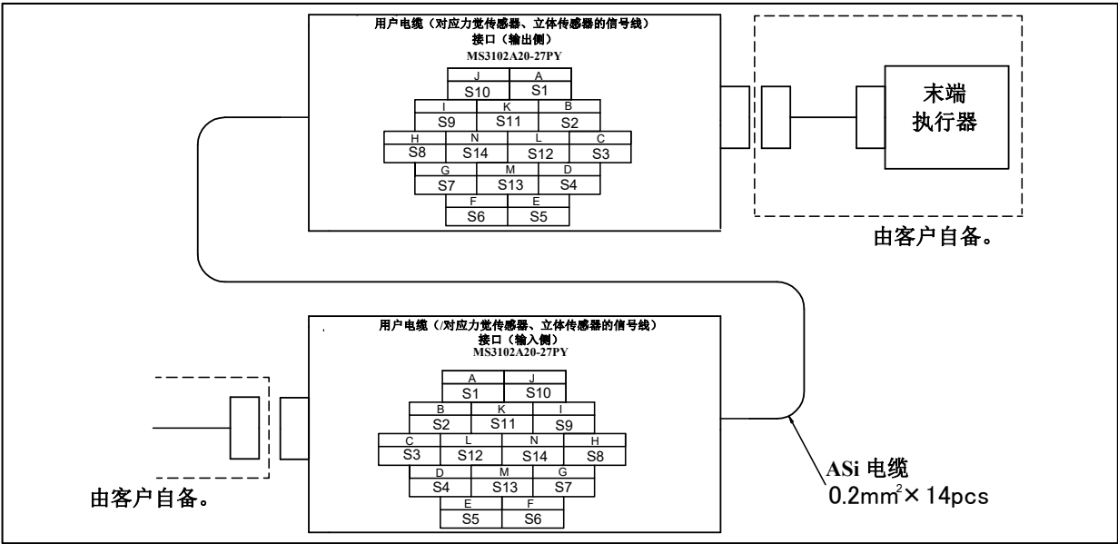
图 5.3 (m) 用户电缆（对应应力觉传感器、立体传感器的信号线）(ASi)接口的插针排列（可选项项） (指定 A05B-1228-H222#□□时)
