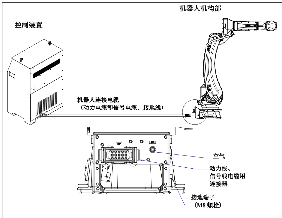
图 2 (a) 电缆连接图
