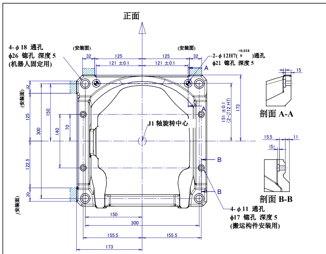
图 1.2 (a) 机器人机座尺寸
