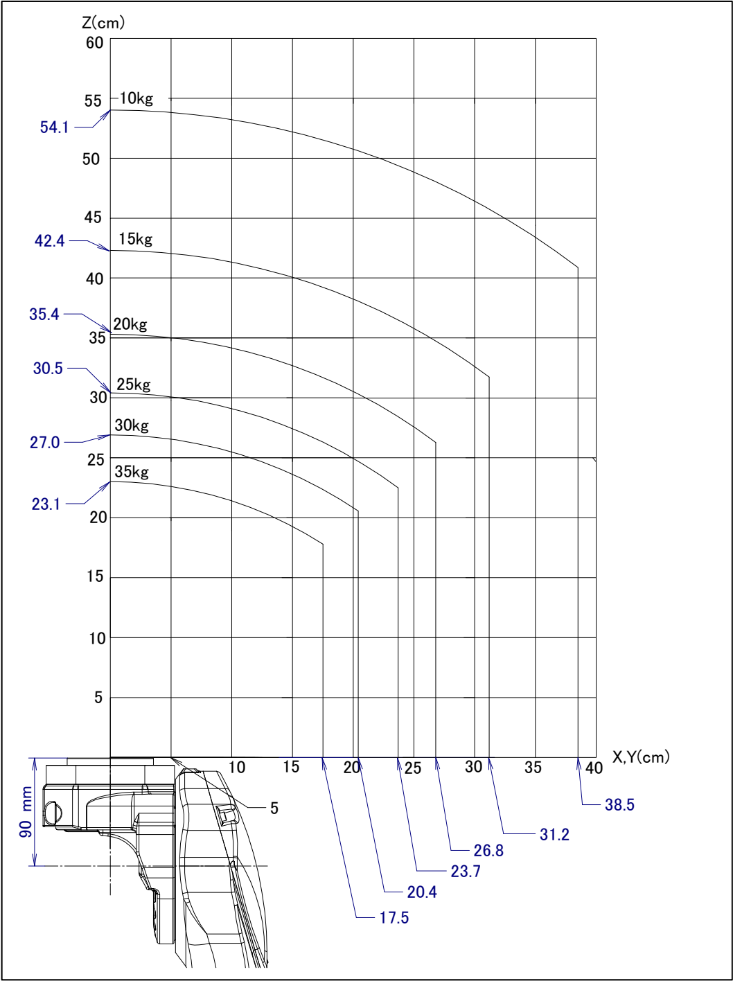
图 3.5 (d) 手腕部允许负载线图 (ARC Mate 120iD/35, M-20iD/35)
