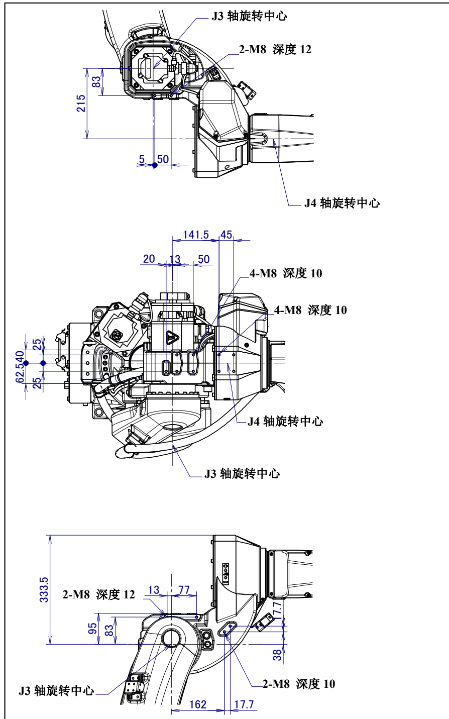
图 4.2 (b) 设备安装面尺寸 (1/2) (A+B+C 部)
