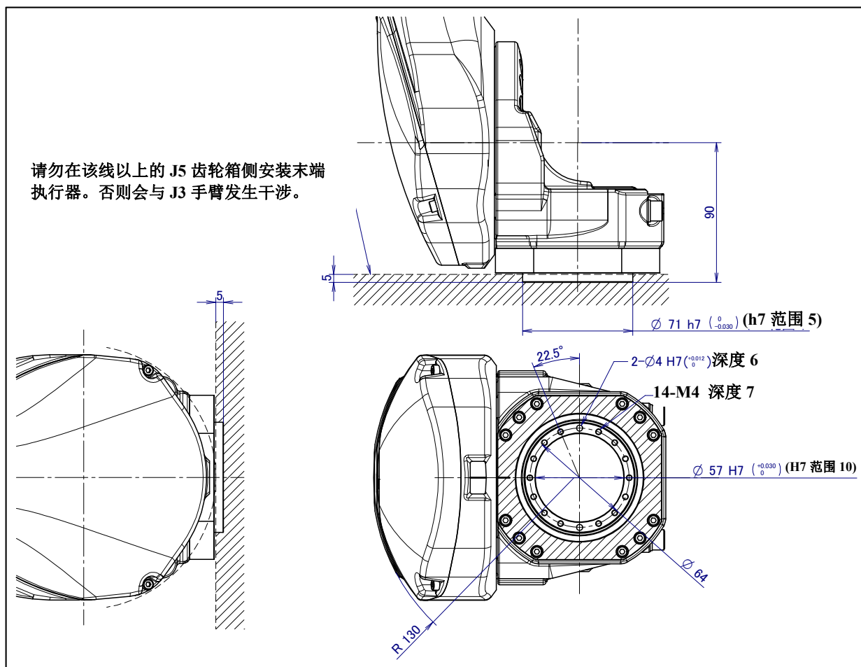
图 4.1 (a) 末端执行器安装面(ARC Mate 120iD, ARC Mate 120iD/35, M-20iD/25/35)
