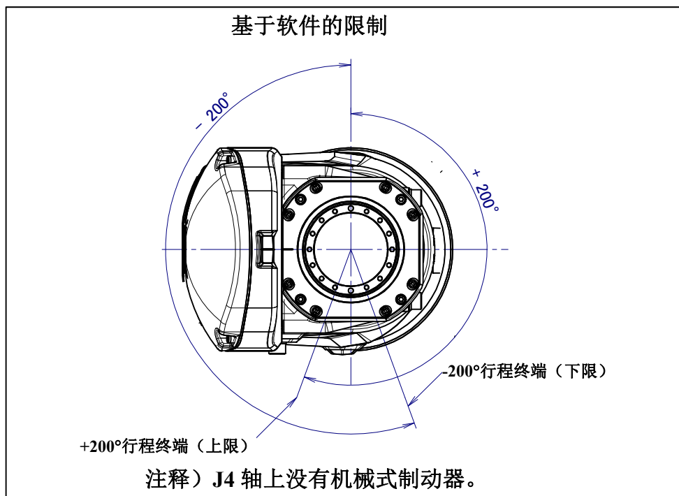
图 3.3 (g) J4 轴可动范围
