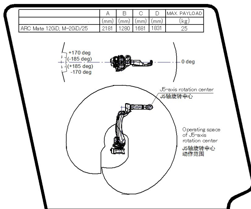
图 4 (f) 动作范围标签 (例: ARC Mate 120iD, M-20iD/25)
