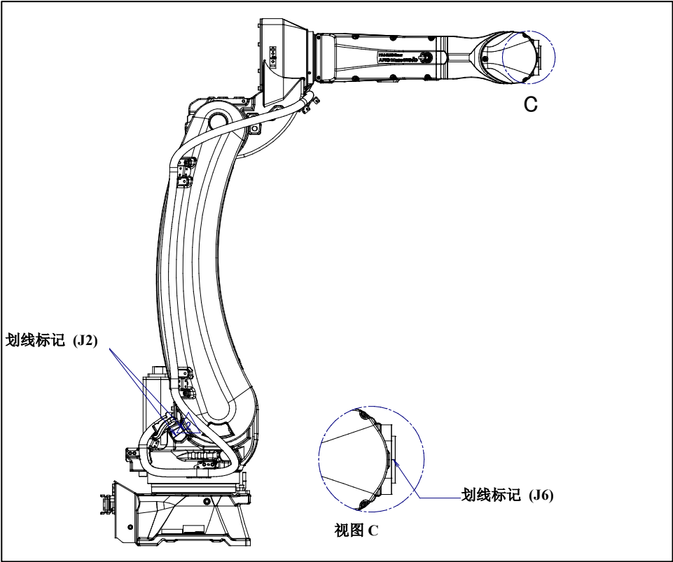
图 8.3 (b) 各轴的对合标记位置
