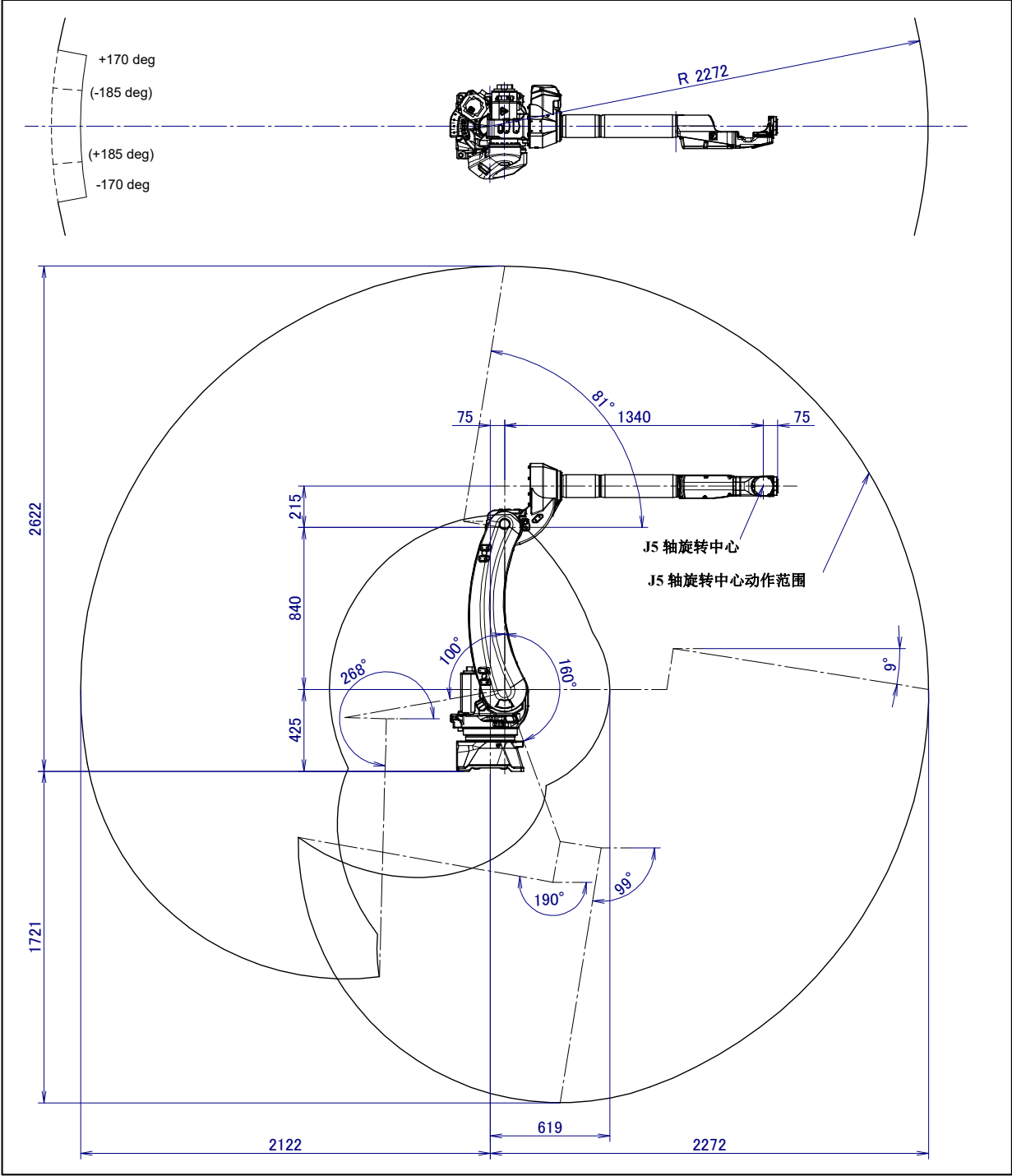
图 3.2 (b) 动作范围图 (ARC Mate 120iD/12L, M-20iD/12L)
