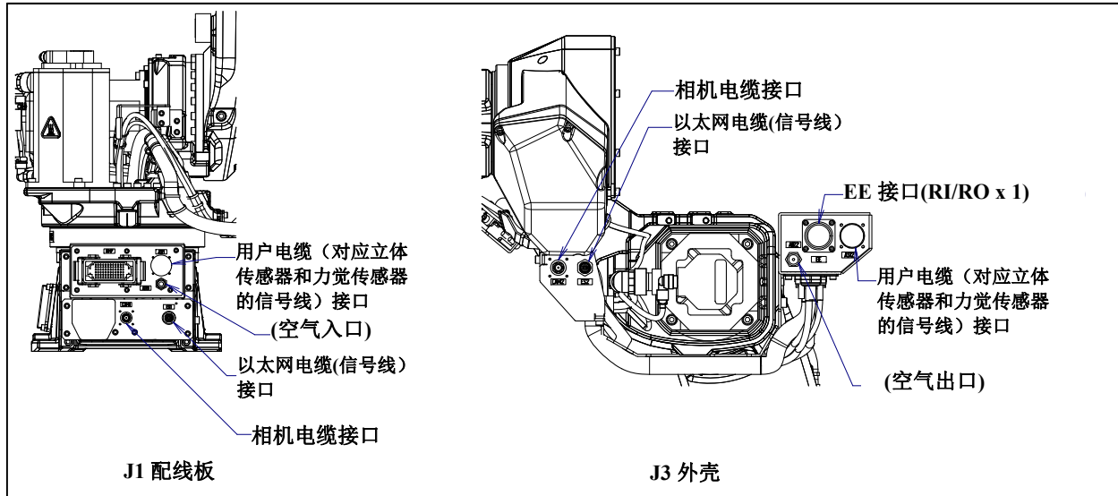
图 5.3 (f) 可选项电缆用接口 (指定 A05B-1228-H224#□□时)
