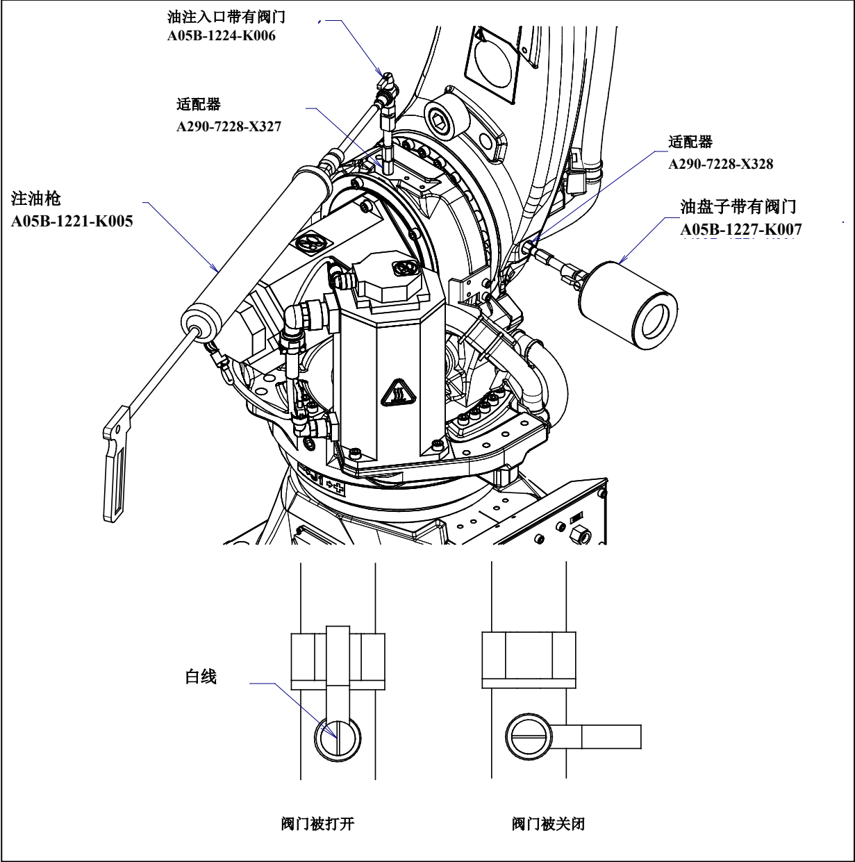
图 7.3.2.3 (c) 用注油枪供油（J2 轴减速机的供油）（地面安装的例）
