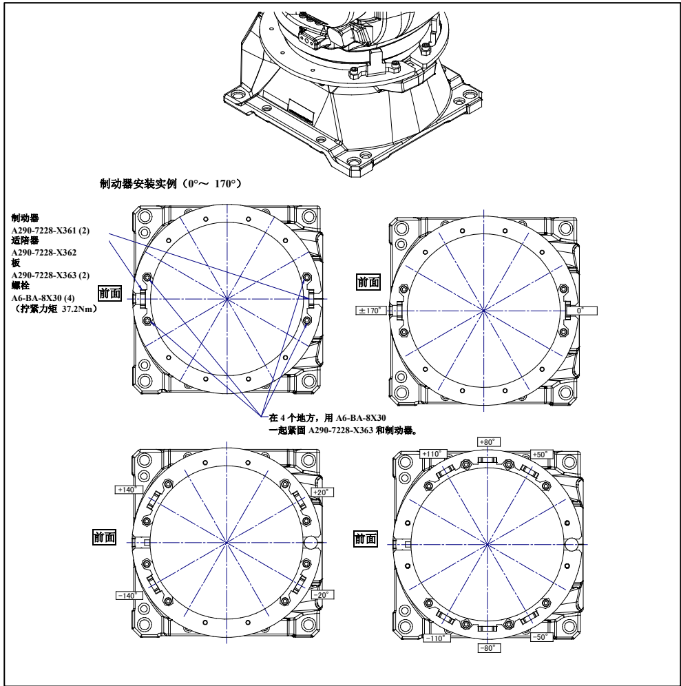
图 6.2.1 (a) J1 轴机械式可变制动器的安装
