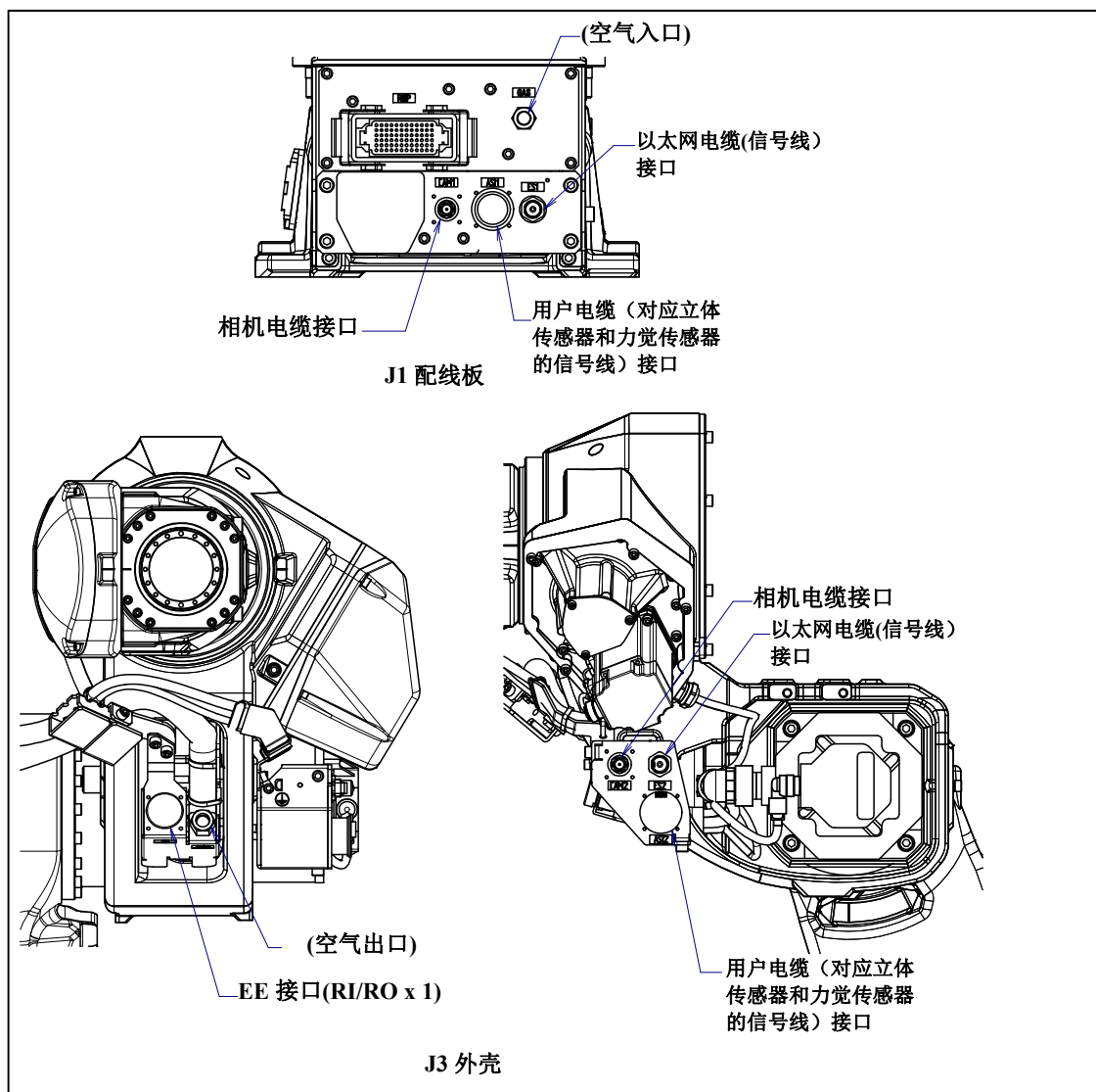
图 5.3 (d) 可选项电缆用接口 (指定 A05B-1228-H222#□□时)
