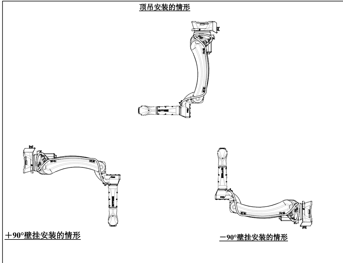
图 7.3.2 (a) 安装形式
