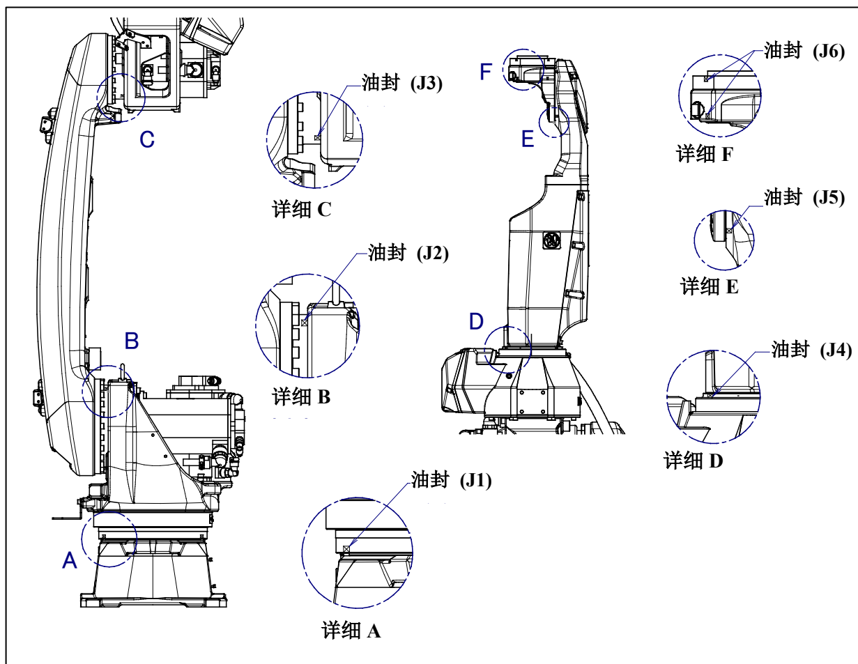
图 7.2.1 (a) 渗油的检查部位
