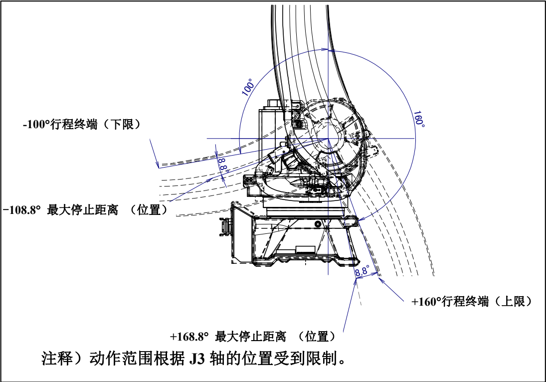
图 3.3 (e) J2 轴可动范围
