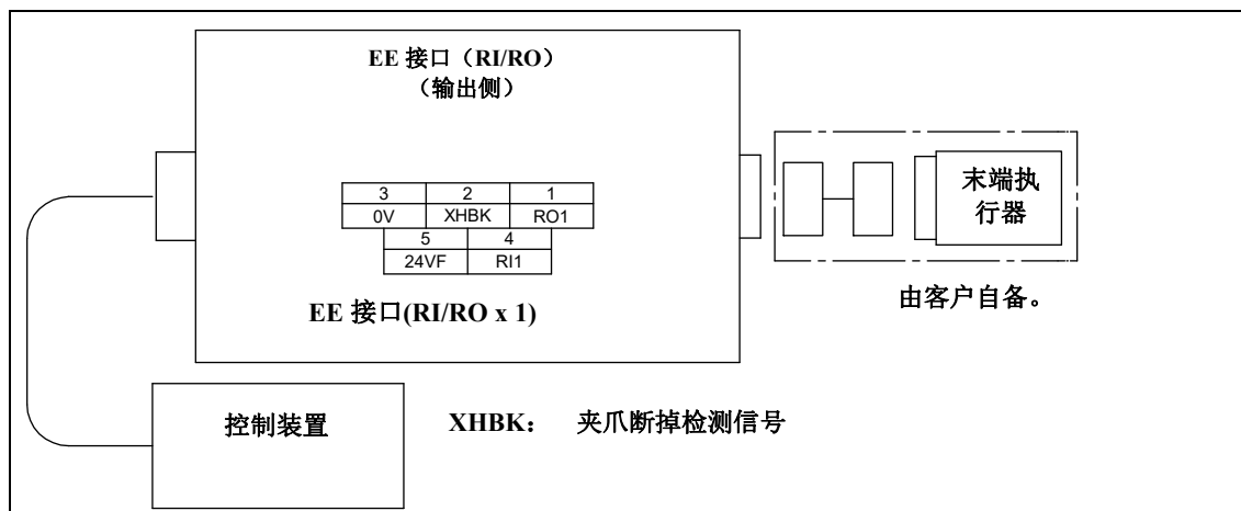
图 5.3 (g) EE 接口(RI/RO)的插针排列 RI/RO 各 1 点 (可选项) (指定 A05B-1228- H201#□□, H205#□□时)
