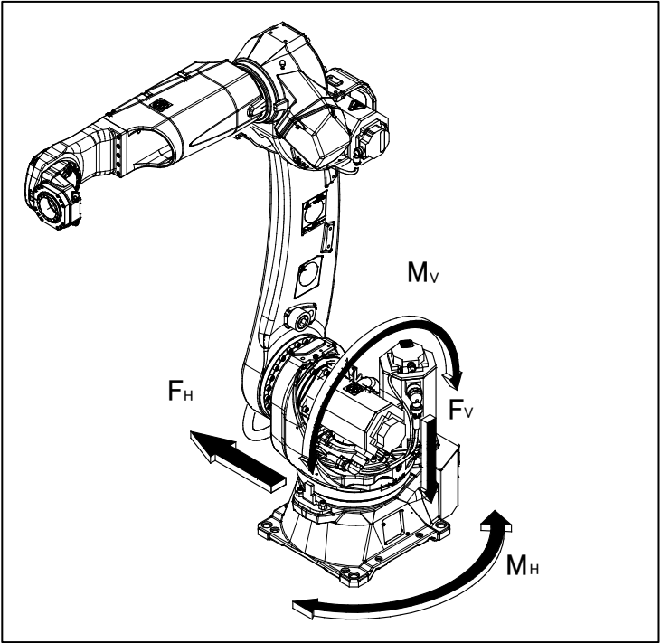
图 1.2.1 (b) 作用于机器人机座的力和力矩
