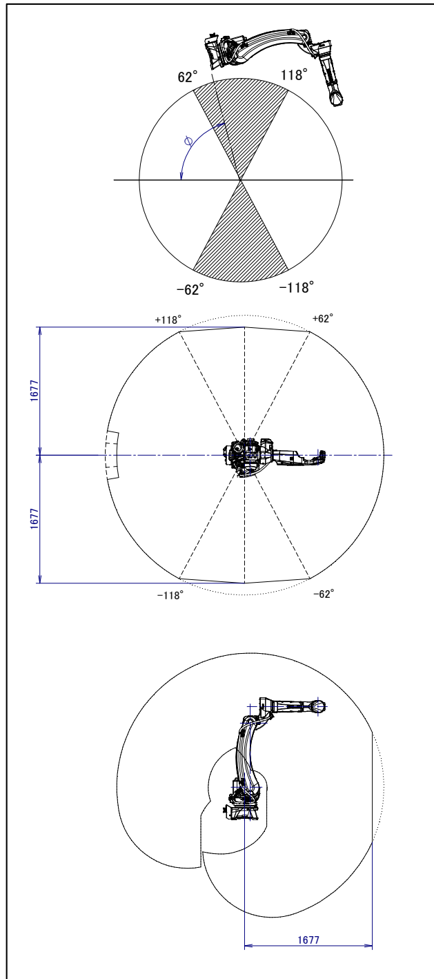
图 3.6 (c) 设置范围 (2) 动作范围图(ARC Mate 120iD, M-20iD/25) (-118^\circ < \phi < -62^\circ, 62^\circ < \phi < 118^\circ)
