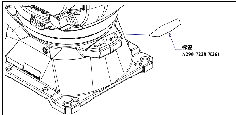
图 6.2.1 (b) J1 轴机械式可变制动器安装部保护标签
