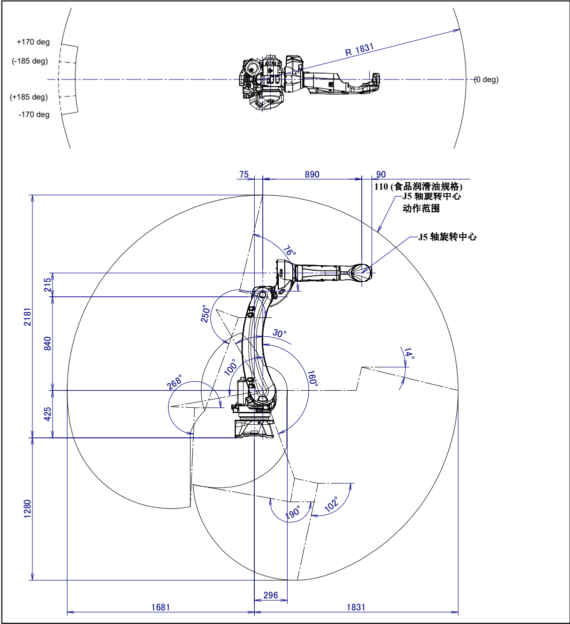
图 3.2 (a) 动作范围图 (ARC Mate 120iD, ARC Mate 120iD/35, M-20iD/25/35)
