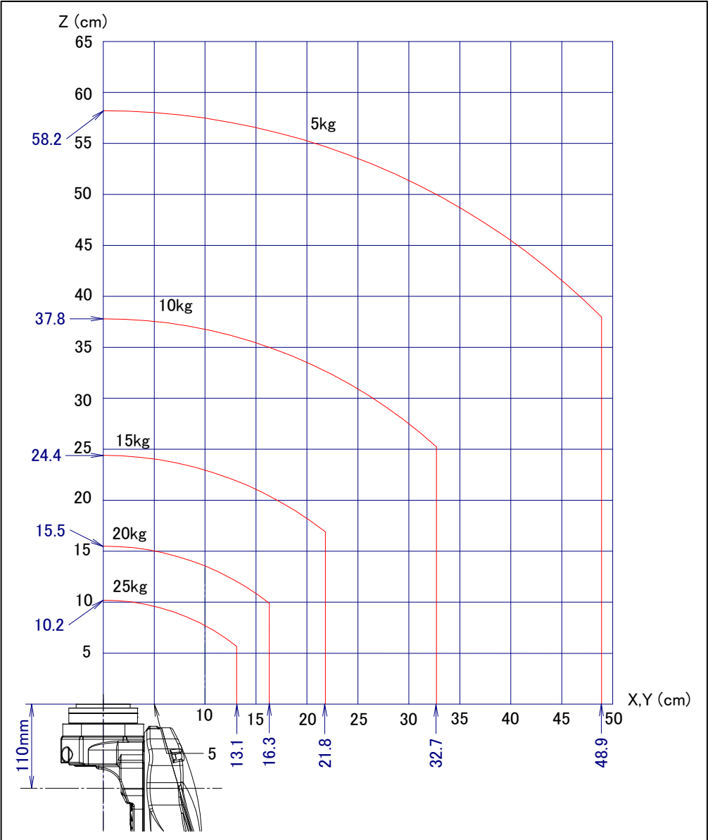
图 3.5 (b) 手腕部允许负载线图 (M-20iD/25 食品润滑油规格)
