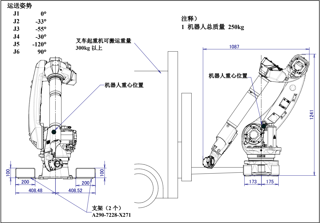
图 1.1 (d) 用叉车起重机搬运 (ARC Mate 120iD/12L, M-20iD/12L)
