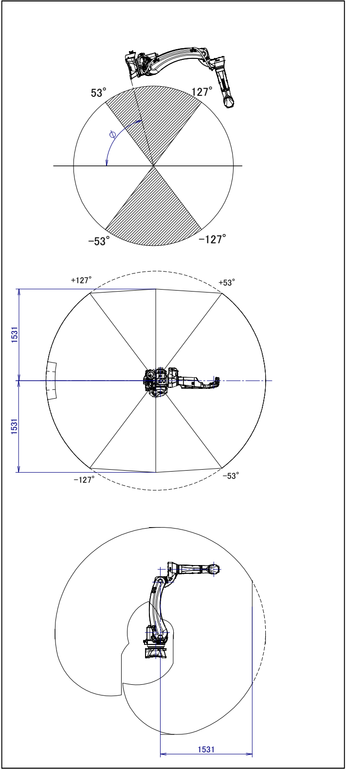
图 3.6 (c) 设置范围 (2) 动作范围图(ARC Mate 120iD/35, M-20iD/35) ( -127^{\circ} < \phi < -53^{\circ} , 53^{\circ} < \phi < 127^{\circ} )
