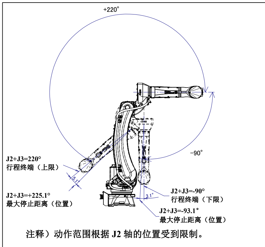
图 3.3 (f) J3 轴可动范围
