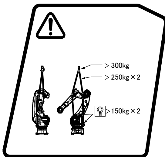
图 4 (d) 搬运标签
