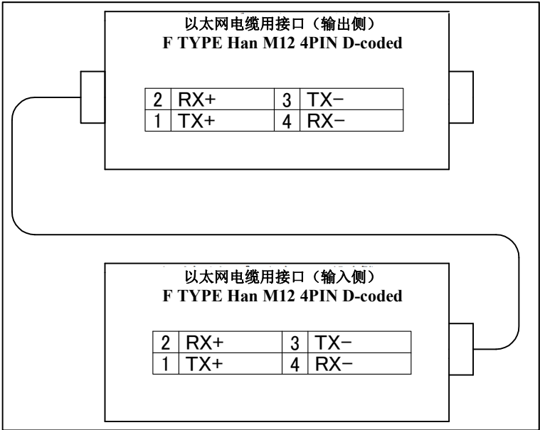
图 5.3 (n) 以太网电缆(ES)用接口的插针排列（可选项项） (指定 A05B-1228-H222#□□时)
