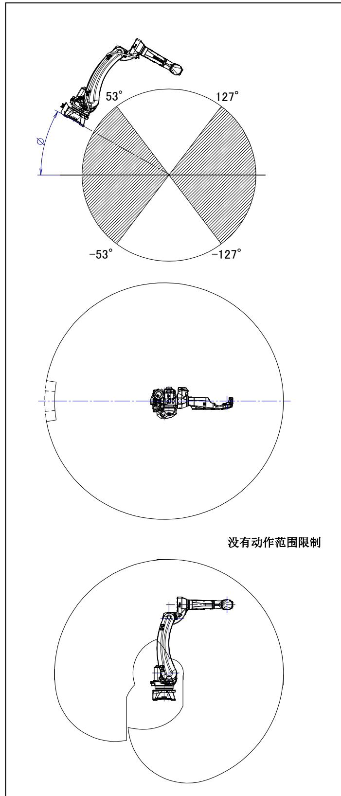
图 3.6 (d) 设置范围 (1) 动作范围图(ARC Mate 120iD/35, M-20iD/35) (-180^{\circ} \leq \phi \leq -127^{\circ}, -53^{\circ} \leq \phi \leq 53^{\circ}, 127^{\circ} \leq \phi \leq 180^{\circ})
