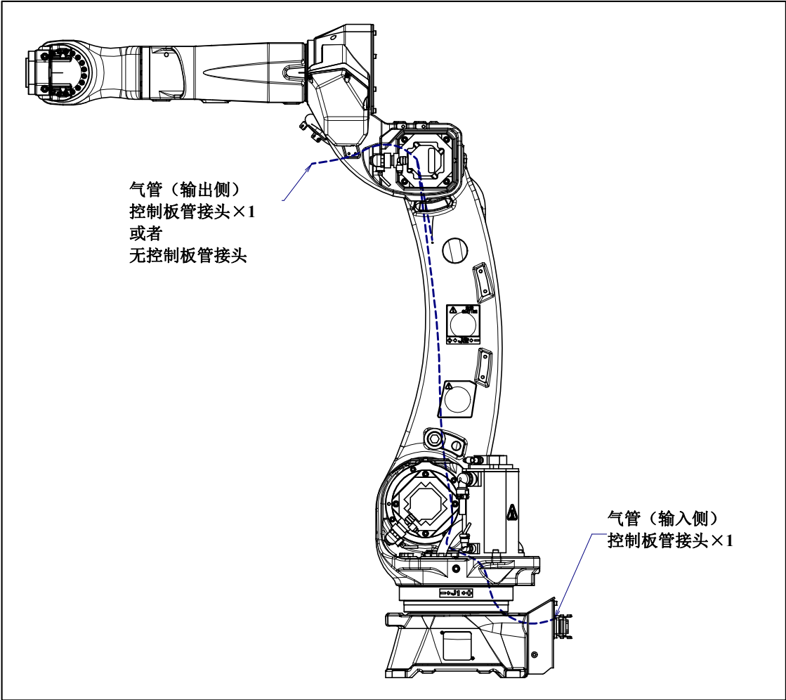
图 5.1 (a) 气压供应口（可选项）
