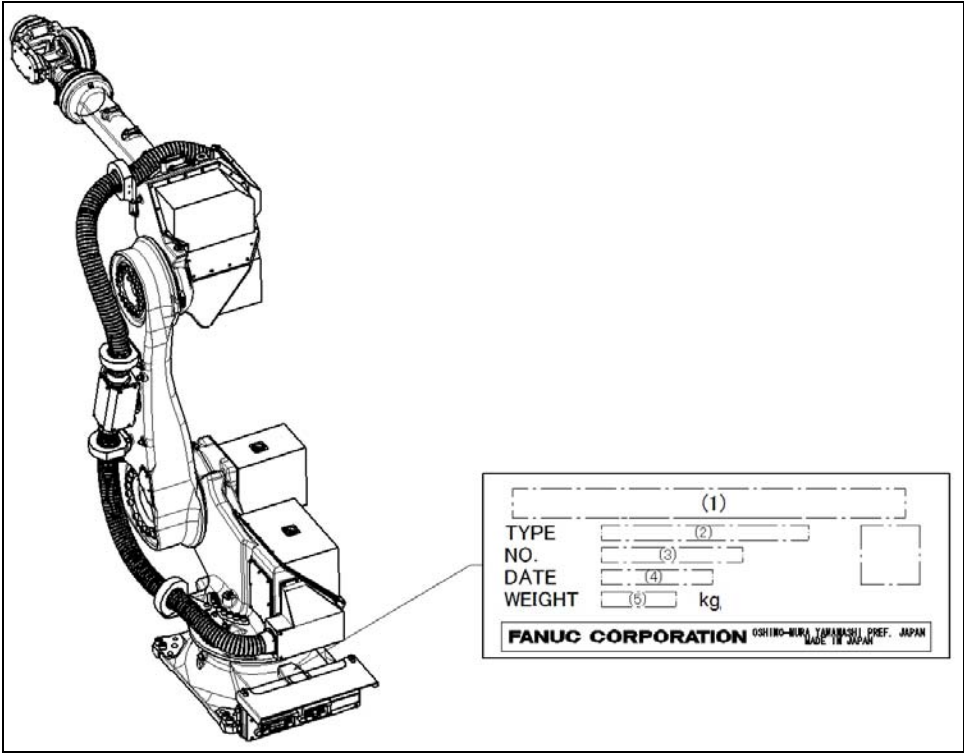
机构部规格编号粘贴位置
