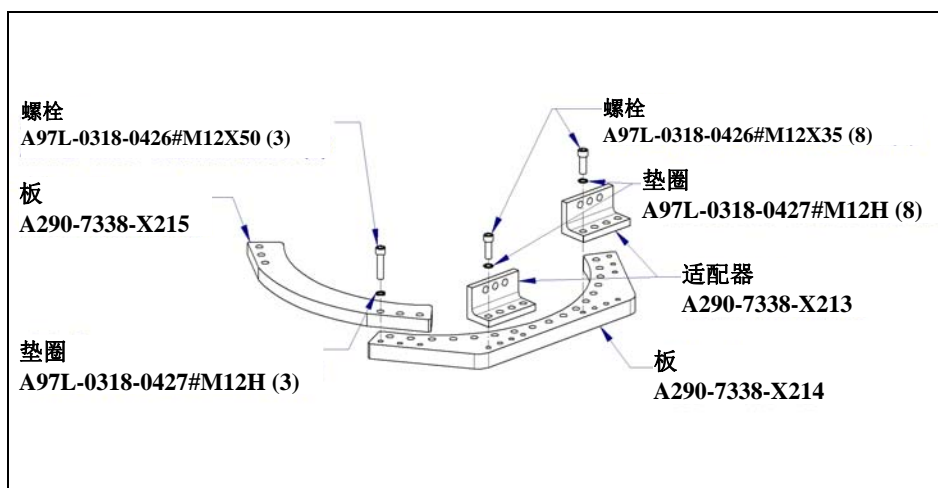
图 6.2.1 (e) J1 轴机械式可变制动器的安装 (4/7)
