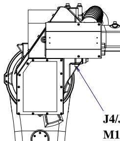
图 7.3.2 (c) J4/J5/J6 轴齿轮箱的润滑油的更换
