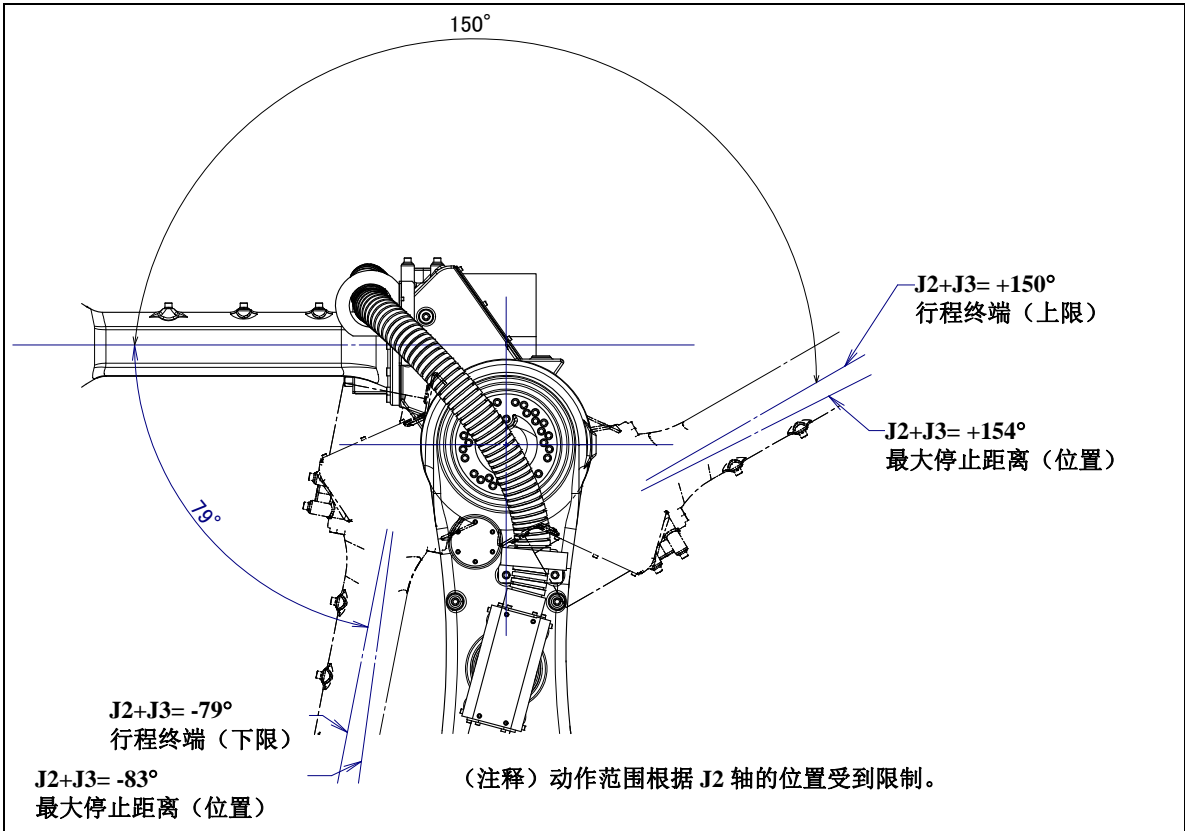
图 3.3 (d) J3 轴可动范围
