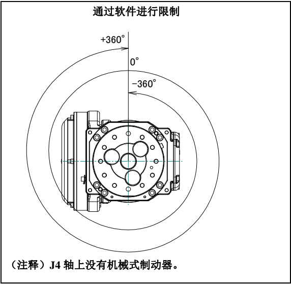
图 3.3 (e) J4 轴可动范围
