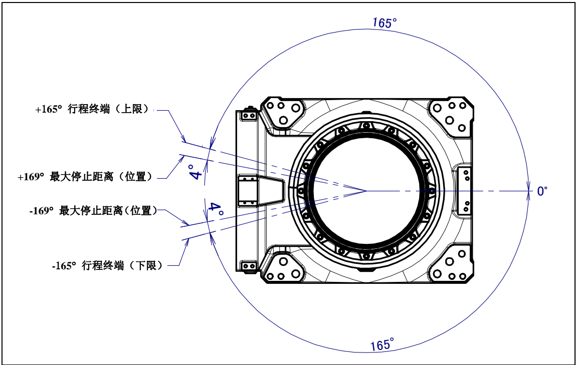
图 3.3 (b) J1 轴可动范围
