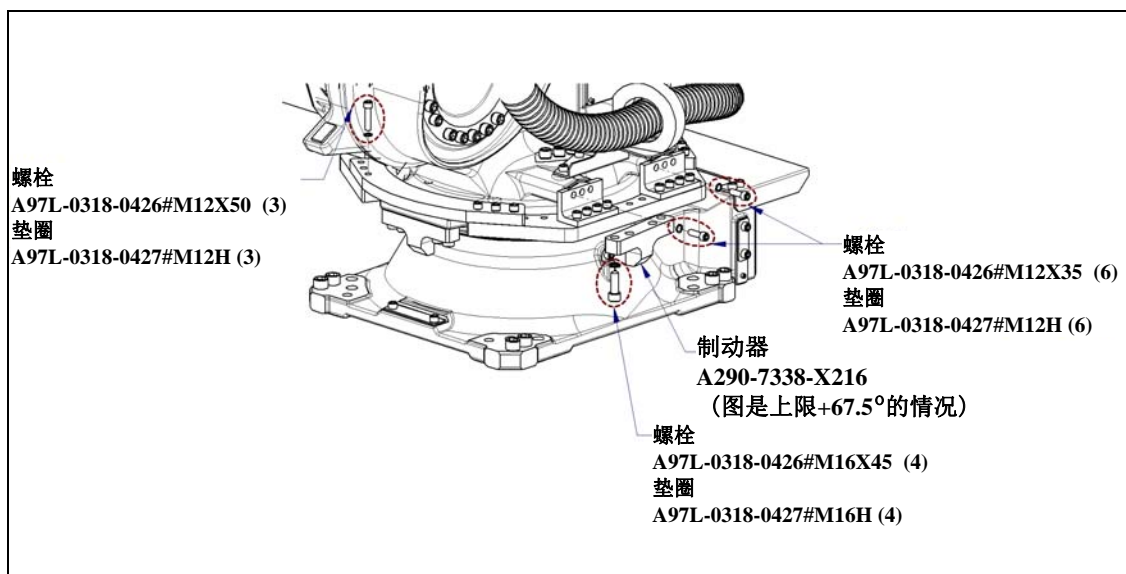
图 6.2.1 (f) J1 轴机械式可变制动器的安装 (5/7)
