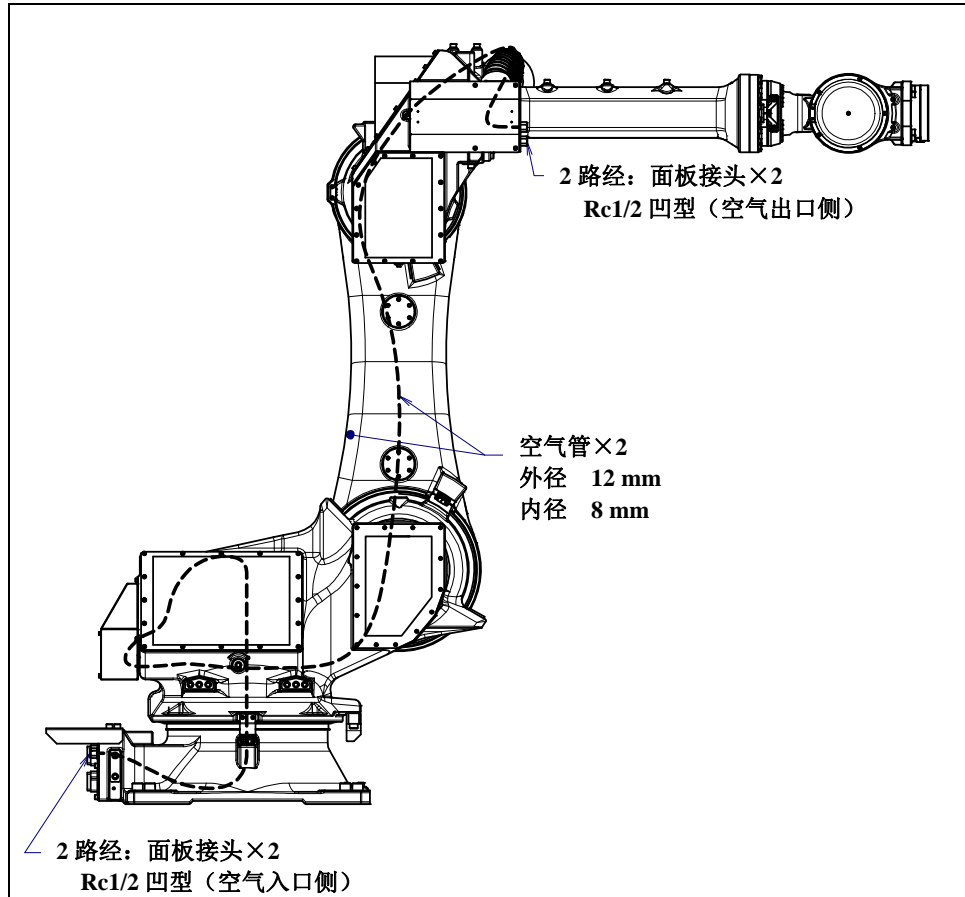
图 5.1 (a) 气压供应口（可选项项）
