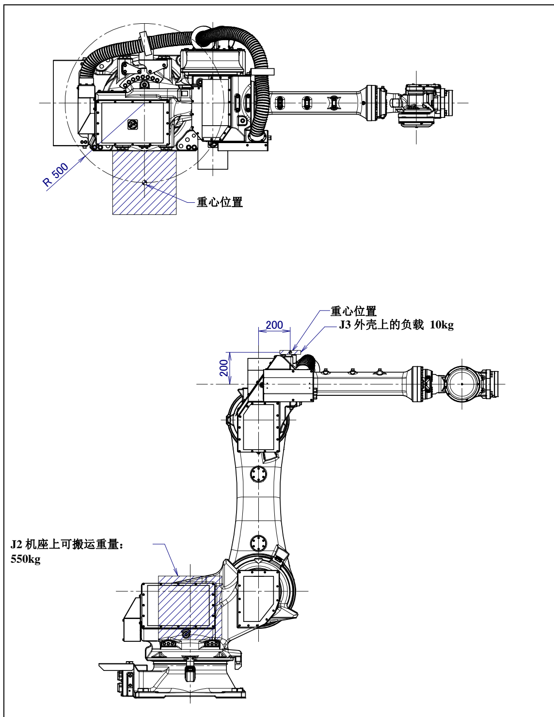
图 3.5 (a) J2 机座/J3 外壳上的负载条件
