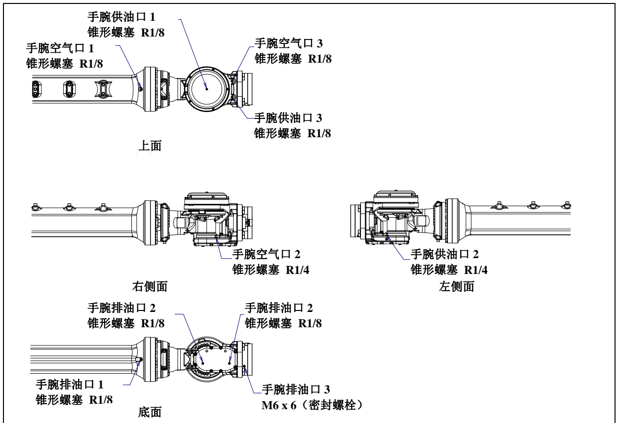
图 7.3.2 (d) 手腕的润滑油的更换
