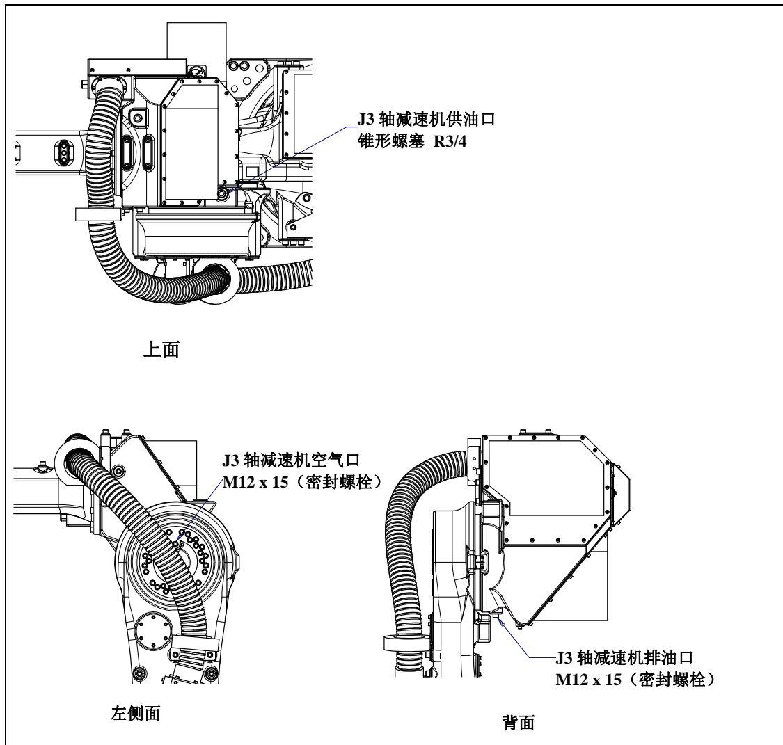
图 7.3.2 (b) J3 轴减速机的润滑油的更换
