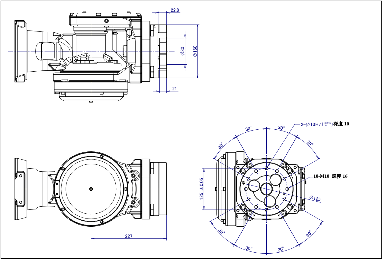
图 4.1 (a) 末端执行器安装面 (ISO 法兰盘)
