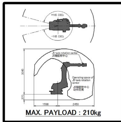
图 5 (e) 动作范围、可搬运重量标签
