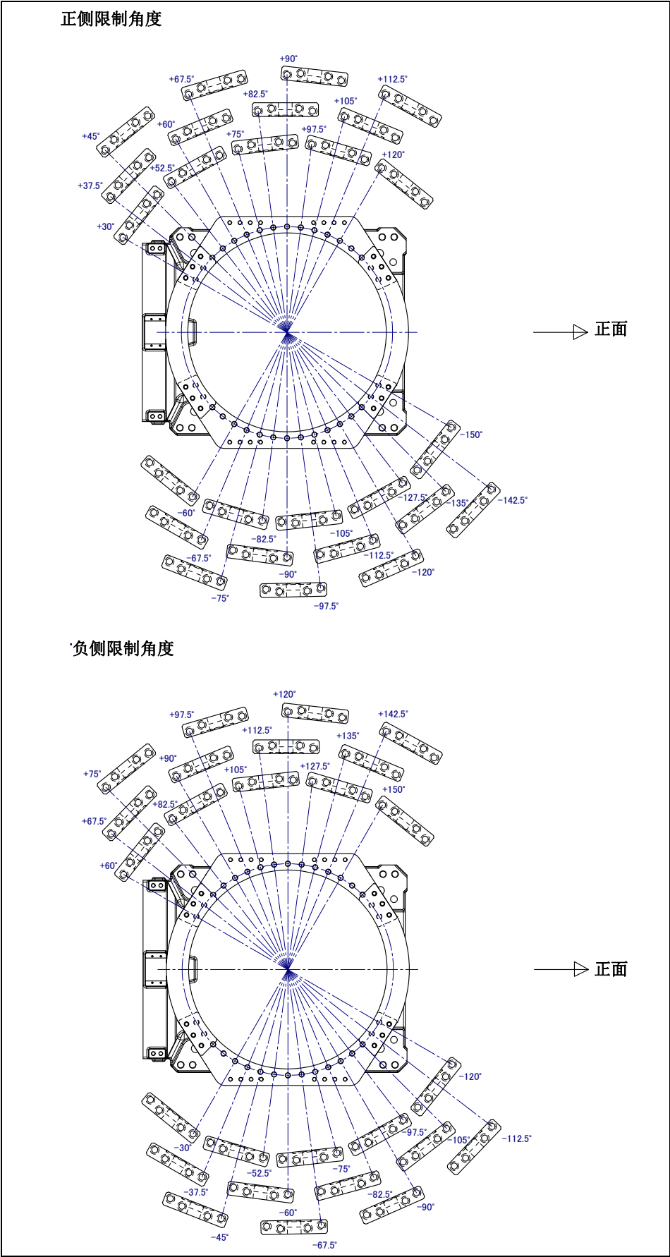
图 6.2.1 (h) J1 轴机械式可变制动器的安装 (7/7)
