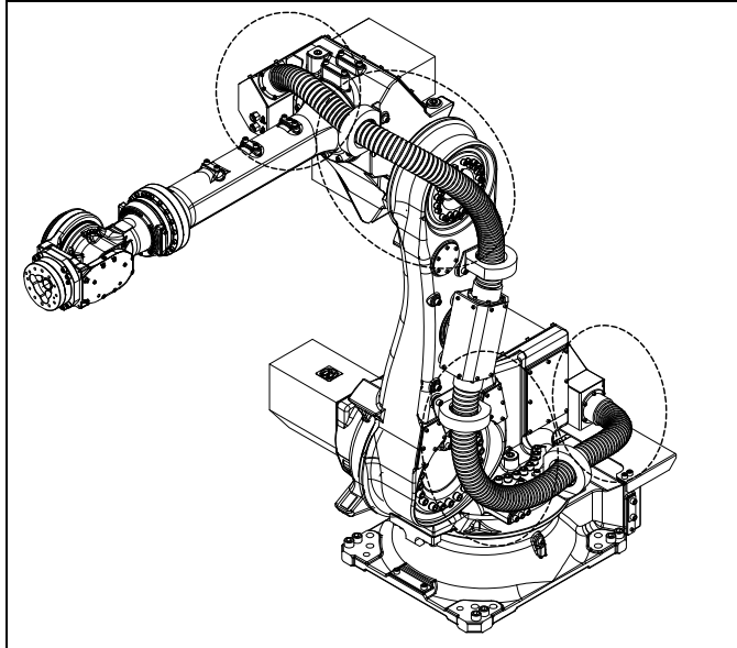
图 7.2.3 (a) 机构部内电缆的检修部位
