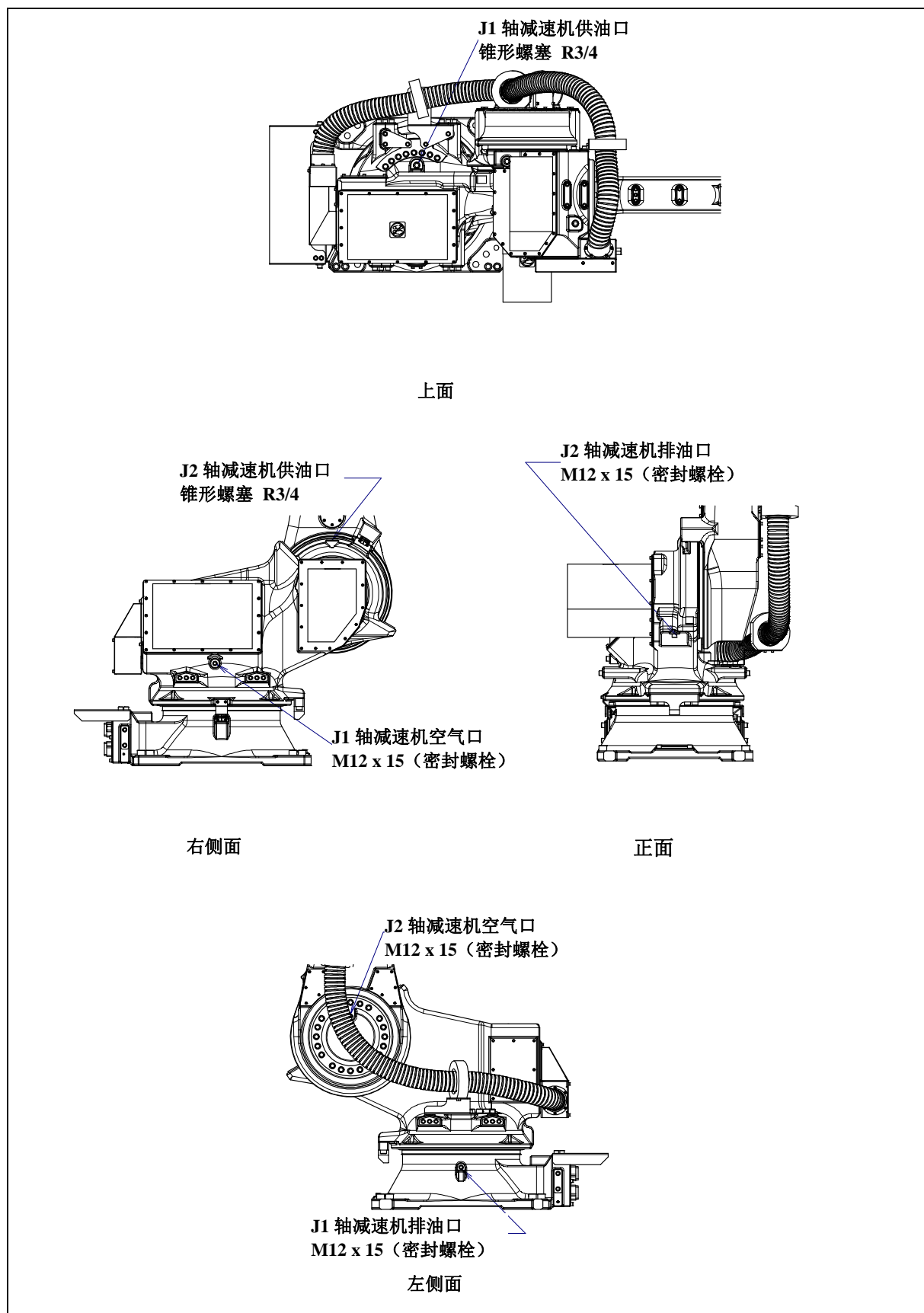
图 7.3.2 (a) J1/J2 轴减速机的润滑油的更换
