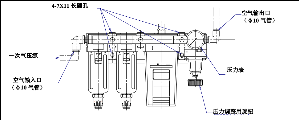
图 7.2.2 (b) 气压组件用调节器组件（可选项）
