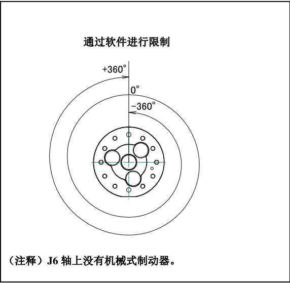
图 3.3 (g) J6 轴可动范围
