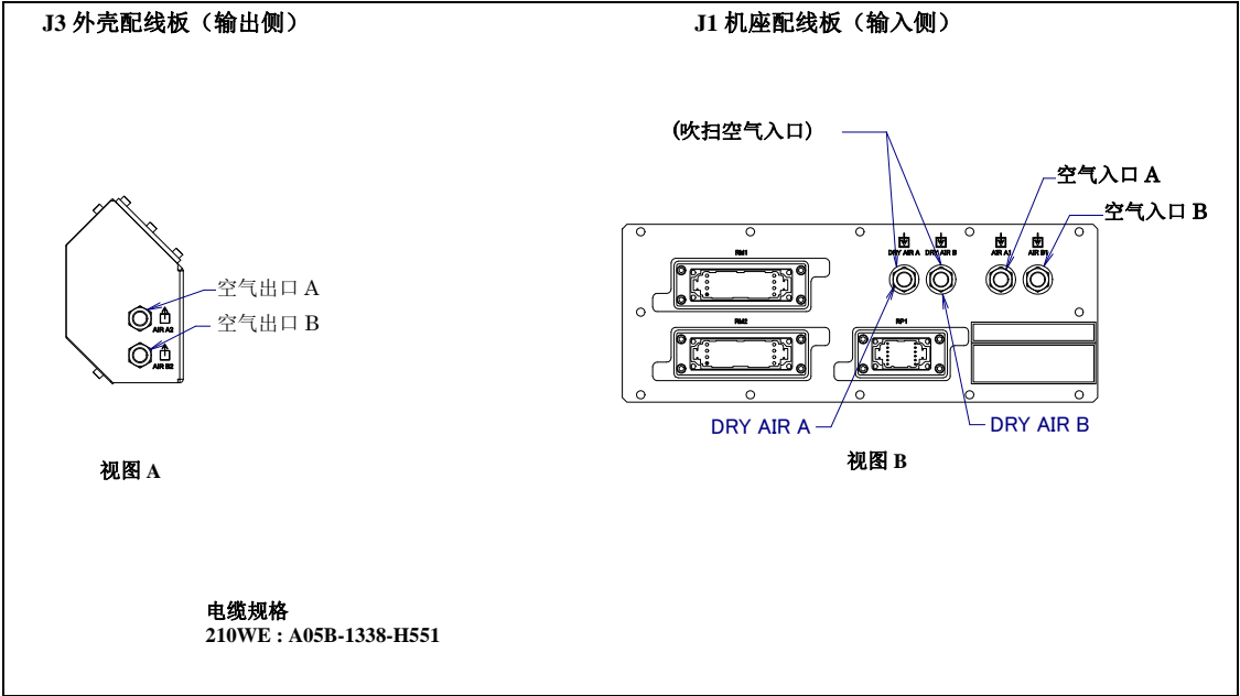
图 5.3 (b) 空气用接口
