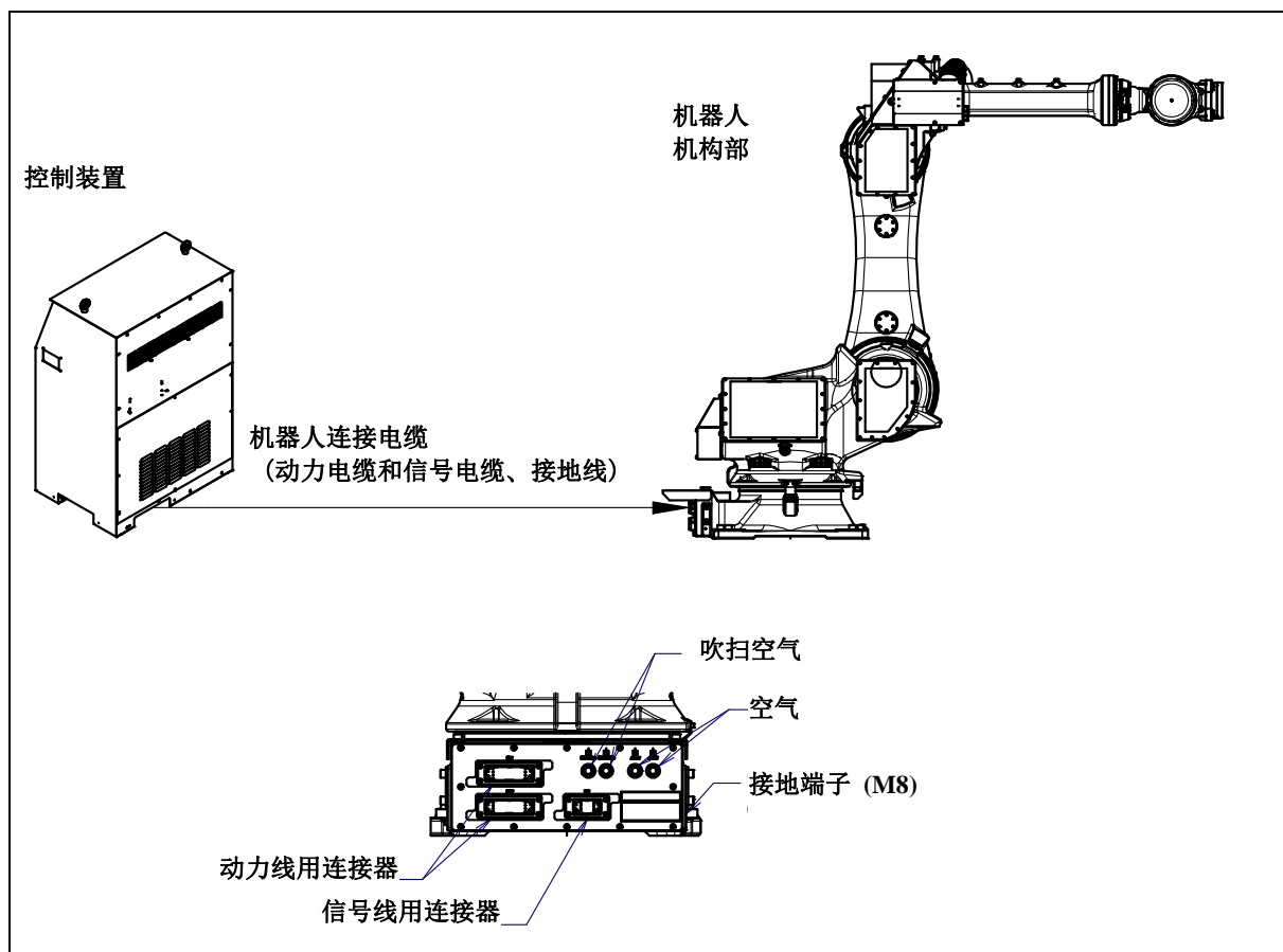
图 2.1 (a) 电缆连接图
