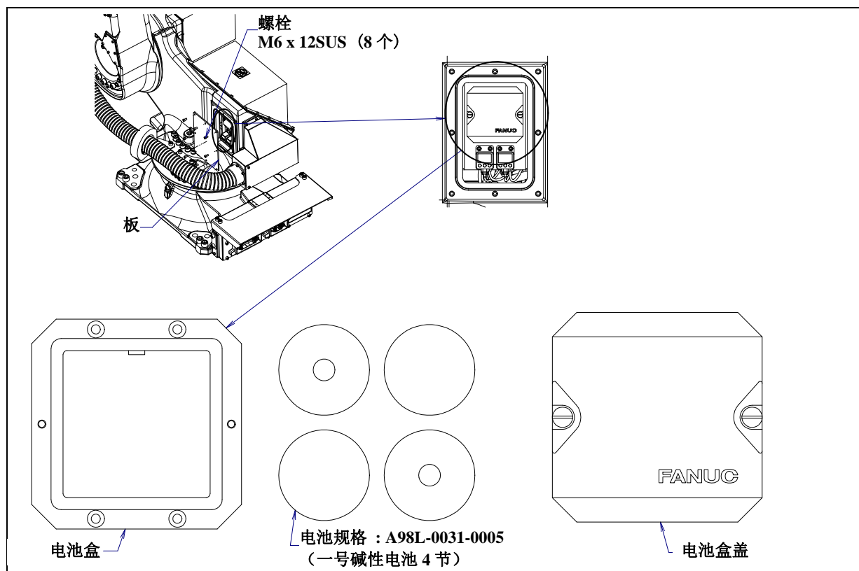
图 7.3.1 (a) 电池的更换
