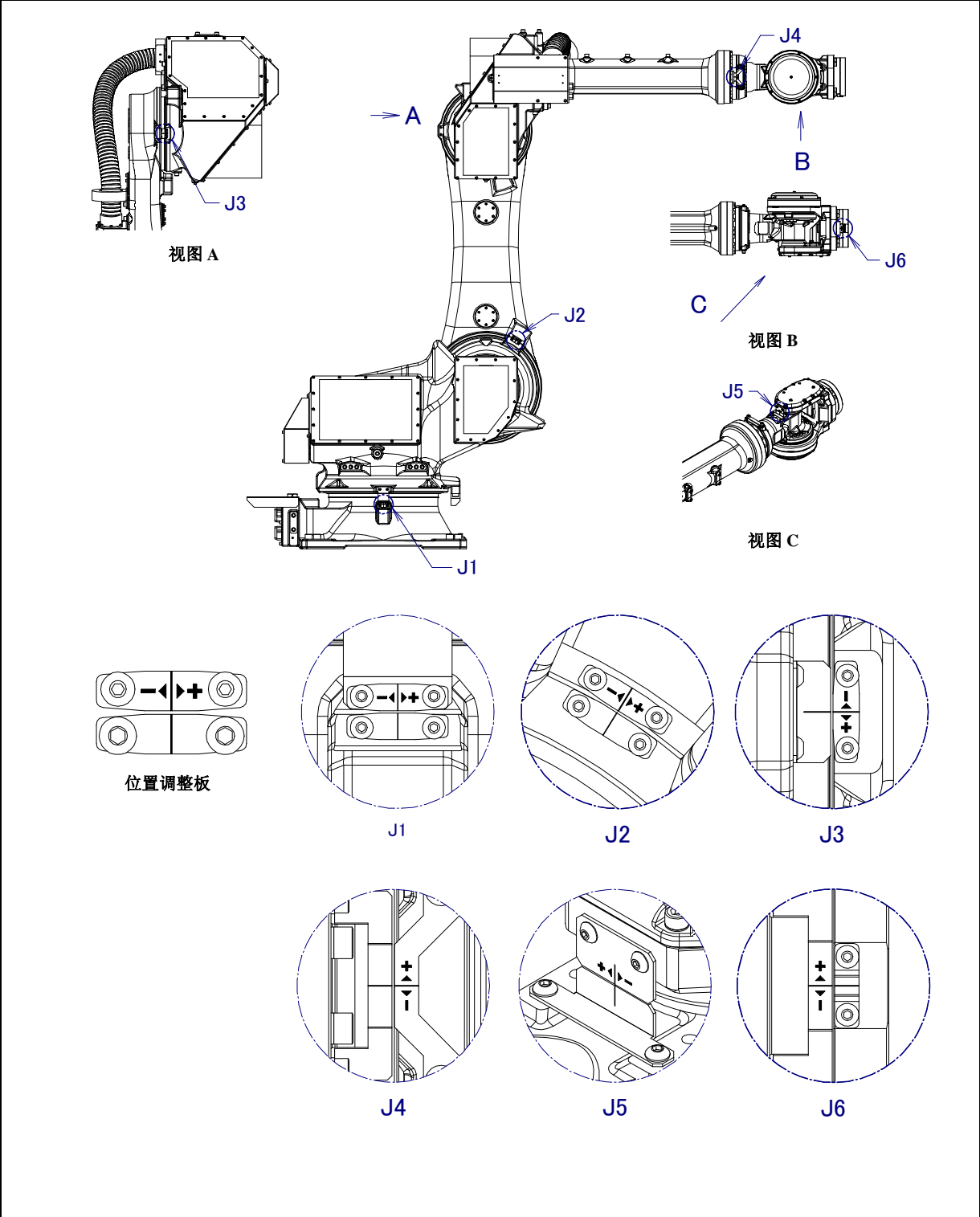
图 8.3 (a) 各轴的对合标记位置
