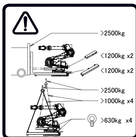
图 5 (d) 搬运标签
