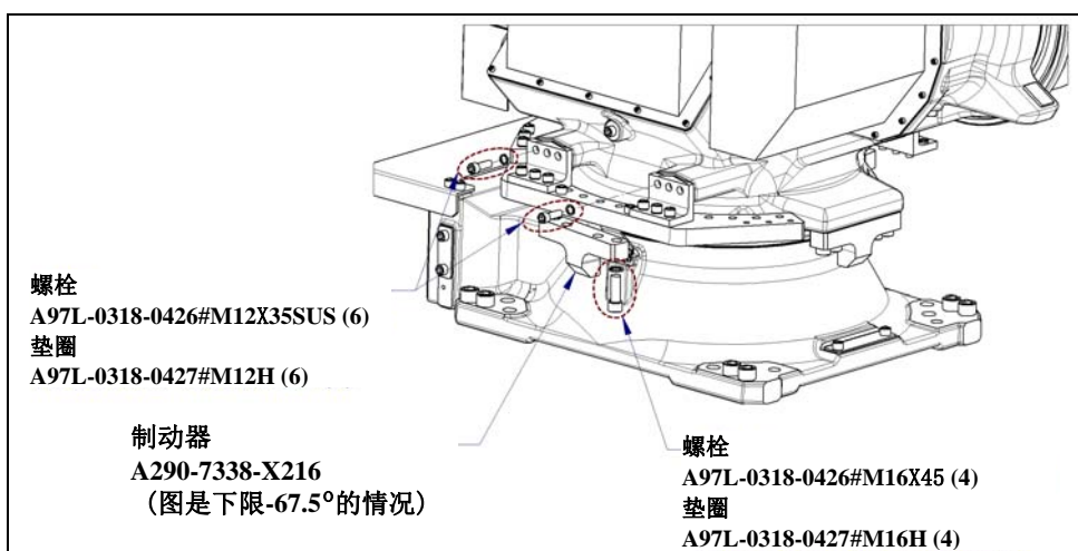
图 6.2.1 (d) J1 轴机械式可变制动器的安装 (3/7)
