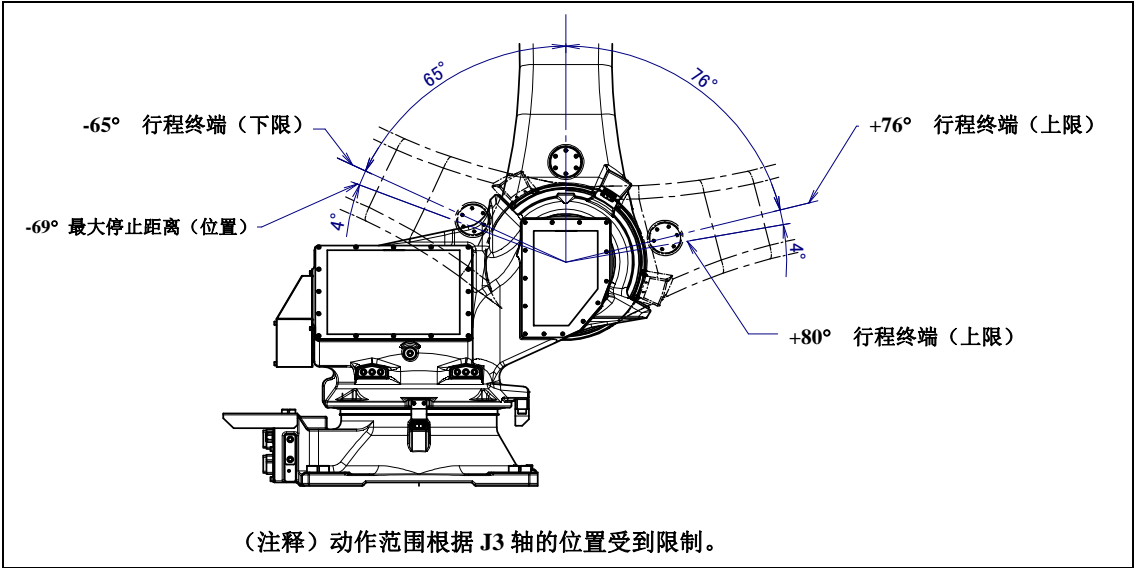
图 3.3 (c) J2 轴可动范围
