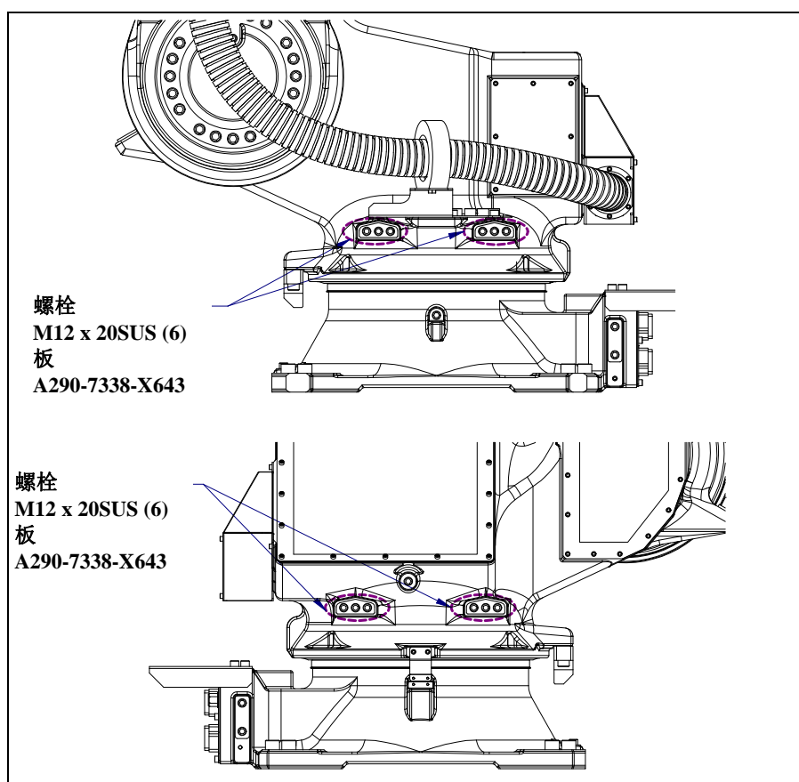
图 6.2.1 (b) J1 轴机械式可变制动器的安装 (1/7)
