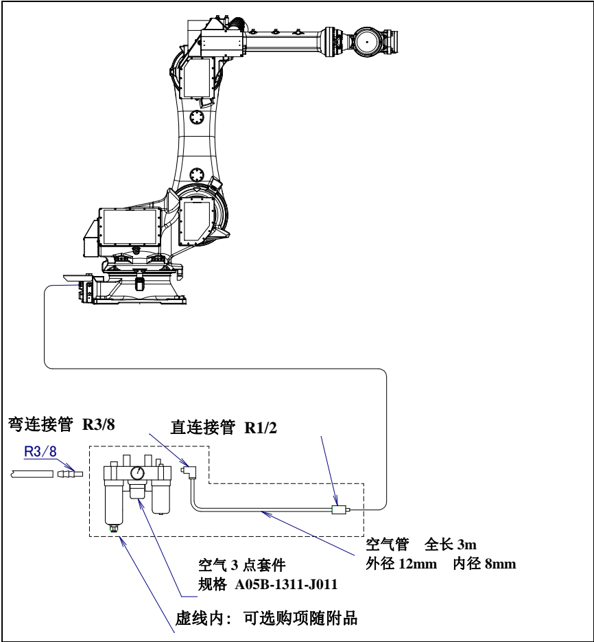
图 5.2 (a) 空气配管（可选项）
