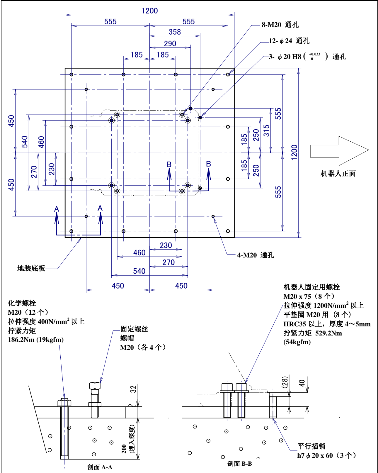
图 1.2.1 (b) 安装方法 II
