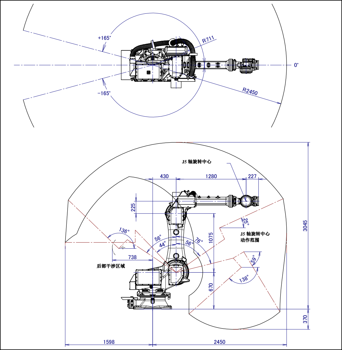
图 3.2 (a) 动作范围图
