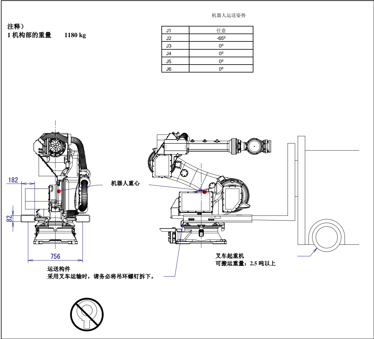
图 1.1 (b) 采用叉车起重机搬运
