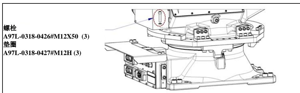
图 6.2.1 (g) J1 轴机械式可变制动器的安装 (6/7)
