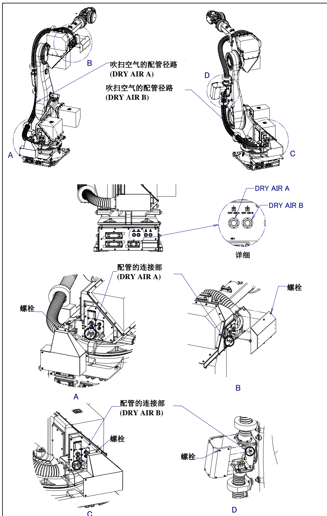
图 7.2.5 (a) 吹扫空气的配管的检查
