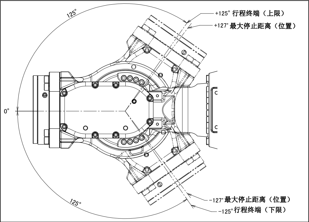
图 3.3 (f) J5 轴可动范围
