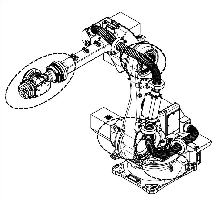
图 7.2.1 (a) 渗油的检查部位
