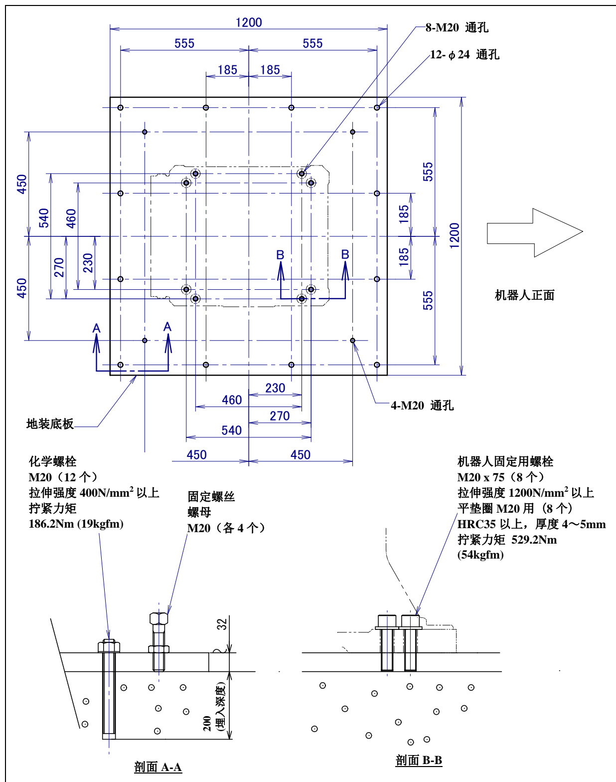
图 1.2.1 (c) 安装方法III
