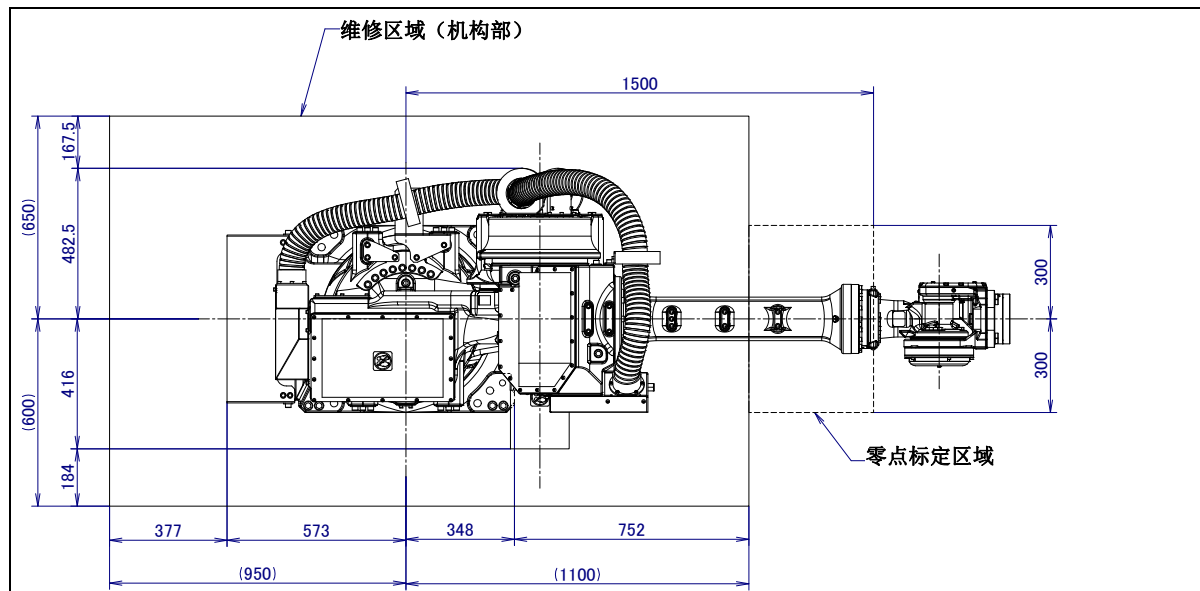
图 1.3 (a) 维修空间的布局图
