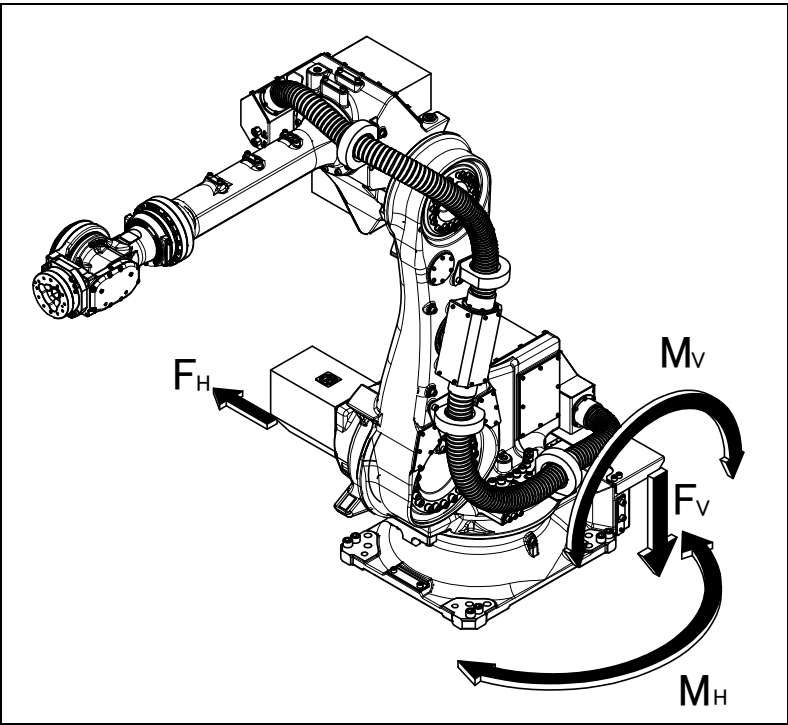
图 1.2.1 (d) 断电停止时作用的力以及力矩
