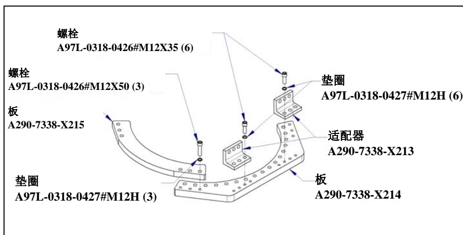
图 6.2.1 (c) J1 轴机械式可变制动器的安装 (2/7)
