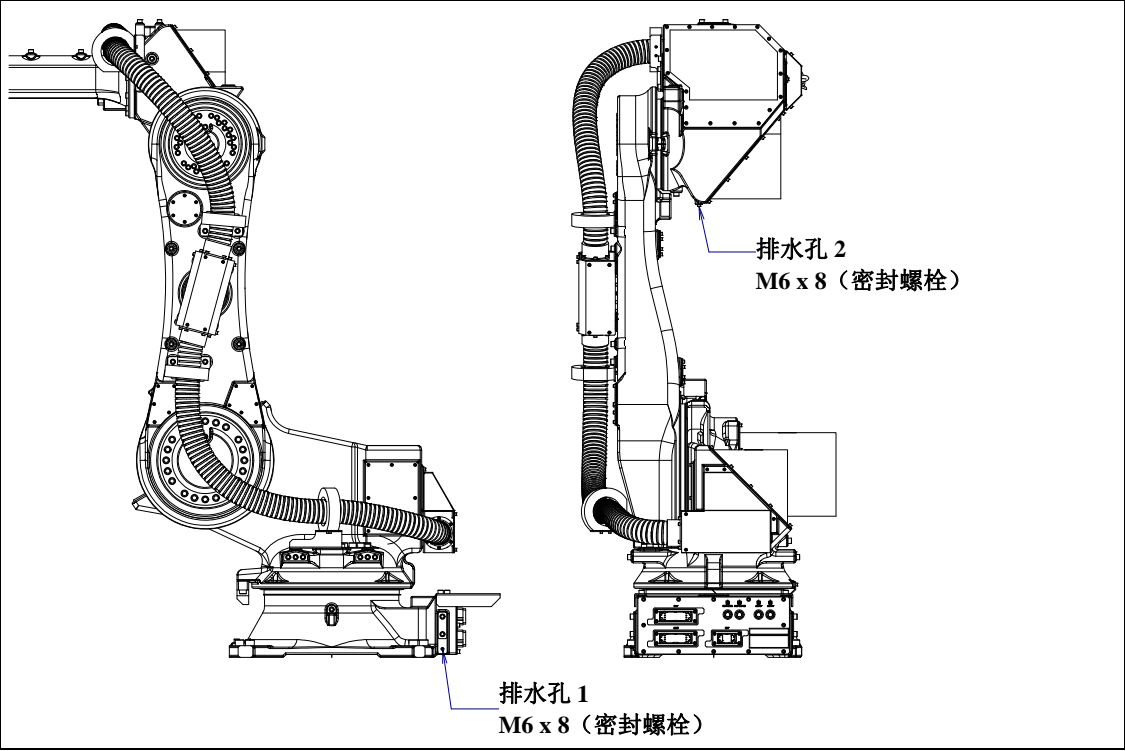
图 7.2.5 (b) 排水孔的检查
