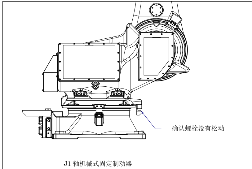
图 7.2.4 (a) 机械式固定制动器、机械式可变制动器的检修
