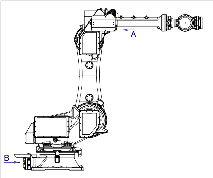
图 5.3 (a) 可选项项电缆用接口的位置（可选项项）
