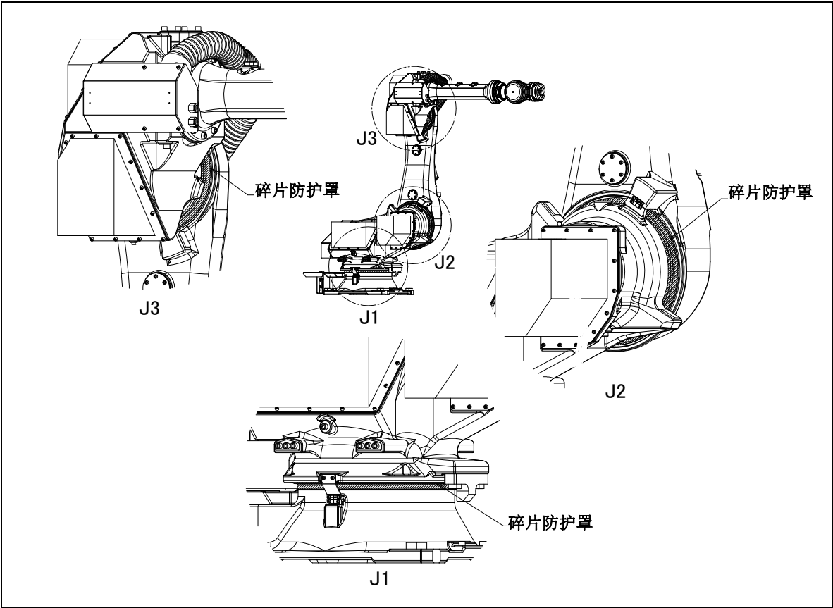
图 7.2.6 (a) 碎片防护罩的检查
