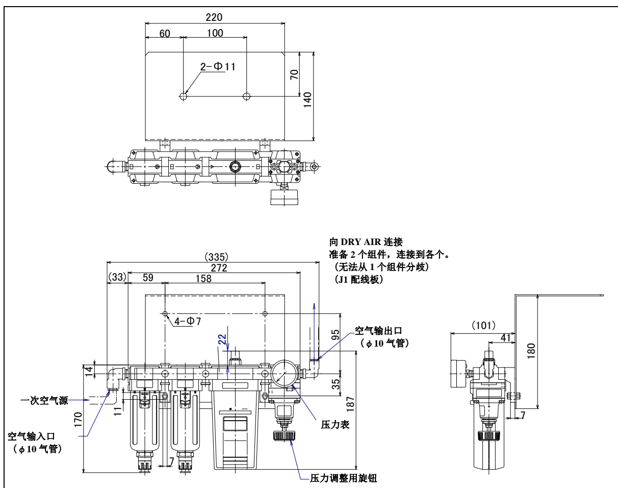
图 5.4 (a) 气压组件用调节器组件的外形尺寸
