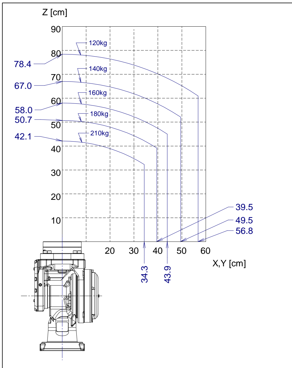
图 3.4 (a) 手腕部允许负载线图 (ISO 法兰盘)
