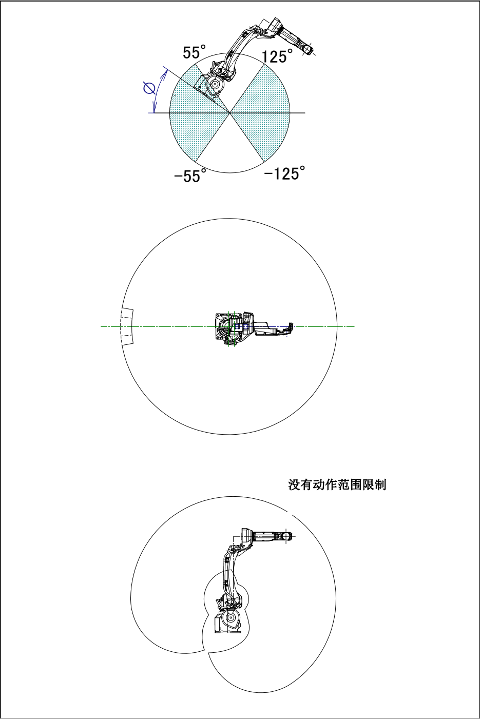
图 3.6 (b) 设置范围 (1) 动作范围图 (ARC Mate 100iD, M-10iD/12) ( -180^\circ \leq \phi \leq -125^\circ , -55^\circ \leq \phi \leq 55^\circ , 125^\circ \leq \phi \leq 180^\circ )
