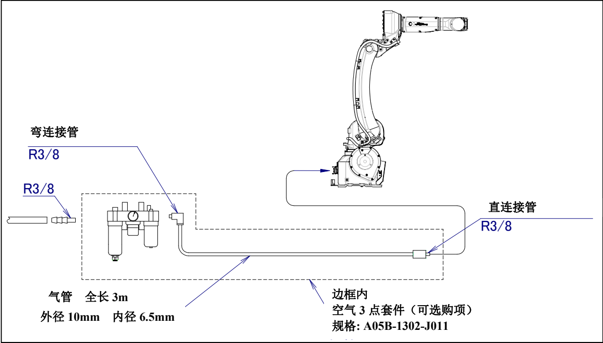
图 5.2 (a) 空气配管（可选项项）
