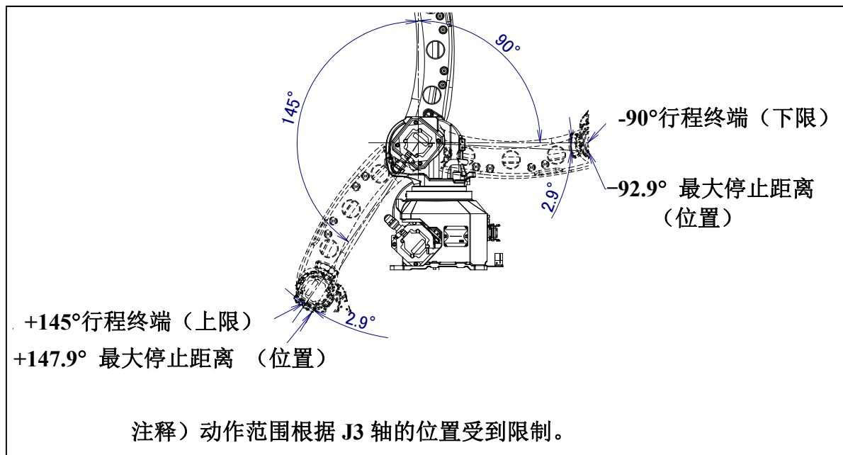
图 3.3 (d) J2 轴可动范围
