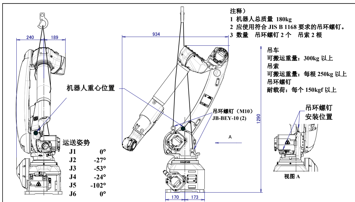
图 1.1 (c) 用吊车搬运 (ARC Mate 100iD/8L, M-10iD/8L)
