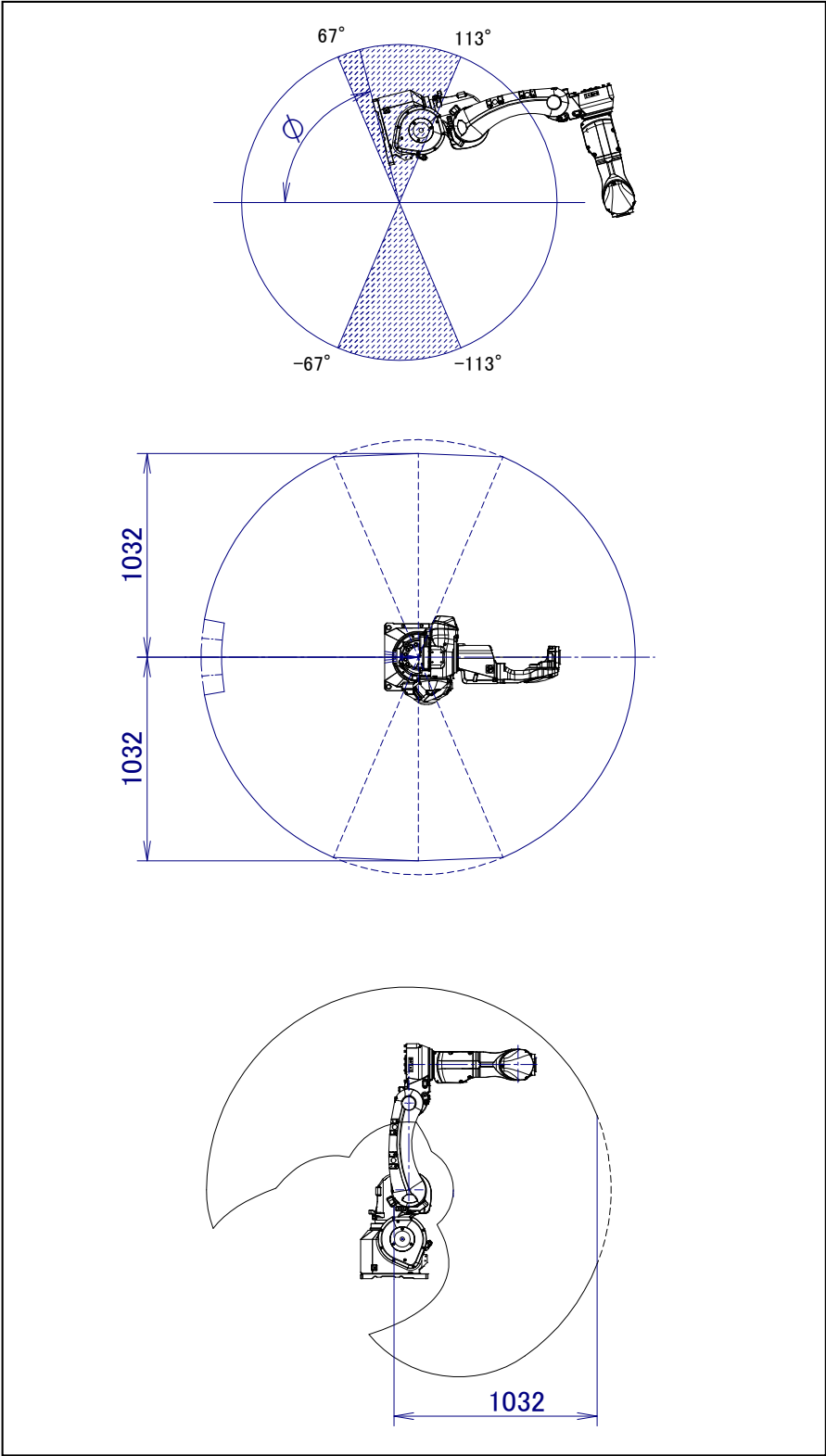
图 3.6 (i) 设置范围 (2) 动作范围图 (ARC Mate 100iD/16S, M-10iD/16S) ( -113^\circ < \phi < -67^\circ , 67^\circ < \phi < 113^\circ )
