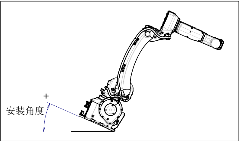
图 1.2.2 (a) 机器人的安装角度
