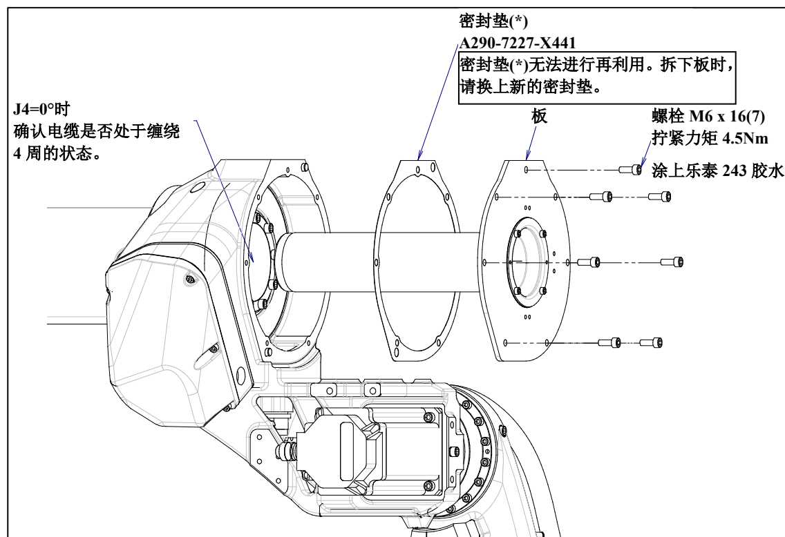
图 8.1 (b) 确认电缆的状态 (J4 轴)
