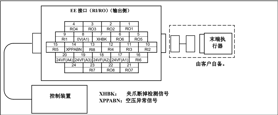
图 5.3 (j) EE 接口(RI/RO)的插脚排列 RI/RO 各 8 点 (指定 A05B-1227- H223#□□, H224#□□时)
