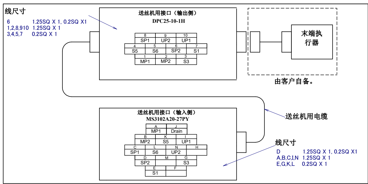
图 5.3 (l) DAIHEN 送丝机(W/F)用接口的插针排列（可选项项） (指定 A05B-1227- H205#□□D 时)
