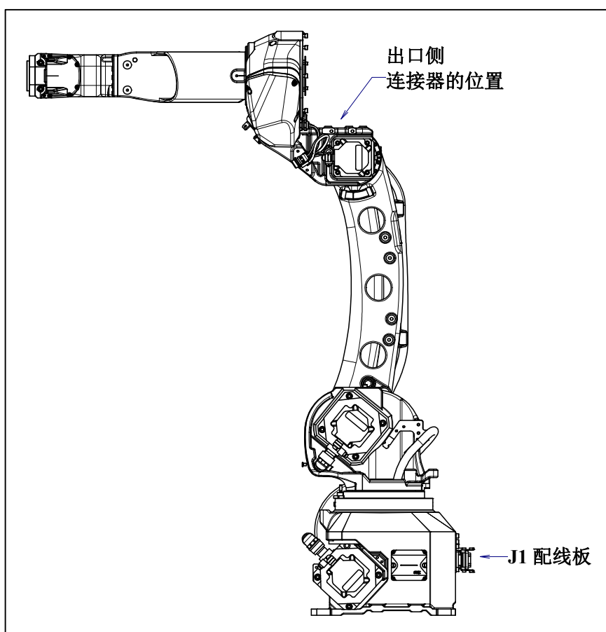
图 5.3 (a) 可选项项电缆用接口的位置（可选项项）
