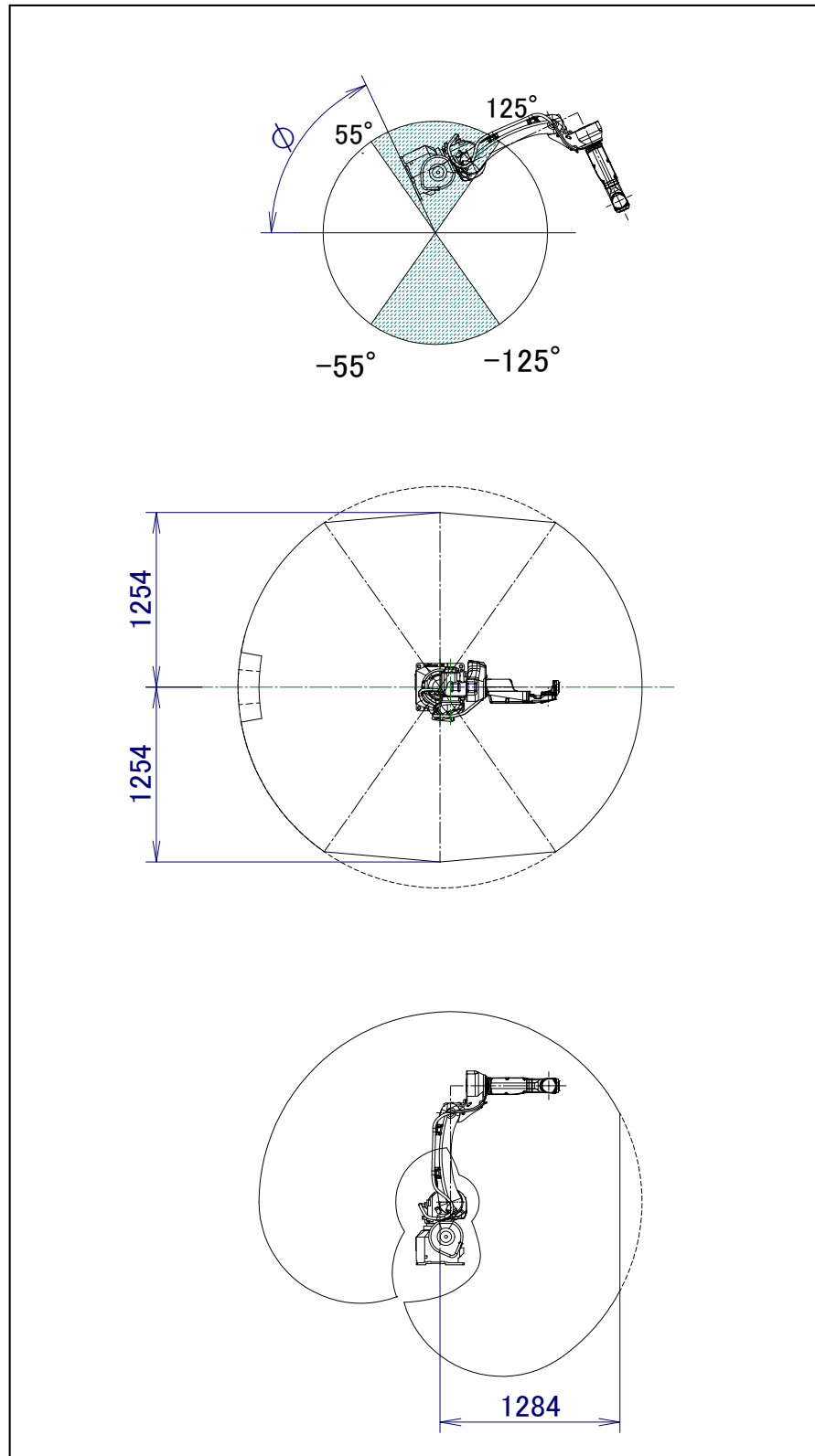
图 3.6 (c) 设置范围 (2) 动作范围图 (ARC Mate 100iD, M-10iD/12) (-125^\circ < \phi < -55^\circ, 55^\circ < \phi < 125^\circ)
