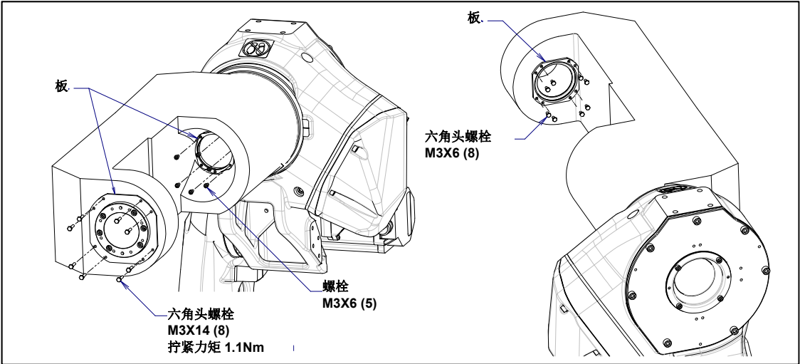
图 7.3.3 (b) 手腕外罩安装螺栓的拆除
