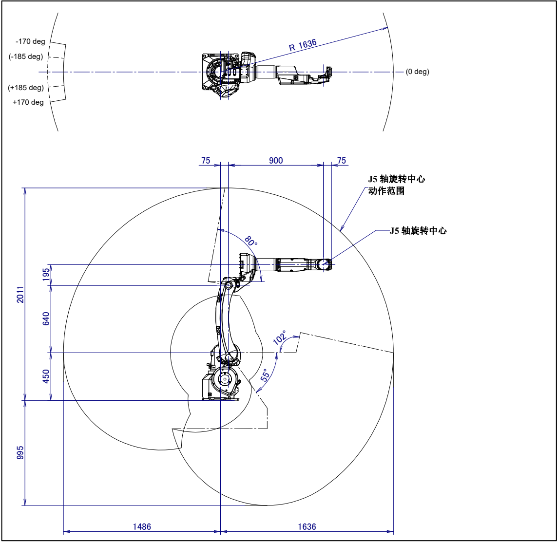
图 3.2 (b) 动作范围图 (ARC Mate 100iD/10L, M-10iD/10L)
