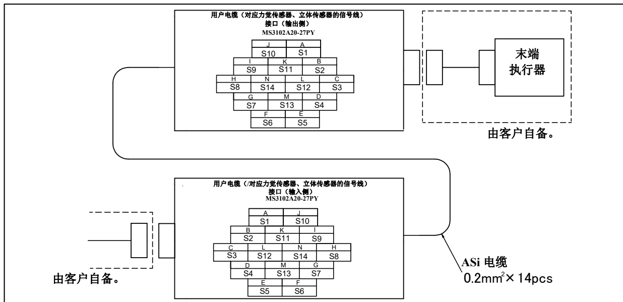
图 5.3 (n) 用户电缆 (对应应力觉传感器、立体传感器的信号线) (ASi)接口的插针排列 (可选项) (指定 A05B-1227-H222#□□□时)
