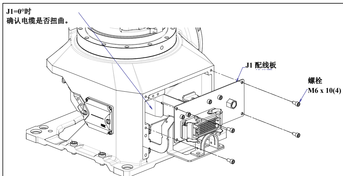
图 8.1 (a) 确认电缆的状态 (J1 轴)
