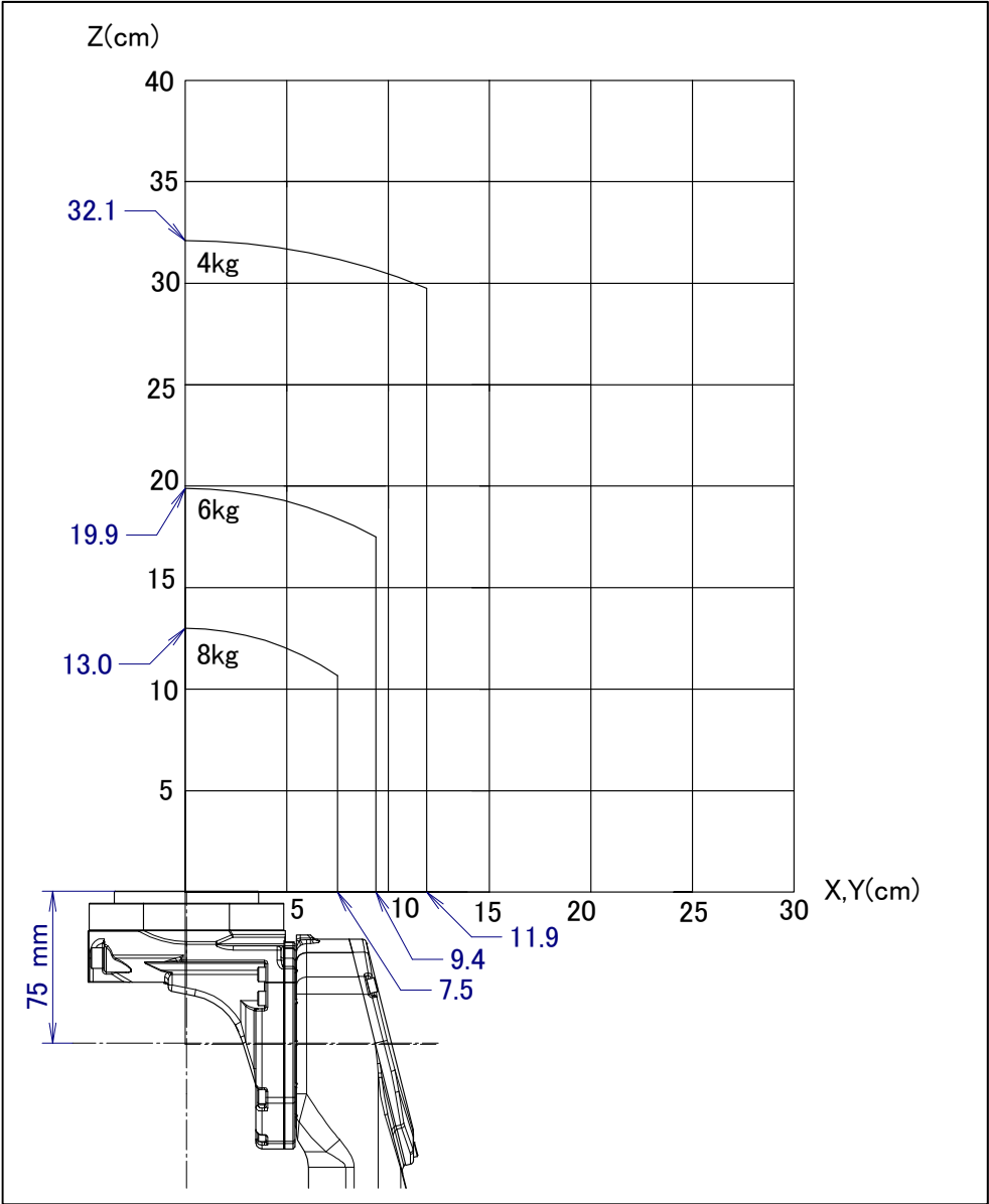
图 3.5 (d) 手腕部允许负载线图 (ARC Mate 100iD/8L, M-10iD/8L)
