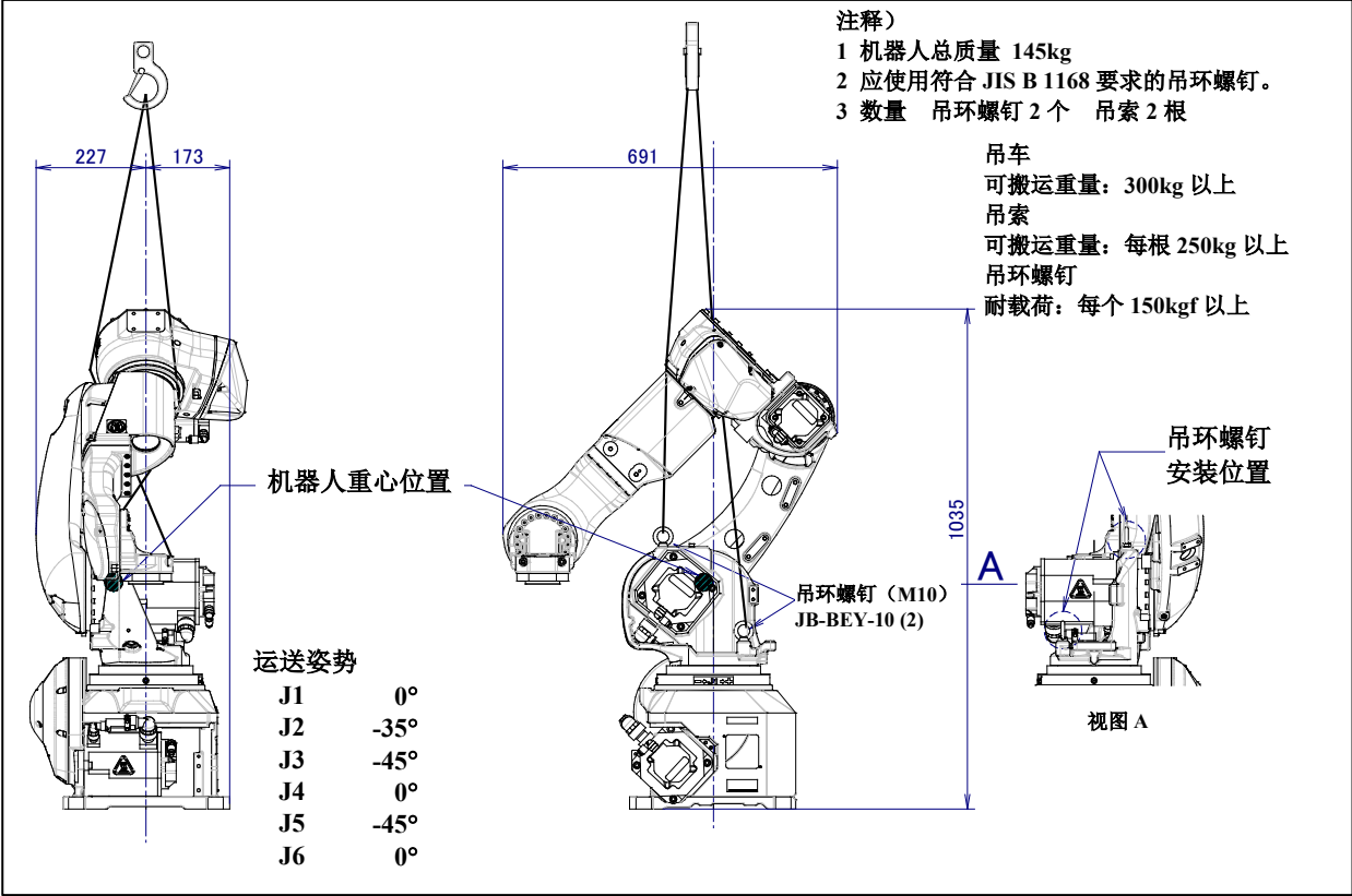
图 1.1 (d) 用吊车搬运 (ARC Mate 100iD/16S, M-10iD/16S)
