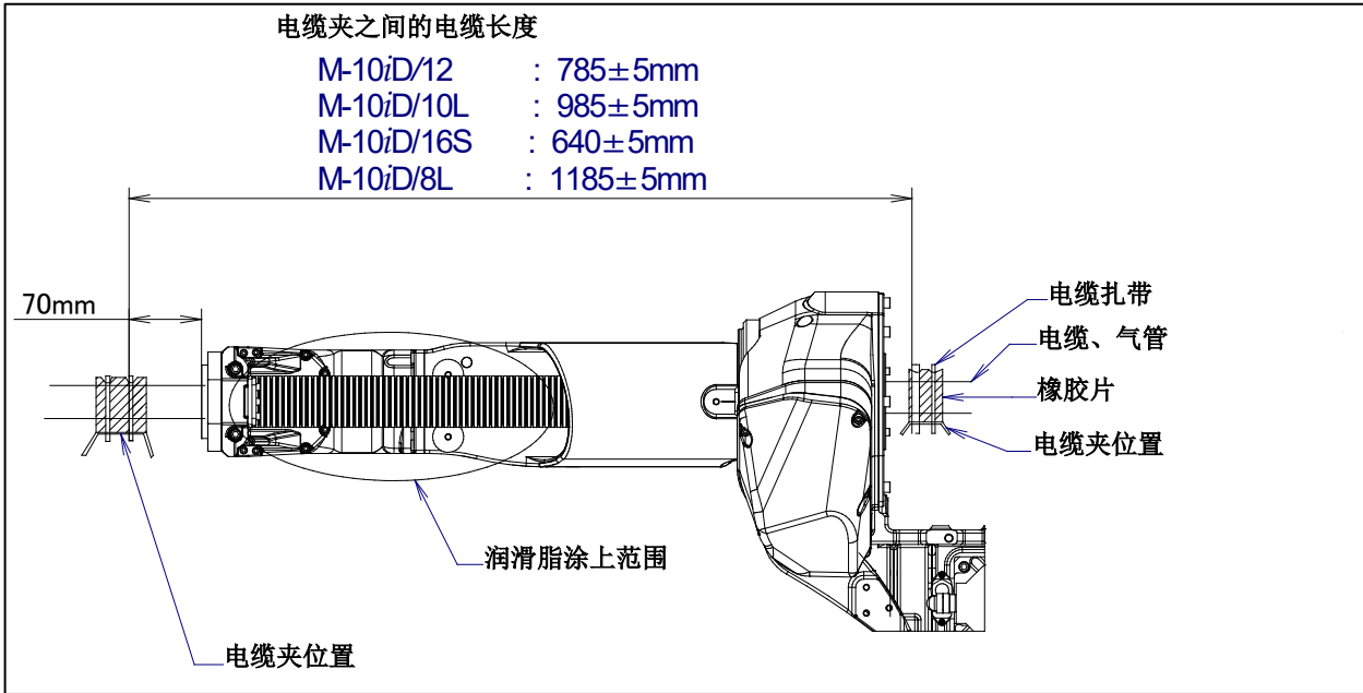
图 10.1 (a) 电缆夹之间的距离
