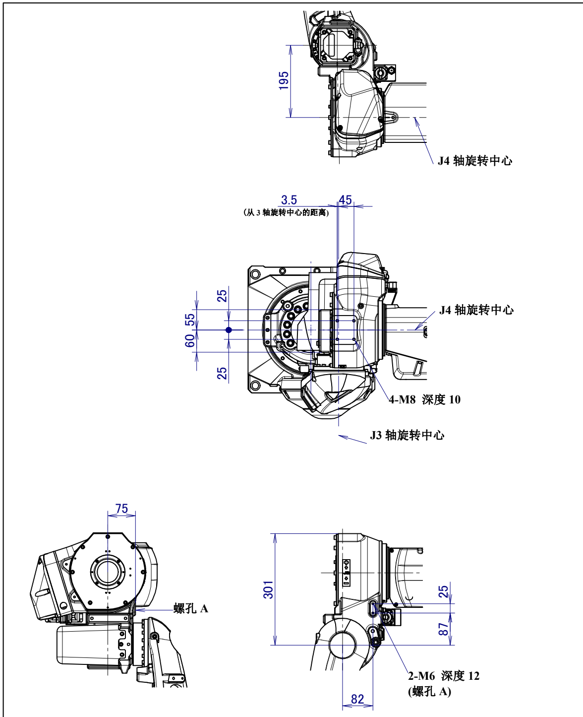
图 4.2 (d) 设备安装面尺寸 (ARC Mate 100iD/16S, M-10iD/16S)
