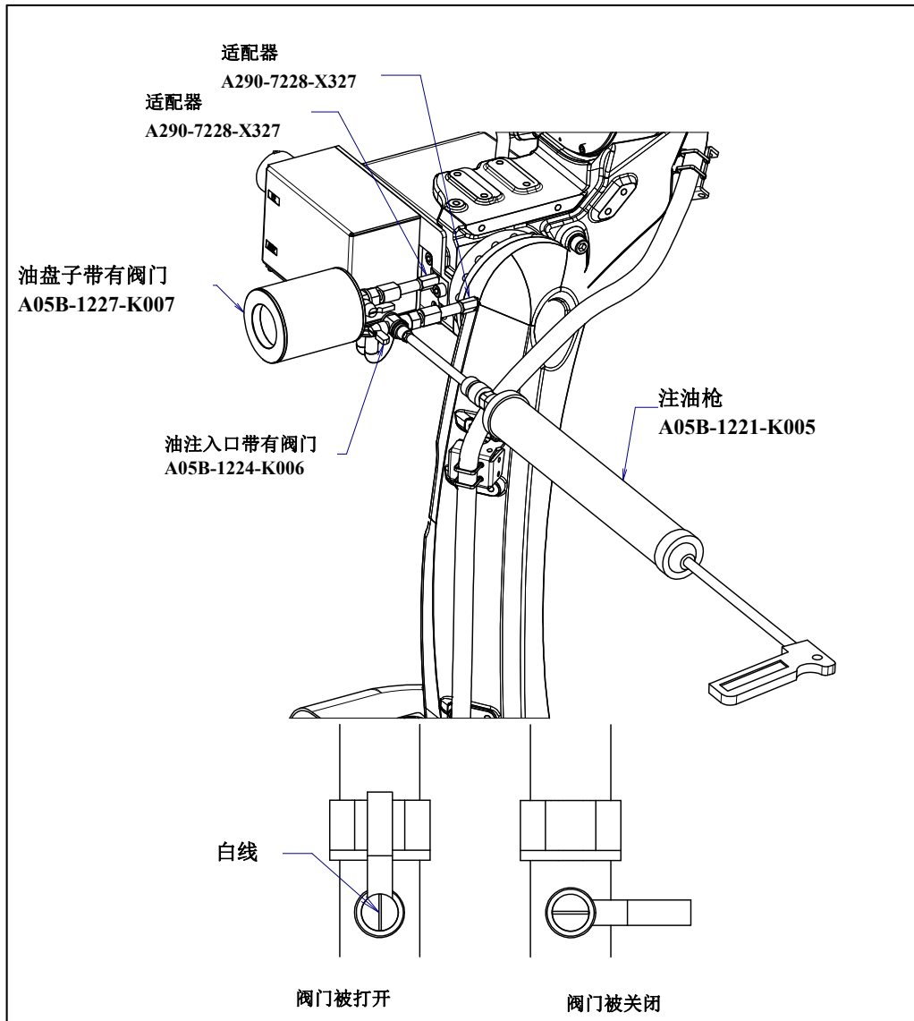
图 7.3.2.3 (c) 用注油枪供油 (J3 轴减速机的供油) (地面安装的例)
