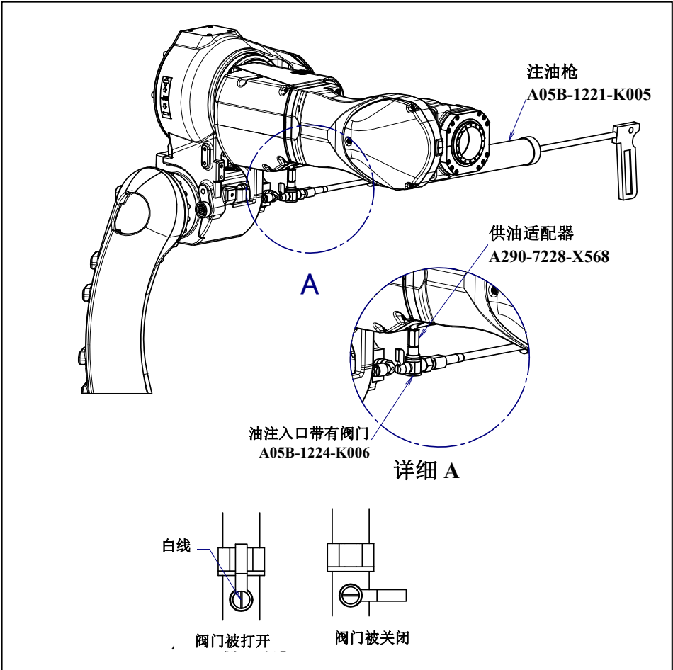
图 7.3.2.8 (b) 用注油枪供油
