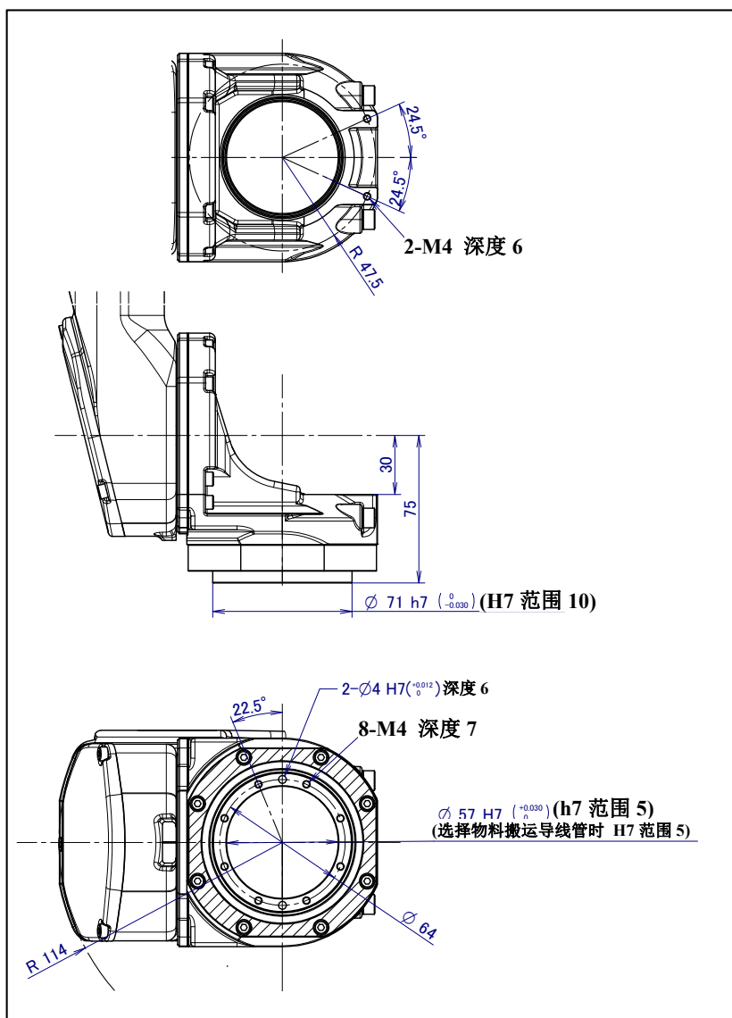
图 4.1 (a) 末端执行器安装面 (ARC Mate 100iD, M-10iD/12, ARC Mate 100iD/10L, M-10iD/10L, ARC Mate 100iD/8L, M-10iD/8L)
