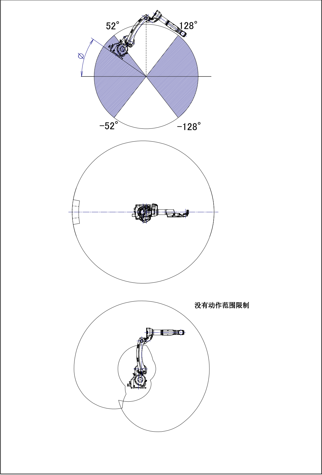
图 3.6 (d) 设置范围 (1) 动作范围图 (ARC Mate 100iD/10L, M-10iD/10L) ( -180^\circ \leq \phi \leq -128^\circ , -52^\circ \leq \phi \leq 52^\circ , 128^\circ \leq \phi \leq 180^\circ )
