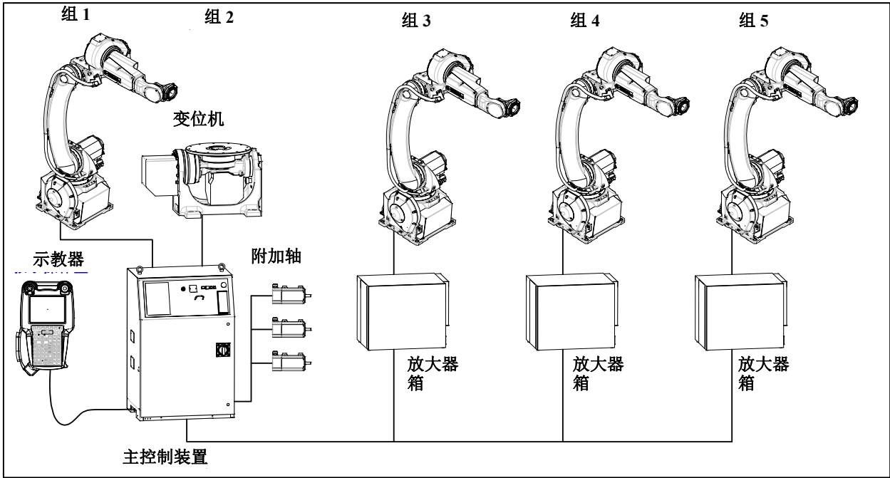
图 D (a) 多台机器人控制
