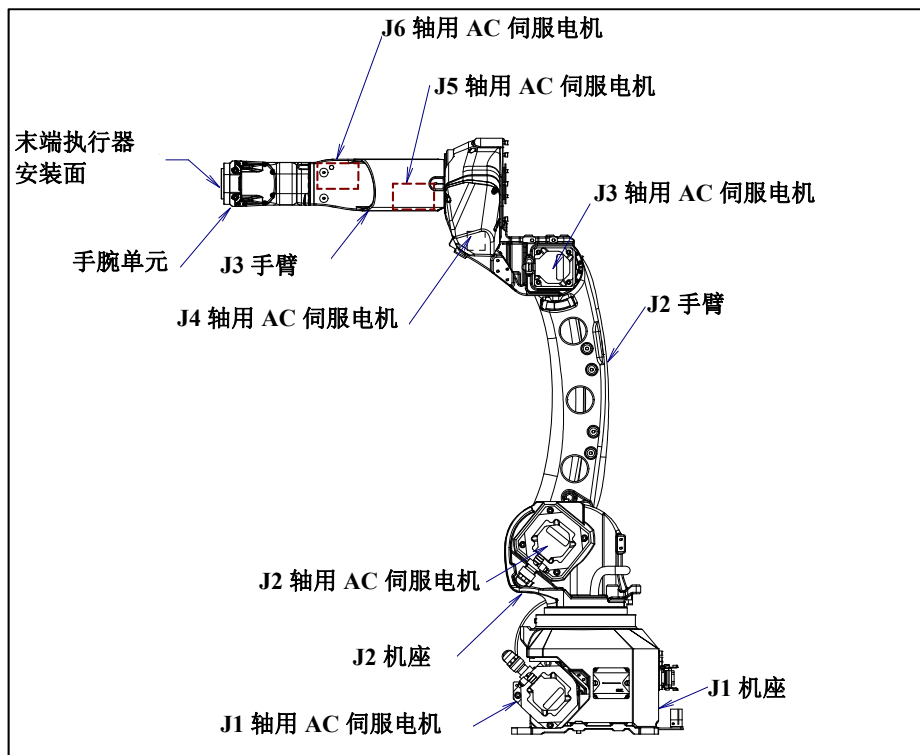
图 3.1 (a) 机构部的构成
