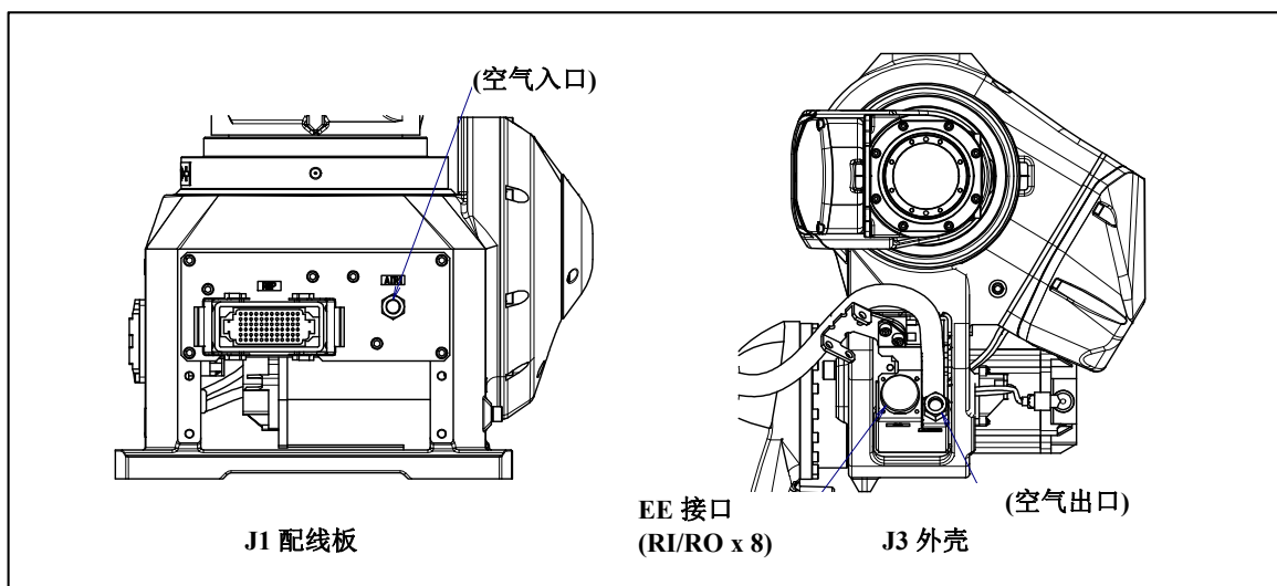
图 5.3 (d) 可选项项电缆用接口 (指定 A05B-1227- H221#□□时)
