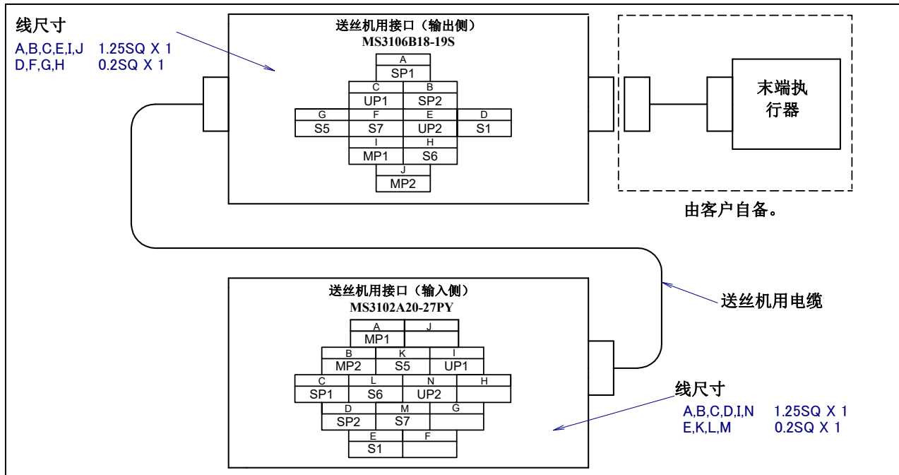
图 5.3 (m) FANUC 丝机(W/F)用接口的插针排列 (可选项) (A05B-1227- H205#□□H 指定時)
