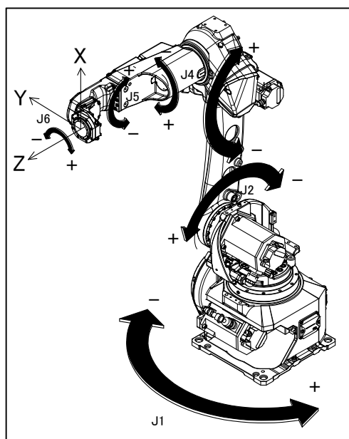
图 3.1 (b) 各轴坐标和机械接口坐标
