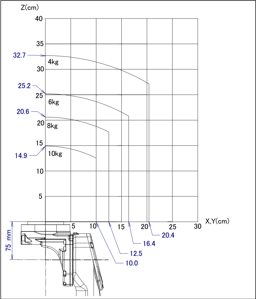
图 3.5 (c) 手腕部允许负载线图 (ARC Mate 100iD/10L, M-10iD/10L)
