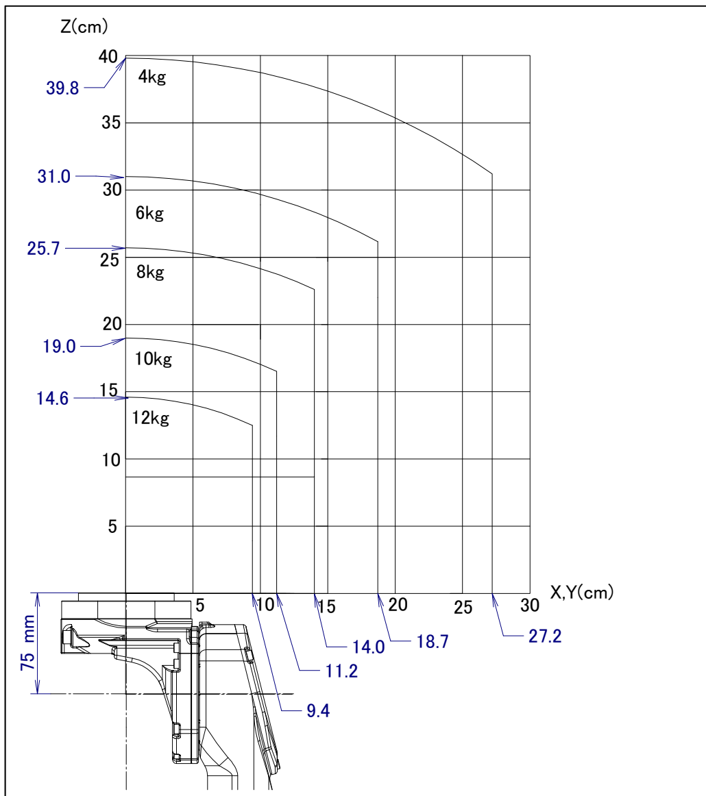
图 3.5 (a) 手腕部允许负载线图 (ARC Mate 100iD, M-10iD/12)
