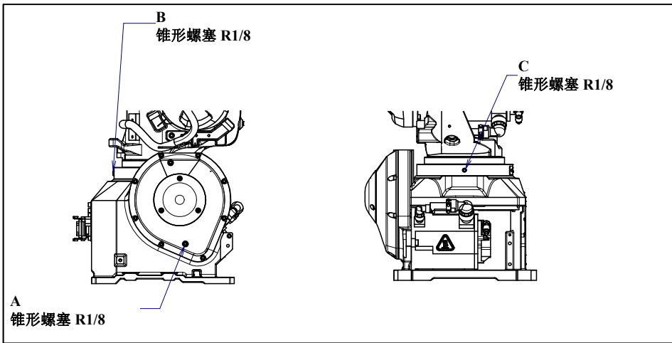
图 7.3.2.5 (a) J1 轴齿轮箱的供脂部位
