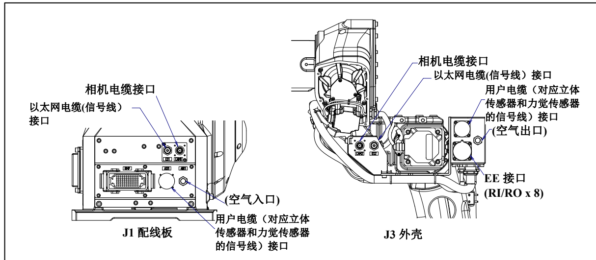
图 5.3 (g) 可选项电缆用接口(指定 A05B-1227-H224#□□□时)
