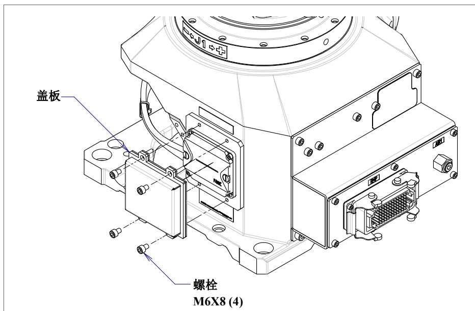
图 7.3.1 (b) 电池盖板的拆除
