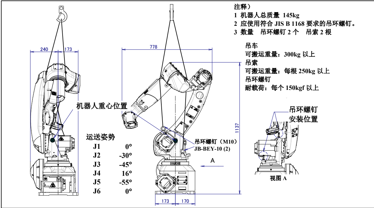
图 1.1 (a) 用吊车搬运（ARC Mate 100iD, M-10iD/12）
