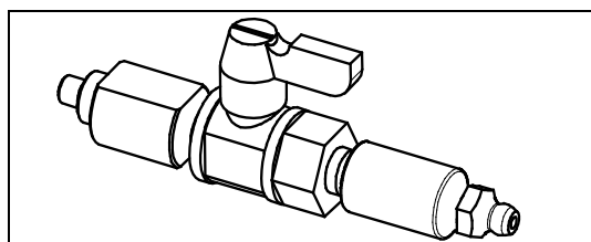
图 7.3.2.7 (c) 油注入口带有阀门 (A05B-1224-K006)
