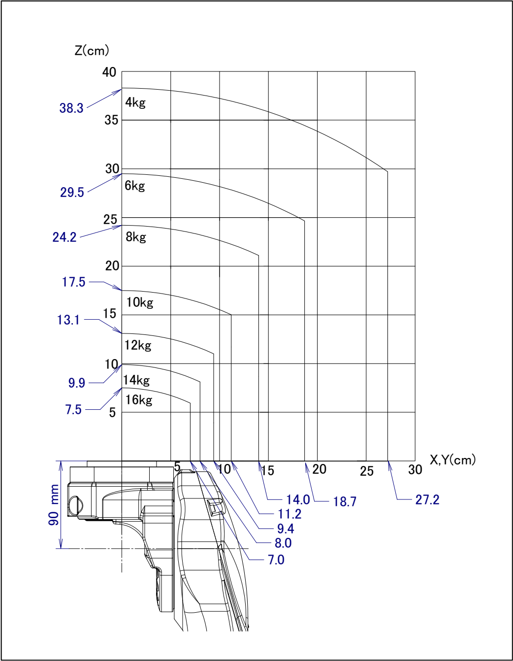
图 3.5 (e) 手腕部允许负载线图 (ARC Mate 100iD/16S, M-10iD/16S)
