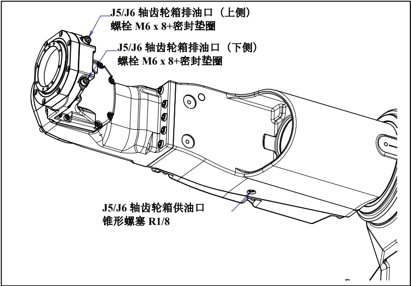
图 7.3.2.7 (a) 供油口和排油口
