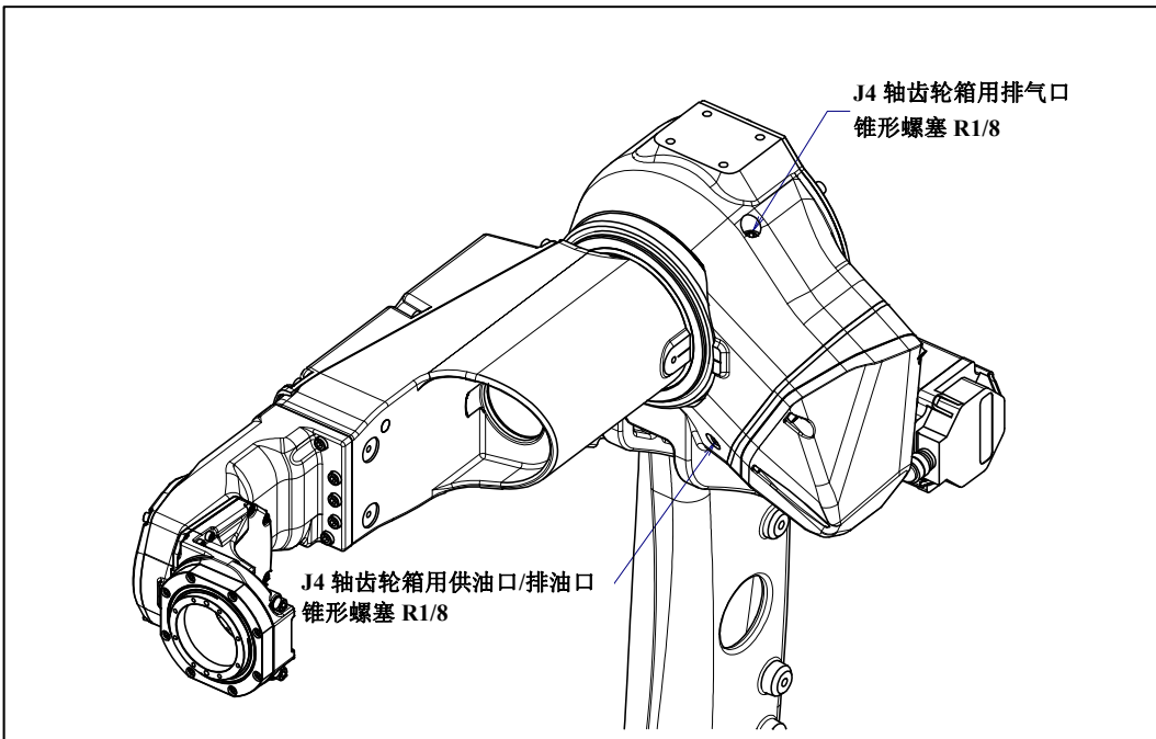
图 7.3.2.6 (a) J4 轴齿轮箱的供脂部位
