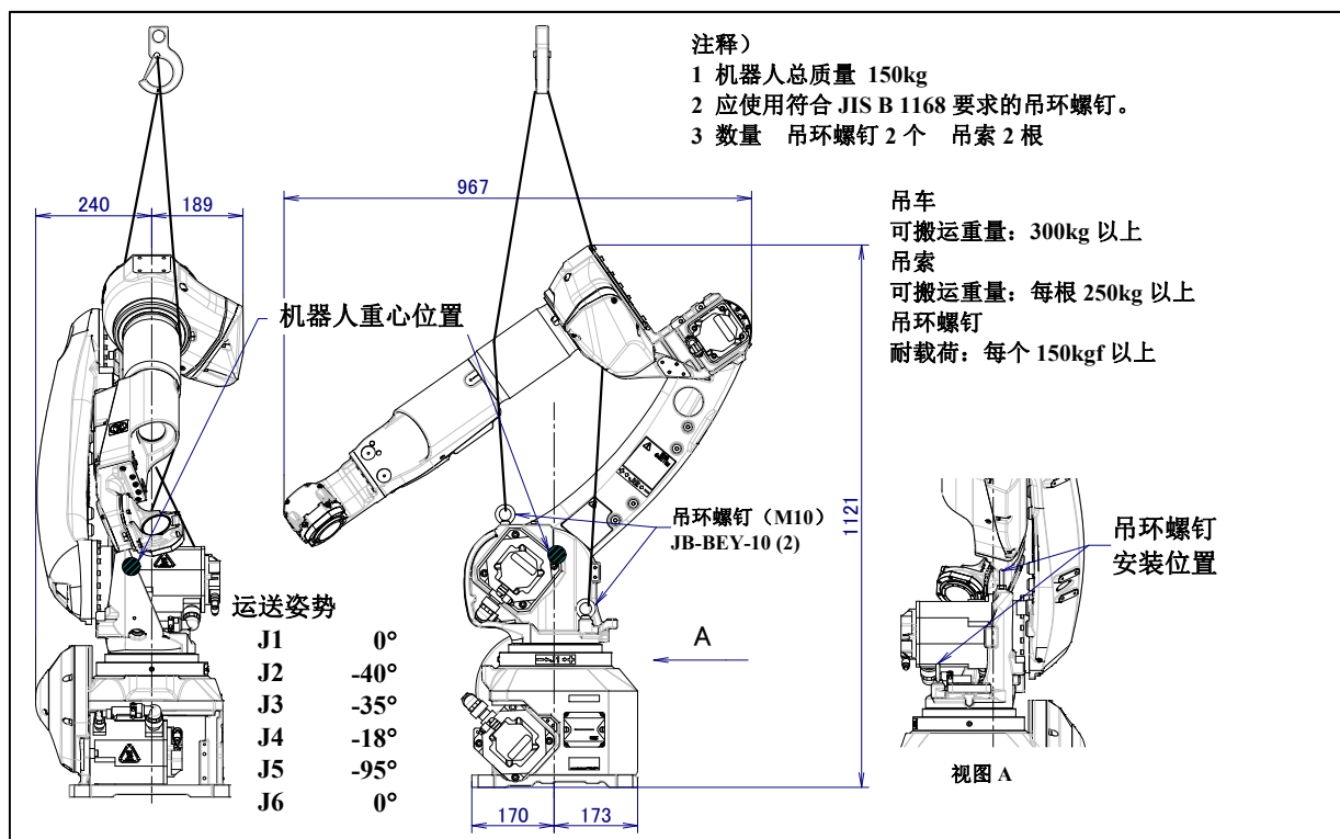
图 1.1 (b) 用吊车搬运 (ARC Mate 100iD/10L, M-10iD/10L)
