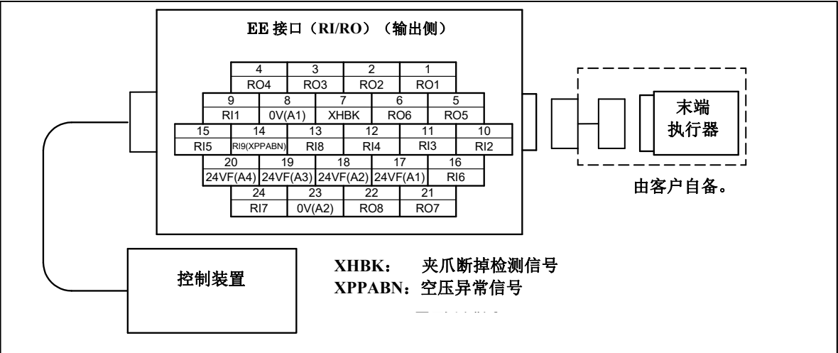
图 5.3 (i) EE 接口(RI/RO)的插针排列 RI/RO 各 8 点 (可选项) (指定 A05B-1227- H221#□□, H222#□□时)
