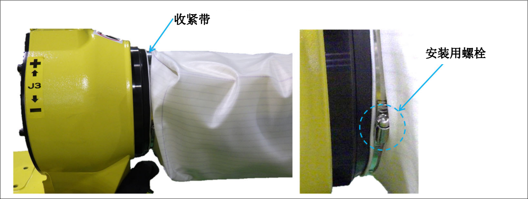
图 7.3.3 (a) 手腕外罩收紧带的拆除
