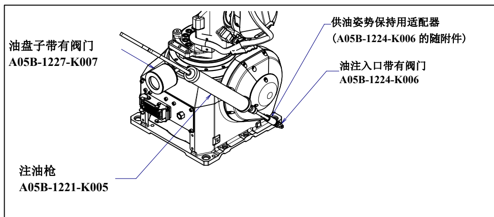
图 7.3.2.3 (b) 用注油枪供油 (J1 轴齿轮箱的供油)
