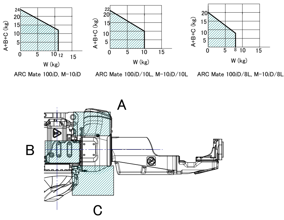
图 4.2 (a) 负载条件
