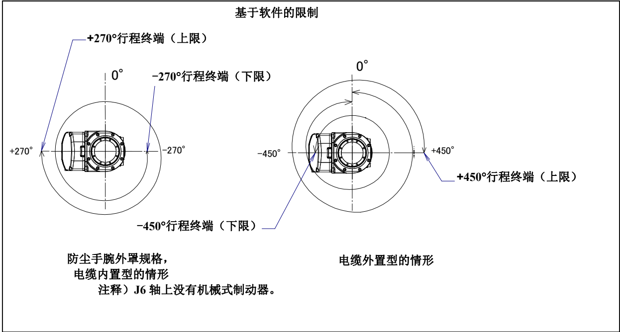
图 3.3 (h) J6 轴可动范围
