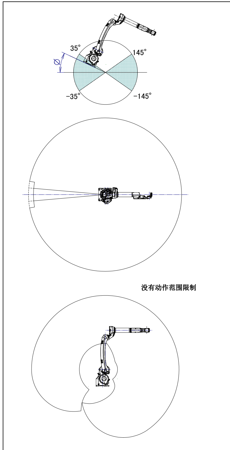
图 3.6 (f) 设置范围 (1) 动作范围图 (ARC Mate 100iD/8L, M-10iD/8L) (-180^\circ \leq \phi \leq -145^\circ, -35^\circ \leq \phi \leq 35^\circ, 145^\circ \leq \phi \leq 180^\circ)
