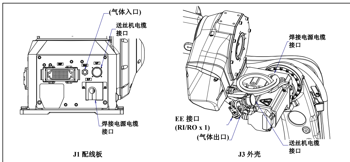
图 5.3 (c) 可选项项电缆用接口 (指定 A05B-1227-H205#□□时)
