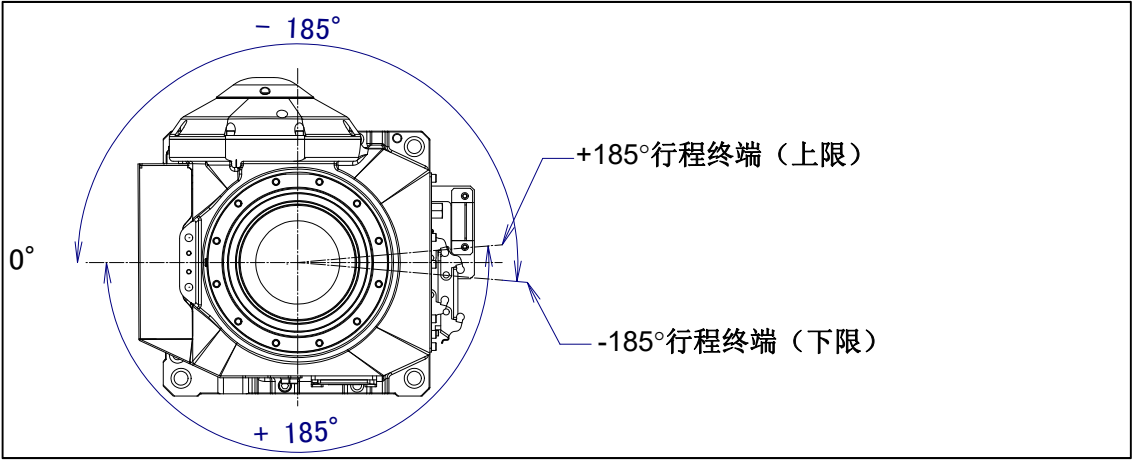
图 3.3 (b) J1 轴可动范围（未选择机械式制动器时）
