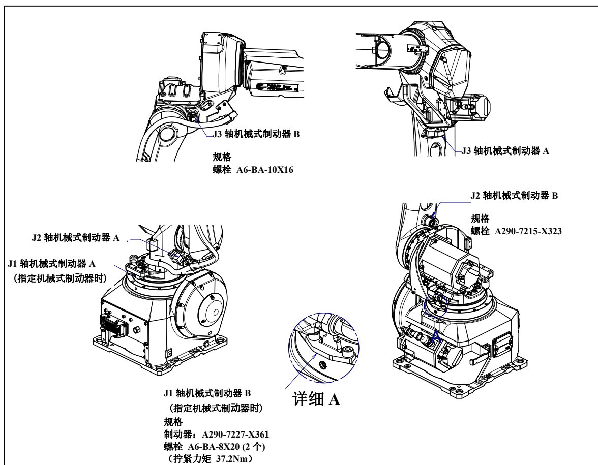
图 3.3 (a) 机械式制动器的位置
