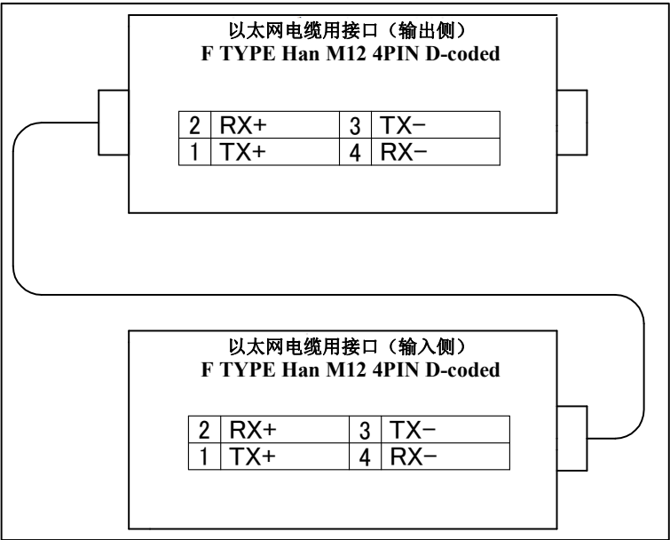
图 5.3 (o) 以太网电缆(ES)用接口的插针排列（可选项） (指定 A05B-1227-H222#12, H222#LG 时)
