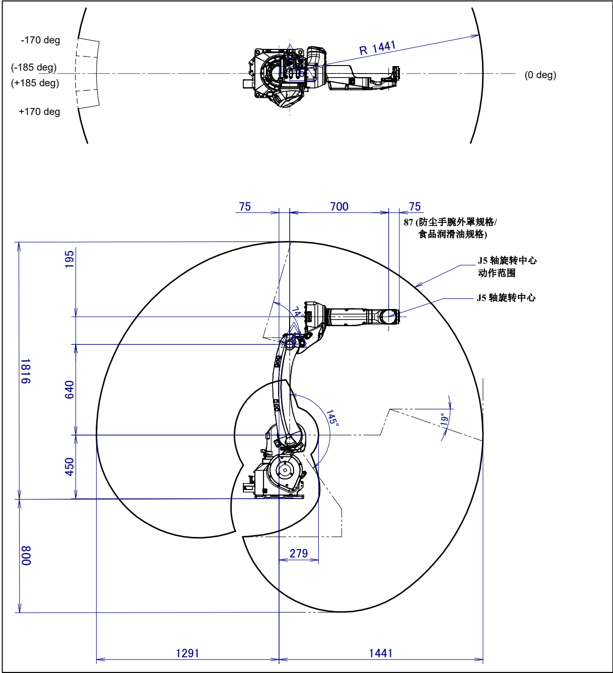
图 3.2 (a) 动作范围图 (ARC Mate 100iD, M-10iD/12)
