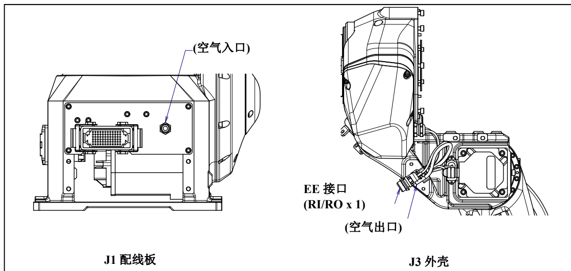
图 5.3 (b) 可选项项电缆用接口 (指定 A05B-1227-H201#□□, H291#12 时)
