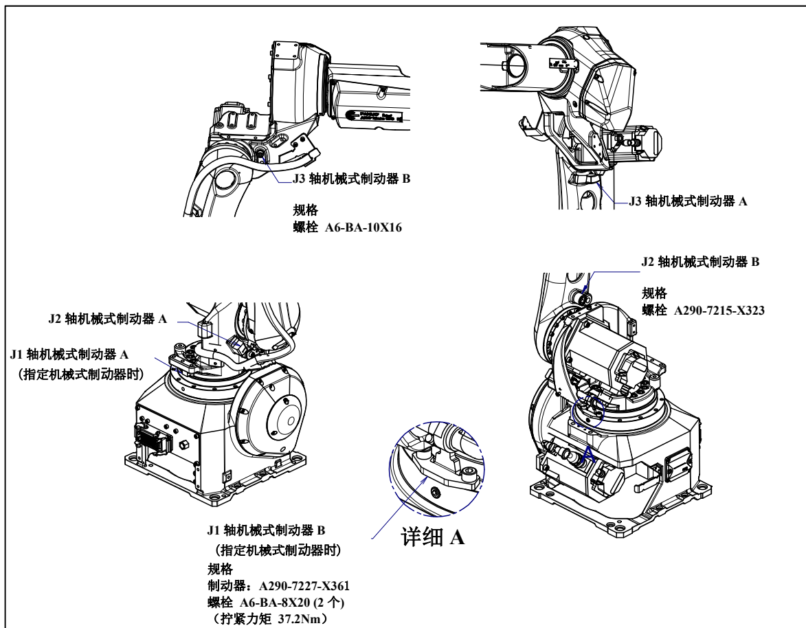
图 7.2.4 (a) 机械式固定制动器、机械式可变制动器的检修
