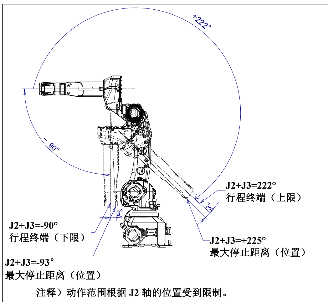
图 3.3 (e) J3 轴可动范围
