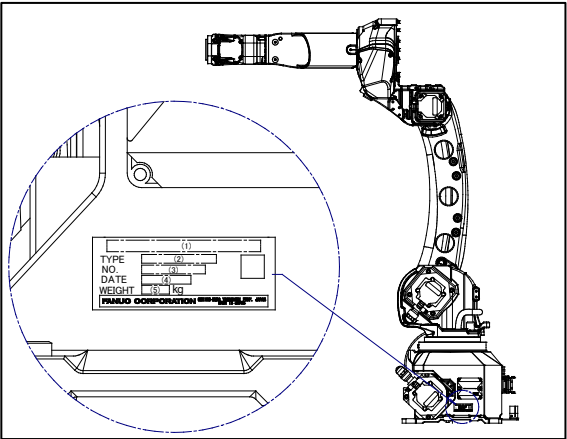
机构部规格编号标贴位置
