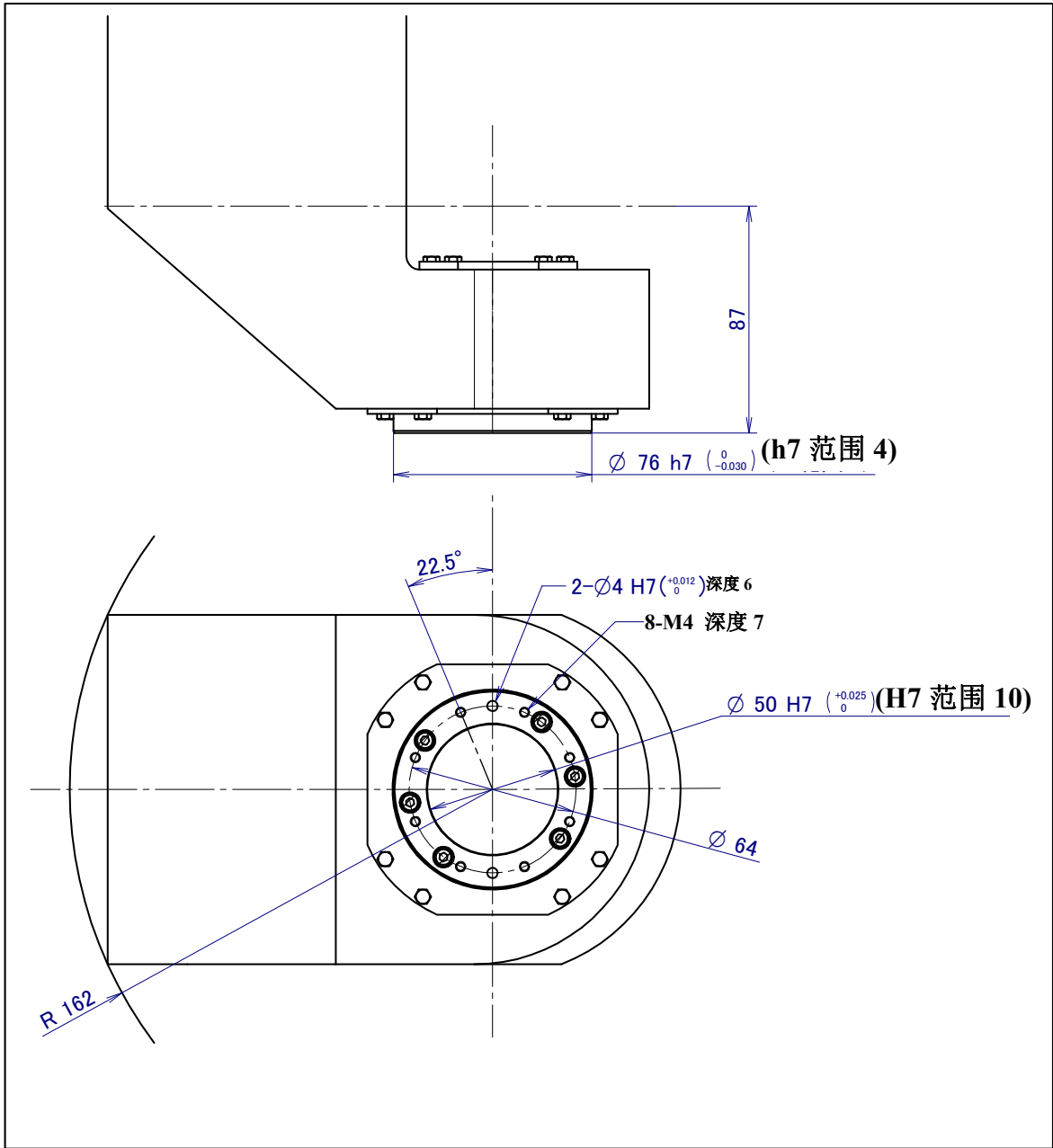
图 4.1 (b) 末端执行器安装面 (M-10iD/12 防尘手腕外罩规格)
