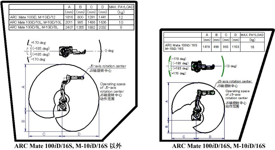
图 4 (f) 动作范围标签
