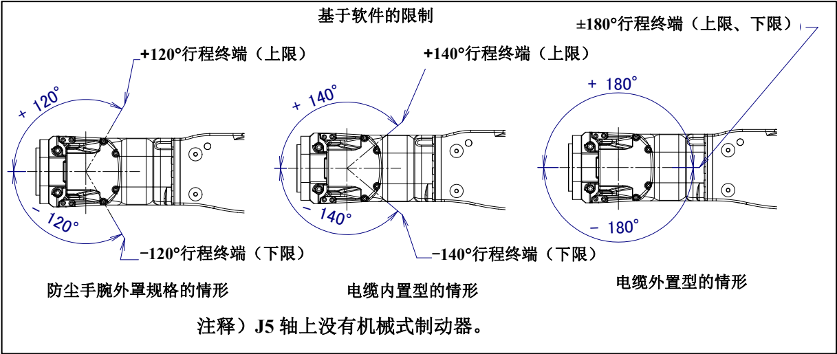
图 3.3 (g) J5 轴可动范围
