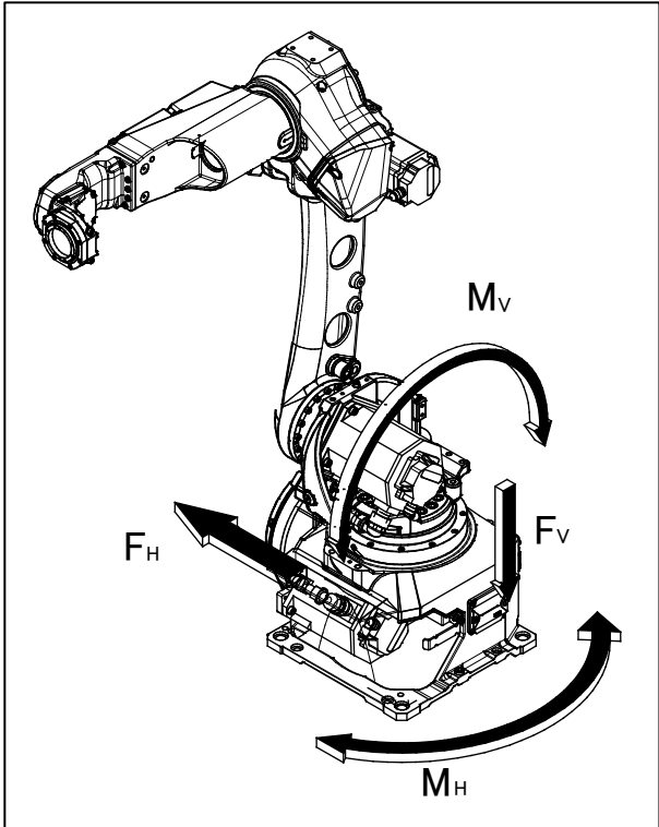
图 1.2.1 (b) 作用于机器人机座的力和力矩
