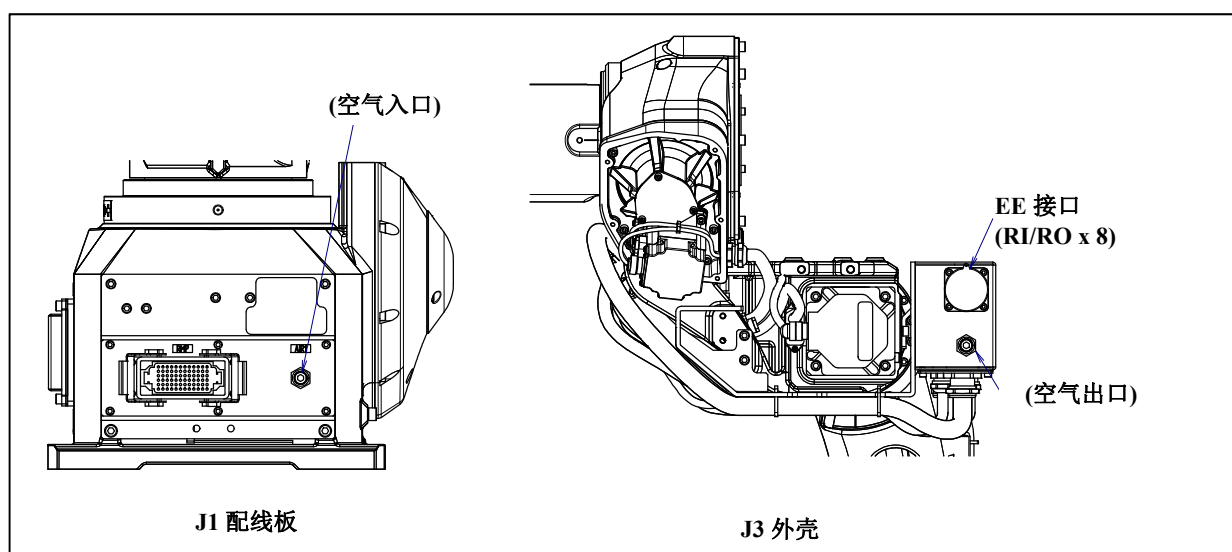
图 5.3 (f) 可选项项电缆用接口(指定 A05B-1227-H223#□□时)
