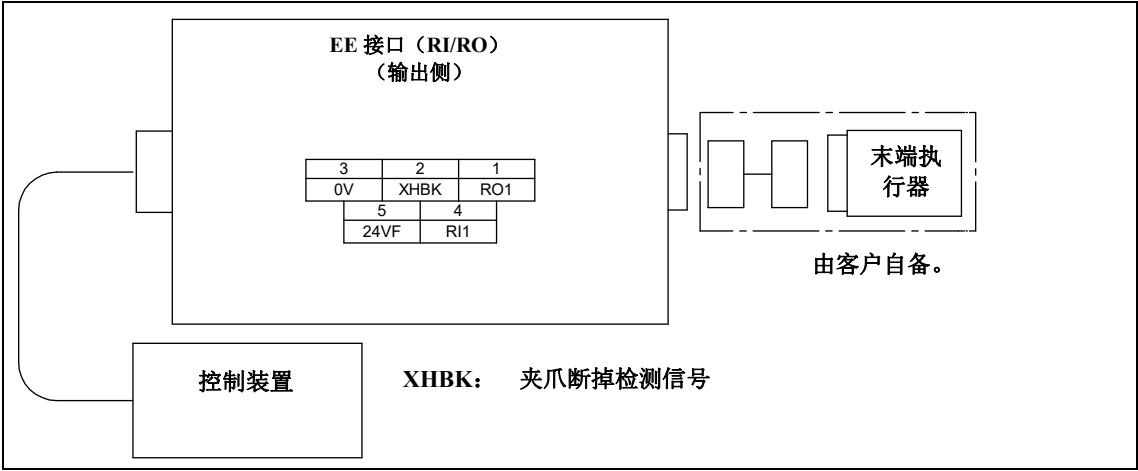
图 5.3 (h) EE 接口(RI/RO)的插针排列 RI/RO 各 1 点 (可选项) (指定 A05B-1227-H201#□□, H205#□□, H291#12 时)
