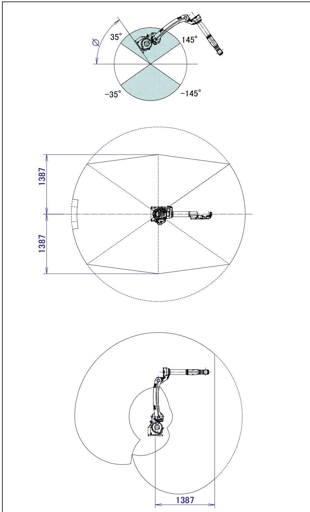
图 3.6 (g) 设置范围 (2) 动作范围图 (ARC Mate 100iD/8L, M-10iD/8L) (-145^\circ < \phi < -35^\circ, 35^\circ < \phi < 145^\circ)
