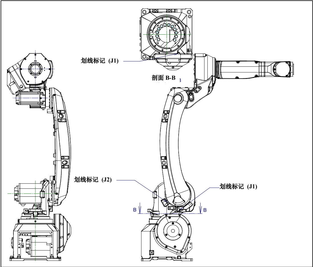
图 8.3 (b) 各轴的对合标记位置
