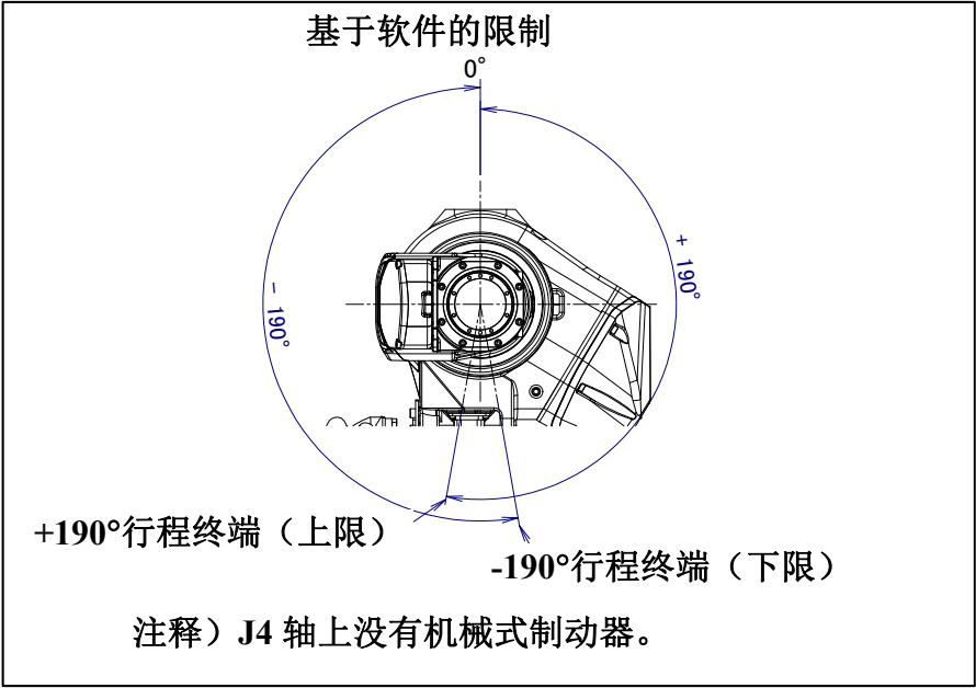
图 3.3 (f) J4 轴可动范围
