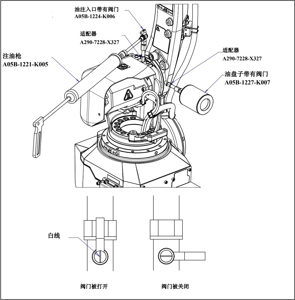
图 7.3.2.3 (b) 用注油枪供油（J2 轴减速机的供油）（地面安装的例）
