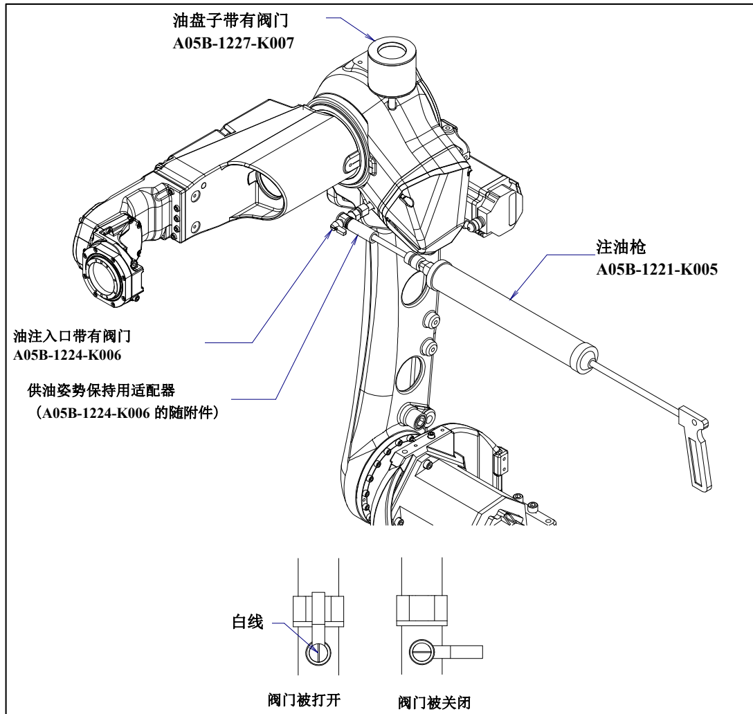
图 7.3.2.6 (b) 用注油枪供油 (J4 轴齿轮箱的供油)
