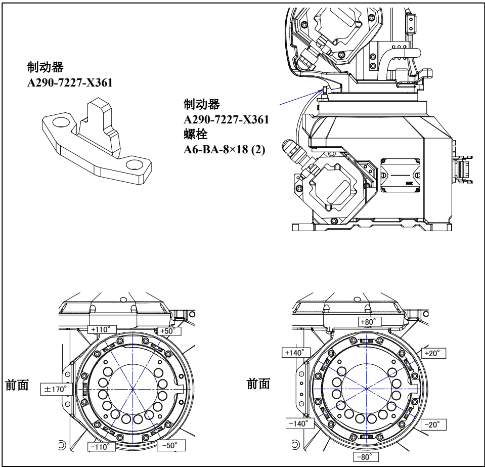
图 6.2.1 (a) J1 轴机械式可变制动器的安装
