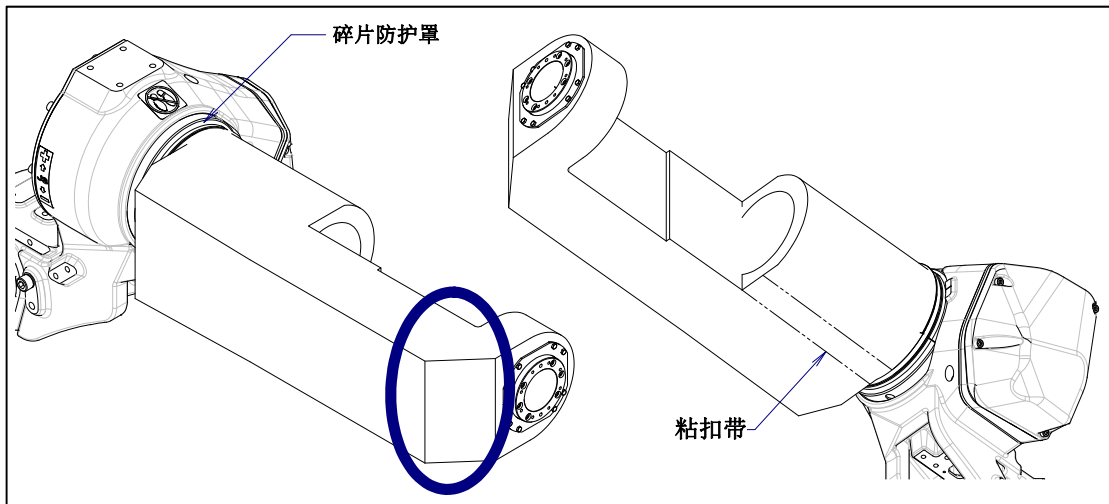
图 7.2.5 (a) 手腕外罩和碎片防护罩的确认部位
