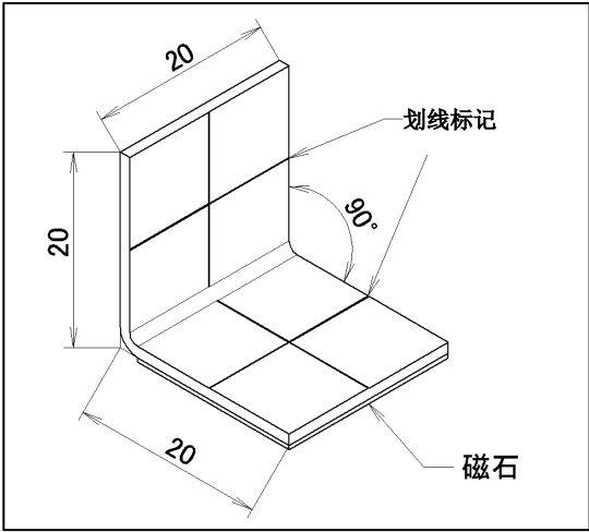
图 8.3 (c) 划线标记定位夹具的外观
