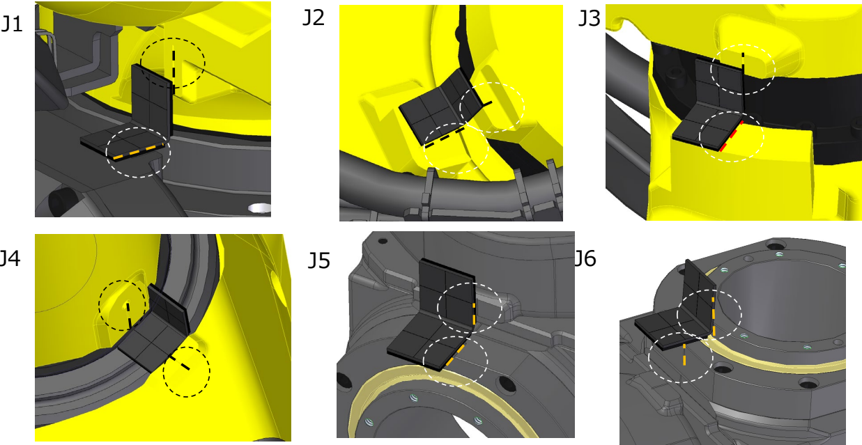
图 8.3 (d) 划线标记定位夹具的使用方法
