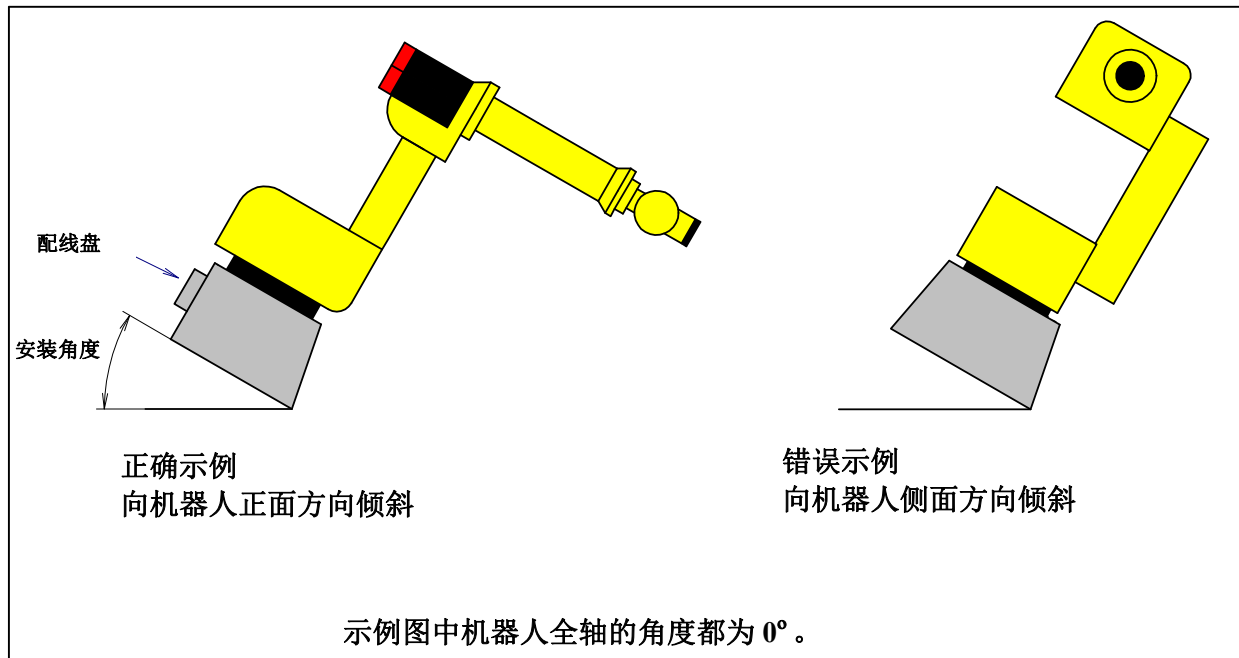
图 3.6 (a) 机器人的壁挂、倾斜角安装的方向
