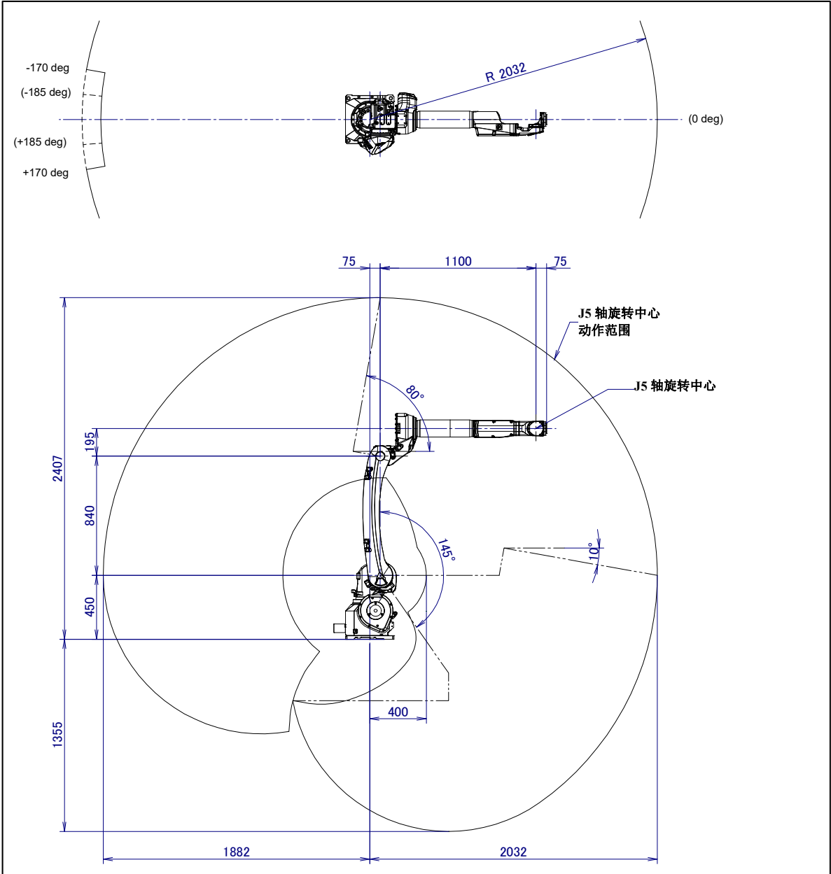
图 3.2 (c) 动作范围图 (ARC Mate 100iD/8L, M-10iD/8L)
