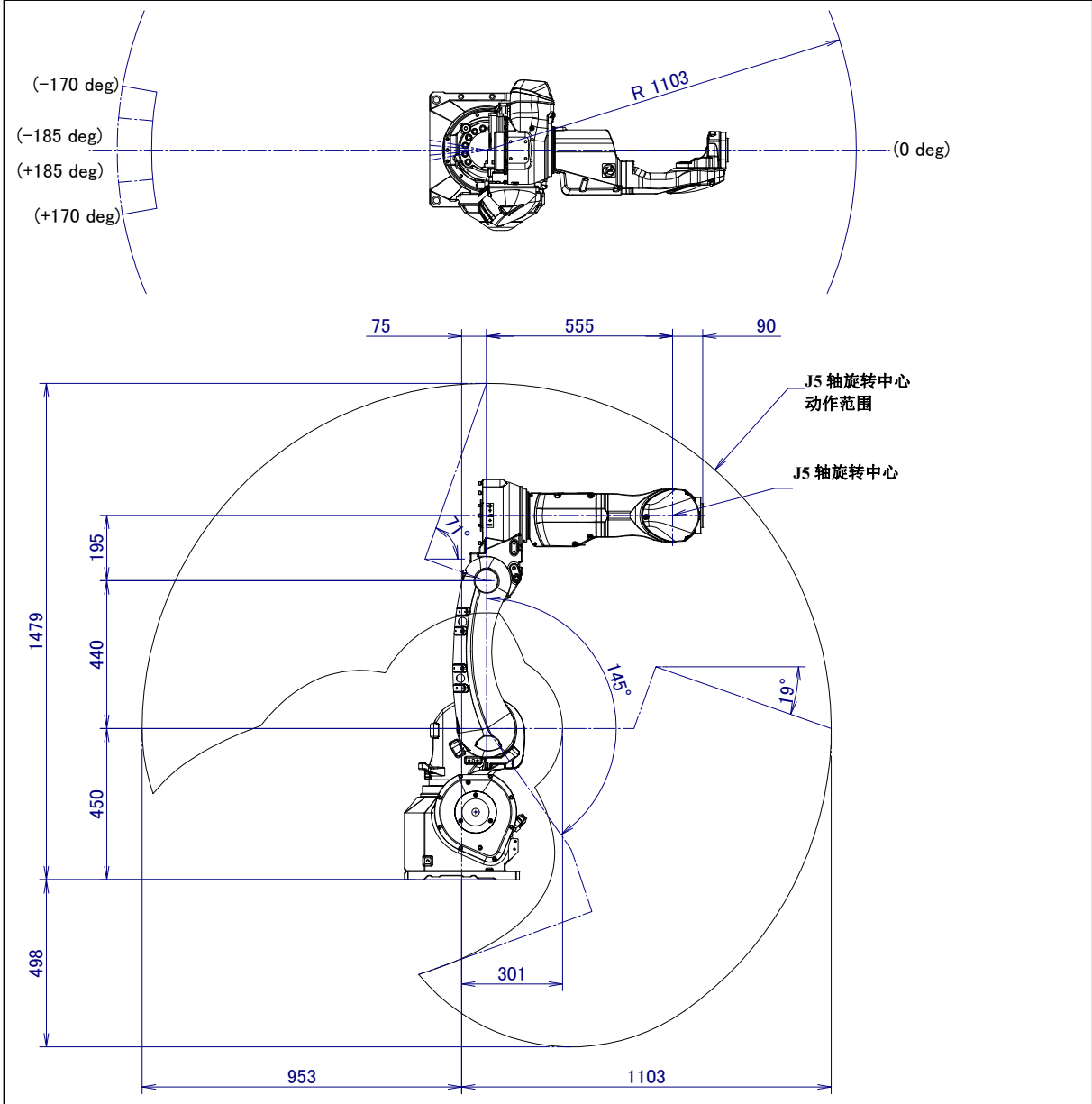
图 3.2 (d) 动作范围图 (ARC Mate 100iD/16S, M-10iD/16S)
