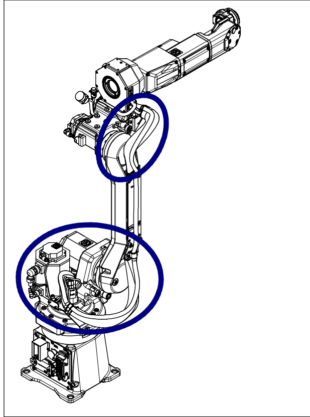
图 7.2.3 (a) 机构部内电缆的检修部位
