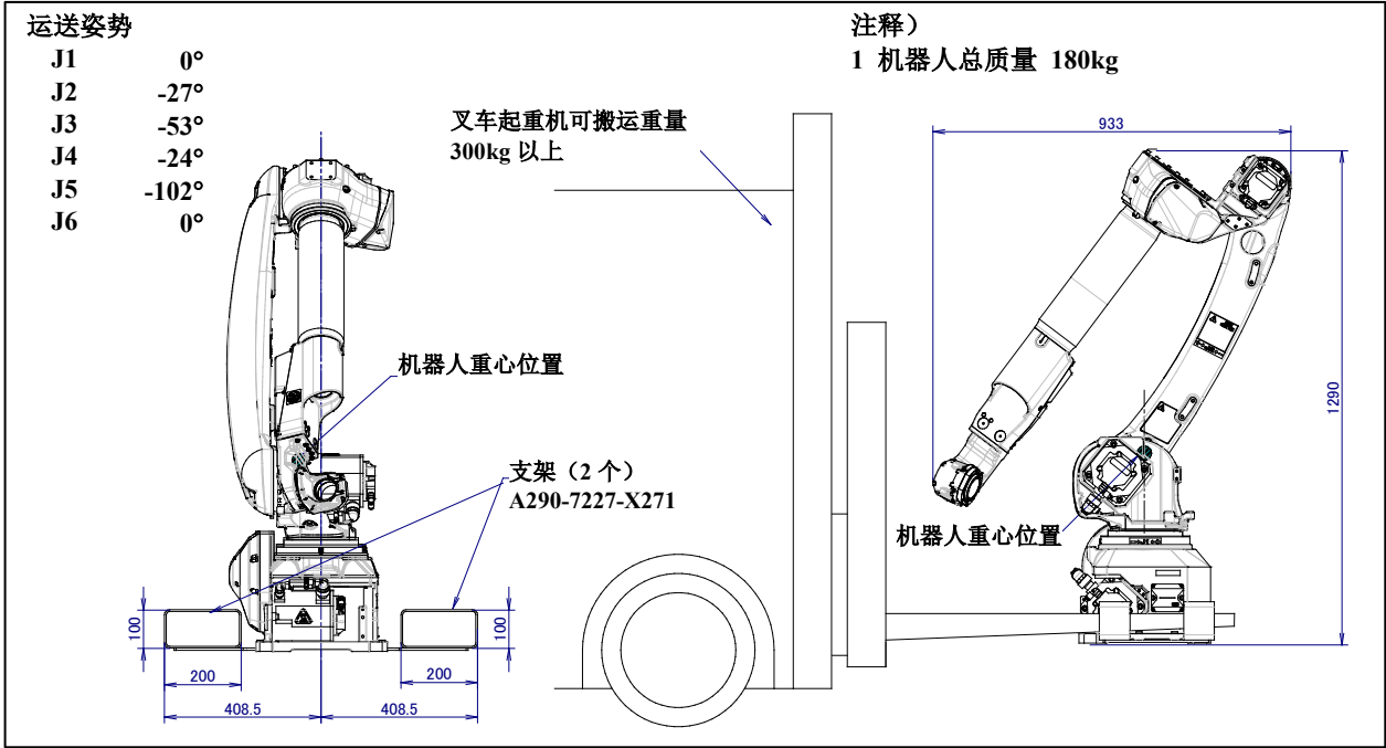
图 1.1 (g) 用叉车起重机搬运 (ARC Mate 100iD/8L, M-10iD/8L)
