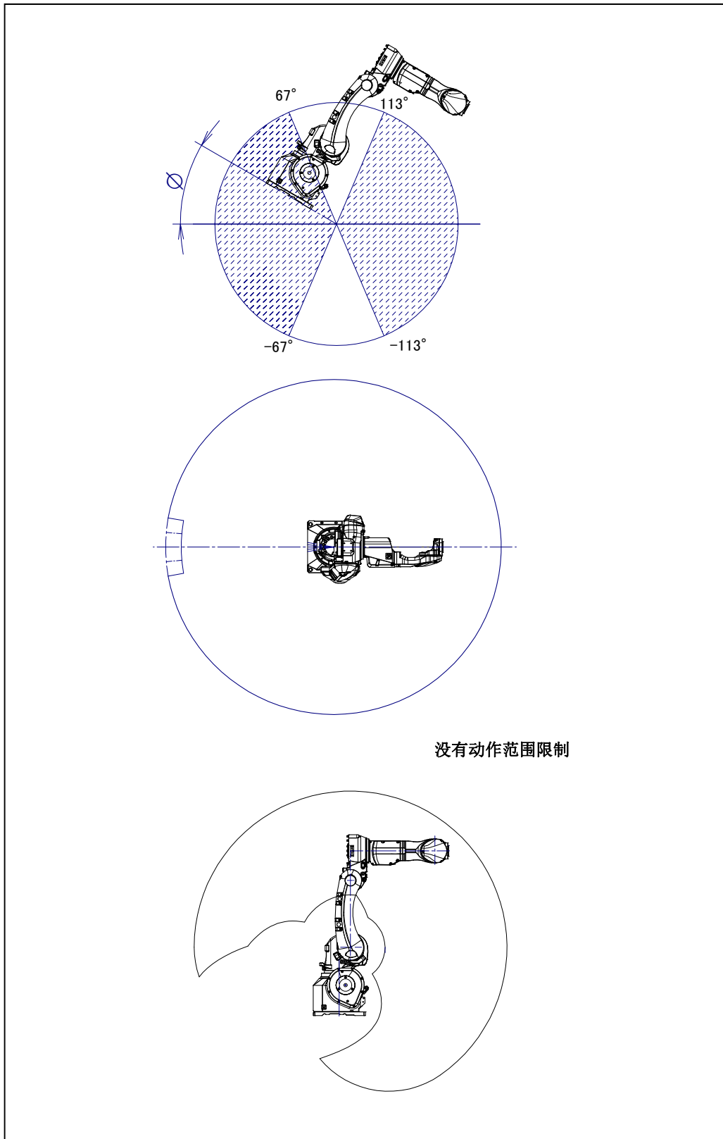
图 3.6 (h) 设置范围 (1) 动作范围图 (ARC Mate 100iD/16S, M-10iD/16S) (-180^\circ \leq \phi \leq -113^\circ, -67^\circ \leq \phi \leq 67^\circ, 113^\circ \leq \phi \leq 180^\circ)
