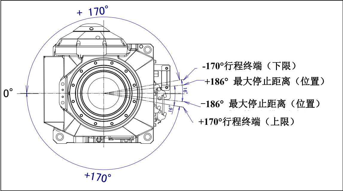
图 3.3 (c) J1 轴可动范围（选择机械式制动器时）
