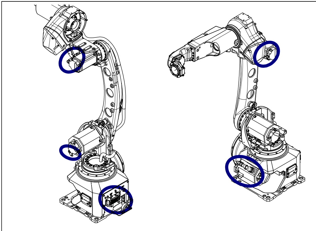
图 7.2.3 (b) 连接器的检修部位
