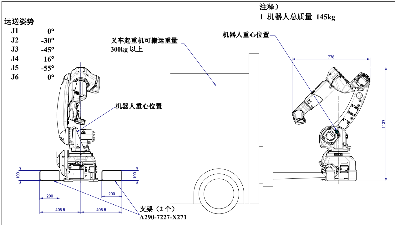
图 1.1 (e) 用叉车起重机搬运 (ARC Mate 100iD, M-10iD/12)
