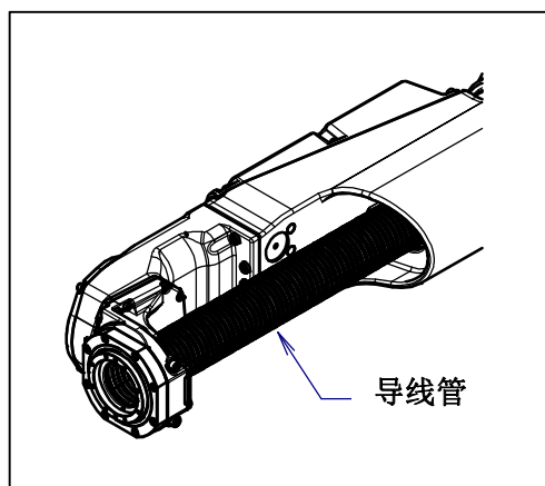
图 3.4 (a) 电缆内置型例
