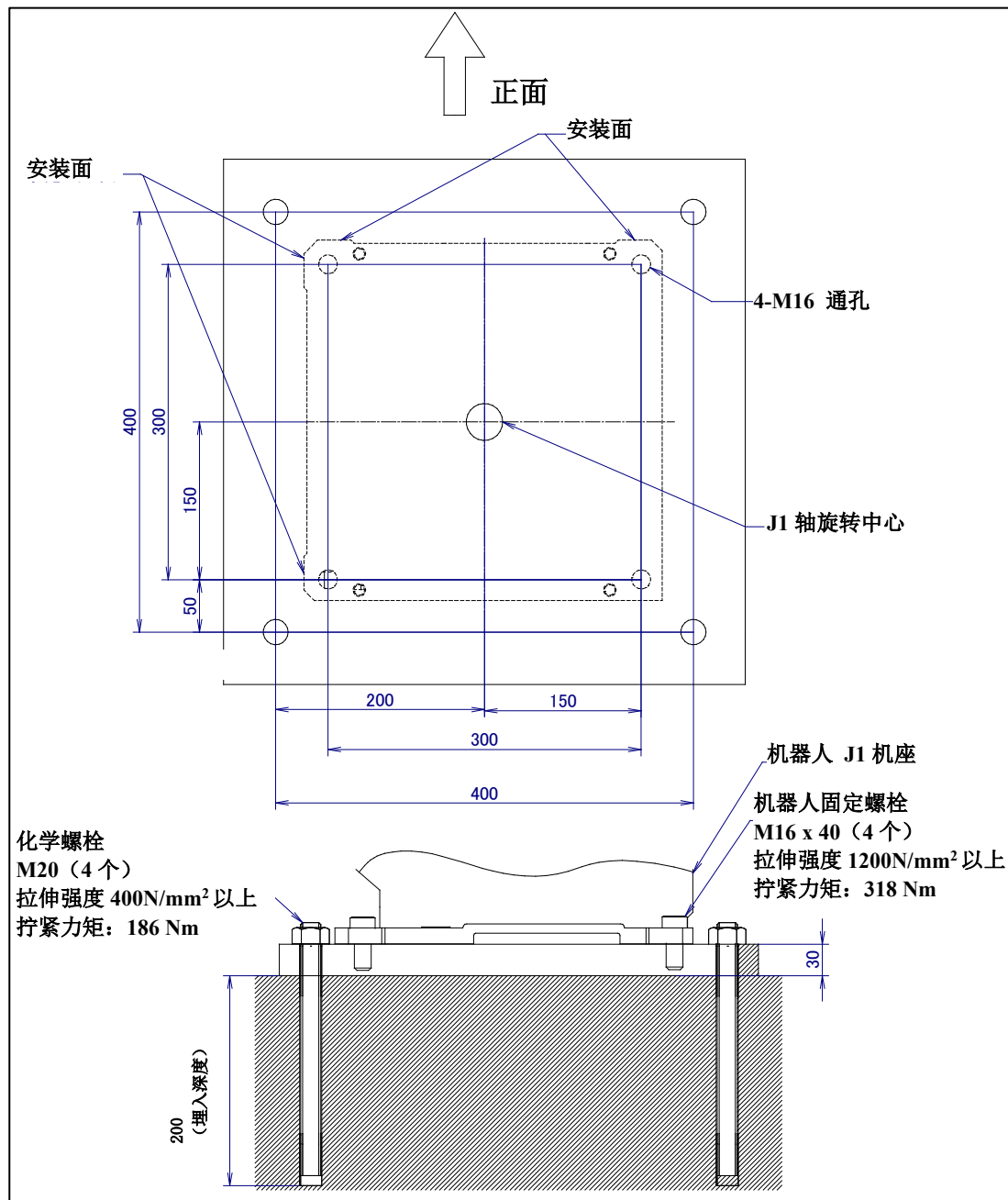
图 1.2.1 (a) 机器人安装具体例
