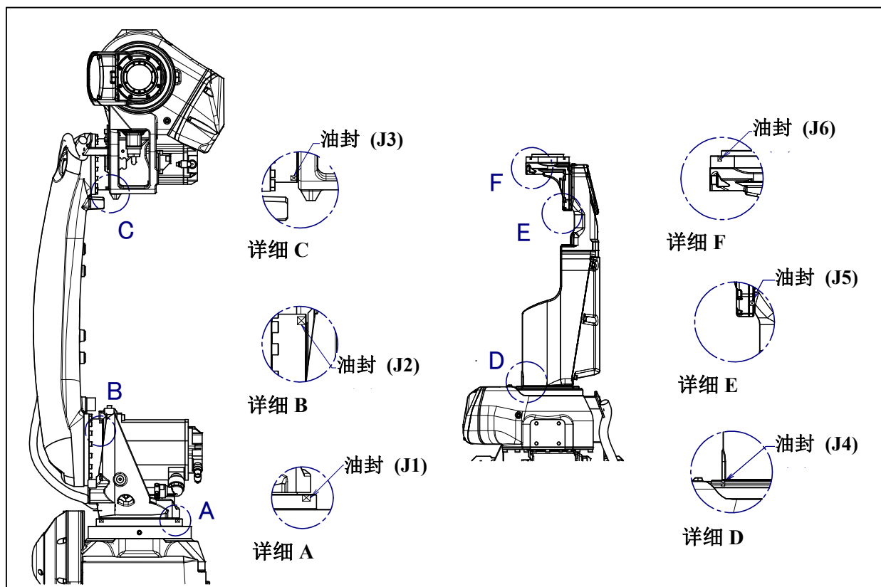
图 7.2.1 (a) 渗油的检查部位
