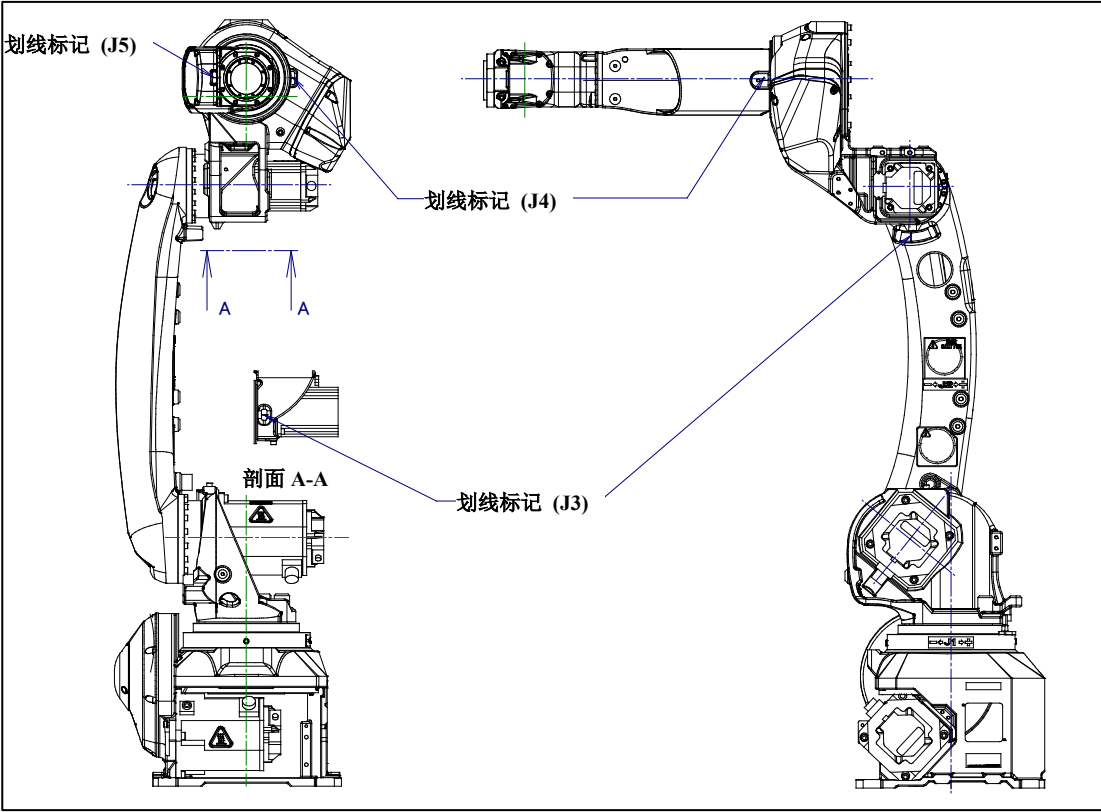
图 8.3 (a) 各轴的对合标记位置
