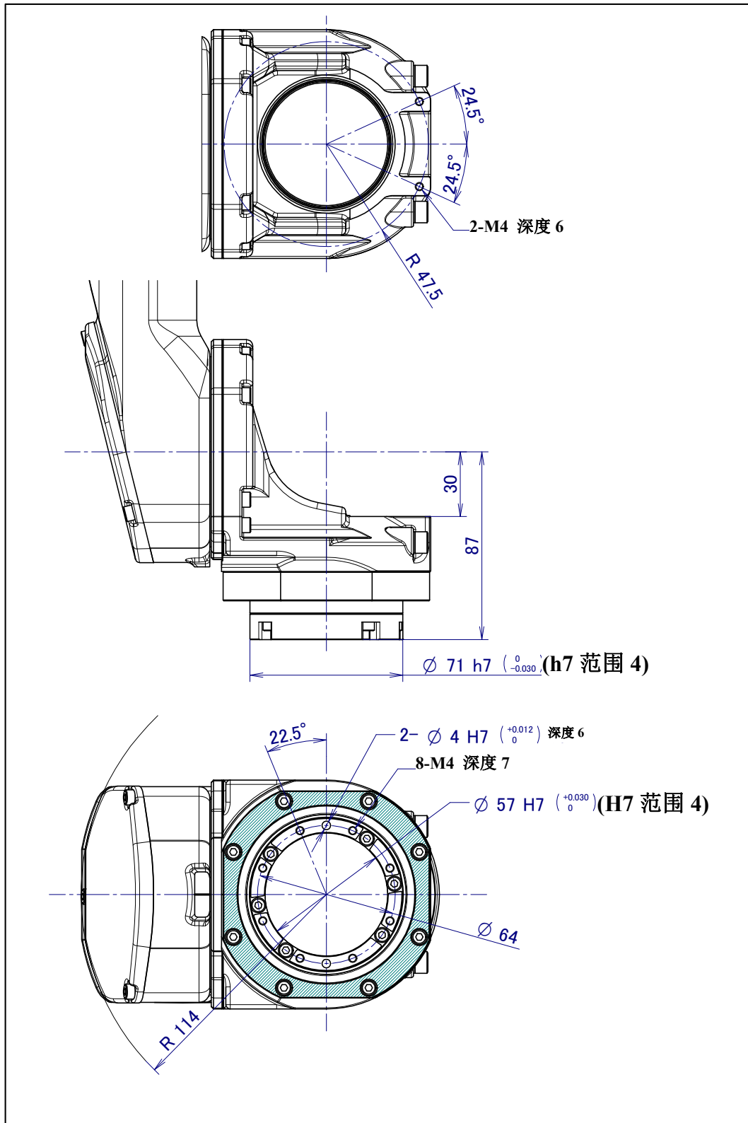
图 4.1 (c) 末端执行器安装面 (M-10iD/12 食品润滑油规格)
