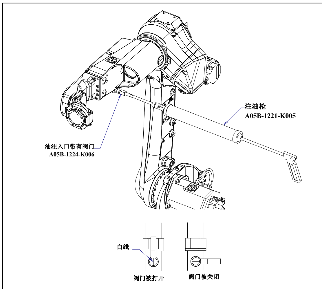
图 7.3.2.7 (b) 用注油枪供油
