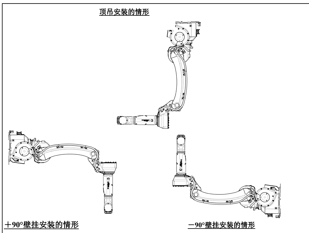
图 7.3.2 (a) 安装形式
