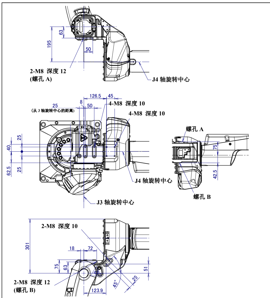
图 4.2 (b) 设备安装面尺寸
