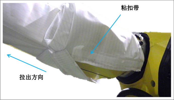
图 7.3.3 (c) 手腕外罩的拆除
