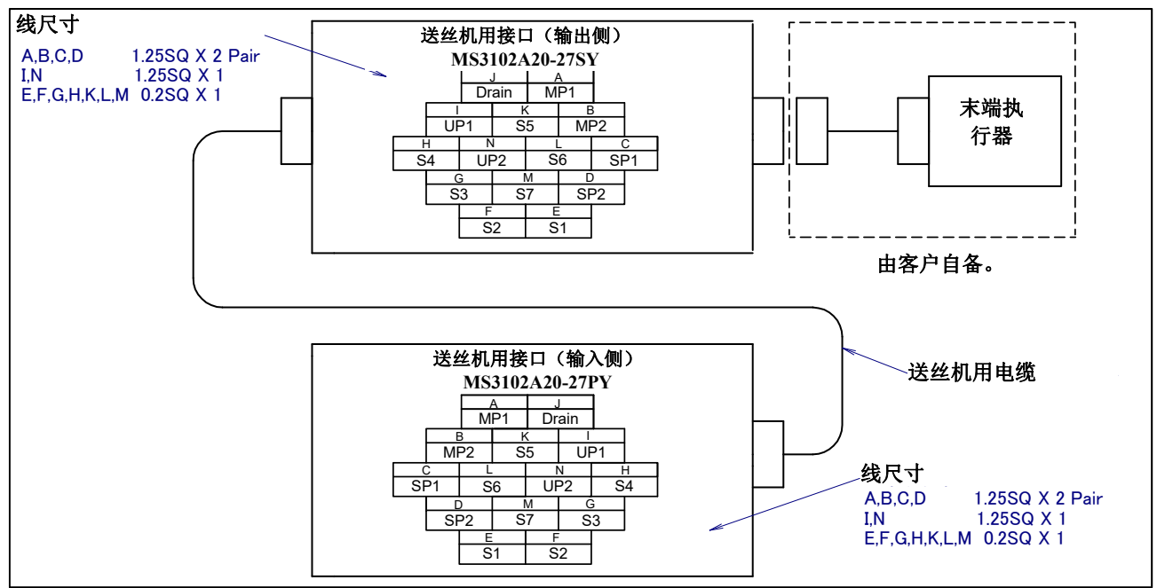
图 5.3 (k) 林肯电气送丝机用接口的插脚排列（可选项项） (指定 A05B-1227- H205#□□L,时)
