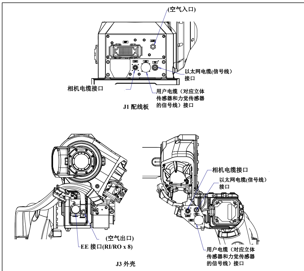
图 5.3 (e) 可选项项电缆用接口(指定 A05B-1227-H222#□□时)
