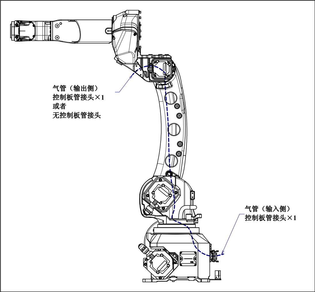
图 5.1 (a) 气压供应口（可选项项）
