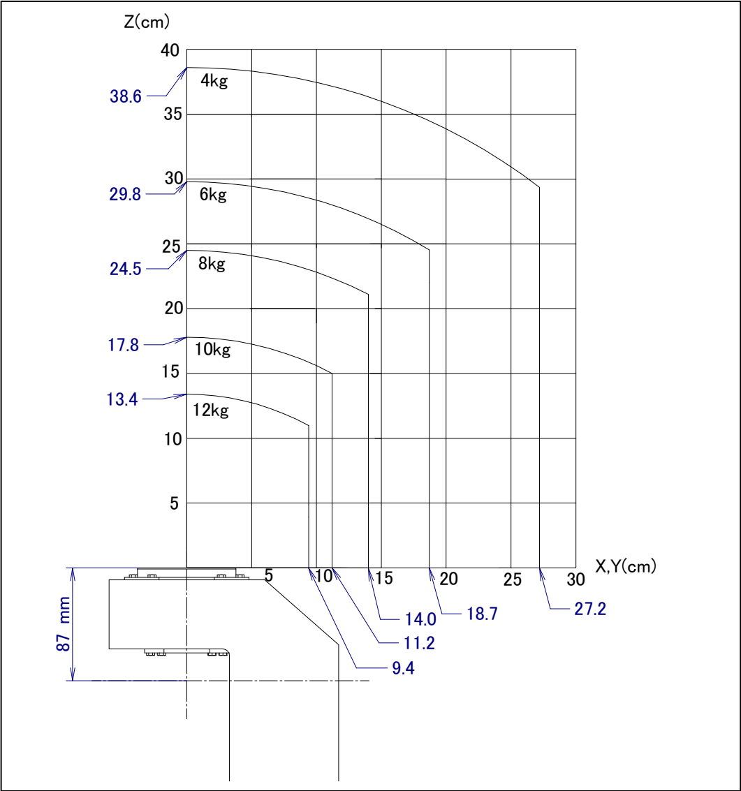
图 3.5 (b) 手腕部允许负载线图 (M-10iD/12 防尘手腕外罩规格, M-10iD/12 食品润滑油规格)
