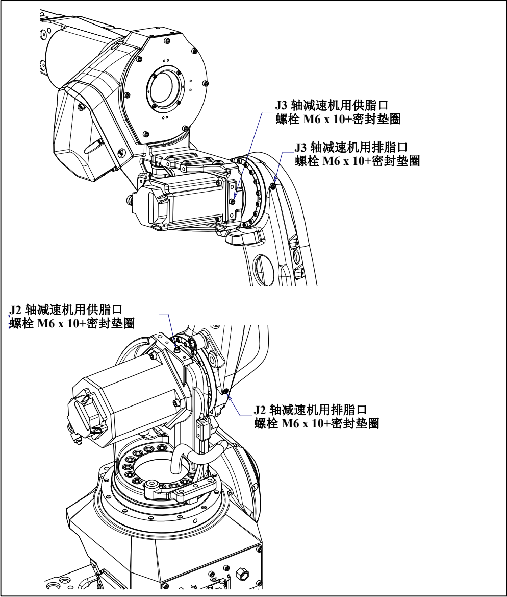
图 7.3.2.1 (a) J2, J3 轴的供脂部位
