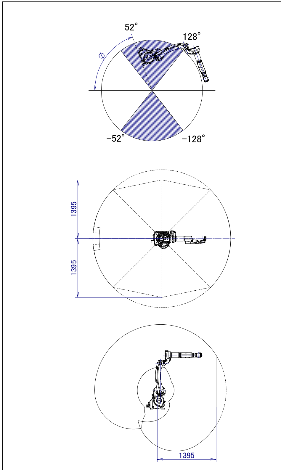
图 3.6 (e) 设置范围 (2) 动作范围图 (ARC Mate 100iD/10L, M-10iD/10L) (-128^\circ < \phi < -52^\circ, 52^\circ < \phi < 128^\circ)
