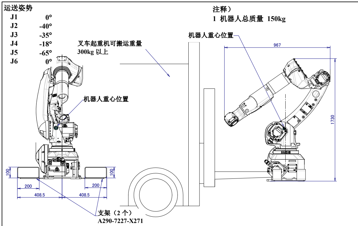
图 1.1 (f) 用叉车起重机搬运 (ARC Mate 100iD/10L, M-10iD/10L)
