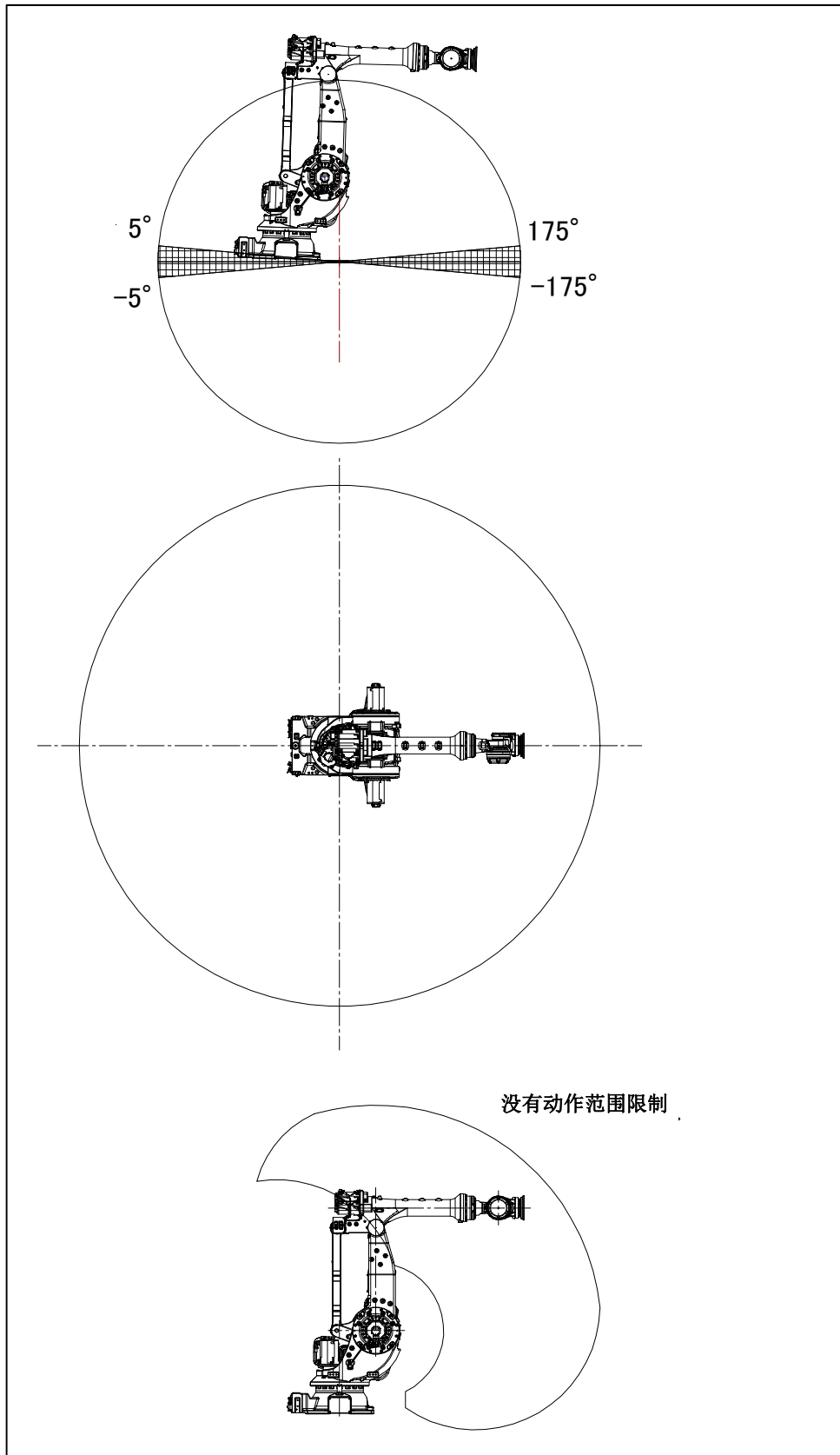
图 3.6 (b) 机器人设置角度范围(1)的动作范围 (-180^\circ \leq \phi \leq -175^\circ, -5^\circ \leq \phi \leq 5^\circ, 175^\circ \leq \phi \leq 180^\circ) (M-900iB/360/360E)
