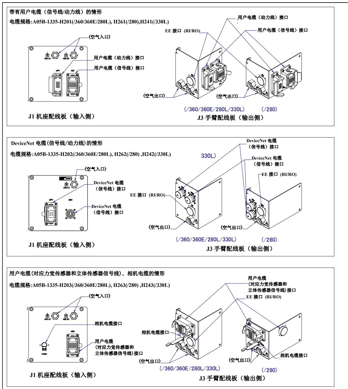
图 5.3 (b) 可选项项电缆用接口 (1/2)
