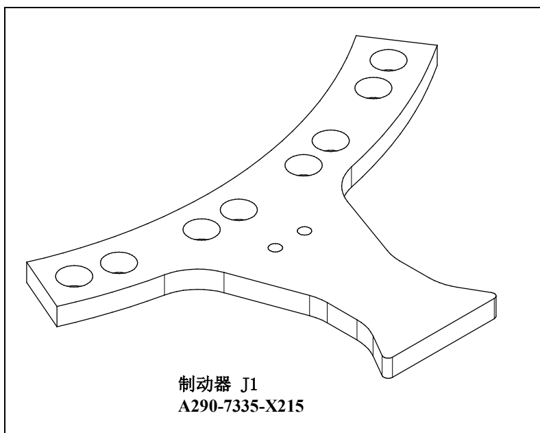
图 6.2.1 (a) J1 轴机械式可变制动器 (可选项)
