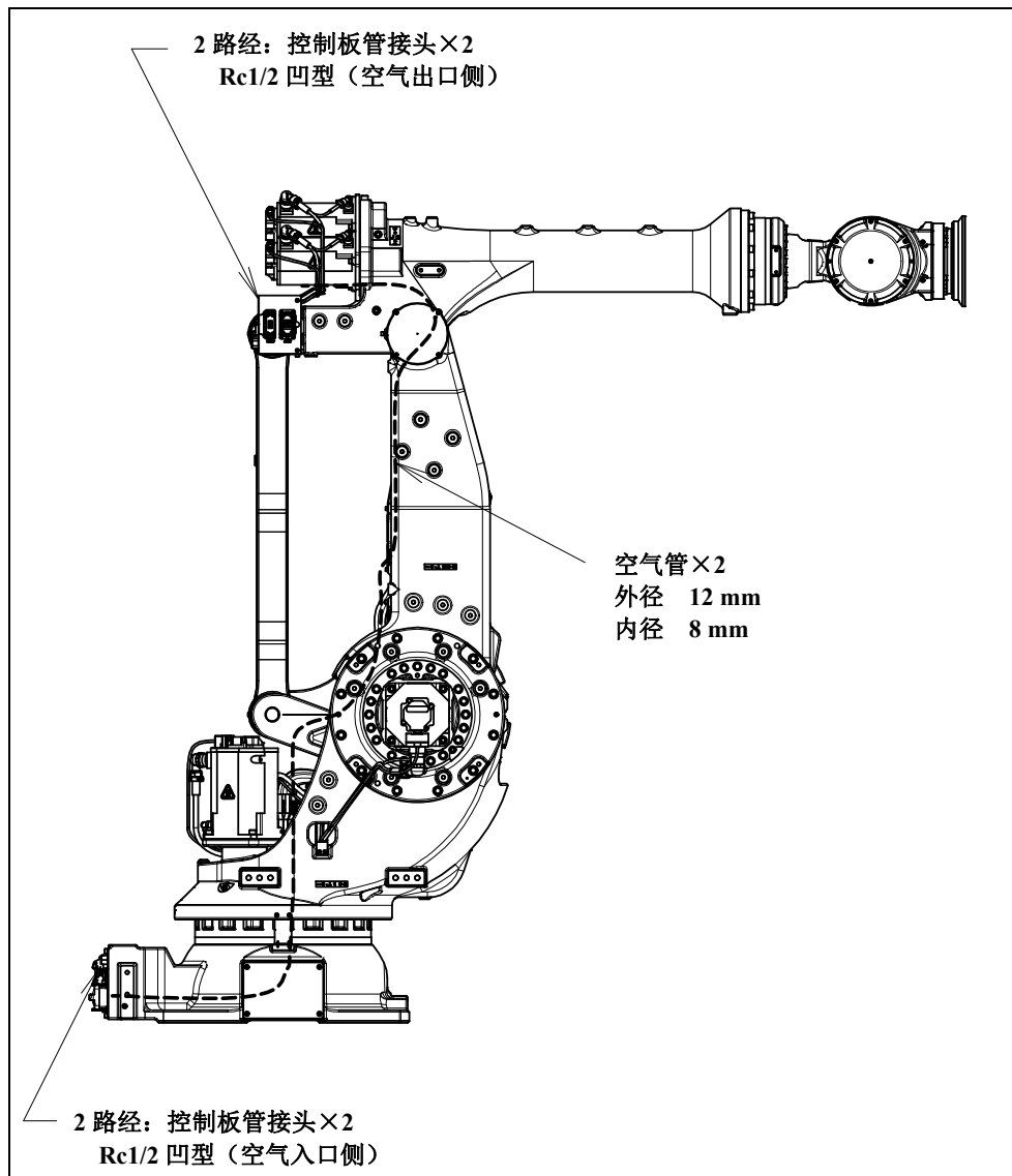
图 5.1 (a) 气压供应口（可选购项）
