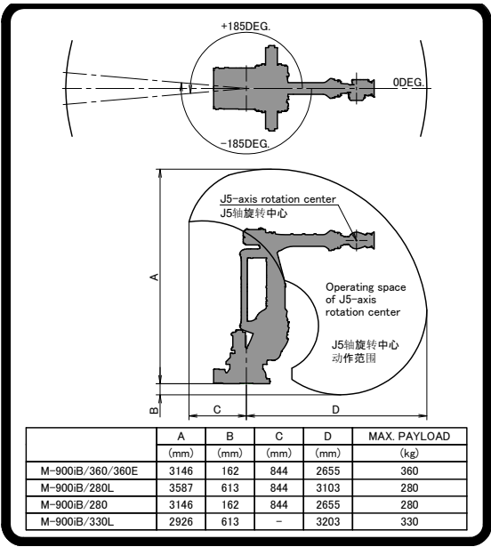
图 4 (e) 动作范围、可搬运重量标签
