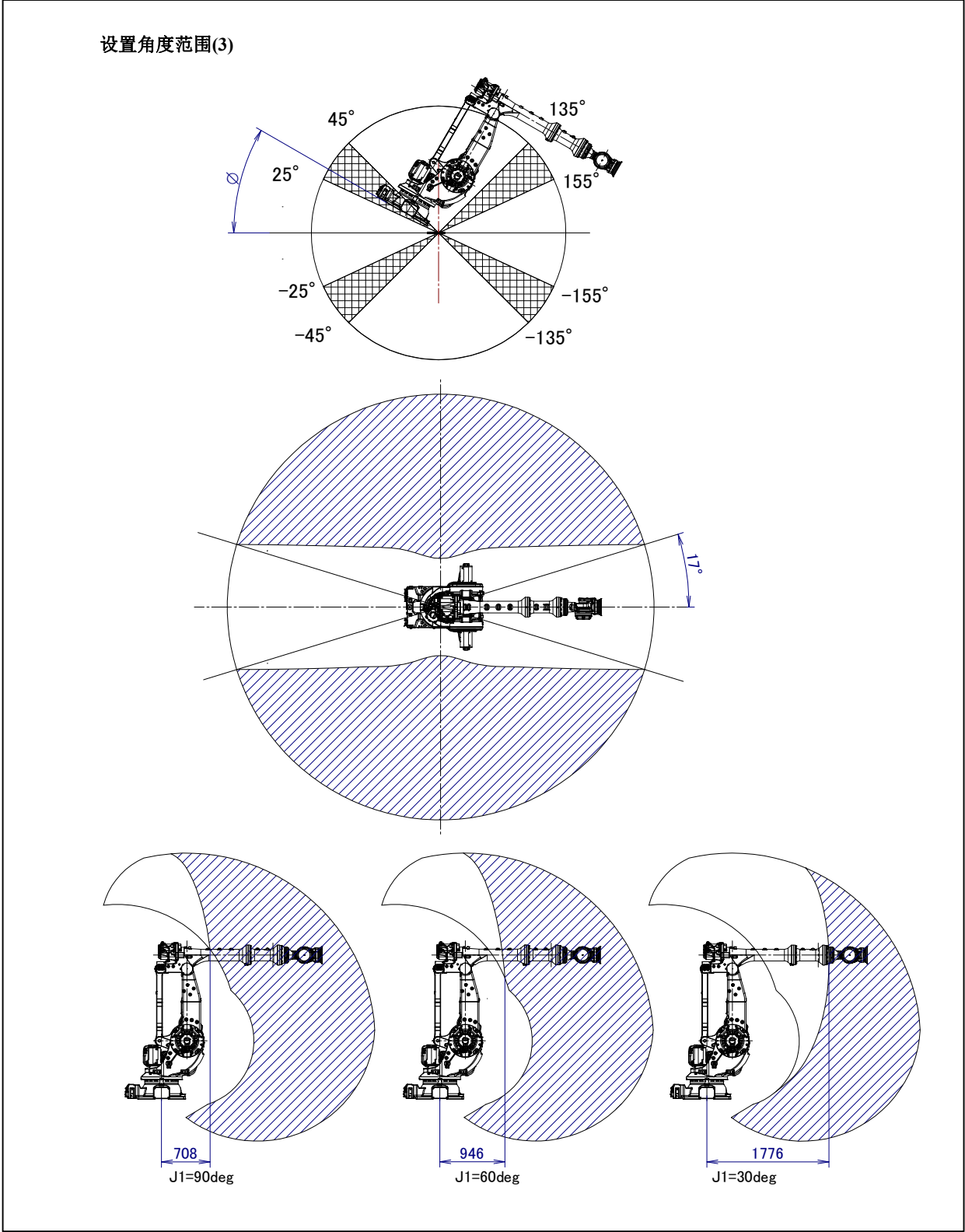
图 3.6 (h) 机器人设置角度范围(3)的动作范围 ( -155^\circ < \phi \leq -135^\circ , -45^\circ \leq \phi < 25^\circ , 25^\circ < \phi \leq 45^\circ , 135^\circ \leq \phi < 155^\circ ) (M-900;B/280L)
