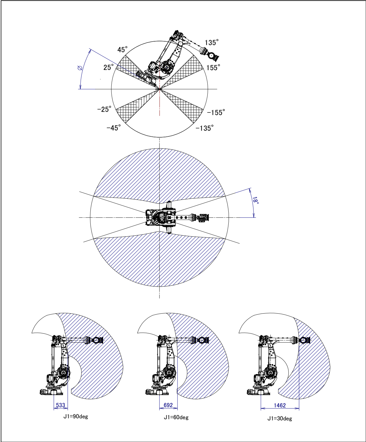
图 3.6 (d) 机器人设置角度范围(3)的动作范围 ( -155^{\circ} < \phi \leq -135^{\circ} , -45^{\circ} \leq \phi < 25^{\circ} , 25^{\circ} < \phi \leq 45^{\circ} , 135^{\circ} \leq \phi < 155^{\circ} ) (M-900iB/360/360E)
