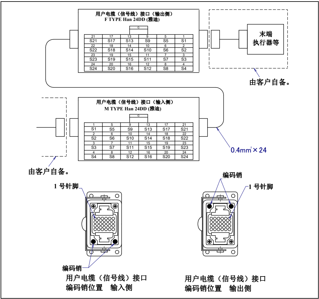
图 5.3 (g) 用户电缆（信号线）(AS) 接口的插针排列和编码销的配置位置（可选项）
