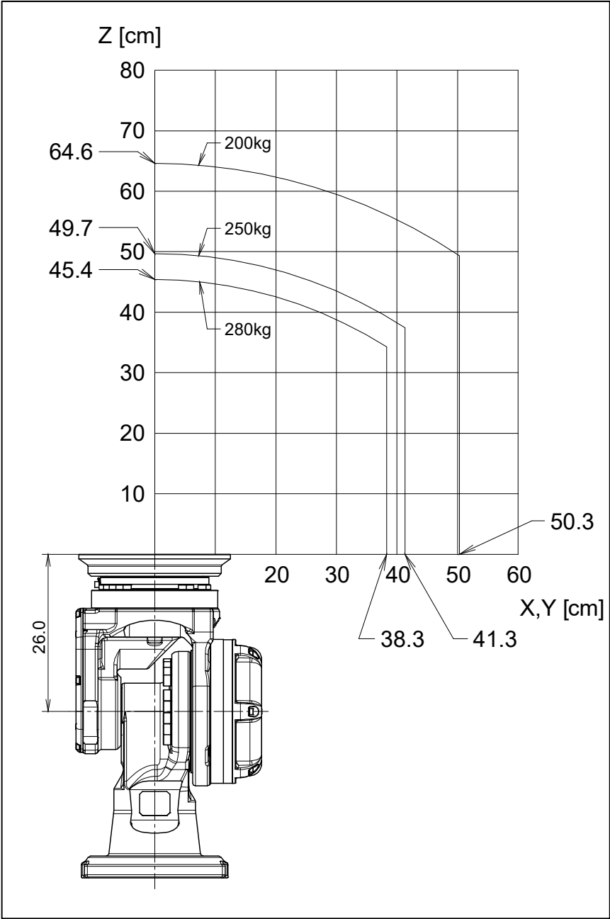
图 3.4 (g) 手腕部允许负载线图 (ISO 法兰盘) (M-900iB/280)
