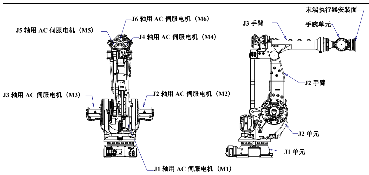
图 3.1 (a) 机构部的构成 (M-900iB/360/360E/280L)
