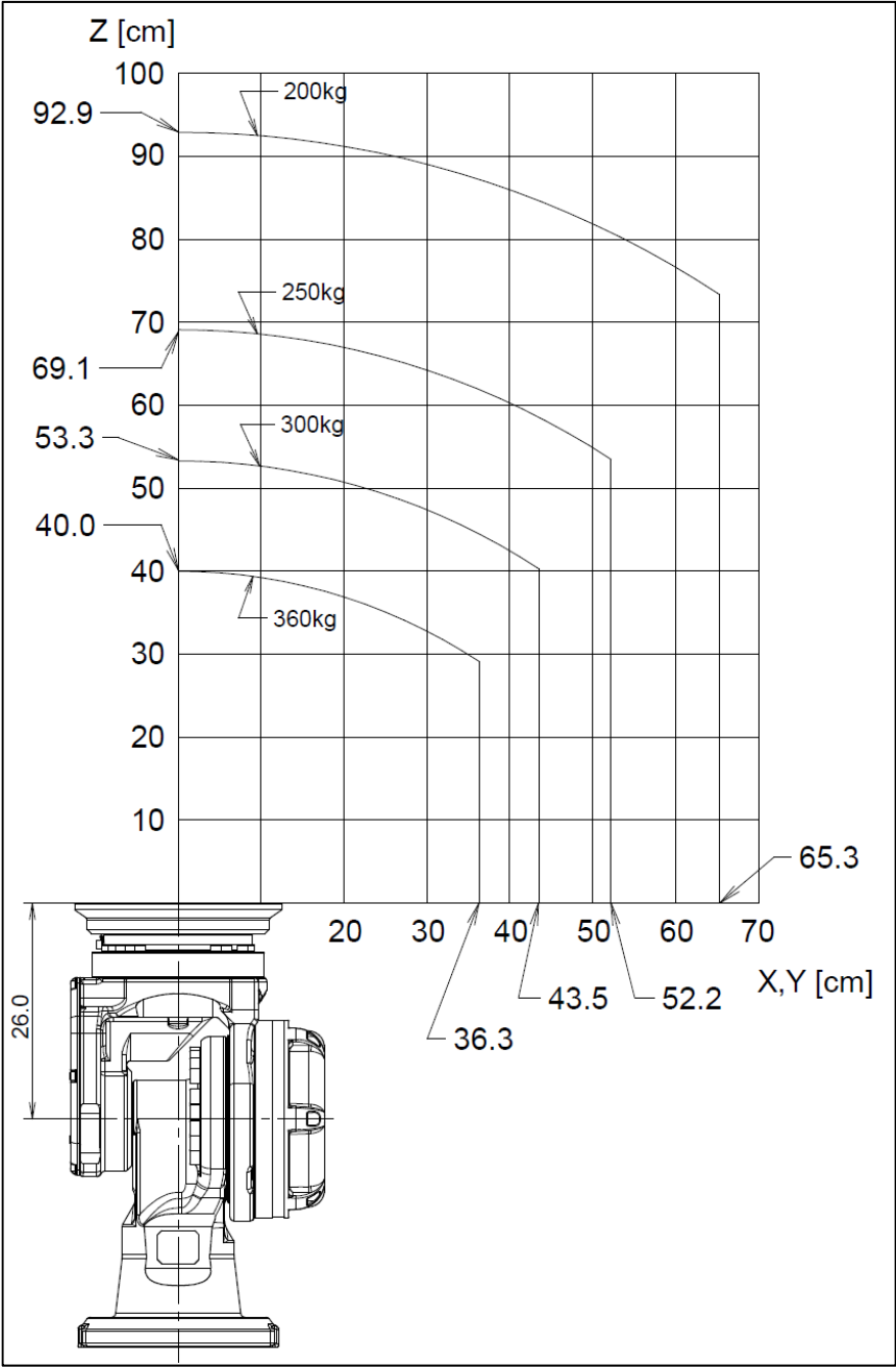
图 3.4 (c) 手腕部允许负载线图 (ISO 法兰盘) (M-900iB/360E)
