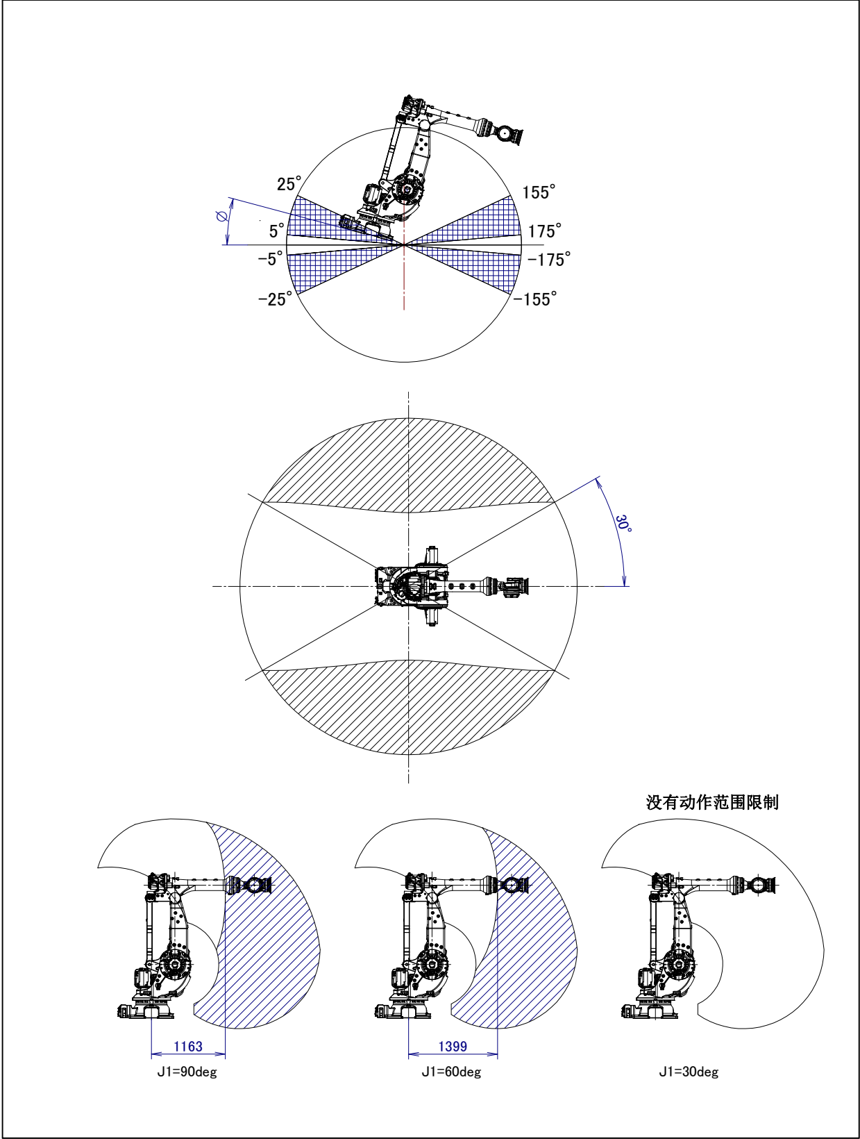
图 3.6 (c) 机器人设置角度范围(2)的动作范围 ( -175^\circ < \phi \leq -155^\circ , -25^\circ \leq \phi < -5^\circ , 5^\circ < \phi \leq 25^\circ , 155^\circ \leq \phi < 175^\circ ) (M-900iB/360/360E)
