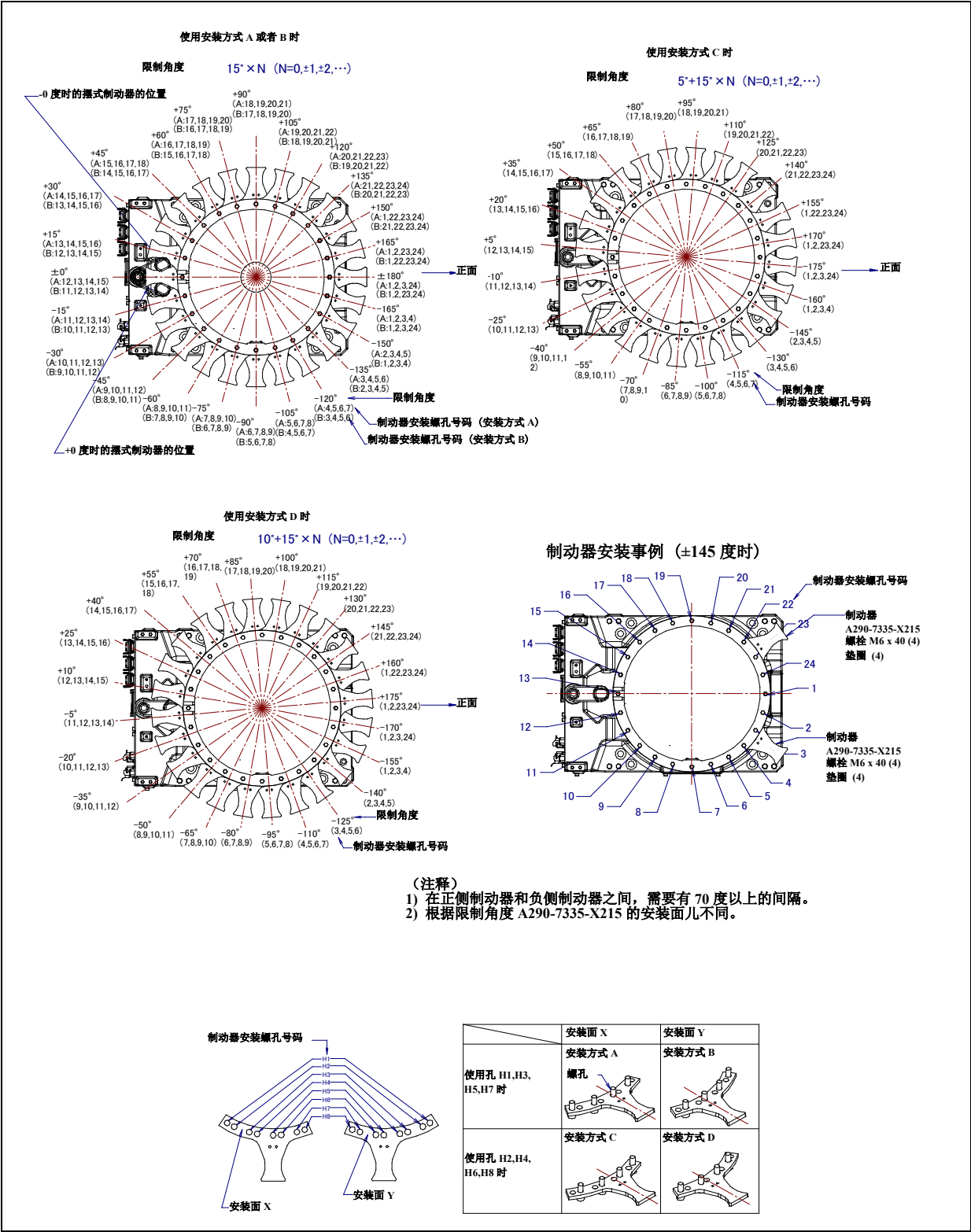
图 6.2.1 (c) J1 轴机械式可变制动器的安装 (2/2)
