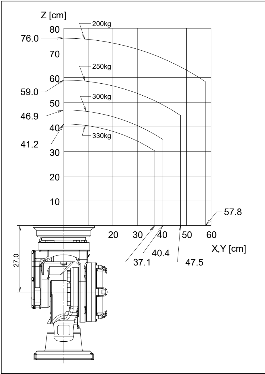
图 3.4 (j) 手腕部允许负载线图（绝缘 ISO 法兰盘） (M-900iB/330L)
