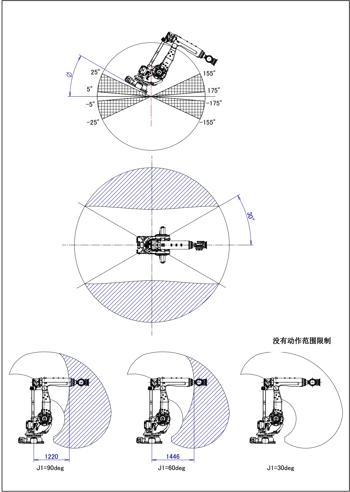
图 3.6 (k) 机器人设置角度范围(2)的动作范围 ( -175^\circ < \phi \leq -155^\circ , -25^\circ \leq \phi < -5^\circ , 5^\circ < \phi \leq 25^\circ , 155^\circ \leq \phi < 175^\circ ) (M-900iB/280)
