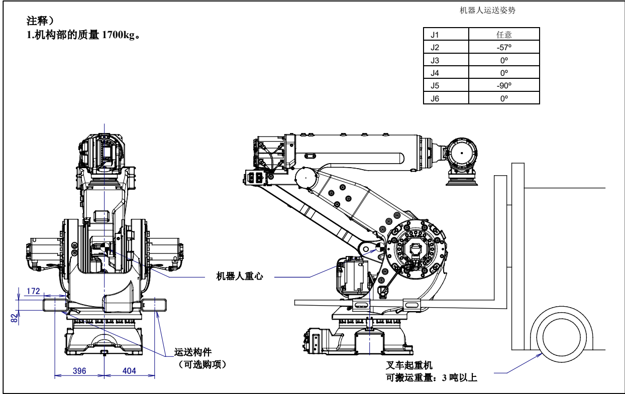
图 1.1 (h) 采用叉车起重机搬运(M-900iB/280)
