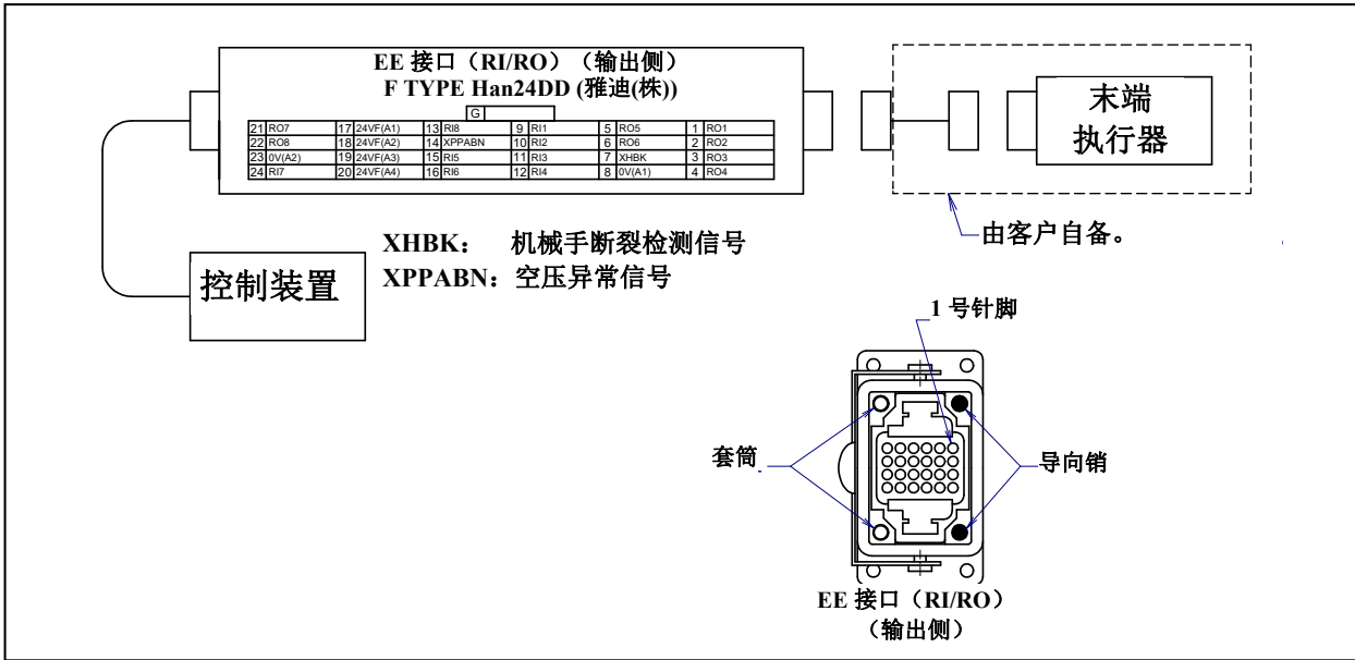
图 5.3 (q) EE 接口(RI/RO) (选择防尘防液强化组件时) 的插针排列 (可选项)
