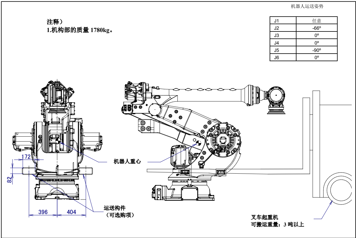
图 1.1 (i) 采用叉口起重机搬运(M-900iB/330L)
