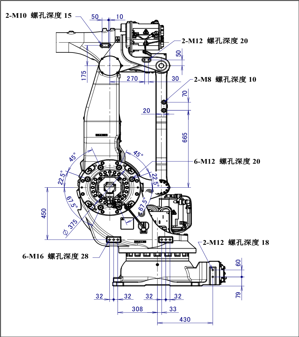
图 4.2 (b) 设备安装面尺寸 (M-900iB/360/360E (2/2))
