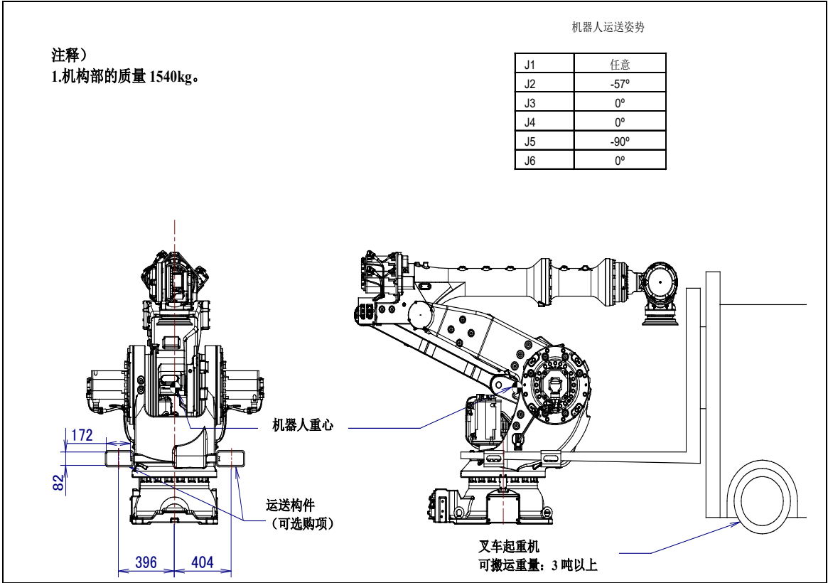
图 1.1 (f) 采用叉车起重机搬运(M-900iB/360/360E)
