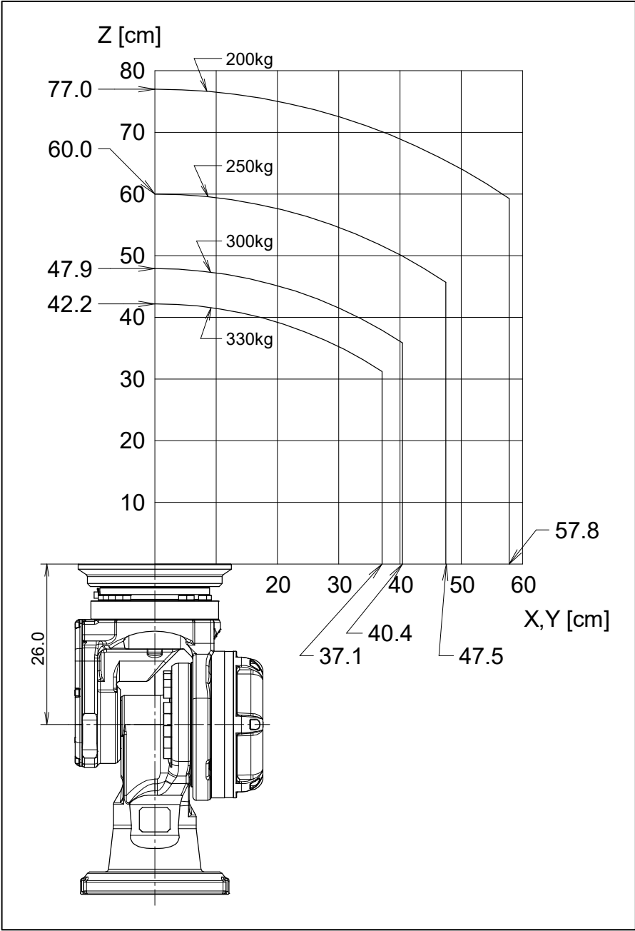
图 3.4 (i) 手腕部允许负载线图 (ISO 法兰盘) (M-900iB/330L)
