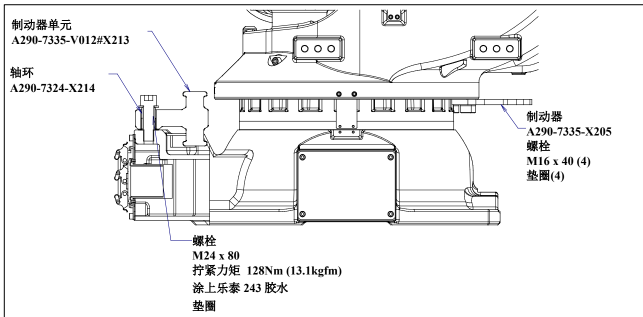
图 6.2.1 (b) J1 轴机械式可变制动器的安装 (1/2)
