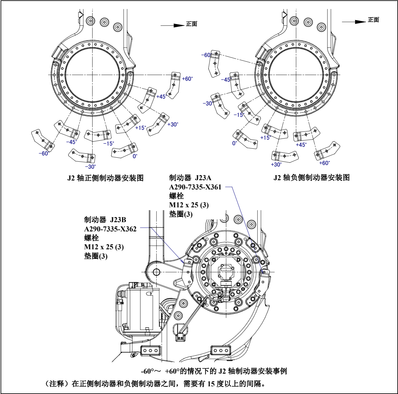
图 6.2.1 (e) J2 轴机械式可变制动器的安装
