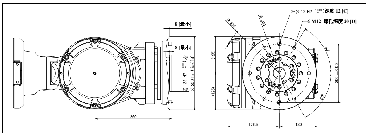
图 4.1 (a) 末端执行器安装面 (ISO 法兰盘)
