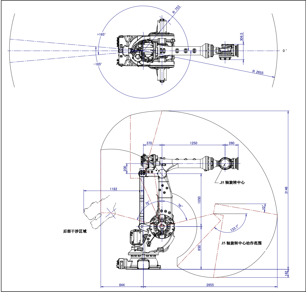
图 3.2 (a) 动作范围图 (M-900iB/360/360E)
