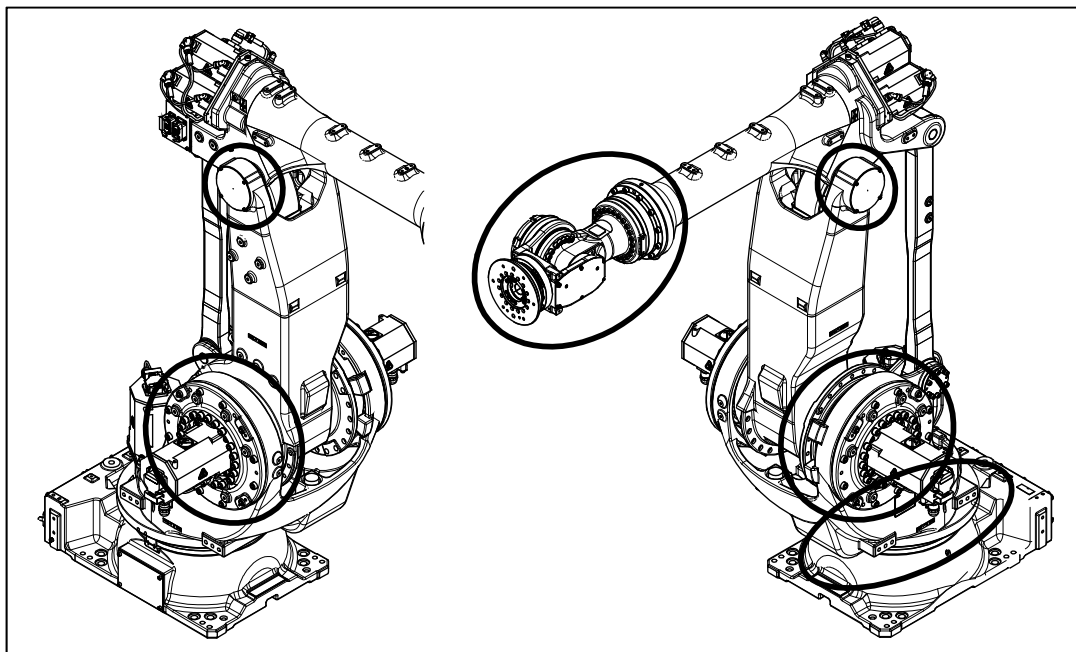
图 7.2.1 (a) 渗油的检查部位
