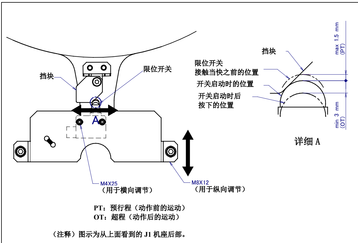
图 6.4 (a) J1 轴限位开关的调节（可选项）
