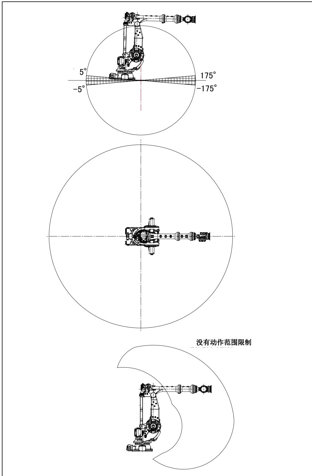
图 3.6 (f) 机器人设置角度范围(1)的动作范围 (-180^\circ \leq \phi \leq -175^\circ, -5^\circ \leq \phi \leq 5^\circ, 175^\circ \leq \phi \leq 180^\circ) (M-900iB/280L)
