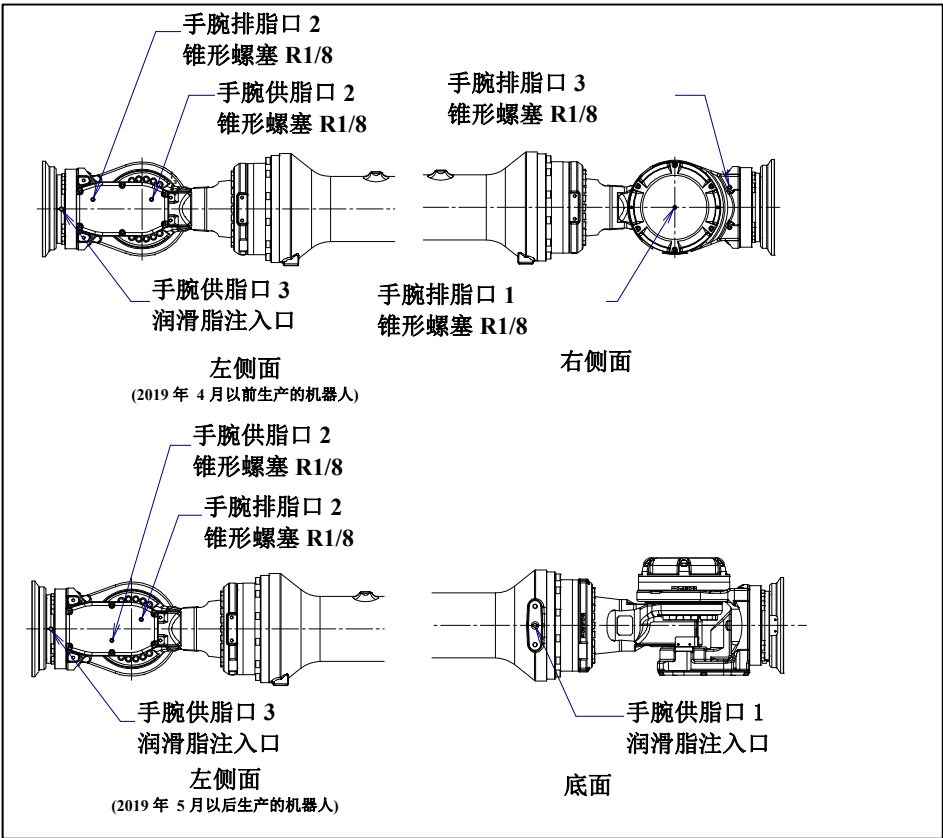
图 7.3.3 (b) 手腕的润滑脂的更换
