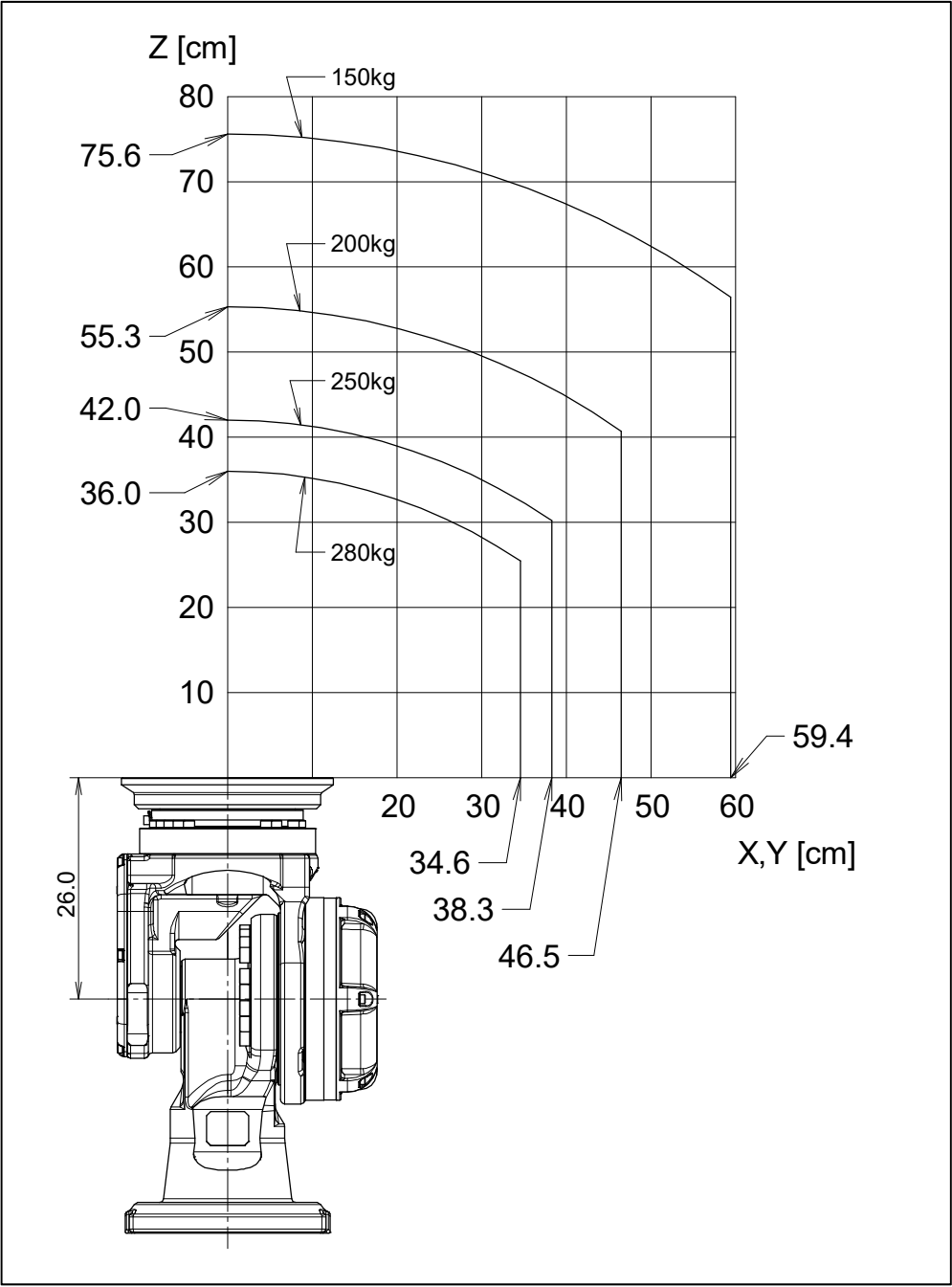
图 3.4 (e) 手腕部允许负载线图 (ISO 法兰盘) (M-900iB/280L)
