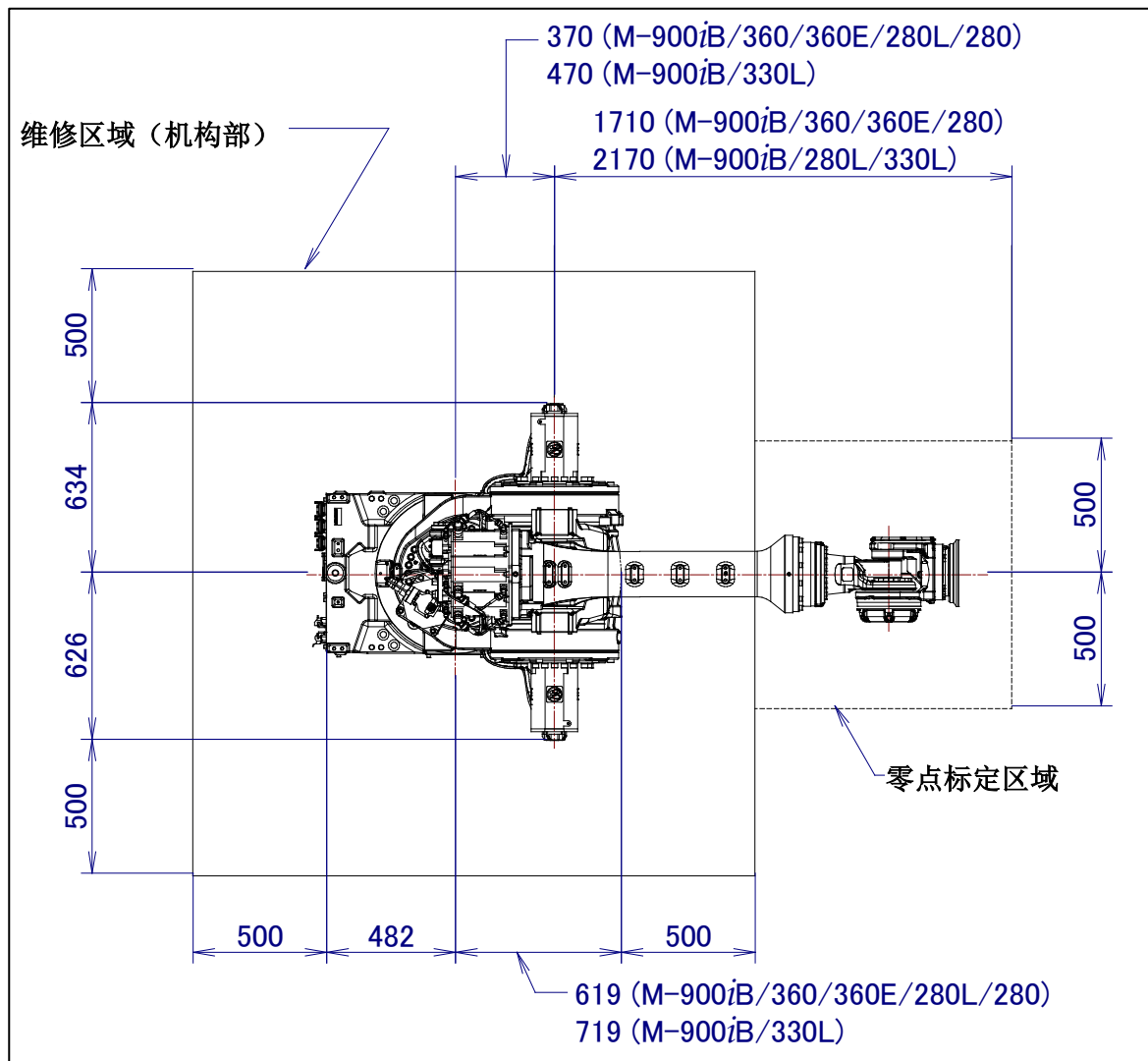
图 1.3 (a) 维修空间的布局图
