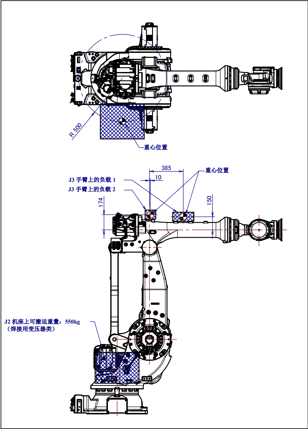
图 3.5 (a) J2 机座/J3 手臂上的负载条件 (M-900iB/360/360E/280L/330L)
