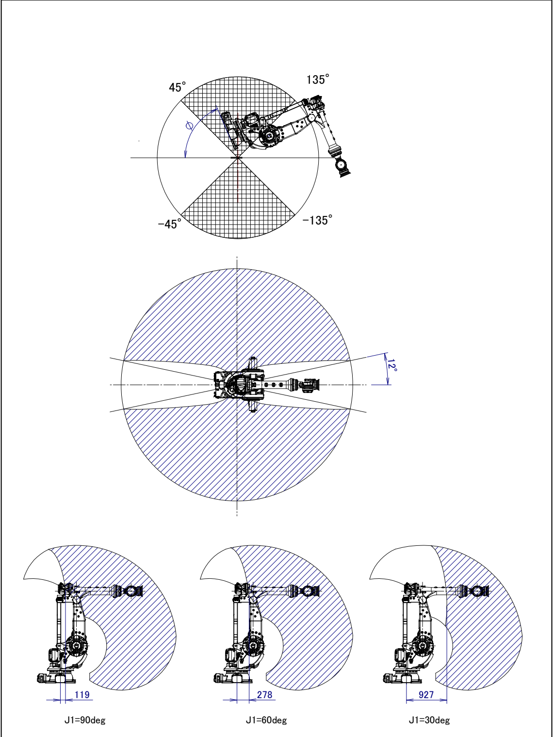
图 3.6 (e) 机器人设置角度范围(4)的动作范围 ( -135^\circ < \phi < -45^\circ , 45^\circ < \phi < 135^\circ ) (M-900iB/360/360E)
