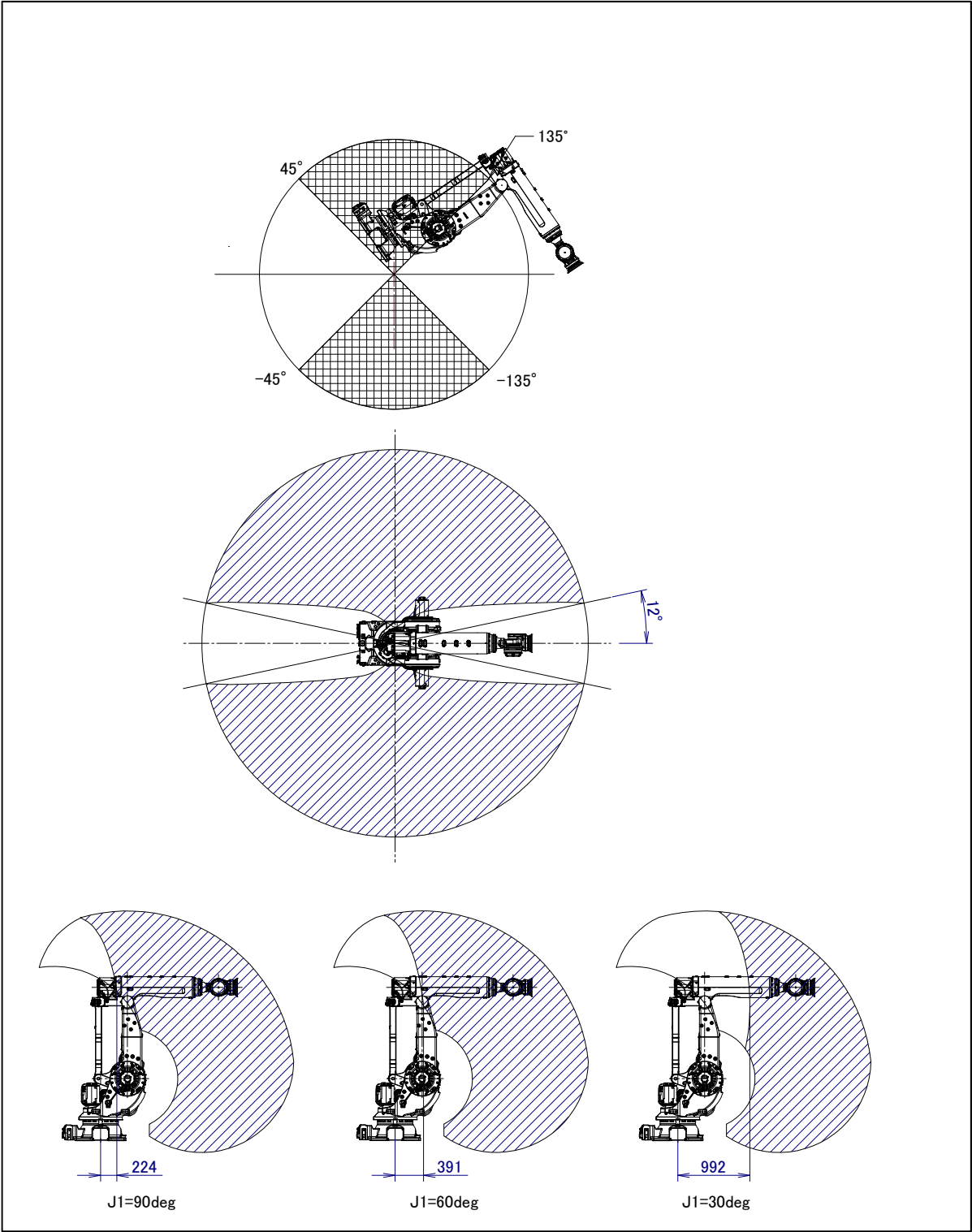
图 3.6 (m) 机器人设置角度范围(4)的动作范围 ( -135^{\circ} < \phi < -45^{\circ} , 45^{\circ} < \phi < 135^{\circ} ) (M-900iB/280)
