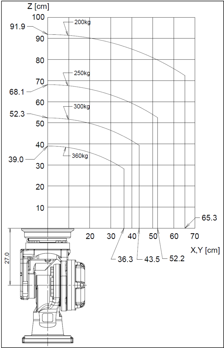
图 3.4 (d) 手腕部允许负载线图（绝缘 ISO 法兰盘） (M-900iB/360E)
