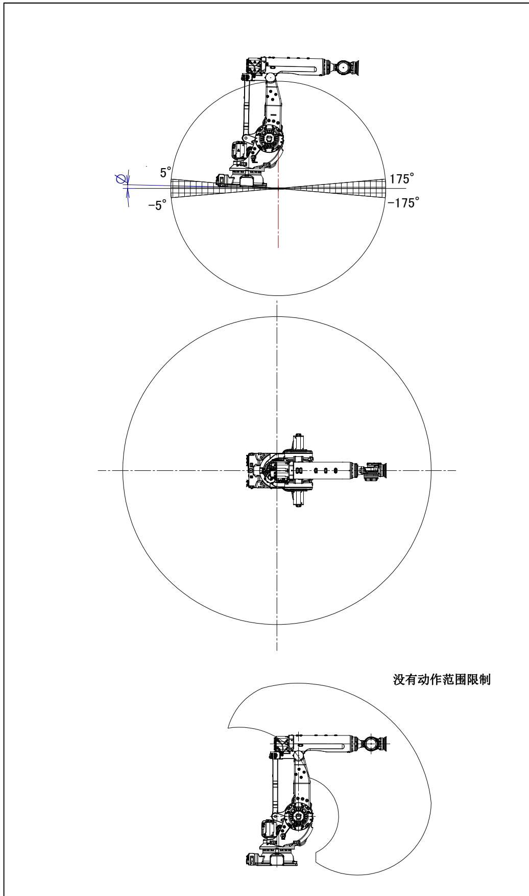
图 3.6 (j) 机器人设置角度范围(1)的动作范围 (-180^\circ \leq \phi \leq -175^\circ, -5^\circ \leq \phi \leq 5^\circ, 175^\circ \leq \phi \leq 180^\circ) (M-900iB/280)
