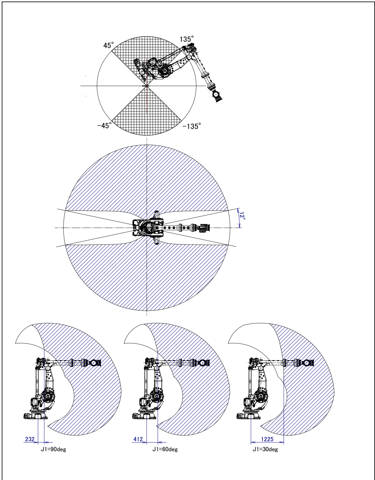
图 3.6 (i) 机器人设置角度范围(4)的动作范围 (-135^\circ < \phi < -45^\circ, 45^\circ < \phi < 135^\circ) (M-900iB/280L)
