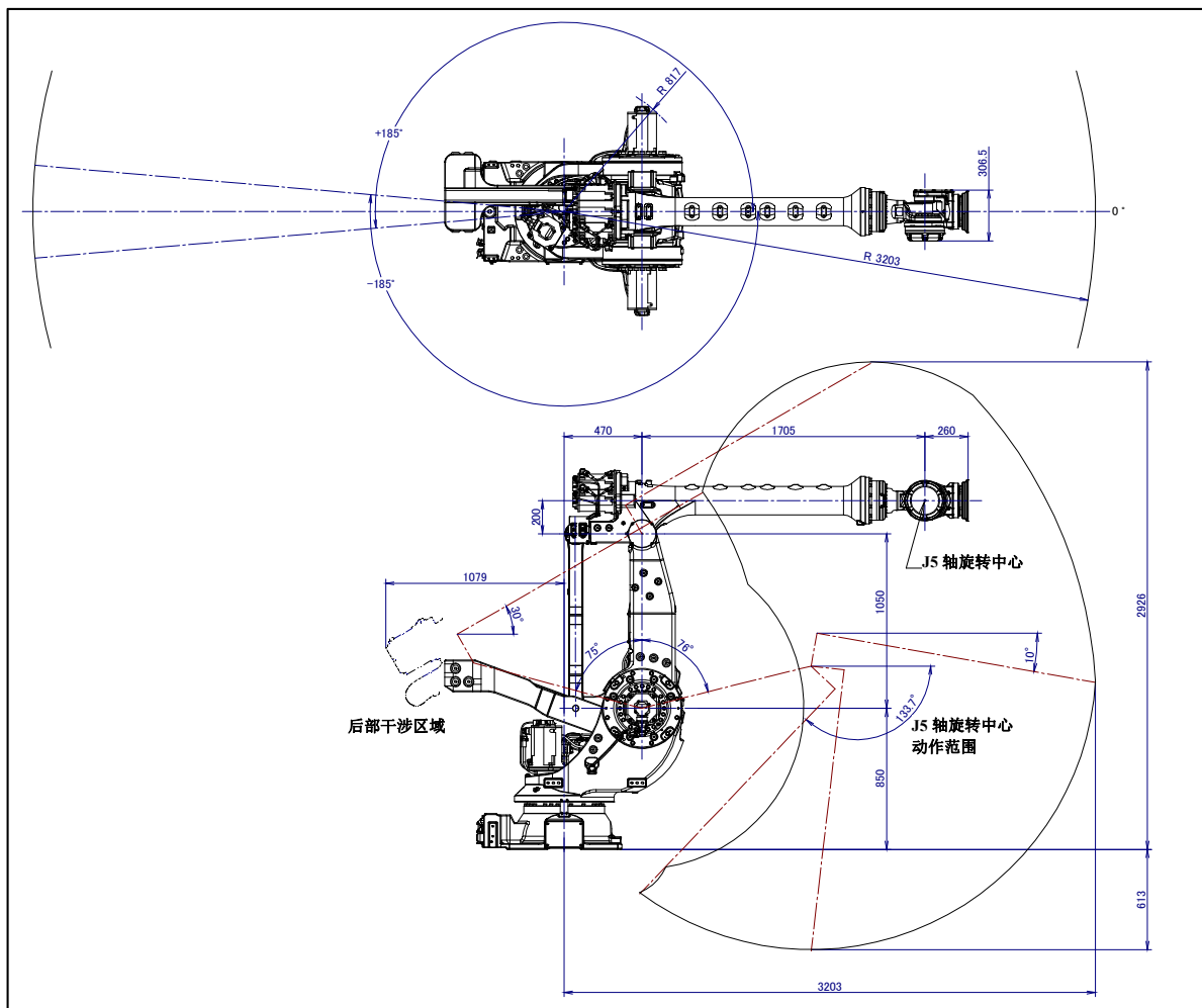
图 3.2 (d) 动作范围图 (M-900iB/330L)
