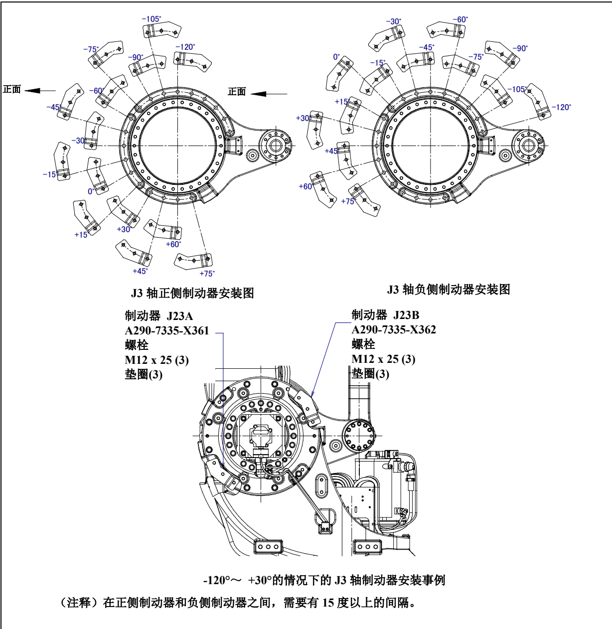
图 6.2.1 (f) J3 轴机械式可变制动器的安装
