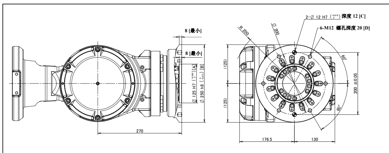
图 4.1 (b) 末端执行器安装面 (绝缘 ISO 法兰盘)
