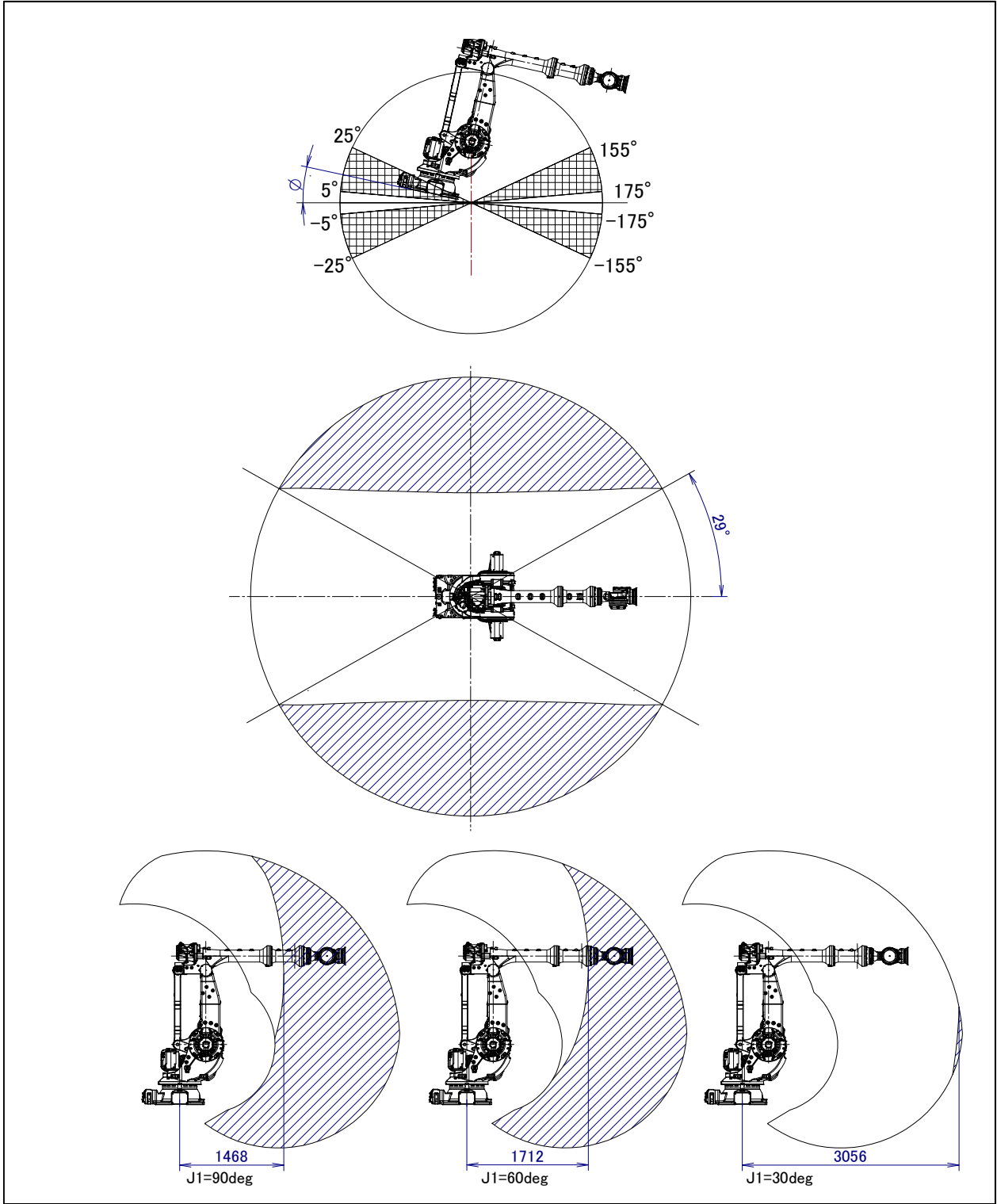
图 3.6 (g) 机器人设置角度范围(2)的动作范围 ( -175^\circ < \phi \leq -155^\circ , -25^\circ \leq \phi < -5^\circ , 5^\circ < \phi \leq 25^\circ , 135^\circ \leq \phi < 155^\circ ) (M-900iB/280L)
