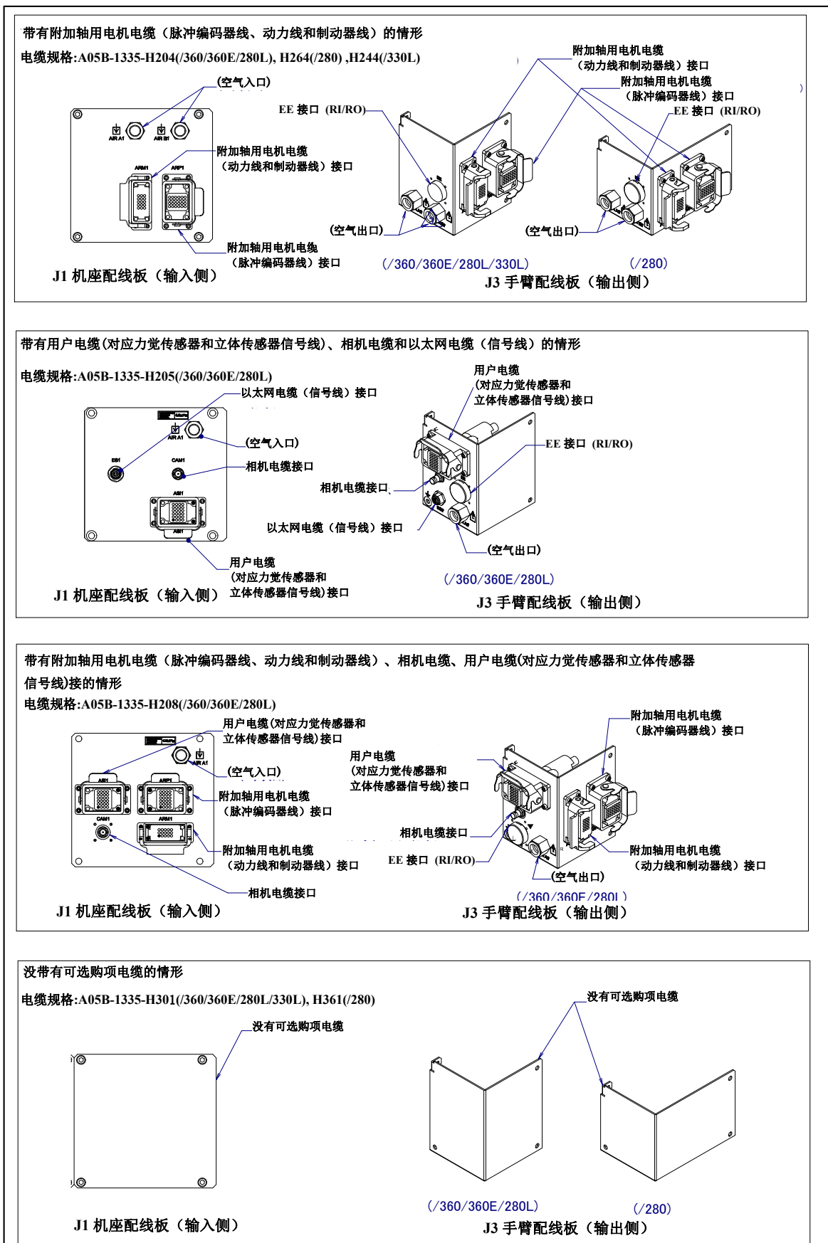
图 5.3 (c) 可选购项电缆用接口 (2/2)
