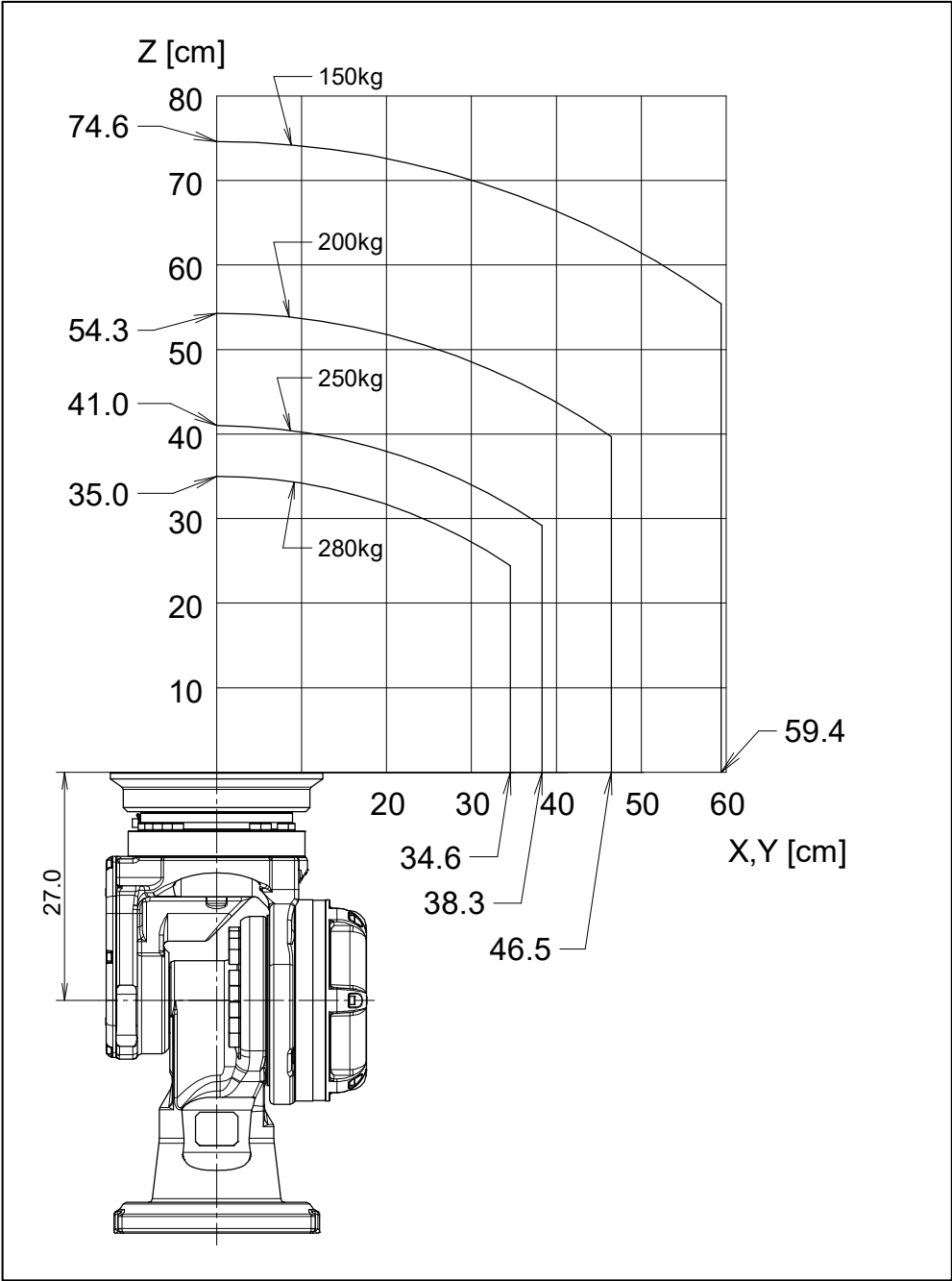
图 3.4 (f) 手腕部允许负载线图 (绝缘 ISO 法兰盘) (M-900iB/280L)
