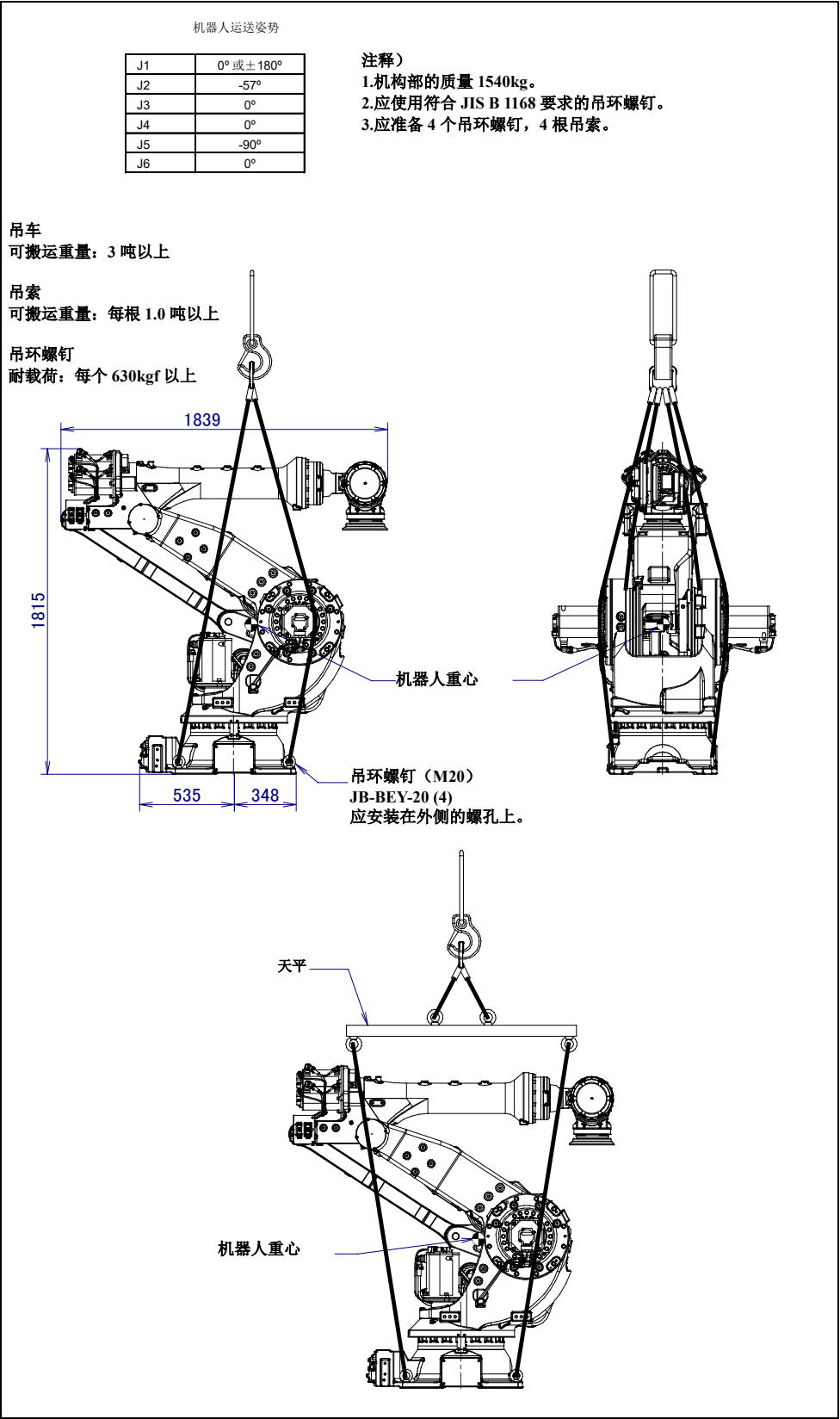
图 1.1 (b) 采用吊车搬运 (M-900iB/360/360E)
