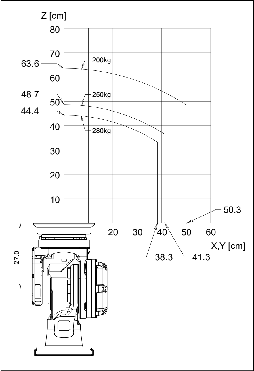
图 3.4 (h) 手腕部允许负载线图（绝缘 ISO 法兰盘） (M-900iB/280)
