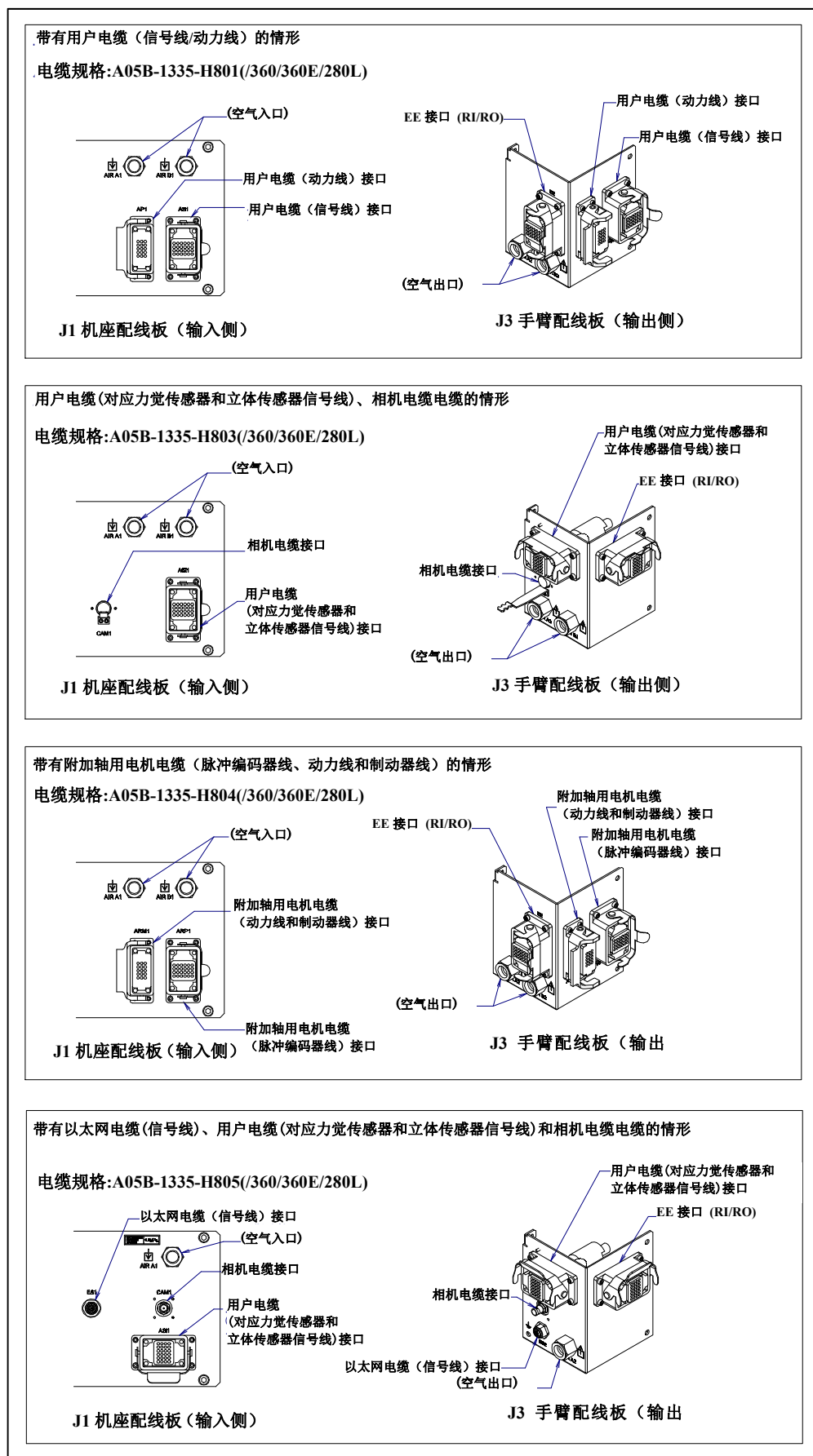
图 5.3 (d) 可选项电缆用接口 (选择防尘防液强化组件时)
