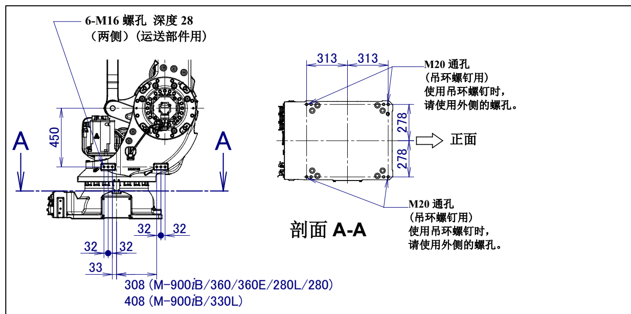
图 1.1 (a) 吊环螺钉、搬运构件安装位置
