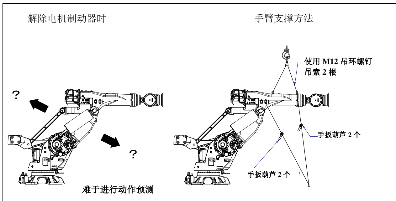
图 5.4 (a) 解除 J2 轴的电机制动器造成的手臂动作和事先采取的措施例
