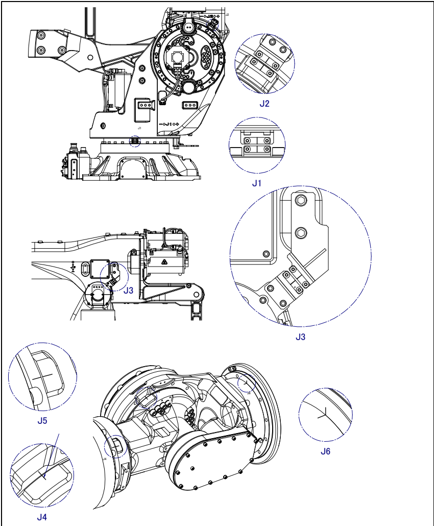
图 8.7 (a) 检测靶标盖板
