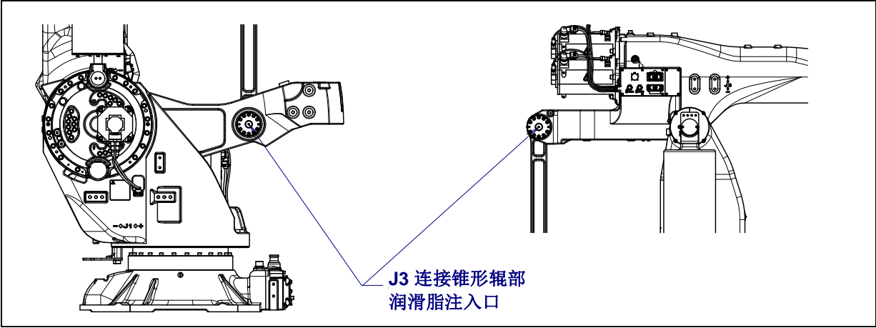
图 7.3.1 (a) J3 连接锥形辊的供脂部位
