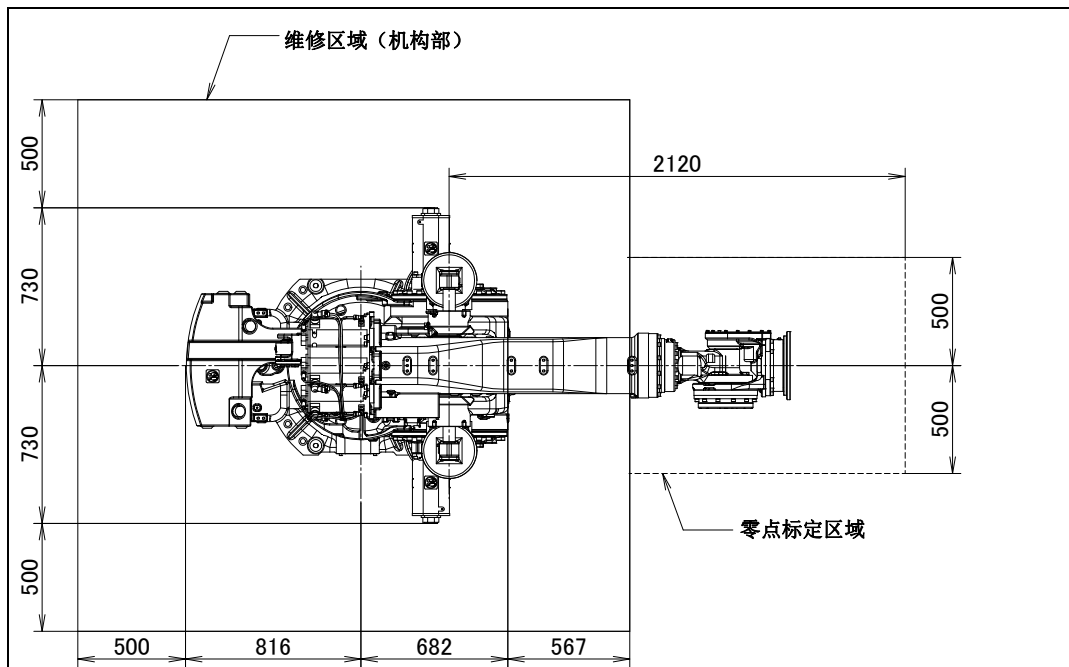
图 1.3 (a) 维修空间的布局图 (M-900iB/700)
