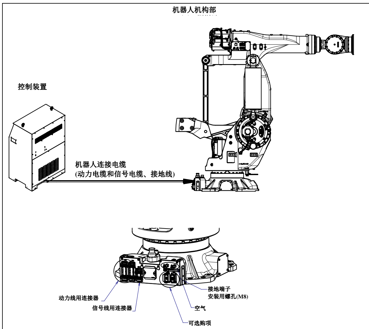
图 2.1 电缆连接图
