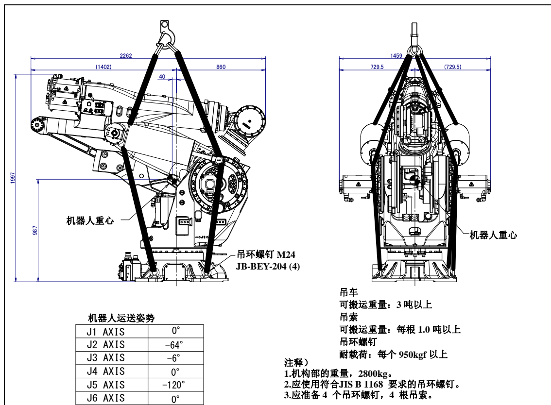
图 1.1 (c) 采用吊车搬运 (M-900iB/700)
