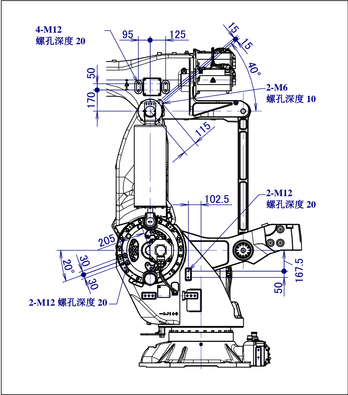
图 4.2 (b) 设备安装面尺寸 (M-900iB/700) (2/2)
