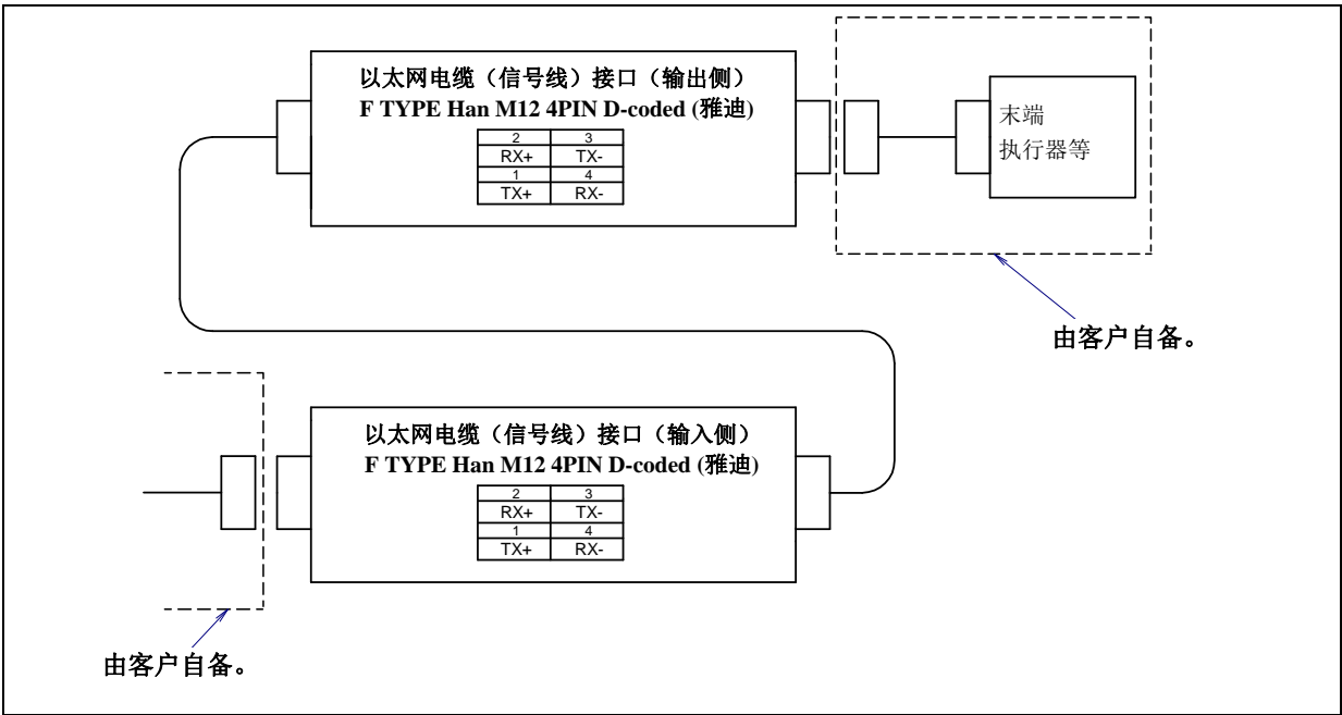
图 5.3 (n) 以太网电缆（信号线）(ES)接口的插针排列（可选项）
