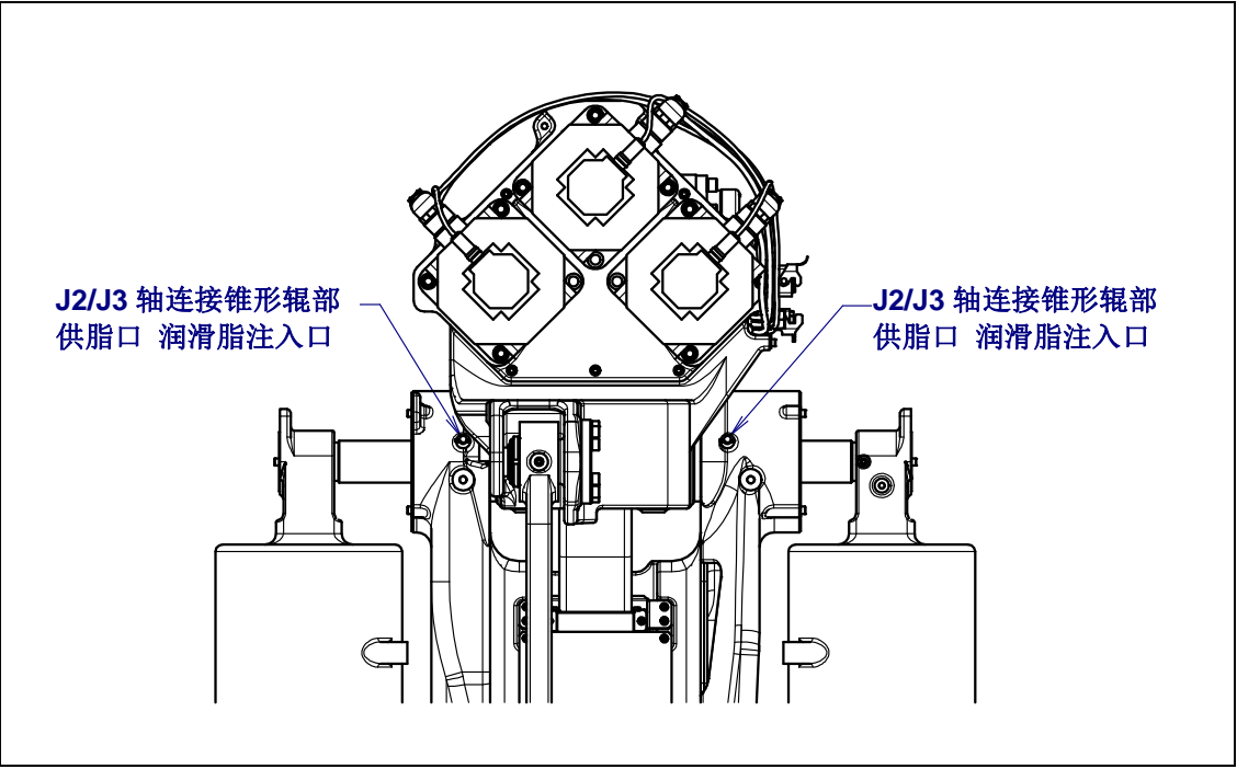
图 7.3.1 (b) J2/J3 轴连接部锥形辊的供脂部位
