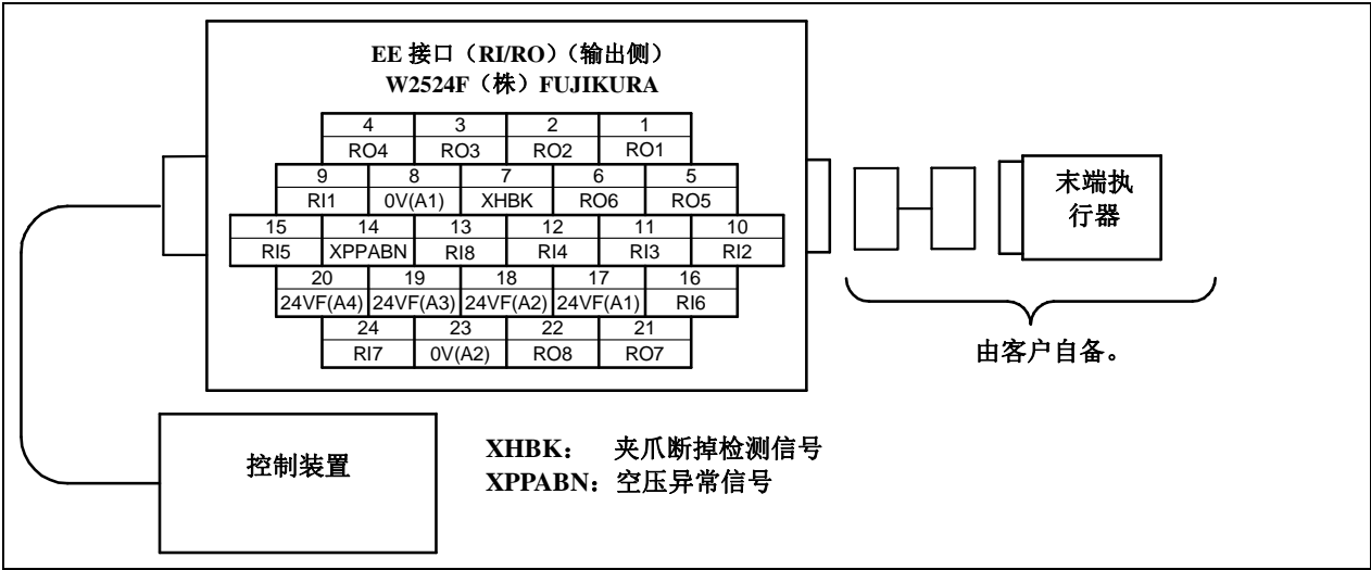
图 5.3 (e) EE 接口(RI/RO)的插针排列 (可选项)
