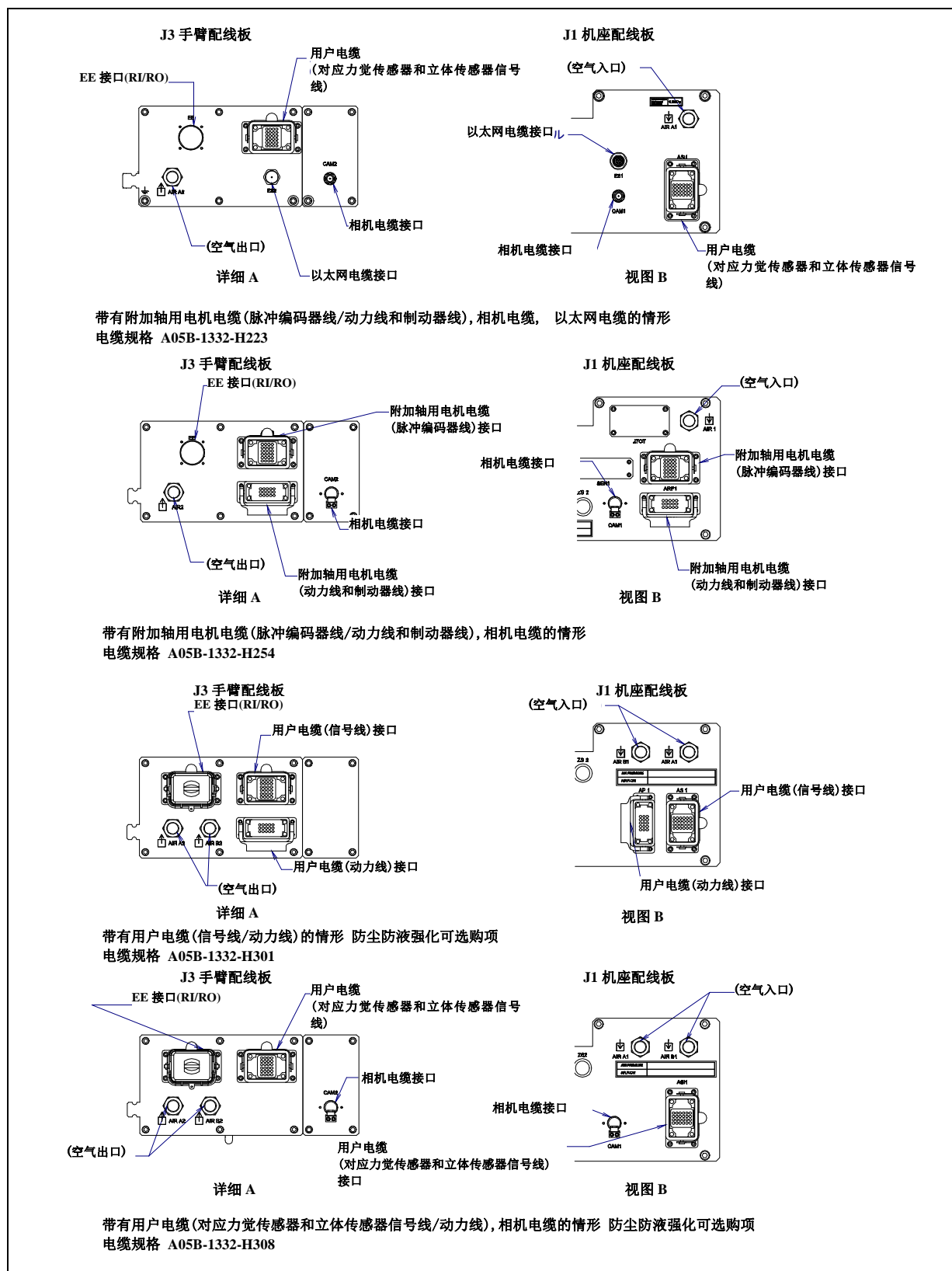
图 5.3 (c) 可选项电缆用接口 (2/3)
