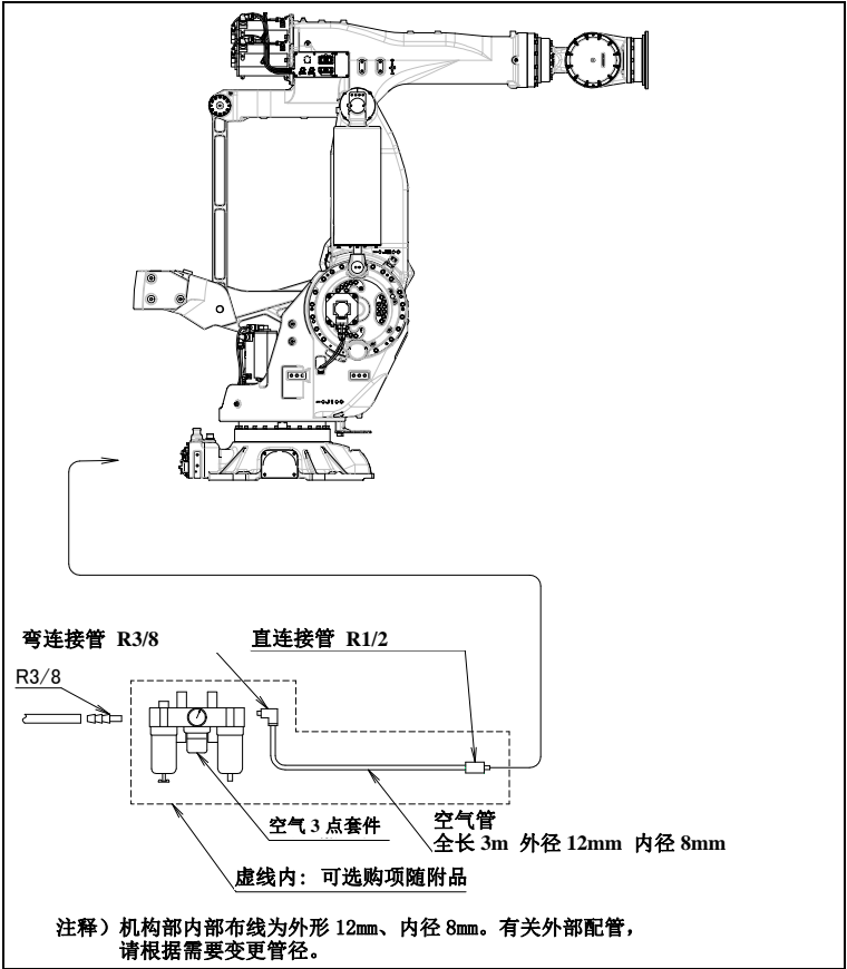
图 5.2 (a) 空气配管（可选项项）
