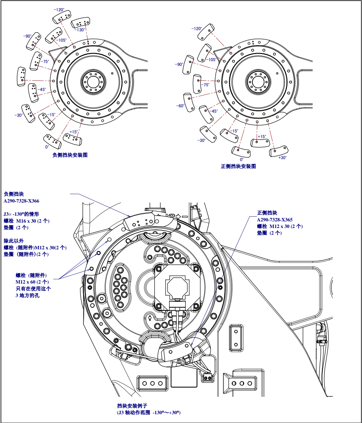
图 6.2 (f) 变更 J3 轴挡块（可选项）
