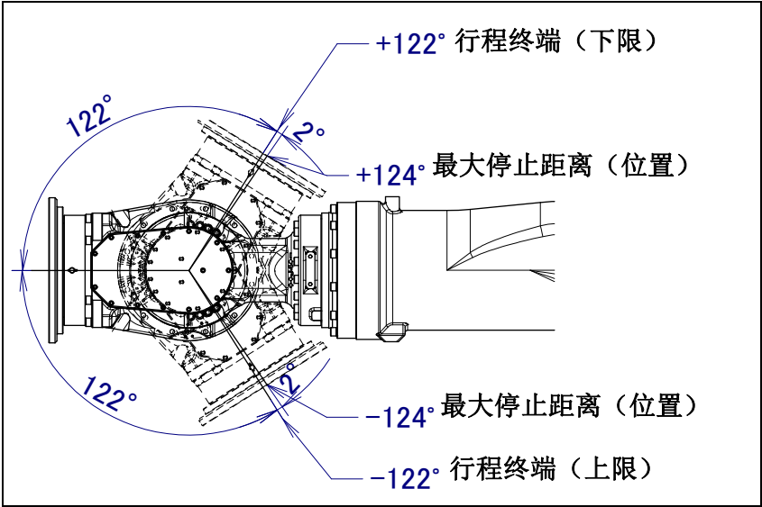
图 3.3 (h) J5 轴可动范围
