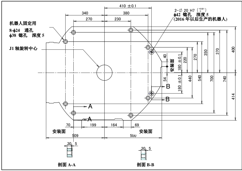
图 1.2 (a) 机器人机座尺寸
