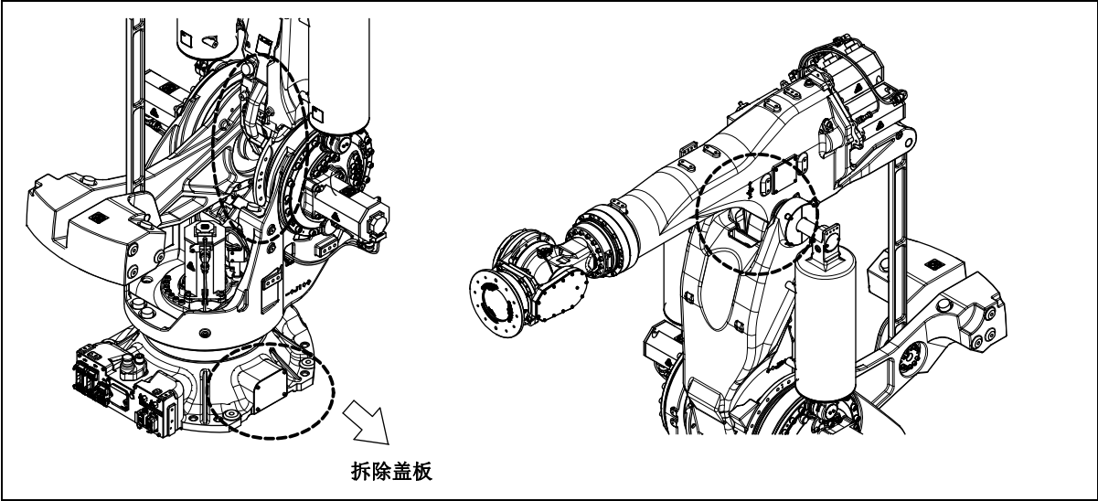
图 7.2.3 (a) 机构部内电缆的检修部位
