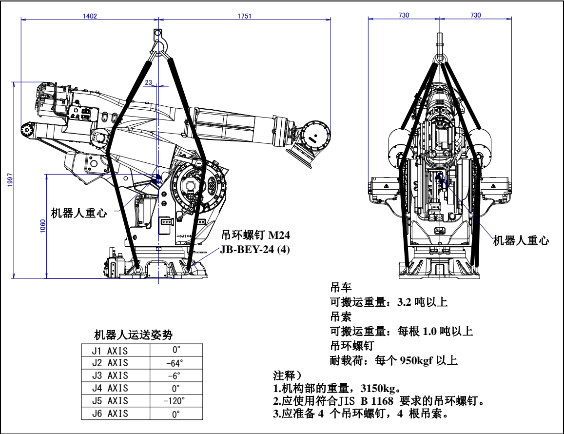
图 1.1 (d) 采用吊车搬运 (M-900iB/400L)
