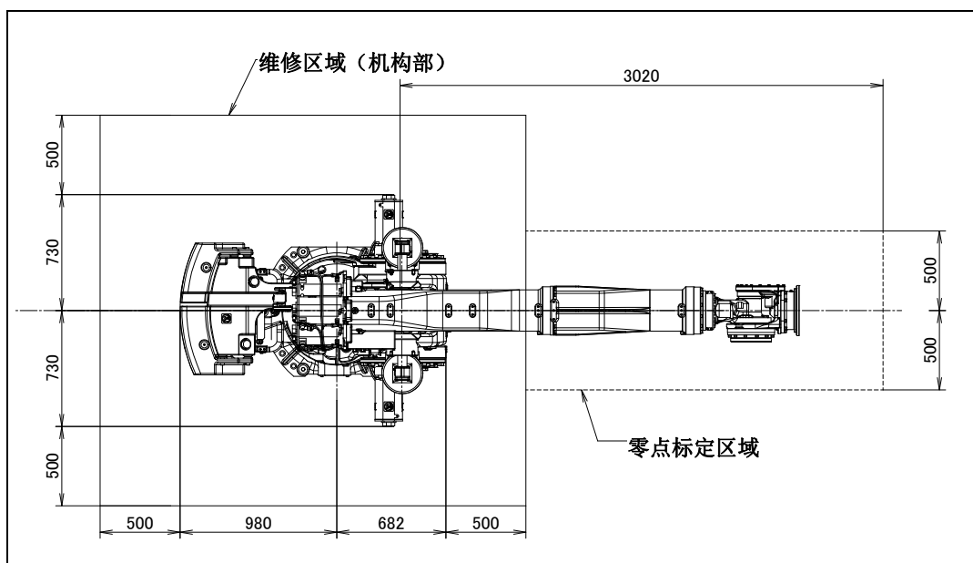
图 1.3 (b) 维修空间的布局图 (M-900iB/400L)
