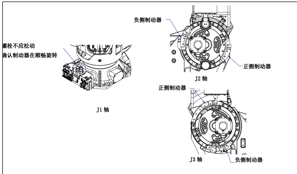
图 7.2.4 机械式固定制动器、机械式可变制动器的检修
