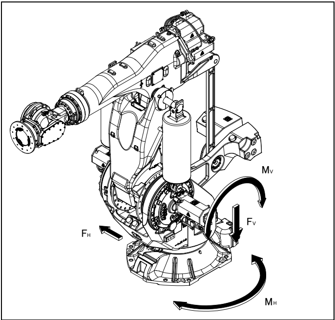
图 1.2.(b) 作用于机器人机座力以及力矩
