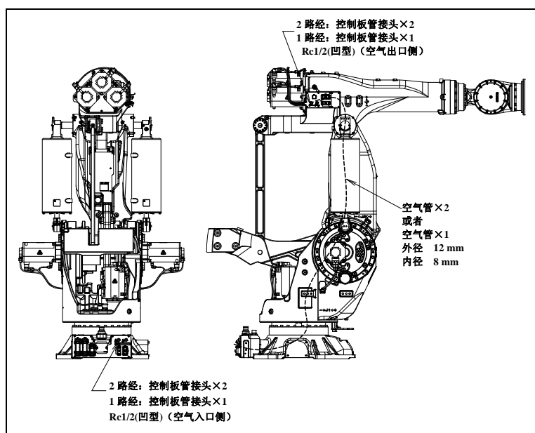
图 5.1 气压供应口（可选项项）
