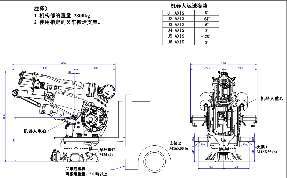
图 1.1 (e) 采用叉车起重机搬运 (M-900iB/700)
