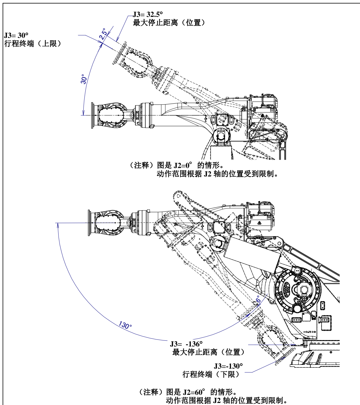
图 3.3 (e) J3 轴可动范围
