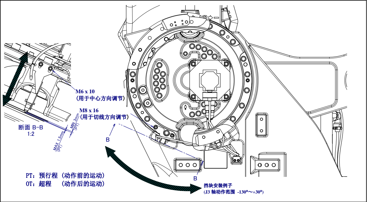
图 6.3 (c) J3 轴限位开关的调节 (可选项)
