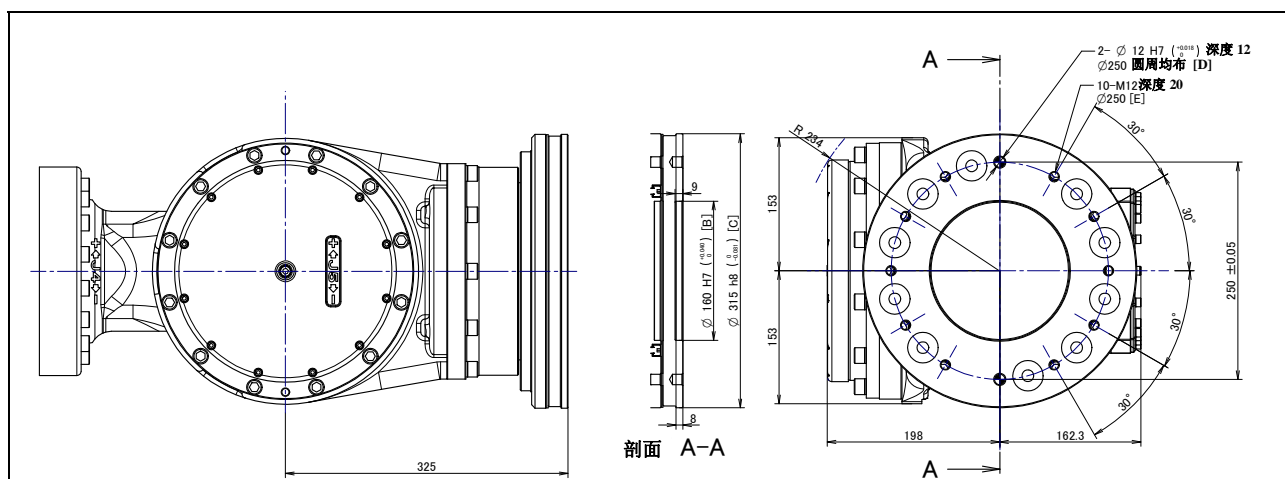
图 4.1 (b) 末端执行器接口尺寸 (绝缘 ISO 法兰盘)
