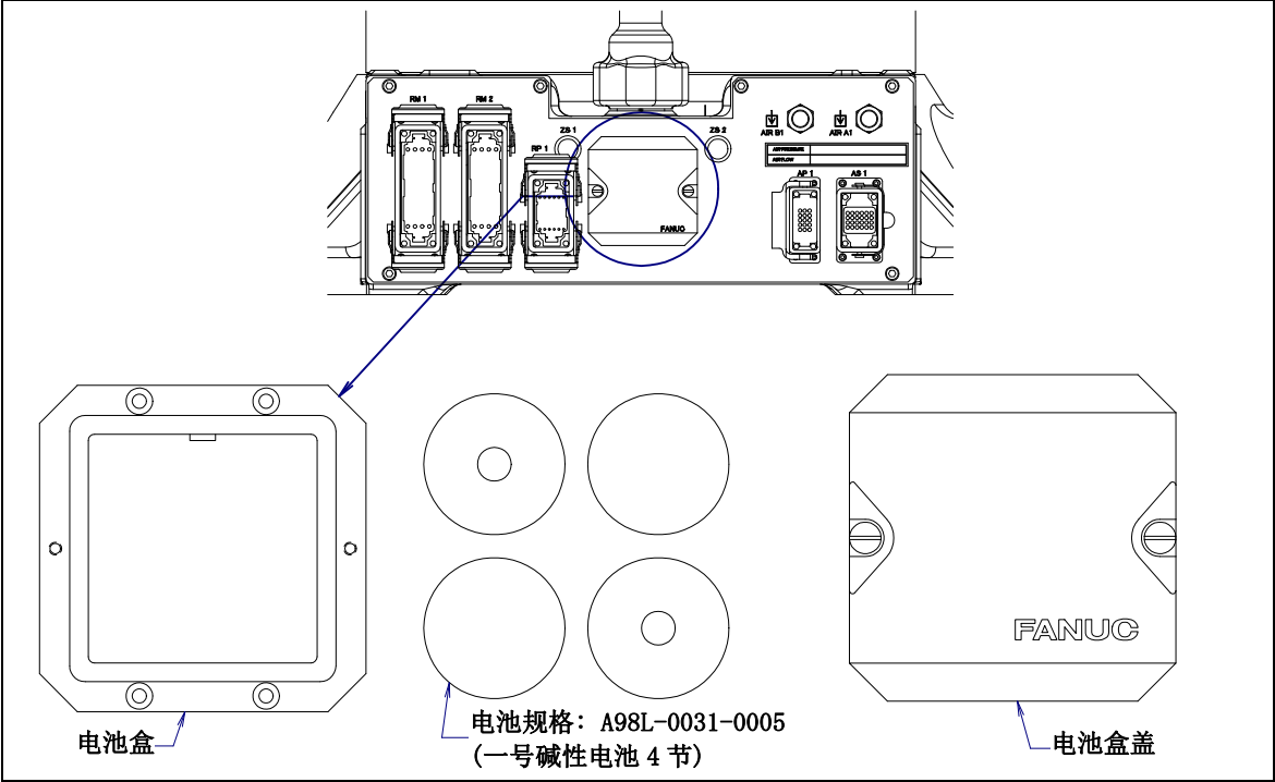
图 7.3.2 (a) 更换电池
