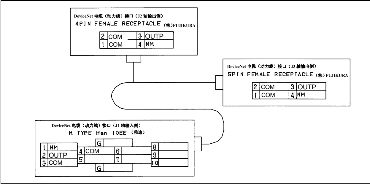
图 5.3 (k) DeviceNet 电缆（动力线）(DP)接口的插针排列（可选项）
