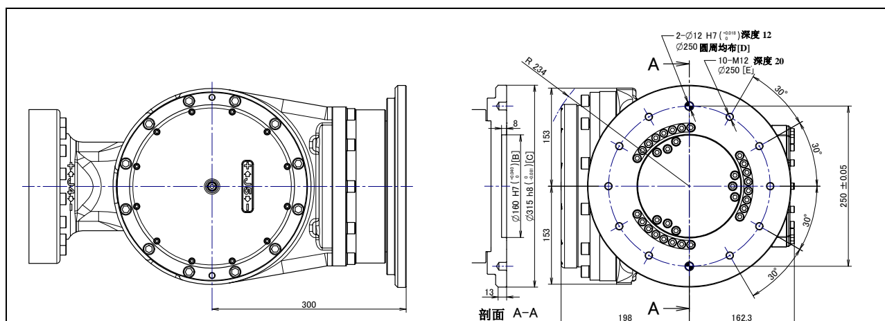
图 4.1 (a) 末端执行器接口尺寸 (ISO 法兰盘)
