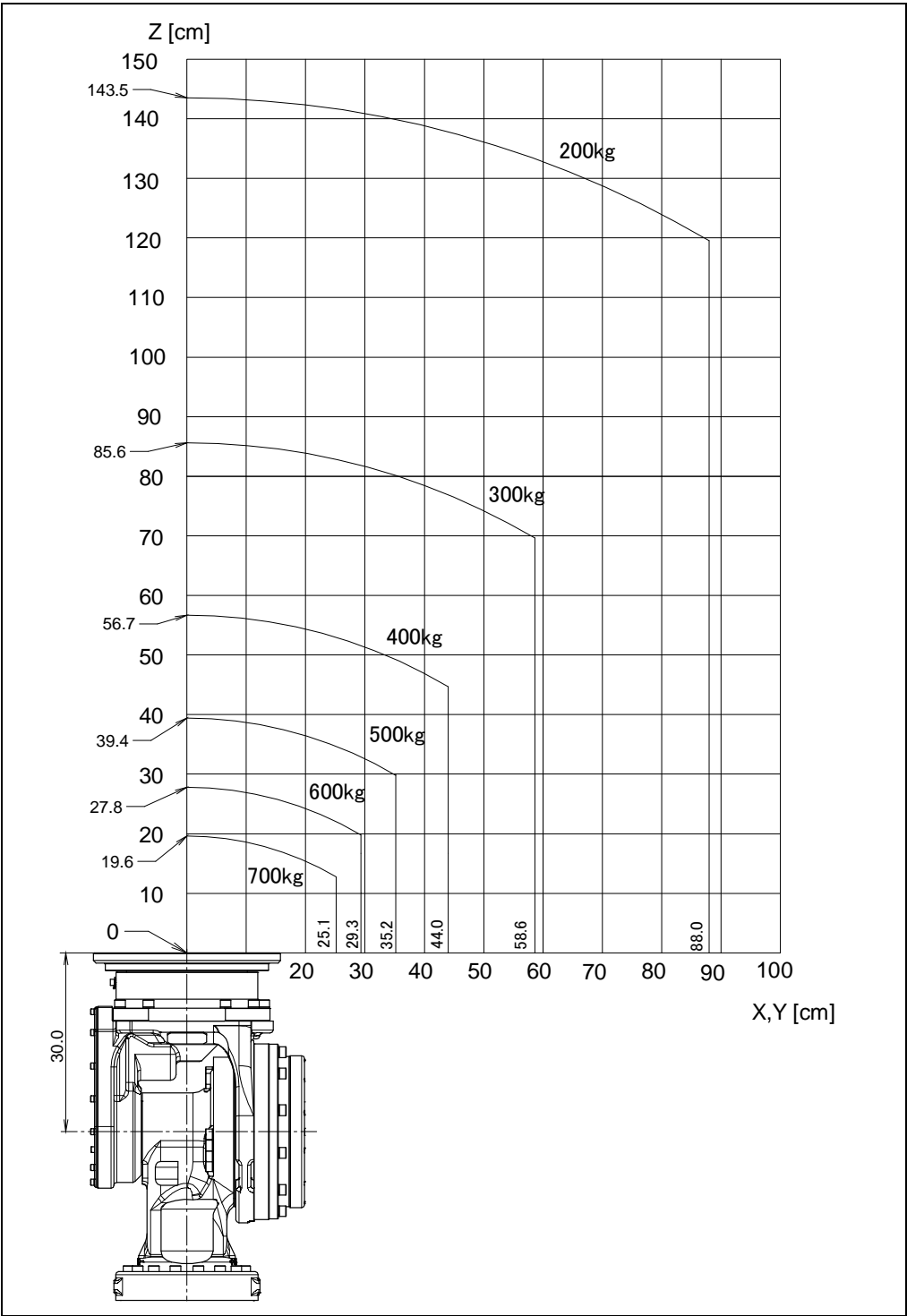
图 3.4 (a) 手腕部允许负载线图(M-900iB/700) (ISO 法兰盘)
