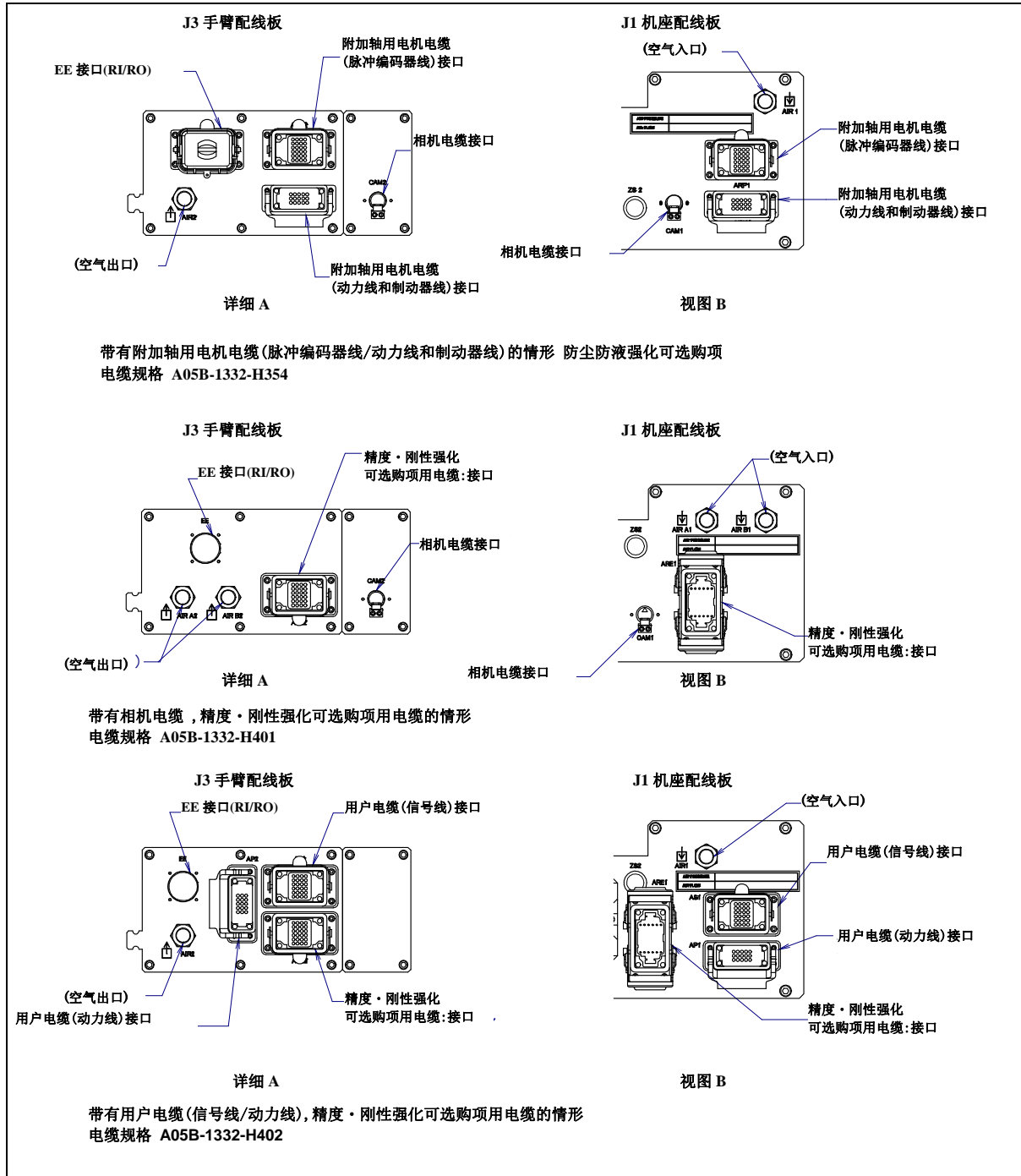
图 5.3 (d) 可选项项电缆用接口 (3/3)
