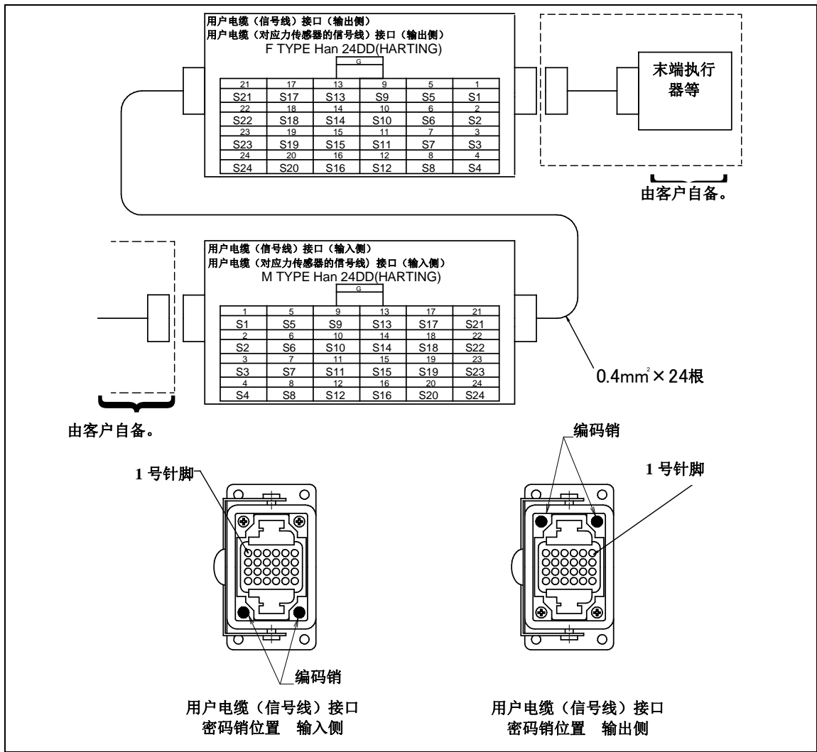
图 5.3 (g) 用户电缆（信号线）(AS)接口的插针排列和编码销的配置位置（可选项项）
