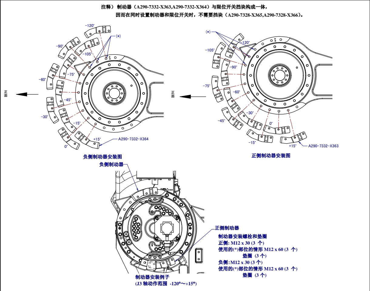
图 6.2 (c) 变更 J3 轴机械式可变制动器 (可选项)
