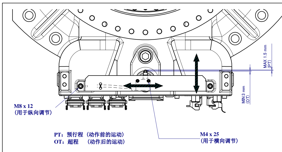
图 6.3 (a) J1 轴限位开关的调节 (可选项)
