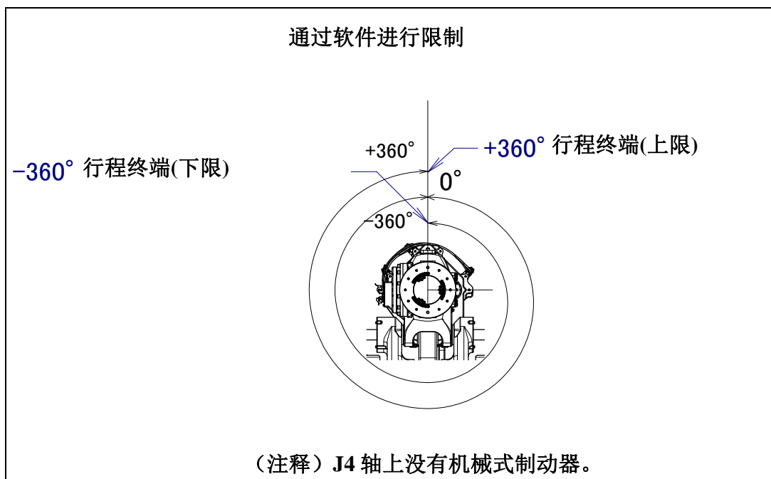
图 3.3 (f) J4 轴可动范围
