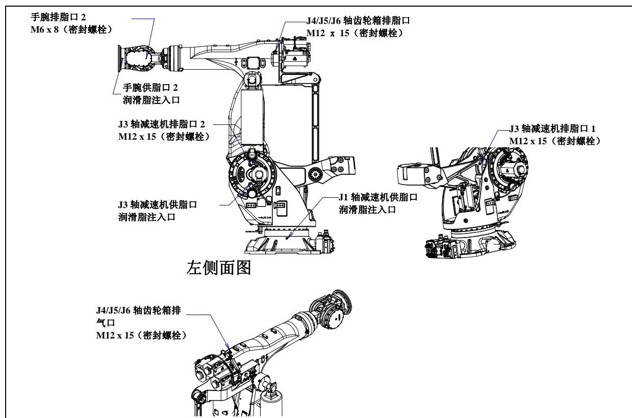
图 7.3.3 (a) 更换减速机的润滑脂 (1/2)
