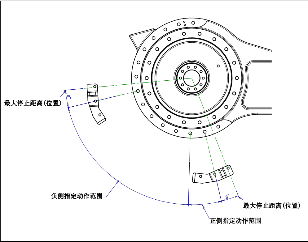
图 6.2 (i) J3 轴机械式可变制动器的最大停止距离（位置）
