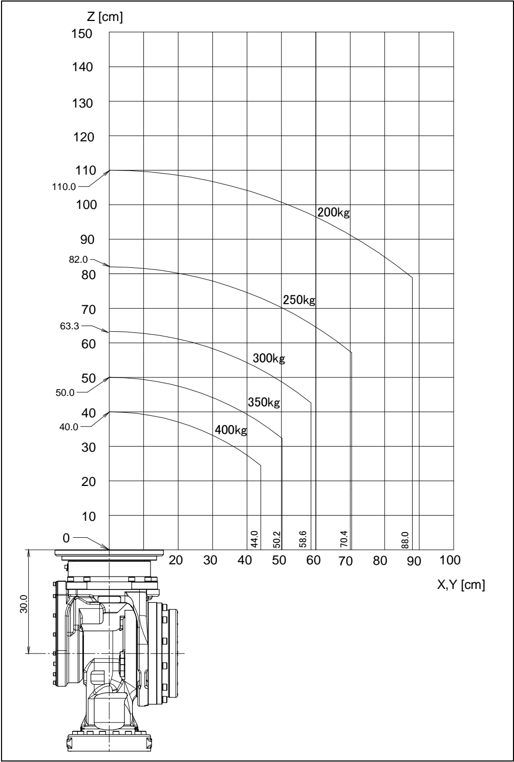
图 3.4 (c) 手腕部允许负载线图 (M-900iB/400L) (ISO 法兰盘)
