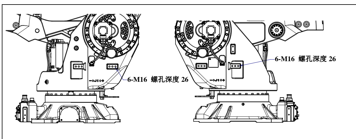
图 1.1 (b) 叉车搬运支架安装位置
