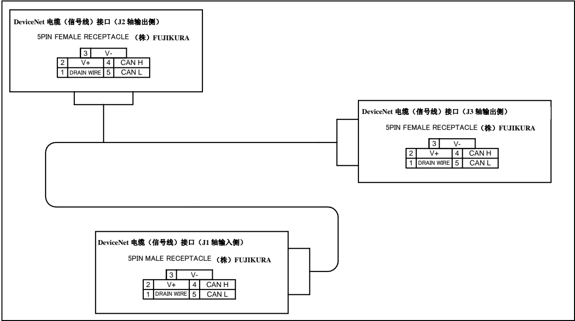
图 5.3 (j) DeviceNet 电缆（信号线）(DS)接口的插针排列（可选项）
