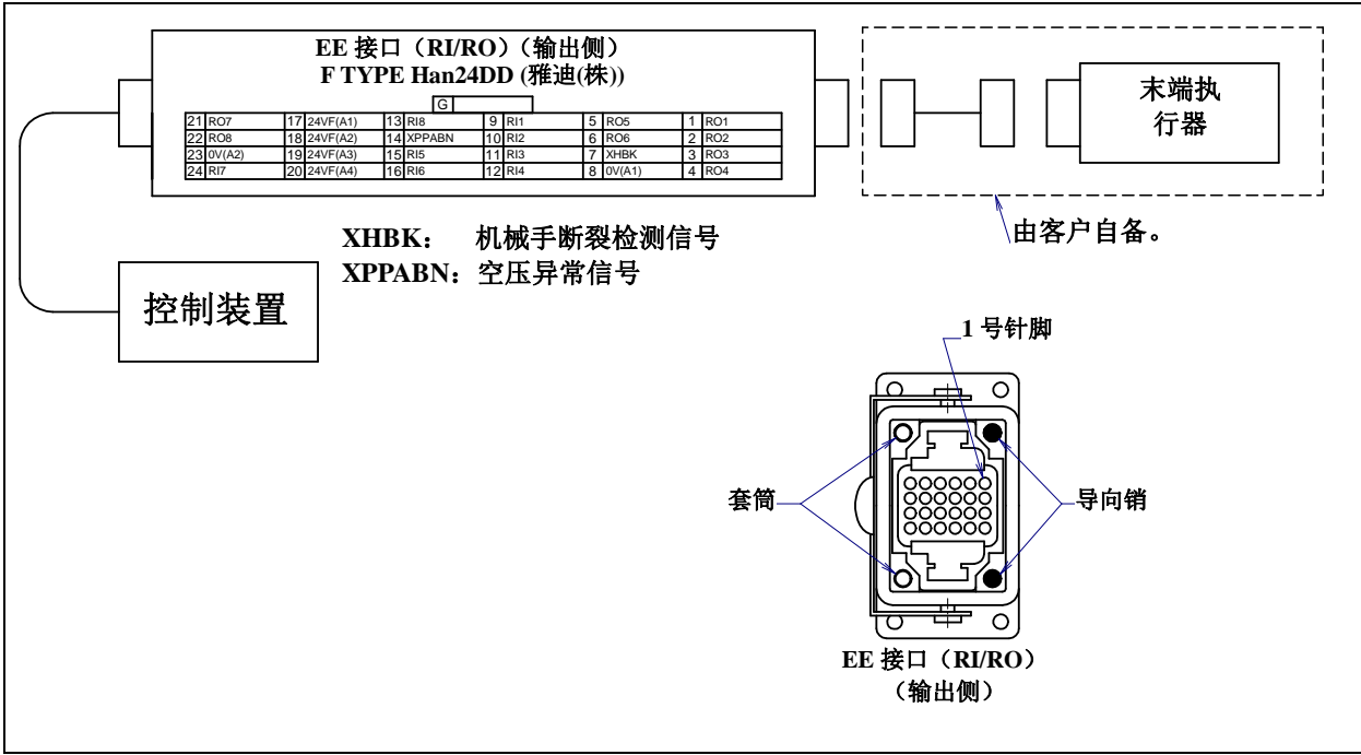
图 5.3 (f) EE 接口(RI/RO) (选择防尘防液强化组件时) 的插针排列 (可选项)
