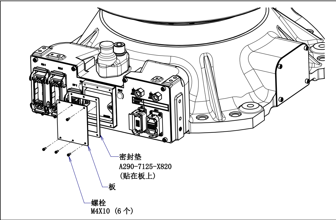
图 7.3.2 (b) 电池盖板的拆除 (指定防尘防液强化可选项时)
