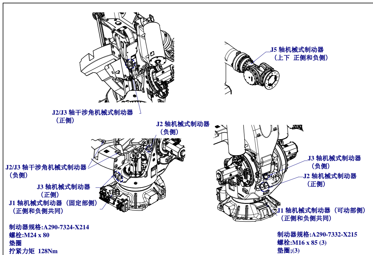
图 3.3 (a) 机械式制动器的位置
