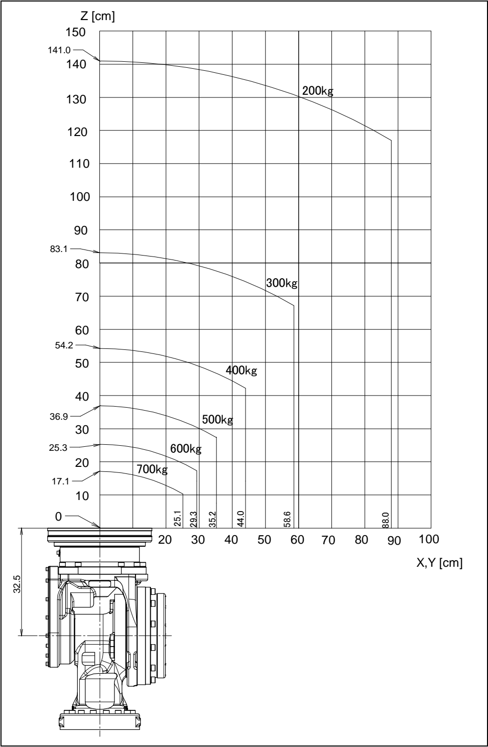
图 3.4 (b) 手腕部允许负载线图(M-900iB/700) (绝缘 ISO 法兰盘)
