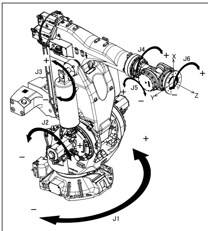
图 3.1 (b) 各轴坐标和机械接口坐标
