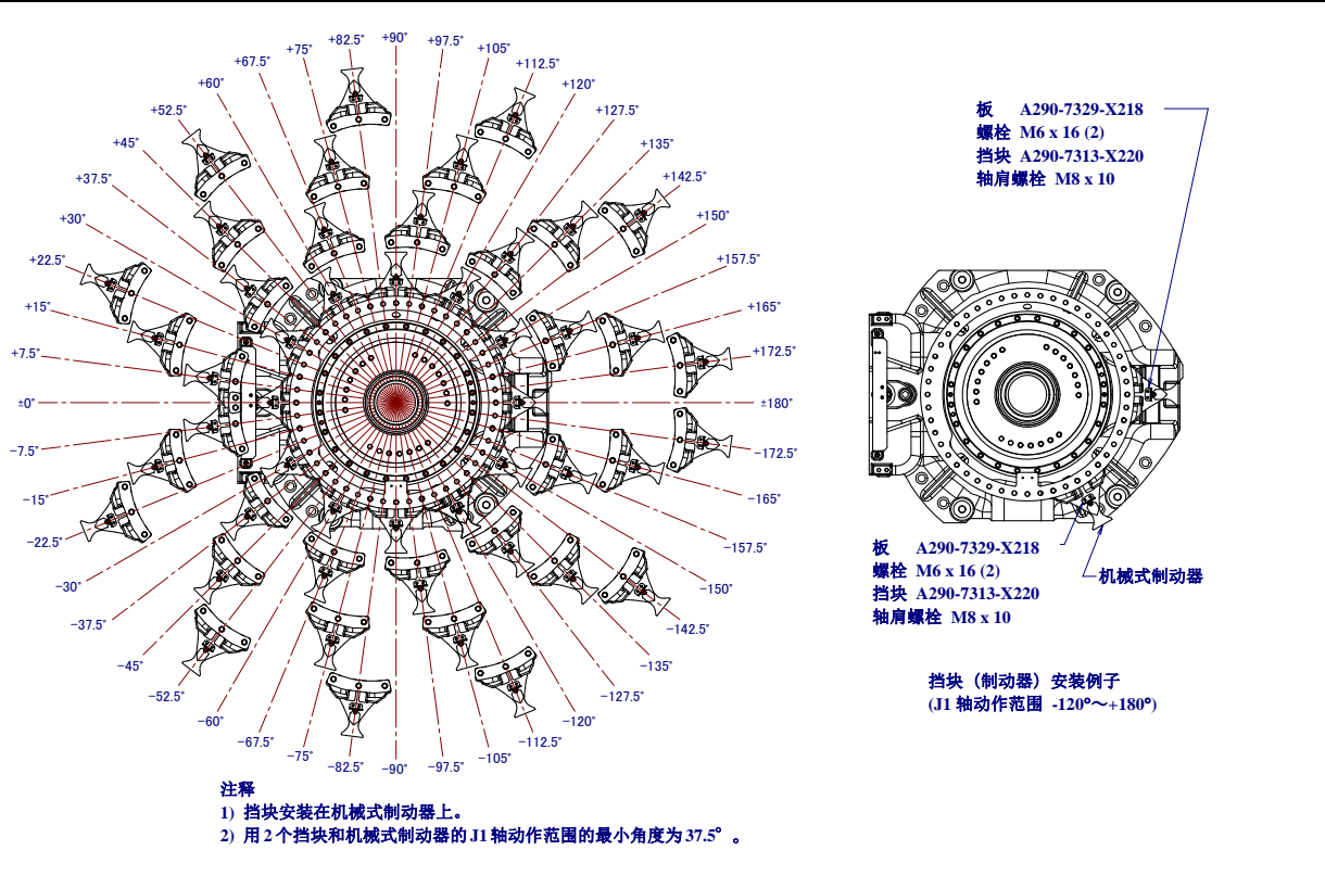
图 6.2 (d) 变更 J1 轴挡块 (可选项)
