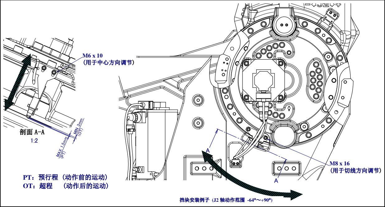
图 6.3 (b) J2 轴限位开关的调节 (可选项)
