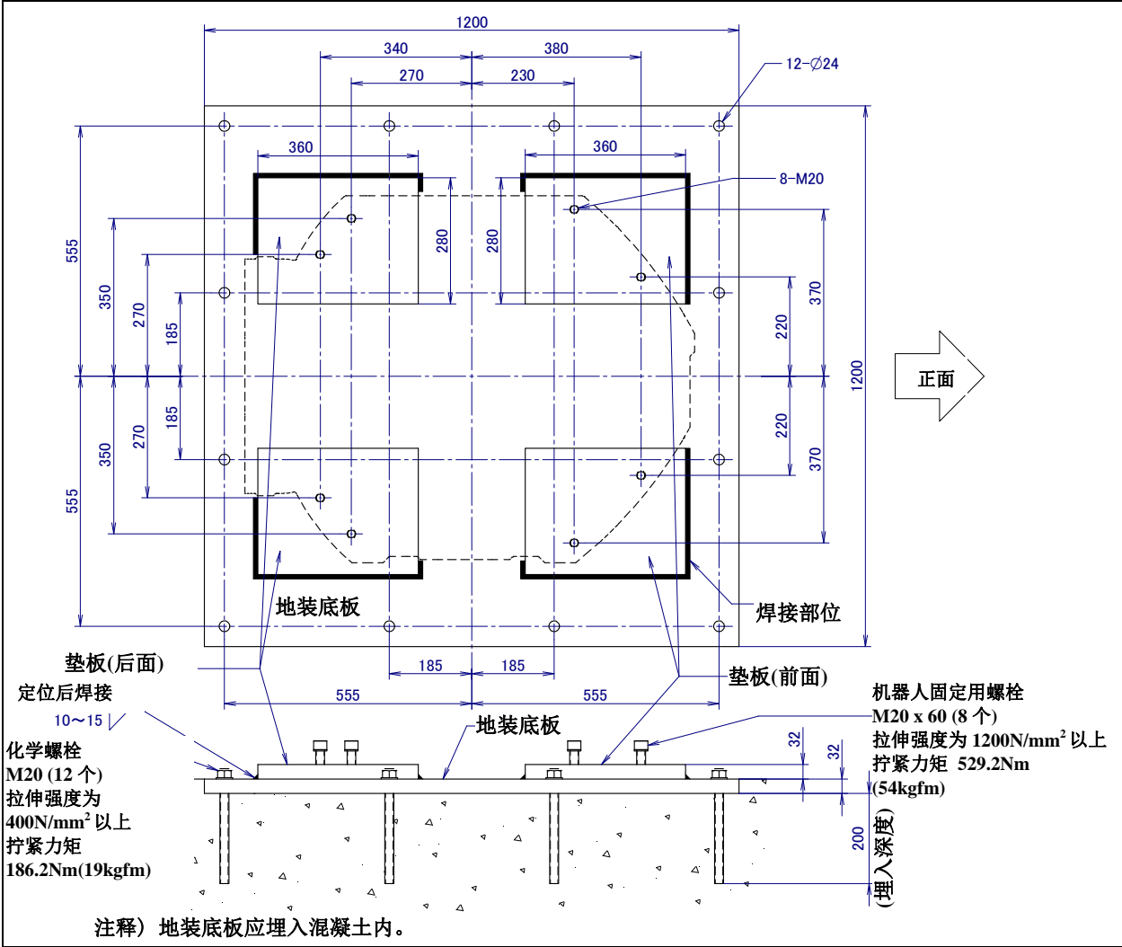
图 1.2.1 安装方法
