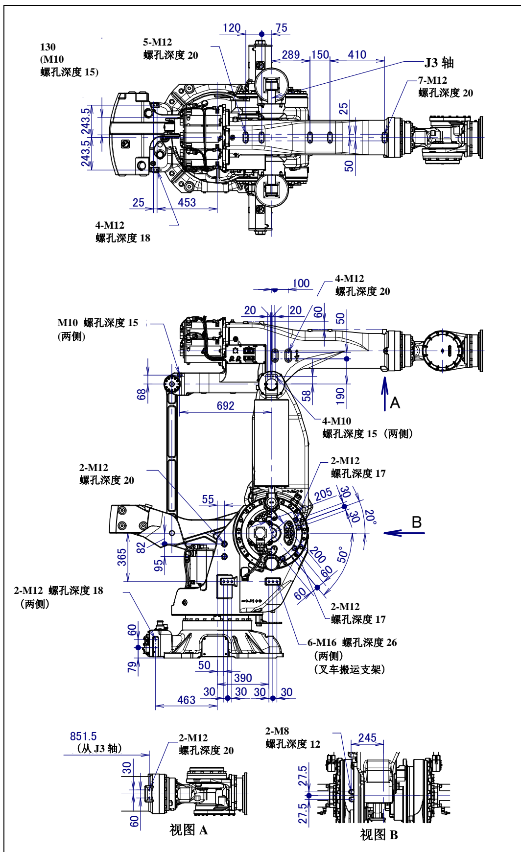
图 4.2 (a) 设备安装面尺寸(M-900iB/700) (1/2)
