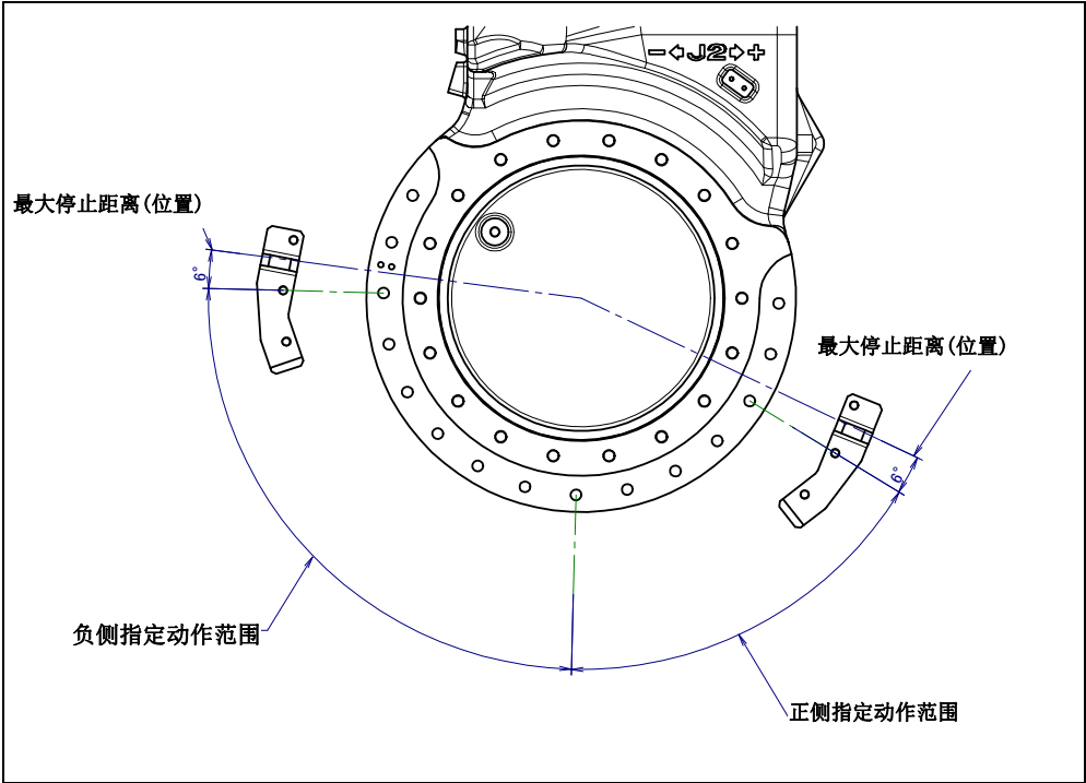
图 6.2 (h) J2 轴机械式可变制动器的最大停止距离（位置）
