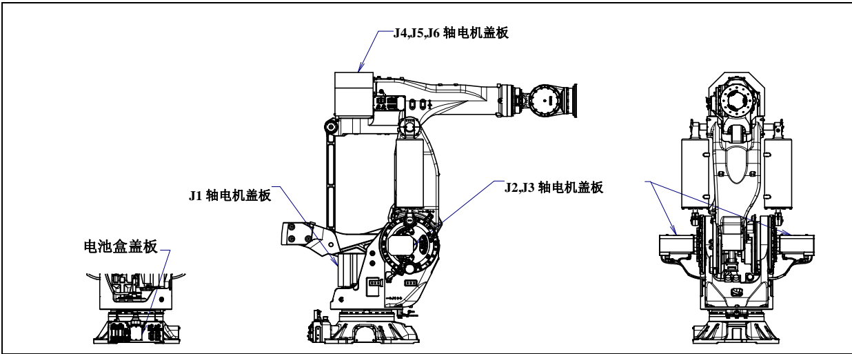
图 10.2 防尘防液强化组件的构成
