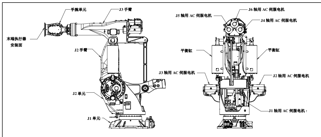
图 3.1 (a) 机构部的构成
