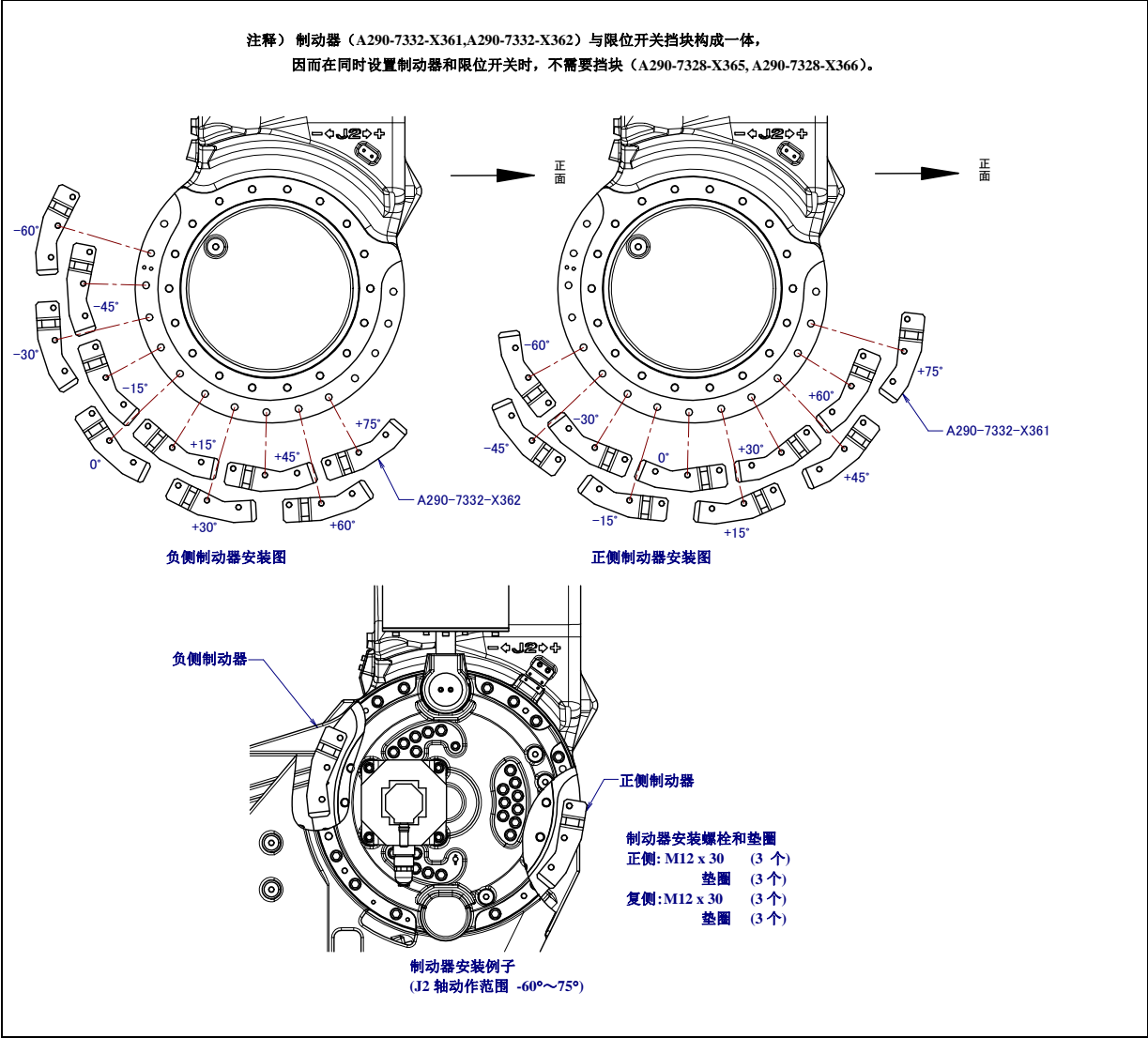
图 6.2 (b) 变更 J2 轴机械式可变制动器 (可选项)
