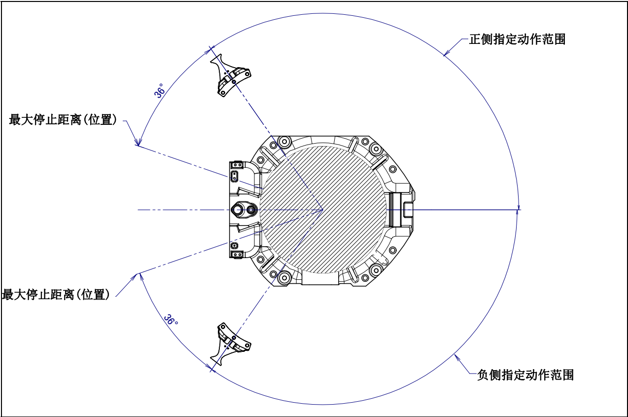
图 6.2 (g) J1 轴机械式可变制动器的最大停止距离（位置）
