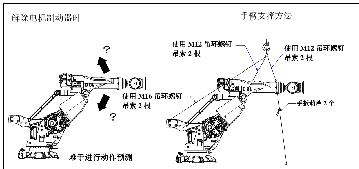
图 5.4 (b) 解除 J3 轴的电机制动器造成的手臂动作和事先采取的措施例
