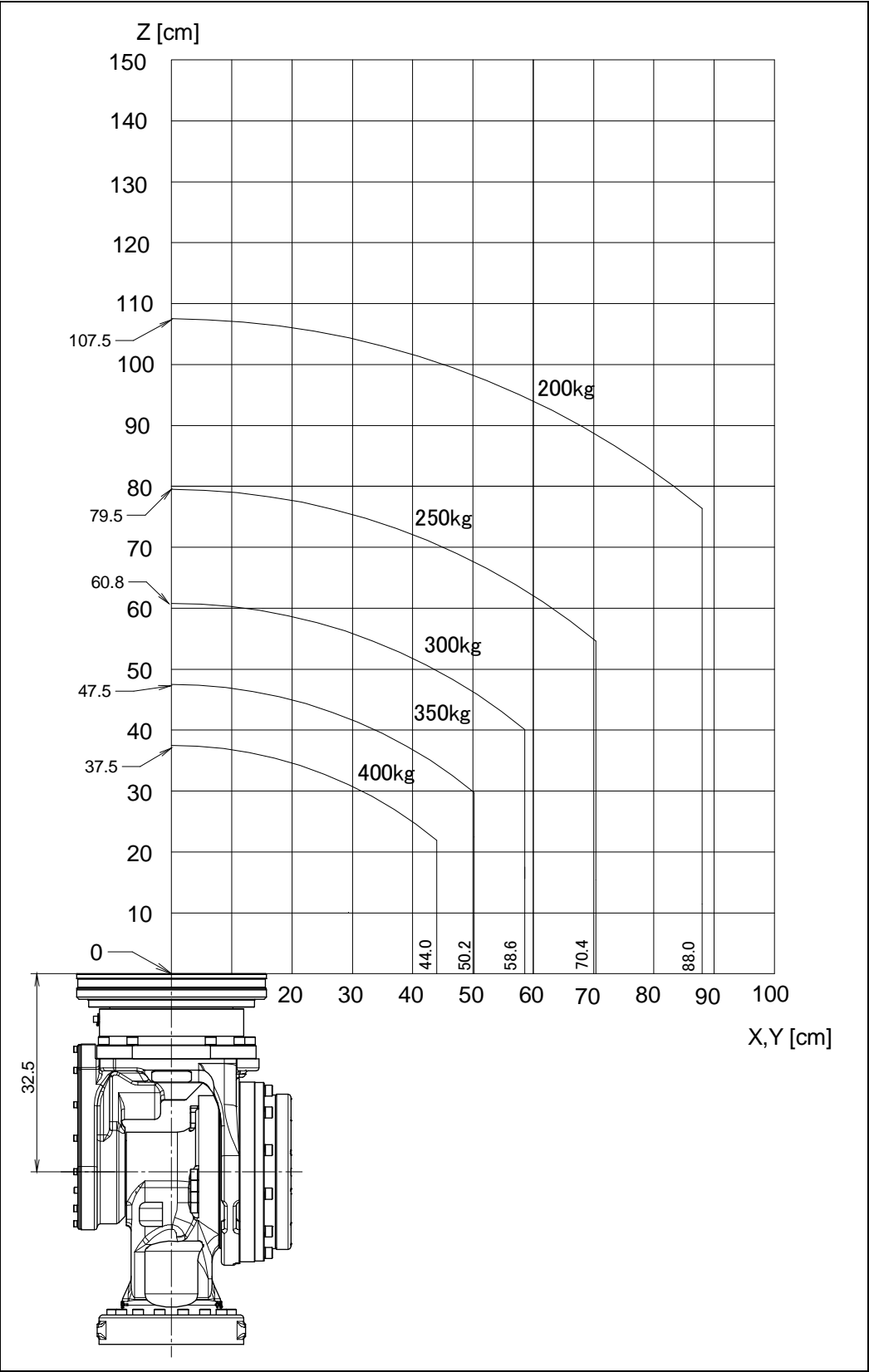
图 3.4 (d) 手腕部允许负载线图(M-900iB/400L) (绝缘 ISO 法兰盘)
