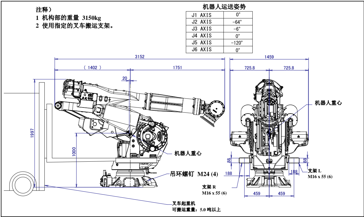
图 1.1 (f) 采用叉车起重机搬运 (M-900iB/400L)
