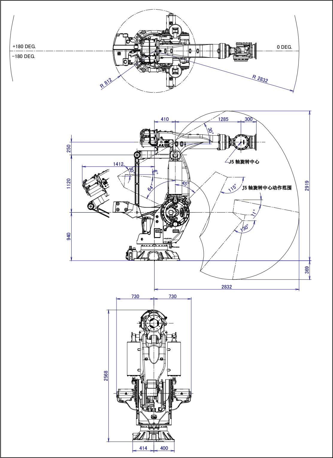
图 3.2 (a) 动作范围图 (M-900/B/700)
