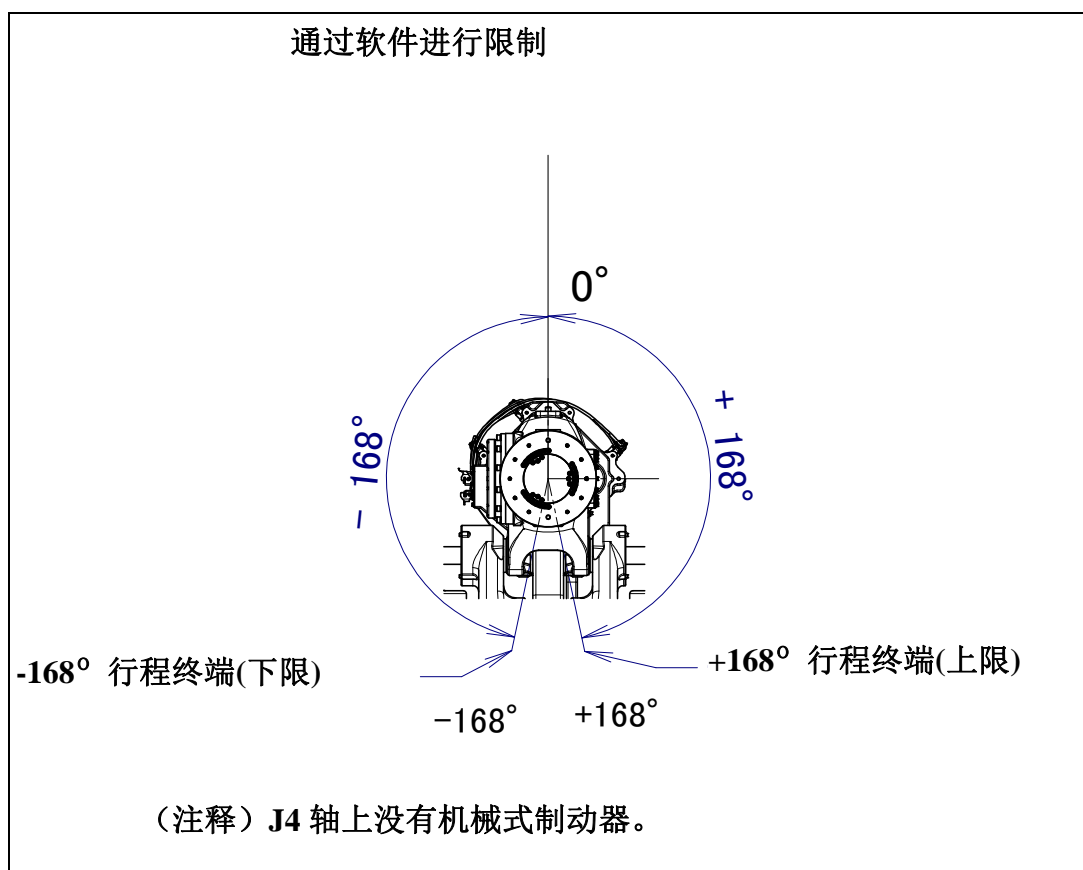
图 3.3 (g) J4 轴可动范围 (指定精度·刚性强化可选项时)
