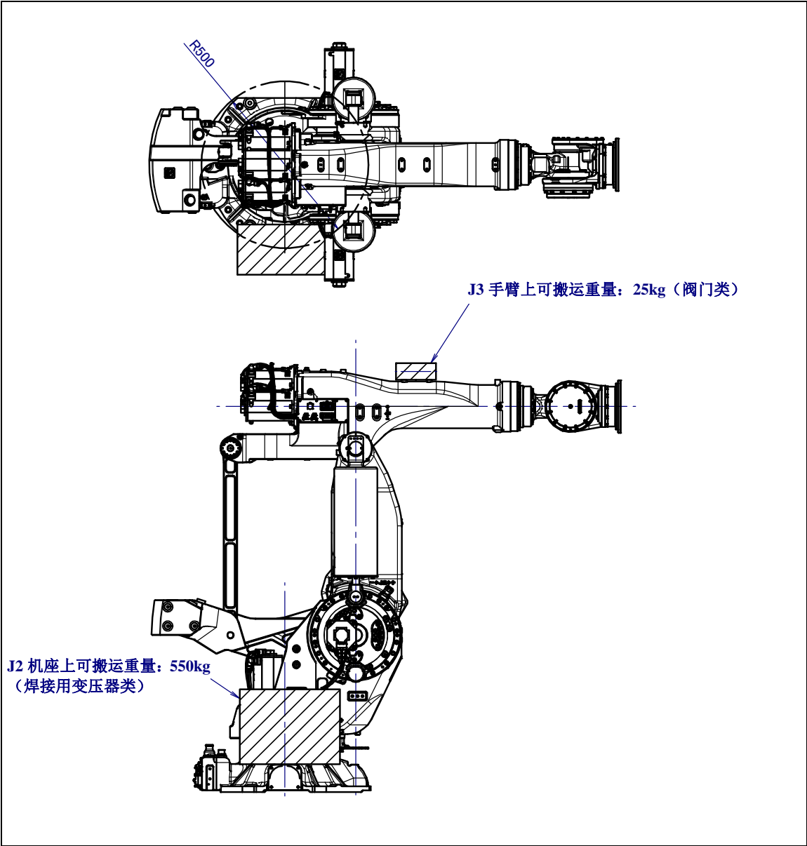
图 3.5 J2 机座/J3 手臂部的负载条件
