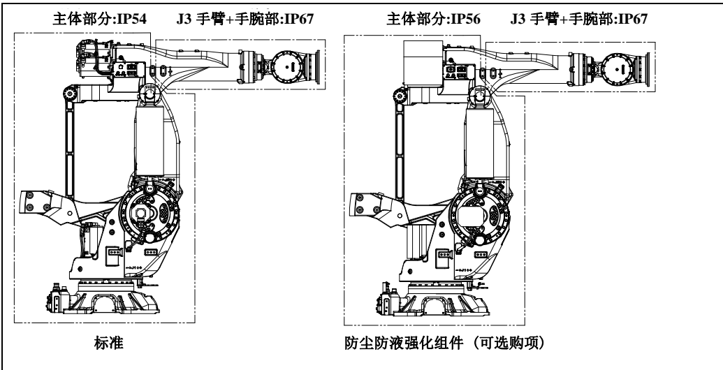
图3.1 (c) M-900iB 的防尘防液性能
