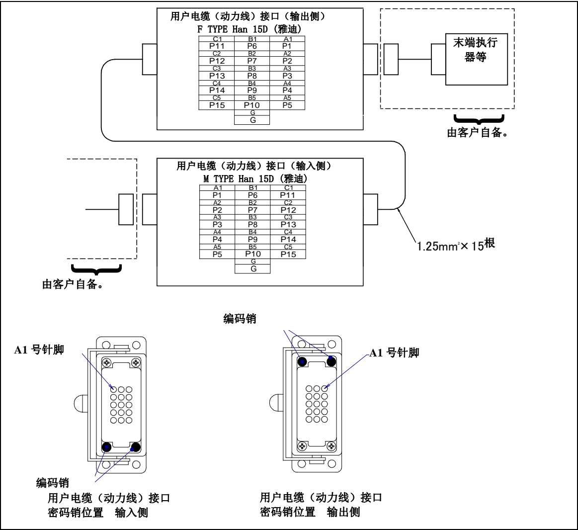
图 5.3 (i) 用户电缆（动力线）(AP)接口的插针排列和编码销配置位置（可选项项）
