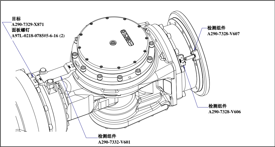
图 8.7 (b) 可拆装式检测靶标
