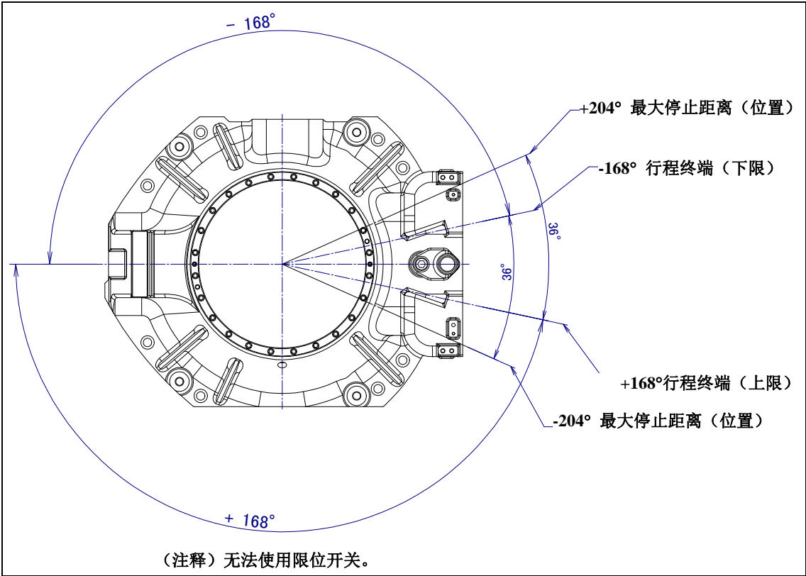
图 3.3 (c) J1 轴可动范围 (指定精度・刚性强化可选购项时)
