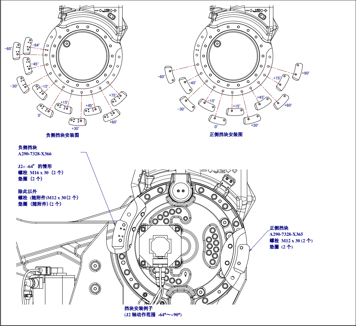
图 6.2 (e) 变更 J2 轴挡块 (可选项)
