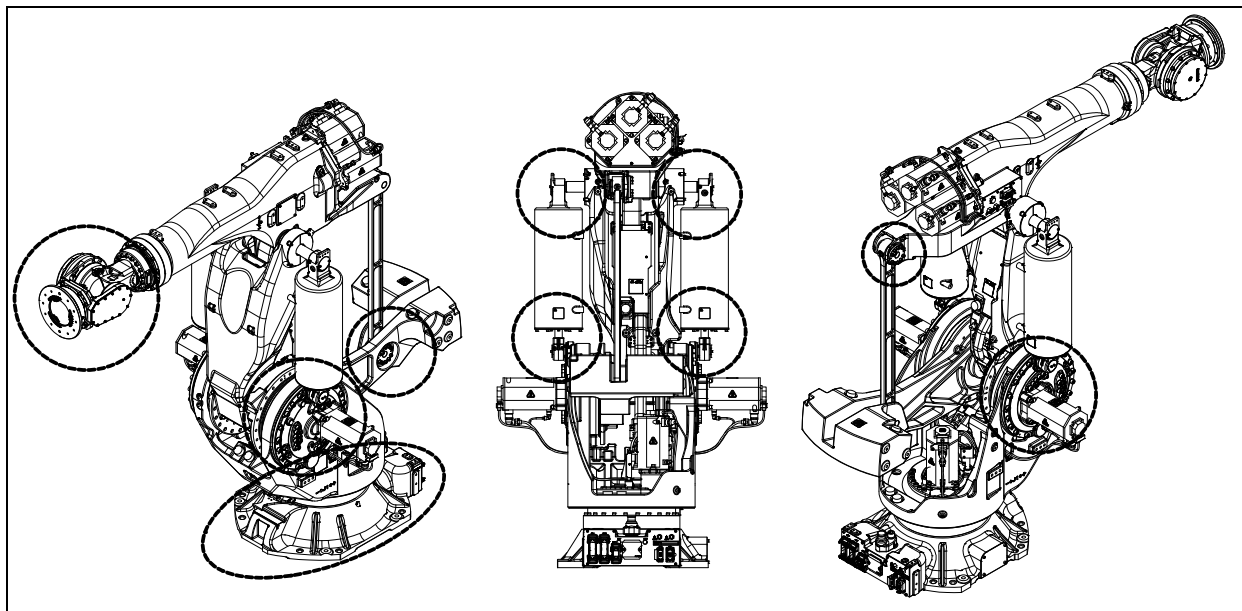
图 7.2.1 渗油的检查部位
