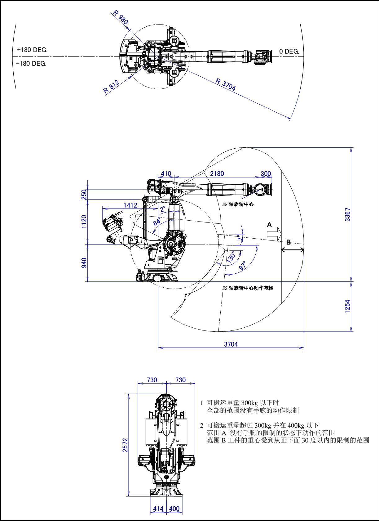
图 3.2 (b) 动作范围图 (M-900iB/400L)
