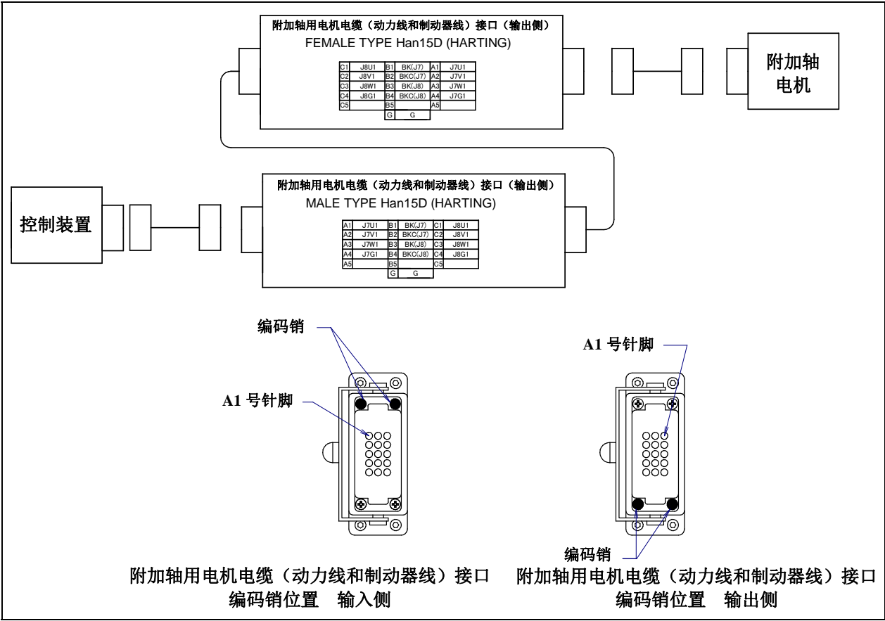
图 5.3 (m) 附加轴用电机电缆（动力线和制动器线）(ARM)接口的插针排列和编码销配置位置（可选项）
