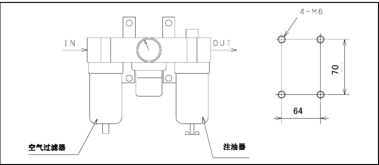
图 5.2 (b) 空气 3 点套件（可选项项）
