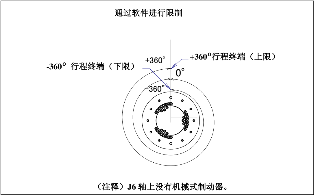
图 3.3 (i) J6 轴可动范围
