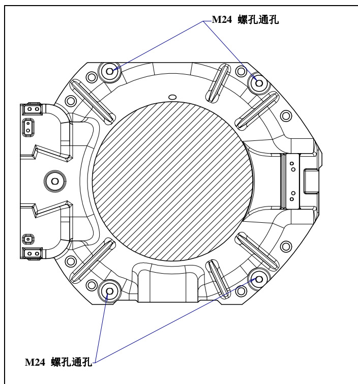
图 1.1 (a) 吊环螺钉安装位置
