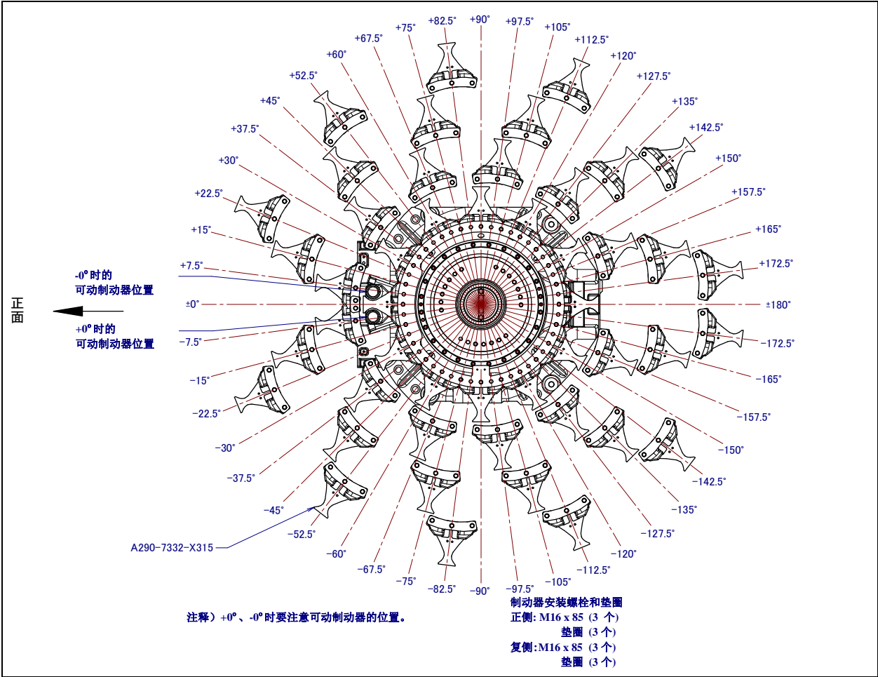
图 6.2 (a) 变更 J1 轴机械式可变制动器 (可选项)
