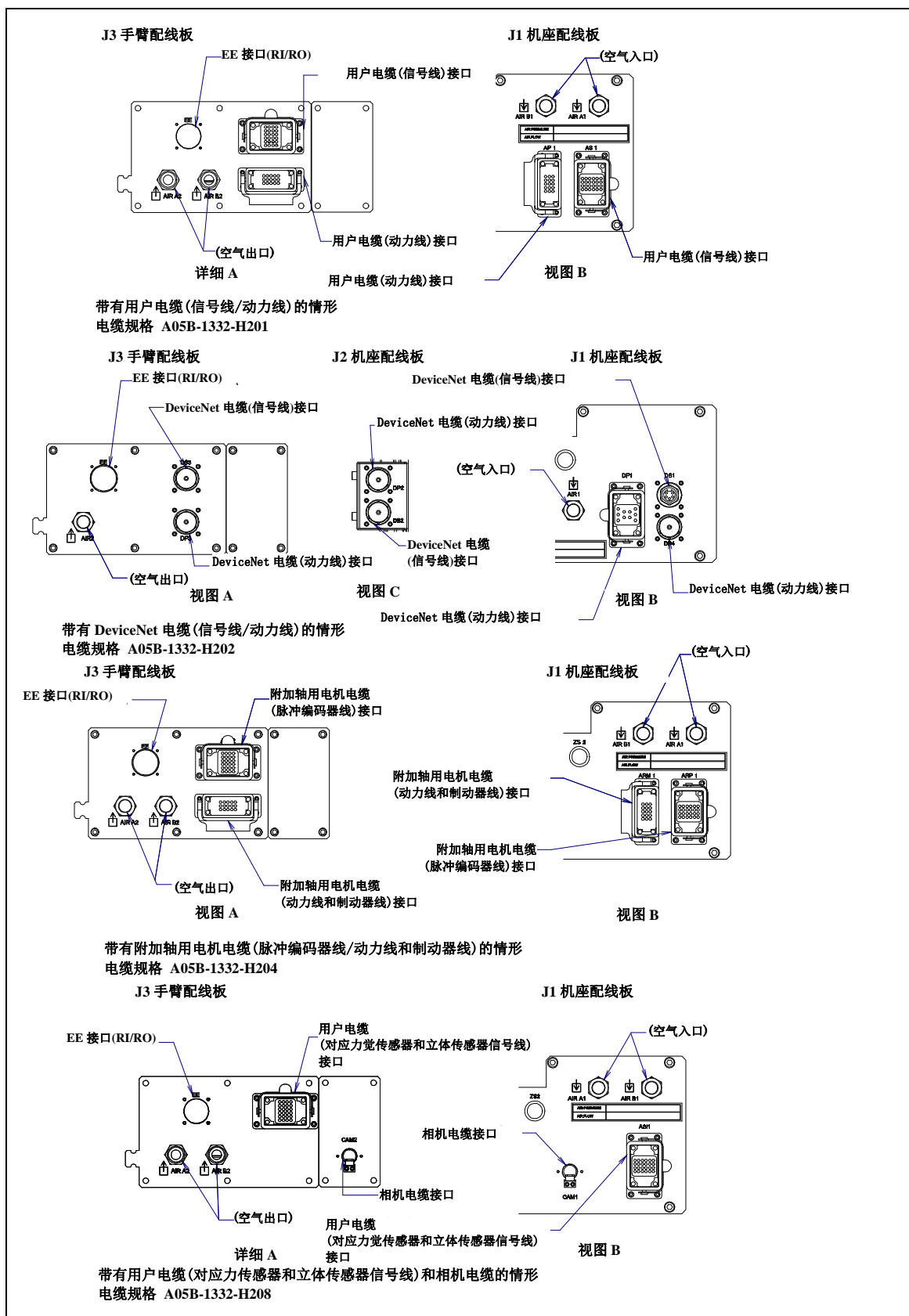
图 5.3 (b) 可选项项电缆用接口 (1/3)
