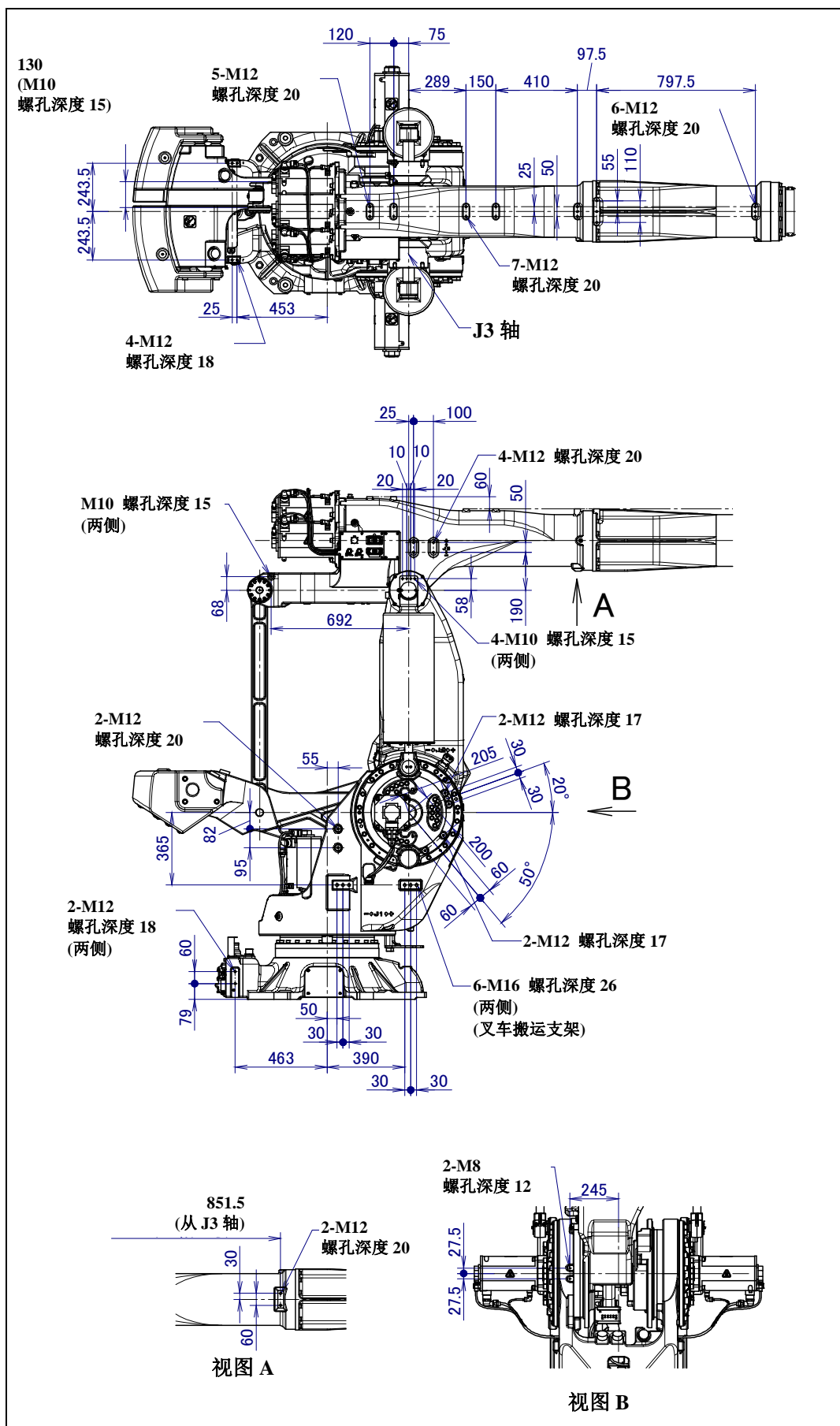
图 4.2 (c) 设备安装面尺寸(M-900iB/400L) (1/2)
