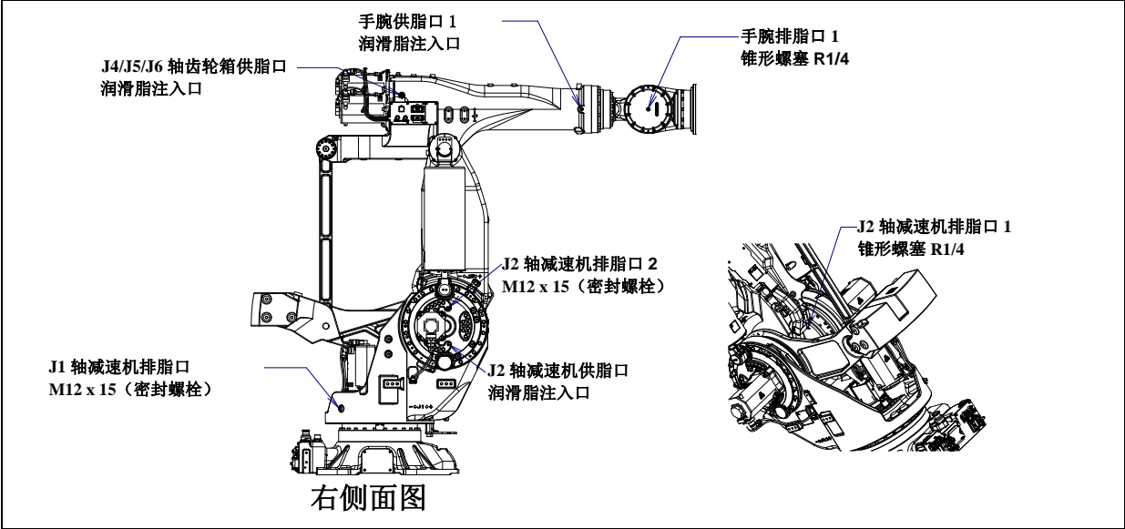
图 7.3.3 (b) 更换减速机的润滑脂 (2/2)
