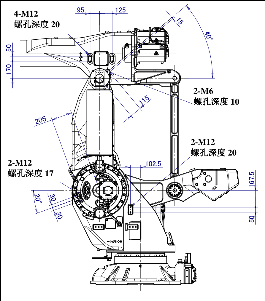
图 4.2 (d) 设备安装面尺寸 (M-900iB/400L) (2/2)
