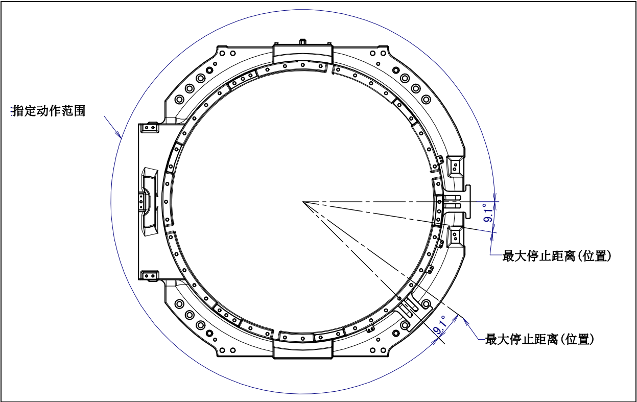
图 6.2.3 (g) J1 轴机械式可变制动器的最大停止距离(位置) (M-2000iA/1700L)
