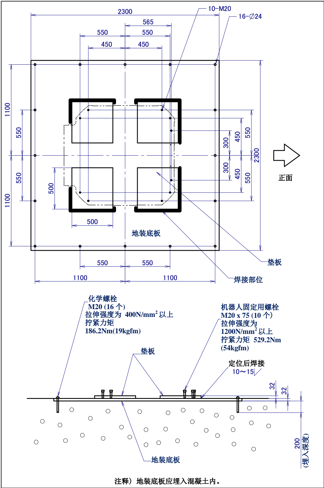
图 1.2.1 (a) 安装方法(M-2000iA/1200/900L)
