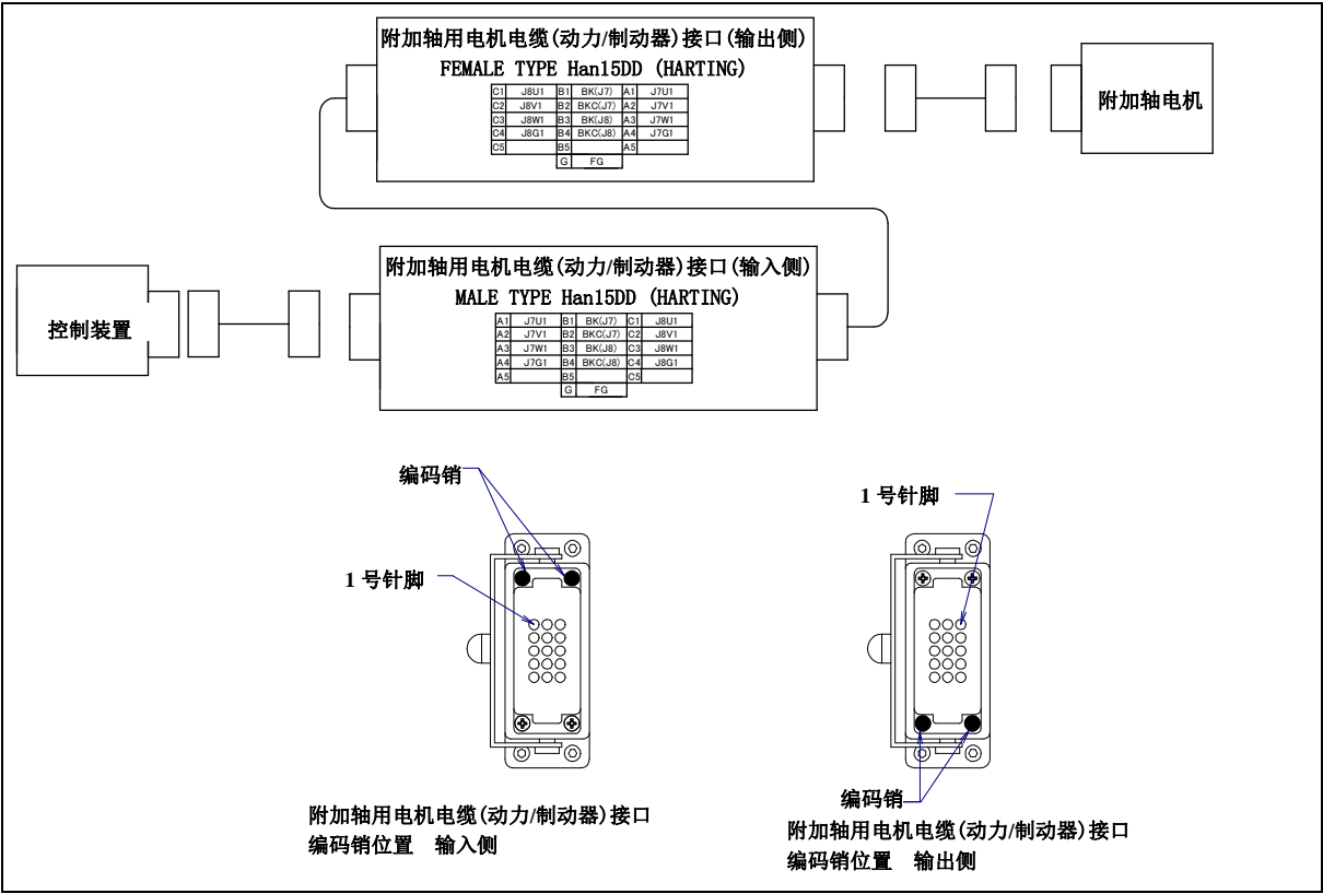
图 5.3 (q) 附加轴（2 轴）用电机电缆（动力线和制动器线）(ARM)接口的插针排列和编码销配置位置（可选项项）
