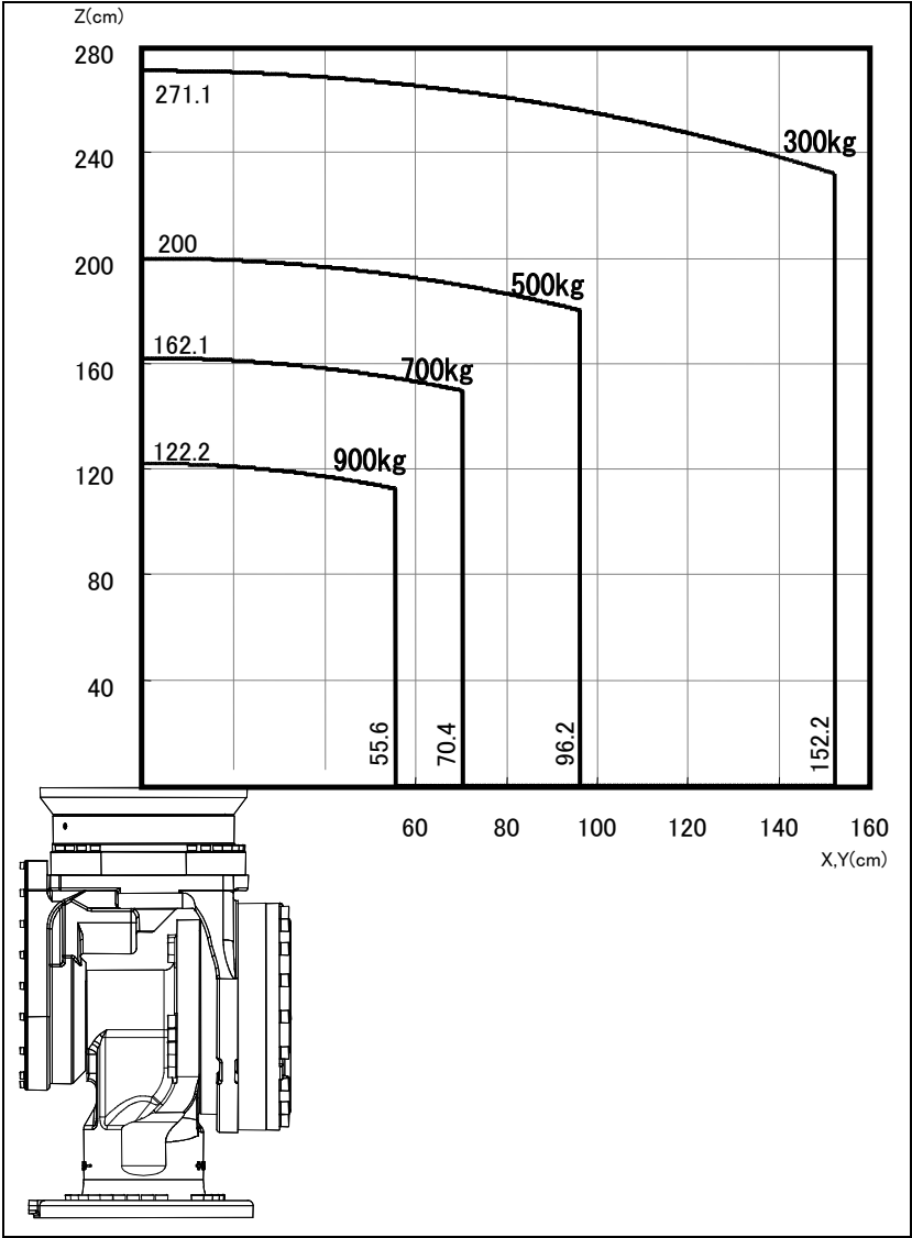
图 3.4 (b) 手腕部允许负载线图 (M-2000iA/900L)
