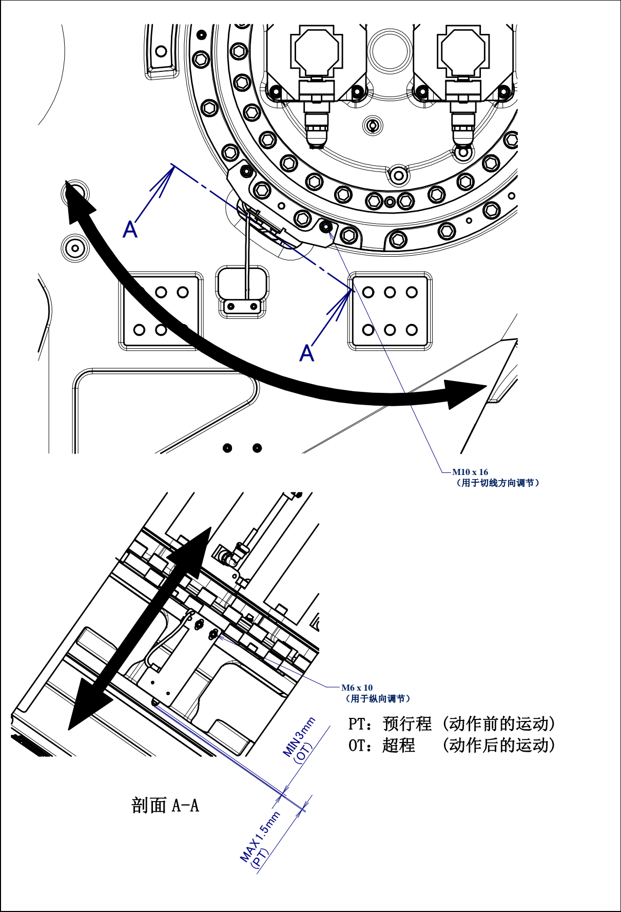
图 6.4 (c) J2 轴限位开关的调节(可选项) (M-2000iA/1200/ 900L)
