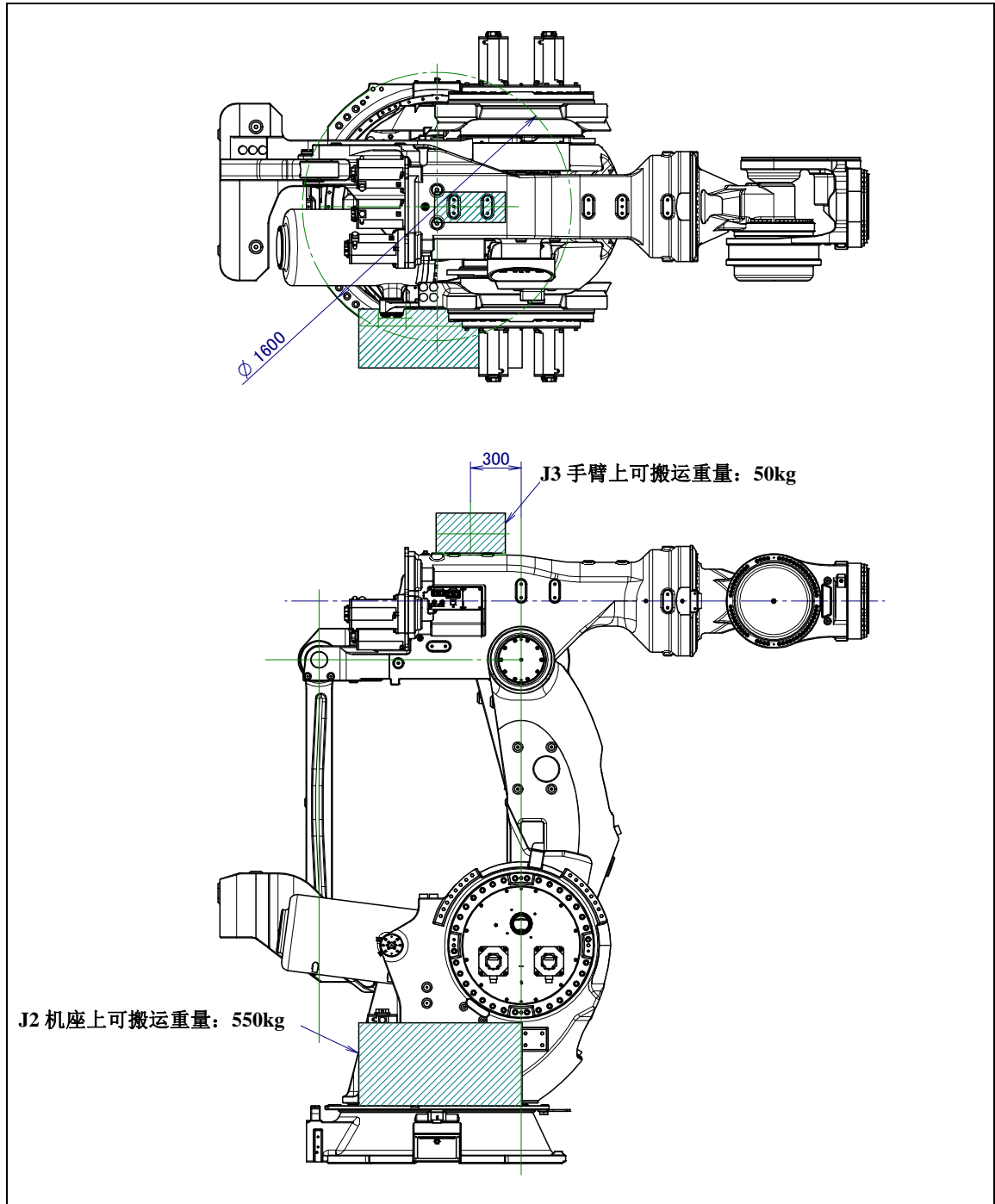
图 3.5 (c) J2 机座上/J3 手臂部的负载条件(M-2000iA/2300/1700L)
