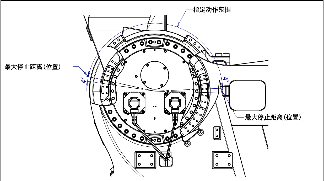
图 6.2.3 (f) J3 轴机械式可变制动器的最大停止距离(位置) (M-2000iA/2300)
