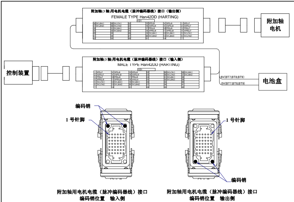
图 5.3 (p) 附加轴(3 轴)用电机电缆（脉冲编码器线）(ARP)接口的插针排列和编码销配置位置(可选项项)
