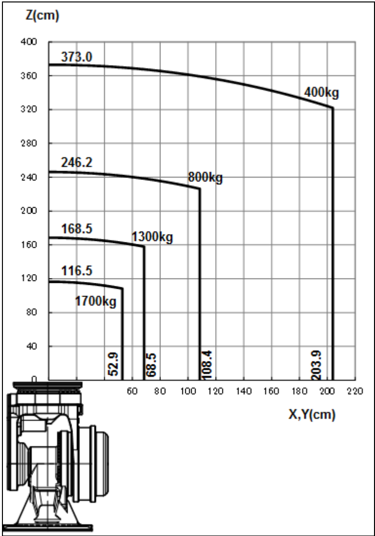
图 3.4 (d) 手腕部允许负载线图 (M-2000iA/1700L)
