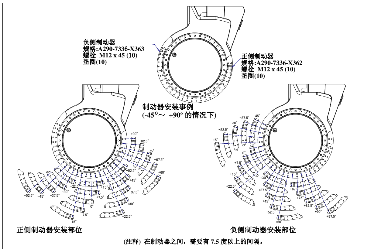
图 6.2.1 (d) J1 轴机械式制动器的安装(可选项) (M-2000iA/2300/1700L)
