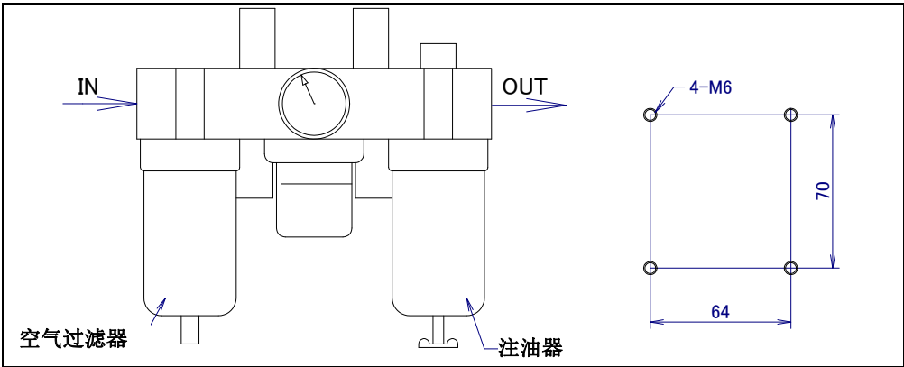
图 5.2 (b) 空气 3 点套件（可选项项）
