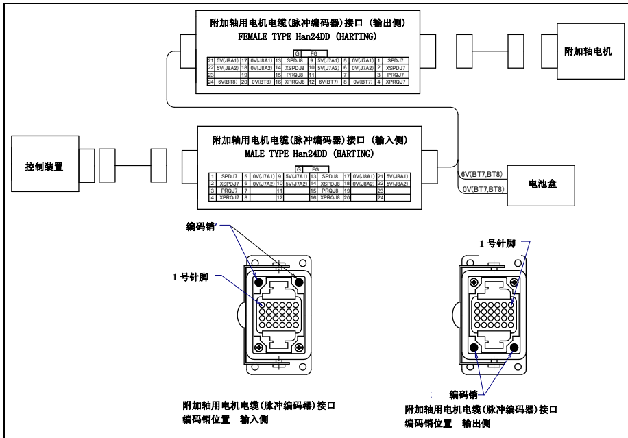
图 5.3 (o) 附加轴（2 轴）用电机电缆（脉冲编码器线）(ARP)接口的插针排列和编码销配置位置(可选项项)
