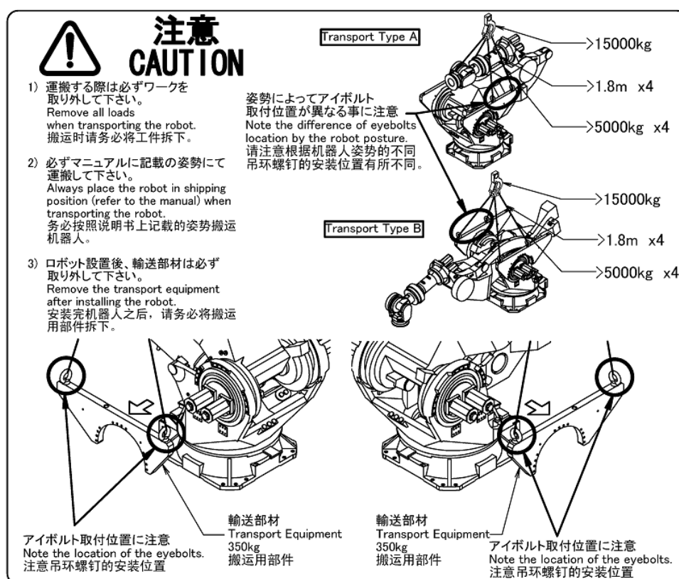
图 4 (k) 搬运注意标签(M-2000iA/1200/900L)
