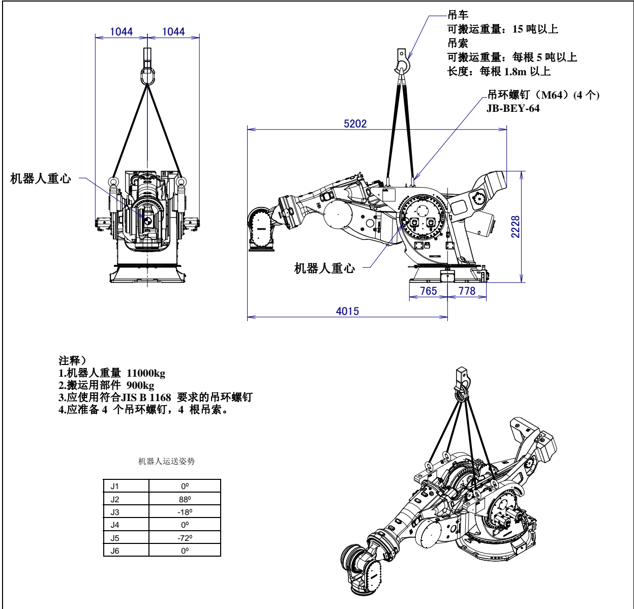
图 1.1 (h) 采用吊车搬运 (M-2000iA/2300 用集装箱的搬运时)
