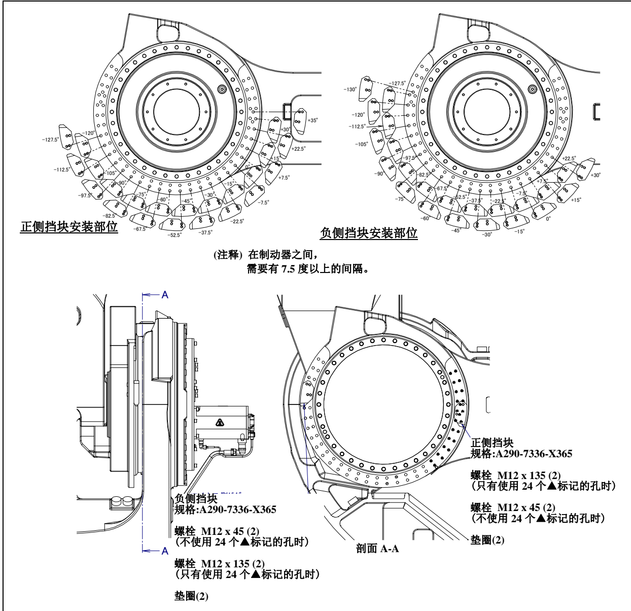
图 6.3 (f) J3 轴的挡块位置和动作范围(可选项) (M-2000iA/2300/1700L)
