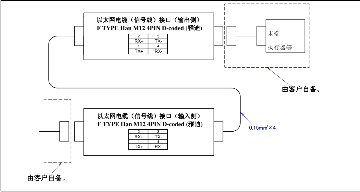
图 5.3 (s) 以太网电缆（信号线）(ES)接口的插针排列（可选项项）
