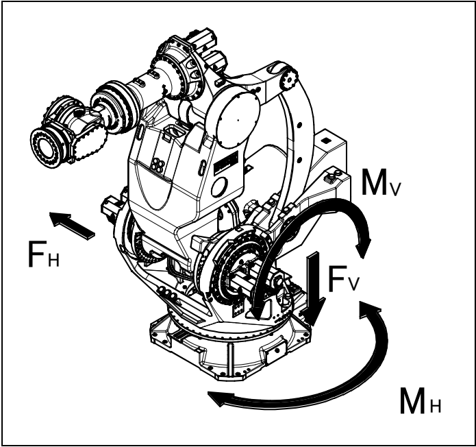
图 1.2 (c) 断电停止时作用的力以及力矩
