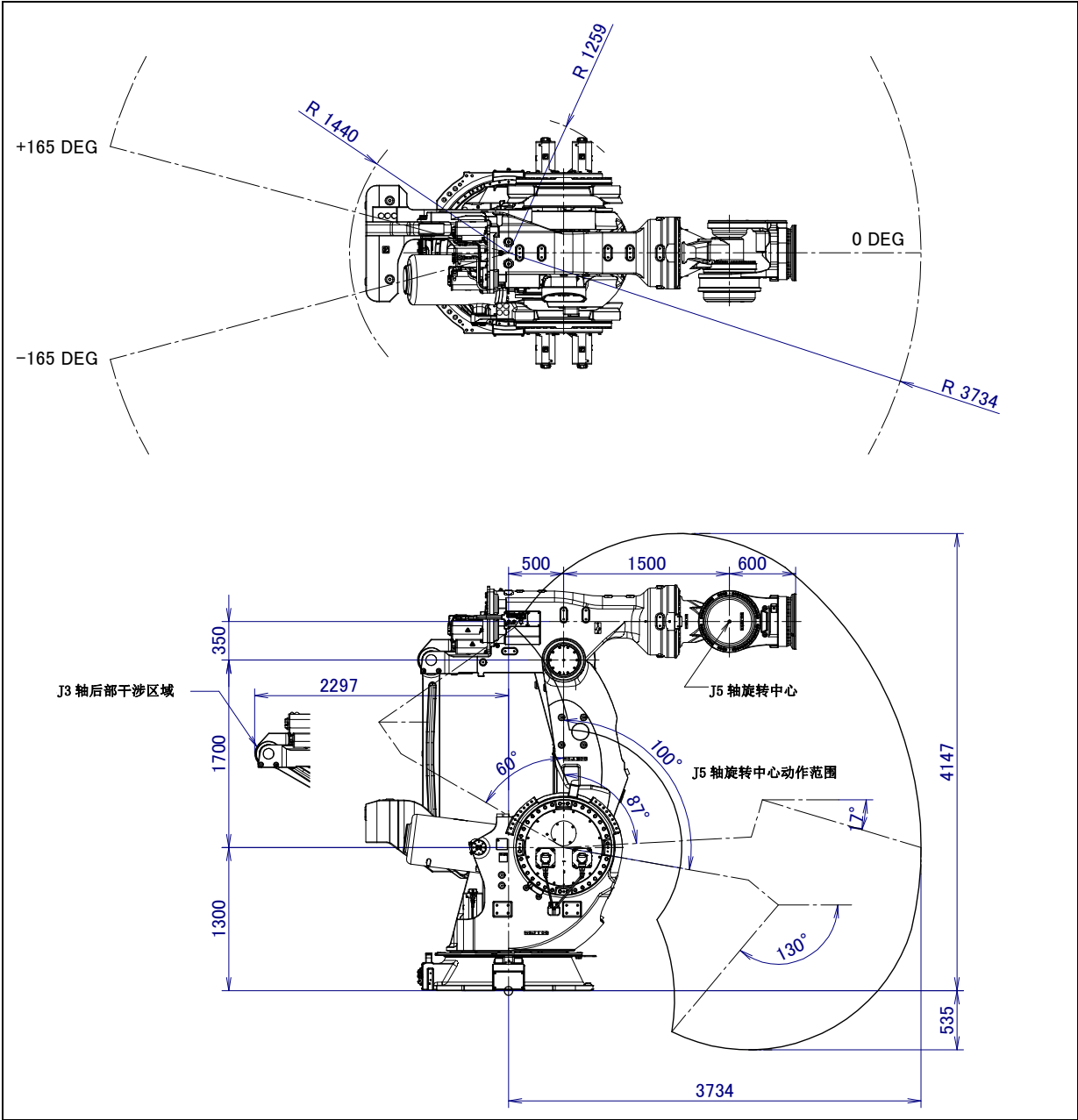
图 3.2 (c) 动作范围图 (M-2000iA/2300)
