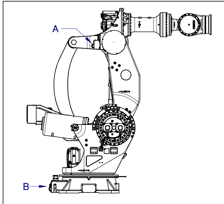
图 5.3 (a) 可选项电缆用接口的位置(可选项) (M-2000iA/1200/900L)
