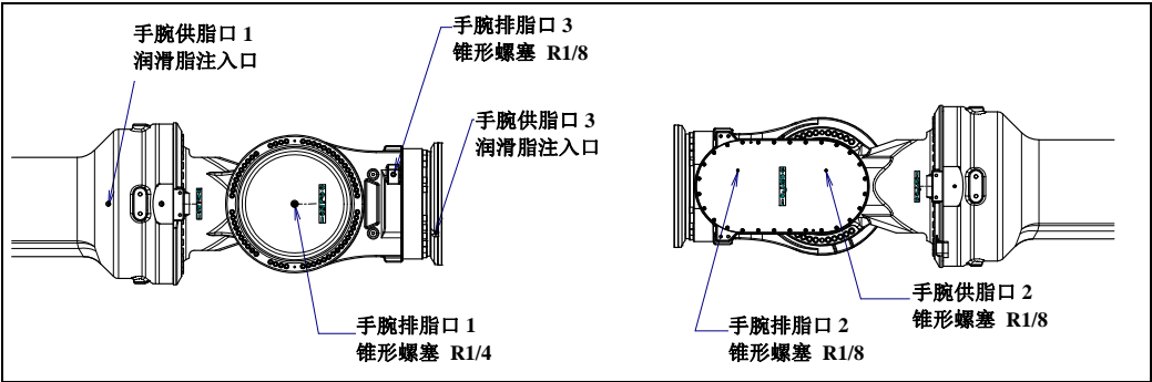
图 7.3.3 (h) 手腕的润滑脂的更换(M-2000iA/2300/1700L)
