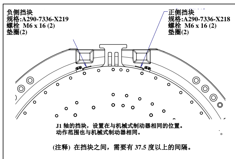
图 6.3 (b) J1 轴的挡块位置(可选项) (M-2000iA/2300/1700L)
