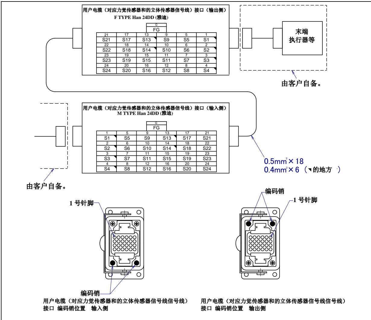
图 5.3 (m) 用户电缆 (对应应力觉传感器和的立体传感器信号线)(ASi) 接口的插针排列和编码销的配置位置 (可选项项)
