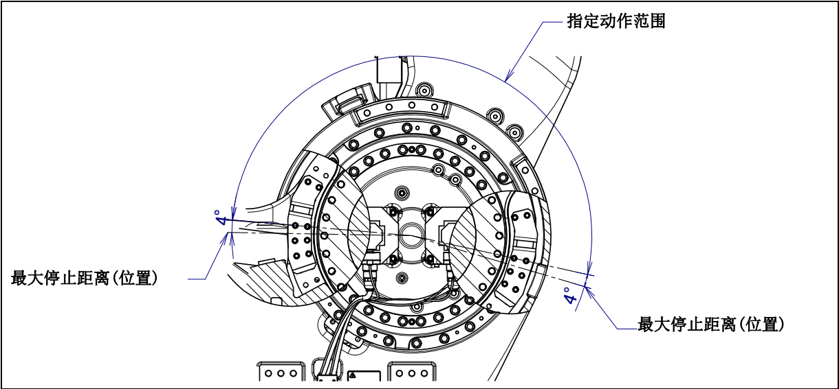
图 6.2.3 (b) J2 轴机械式可变制动器的最大停止距离(位置) (M-2000iA/1200/900L)
