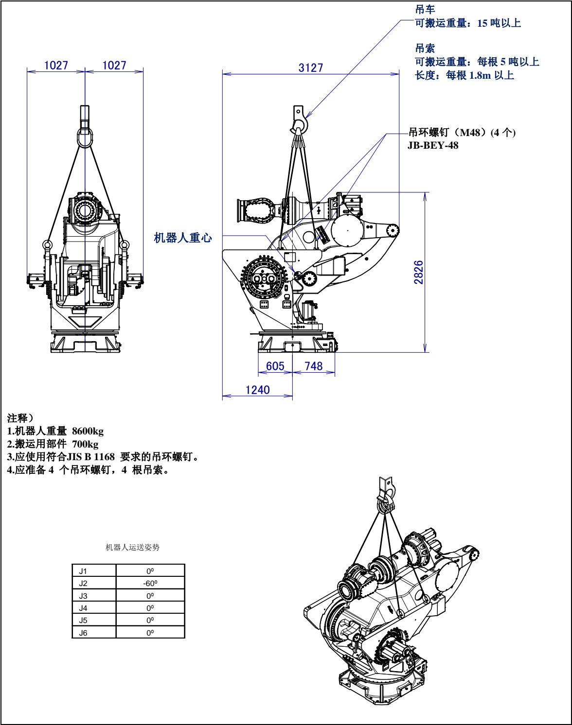
图 1.1 (c) 采用吊车搬运 (M-2000iA/1200 通常搬运时)
