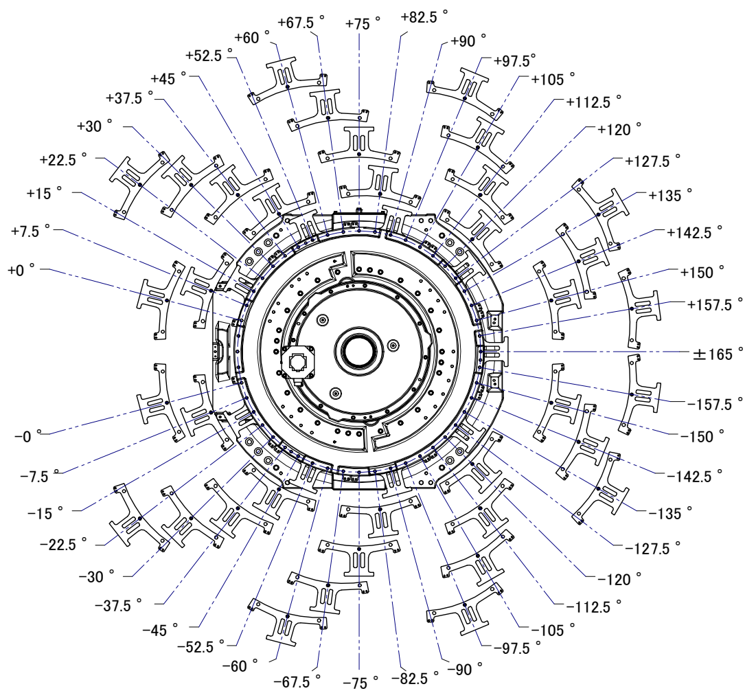
图 6.2.1 (b) J1 轴机械式制动器的安装(可选项) (M-2000iA/2300/1700L)
