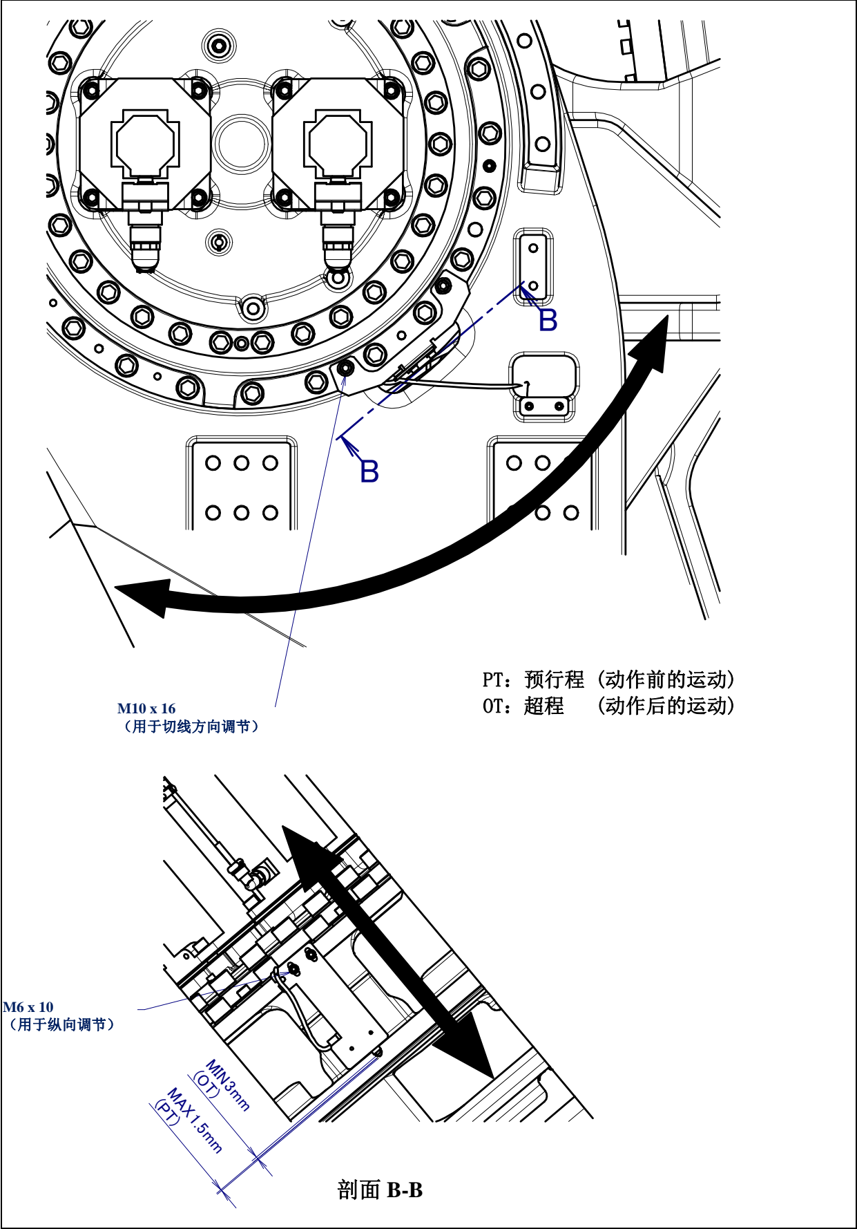
图 6.4 (e) J3 轴限位开关的调节(可选项) (M-2000iA/1200/900L)
