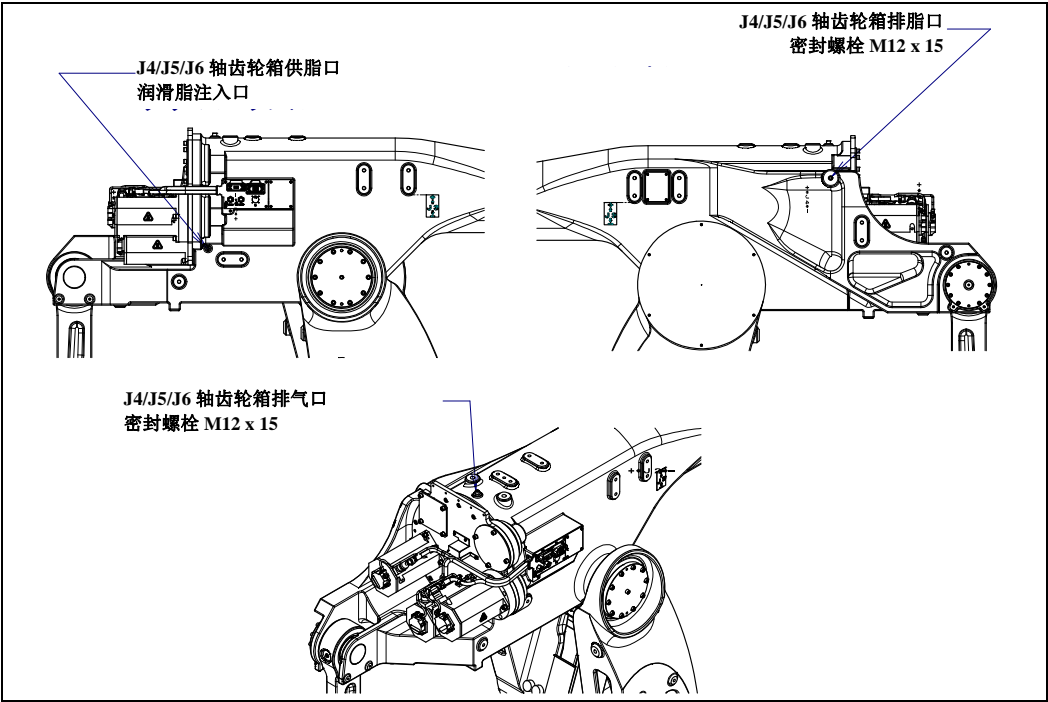
图 7.3.3 (f) J4/J5/J6 轴齿轮箱的润滑脂的更换(M-2000iA/2300/1700L)
