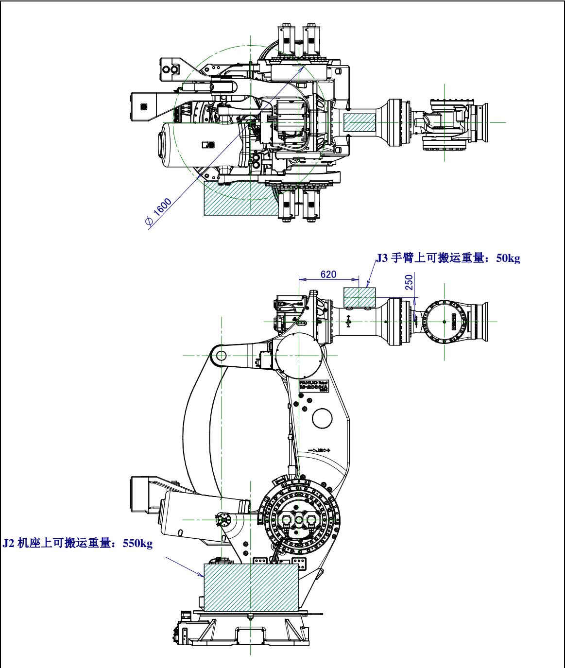
图 3.5 (a) J2 机座上/J3 手臂部的负载条件(M-2000iA/1200)
