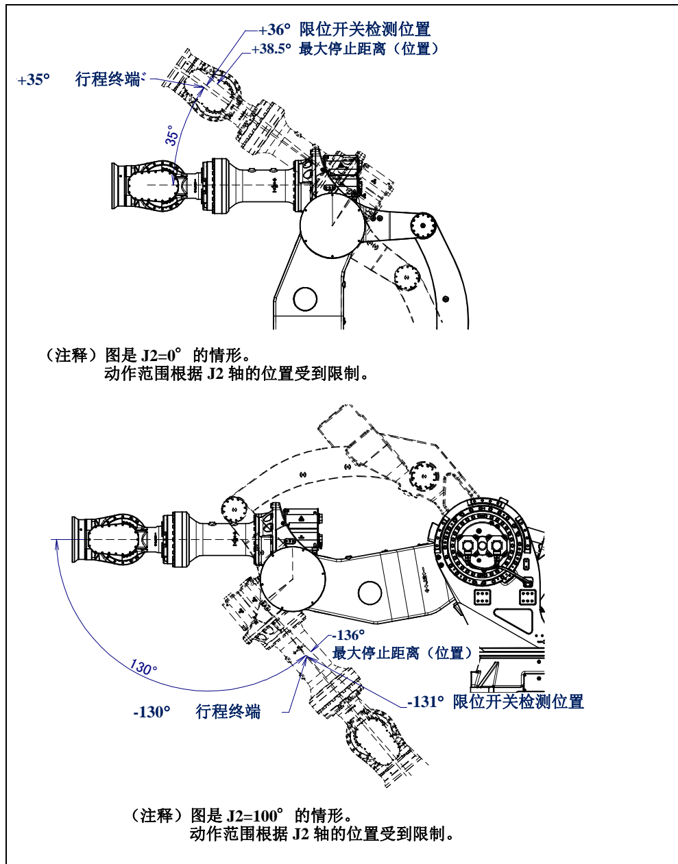
图 3.3 (f) J3 轴可动范围
