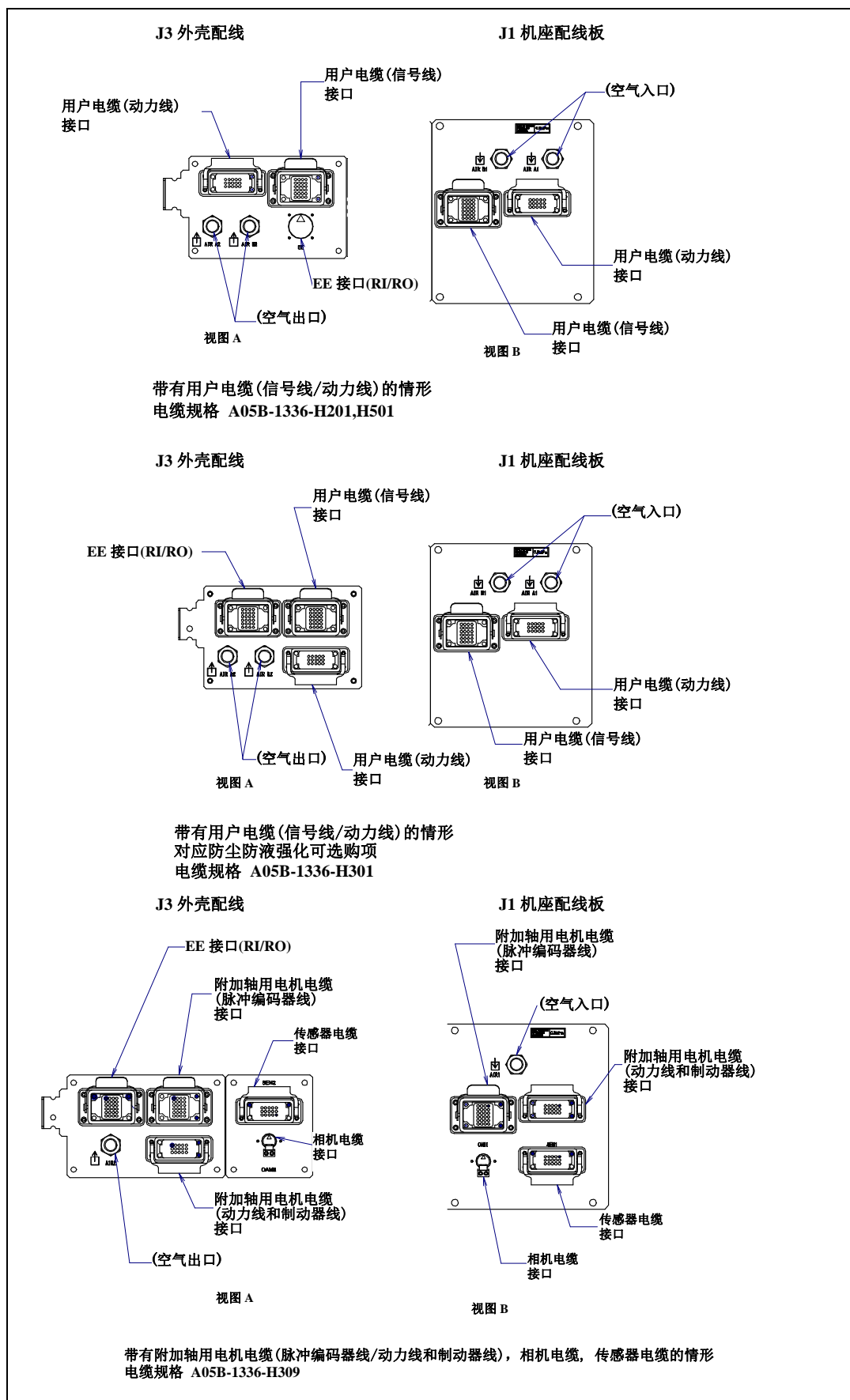
图 5.3 (h) 可选项电缆用接口 (1/2) (M-2000iA/2300/1700L)
