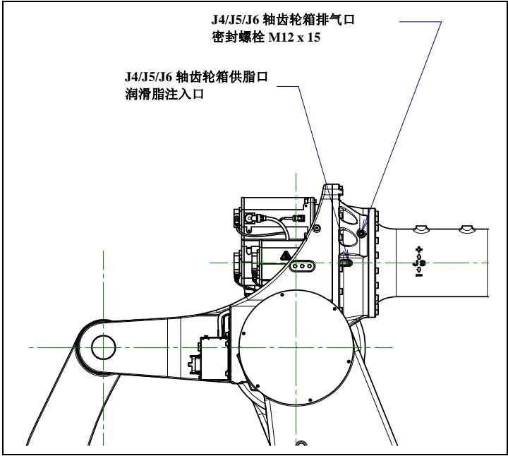
图 7.3.3 (e) J4/J5/J6 轴齿轮箱的润滑脂的更换(M-2000iA/1200/900L)
