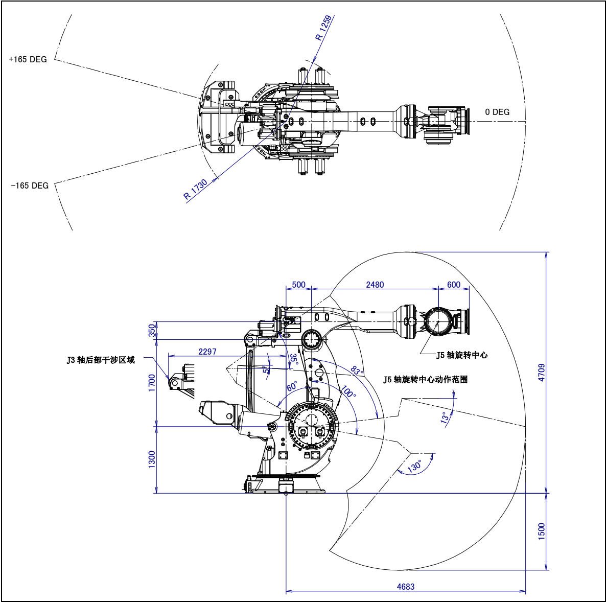
图 3.2 (d) 动作范围图 (M-2000iA/1700L)
