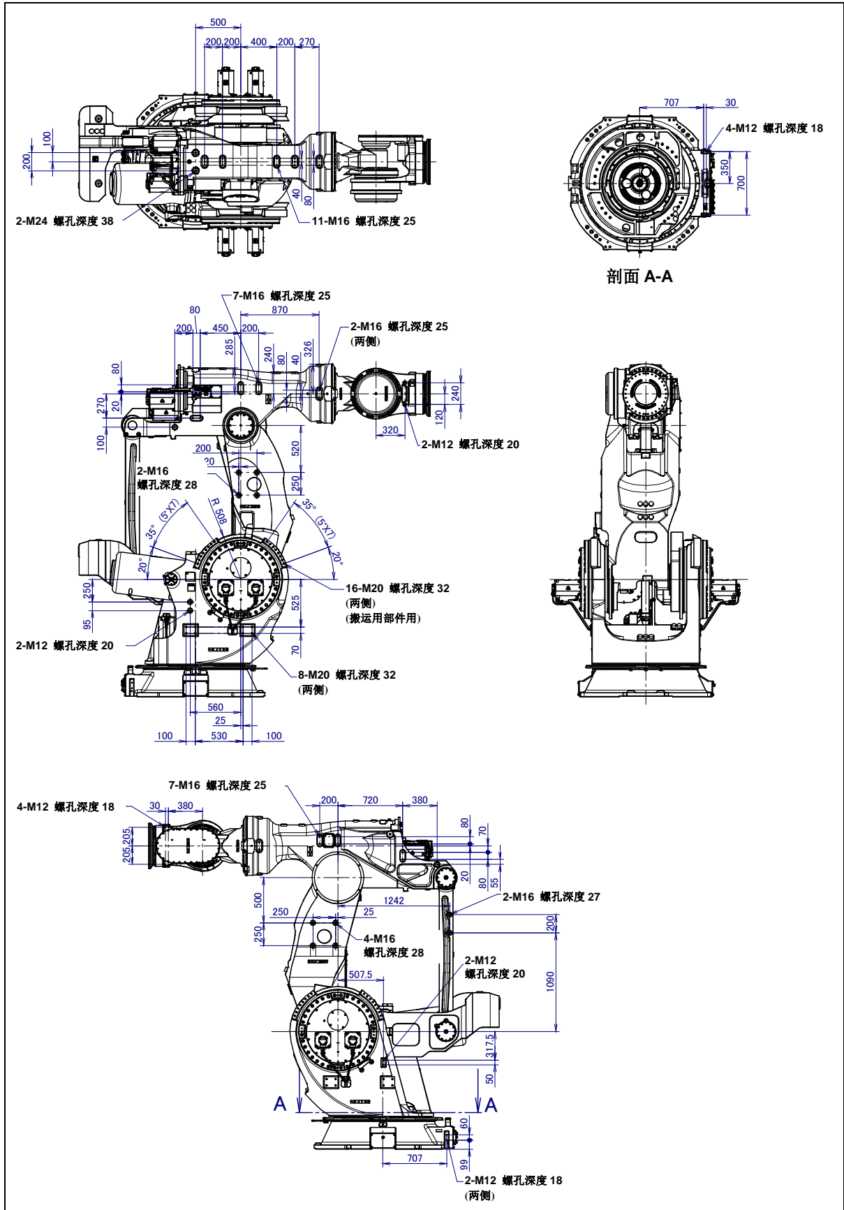
图 4.2 (c) 设备安装面尺寸 (M-2000iA/2300)
