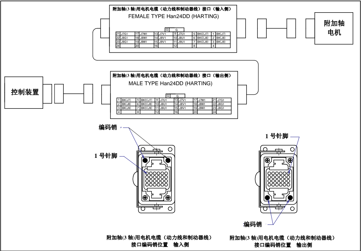
图 5.3 (r) 附加轴（3 轴）用电机电缆（动力线和制动器线）(ARM)接口的插针排列和编码销配置位置（可选项项）
