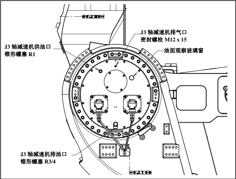
图 7.3.5 (b) J3 轴减速机的润滑油的更换 (M-2000iA/2300/1700L)
