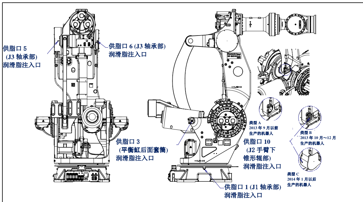
图 7.3.1 (a) 向平衡缸后面套筒和其他的连接部供脂 (M-2000iA/1200/900L)
