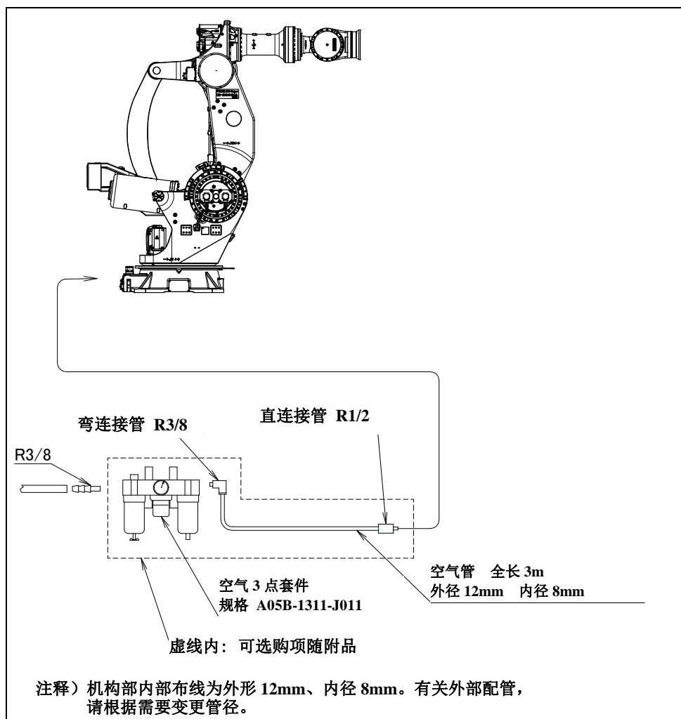
图 5.2 (a) 空气配管（可选项项）
