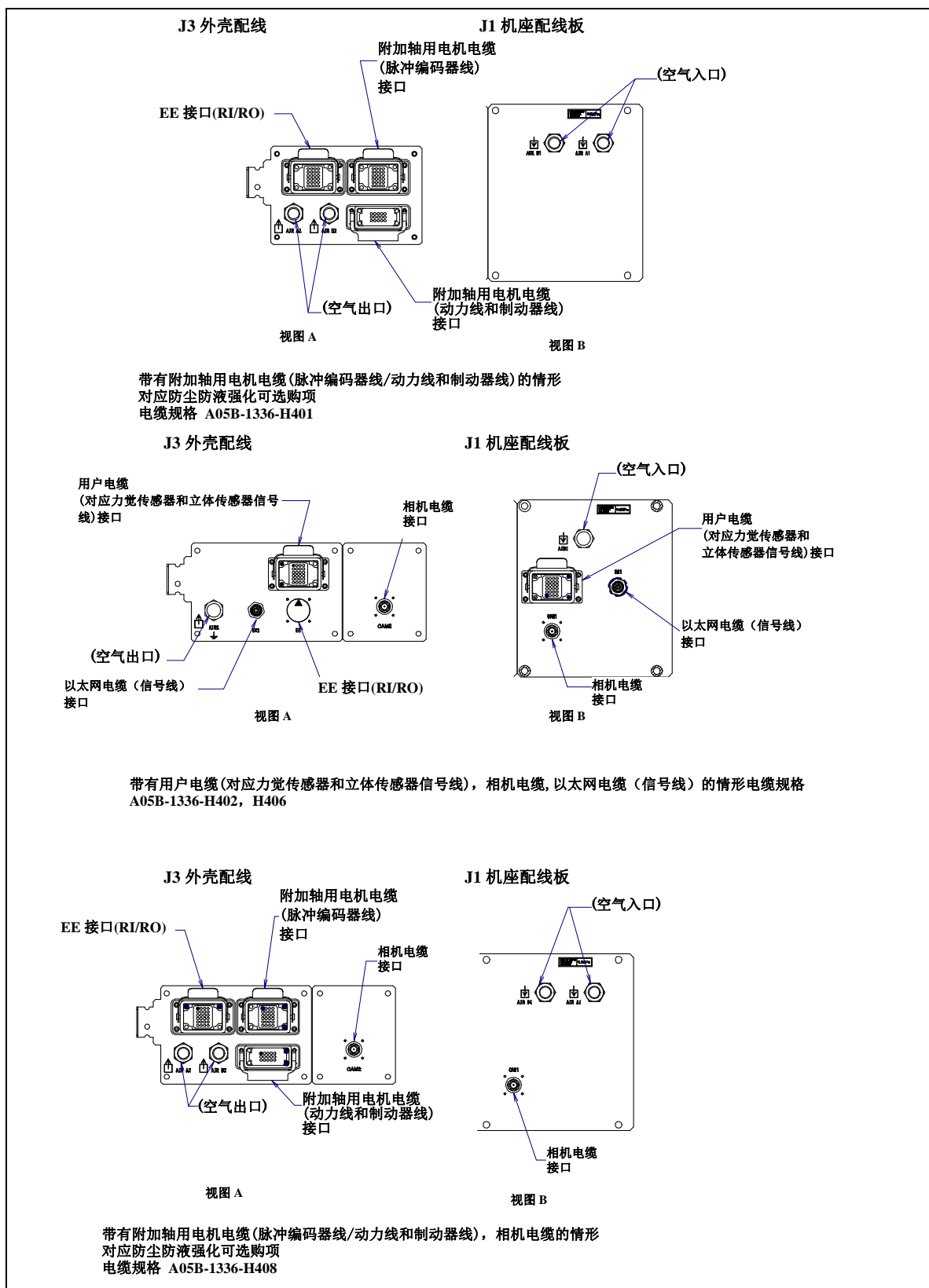
图 5.3 (i) 可选项电缆用接口 (2/2) (M-2000iA/2300/1700L)
