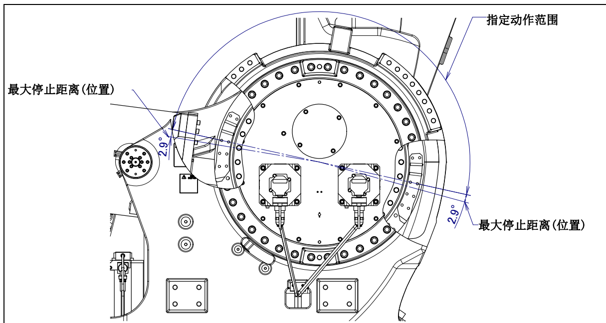
图 6.2.3 (h) J2 轴机械式可变制动器的最大停止距离(位置) (M-2000iA/1700L)
