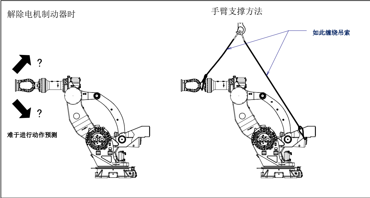
图 3 (b) 解除 J3 轴的电机制动器造成的手臂动作和事先采取的措施例
