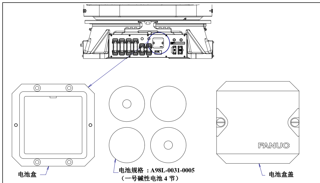
图 7.3.2 (a) 电池的更换
