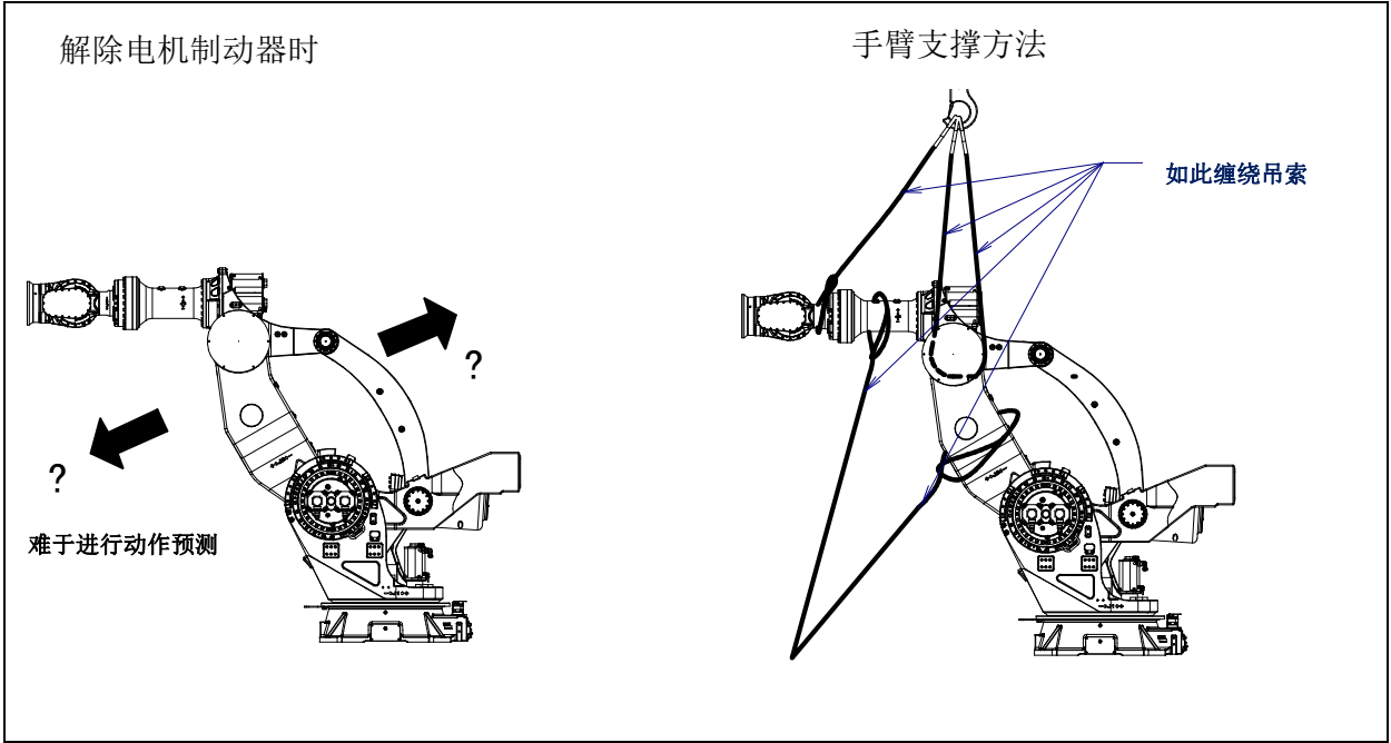
图 3 (a) 解除 J2 轴的电机制动器造成的手臂动作和事先采取的措施例
