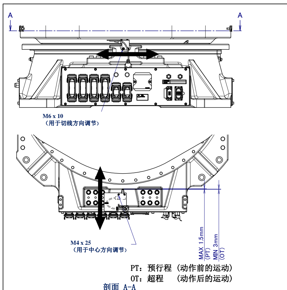
图 6.4 (a) J1 轴限位开关的调节(可选项) (M-2000iA/1200/900L)
