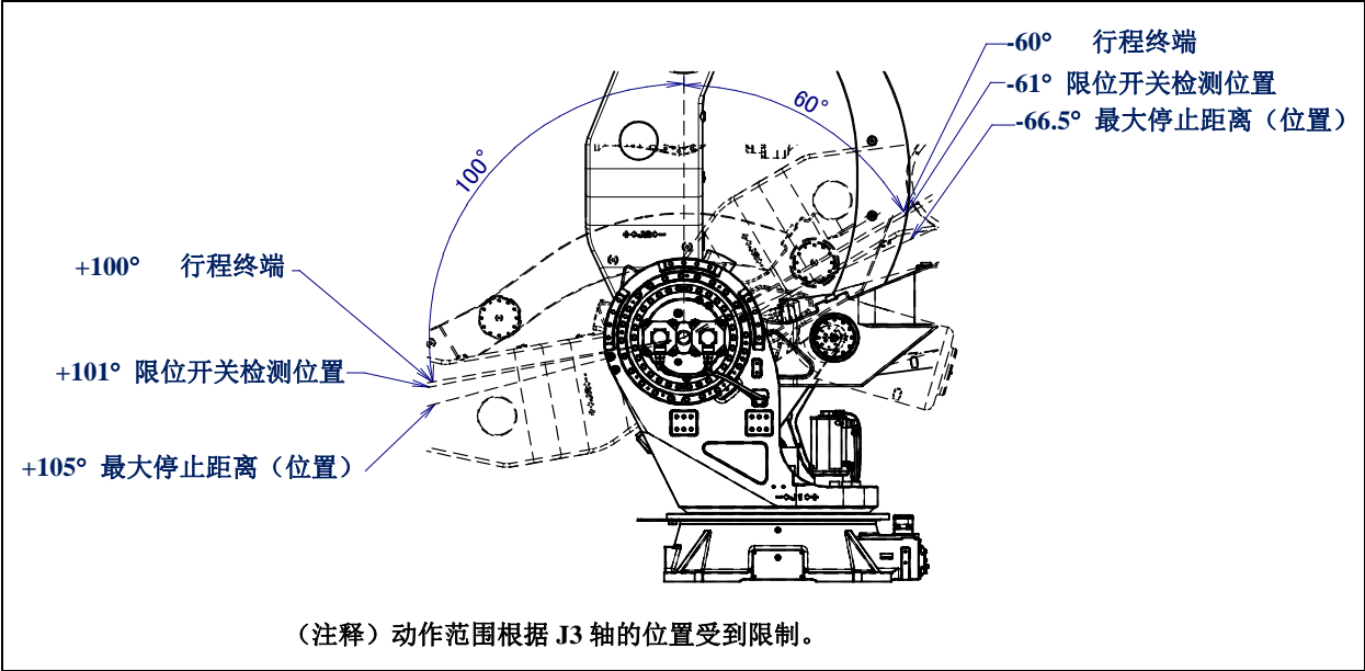
图 3.3 (e) J2 轴可动范围
