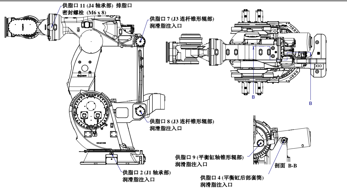
图 7.3.1 (d) 向平衡缸后面套筒和其他的连接部供脂 (M-2000iA/2300/1700L)
