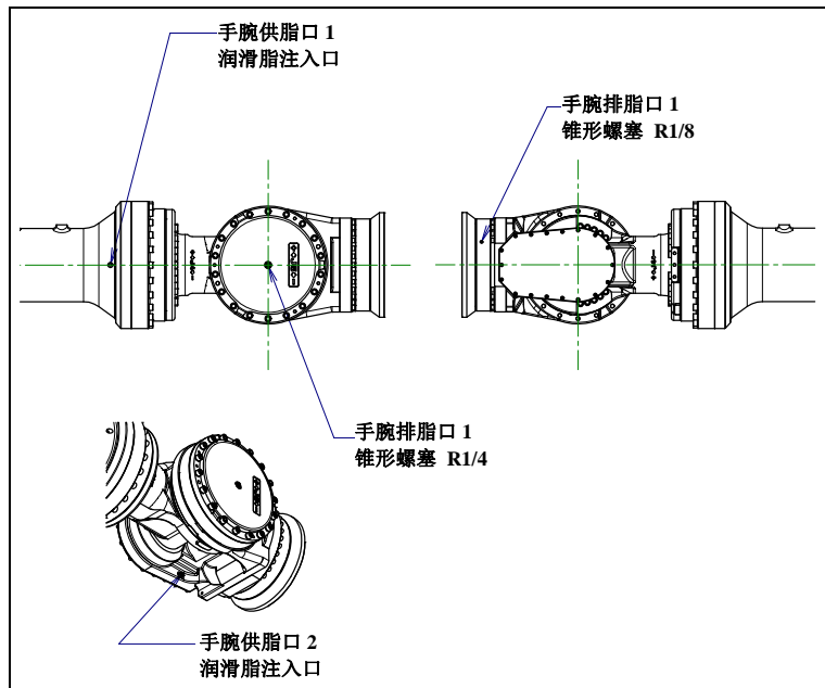
图 7.3.3 (g) 手腕的润滑脂的更换(M-2000iA/1200/900L)
