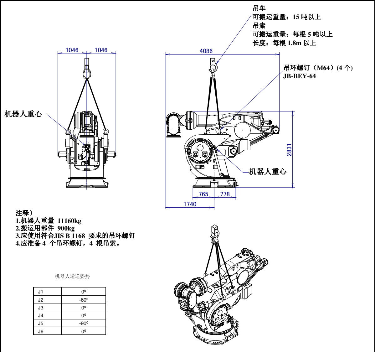
图 1.1 (i) 采用吊车搬运 (M-2000iA/1700L 通常搬运时)
