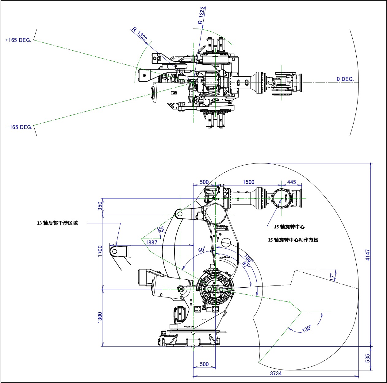
图 3.2 (a) 动作范围图 (M-2000iA/1200)
