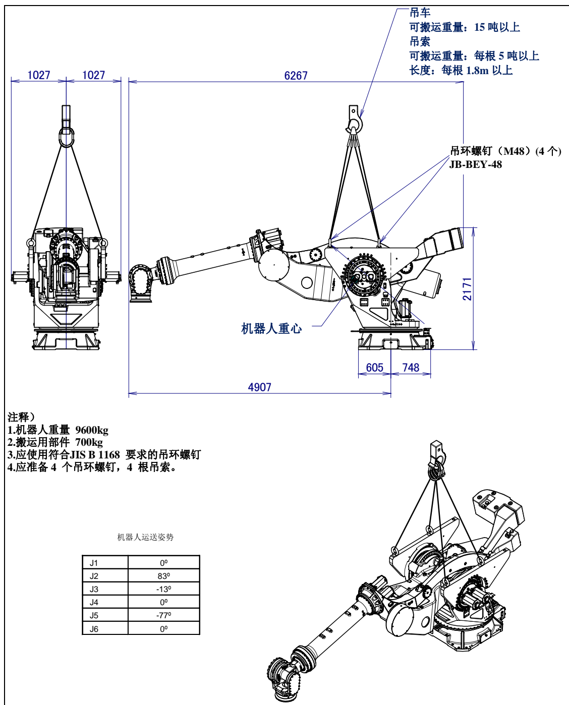
图 1.1 (f) 采用吊车搬运 (M-2000iA/900L 用集装箱的搬运时)
