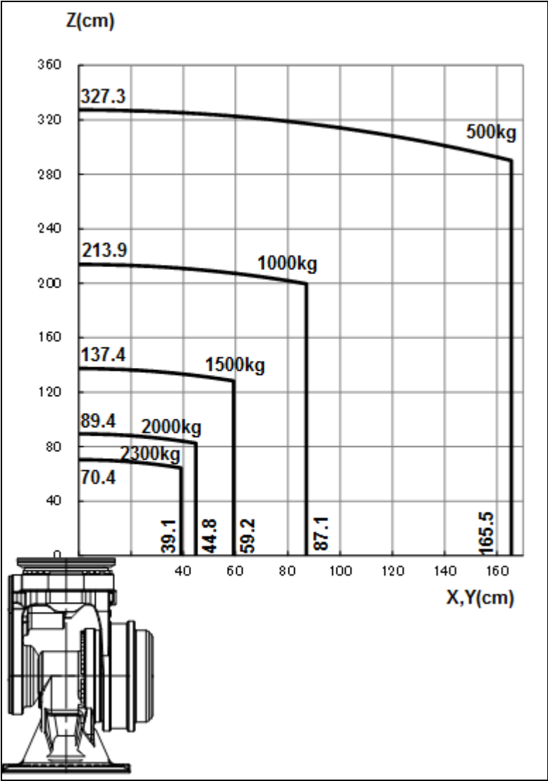
图 3.4 (c) 手腕部允许负载线图 (M-2000iA/2300)
