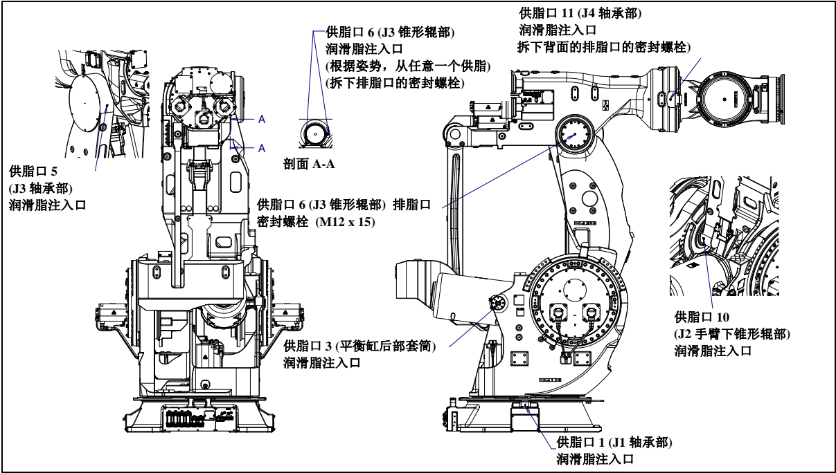
图 7.3.1 (c) 向平衡缸后面套筒和其他的连接部供脂 (M-2000iA/2300/1700L)
