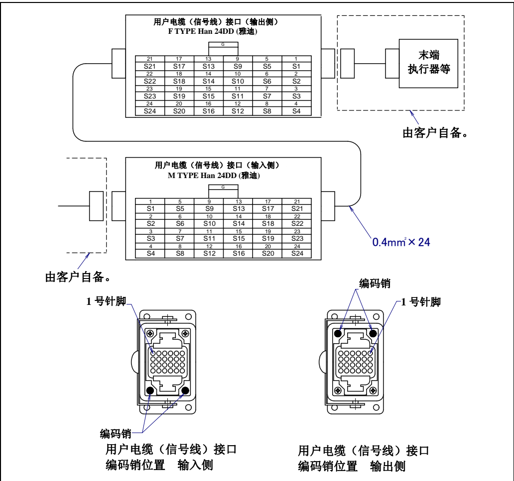
图 5.3 (I) 用户电缆（信号线）(AS)接口的插针排列和编码销的配置位置(可选项项)
