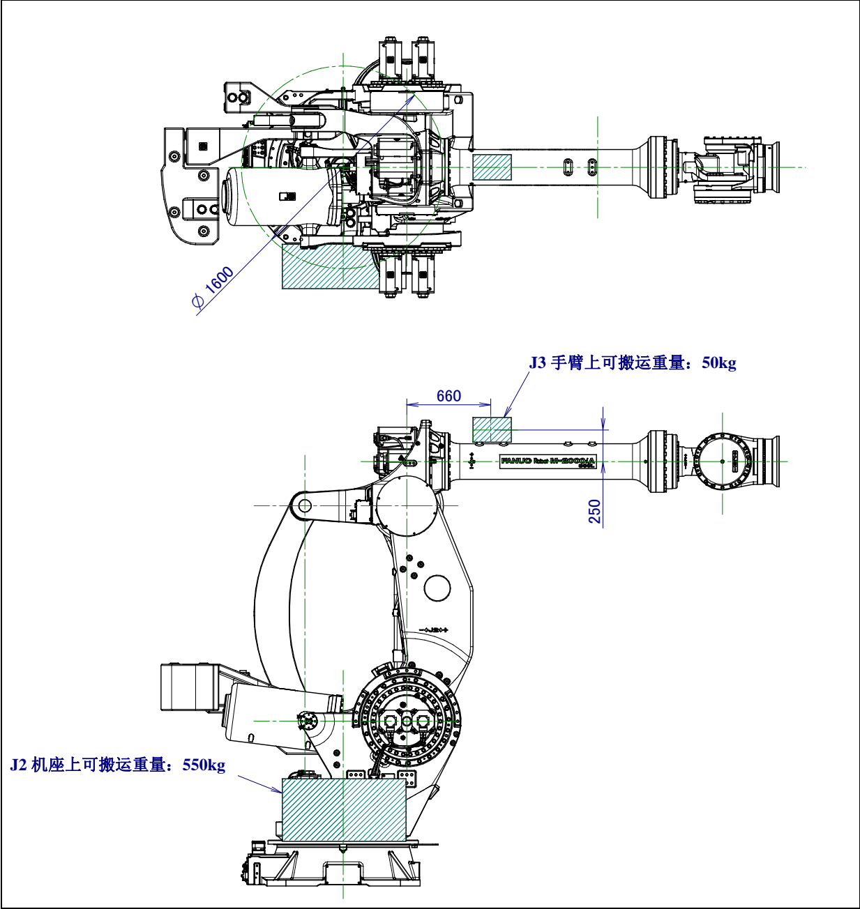
图 3.5 (b) J2 机座上/J3 手臂部的负载条件(M-2000iA/900L)
