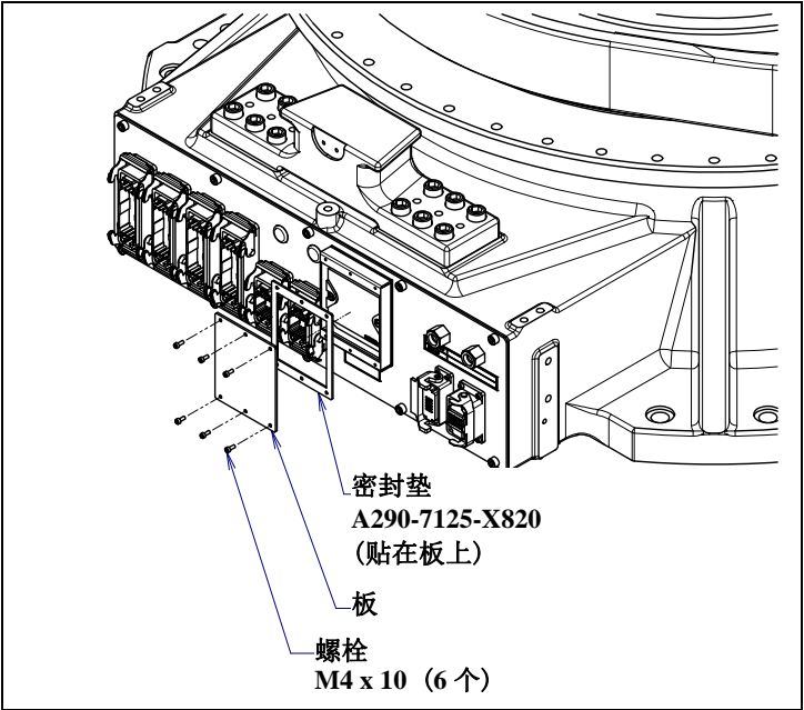
图 7.3.2 (b) 电池盖板的拆除（指定防尘防液强化可选项时）
