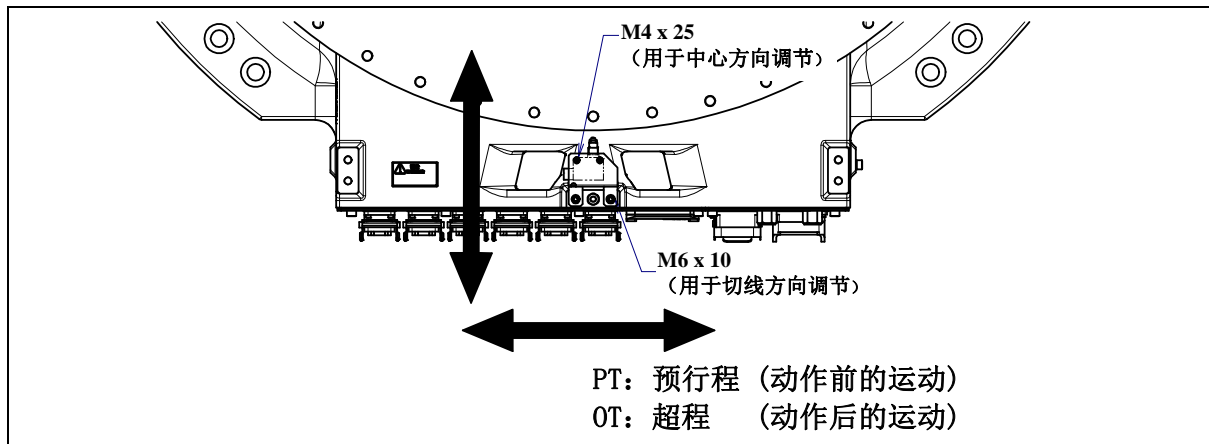
图 6.4 (b) J1 轴限位开关的调节(可选项) (M-2000iA/2300/1700L)
