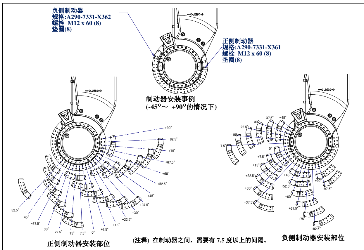
图 6.2.1 (c) J2 轴机械式制动器的安装(可选项) (M-2000iA/1200/900L)
