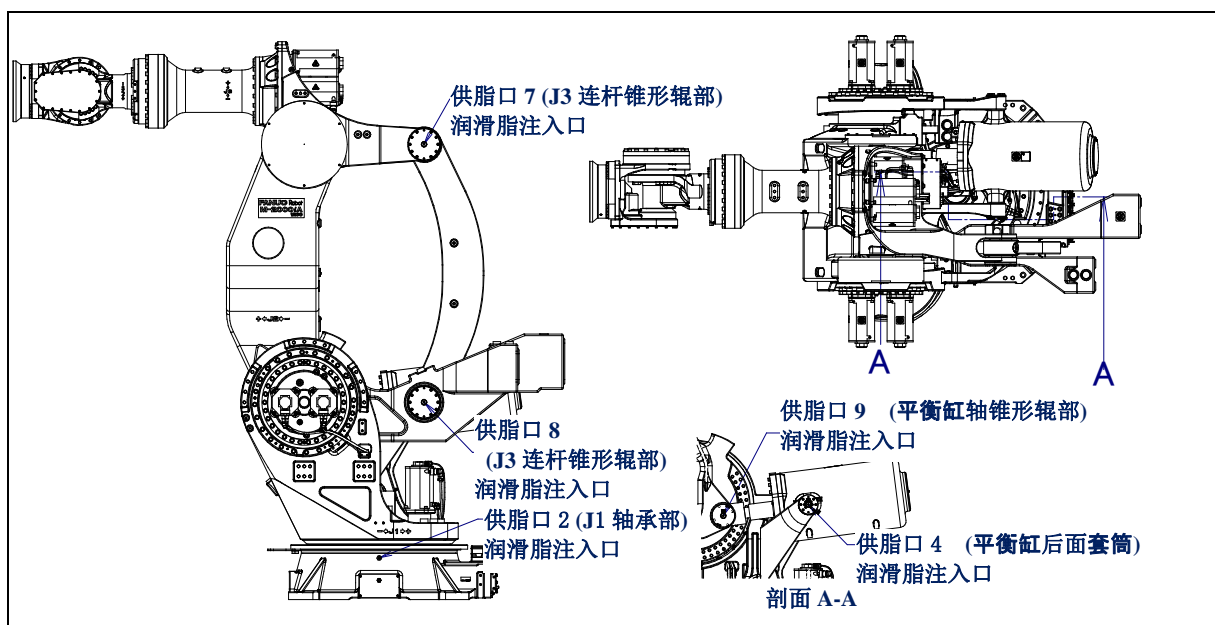
图 7.3.1 (b) 向平衡缸后面套筒和其他的连接部供脂 (M-2000iA/1200/900L)
