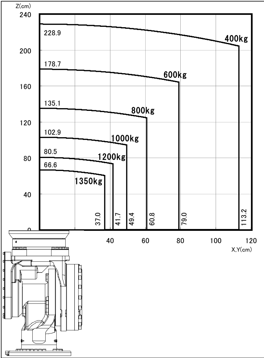
图 3.4 (a) 手腕部允许负载线图 (M-2000iA/1200, M-2000iA/1200 1350kg 可搬运可选项)
