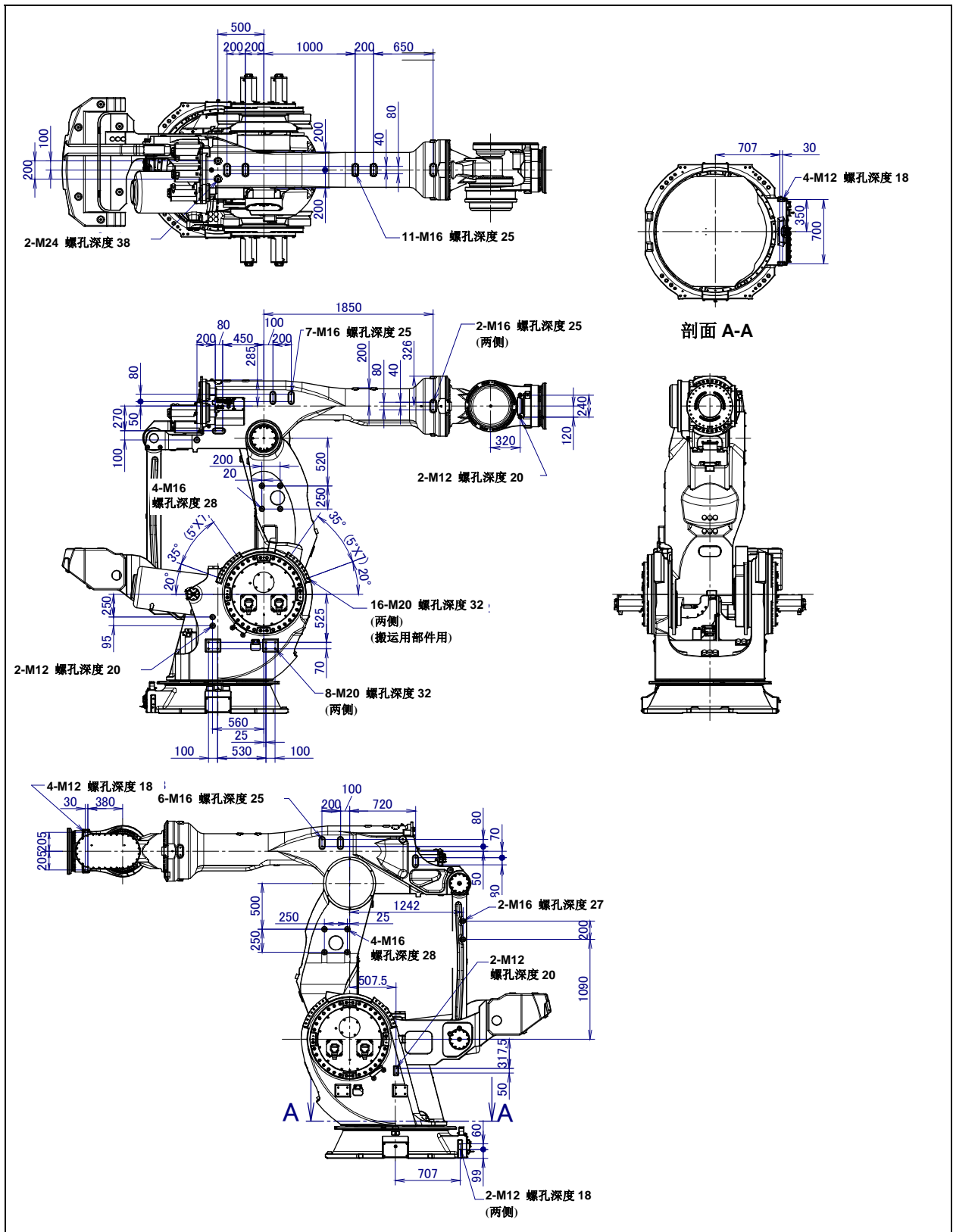
图 4.2 (d) 设备安装面尺寸 (M-2000iA/1700L)
