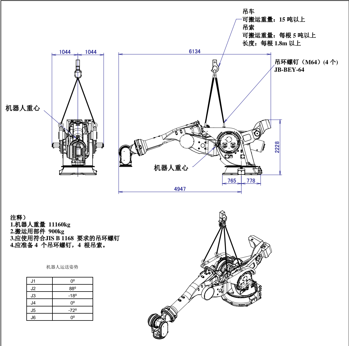
图 1.1 (j) 采用吊车搬运 (M-2000iA/1700L 用集装箱的搬运时)
