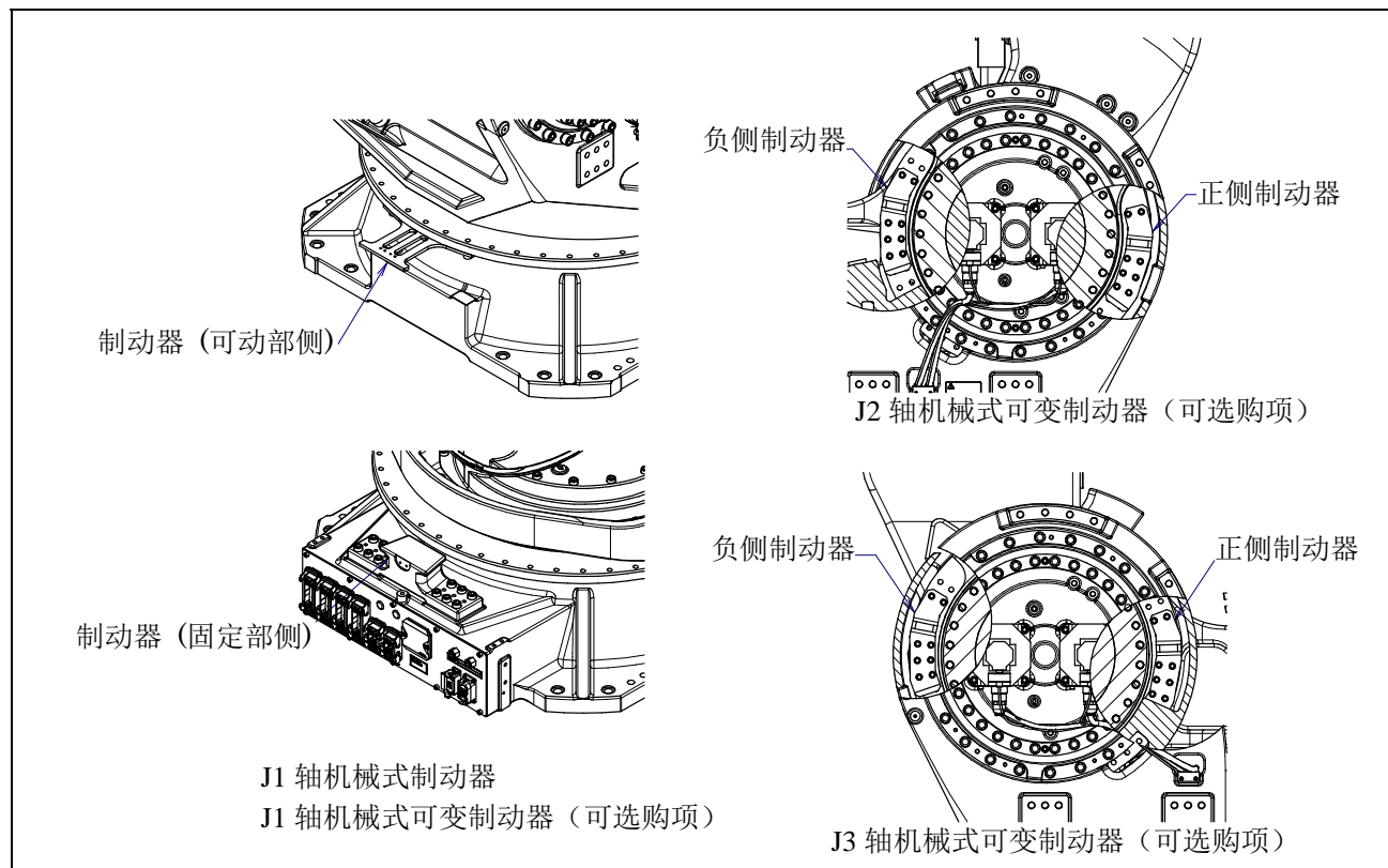
图 7.2.4 机械式固定制动器、机械式可变制动器的检修
