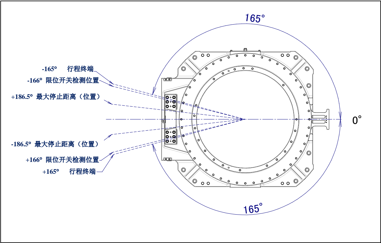
图 3.3 (b) J1 轴可动范围(M-2000iA/1200/900L)
