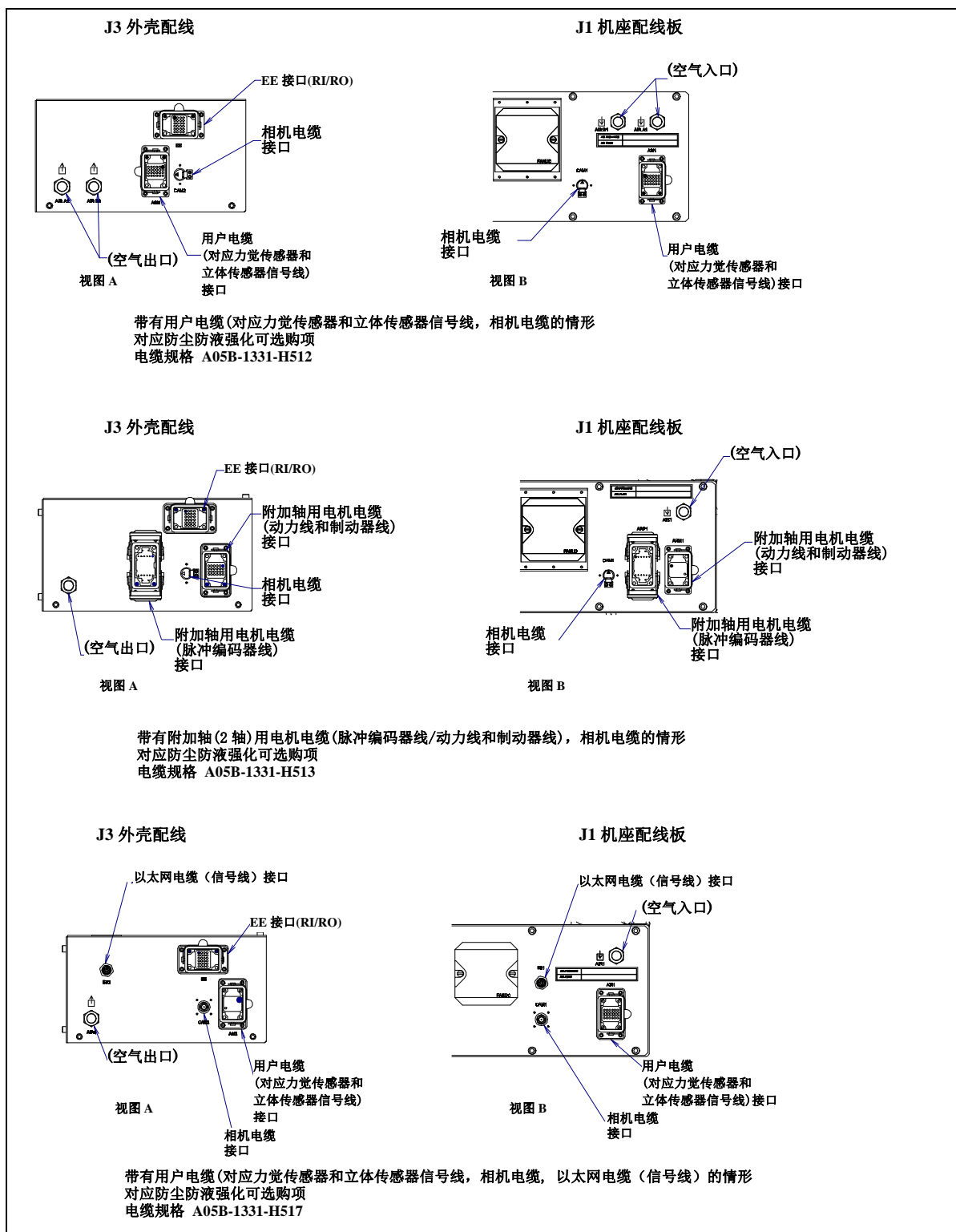
图 5.3 (g) 可选项电缆用接口 (5/5) (M-2000iA/1200/900L)
