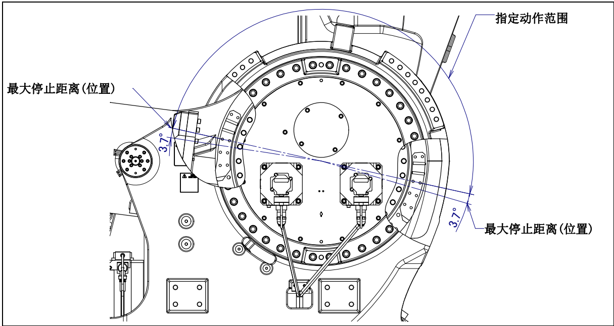
图 6.2.3 (e) J2 轴机械式可变制动器的最大停止距离(位置) (M-2000iA/2300)
