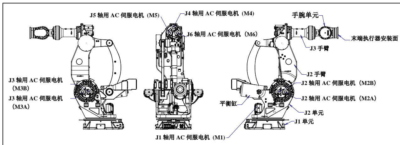
图 3.1 (a) 机构部的构成
