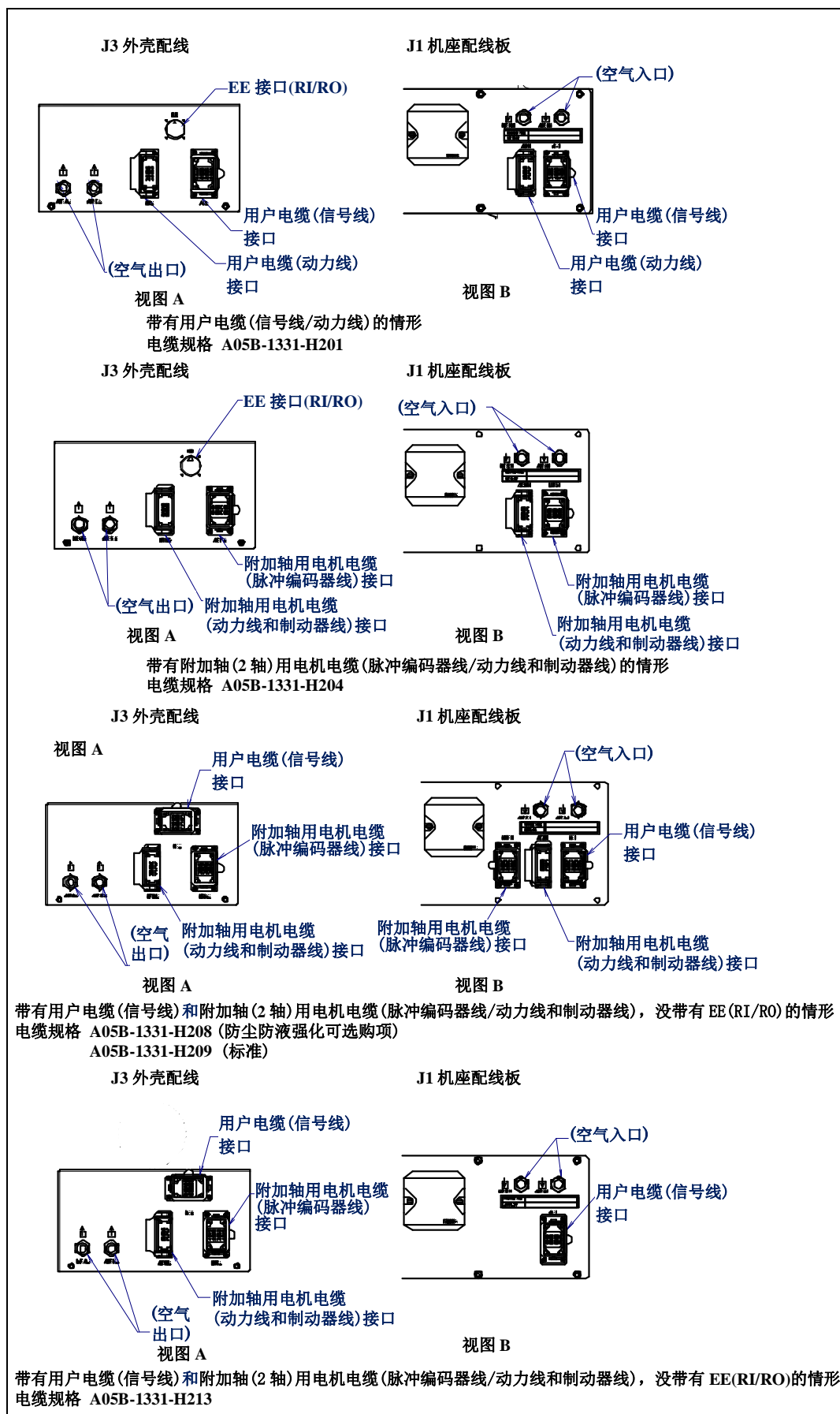
图 5.3 (c) 可选项电缆用接口 (1/5) (M-2000iA/1200/900L)
