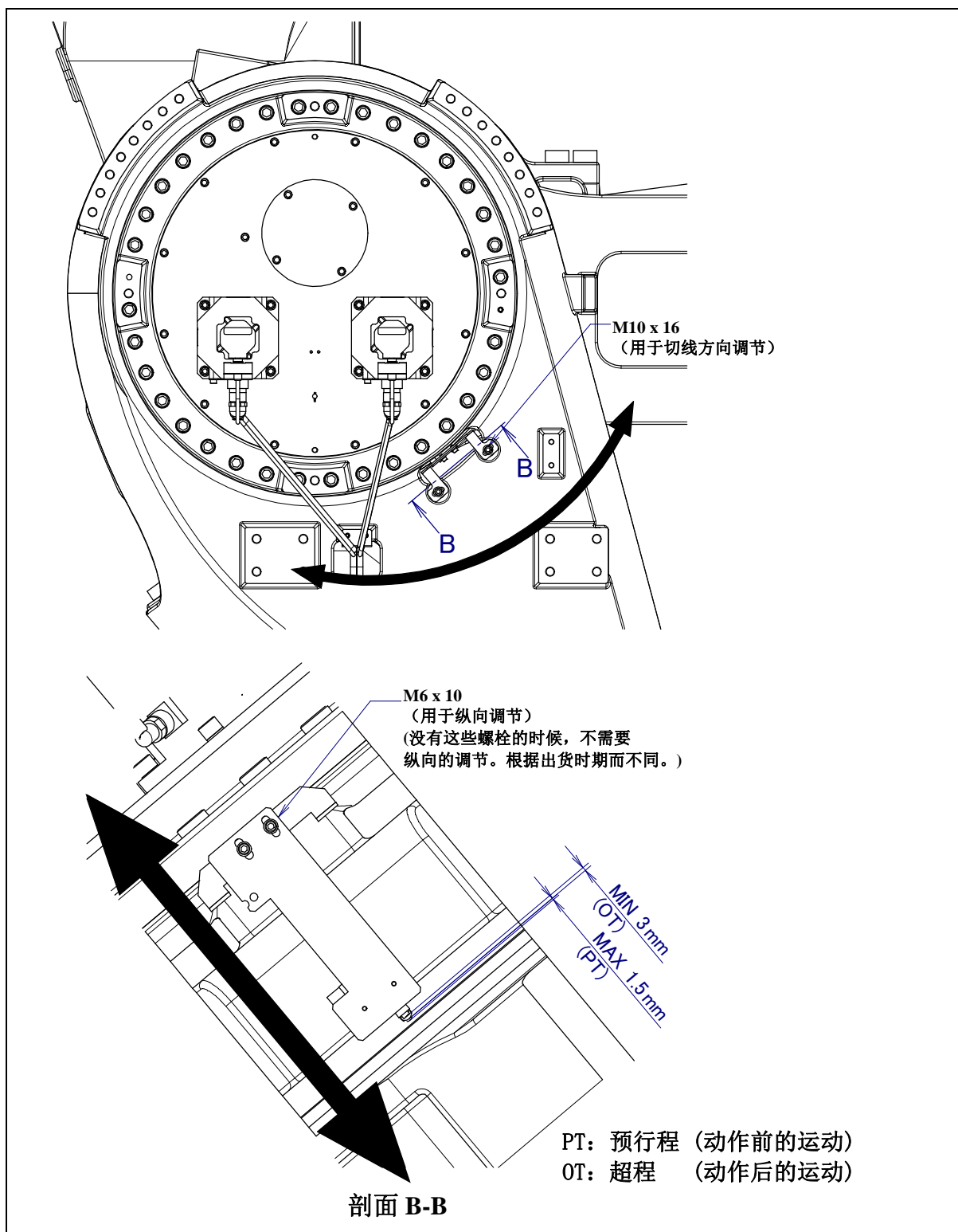
图 6.4 (f) J3 轴限位开关的调节(可选项) (M-2000iA/2300/1700L)
