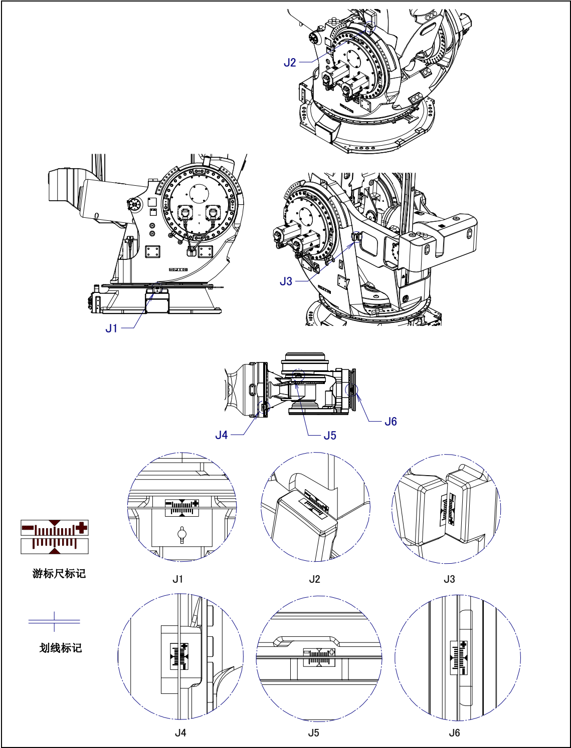
图 8.3 (b) 对合标记位置 (M-2000iA/2300/1700L)
