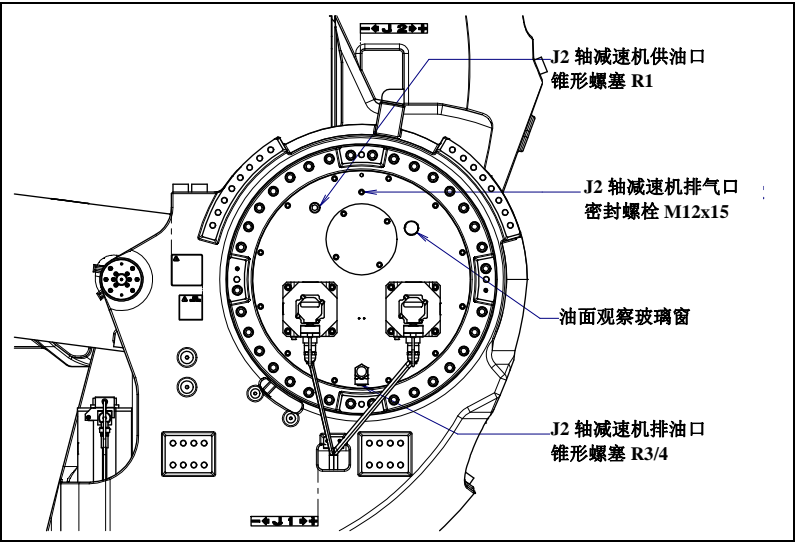
图 7.3.5 (a) J2 轴减速机的润滑油的更换 (M-2000iA/2300/1700L)
