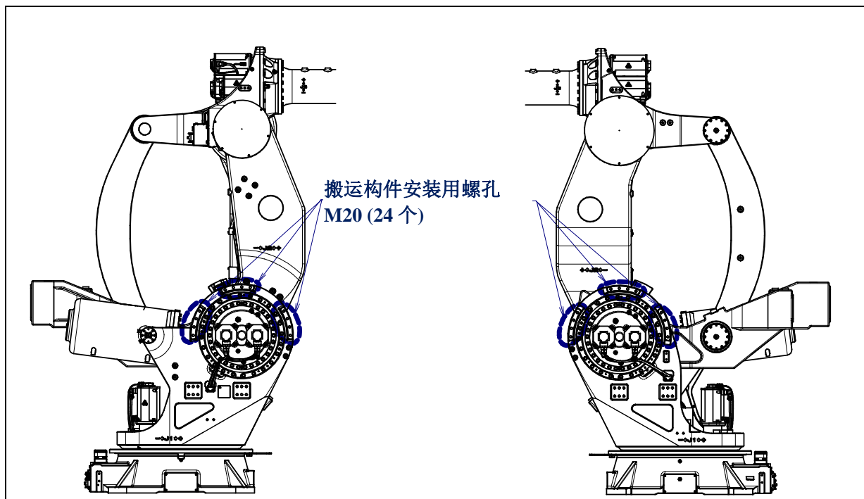
图 1.1 (a) 搬运用部件安装位置 (M-2000iA/1200/900L)
