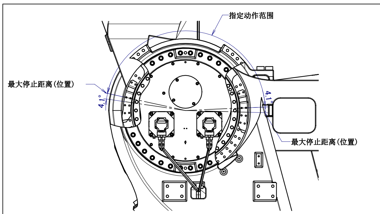
图 6.2.3 (i) J3 轴机械式可变制动器的最大停止距离(位置) (M-2000iA/1700L)
