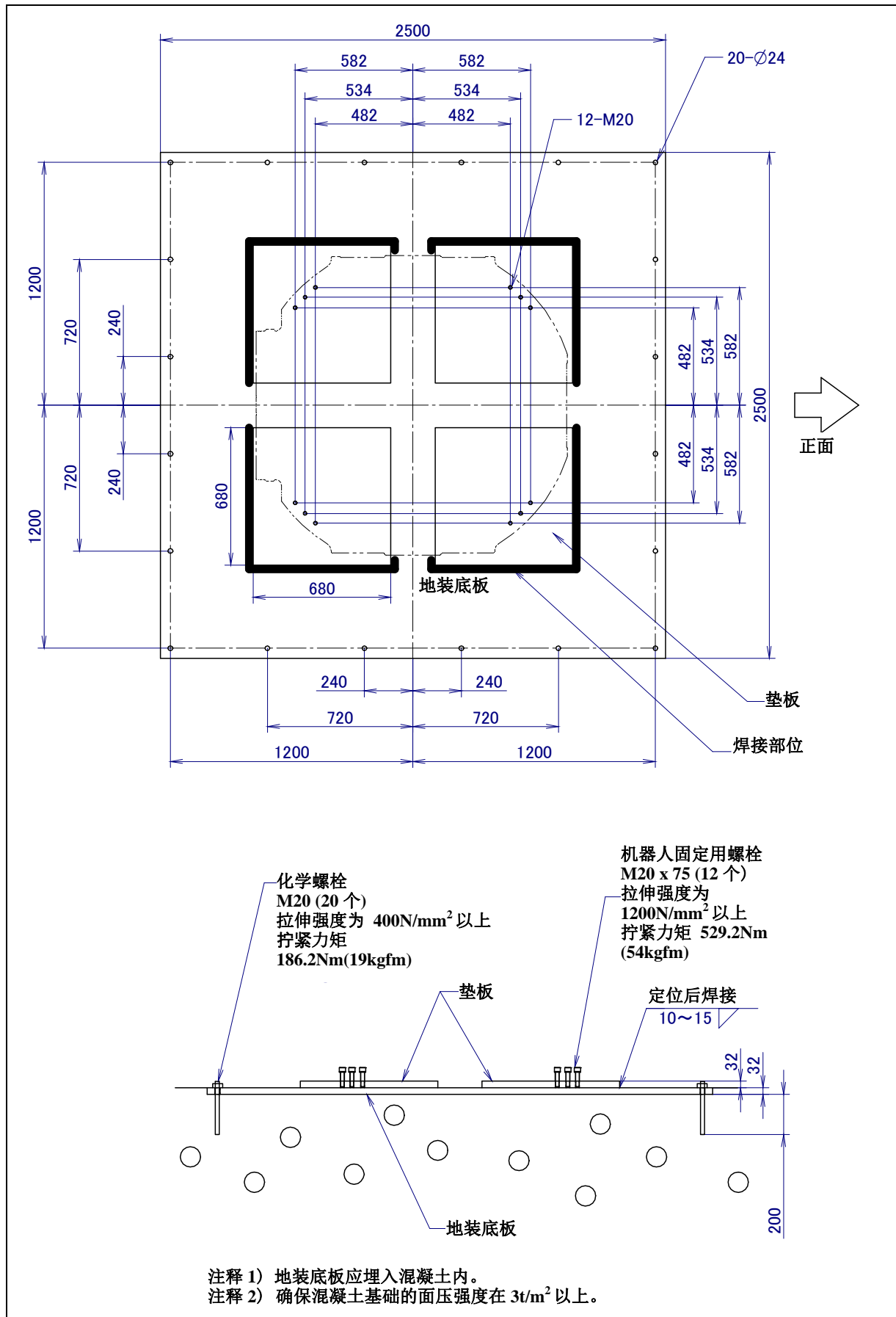
图 1.2.1 (b) 安装方法(M-2000iA/2300/1700L)
