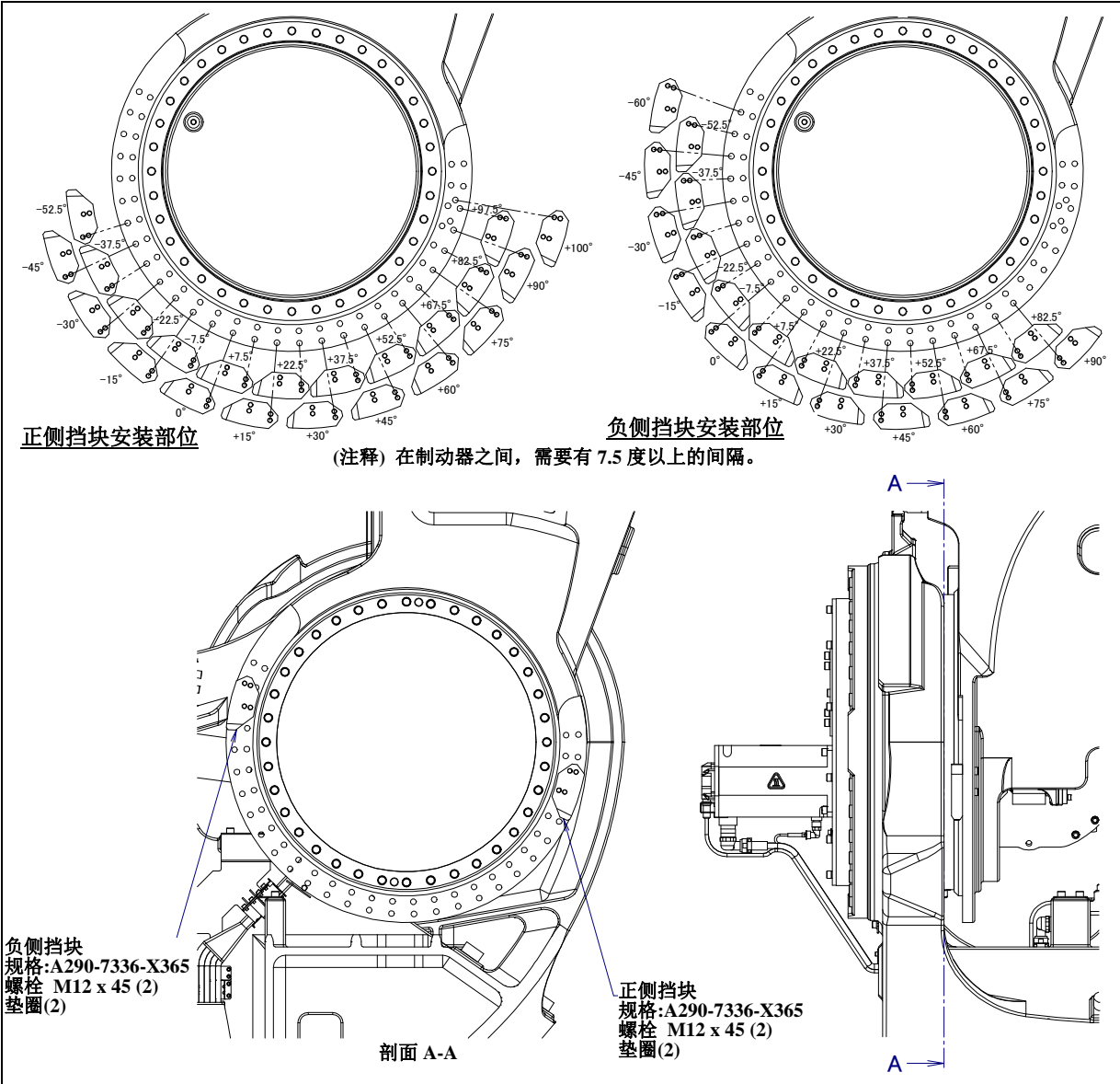
图 6.3 (d) J2 轴的挡块位置和动作范围(可选项)(M-2000iA/2300/1700L)
