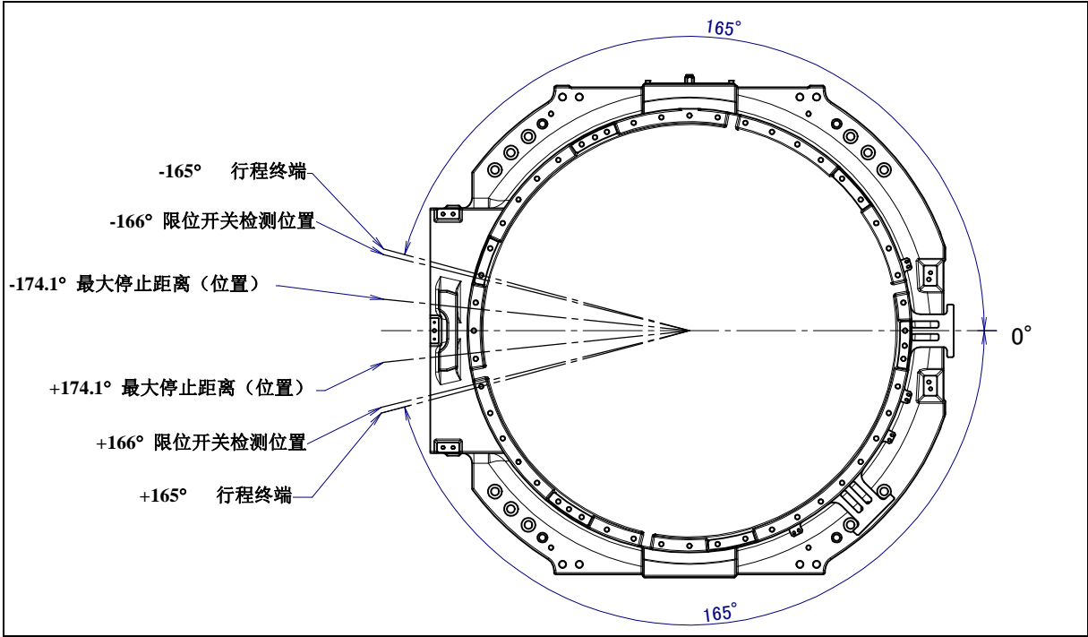
图 3.3 (d) J1 轴可动范围(M-2000iA/1700L)
