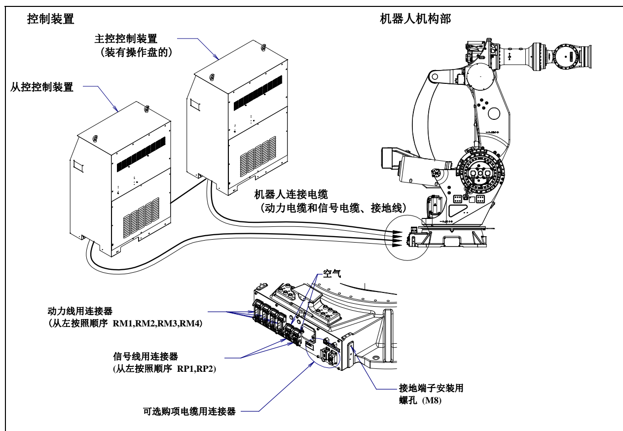
图 2.1 电缆连接图
