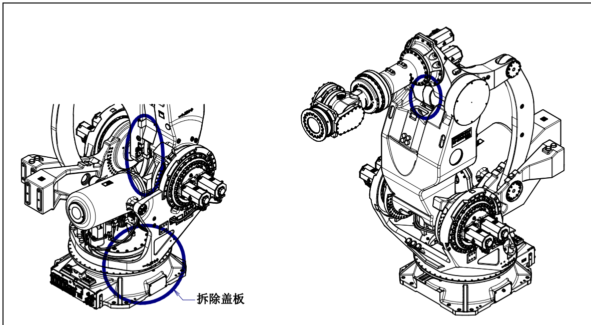
图 7.2.3 (a) 机构部内电缆的检修部位
