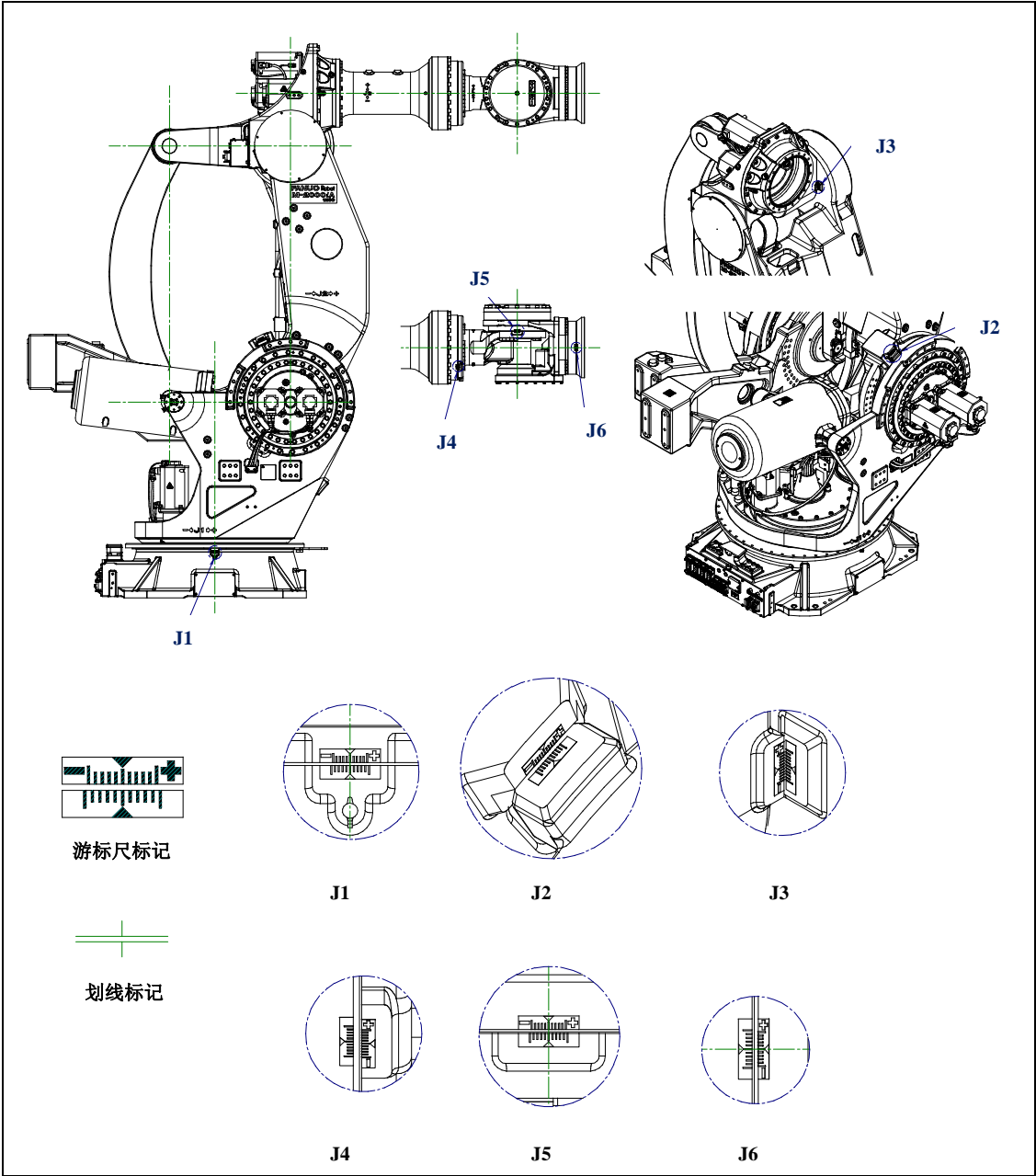
图 8.3 (a) 对合标记位置 (M-2000iA/1200/900L)
