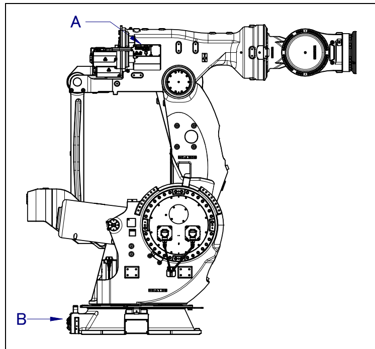
图 5.3 (b) 可选项电缆用接口的位置(可选项) (M-2000iA/2300/1700L)
