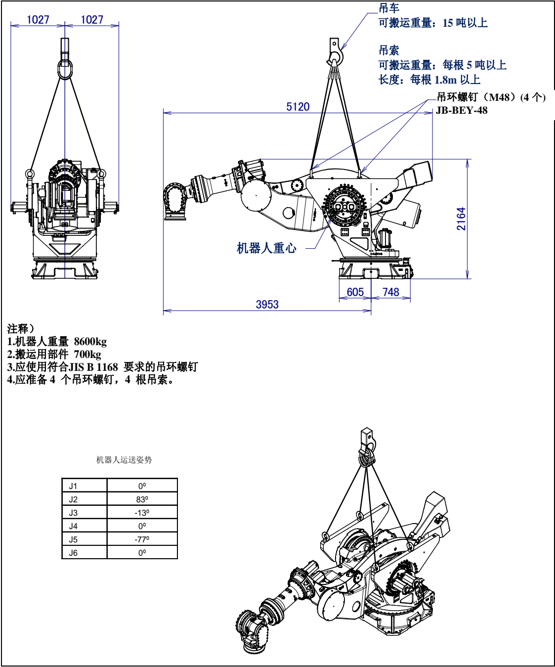
图 1.1 (d) 采用吊车搬运 (M-2000iA/1200 用集装箱的搬运时)
