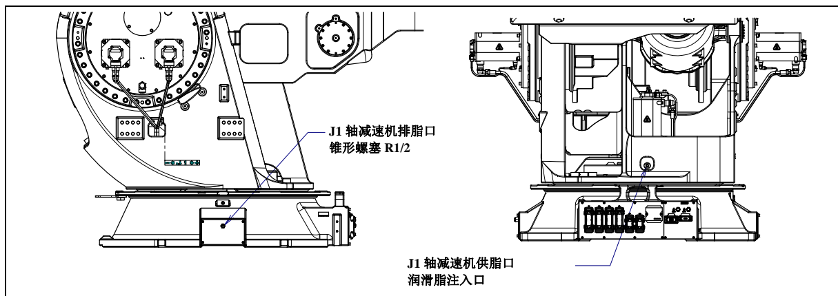
图 7.3.3 (d) J 轴减速机的润滑脂的更换 (M-2000iA/2300/1700L) (1/2)
