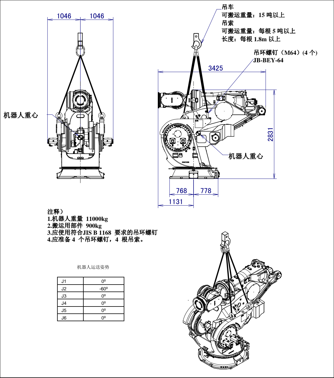
图 1.1 (g) 采用吊车搬运 (M-2000iA/2300 通常搬运时)
