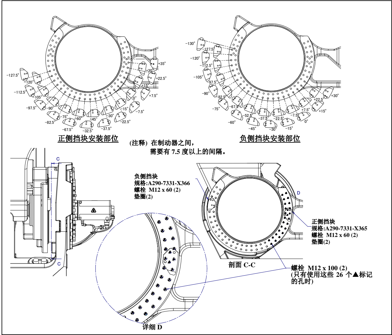
图 6.3 (e) J3 轴的挡块位置和动作范围(可选项项) (M-2000/A/1200/900L)
