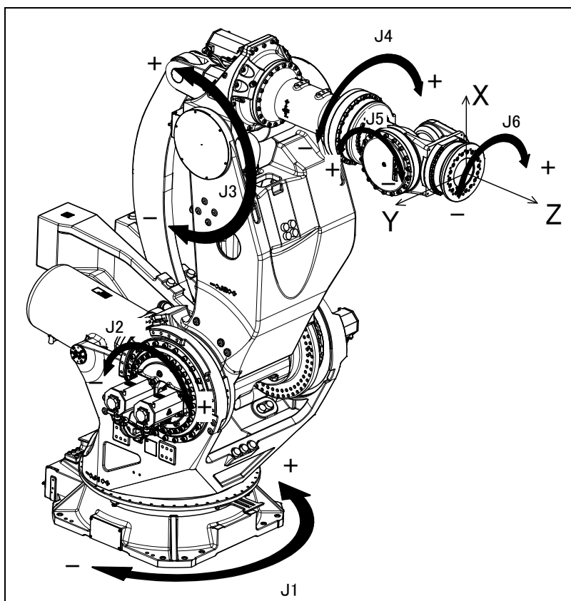
图 3.1 (b) 各轴坐标和机械接口坐标
