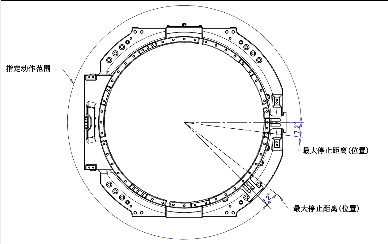
图 6.2.3 (d) J1 轴机械式可变制动器的最大停止距离(位置) (M-2000iA/2300)
