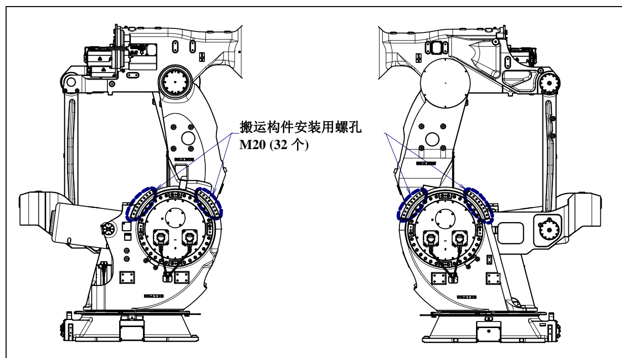
图 1.1 (b) 搬运用部件安装位置 (M-2000iA/2300/1700L)
