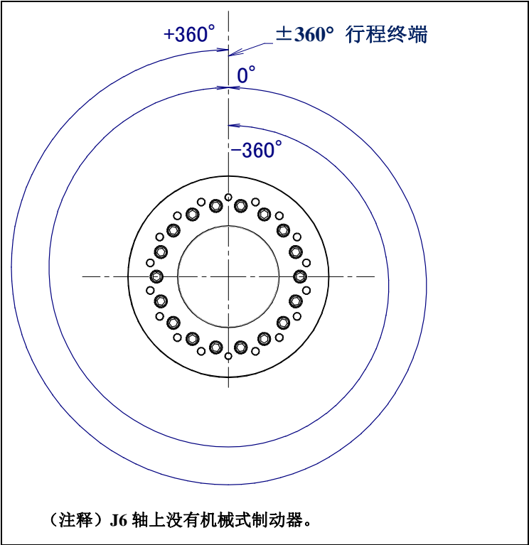
图 3.3 (i) J6 轴可动范围
