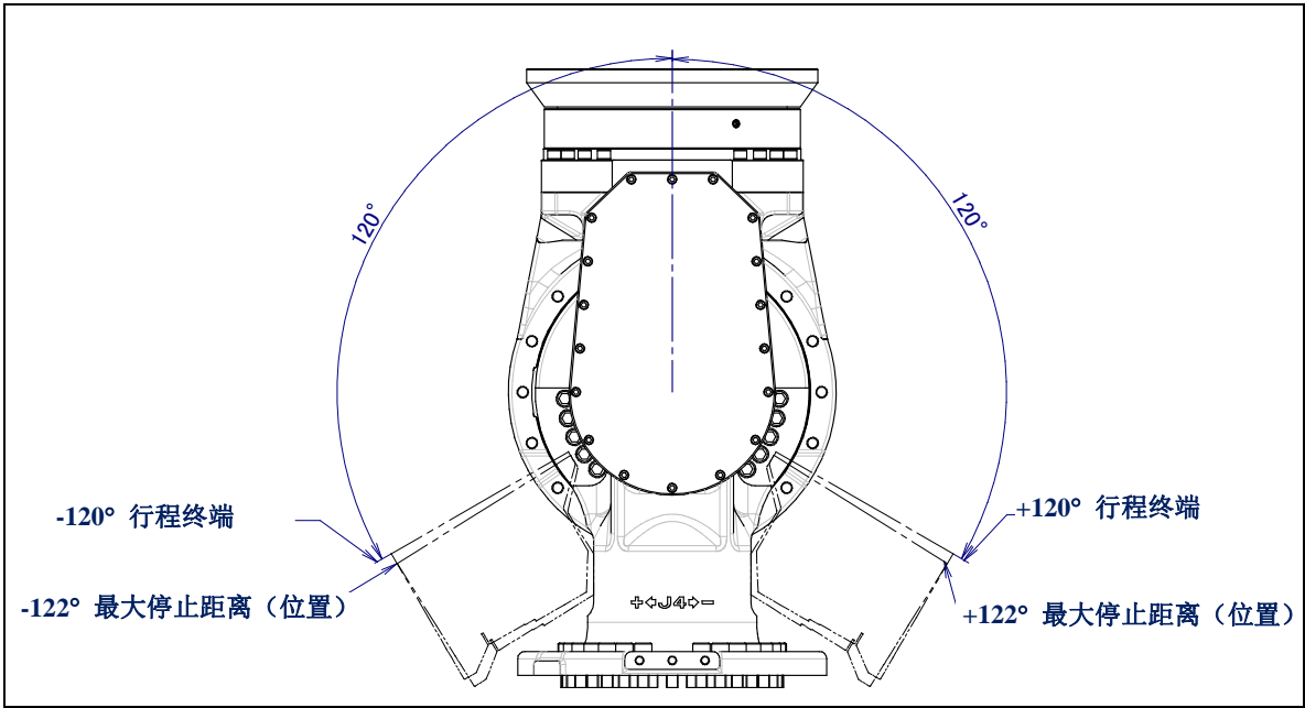
图 3.3 (h) J5 轴可动范围
