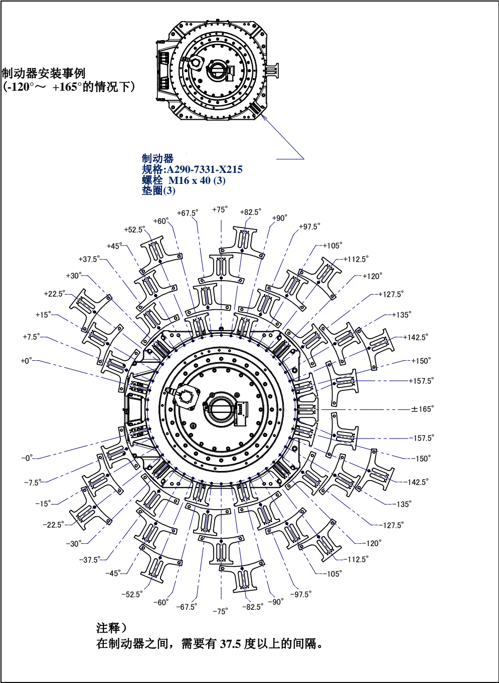
图 6.2.1 (a) J1 轴机械式制动器的安装 (可选项) (M-2000iA/1200/900L)
