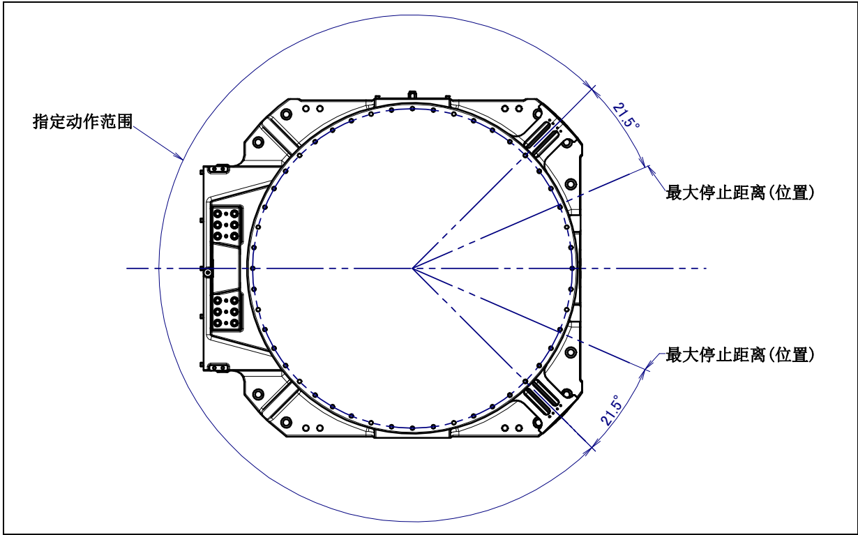
图 6.2.3 (a) J1 轴机械式可变制动器的最大停止距离(位置) (M-2000iA/1200/900L)
