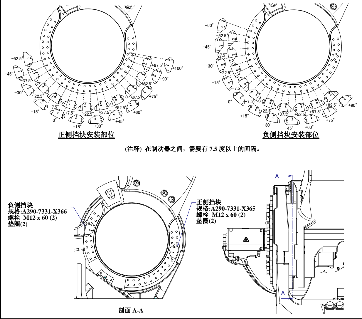
图 6.3 (c) J2 轴的挡块位置和动作范围(可选项) (M-2000iA/1200/900L)
