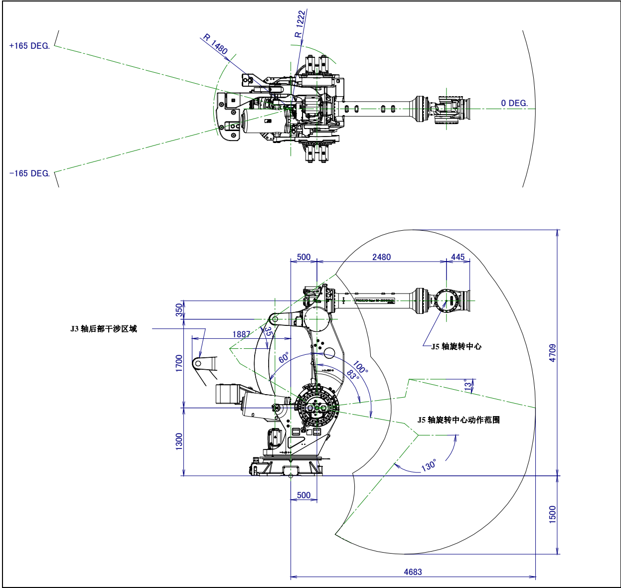
图 3.2 (b) 动作范围图 (M-2000iA/900L)
