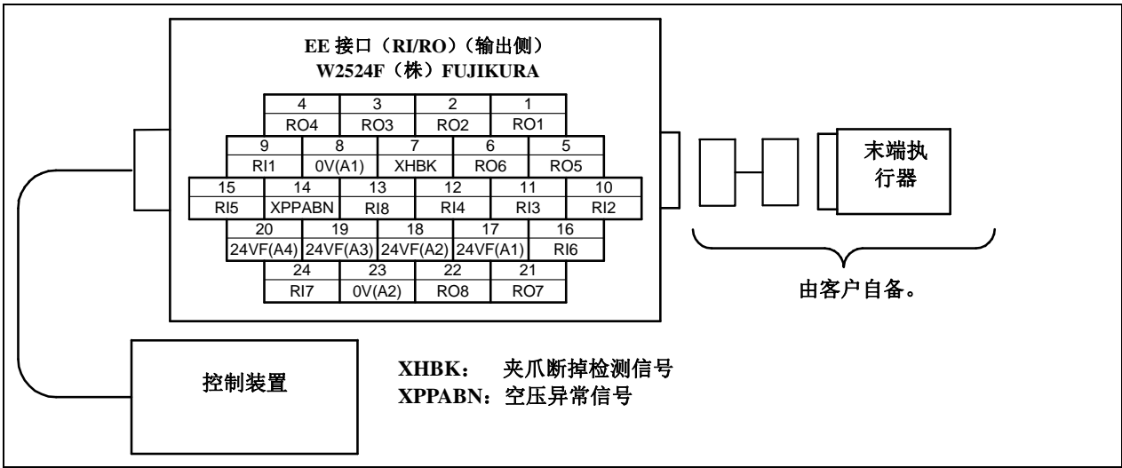
图 5.3 (j) EE 接口(RI/RO)的插针排列 (可选项)
