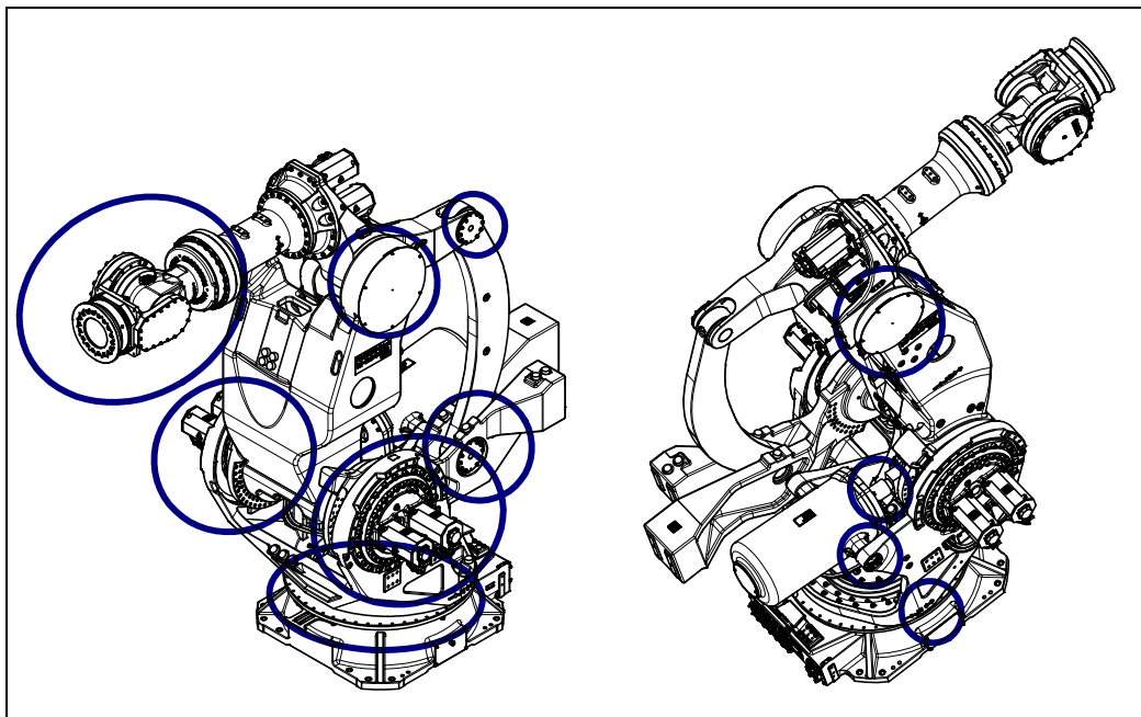
图 7.2.1 渗油的检查部位
