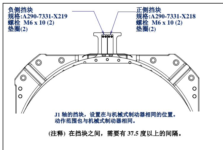
图 6.3 (a) J1 轴的挡块位置(可选项) (M-2000iA/1200/900L)
