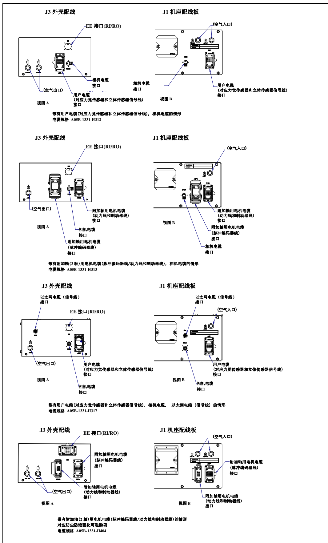
图 5.3 (e) 可选项电缆用接口 (3/5) (M-2000iA/1200/900L)
