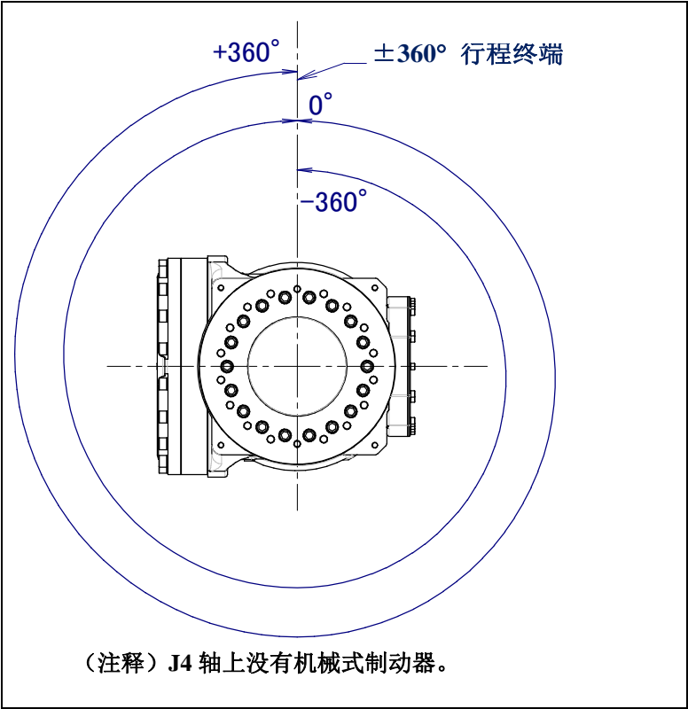
图 3.3 (g) J4 轴可动范围
