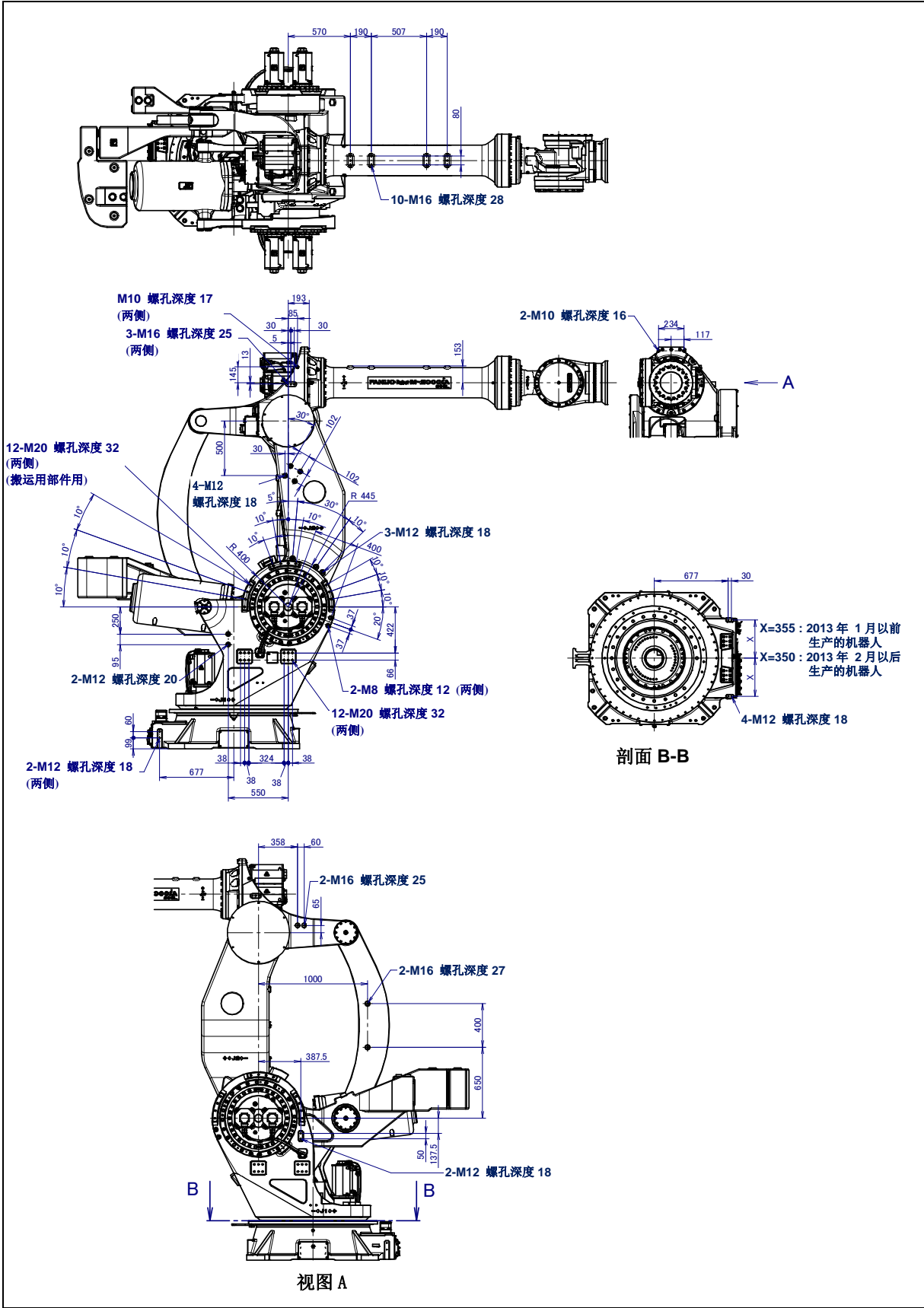
图 4.2 (b) 设备安装面尺寸 (M-2000iA/900L)
