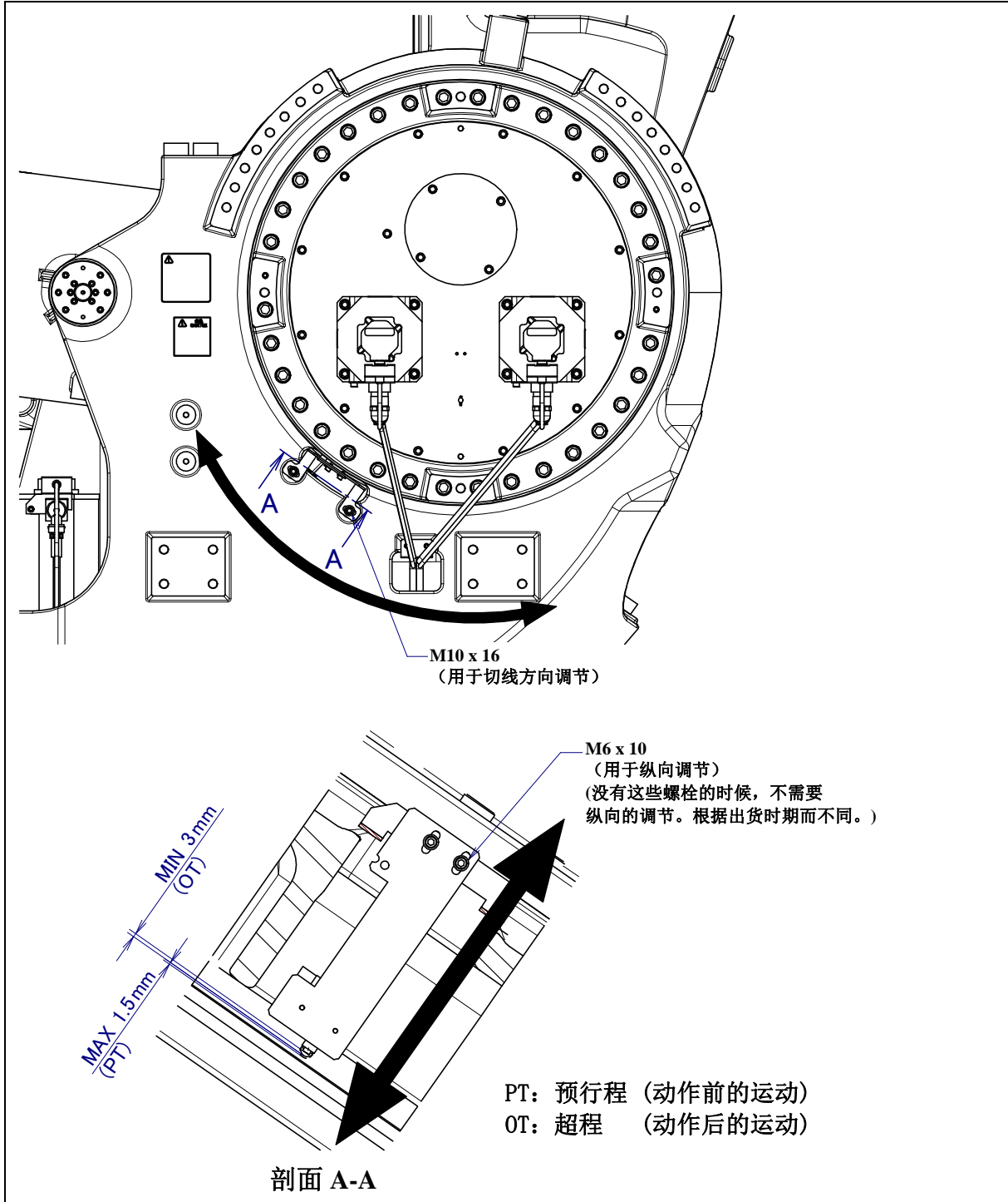
图 6.4 (d) J2 轴限位开关的调节(可选项)(M-2000iA/2300/1700L)
