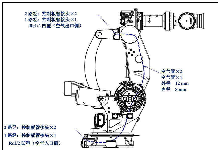
图 5.1 气压供应口（可选项项）
