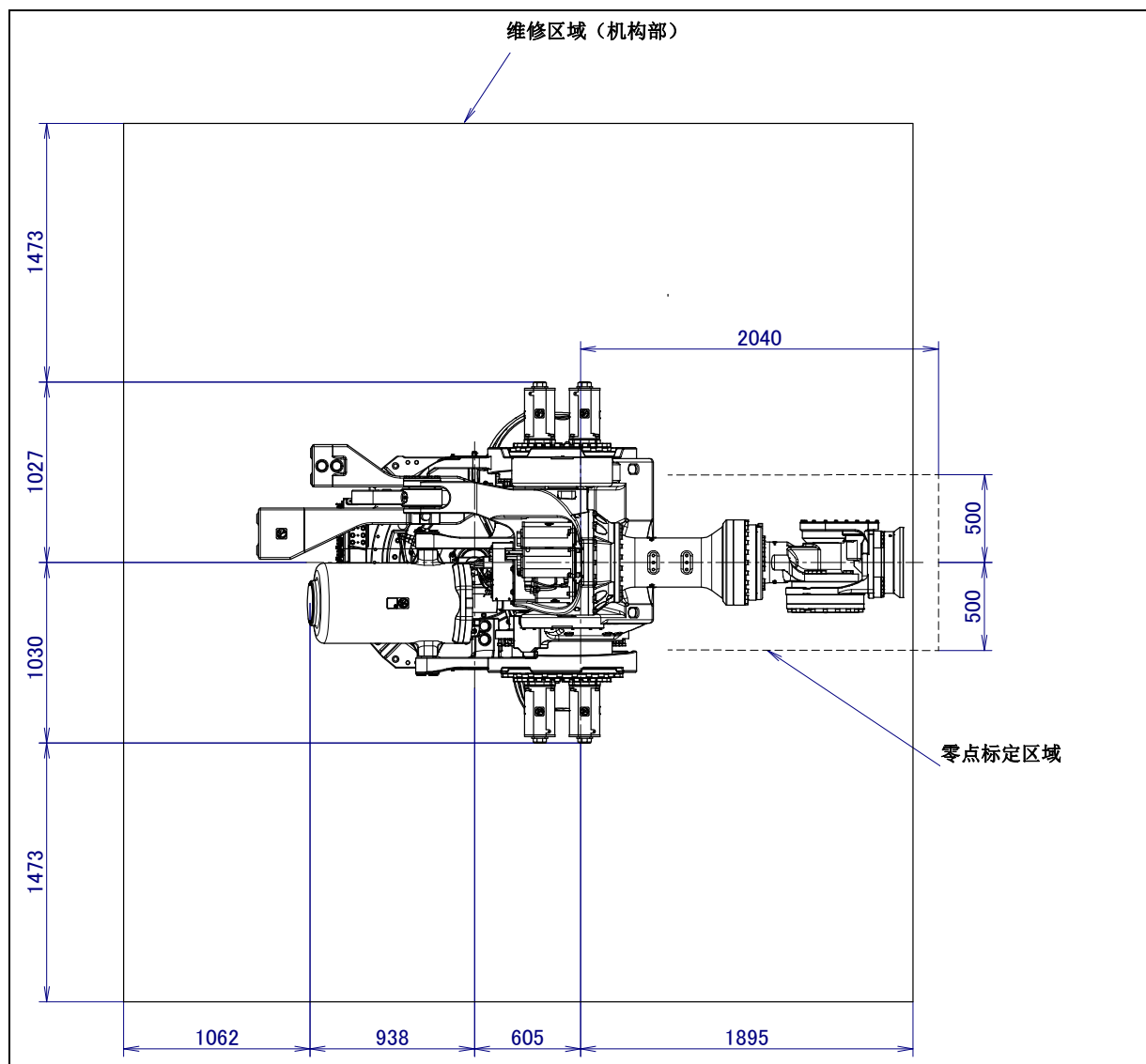
图 1.3 (a) 维修空间的布局图 (M-2000iA/1200/2300)
