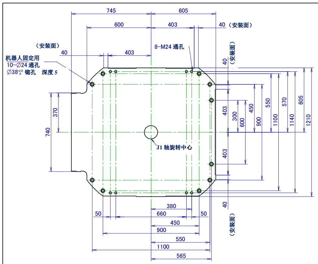
图 1.2 (a) 机器人机座尺寸 (M-2000iA/1200/900L)
