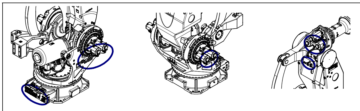
图 7.2.3 (d) 连接器的检修部位
