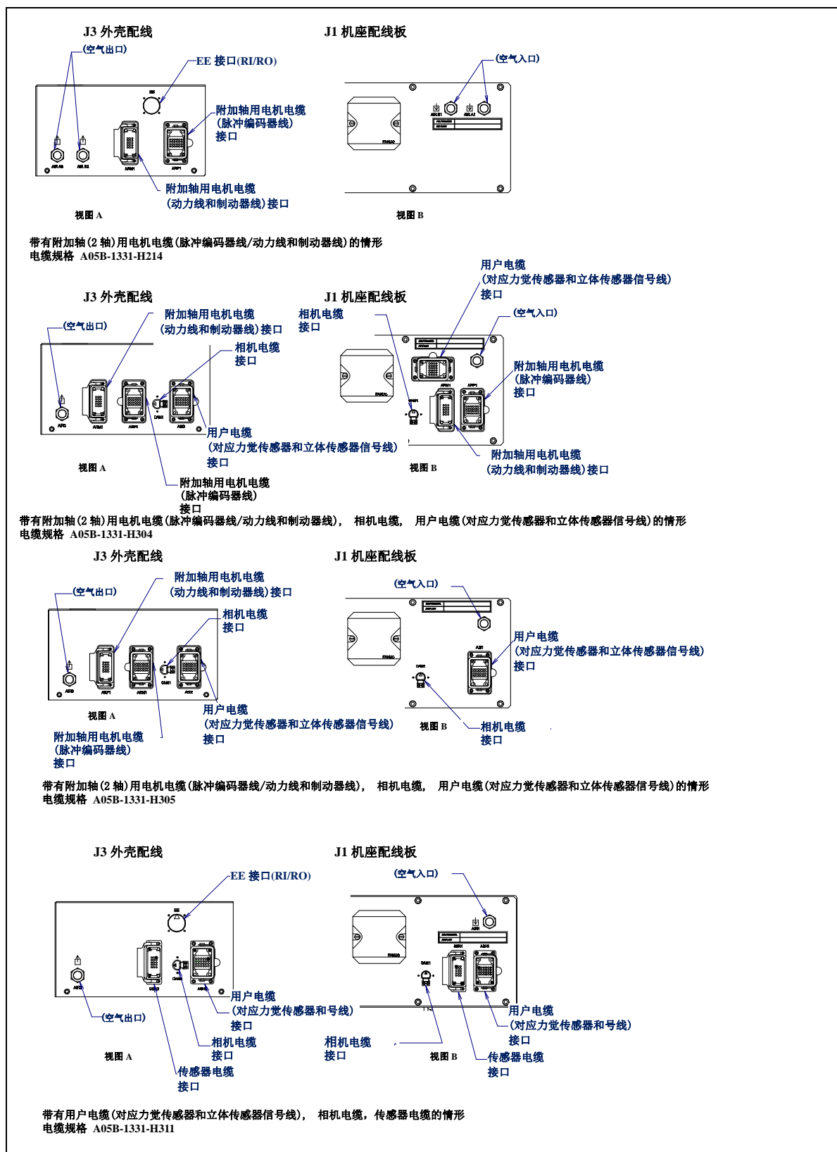
图 5.3 (d) 可选项项电缆用接口 (2/5) (M-2000iA/1200/900L)
