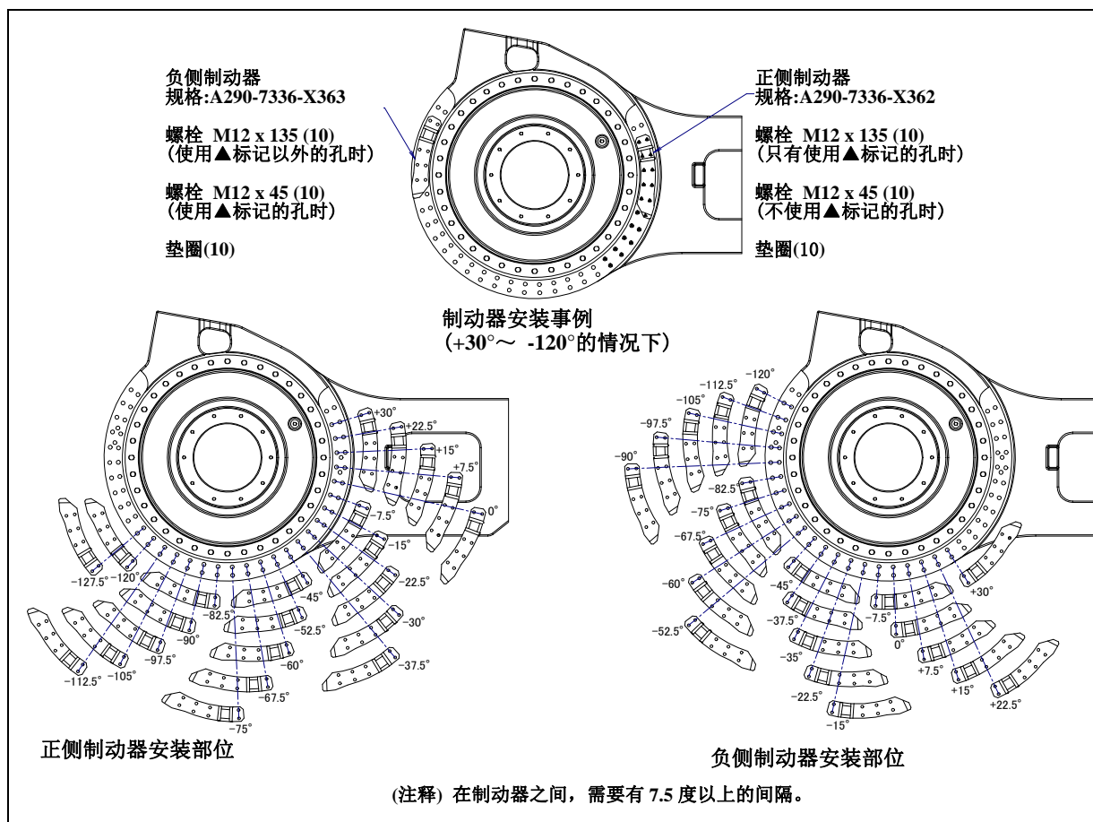
图 6.2.1 (f) J3 轴机械式制动器的安装(可选项项) (M-2000iA/2300/1700L)
