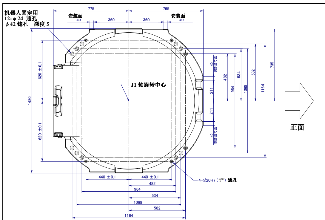
图 1.2 (b) 机器人机座尺寸 (M-2000iA/2300/1700L)
