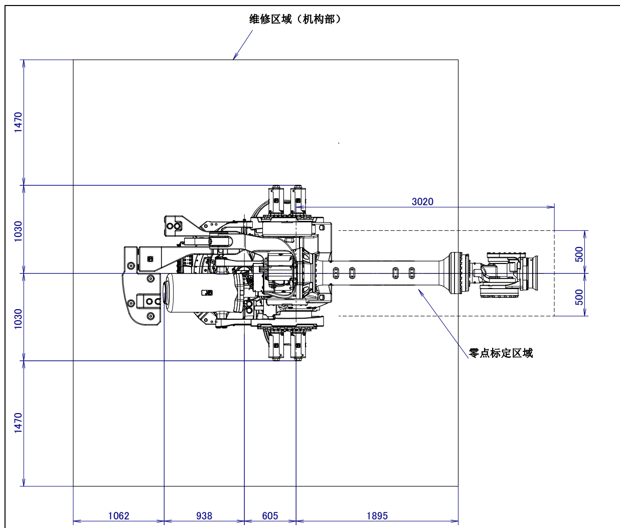
图 1.3 (b) 维修空间的布局图 (M-2000iA/900L/1700L)
