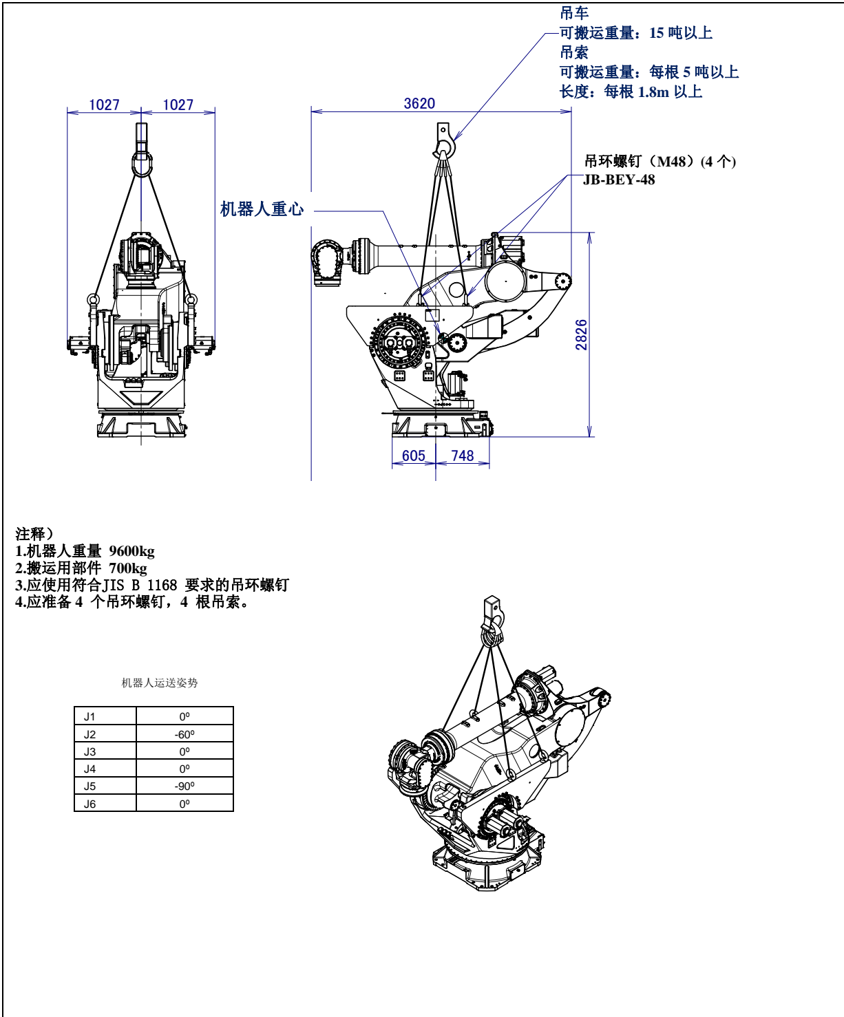
图 1.1 (e) 采用吊车搬运 (M-2000iA/900L 通常搬运时)
