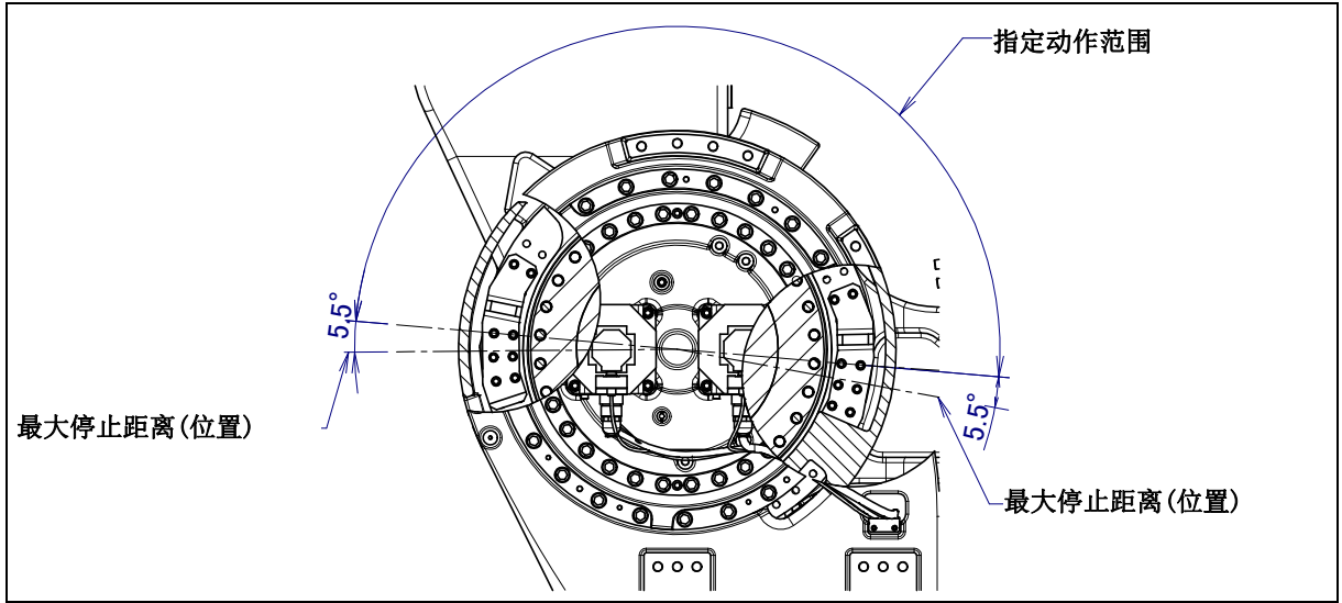
图 6.2.3 (c) J3 轴机械式可变制动器的最大停止距离(位置) (M-2000iA/1200/900L)
