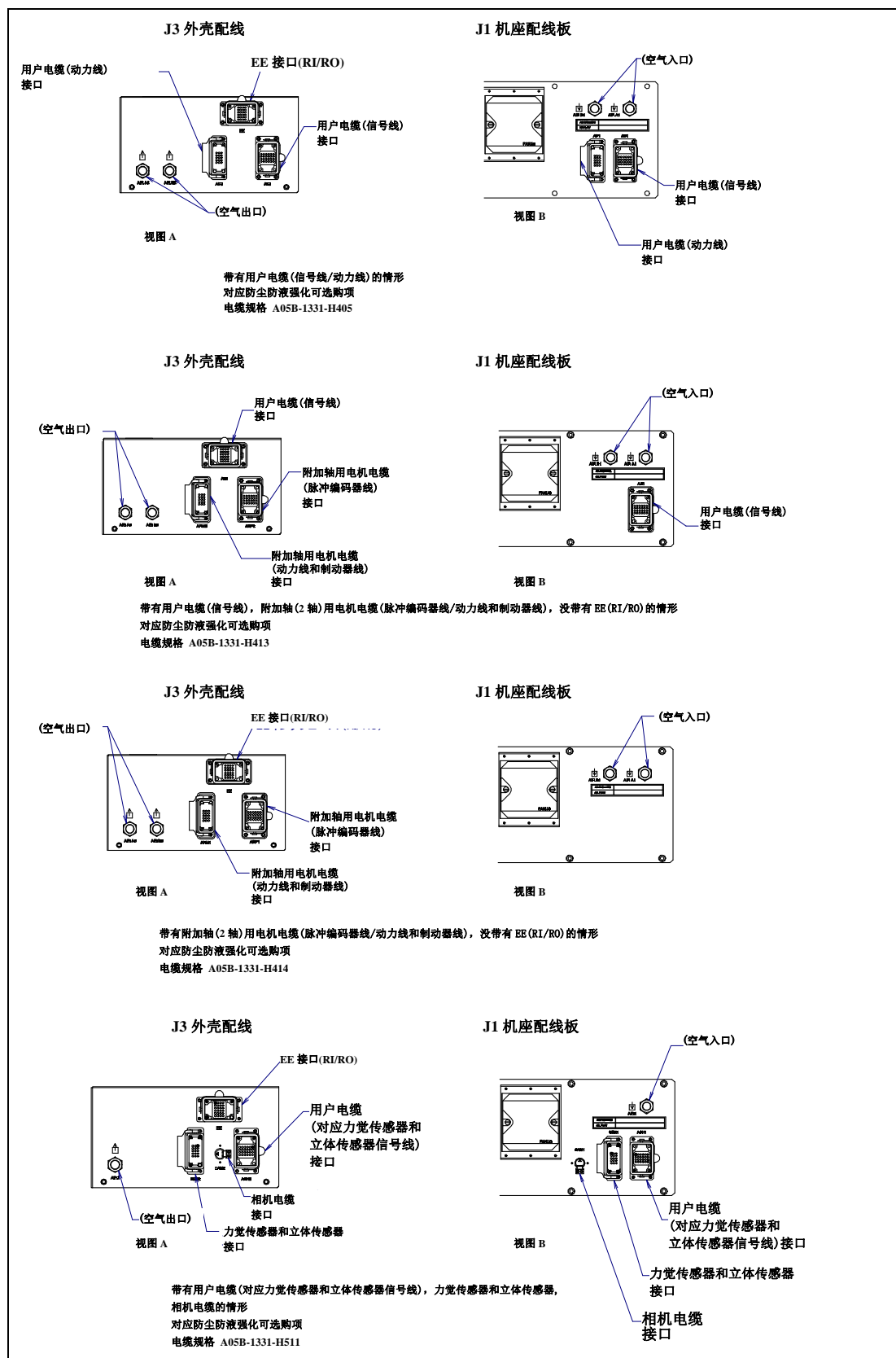
图 5.3 (f) 可选购项电缆用接口 (4/5) (M-2000iA/1200/900L)
