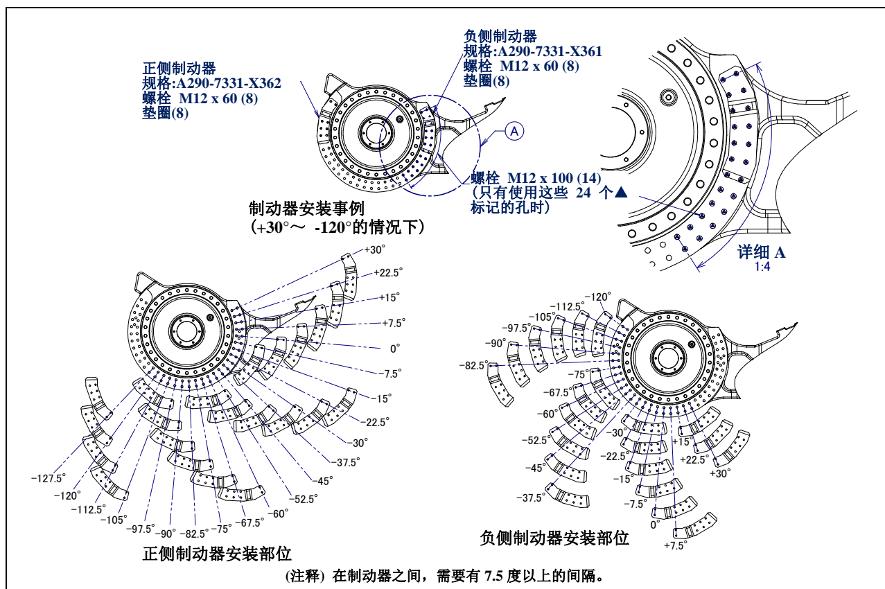
图 6.2.1 (e) J3 轴机械式制动器的安装(可选项项) (M-2000iA/1200/900L)
