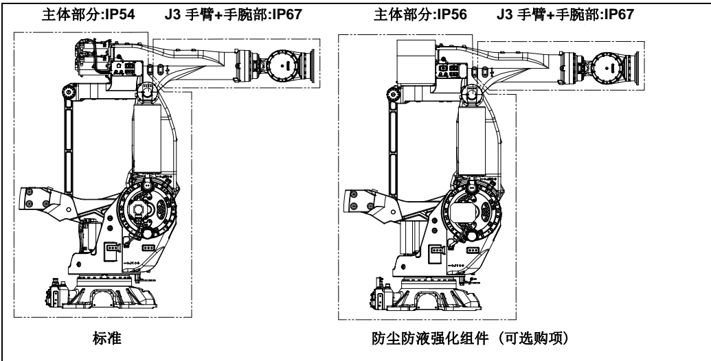
图3.1 (c) M-2000iA 的防尘防液性能
