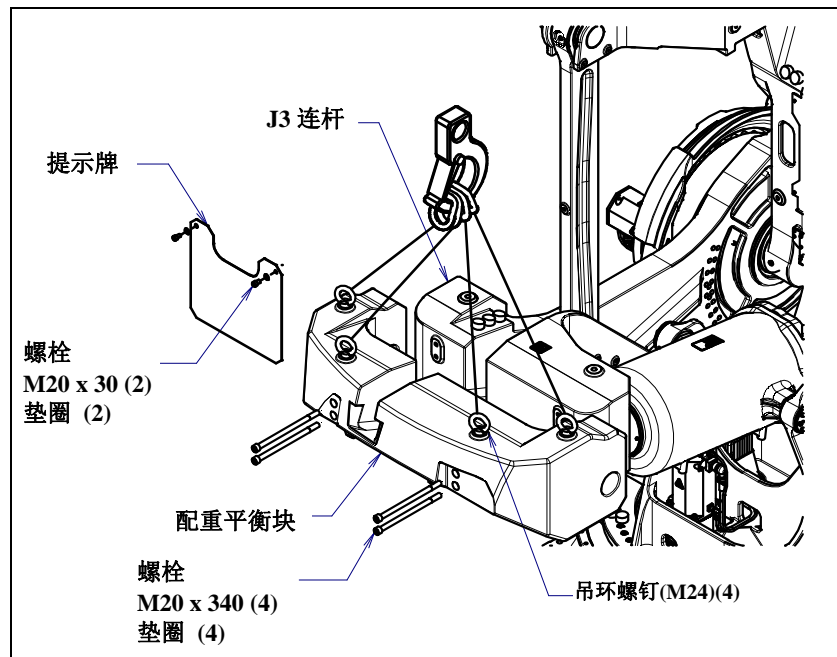
图 1.1.1 配重平衡块的安装和拆卸 (M-2000iA/1700L)
